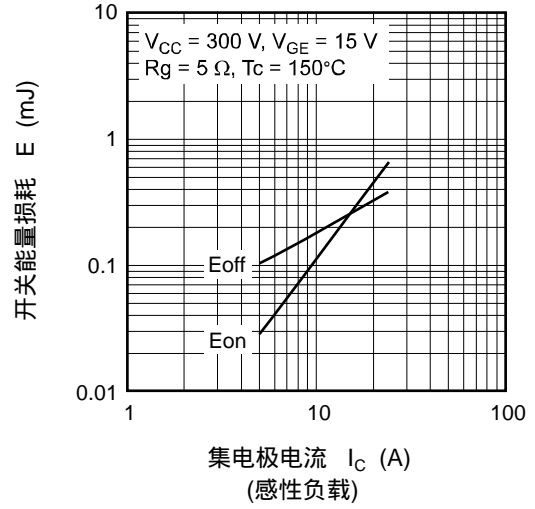
开关特性 (典型) (4)
