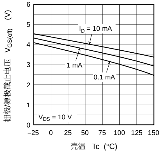
栅极/源极截止电压-壳温 (典型)
