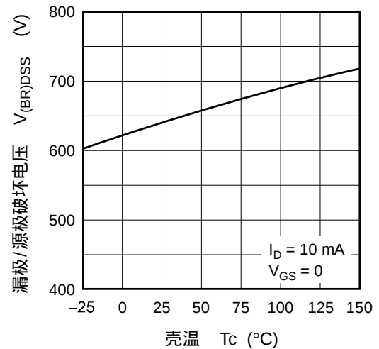
漏极/源极破坏电压-壳温 (典型)
