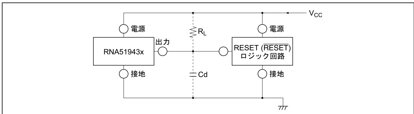
図 1 RNA51943 のリセット回路への応用
