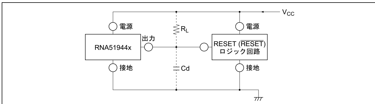
図 1 RNA51944 のリセット回路への応用
