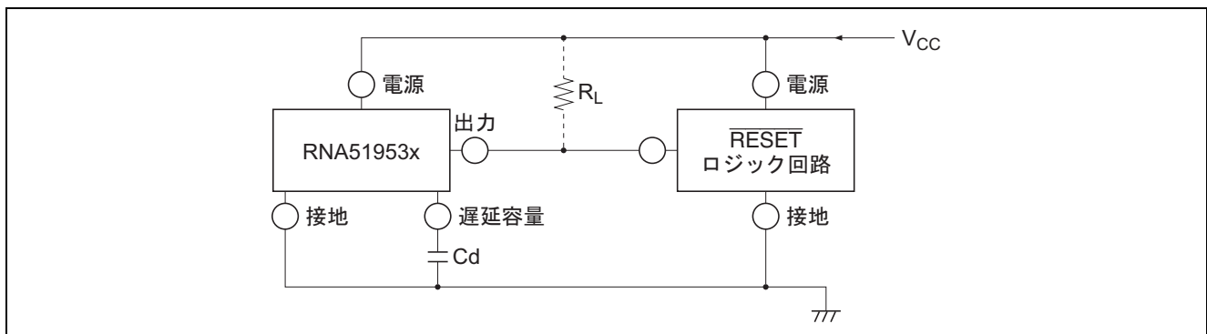
図 1 RNA51953 のリセット回路への応用
