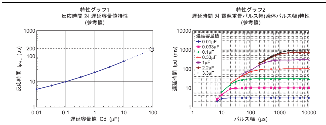
図5 特性グラフ
