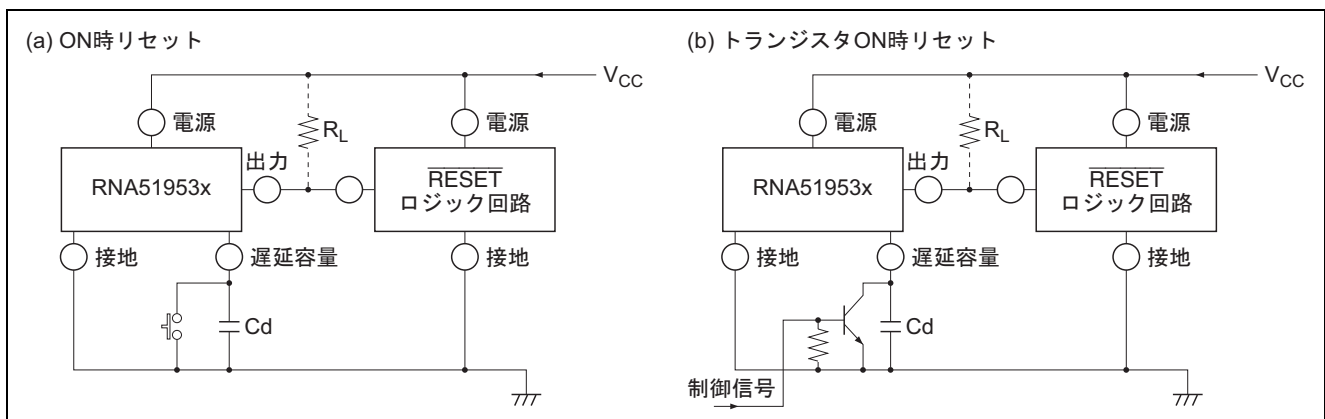
図 2 RNA51953 で電源電圧以外に他のリセット信号を用いる場合
