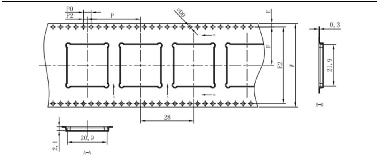
図 8 梱包詳細
