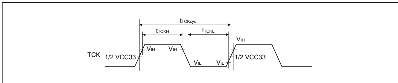
図 2.96 TCK 入力タイミング
