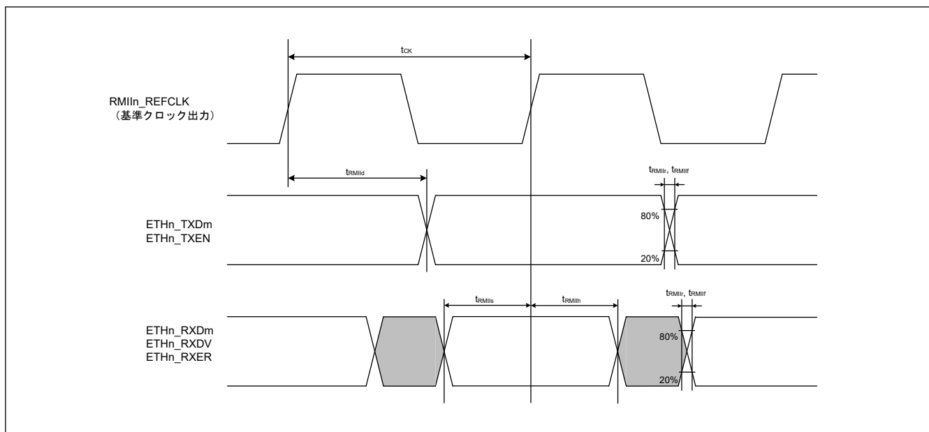
図 2.83 RMIi 送信、受信タイミング (基準クロック出力) (n = 0~2, m = 0~1)
