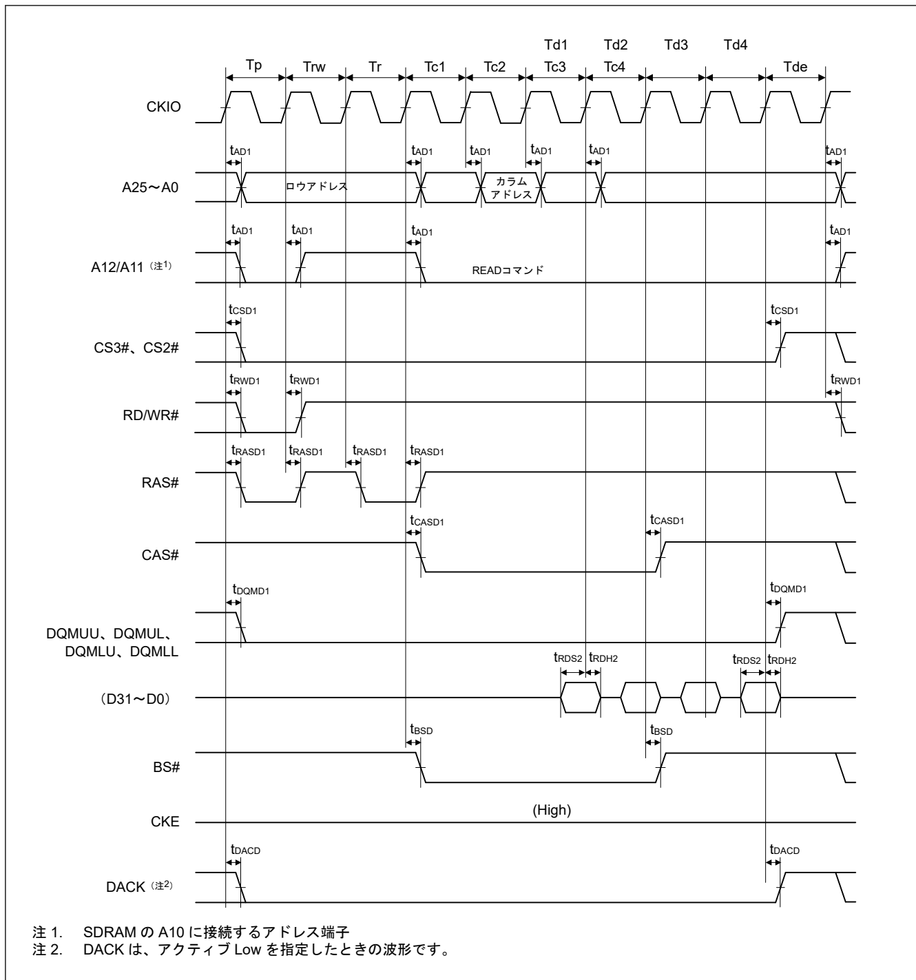
図 2.29 シンクロナス DRAM パーストリードバスサイクル (4 サイクルのリード) (バンクアクティブモード: PRE + ACT + READ コマンド、異なるロウアドレス、CAS レイテンシ 2、WTRCD = 0 サイクル)
