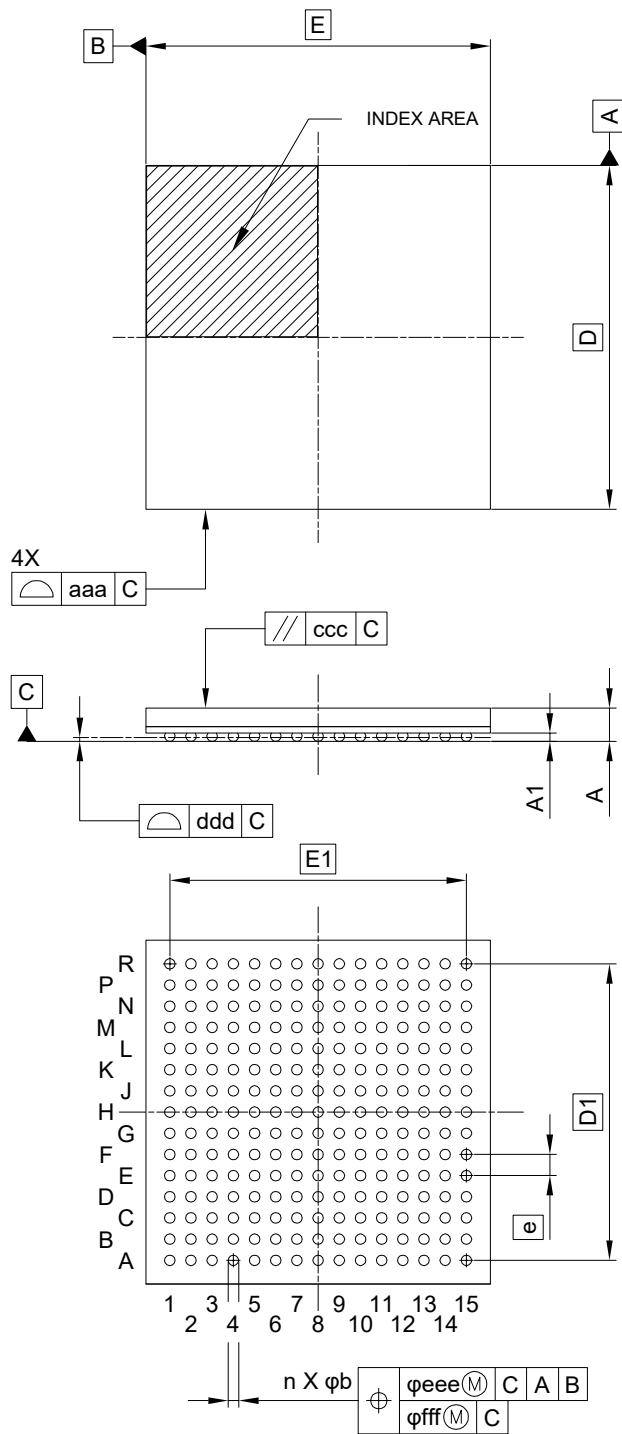
図 A1.2 225 ピン FBGA
