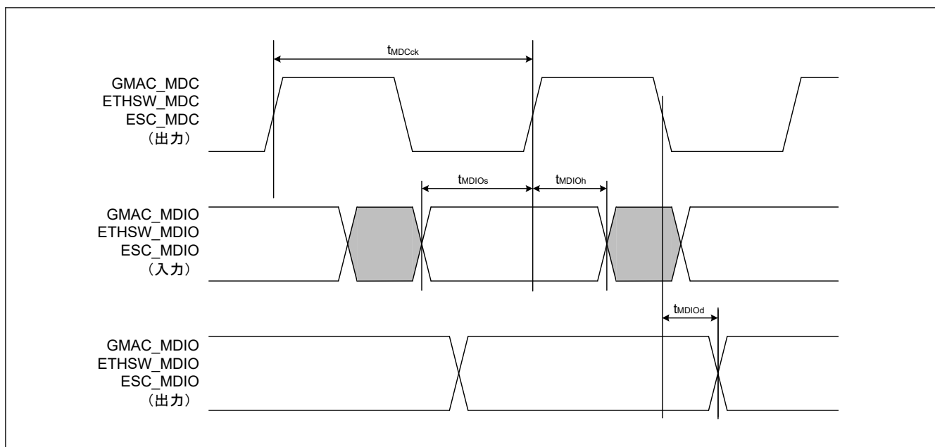
図 2.88 シリアルマネジメントインタフェースタイミング
