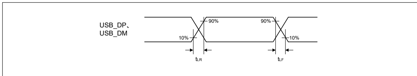
図 2.89 USB_DP、USB_DM の出カタイミング (ロースピード時/ホストのみ)
