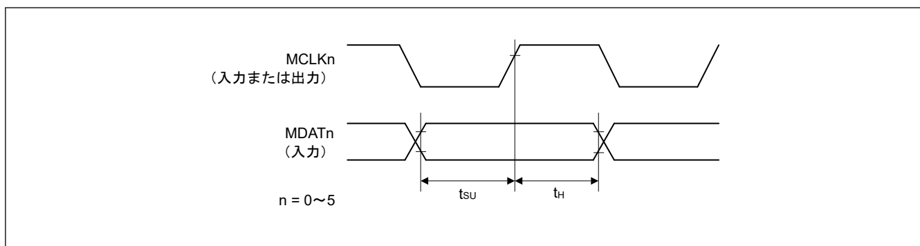
図 2.79 受信タイミング (MCLKn 立ち上がり同期)
