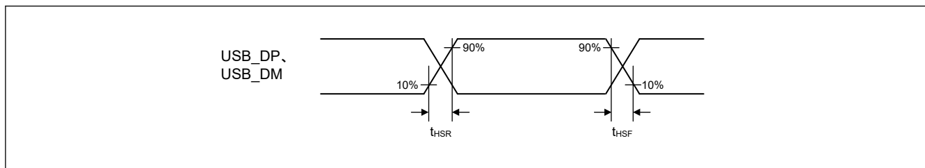
図 2.93 USB_DP、USB_DM の出カタイミング (ハイスピード時)
