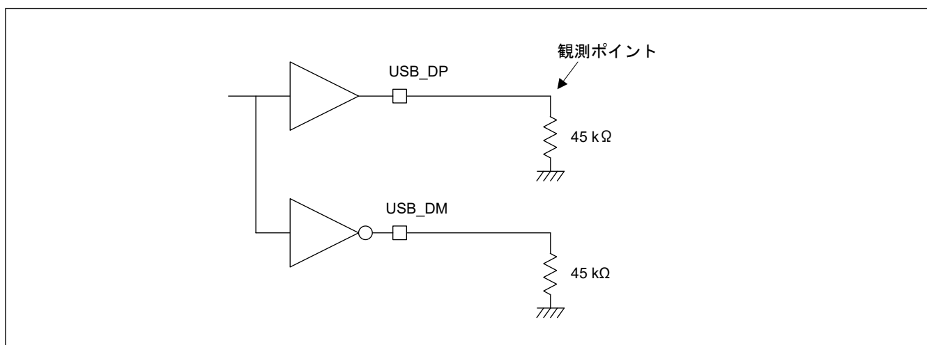
図 2.94 測定回路 (ハイスピード時)
