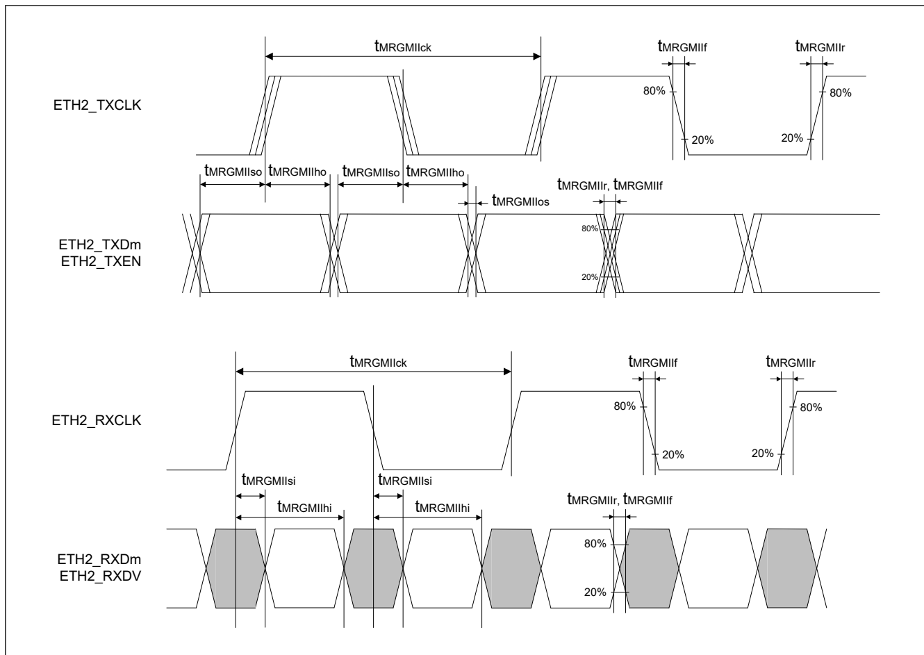
図 2.86 RGMII 送受信タイミング (MAC-to-MAC 接続モード) (m = 0~3)
