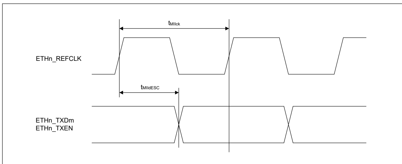
図 2.85 ESC MII 送信タイミング (自動 TX シフト無効) (n = 0~2, m = 0~3)
