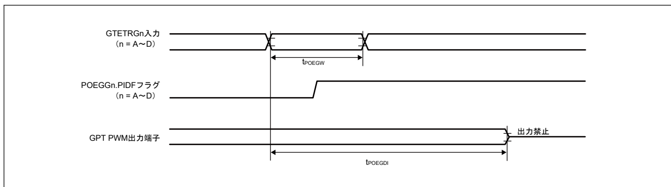
図 2.50 GTETR Gn 端子の入カレベル検出に対応した検出フラグによる POEG の出力禁止時間
