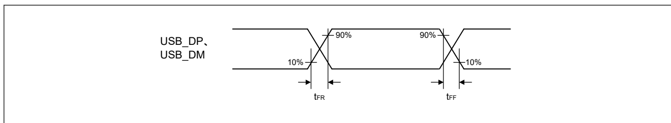
図 2.91 USB_DP、USB_DM の出カタイミング (フルスピード時)
