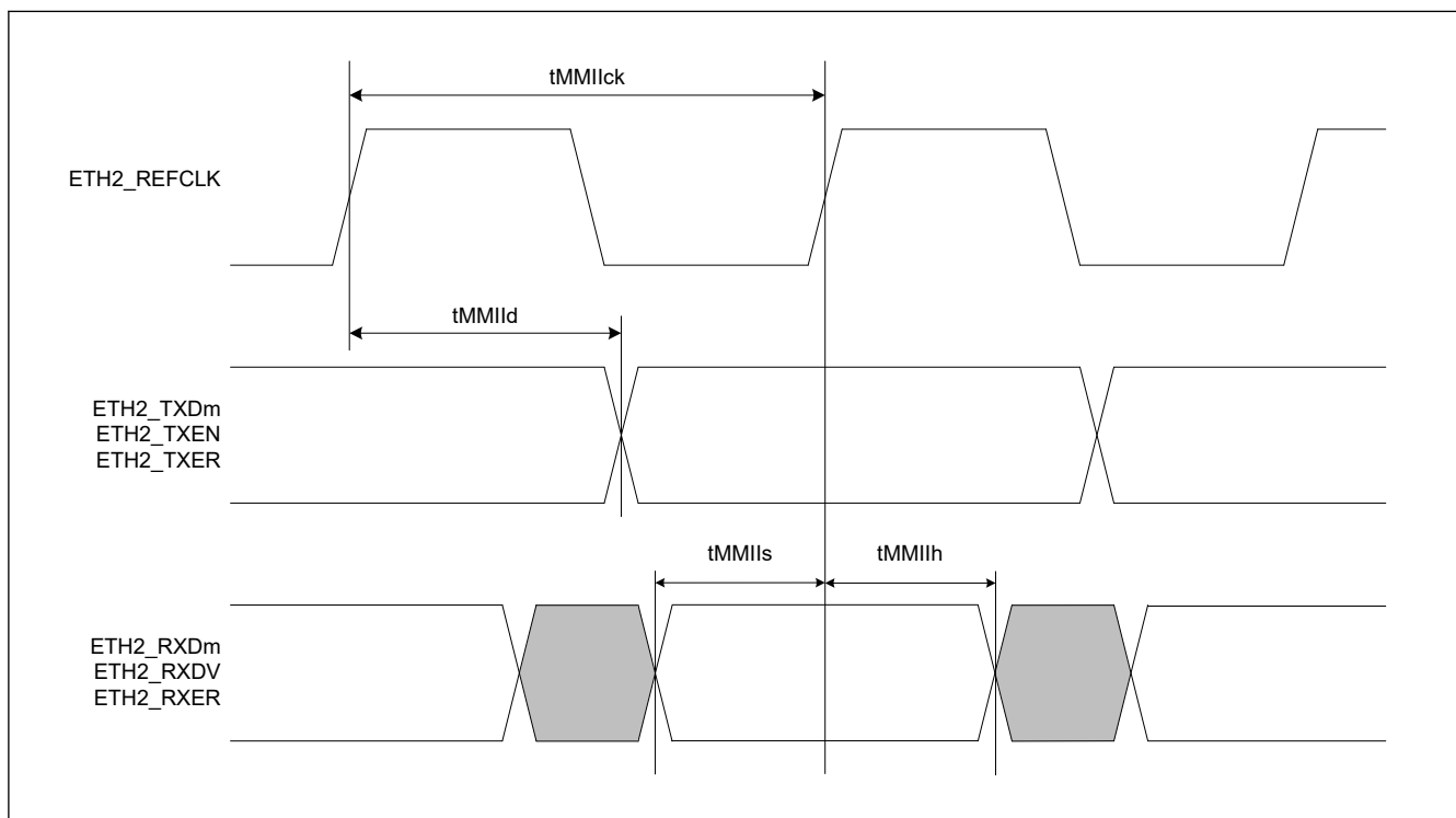
図 2.87 MII 送受信タイミング (MAC-to-MAC 接続モード) (m = 0~3)
