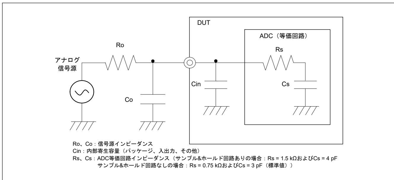
図 2.95 A/D コンバータの等価回路と周辺回路構成図
