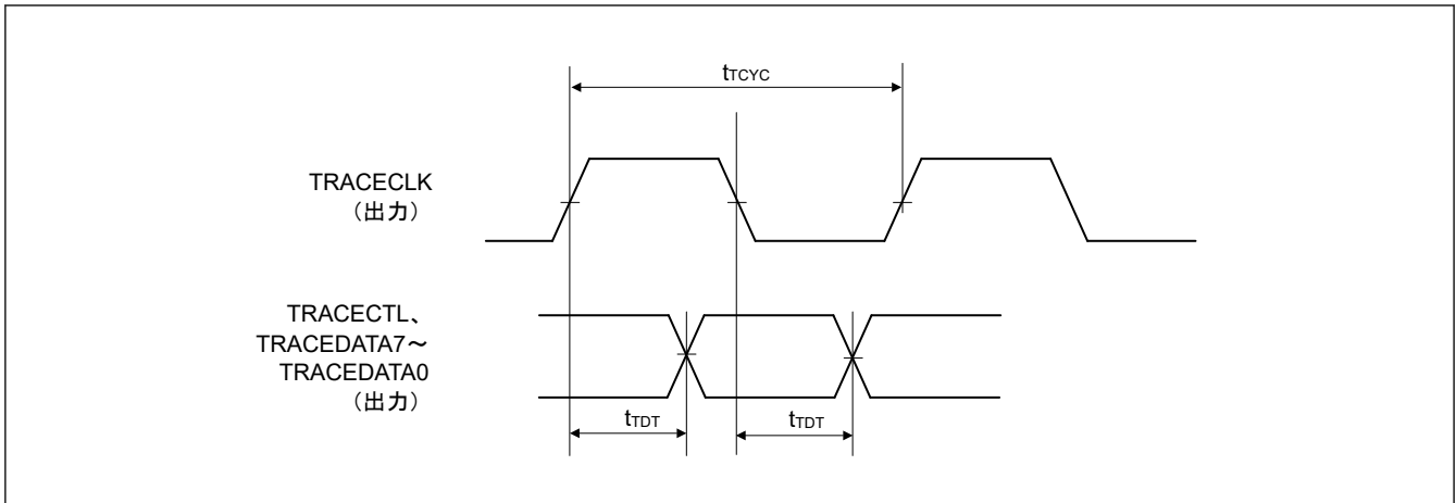
図 2.99 トレースインタフェースタイミング
