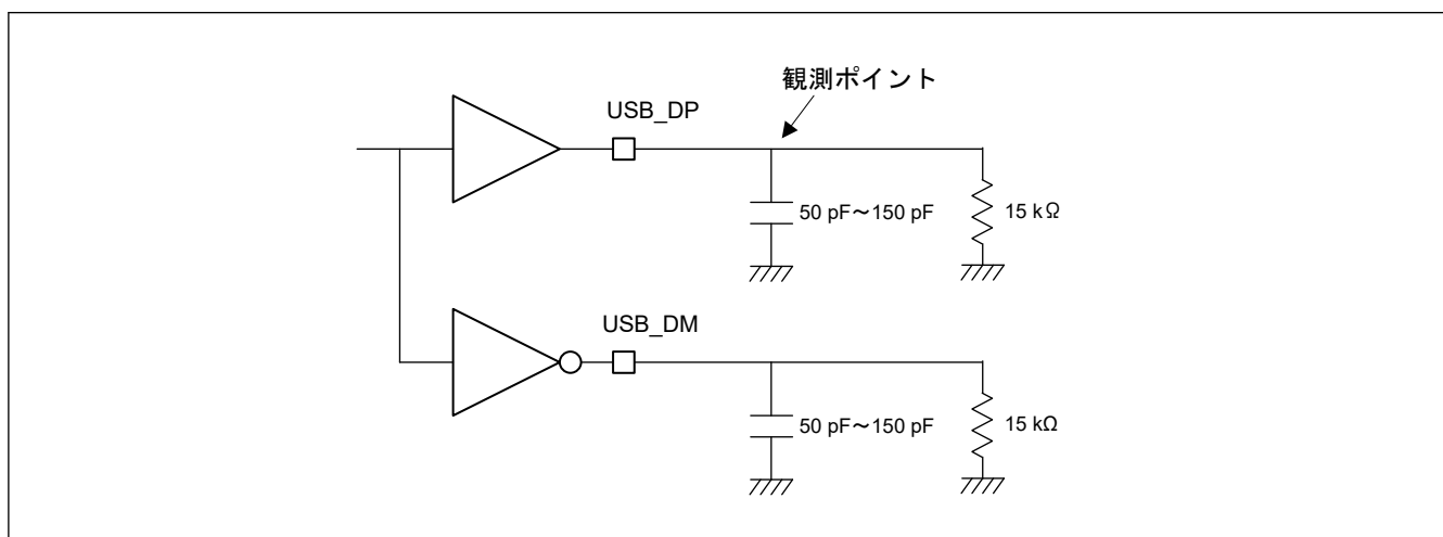
図 2.90 測定回路 (ロースピード時/ホストのみ)
