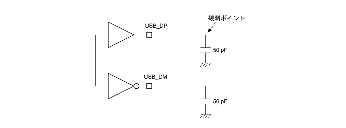
図 2.92 測定回路 (フルスピード時)
