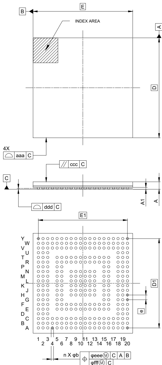
図 A1.1 320 ピン FBGA
