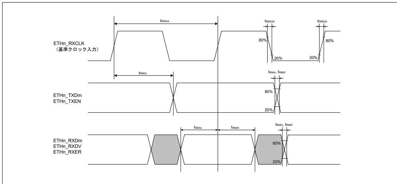
図 2.82 RMIi 送信、受信タイミング (基準クロック入力) (n = 0~2, m = 0~1)
