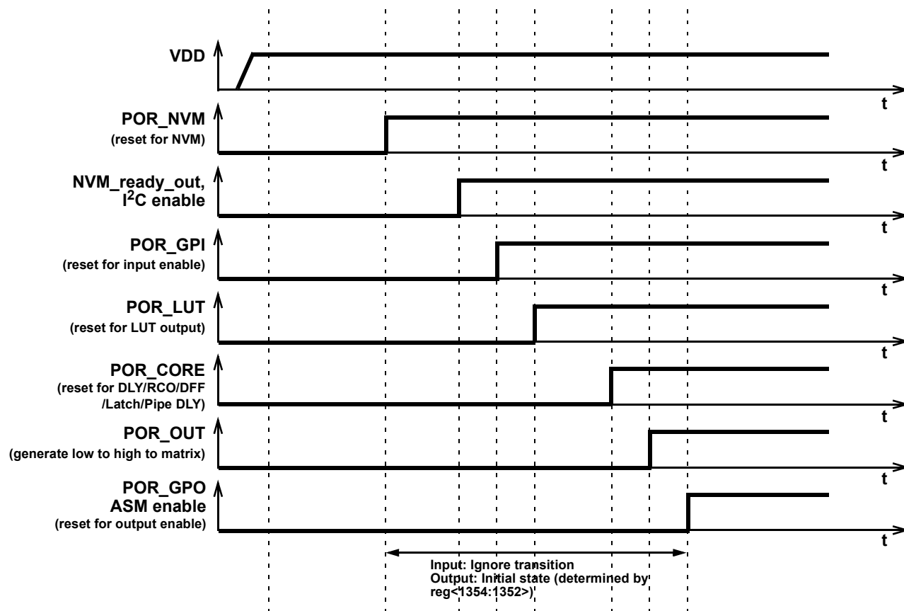
Figure 61. POR sequence
