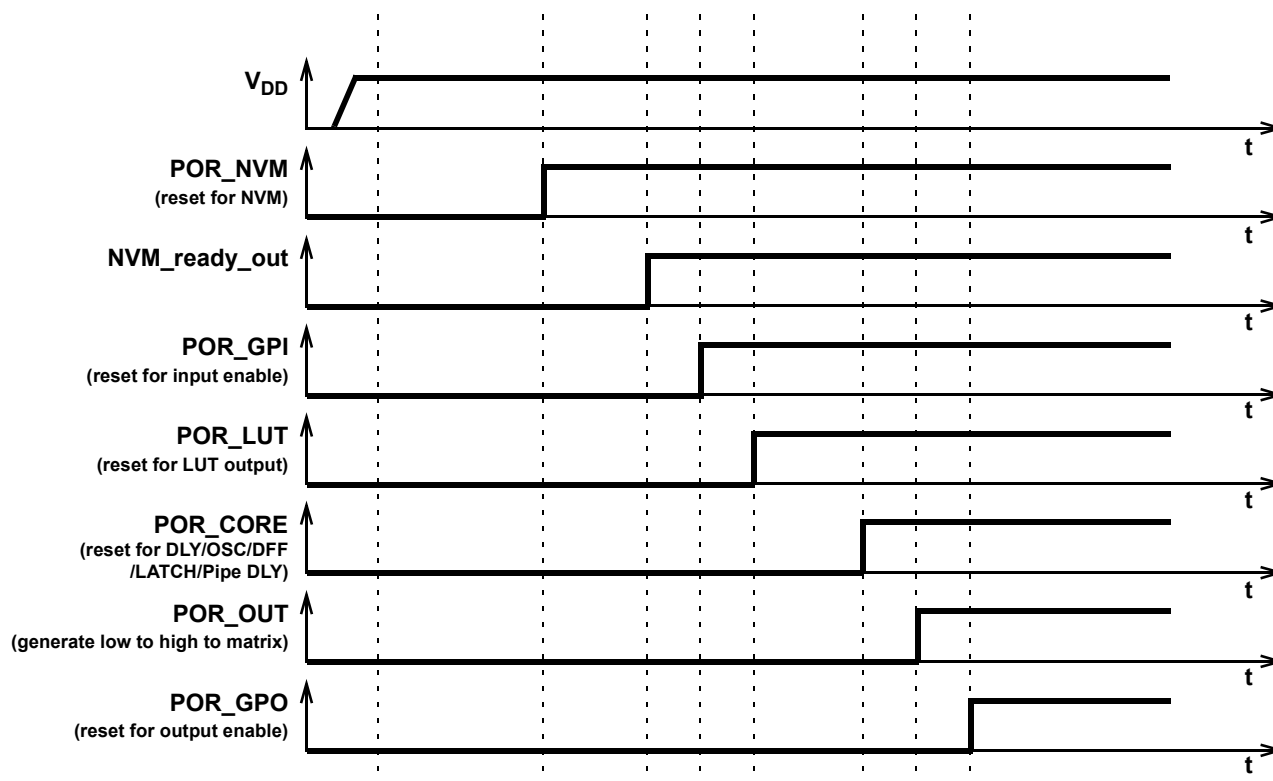
Figure 84. POR Sequence
