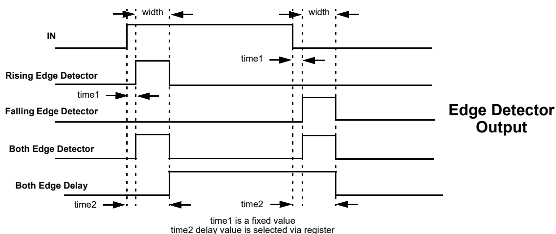
Figure 56. Edge Detector Output
