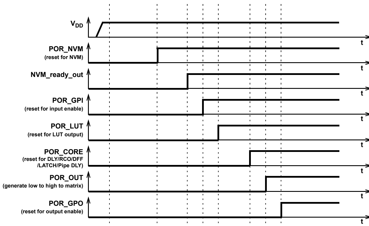
Figure 93. POR Sequence
