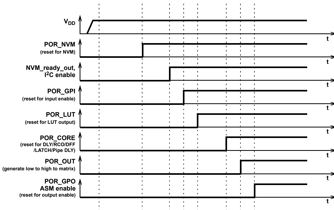
Figure 92. POR Sequence
