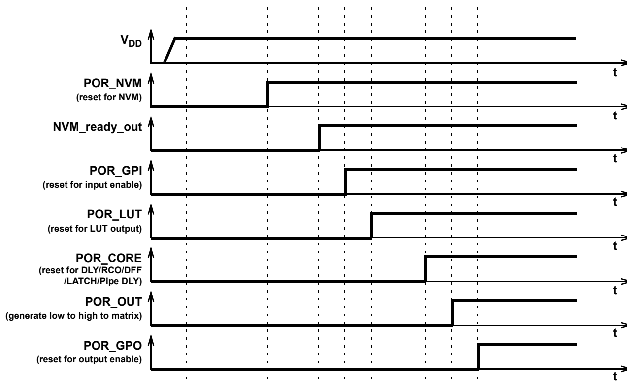
Figure 94. POR Sequence
