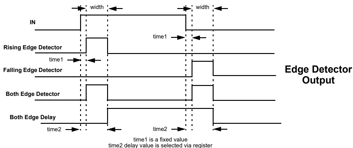
Figure 65. Edge Detector Output
