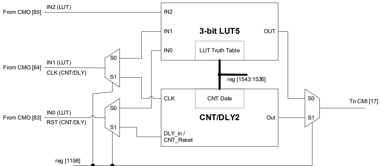
Figure 27. 3-bit LUT5 or CNT/DLY2
