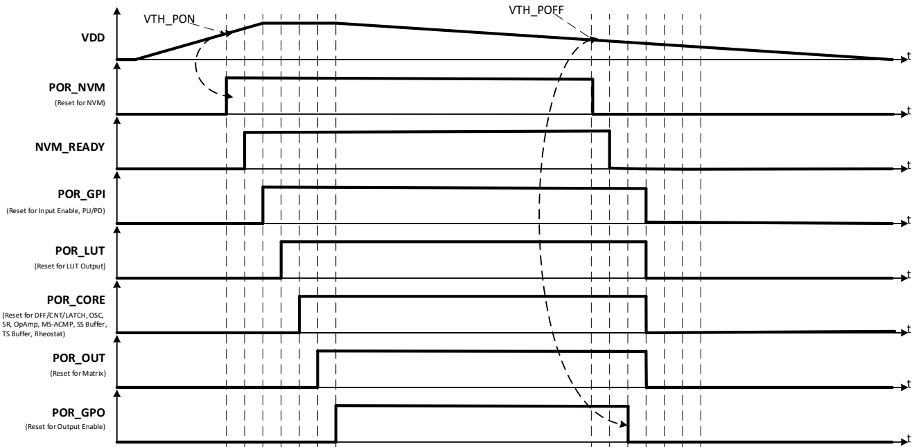
Figure 87. POR Sequence
