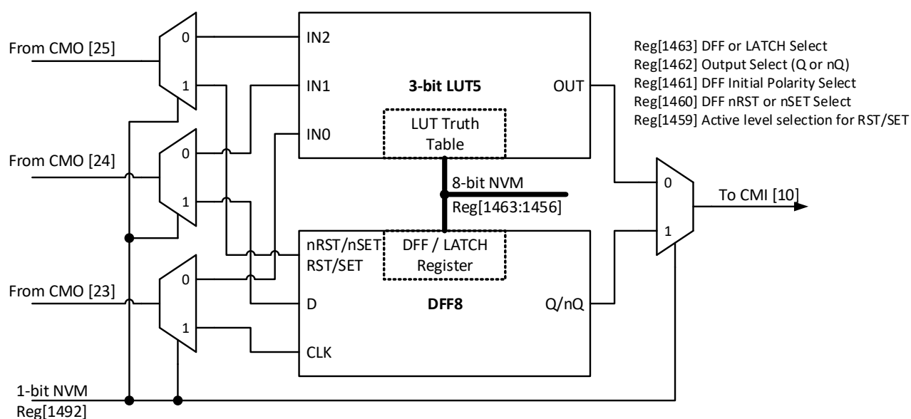
Figure 30. 3-bit LUT5 or DFF8
