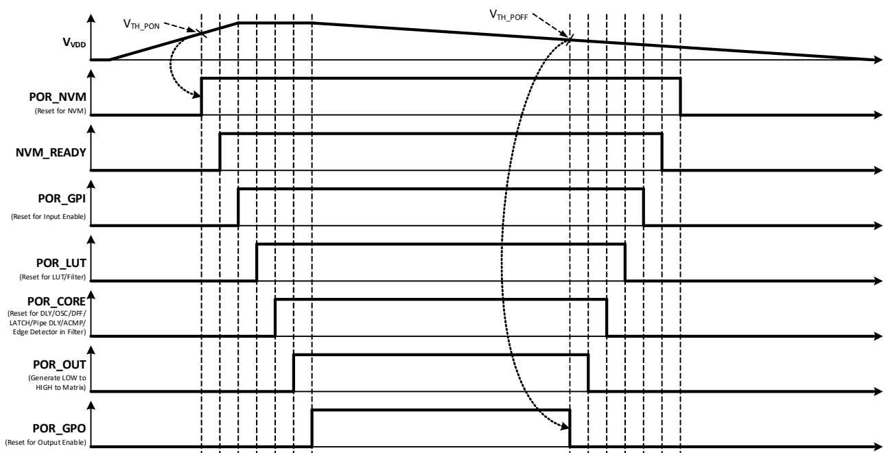
Figure 100. POR Sequence
