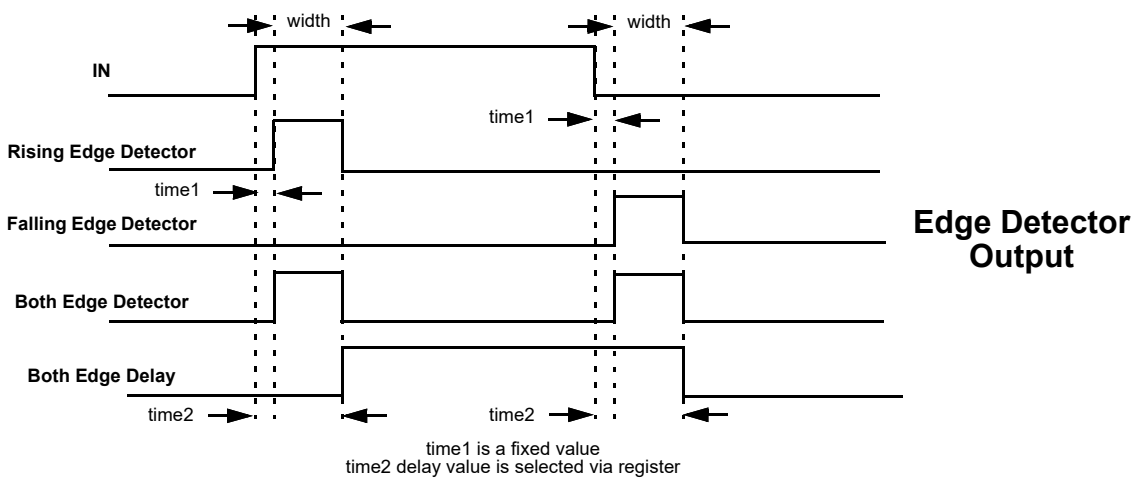
Figure 120. Edge Detector Output
