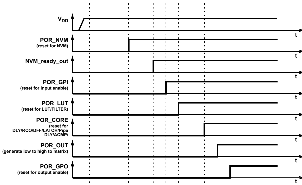
Figure 146. POR Sequence
