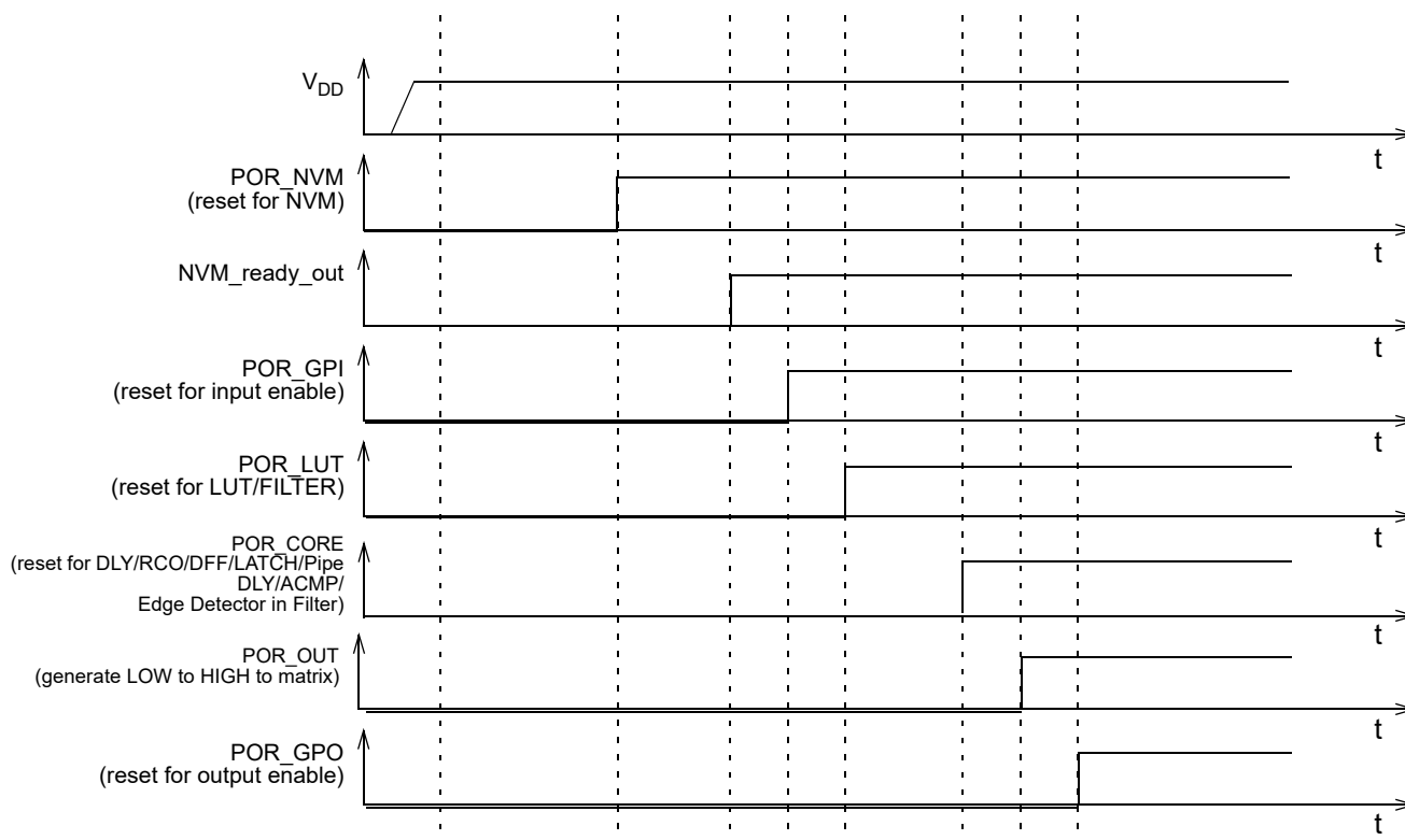
Figure 151. POR Sequence
