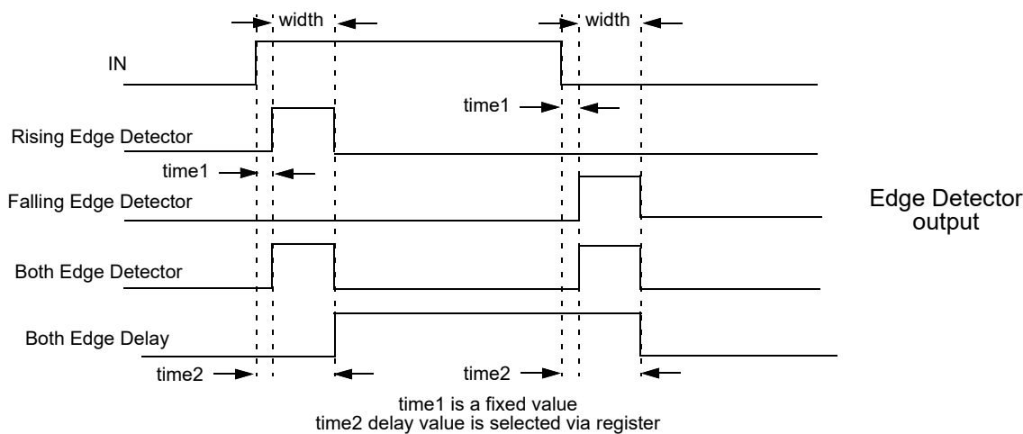
Figure 125. Edge Detector Output
