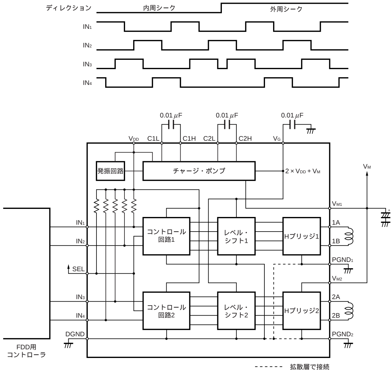
ステッピング・モータ励磁タイミング・チャート
