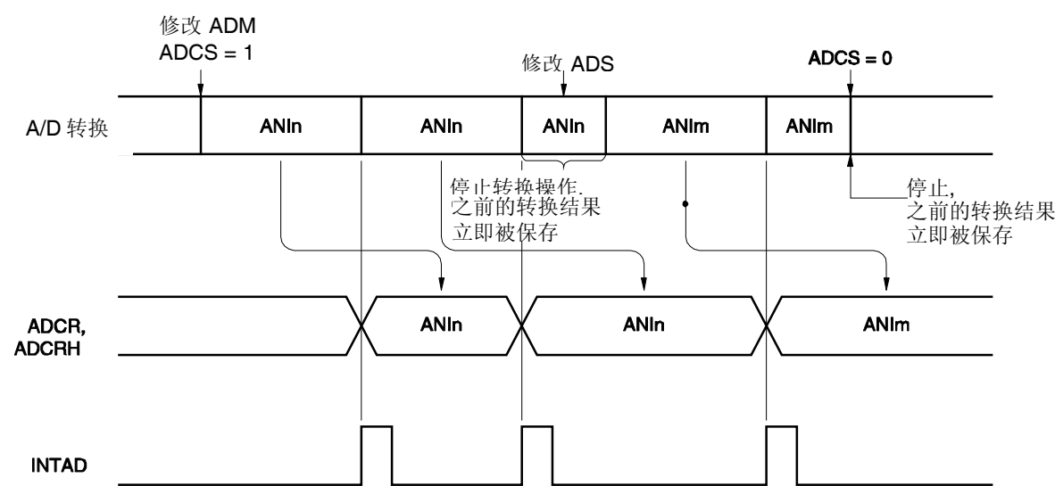
图 12-13. A/D 转换操作
