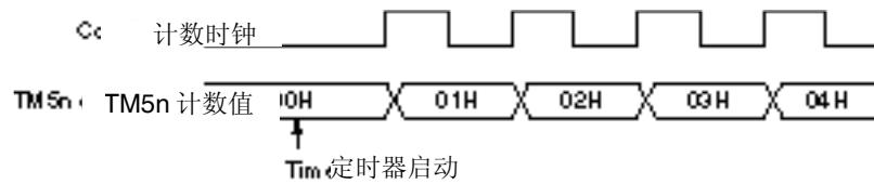
图 7-16. 8 位定时器计数器 5n 启动的时序
