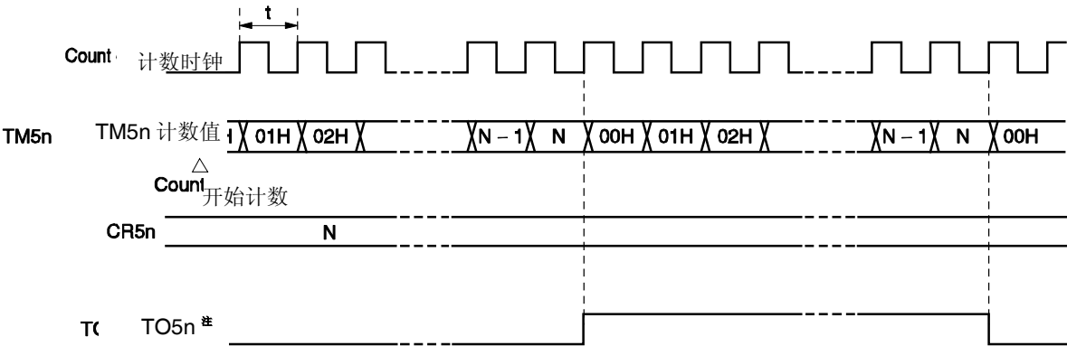
图 7-13. 方波输出操作的时序
