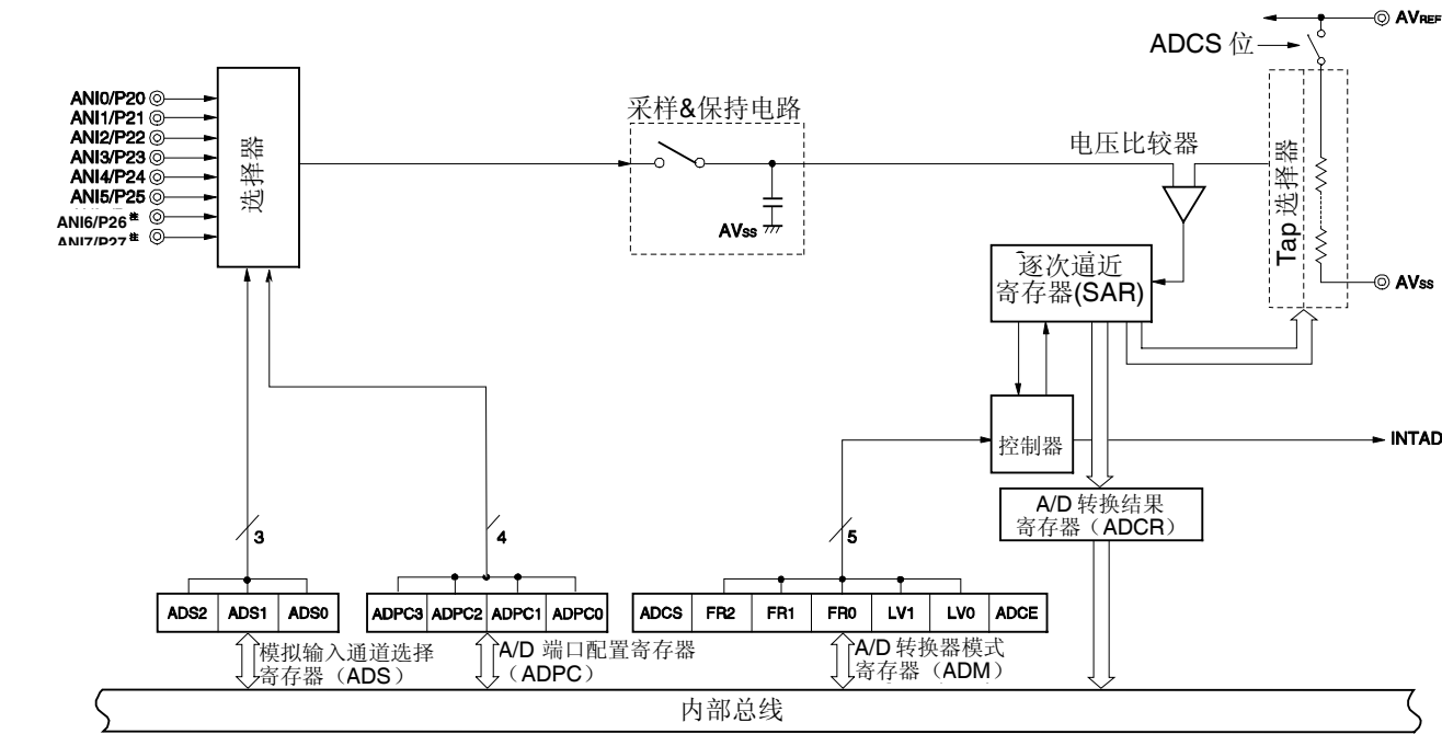
图 12-1. A/D 转换器的框图
