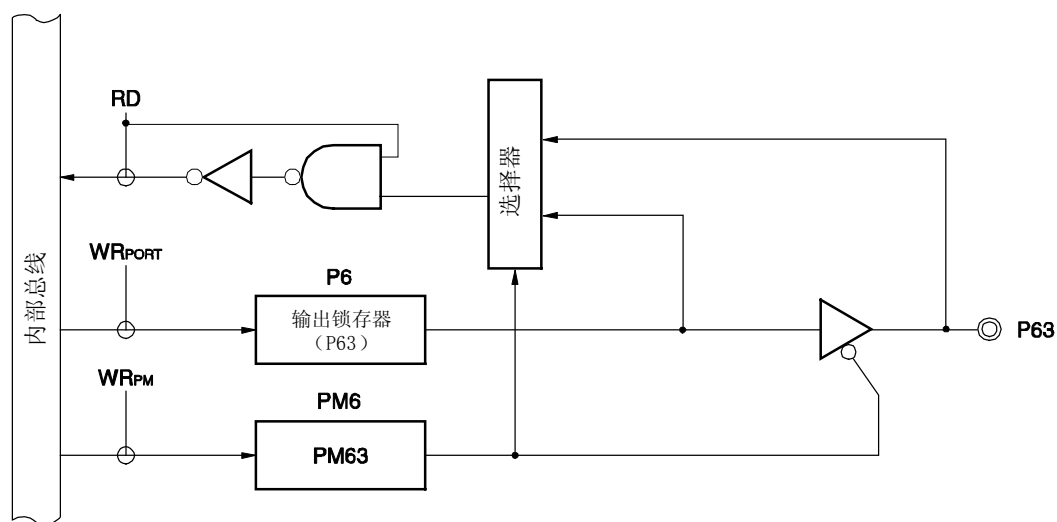
图 4-15. P63 的框图
