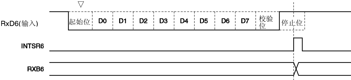
图 14-19. 接收完成中断请求时序
