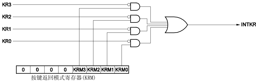
图 19-1. 按键中断的框图
