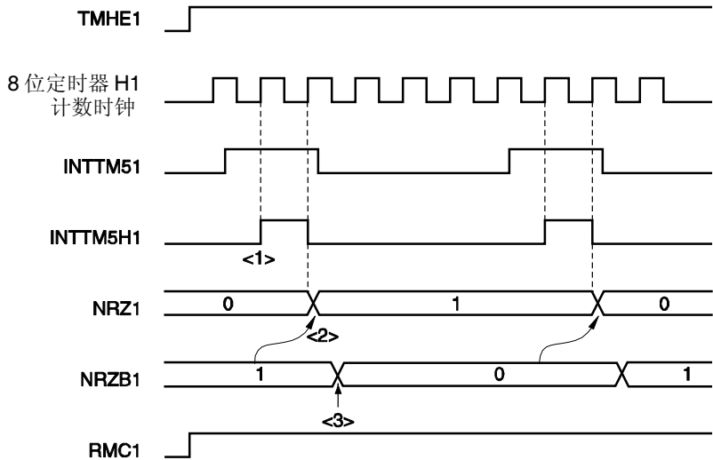
图 8-13. 传送时序
