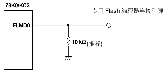
图 25-12. FLMD0 引脚连接示例
