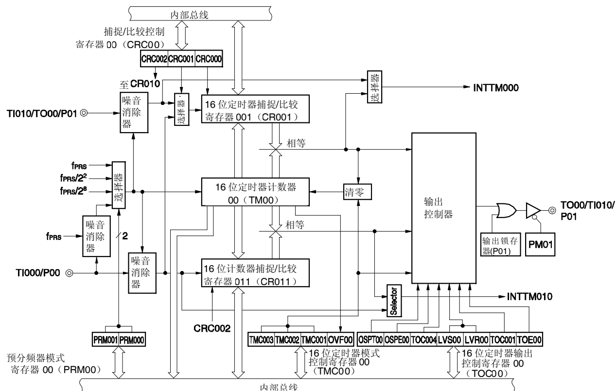
图 6-1. 位定时器/事件计数器 00 的框图
