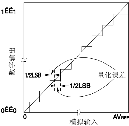
图 12-15. 量化误差
