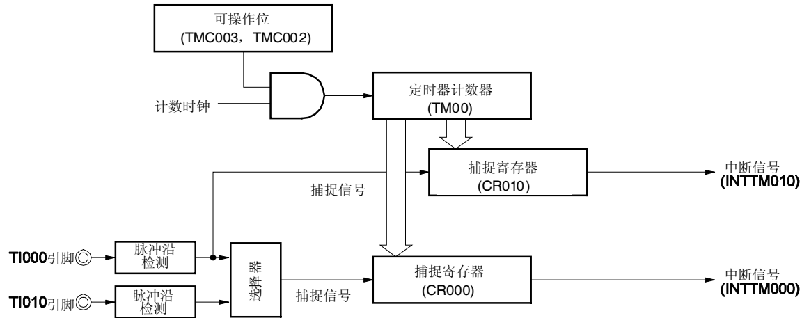
图 6-36. 自由运行定时器模式的框图 (CR000: 捕捉寄存器, CR010: 捕捉寄存器)
