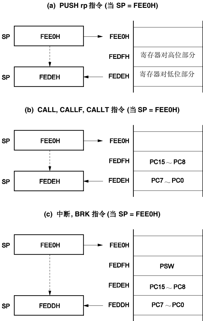
图 3-16. 将数据存入堆栈
