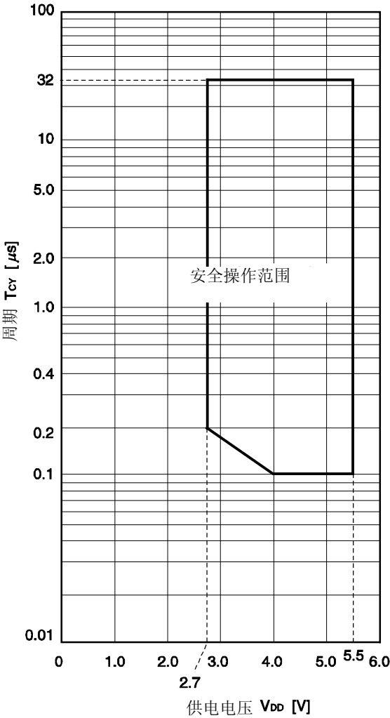
Tcy vs. VDD（主系统时钟操作）
