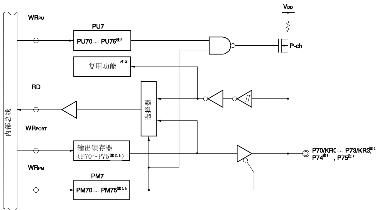
图 4-16. P70 ~ P75 的框图
