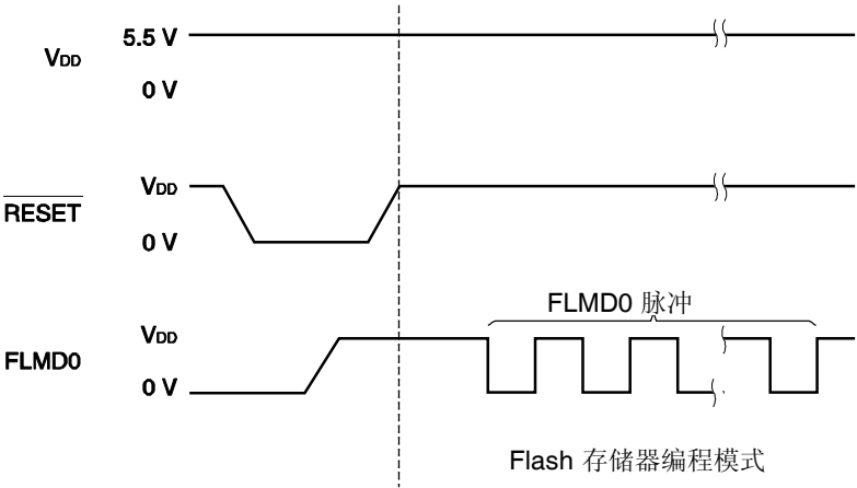
图 25-17. Flash 存储器编程模式
