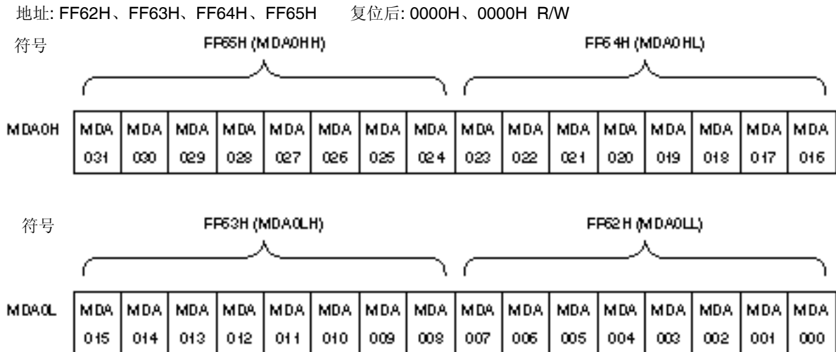
图 17-3. 乘/除数寄存器 A0 (MDA0H、MDA0L)的格式
