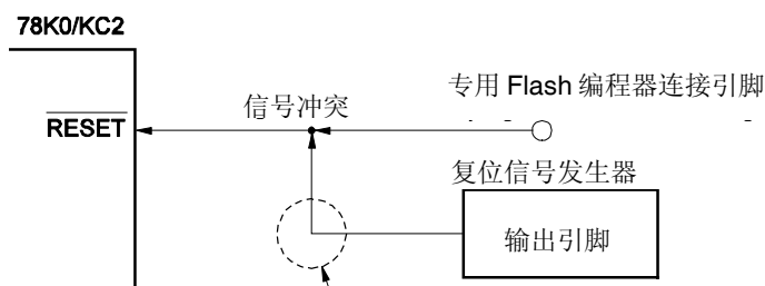
图 25-15. 信号冲突（RESET 引脚）
