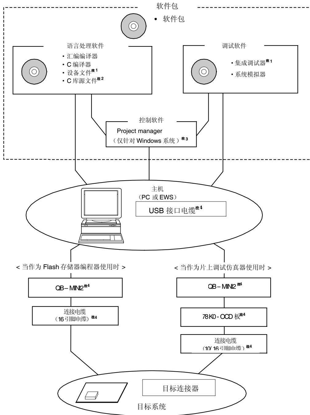
图 A-1. 开发工具的组成 (3/3)
