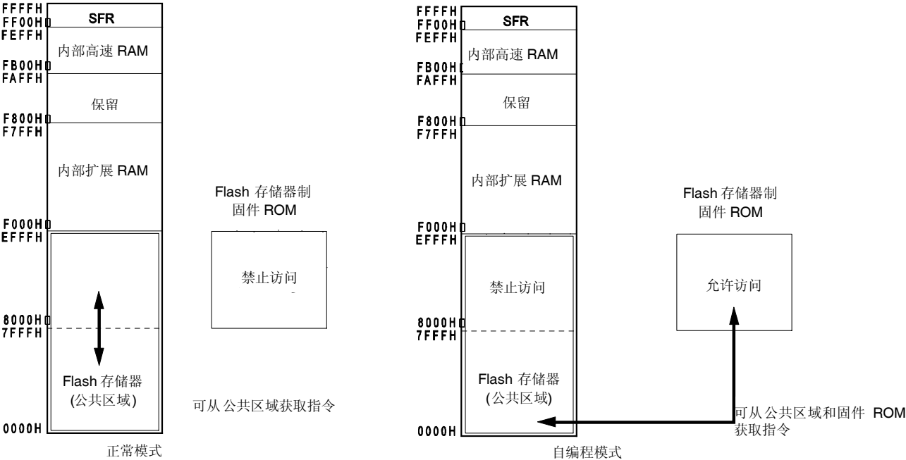
图 25-19. 用于自编程的操作模式与存储器映射(μPD78F0515)
