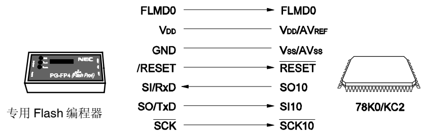
图 25-10. 专用 Flash 存储器编程器的通信 (CSI10)
