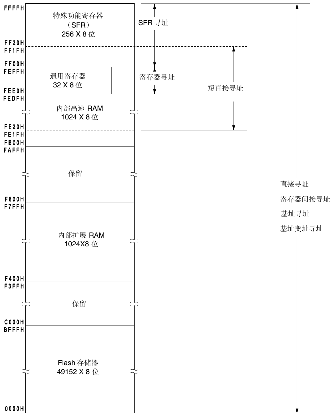
图 3-11. 数据存储空间与寻址方式的对应关系 (μPD78F0514)
