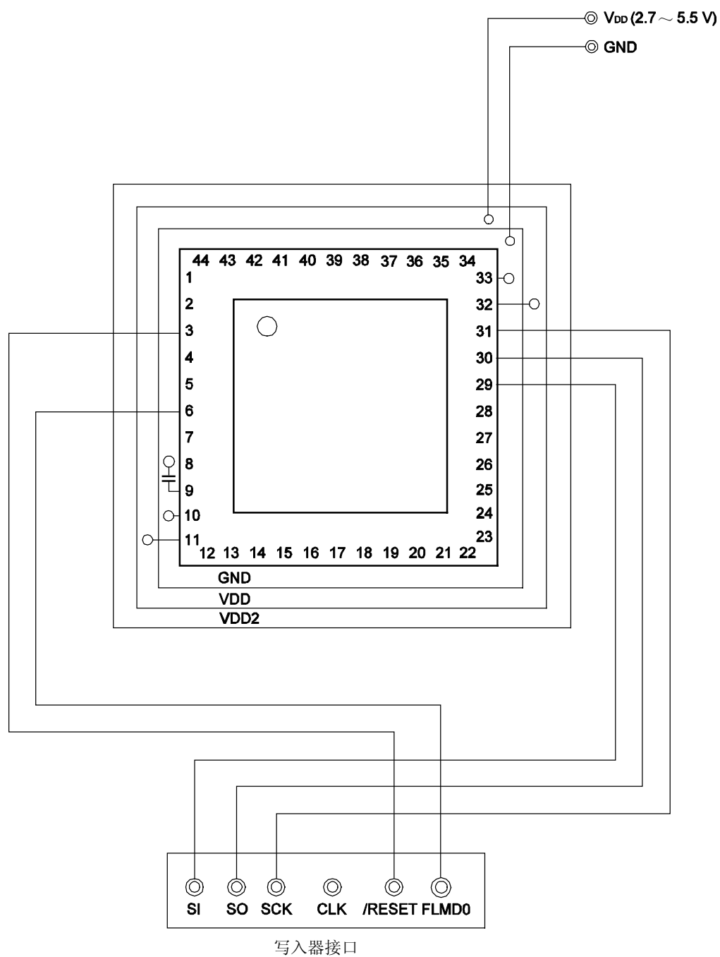
图 25-5. 3 线串行 I/O (CSI10) 模式下使用适配器对 Flash 存储器进行写操作示例(44 引脚产品)
