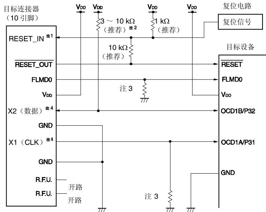
图 26-2. QB-78K0MINI 和 QB-MINI2 与 \mu PD78F0513D, 78F0515D 连接示例 （当使用 OCD1A/P31 和 OCD1B/P32 时）
