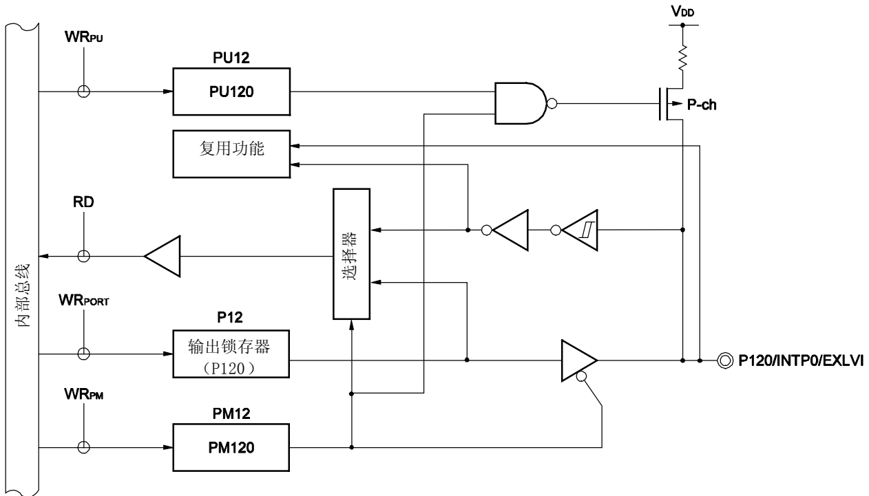
图 4-17. P120 的框图
