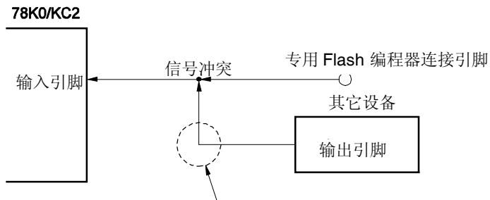
图 25-13. 信号冲突 (串行接口的输入引脚)
