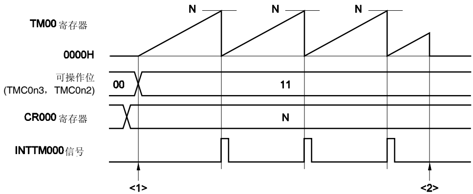
图 6-14. 间隔定时器软件处理示例
