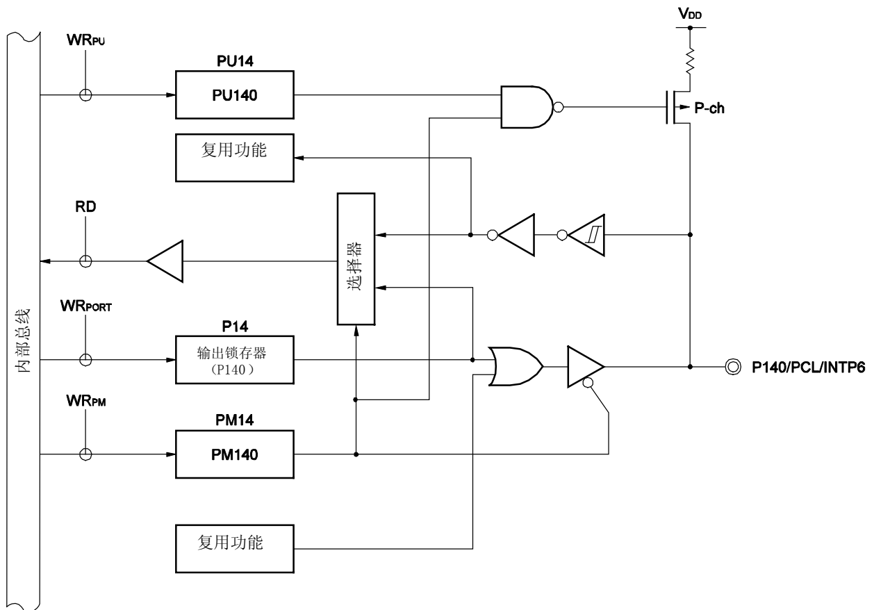
图 4-20. P140 的框图
