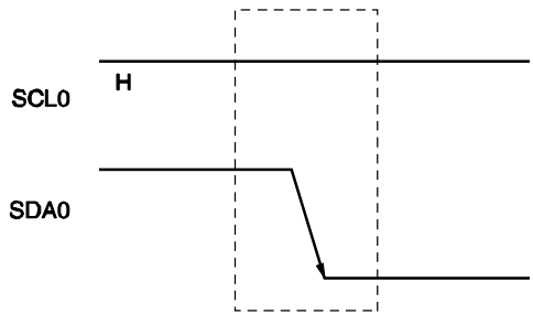
图 16-13. 起始条件
