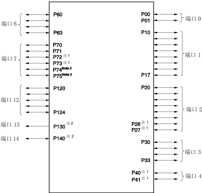
图 4-1. 端口类型
