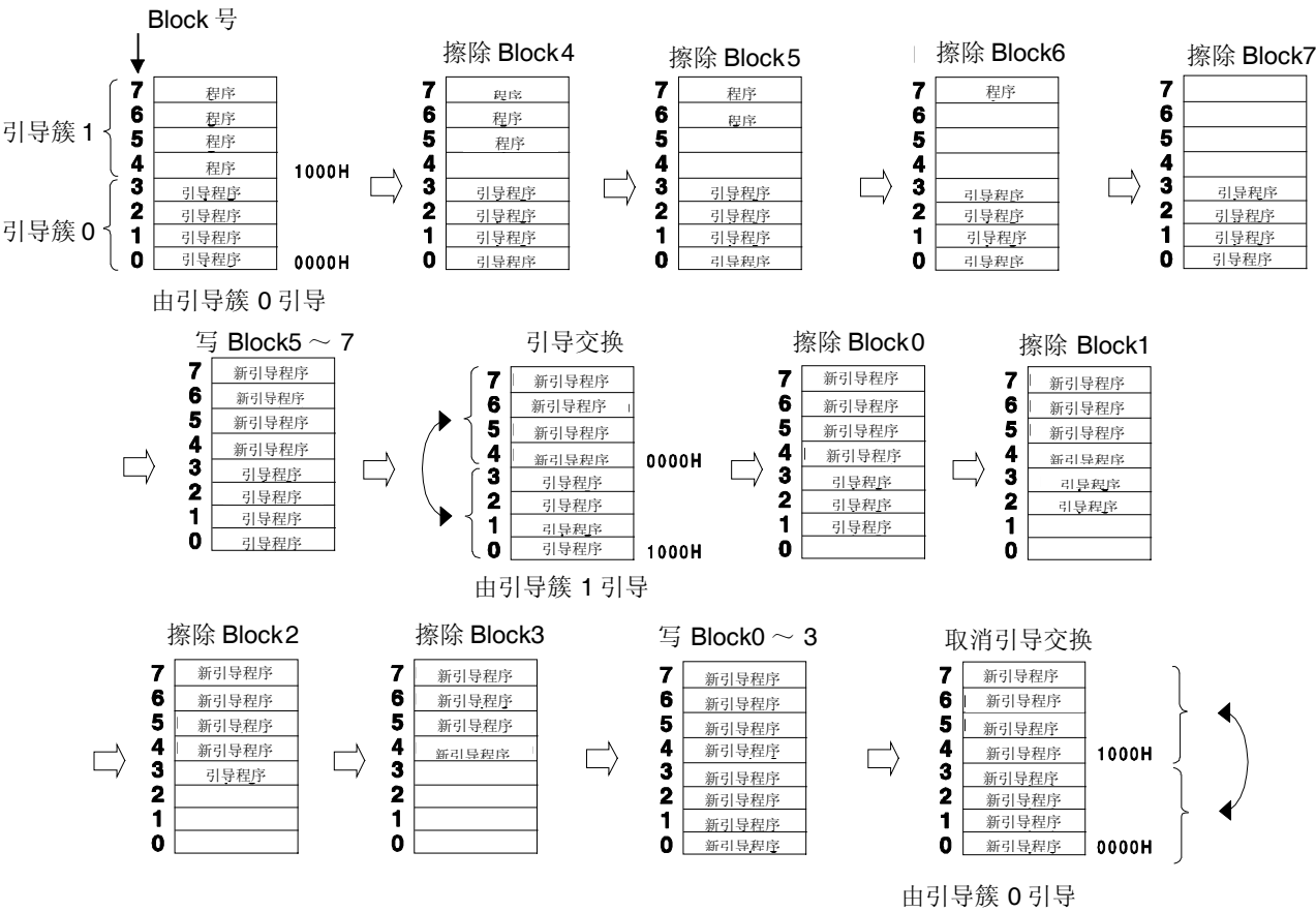
图 25-22. 执行引导交换的示例
