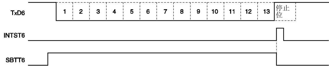
图 14-22. SBF 发送
