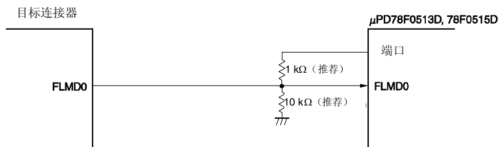
图 26-3. 通过片上调试功能执行自编程时连接 FLMD0 引脚
