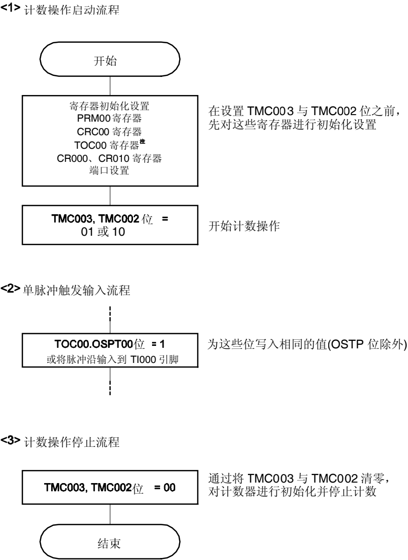
图 6-45. 单脉冲输出操作软件处理示例 (2/2)
