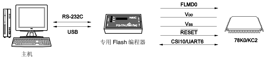
图 25-9. Flash 存储器编程环境
