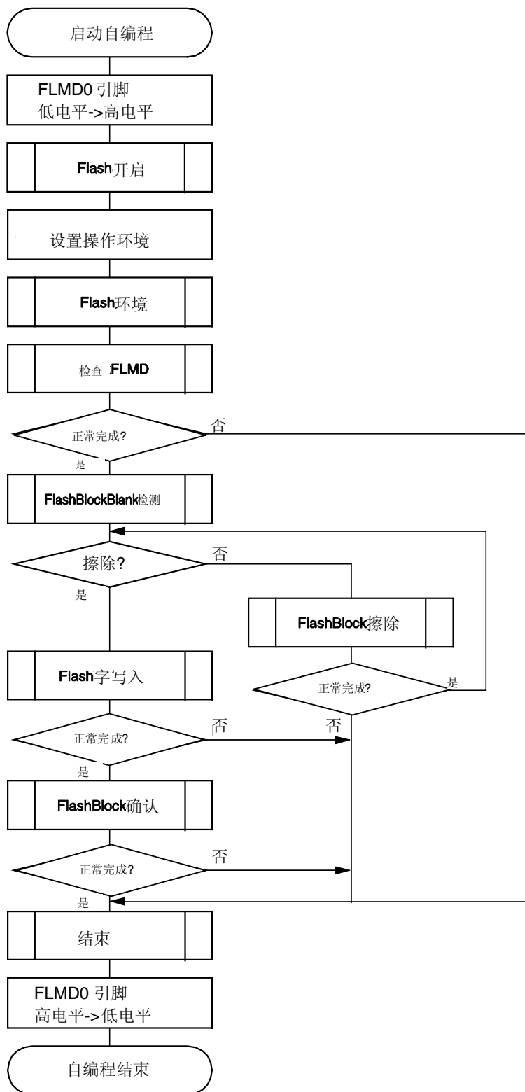
图 25-20. 自编程流程图 (重写 Flash 存储器)
