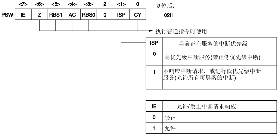
图 18-6. 程序状态字的格式
