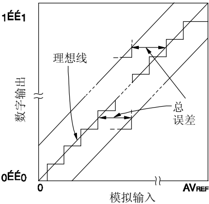
图 12-14. 总误差
