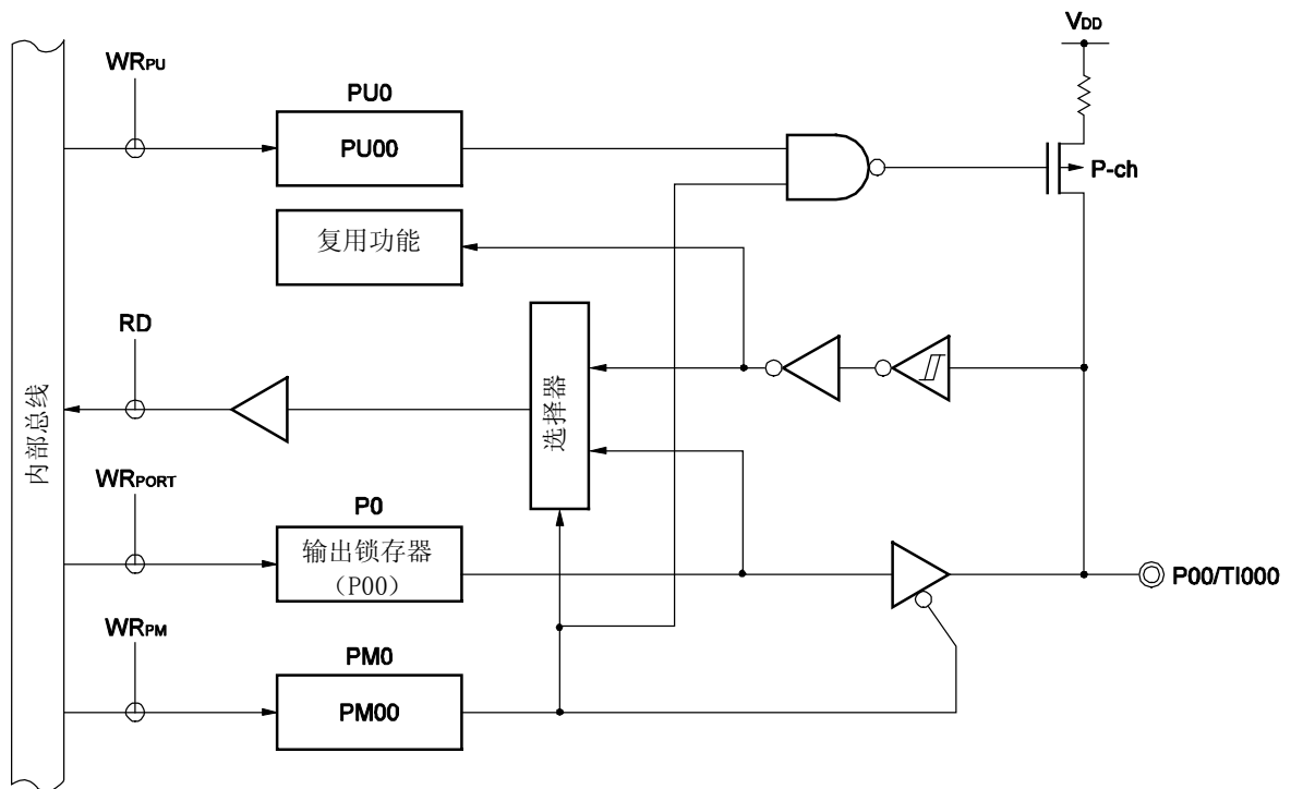
图 4-2. P00 的框图
