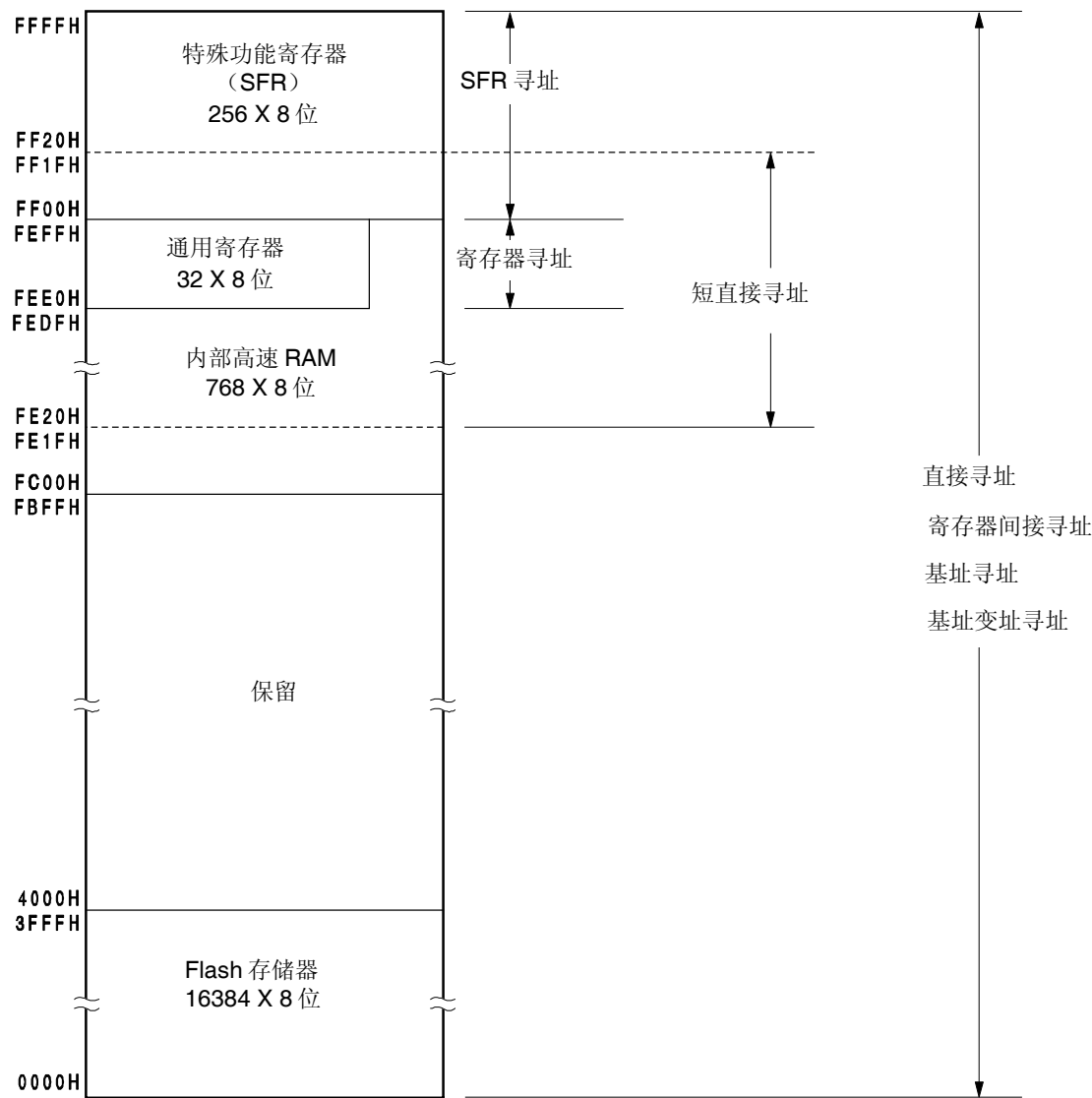
图 3-8. 数据存储空间与寻址方式的对应关系 (μPD78F0511)
