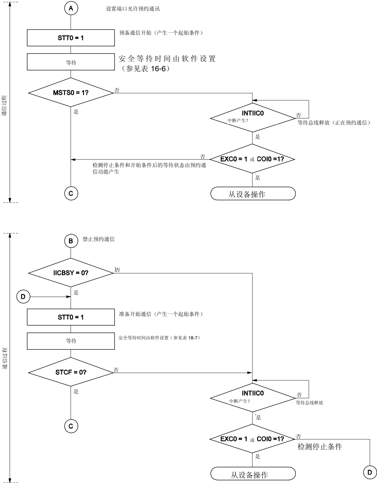
图 16-24. 主设备操作流程(多主设备系统) (2/3)
