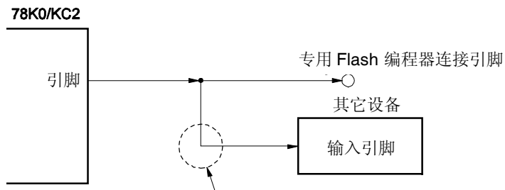
图 25-14. 其它设备的故障
