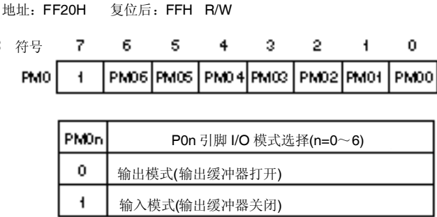
图 6-10. 端口模式寄存器 0 (PM0)的格式
