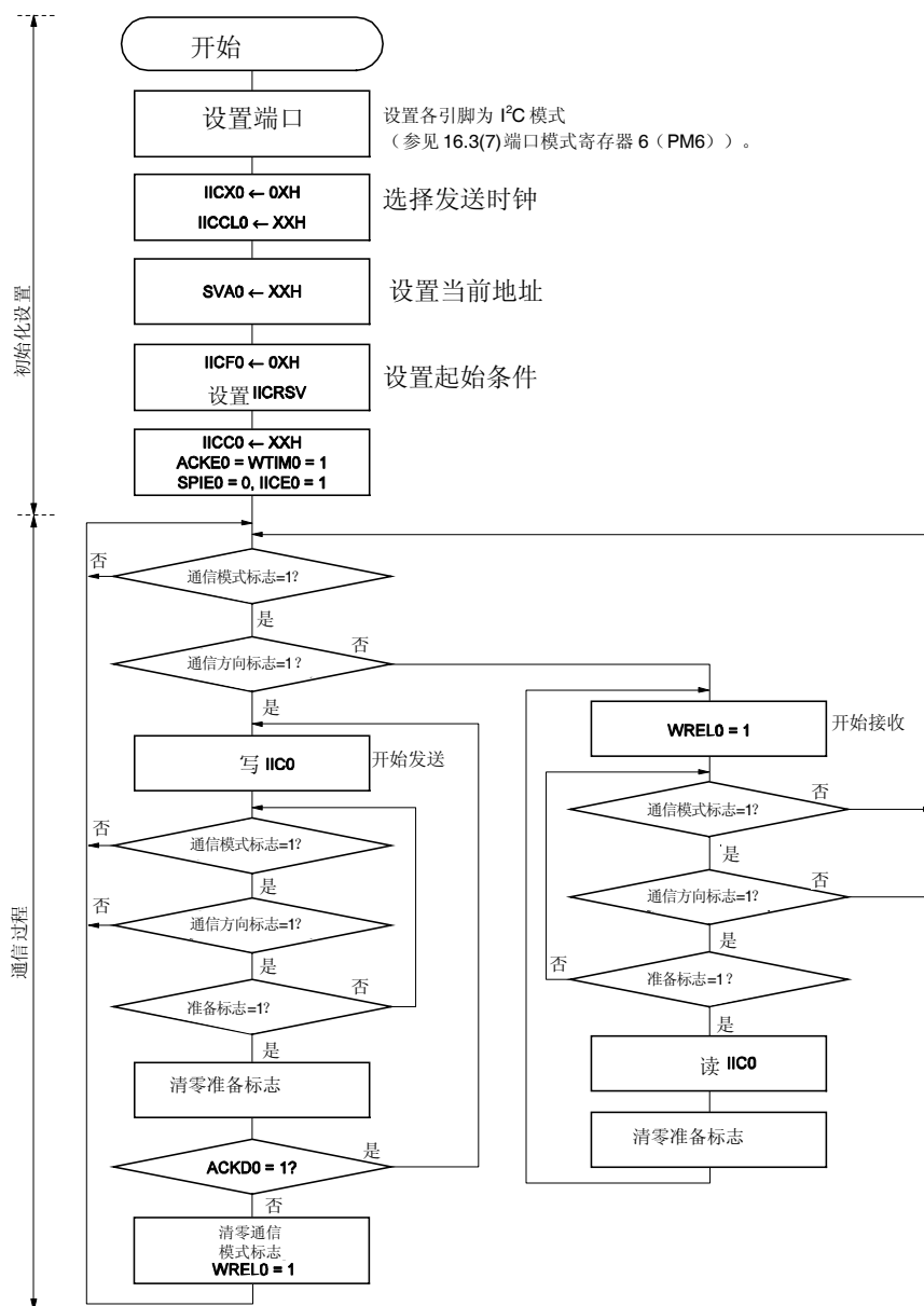
图 16-25. 从设备操作流程图 (1)
