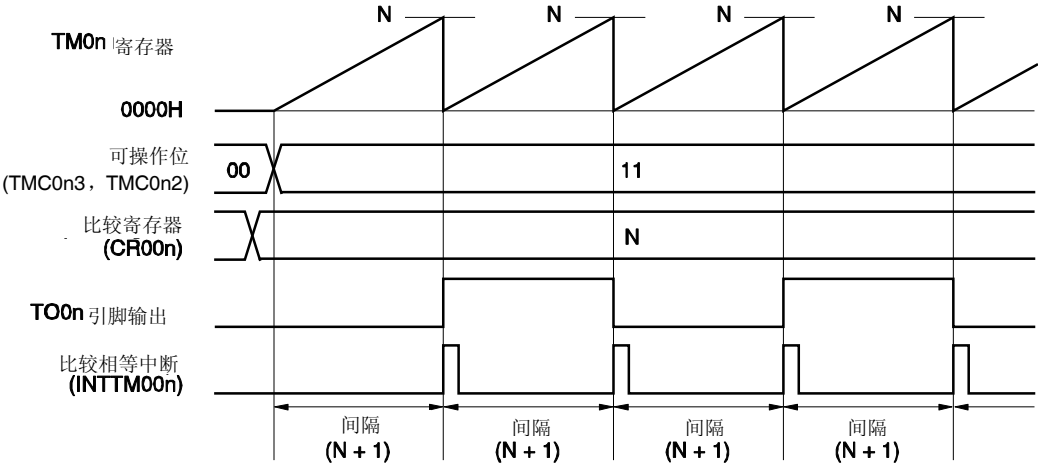
<R> 图 6-16. 方波输出操作的基本时序示例
