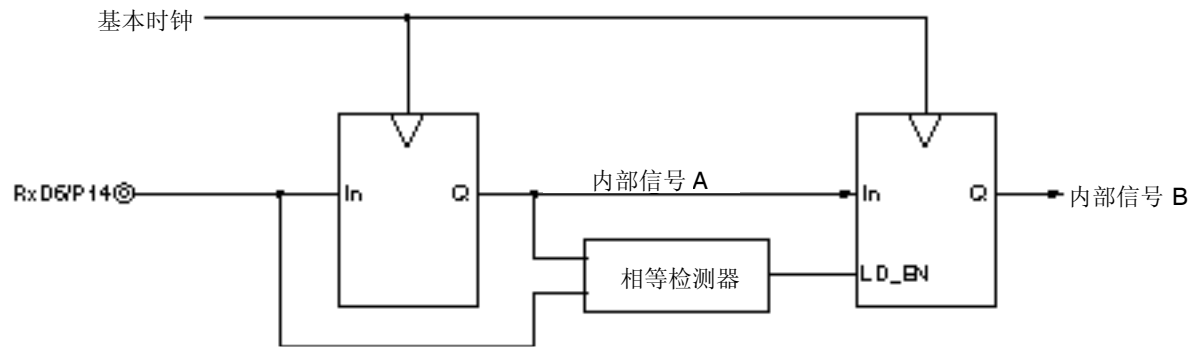
图 14-21. 噪声过滤器电路
