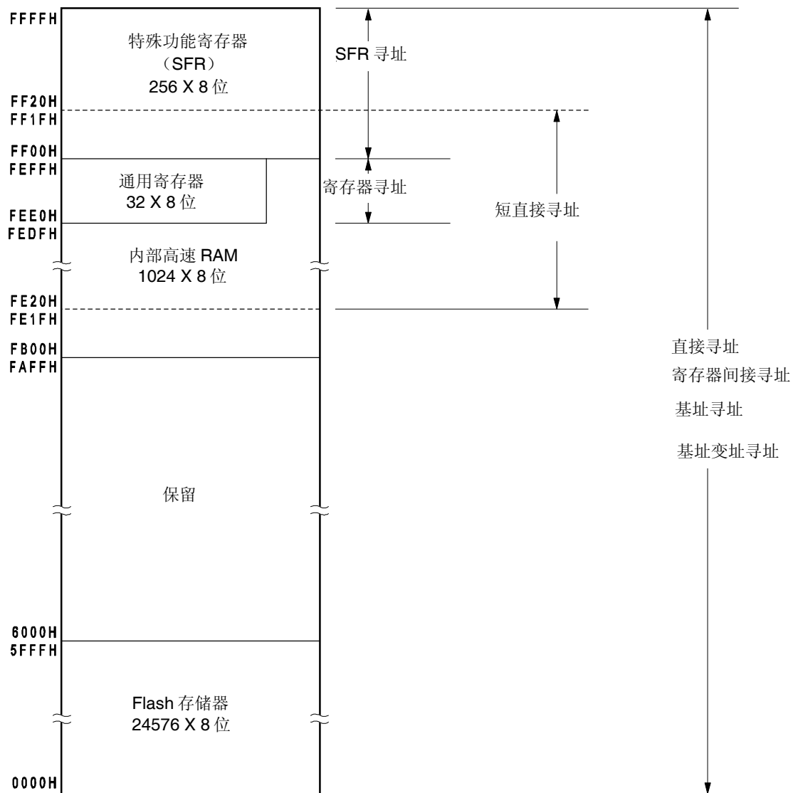
图 3-9. 数据存储空间与寻址方式的对应关系 (μPD78F0512)
