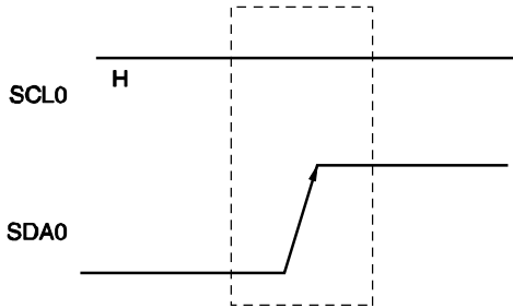
图 16-17. 停止条件
