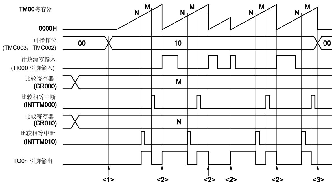
图 6-31. 清零&amp;启动模式(通过 TI000 引脚有效沿输入进入)下软件处理示例
