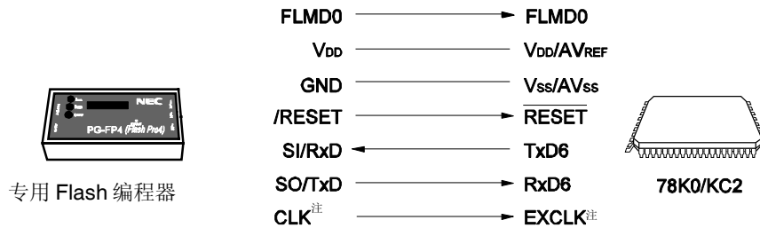
图 25-11. 专用 Flash 编程器的通信(UART6)
