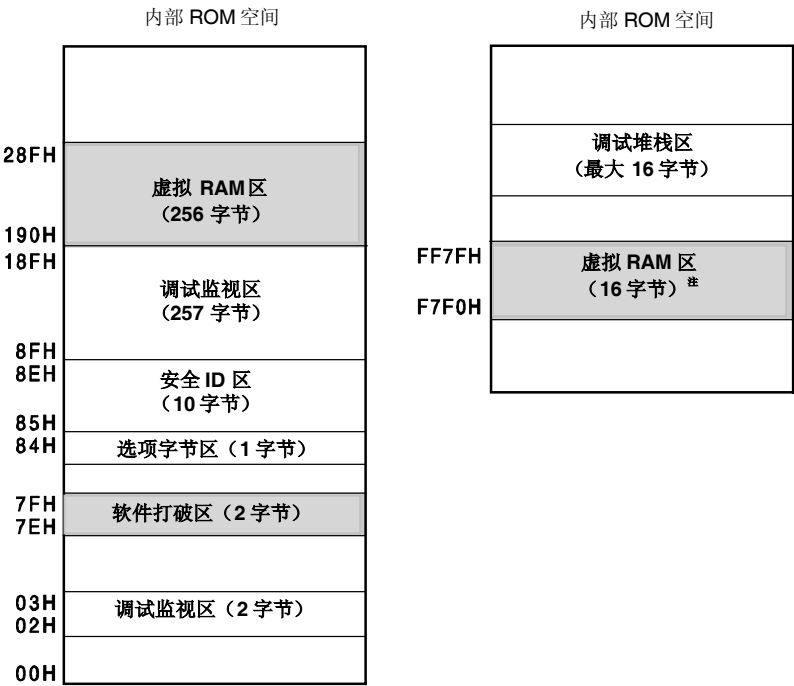
图 26-4. QB-78K0MINI 和 QB-MINI2 使用的保留区域
