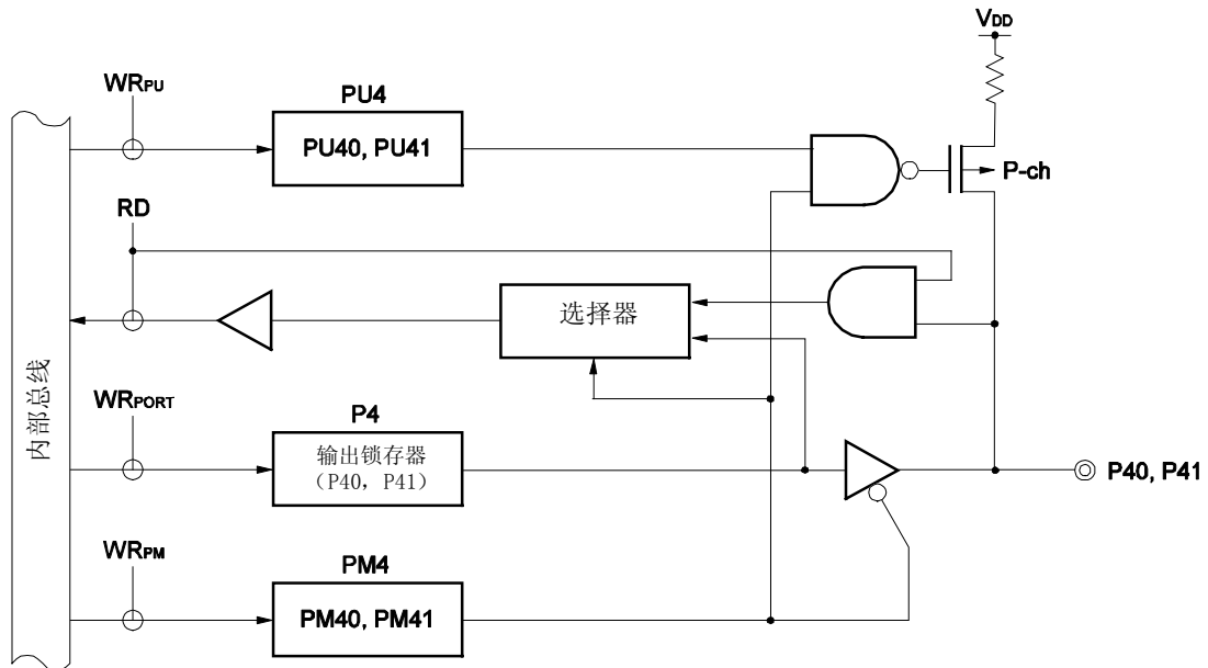
图 4-12. P40, P41 的框图(仅用于 44 引脚和 48 引脚产品)
