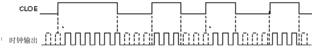
图 11-4. 遥控输出应用举例
