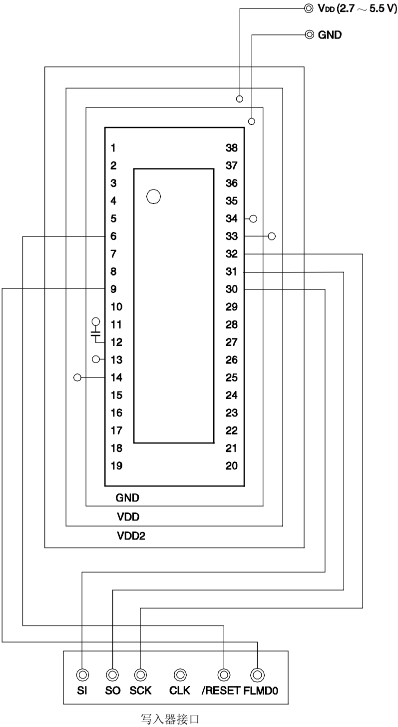
<R> 图 25-3. 3 线串行 I/O (CSI10) 模式下使用适配器对 Flash 存储器进行写操作示例(38 引脚产 品)
