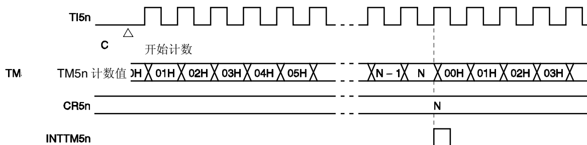
图 7-12. 外部事件计数器操作的时序 (规定上升沿有效)
