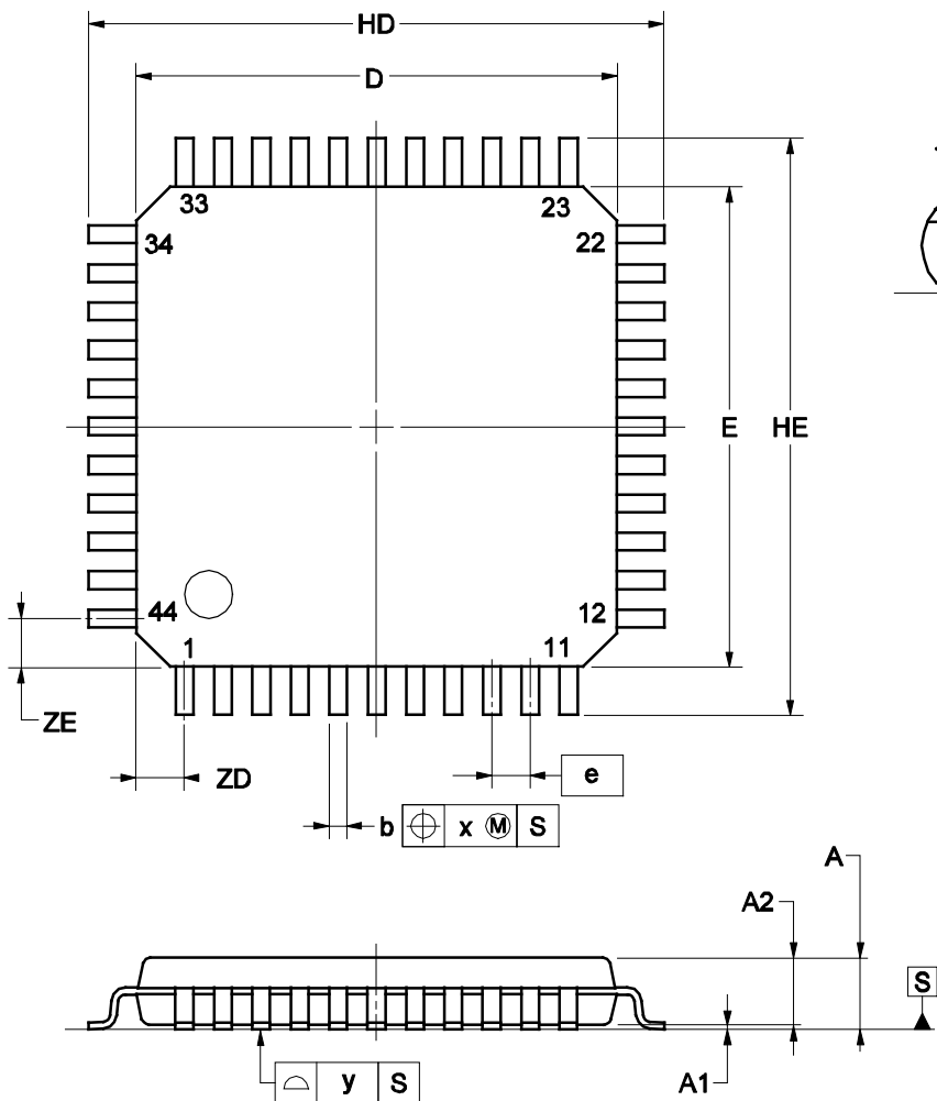
引脚端详图
