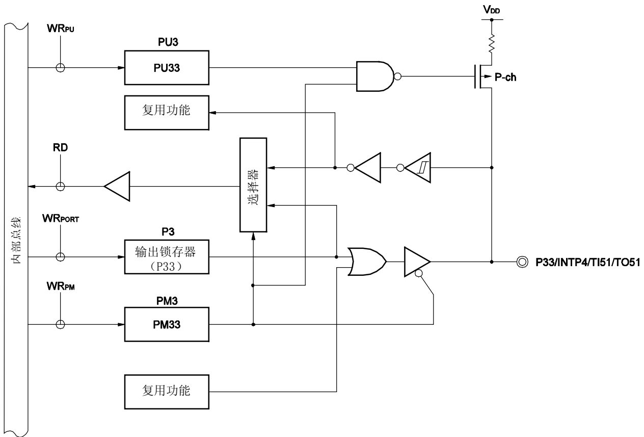
图 4-11. P33 的框图
