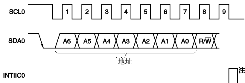
图 16-14. 地址
