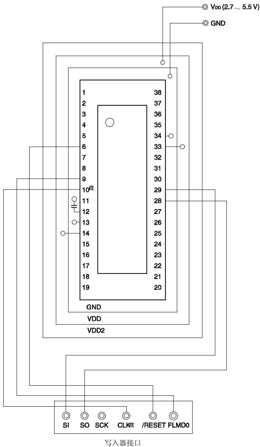
图 25-4. UART (UART6) 模式下使用适配器对 Flash 存储器进行写操作示例(38 引脚产品)
