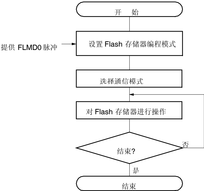
图 25-16. Flash 存储器操作过程
