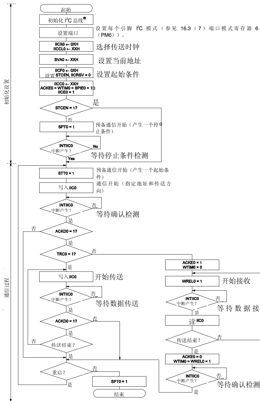
图 16-23. 主设备操作流程图中 (单主设备系统)
