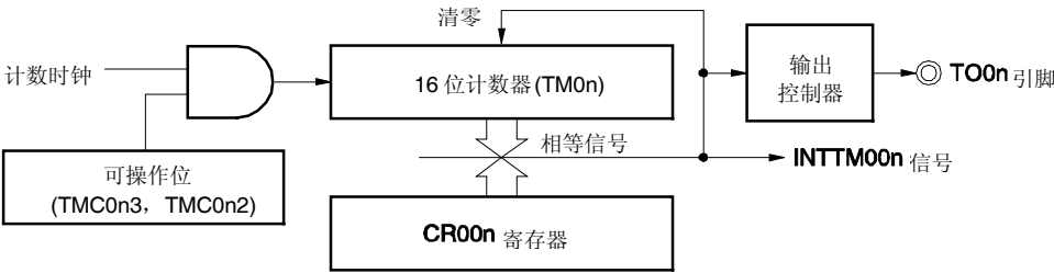
<R> 图 6-15. 方波输出操作框图
