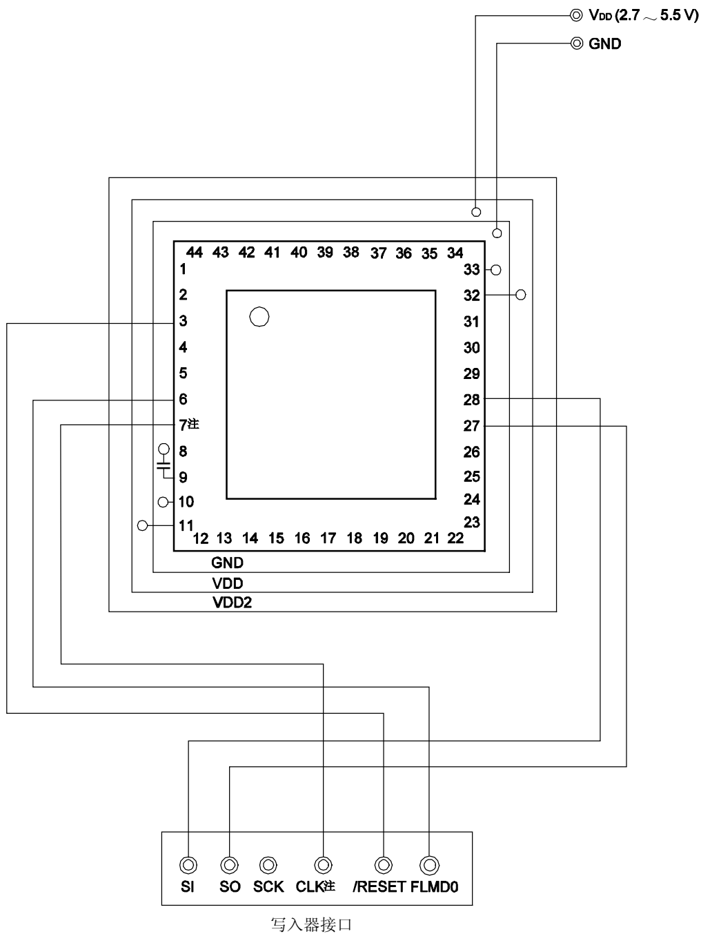
图 25-6. UART (UART6) 模式下使用适配器对 Flash 存储器进行写操作示例(44 引脚产品)
