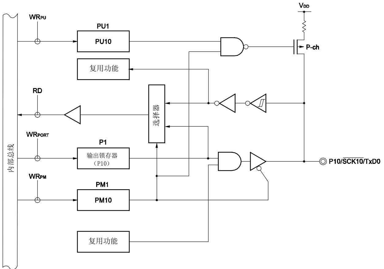
图 4-4. P10 的框图
