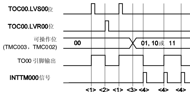
图 6-54. LVR0n 和 LVS0n 时序示例
