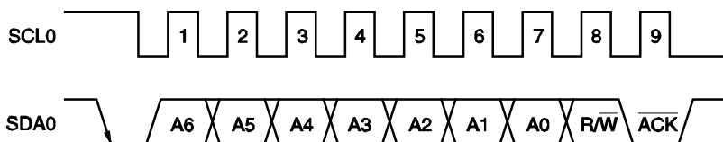
图 16-16. \overline{\text{ACK}} 信号
