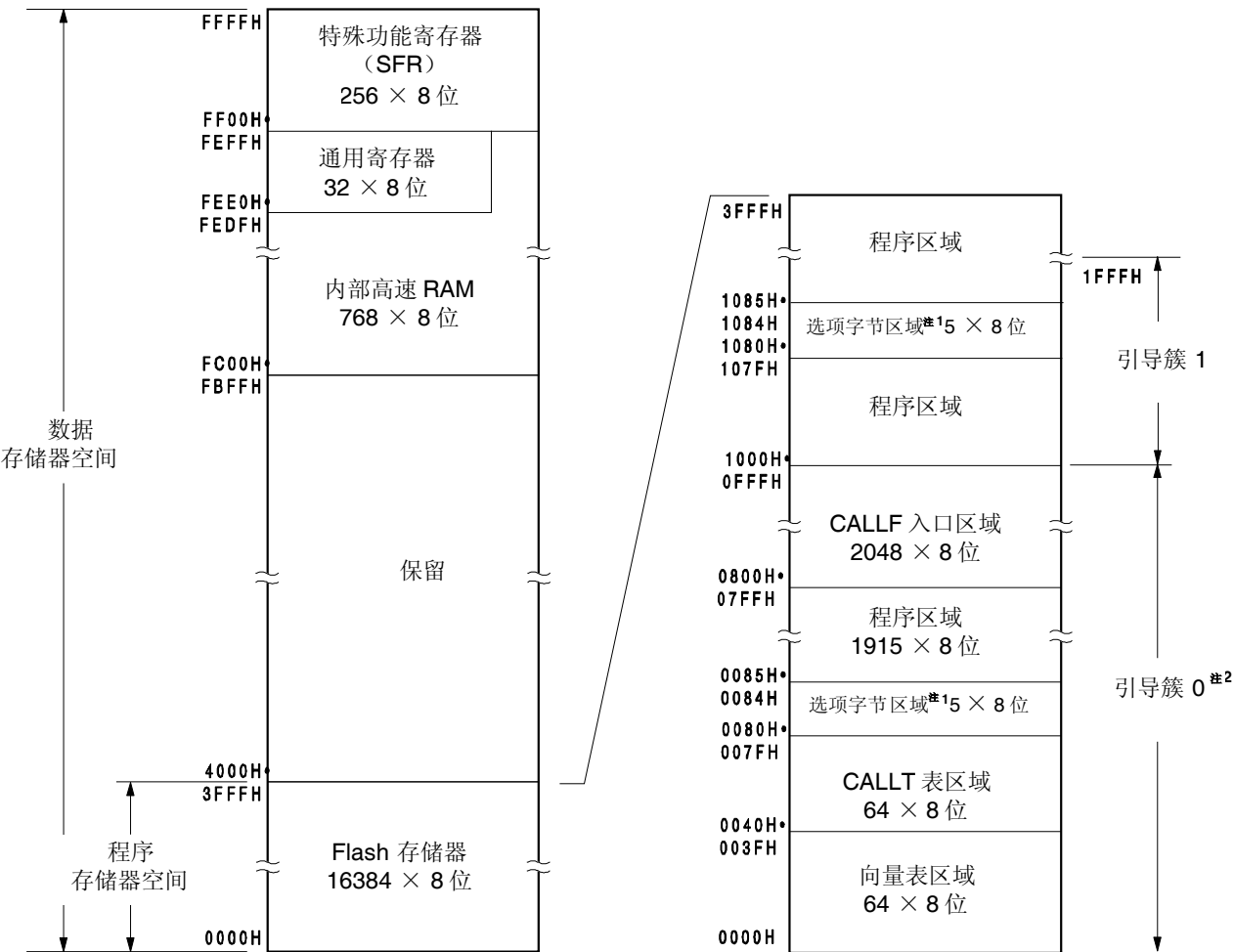
图 3-1. 存储空间映射图 (μPD78F0511)
