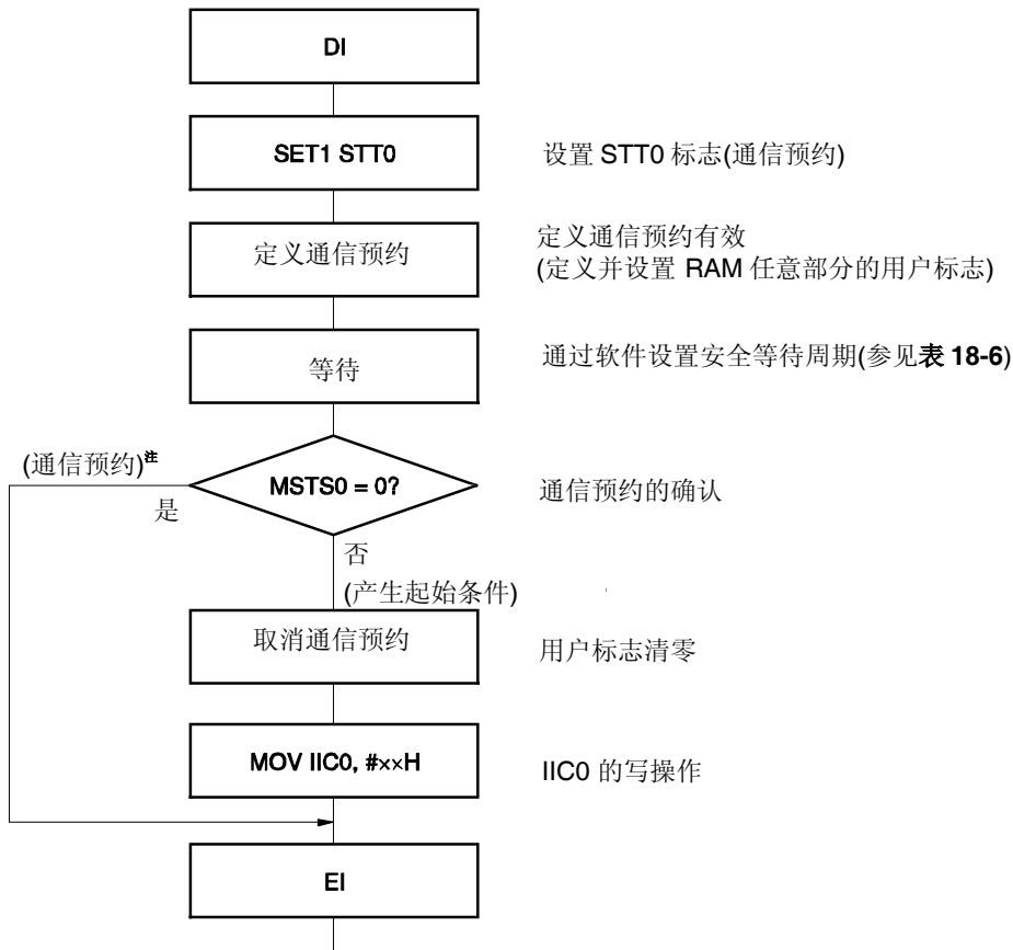
图 16-22. 通信预约方案
