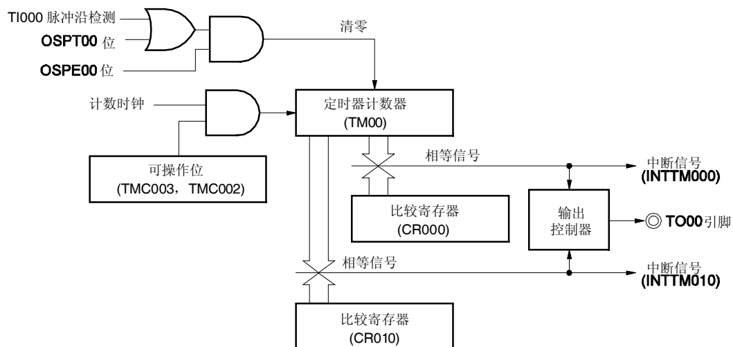
图 6-43. 单脉冲输出操作的框图
