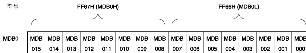
图 17-4. 乘/除数寄存器 B0 (MDB0)的格式
