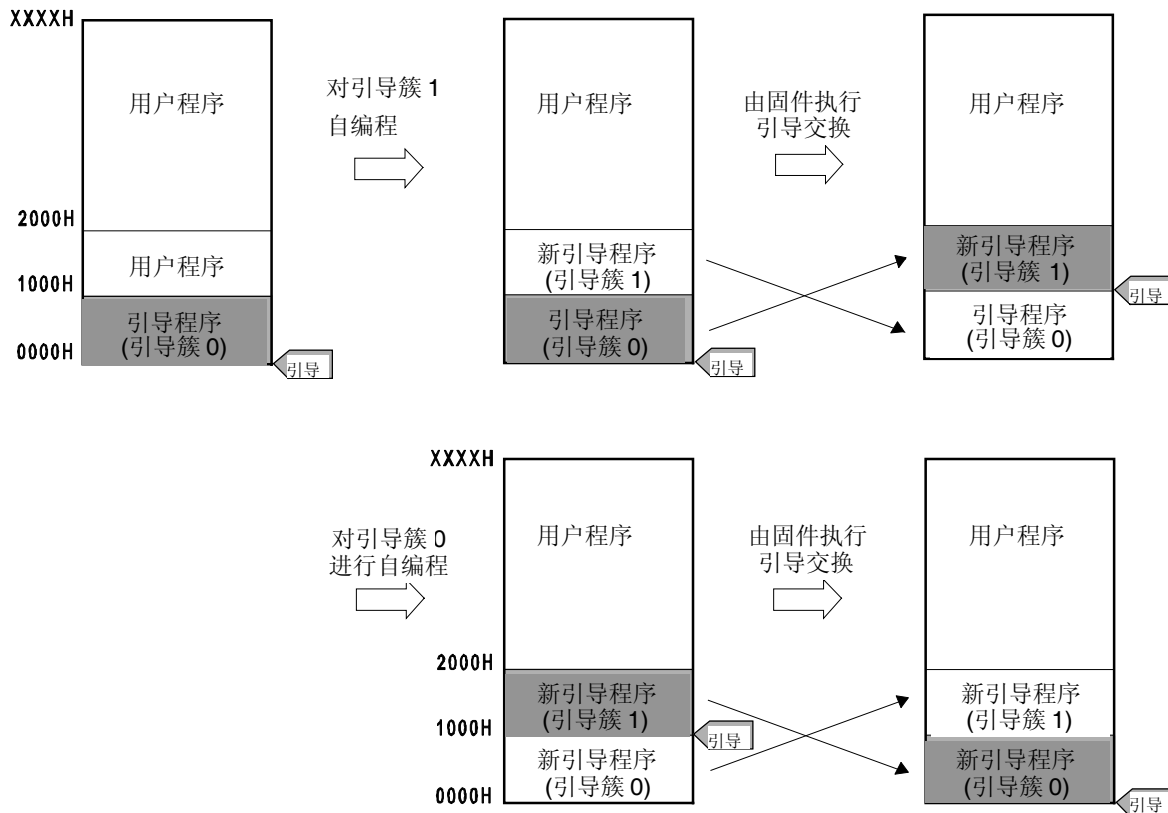
<R> 图 25-21. 引导交换功能
