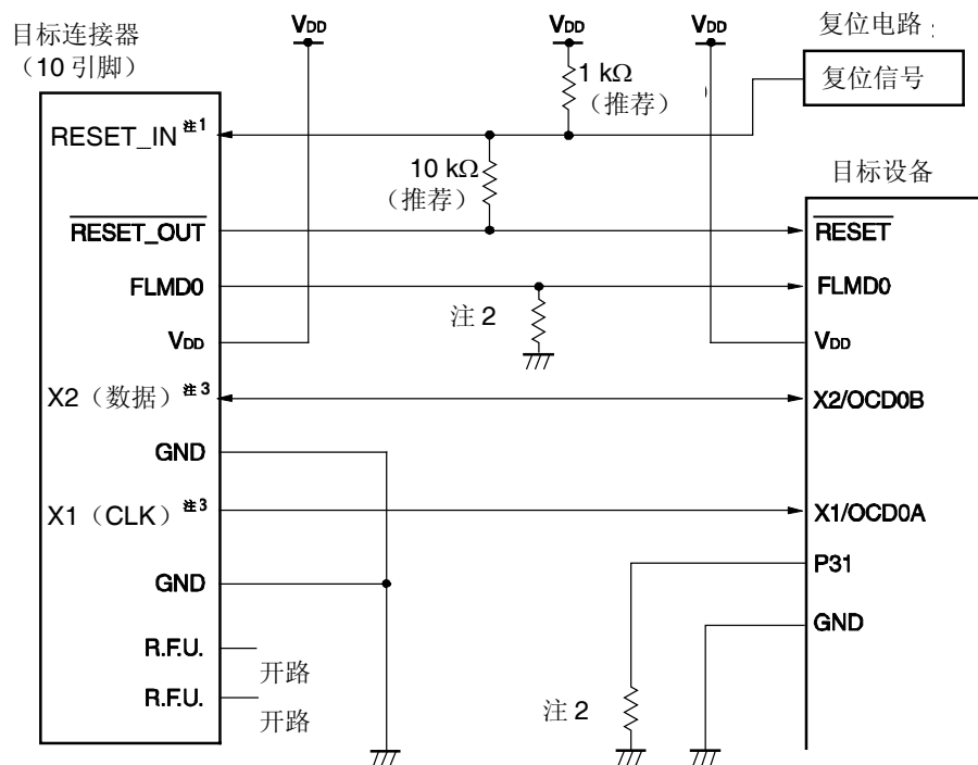
图 26-1. QB-78K0MINI 和 QB-MINI2 与 \mu PD78F0513D 和 78F0515D 的连接示例 （当使用 OCD0A/X1 和 OCD0B/X2 时）
