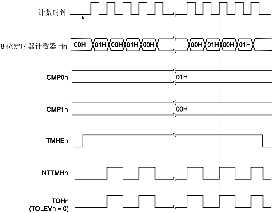
图 8-12. PWM 输出模式下的操作时序 (3/4) (d) 当 CMP0n = 01H, CMP1n = 00H 时的操作
