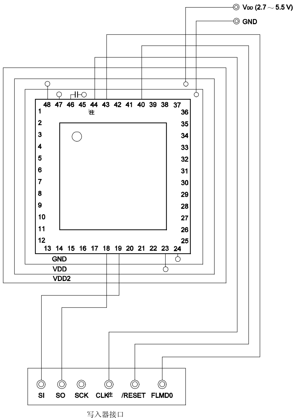
图 25-8. UART (UART6) 模式下使用适配器对 Flash 存储器进行写操作示例(48 引脚产品)
