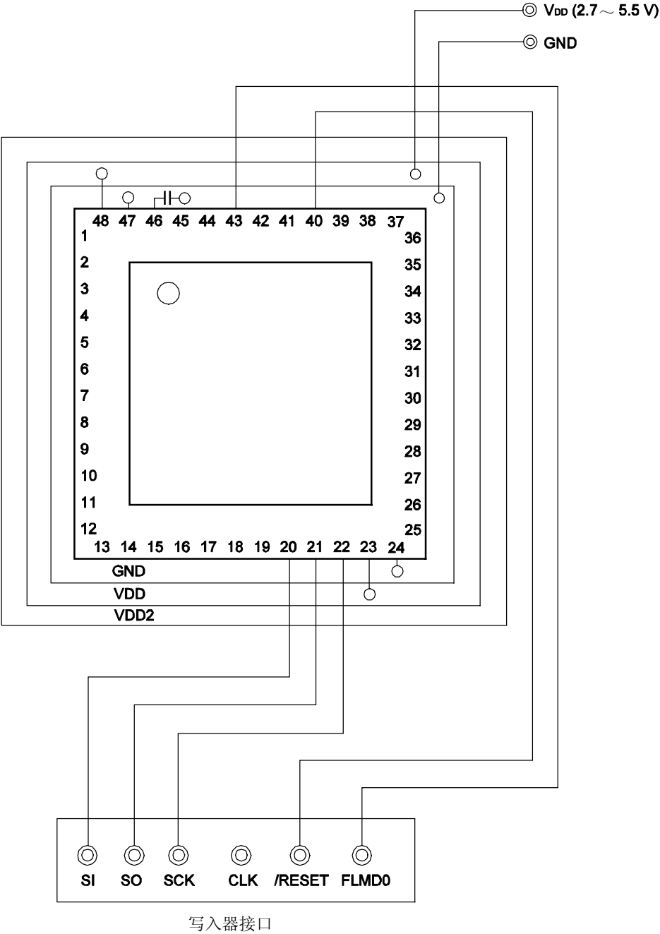
图 25-7 3 线串行 I/O (CSI10) 模式下使用适配器对 Flash 存储器进行写操作示例(48 引脚产品)
