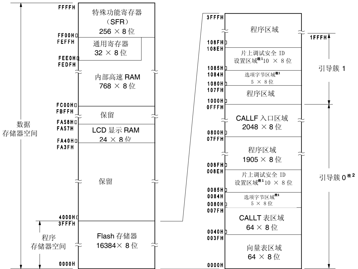
图 3-2. 存储器映射图(μPD78F0421, 78F0431)
