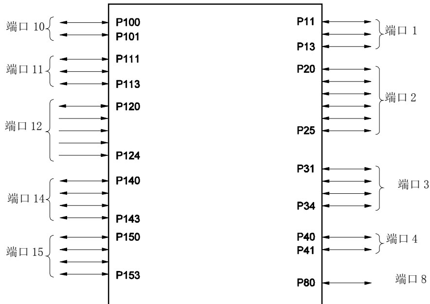
图 4-1. 端口类型
