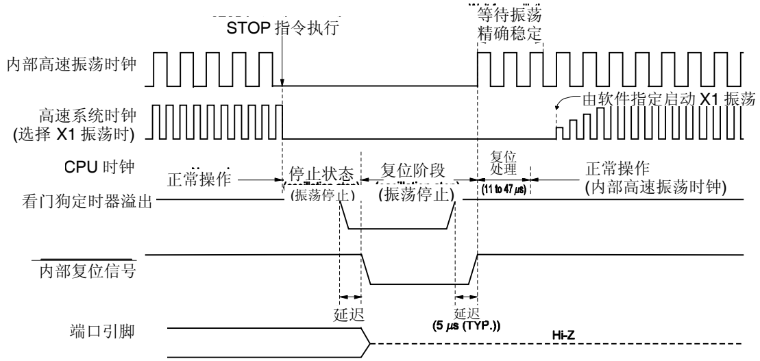
图 22-4. 在 STOP 模式下通过 RESET 输入进行复位的时序
