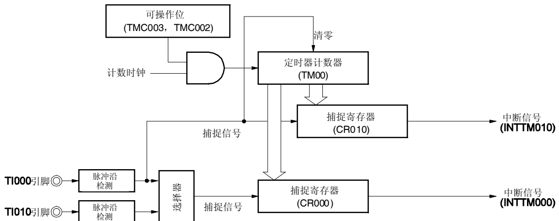
图 6-48. 脉冲宽度测量的框图 (清零&启动模式(通过 TI000 引脚有效沿输入进入))
