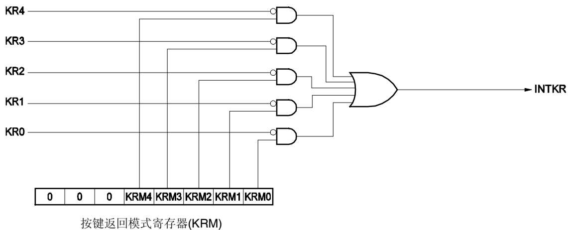
图 20-1. 按键中断的框图
