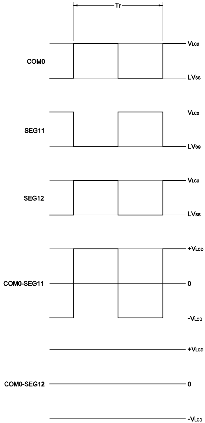
图 16-12. 静态 LCD 驱动波形举例
