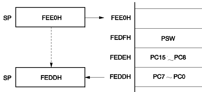
(c) 中断, BRK 指令 (当 SP = FEE0H)
