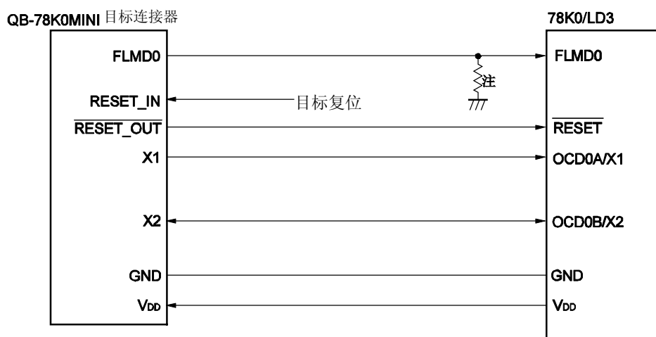
图 27-1. QB-78K0MINI 和 78K0/LD3 连接示例 (当使用 \overline{OCD0A/X1} 和 \overline{OCD0B/X2} 时)
