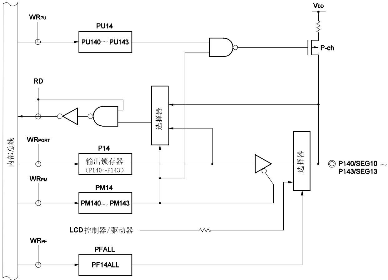
图 4-18. P140~P143 的框图
