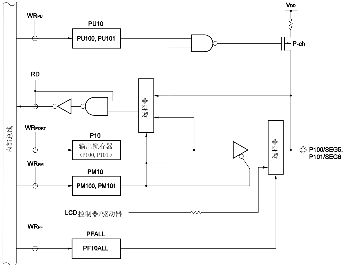
图 4-11. P100 和 P101 的框图
