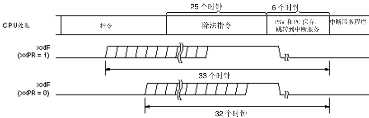
图 19-9. 中断请求响应时序 (最长时间)
