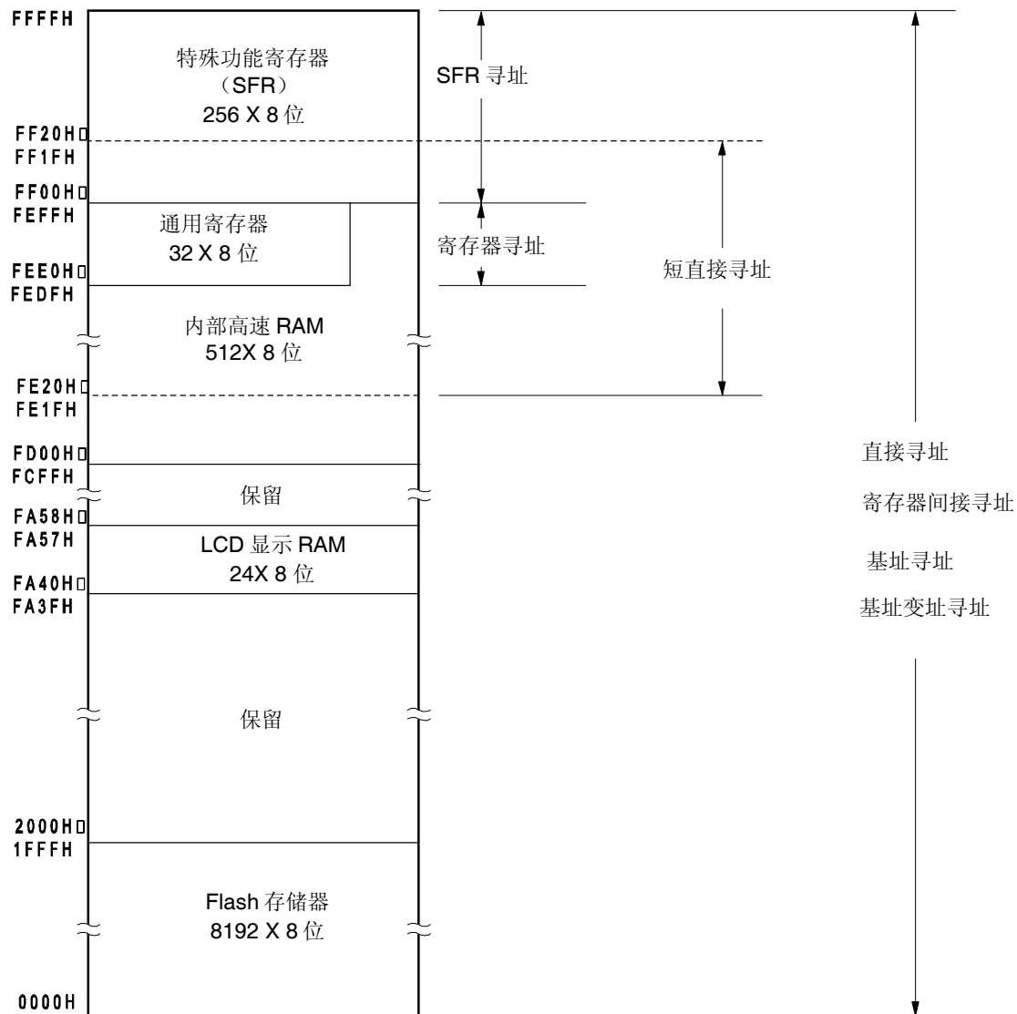
图 3-5. 数据存储与寻址方式的对应关系(μPD78F0420, 78F0430)
