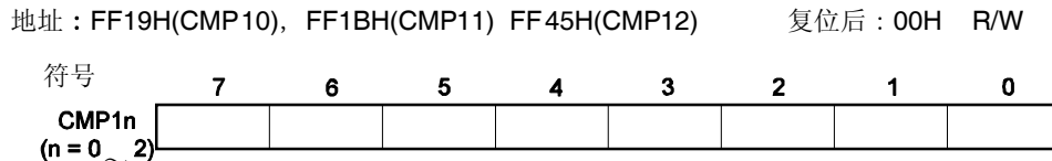
图 8-5. 8 位定时器 H 比较寄存器 1n (CMP1n)的格式
