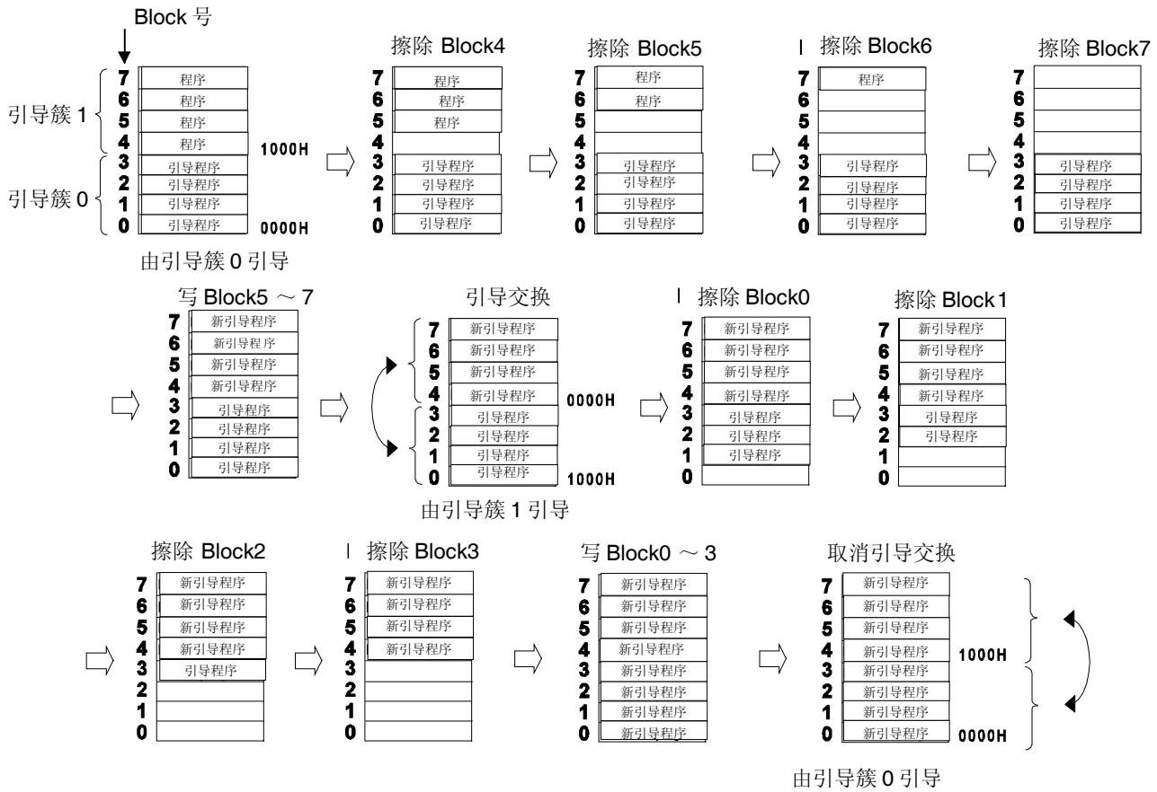
图 26-16. 引导交换执行示例
