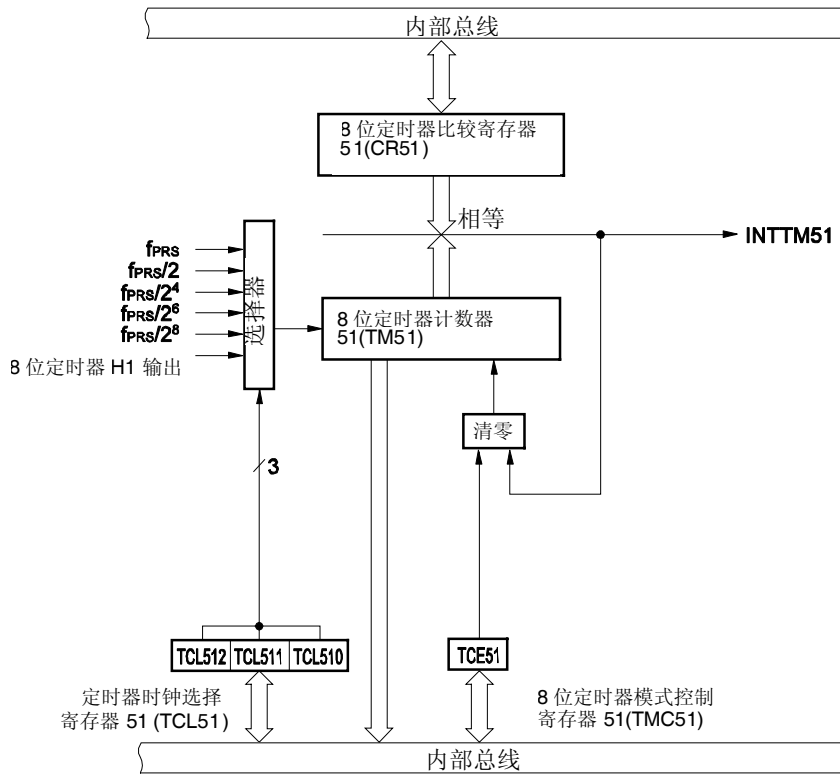
图 7-2. 8 位定时器/事件计数器 51 的框图
