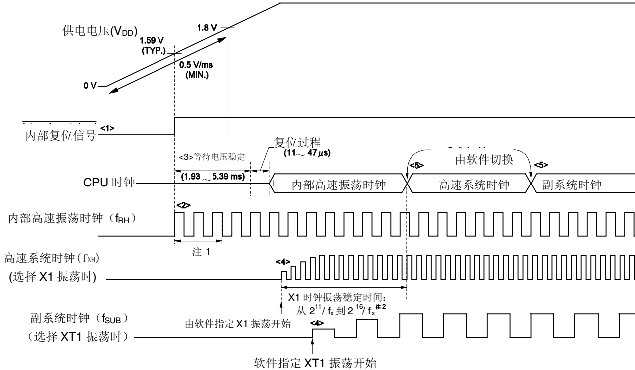
图 5-13. 上电时的时钟发生器操作 (设置 1.59 V POC 模式 (选项字节: POCMODE = 0))
