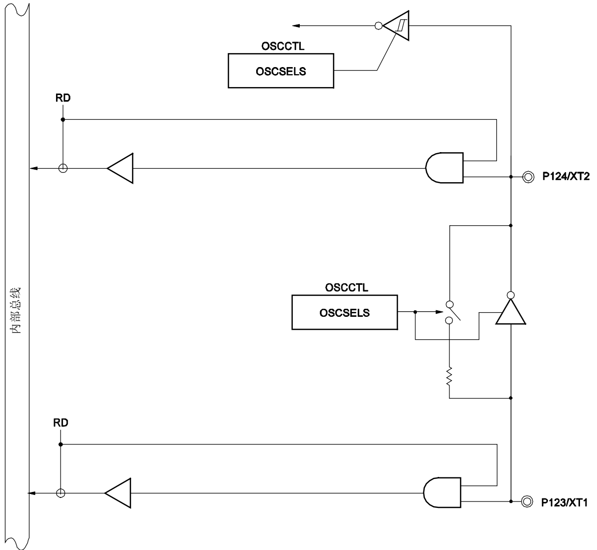
图 4-17. P123 和 P124 的框图
