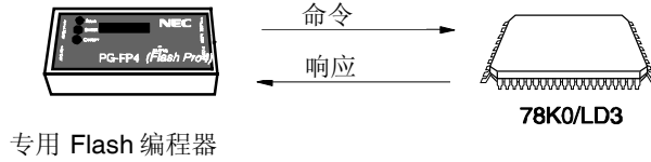
图 26-13. 通信命令
