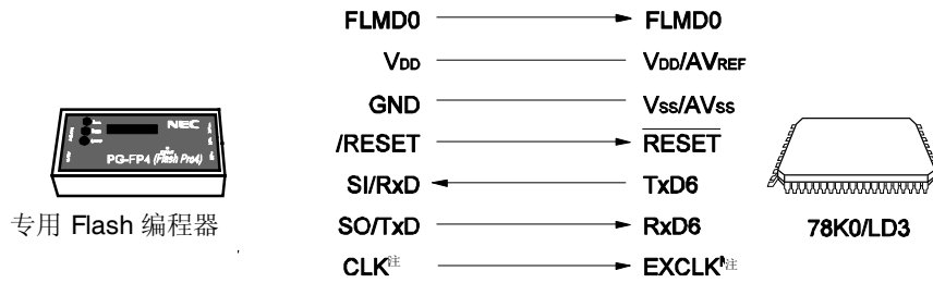
图 26-6. 专用 Flash 编程器的通信(UART6)
