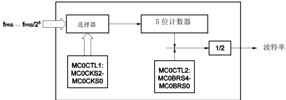
图 17-2. 波特率发生器的框图
