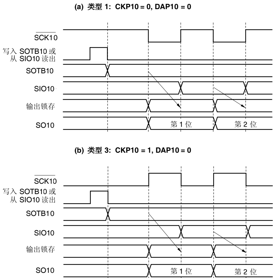
图 15-8. 起始位的输出操作(1/2)
