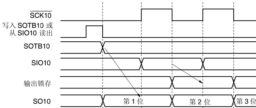
(d) 类型 4: CKP10 = 1, DAP10 = 1
