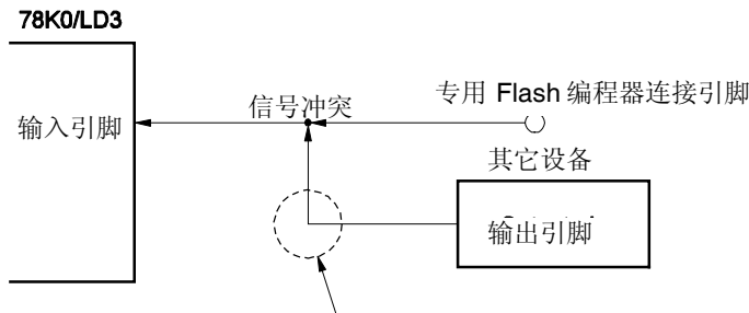
图 26-8. 信号冲突（串行接口的输入引脚）
