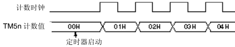
图 7-16. 8 位定时器计数器 5n 启动时序
