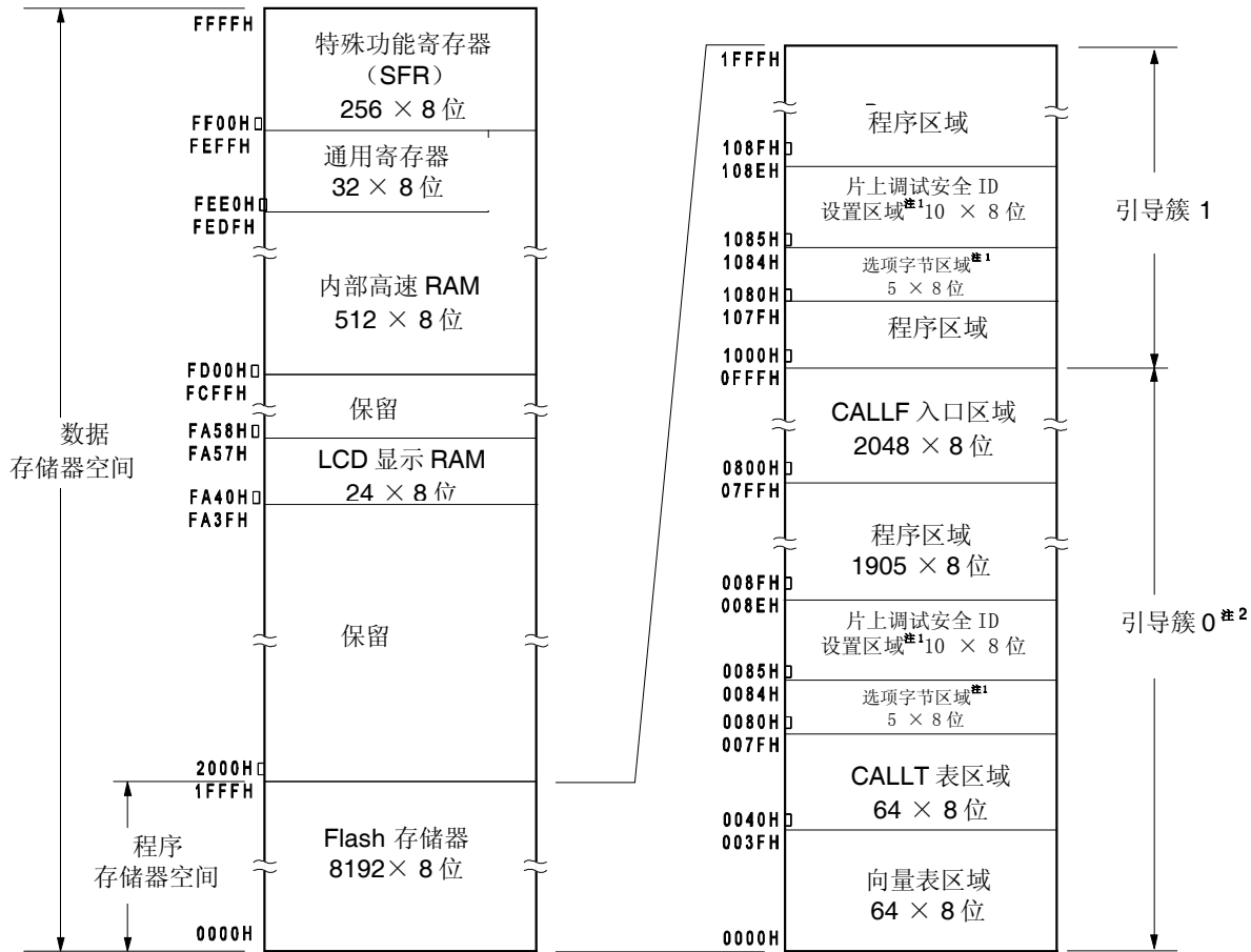
图 3-1. 存储器映射图(μPD78F0420, 78F0430)
