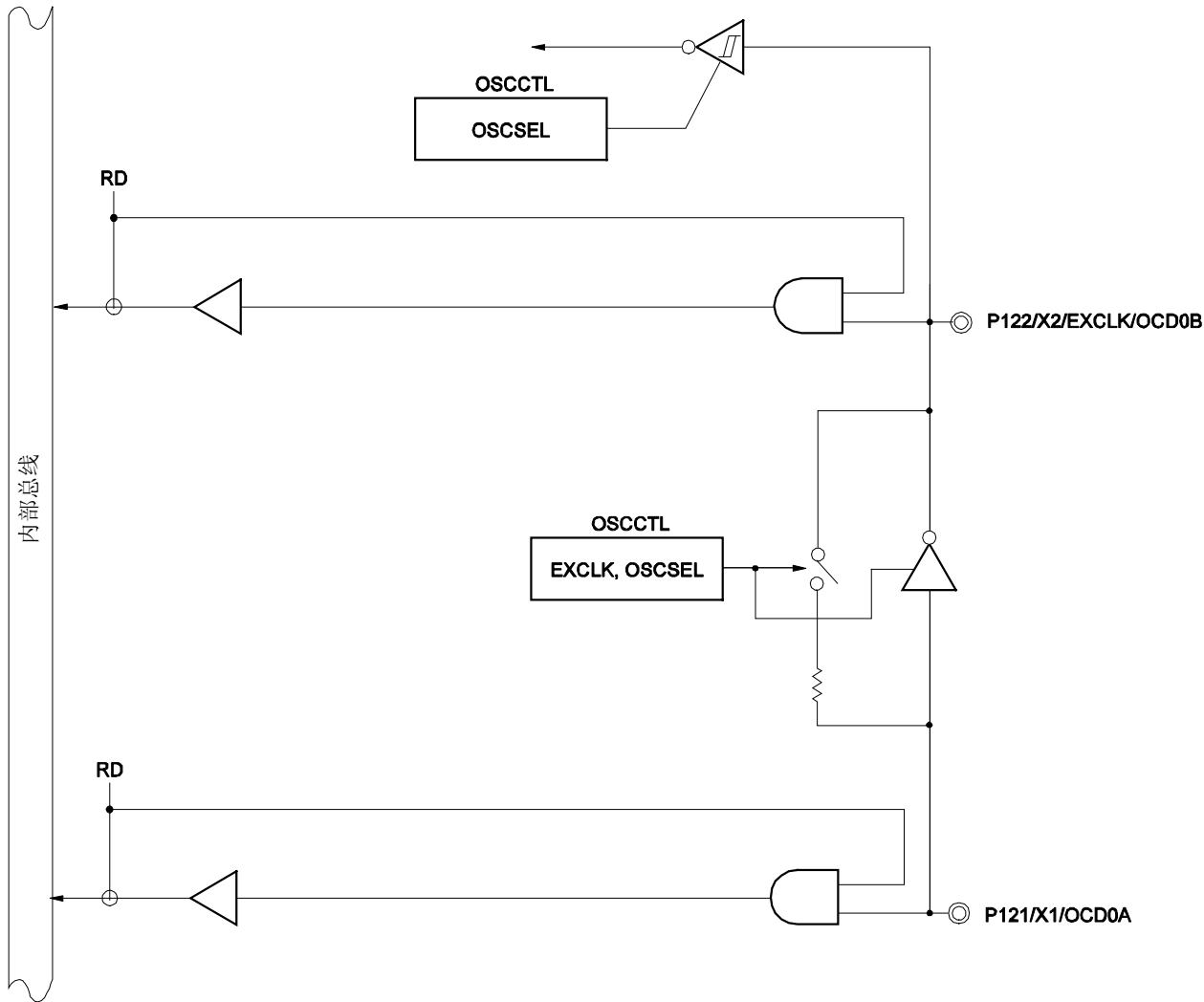
图 4-16. P121 和 P122 的框图
