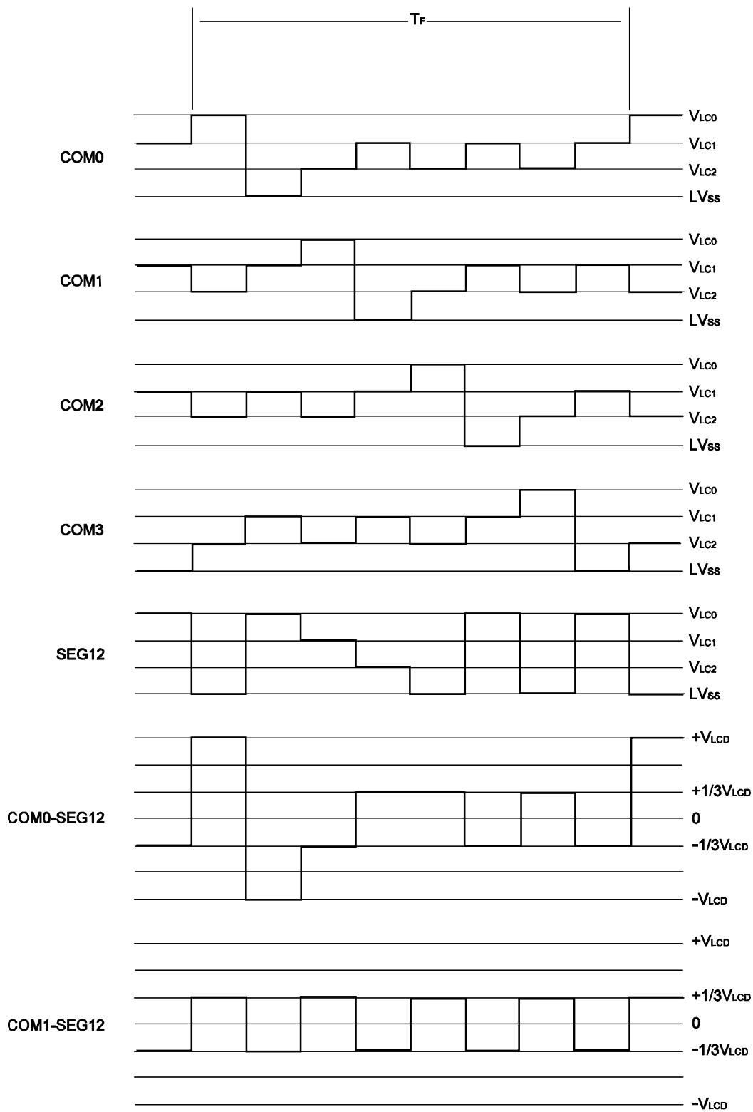
图 16-22. 4 分时分 LCD 驱动波形举例(1/3 偏压方式)
