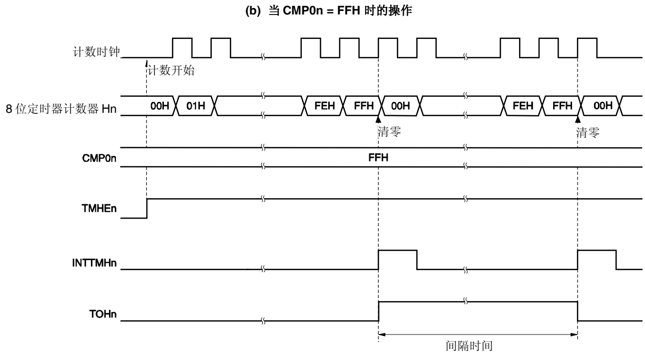
图 8-12. 间隔定时器/方波输出操作时序(2/2)
