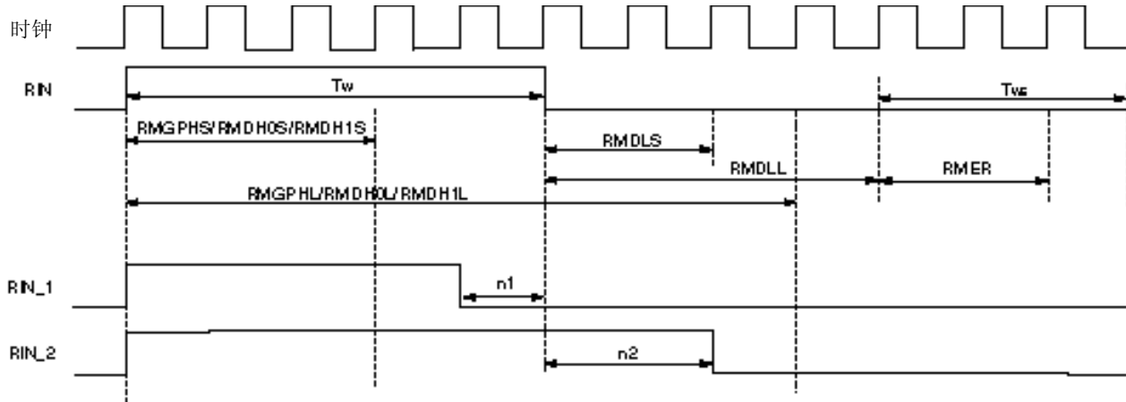
图 18-8. 设置示例(n1 = 1, n2 = 2)
