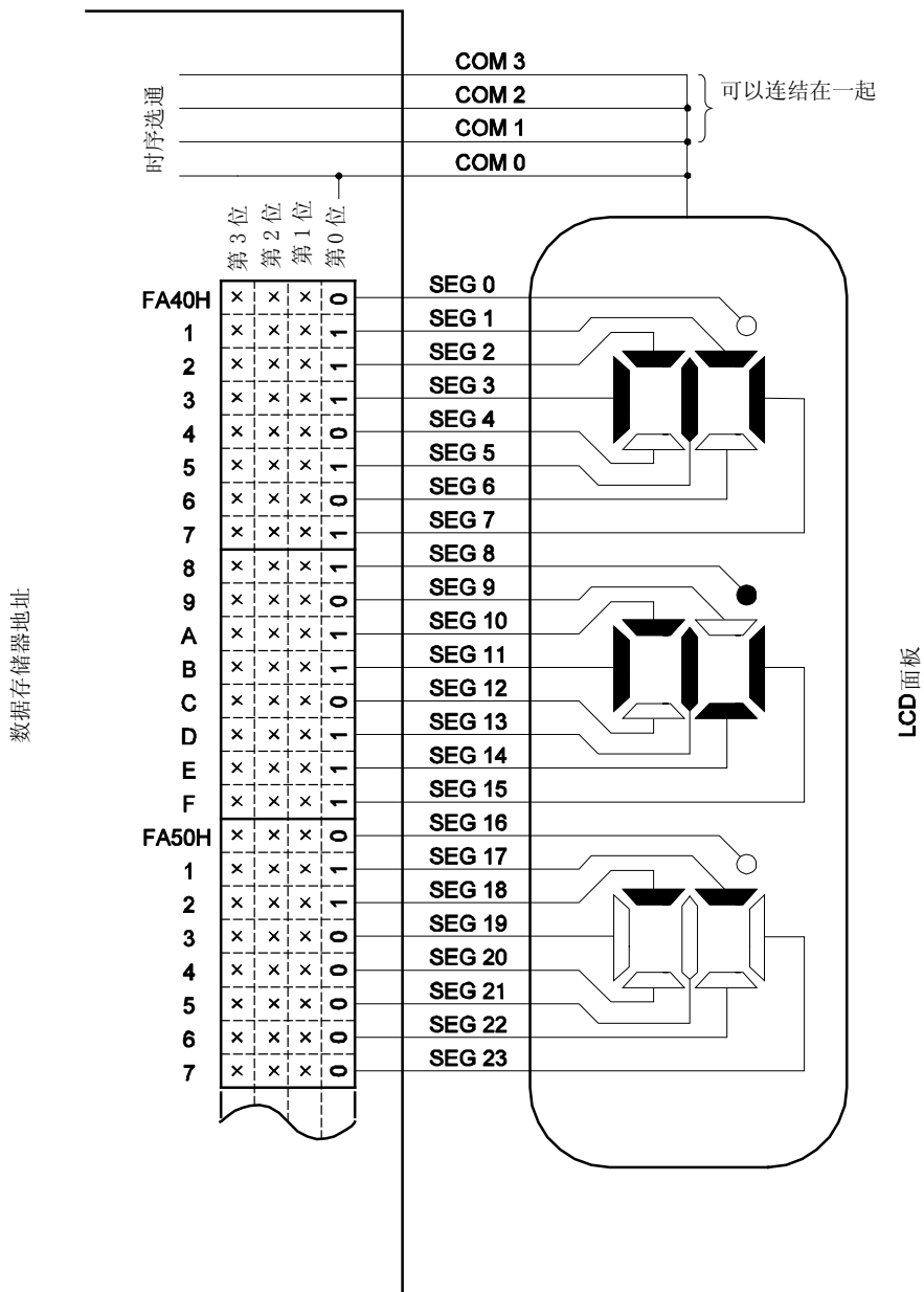
图 16-11. 静态 LCD 面板连接举例
