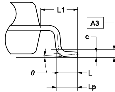
引脚端详图
