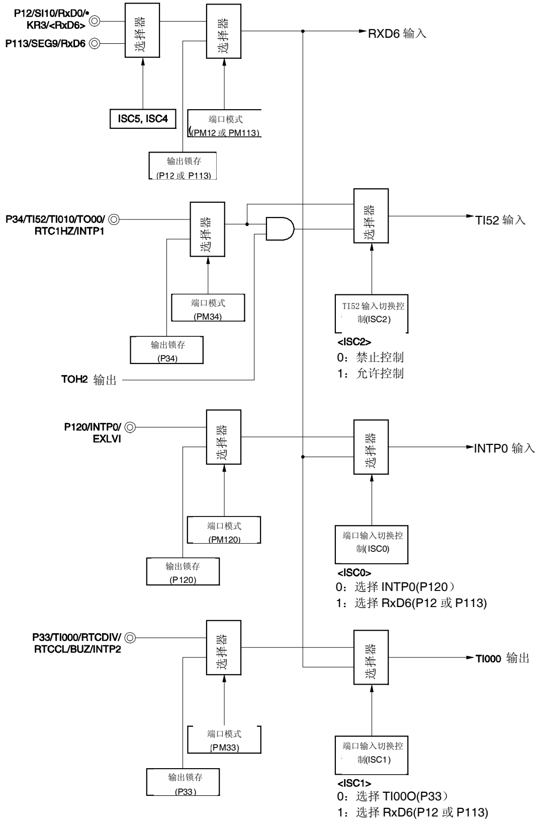
图 14-3. LIN 接收操作的端口配置
