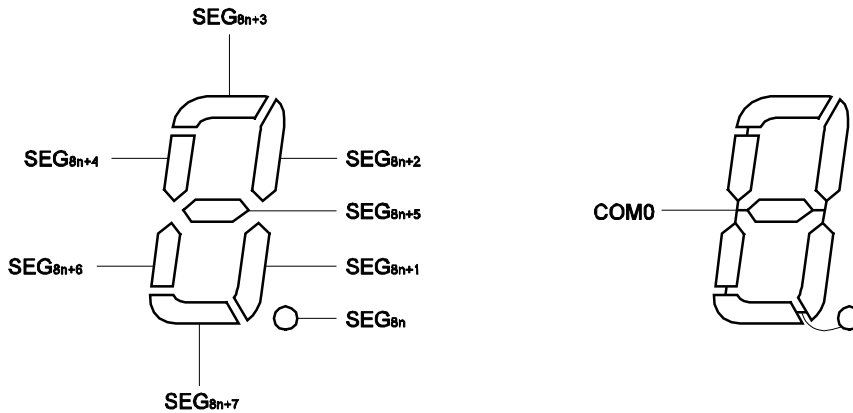
图 16-10. 静态 LCD 显示模式和电极连接
