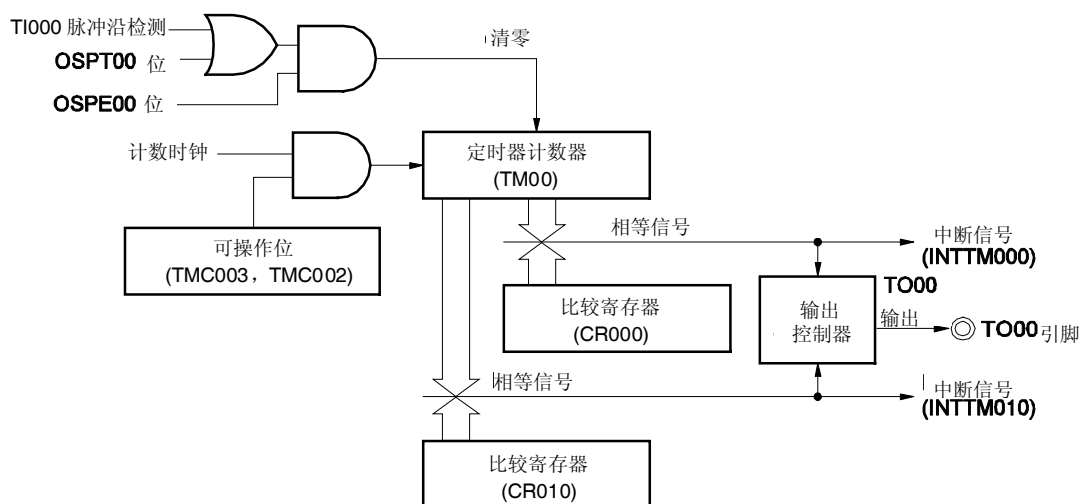
图 6-44. 单脉冲输出操作的框图
