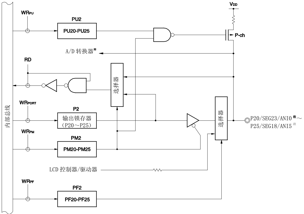
图 4-5. P20~P25 的框图
