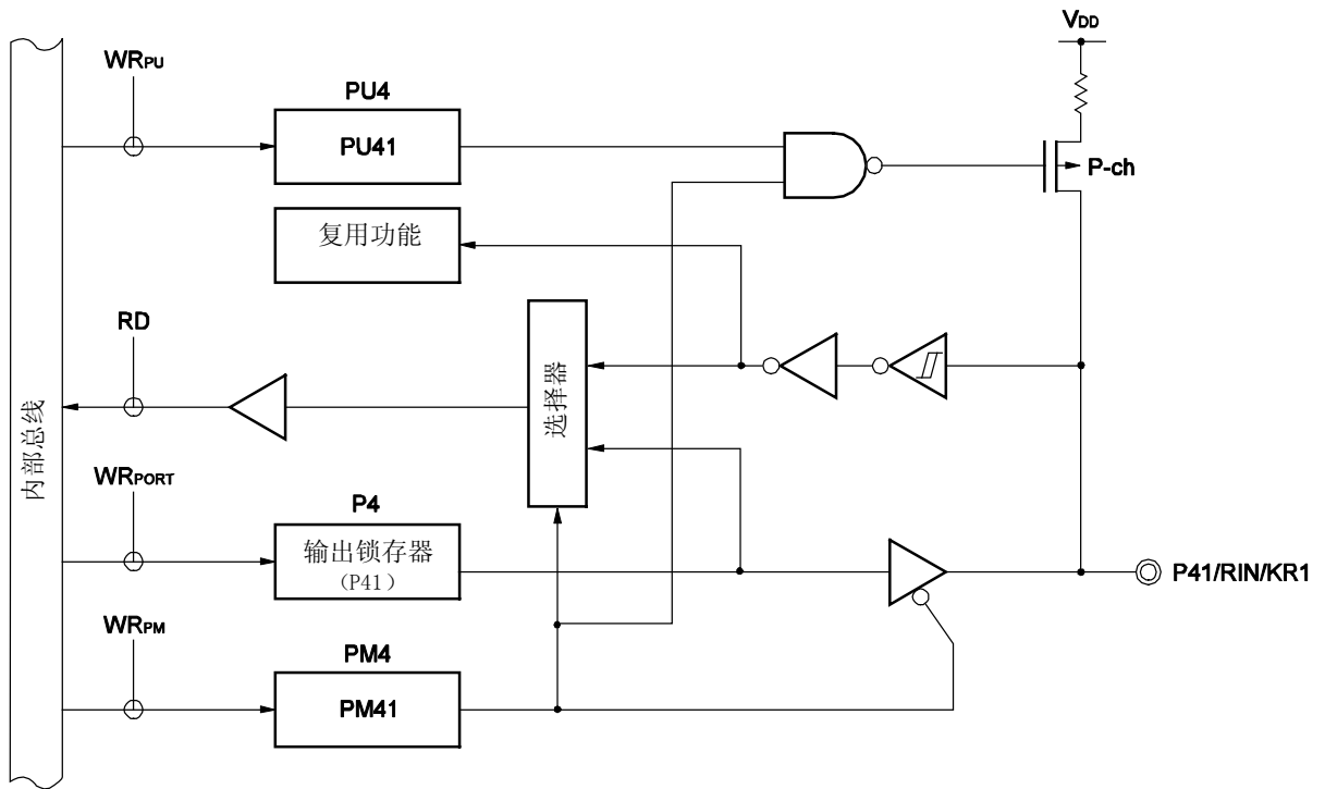
图 4-9. P41 的框图
