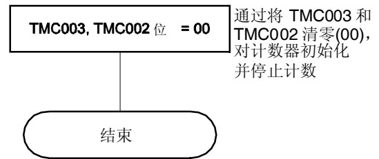
<3> 计数操作停止流程
