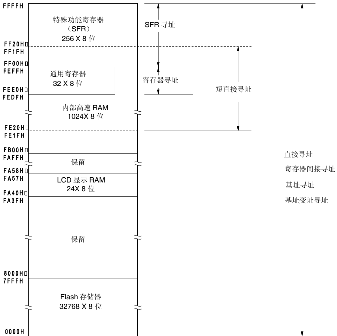
图 3-8. 数据存储器和寻址方式的对应关系( \mu PD78F0423, 78F0433)
