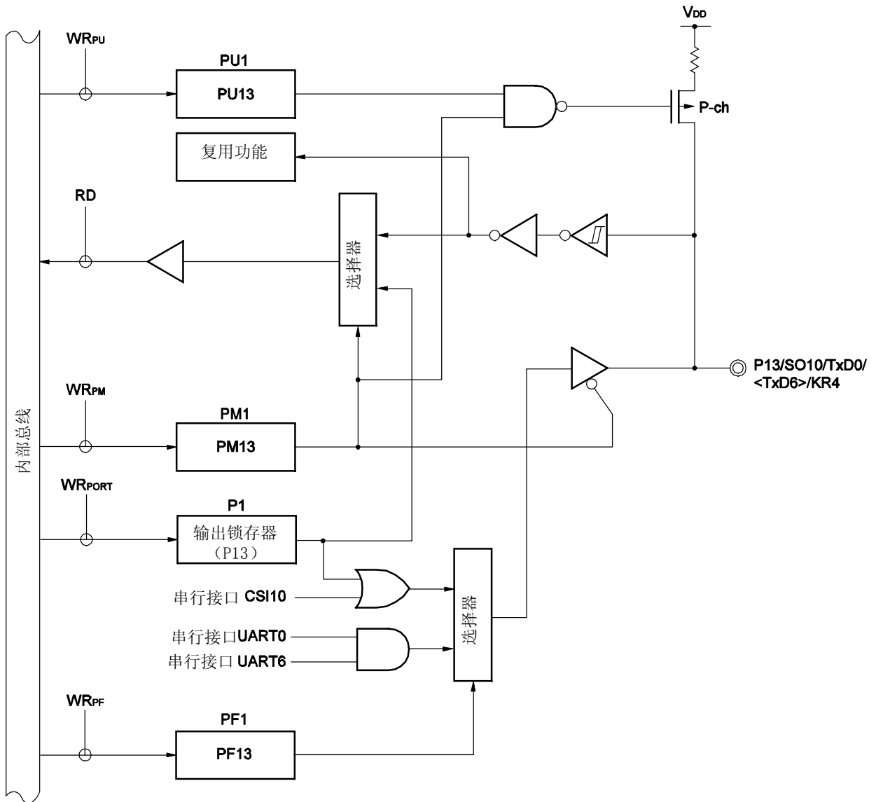
图 4-4. P13 的框图
