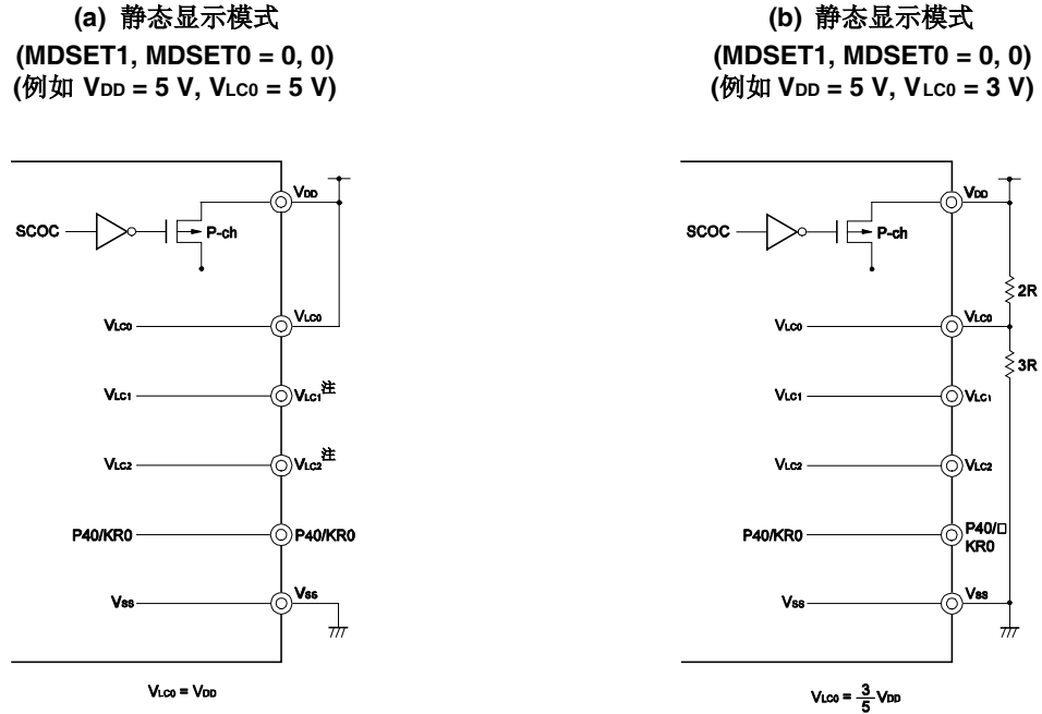
图 16-24. LCD 驱动电压连接举例 (外部电阻分压模式) (1/2)
