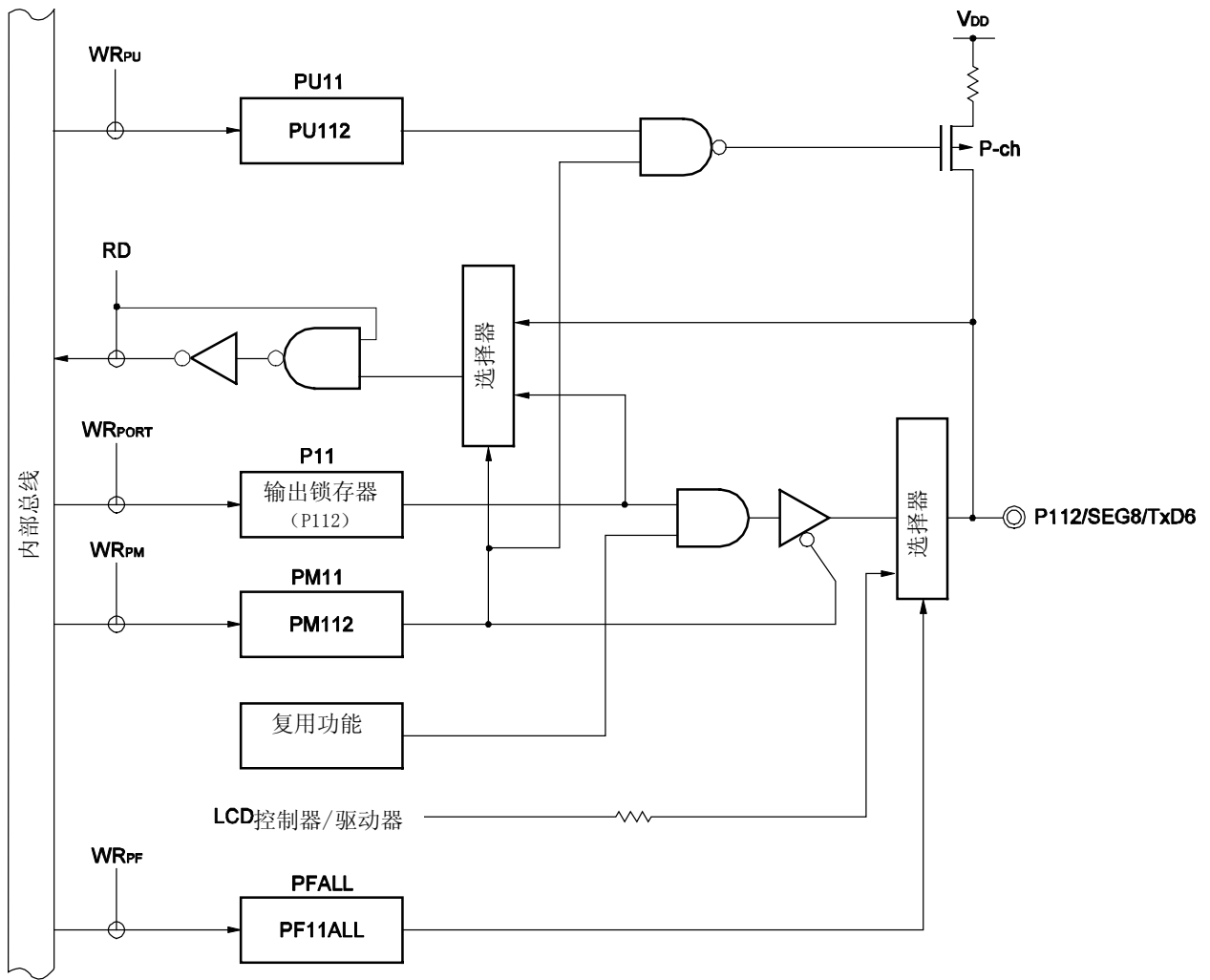
图 4-13. P112 的框图
