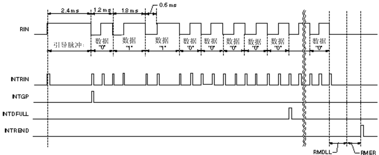
图 18-6. 类型 A 数据格式示例
