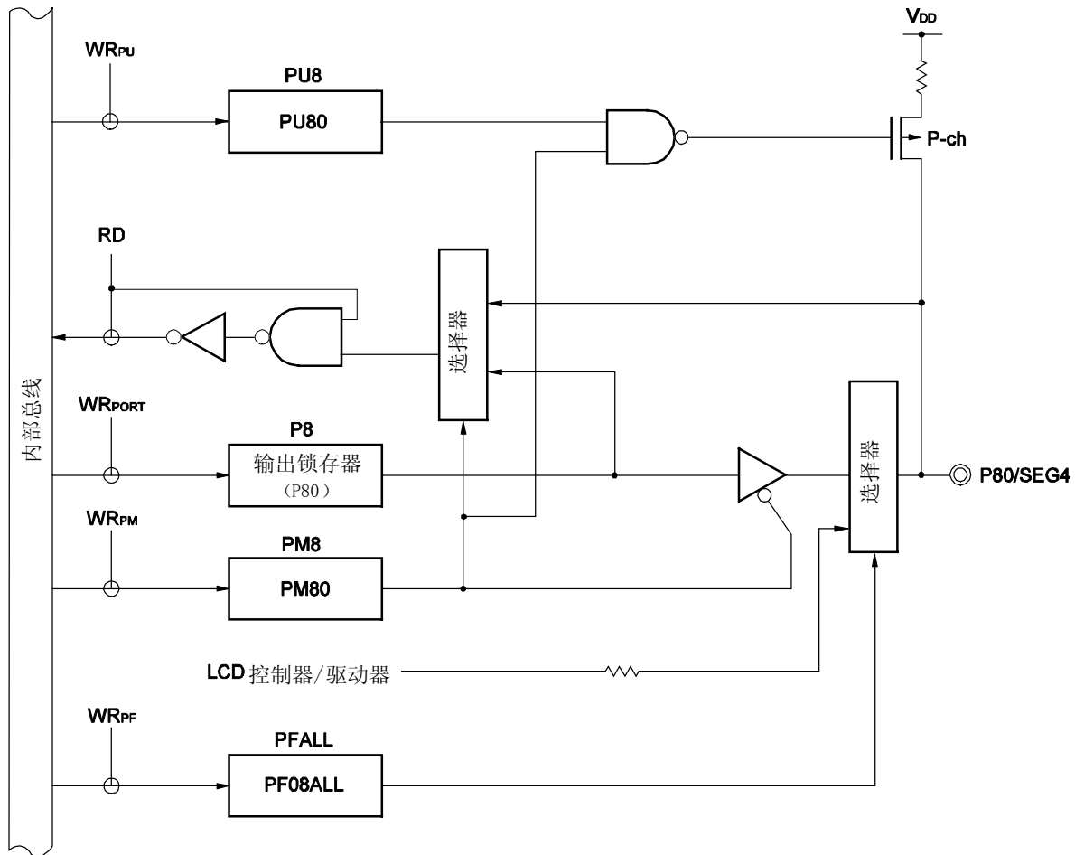
图 4-10. P80 的框图
