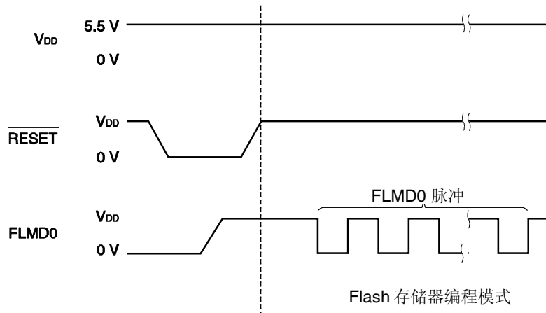
图 26-12. Flash 存储器编程模式
