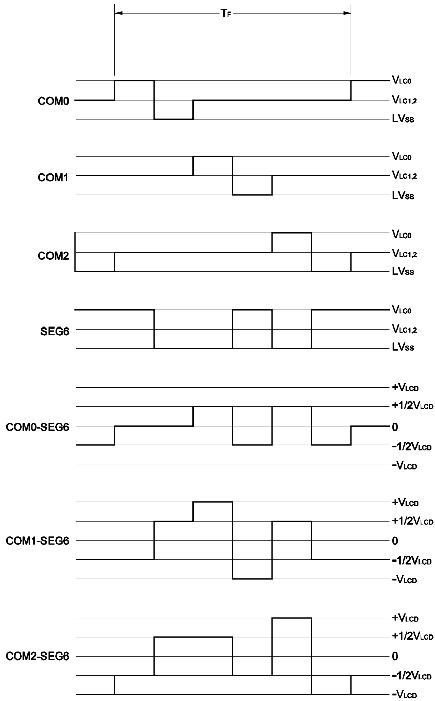
图 16-18. 3 分时 LCD 驱动波形举例(1/2 偏压方式)
