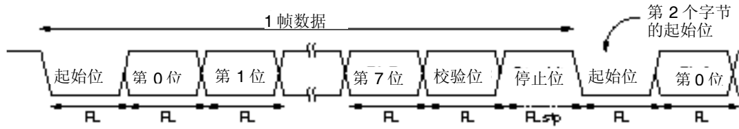
图 14-28. 连续发送期间数据帧的宽度
