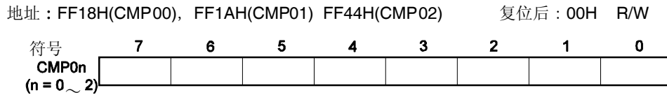
图 8-4. 8 位定时器 H 比较寄存器 0n (CMP0n)的格式
