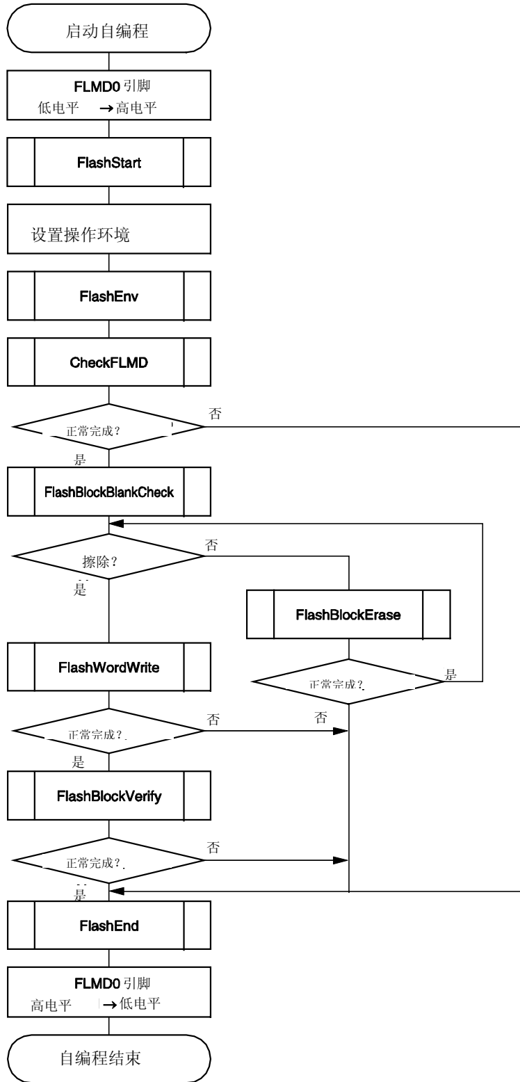
图 26-14. 自编程流程(改写 Flash 存储器)
