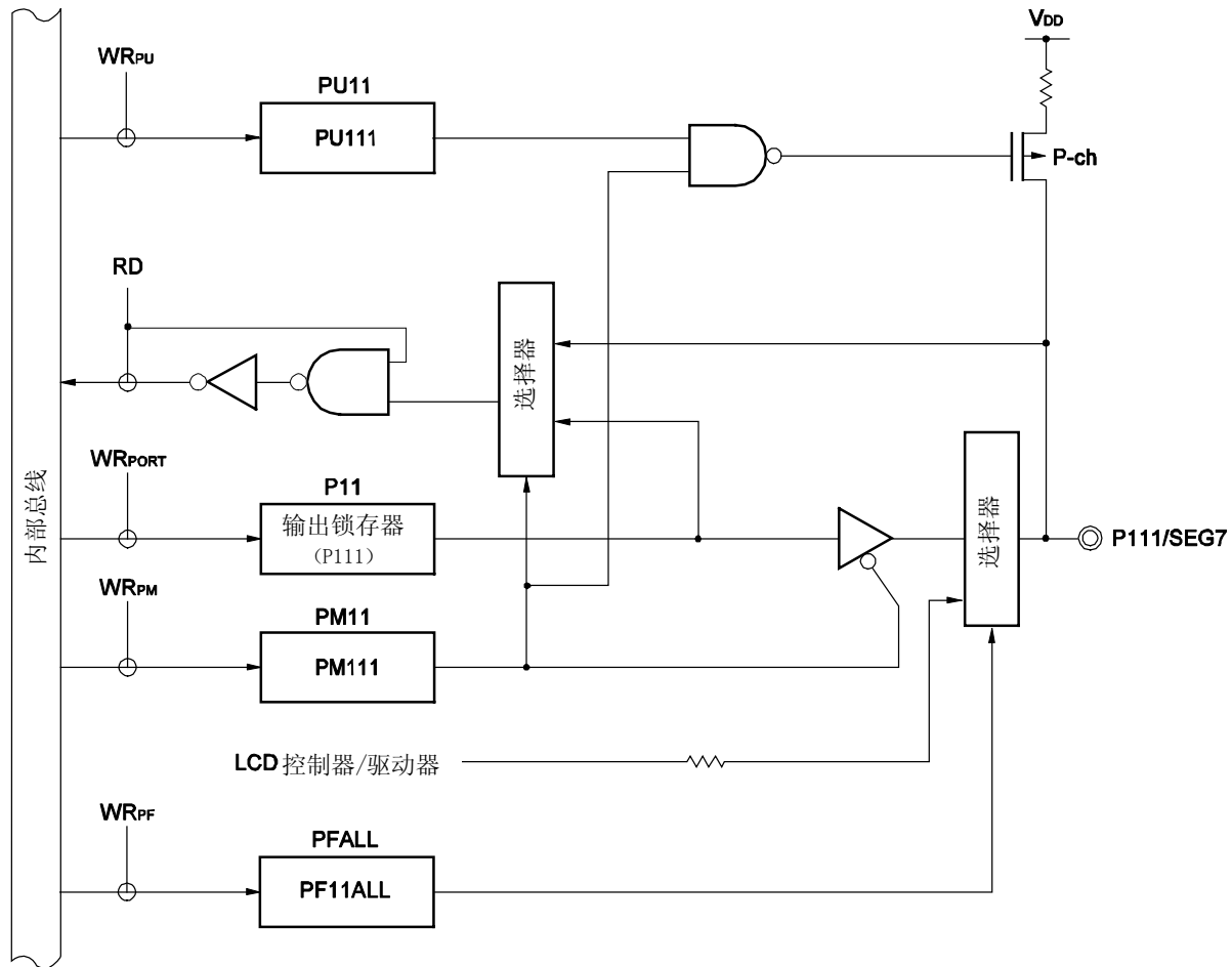
图 4-12. P111 的框图
