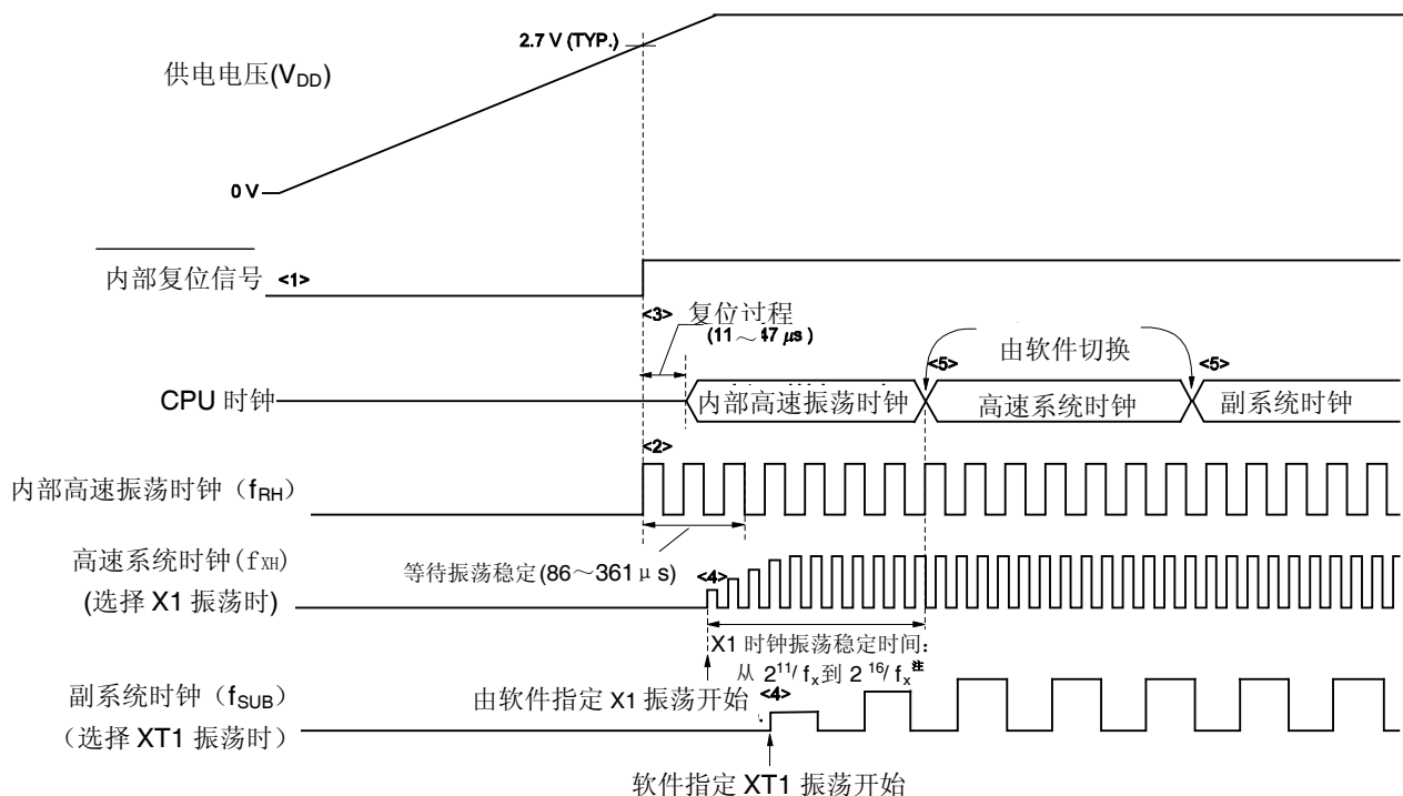
图 5-14. 上电时的时钟发生器操作 (设置 2.7 V/1.59 V POC 模式 (选项字节: POCMODE = 1))
