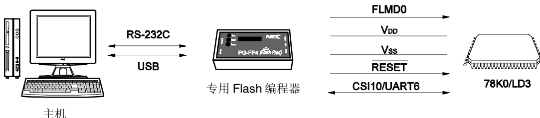
图 26-4. Flash 存储器编程环境
