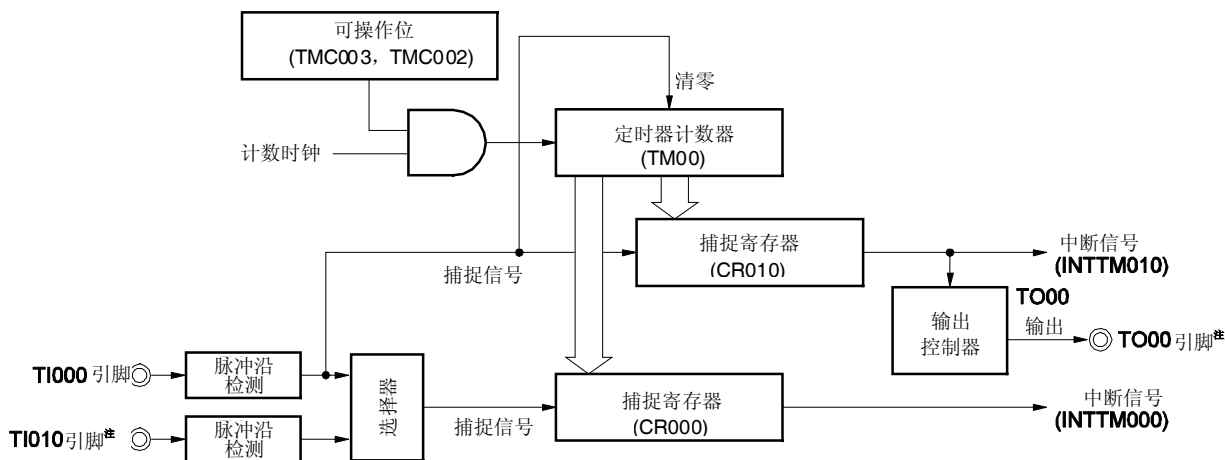
图 6-29. 清零&启动模式(通过 TI000 引脚有效沿输入进入)的框图 (CR000: 捕捉 寄存器, CR010: 捕捉 寄存器)
