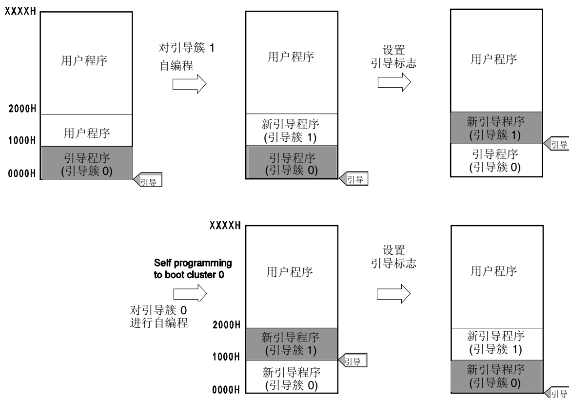
图 26-15. 引导交换功能
