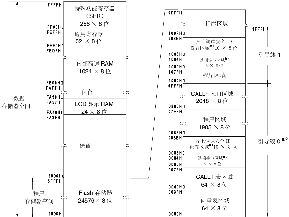
图 3-3. 存储器映射图( \mu PD78F0422, 78F0432)
