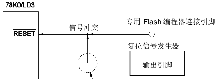
图 26-10. 信号冲突 (RESET 引脚)
