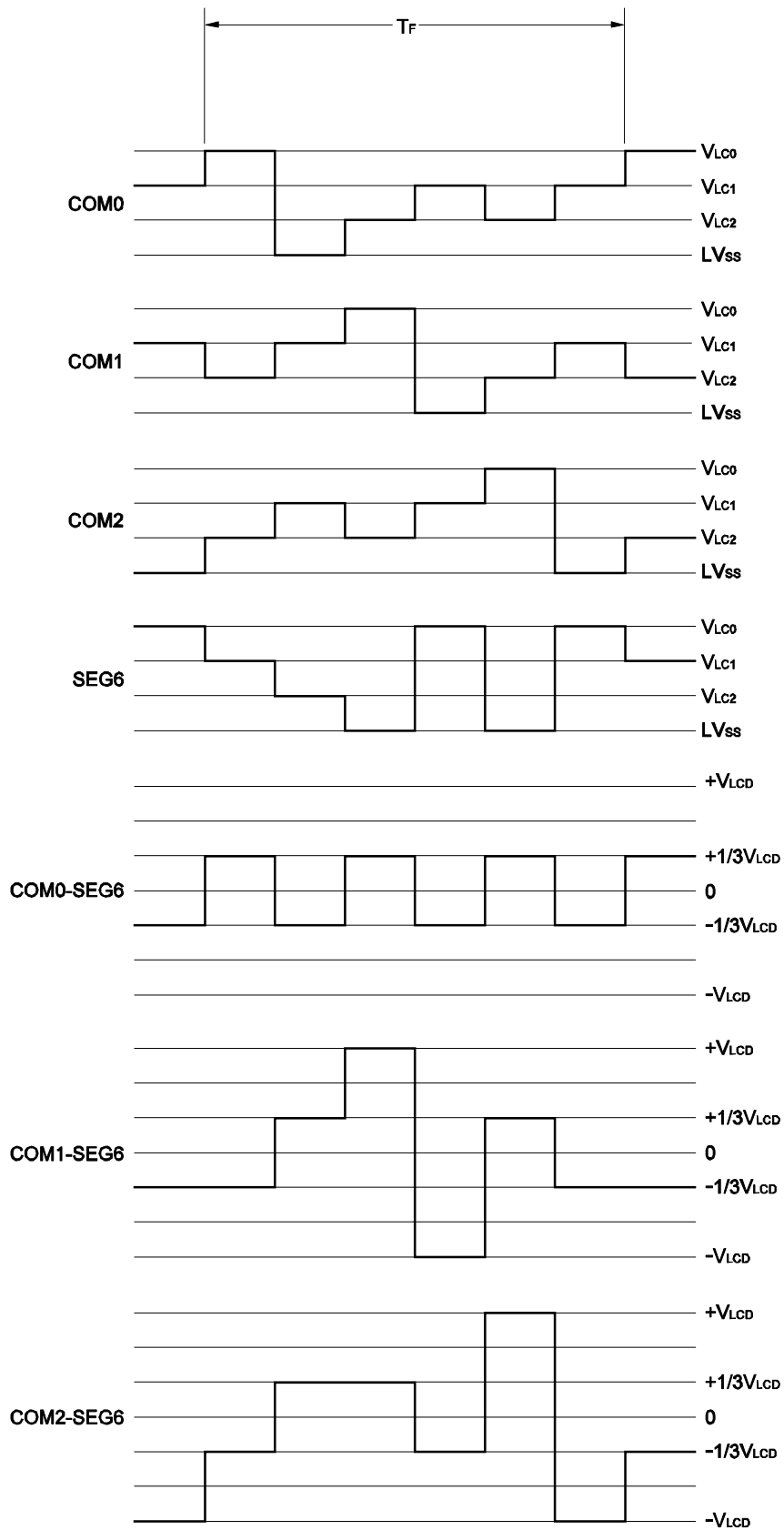
图 16-19. 3 分时 LCD 驱动波形举例(1/3 偏压方式)
