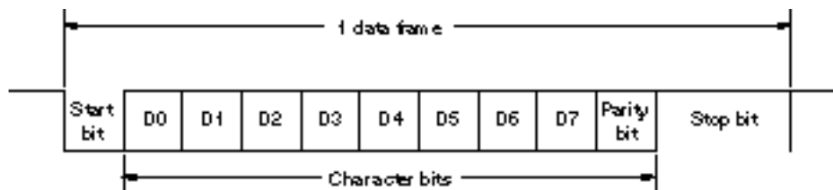
图 13-7. 正常 UART 发送/接收数据的格式
