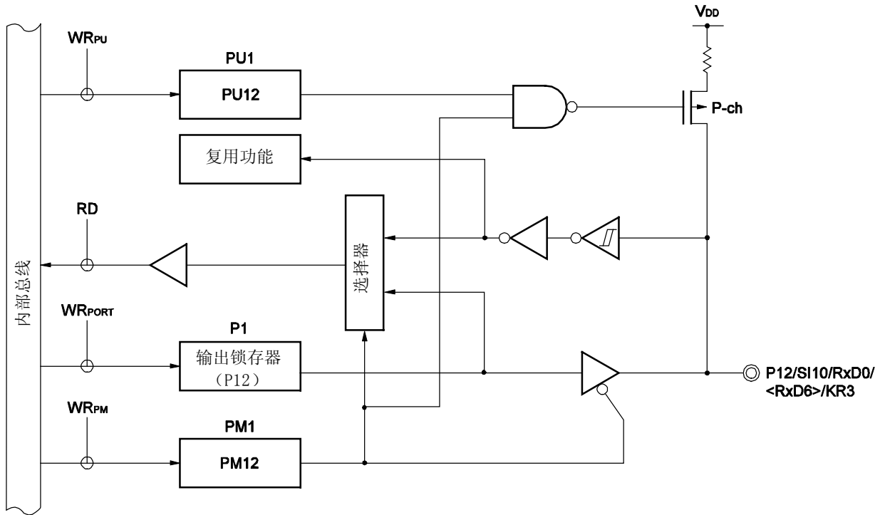
图 4-3. P12 的框图
