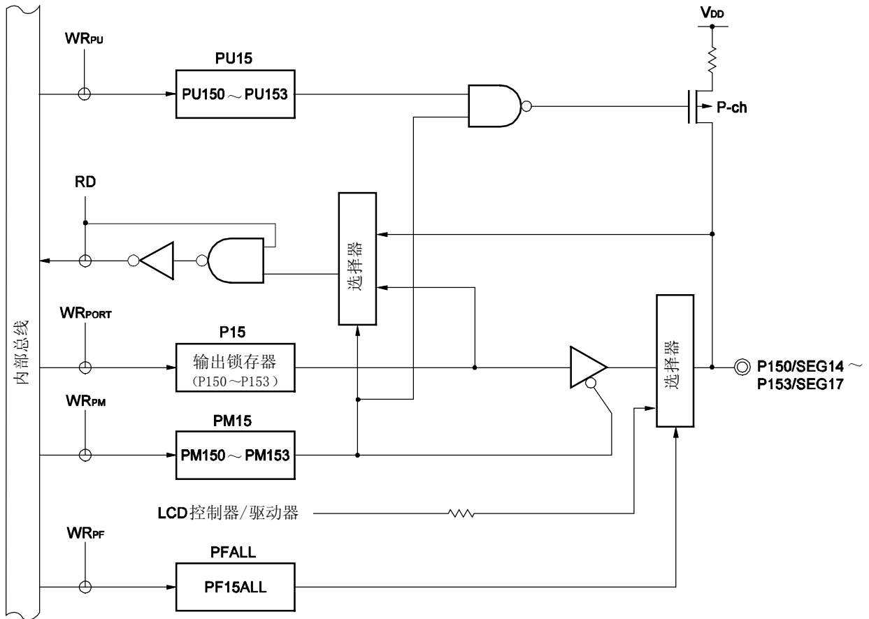
图 4-19. P150~P153 的框图
