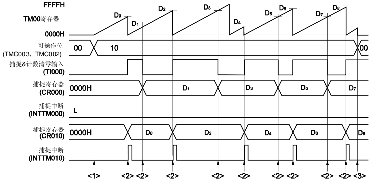
(b) 清零&启动模式(通过 TI000 引脚有效沿进入)示例
