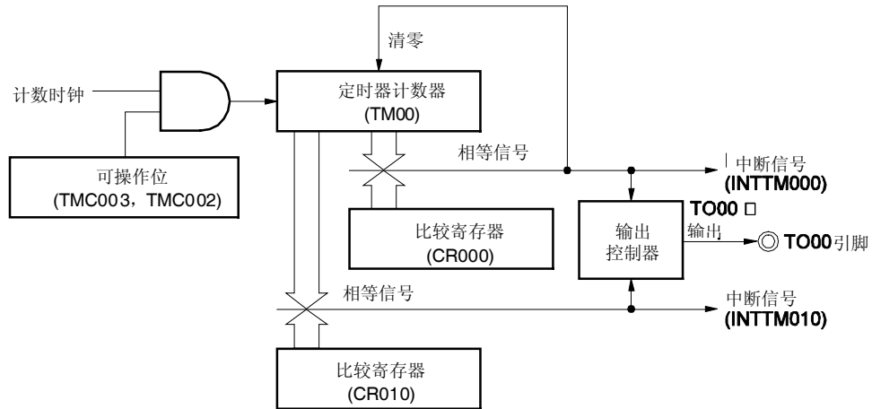
图 6-41. PPG 输出操作的框图
