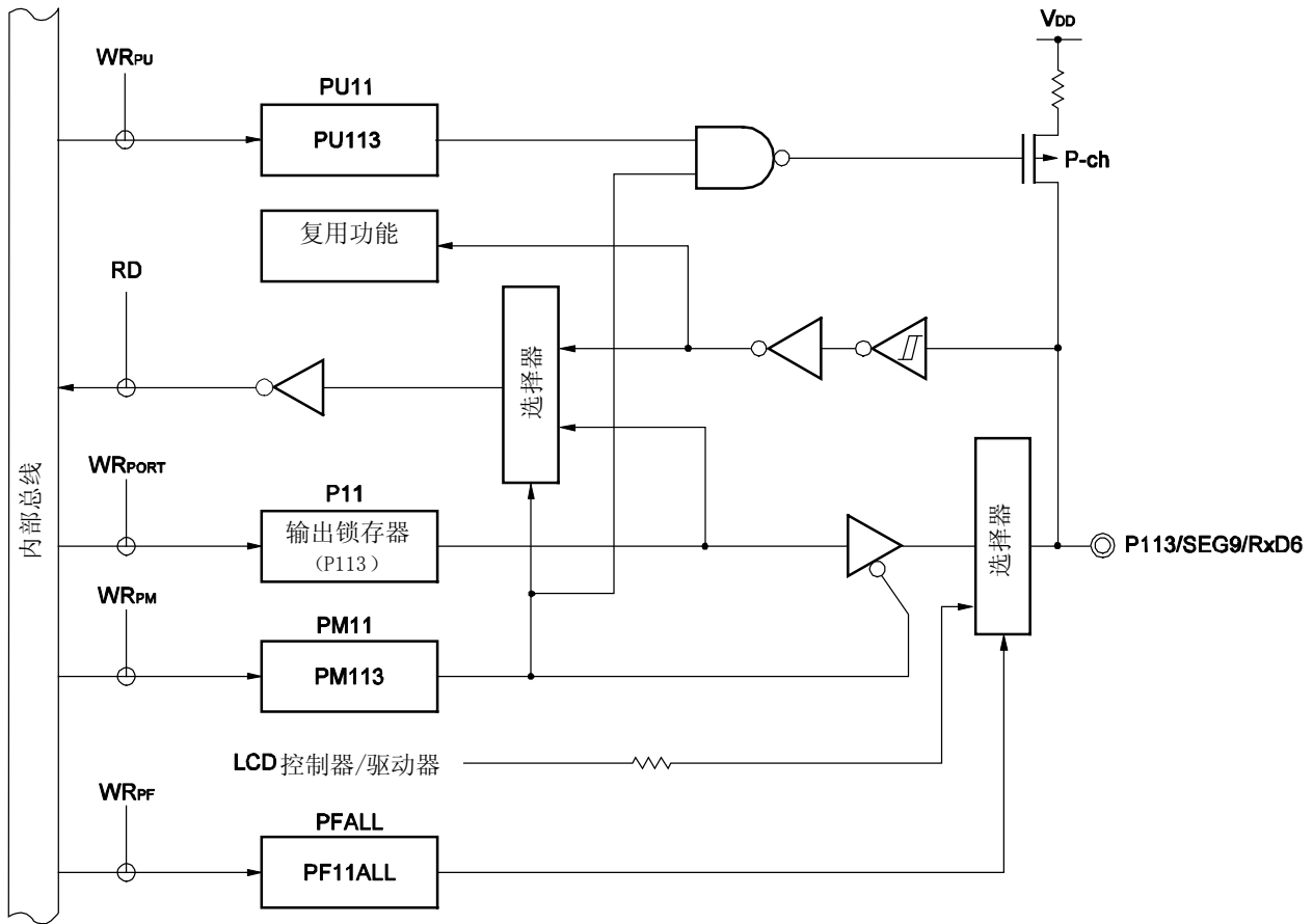
图 4-14. P113 的框图
