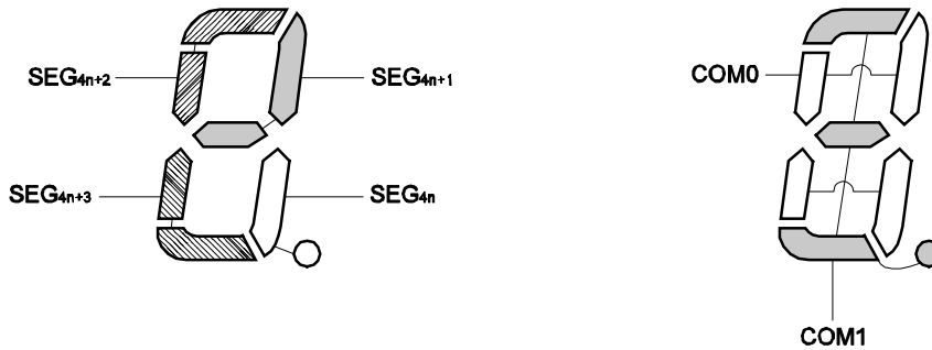
图 16-13. 2 分时 LCD 显示模式和电极连接
