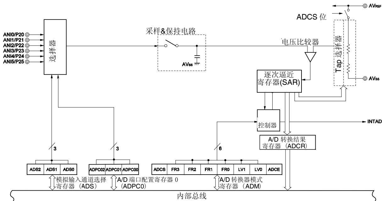
图 12-1. 10 位逐次逼近型 A/D 转换器的框图
