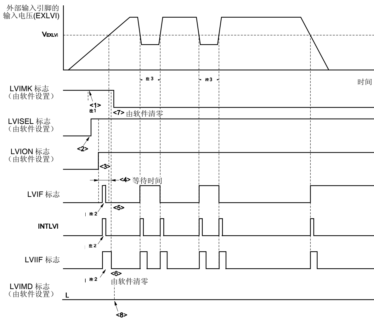
图 24-8. 低电压检测电路中断信号产生时序 (检测外部输入引脚的输入电压 (EXLVI) 等级)
