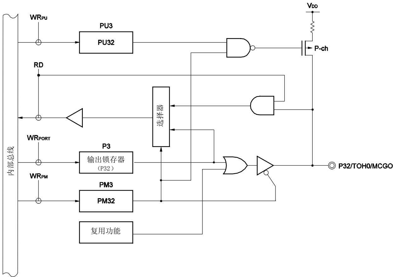
图 4-7. P32 的框图
