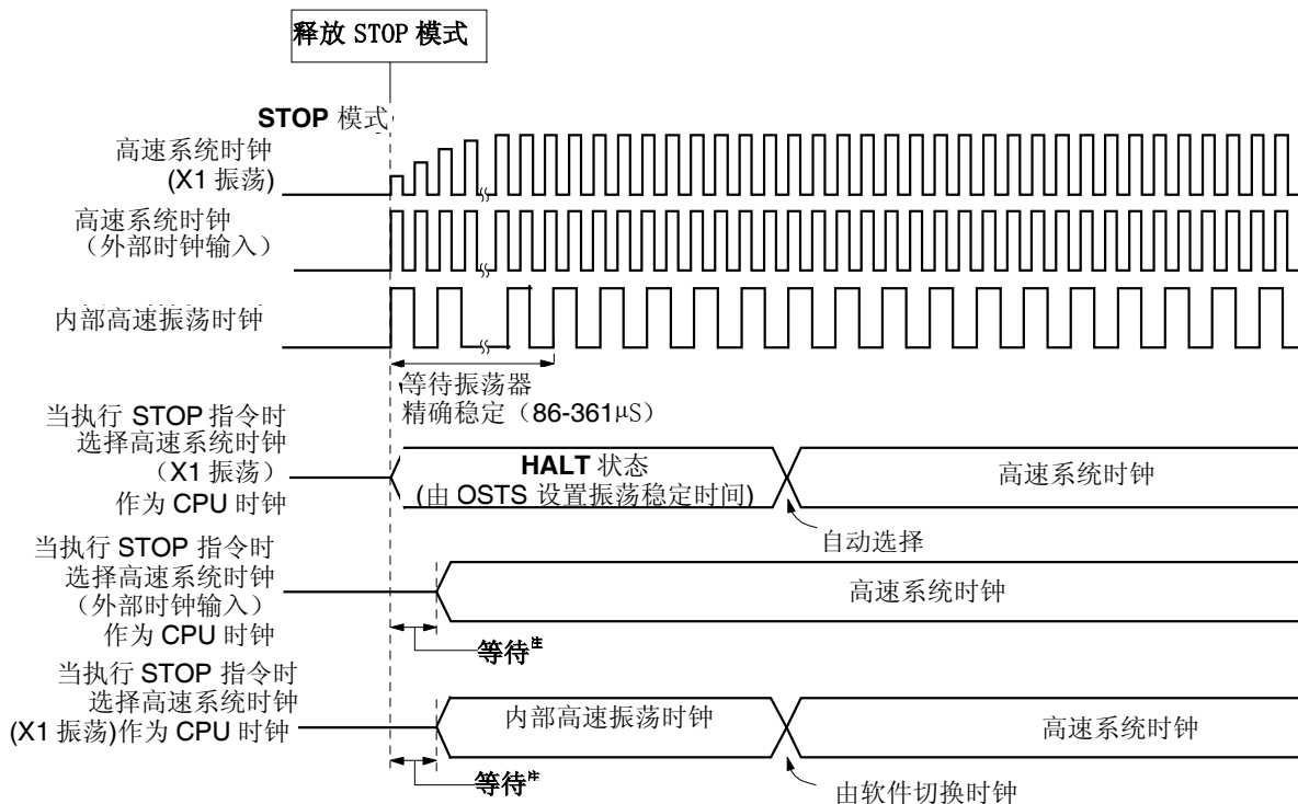
图 21-5. 释放 STOP 模式时的操作时序(当不可屏蔽中断发生时)
