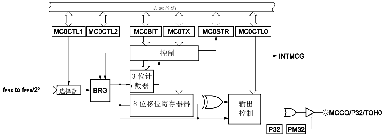
图 17-1. 曼彻斯特编码发生器的框图
