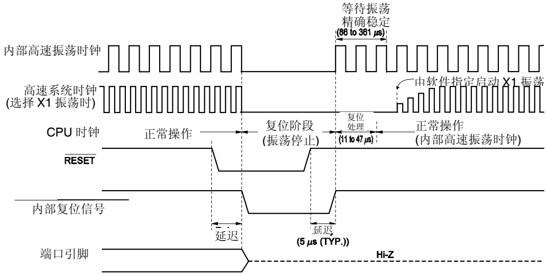
图 22-2. 输入引起的复位的时序
