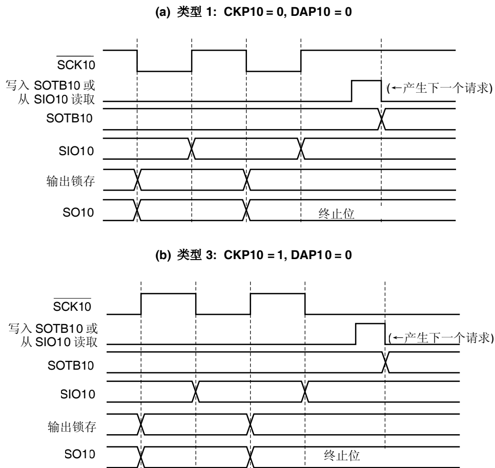
图 15-9. SO10 引脚的输出值 (终止位) (1/2)
