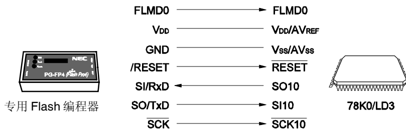
图 26-5. 专用 Flash 编程器的通信 (CSI10)
