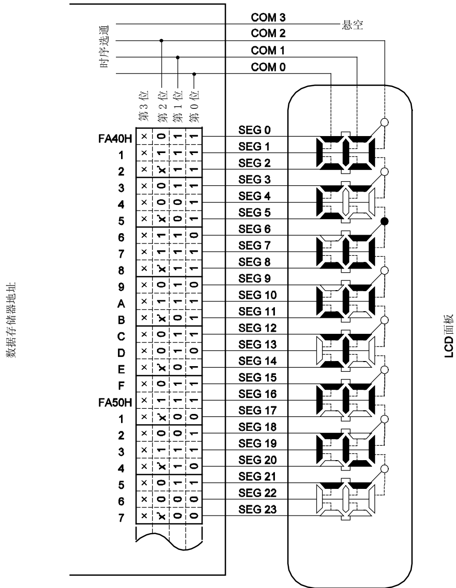
图 16-17. 3 分时 LCD 面板连接举例
