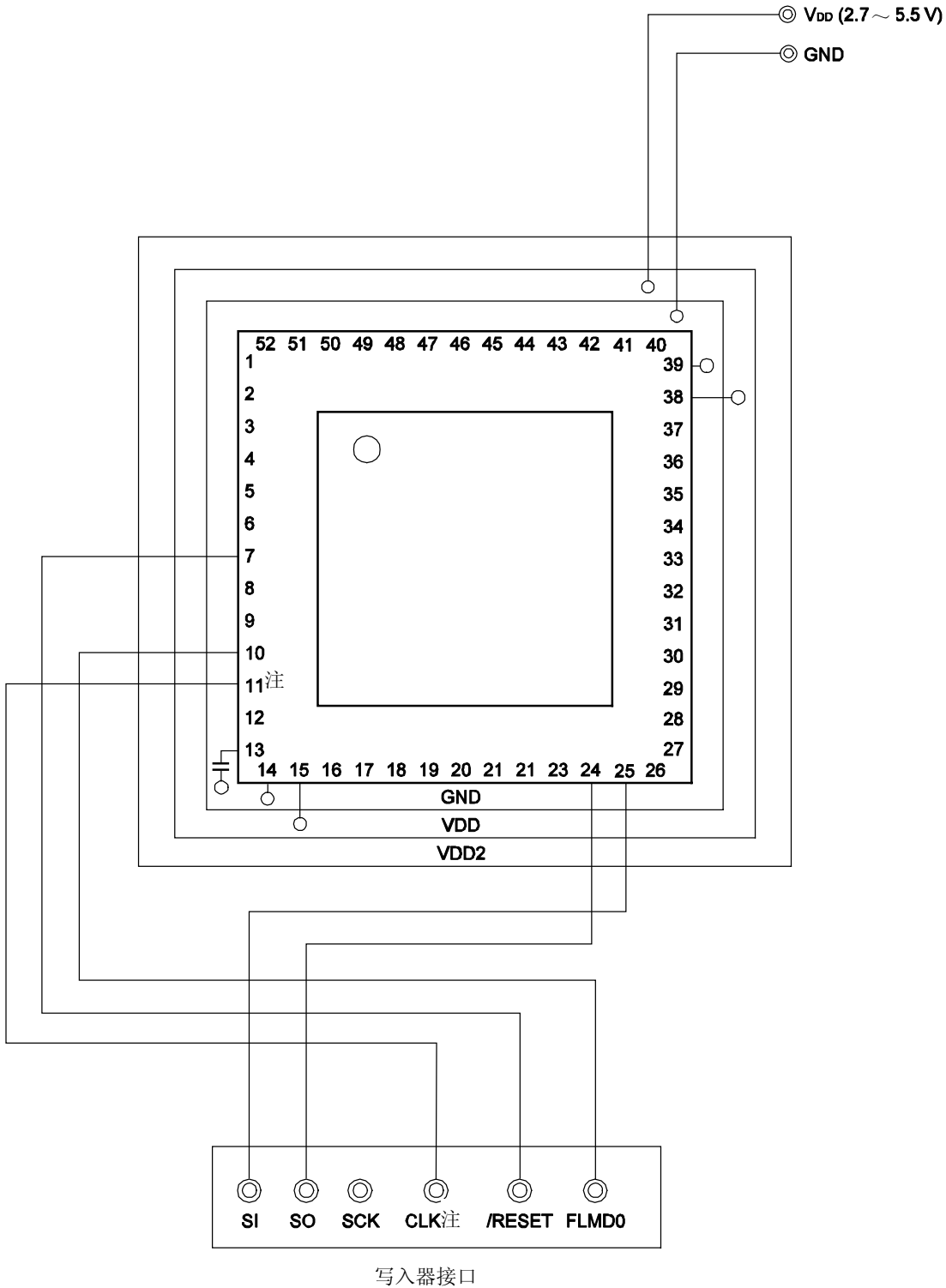
图 26-3. UART (UART6) 模式下使用适配器对 Flash 存储器进行写操作示例
