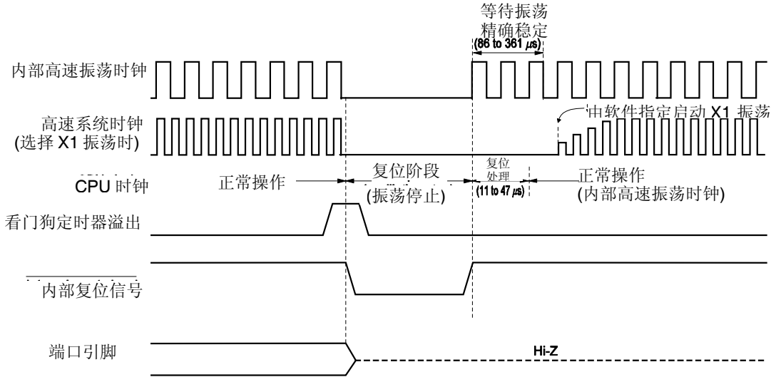
图 22-3. 看门狗定时器溢出引起的复位的时序
