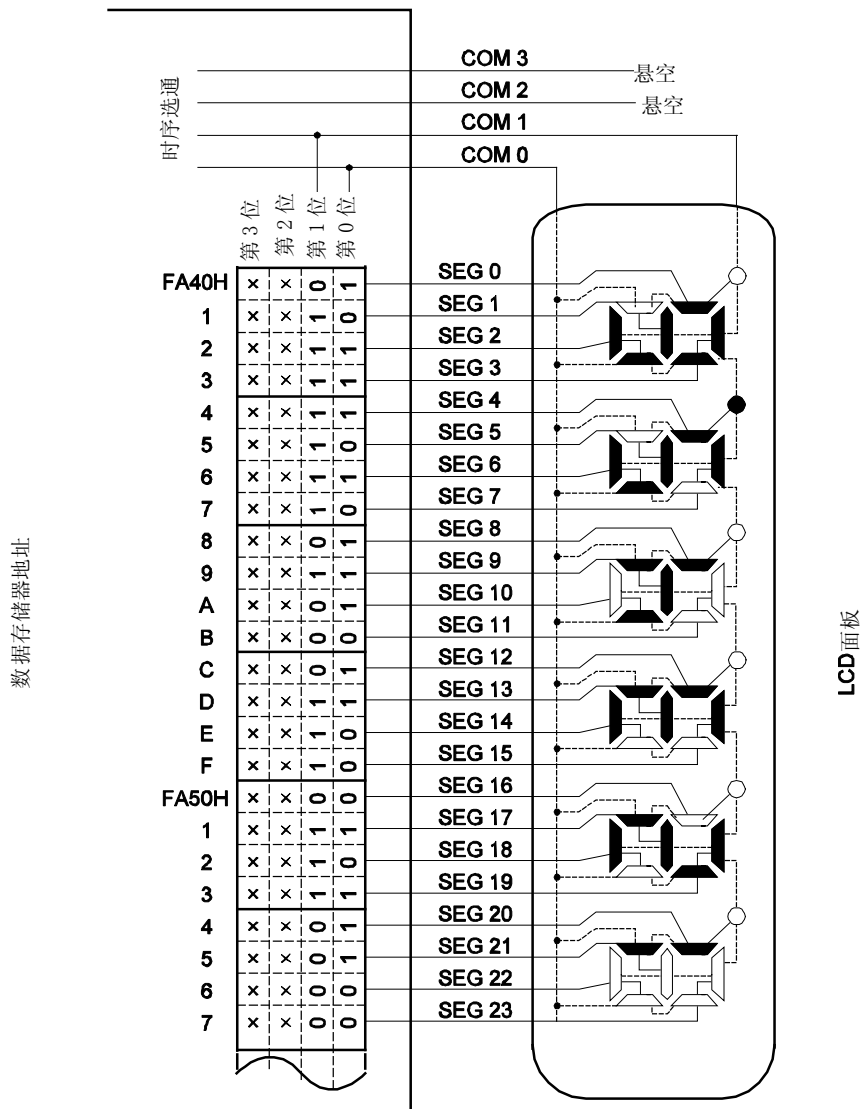
图 16-14. 2 分时 LCD 面板连接举例
