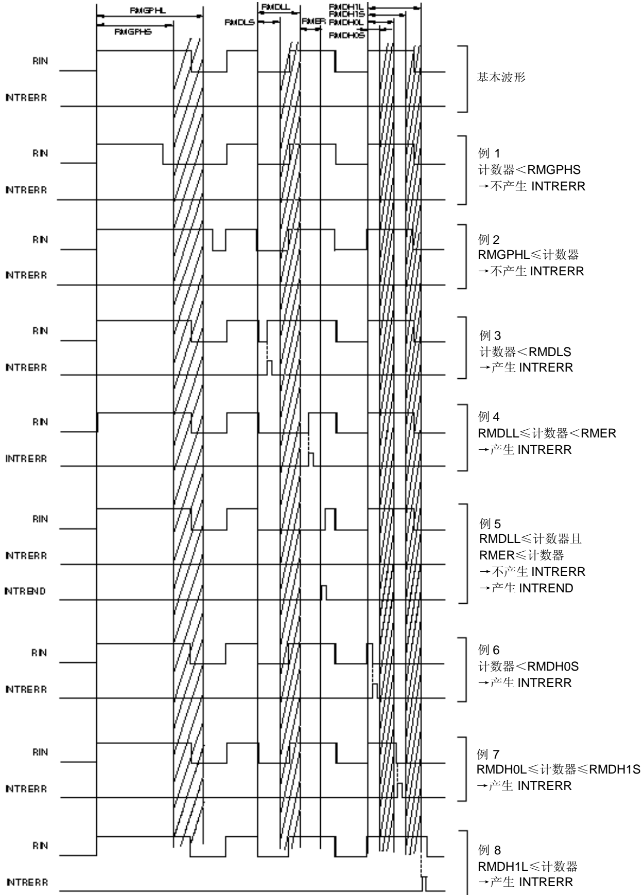
图 18-9. INTRERR 信号的发生时序
