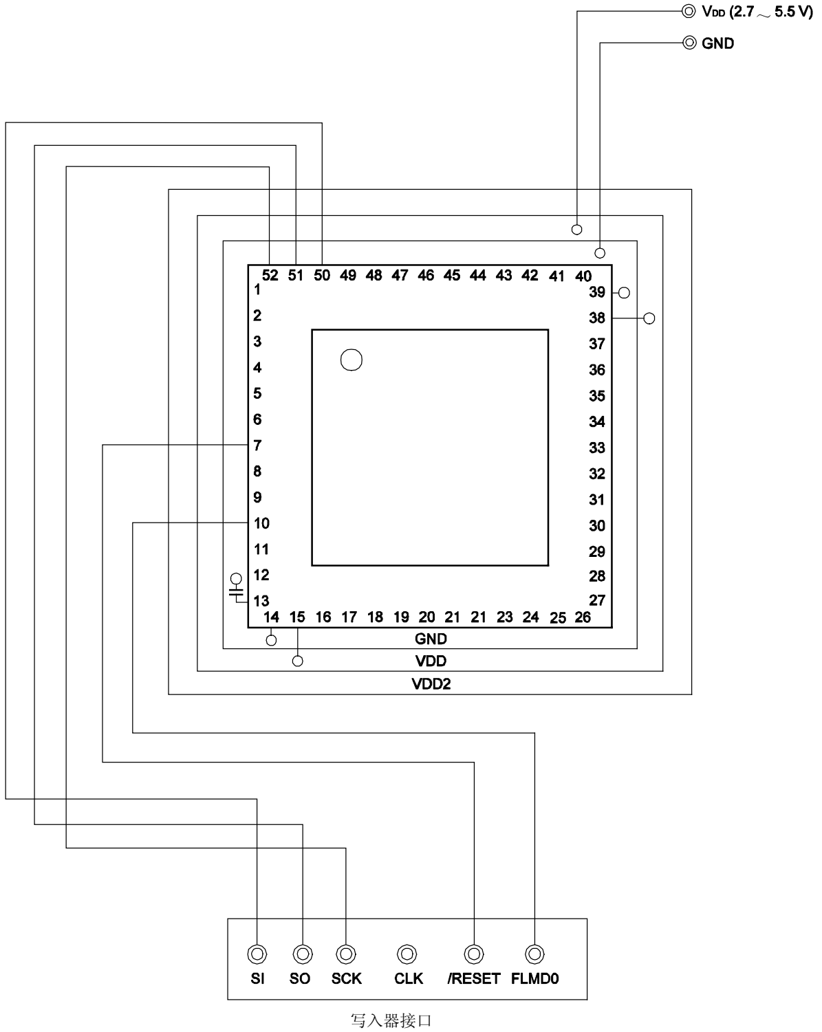
图 26-2. 3 线串行 I/O (CSI10) 模式下使用适配器对 Flash 存储器进行写操作示例
