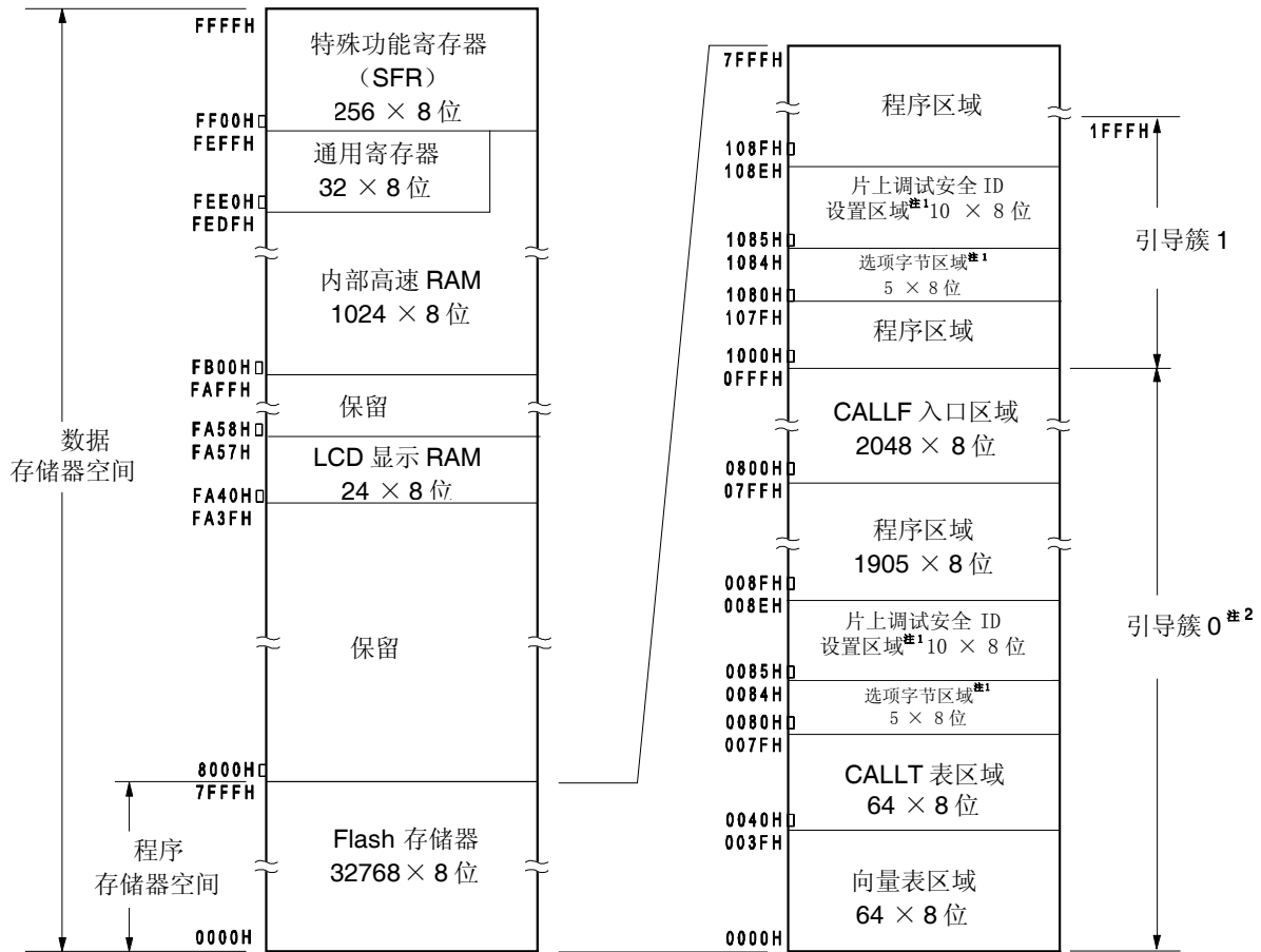
图 3-4. 存储器映射图(μPD78F0423, 78F0433)
