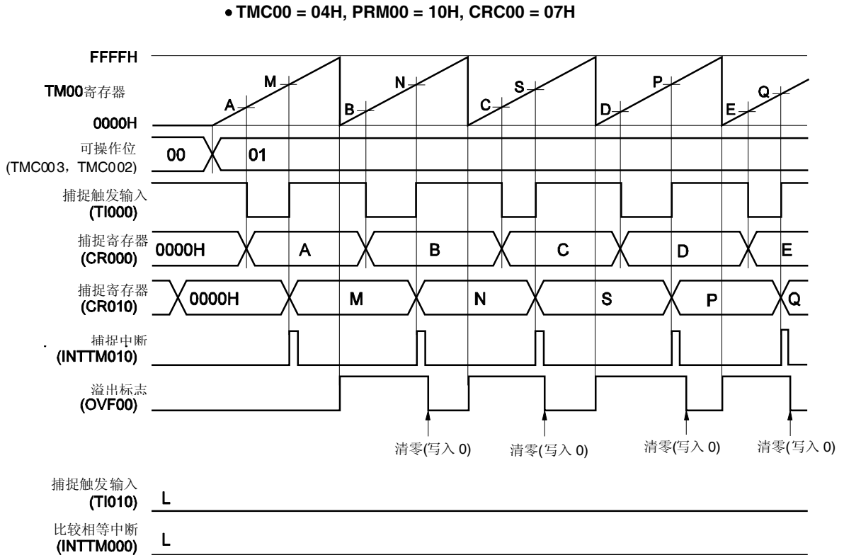
图 6-50. 脉冲宽度测量时序示例 (2)
