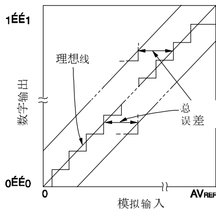
图 12-14. 总误差
