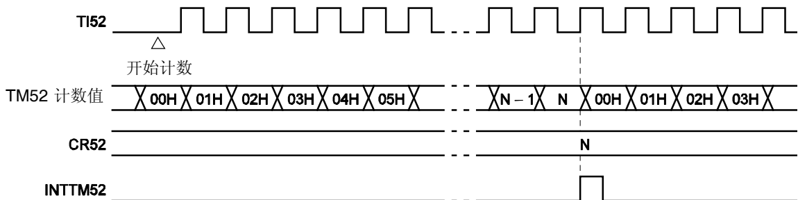
图 7-15. 外部事件计数器操作的时序 (规定上升沿有效)
