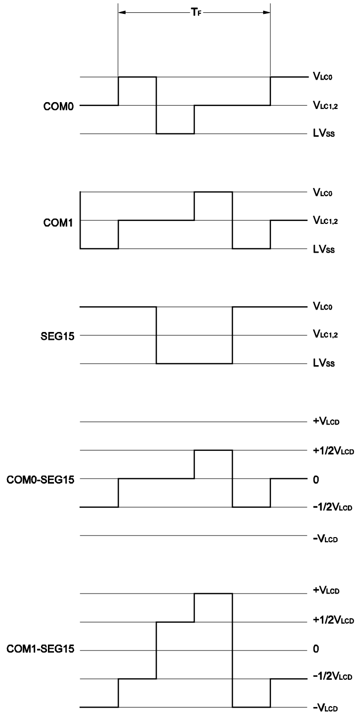
图 16-15. 2 分时 LCD 驱动波形举例(1/2 偏压方式)
