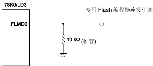
图 26-7. FLMD0 引脚连接示例
