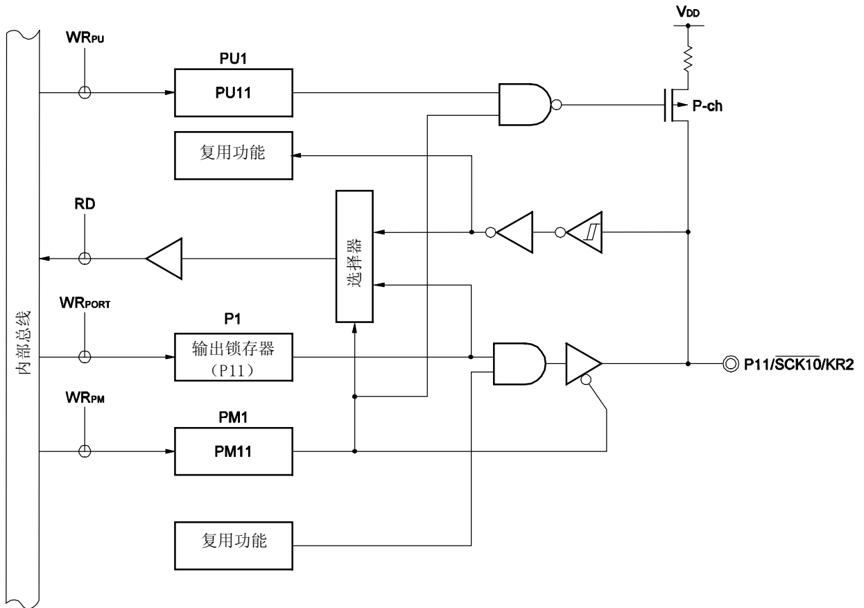
图 4-2. P11 的框图
