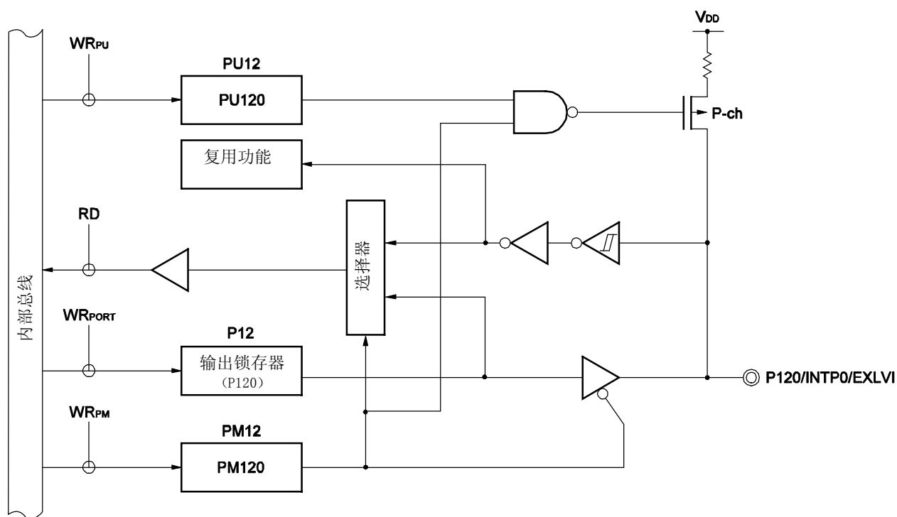
图 4-15. P120 的框图
