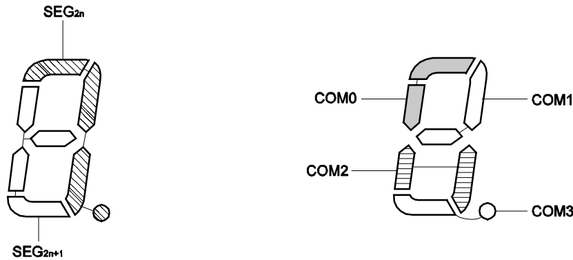
图 16-20. 4 分吋 LCD 显示模式和电极连接
