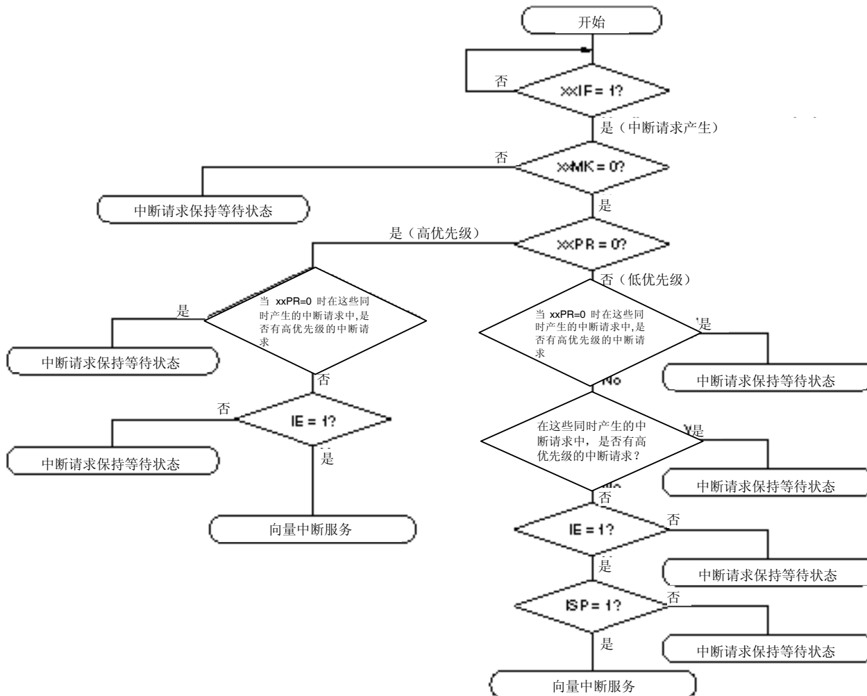
图 19-7. 中断请求响应处理
