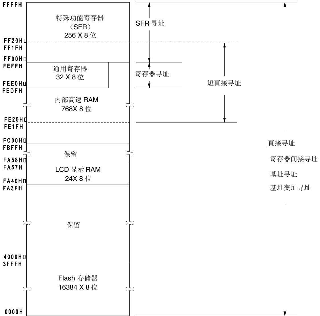
图 3-6. 数据存储器和寻址方式的对应关系( \mu PD78F0421, 78F0431)
