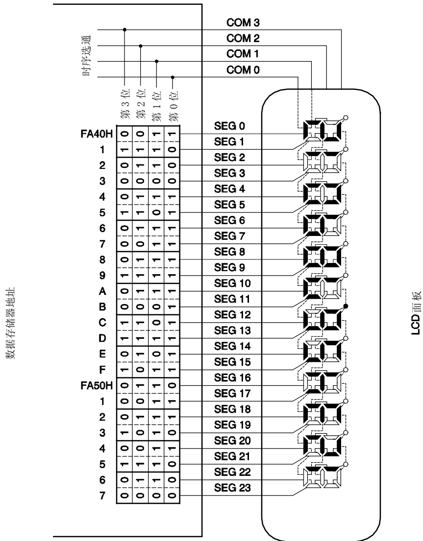
图 16-21. 4 分时 LCD 面板连接举例
