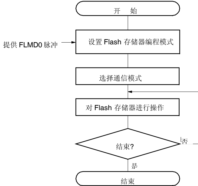
图 26-11. Flash 存储器操作过程
