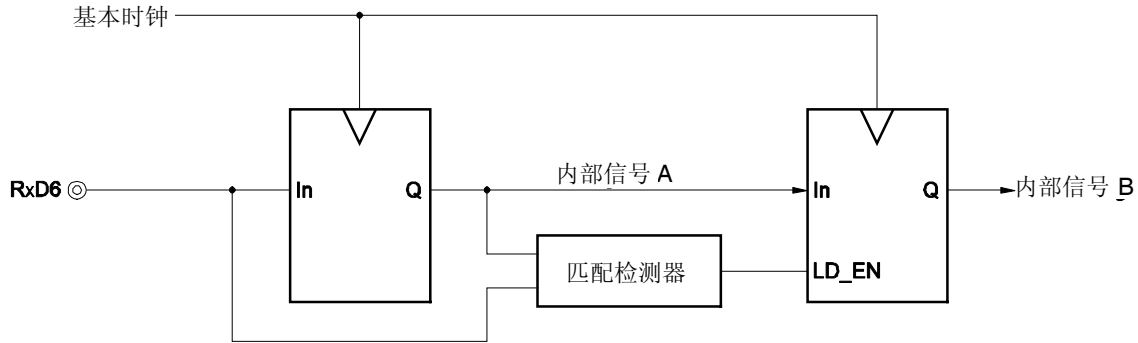
图 14-23. 噪声过滤器电路
