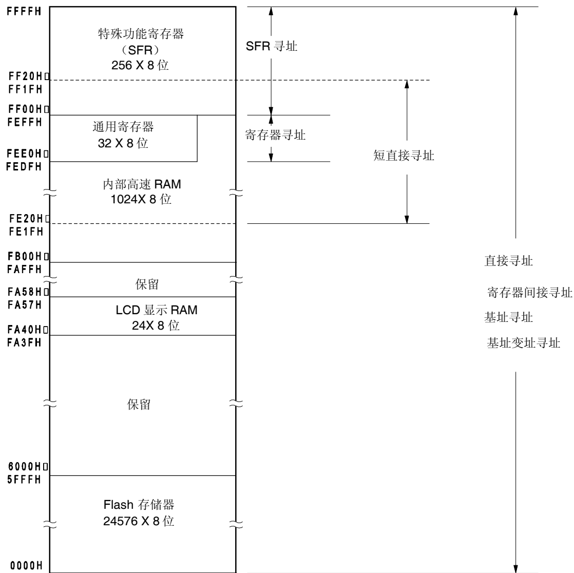
图 3-7. 数据存储与寻址方式的对应关系(μPD78F0422, 78F0432)
