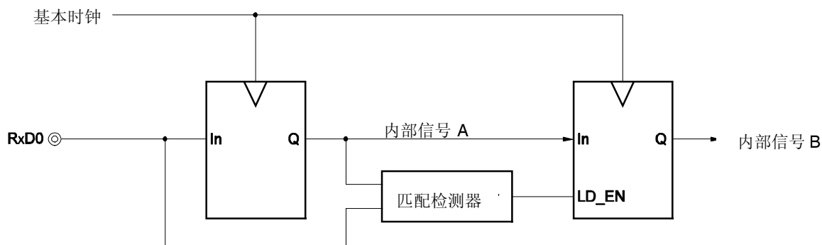
图 13-11. 噪音过滤器电路
