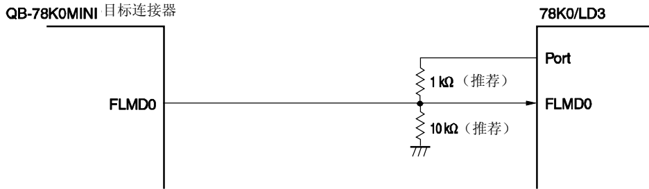
图 27-2. 通过片上调试自编程 FLMD0 引脚的连接
