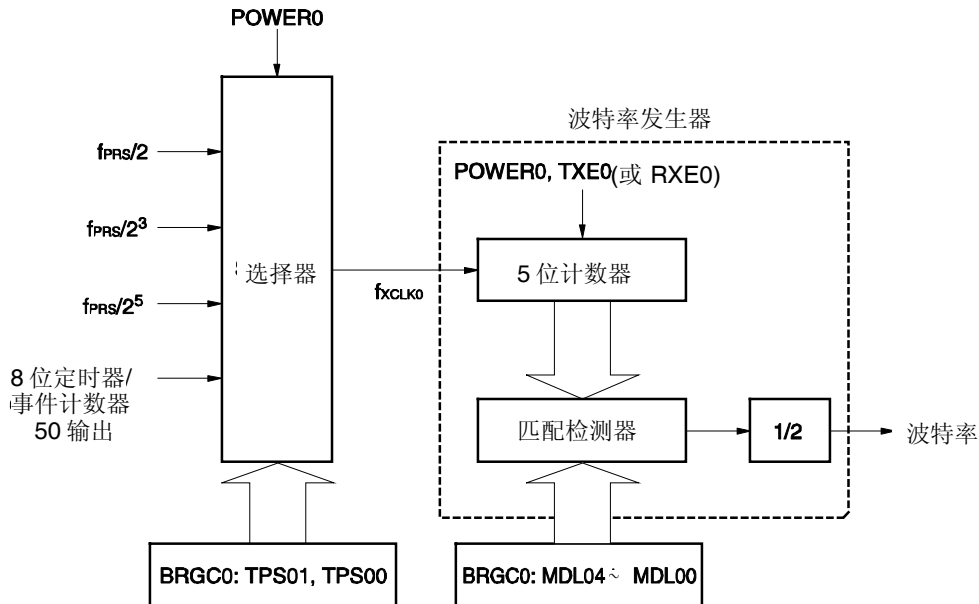
图 13-12. 波特率发生器的配置
