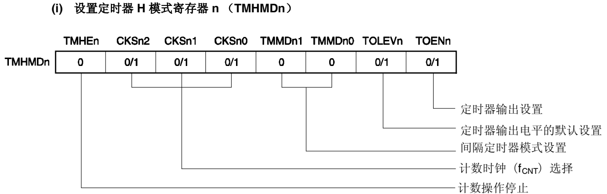
图 8-11. 间隔定时器/方波输出操作期间的寄存器设置
