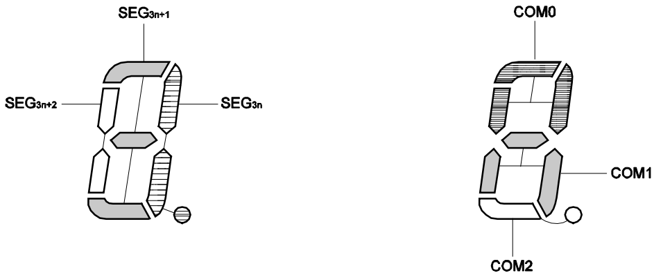
图 16-16. 3 分时 LCD 显示模式和电极连接
