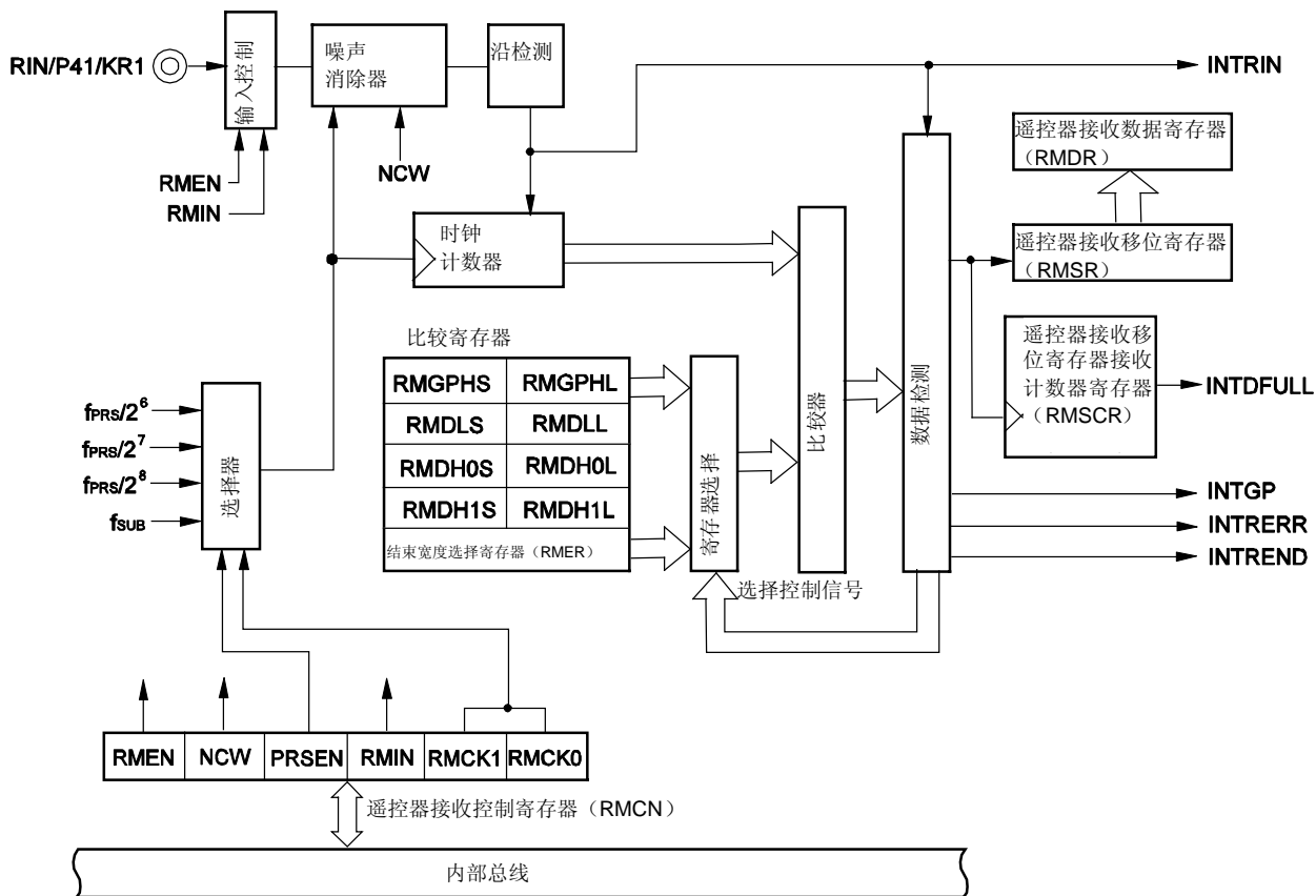
图 18-1. 遥控器接收器的框图
