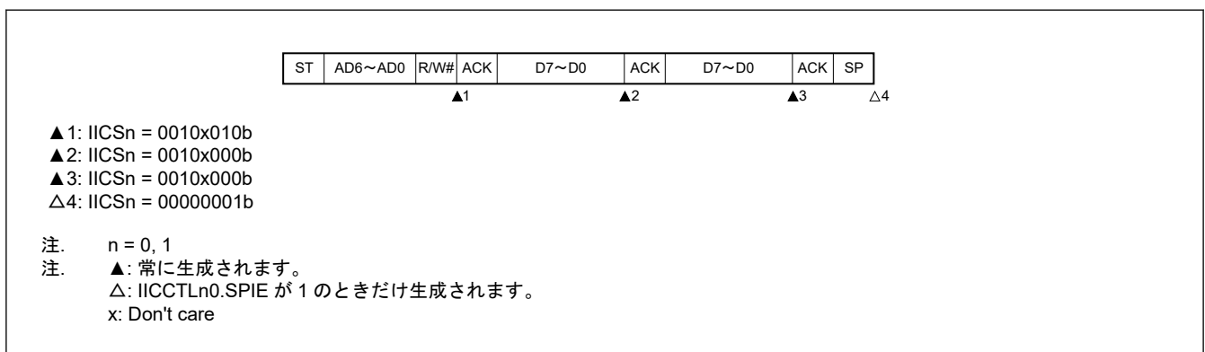
図 22.37 スレーブデバイスの拡張コード受信動作 (IICCTLn0.WTIM が 0 の場合)
