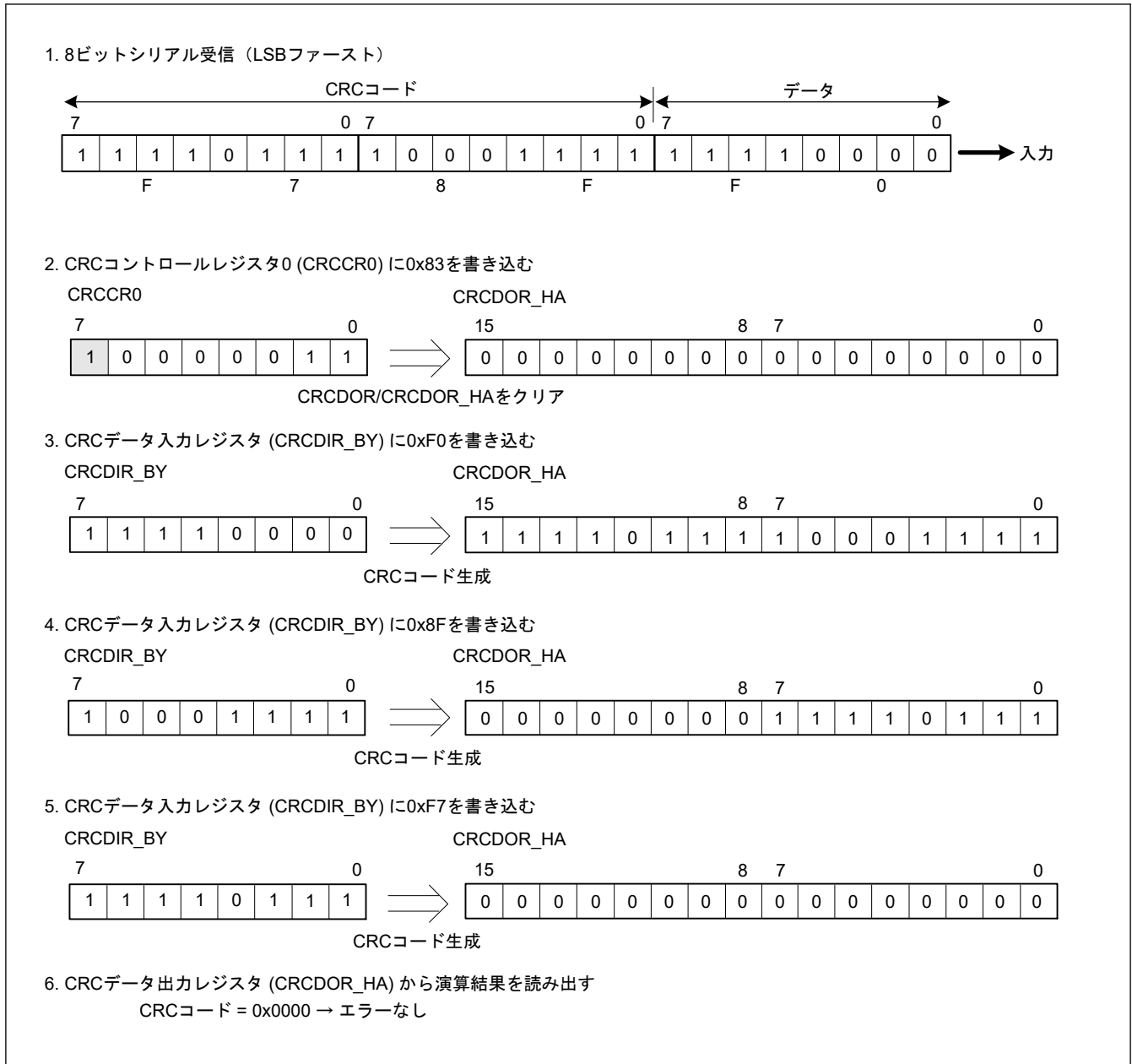
図 24.3 LSB ファーストのデータ受信
