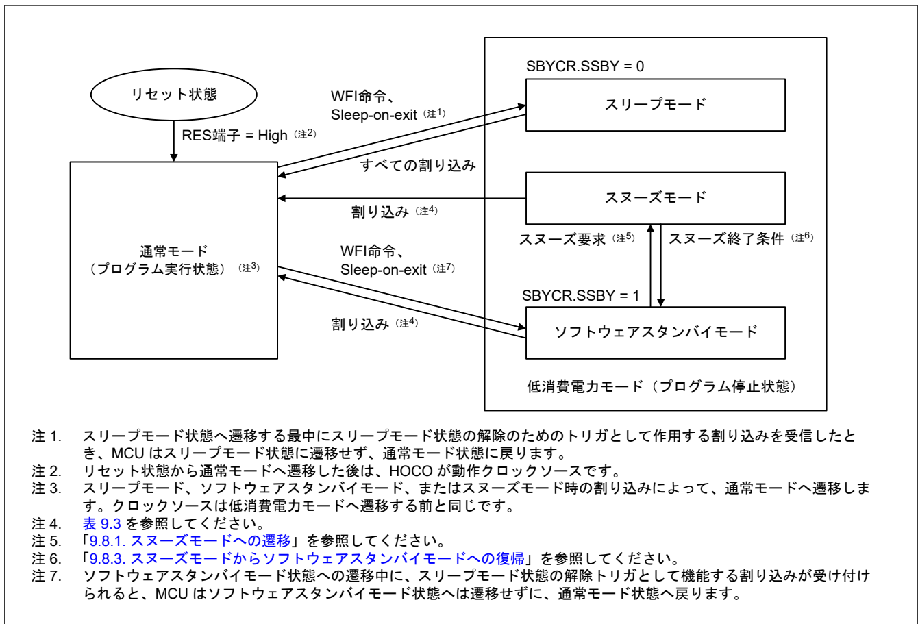
図 9.1 低消費電力モードの遷移
