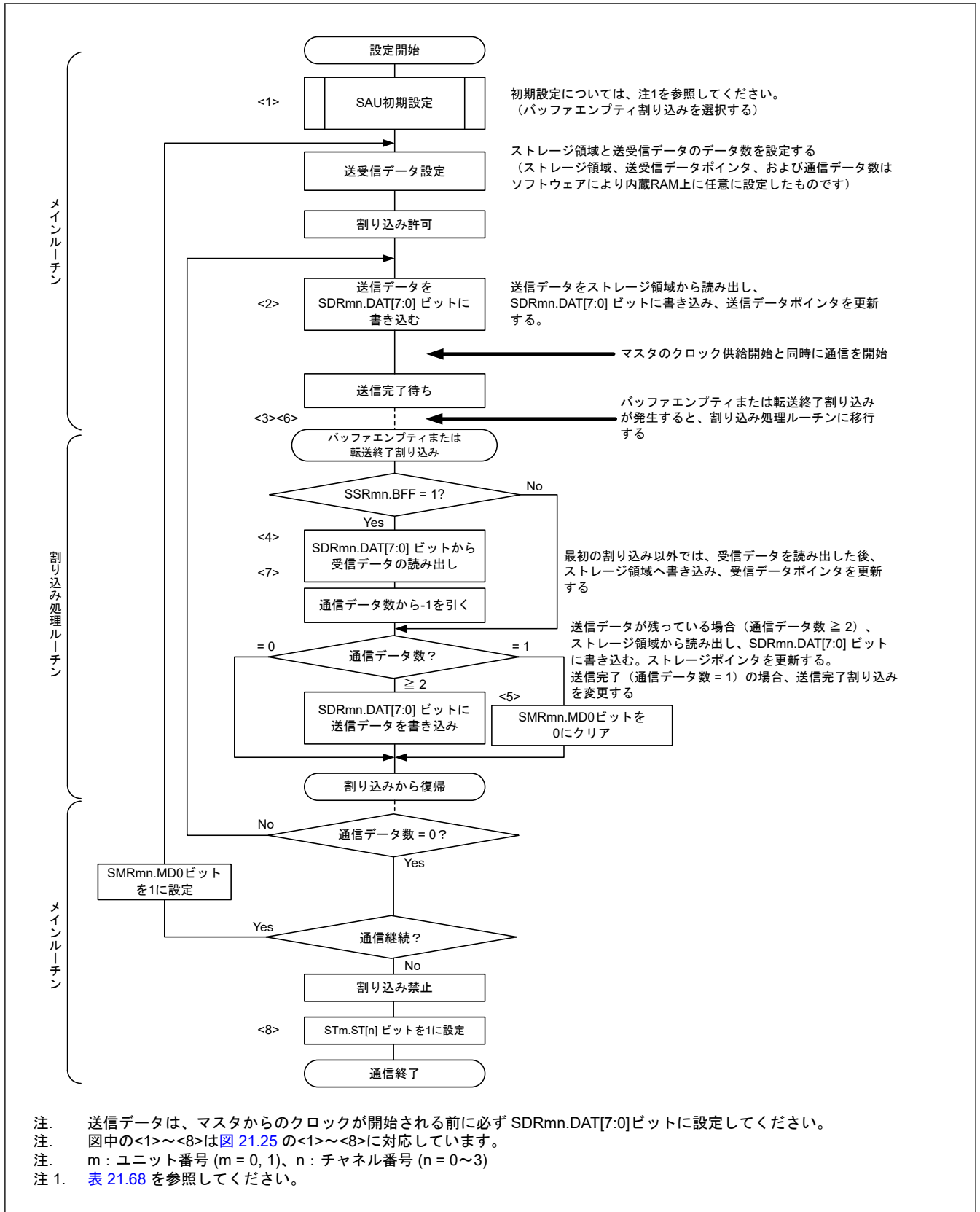
図 21.26 スレーブ送受信のフローチャート (連続送受信モード時)
