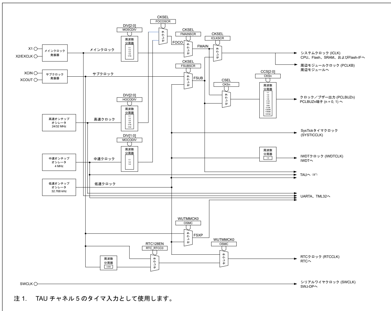
図 8.1 クロック発生回路のブロック図 (64、48、32 ピン)
