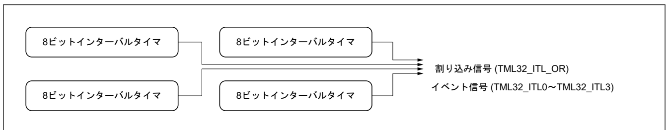
図 18.1 8 ビットインターバルタイマ×4 の機能イメージ
