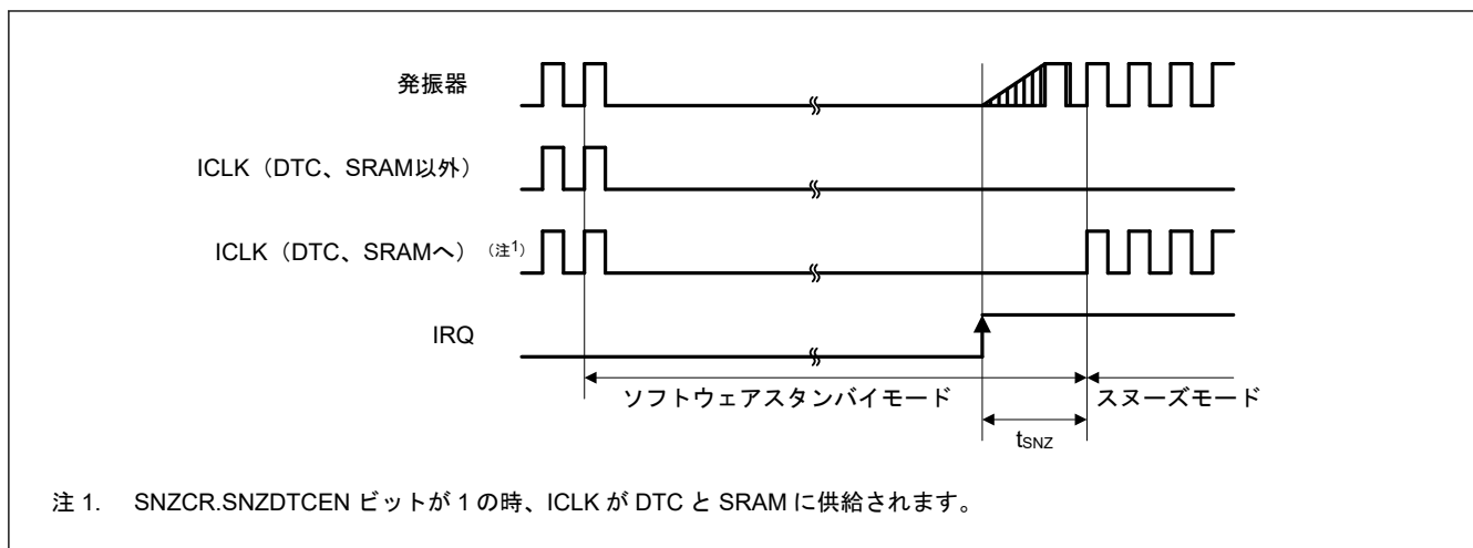
図 31.13 ソフトウェアスタンバイモードからスリープモードへの復帰タイミング
