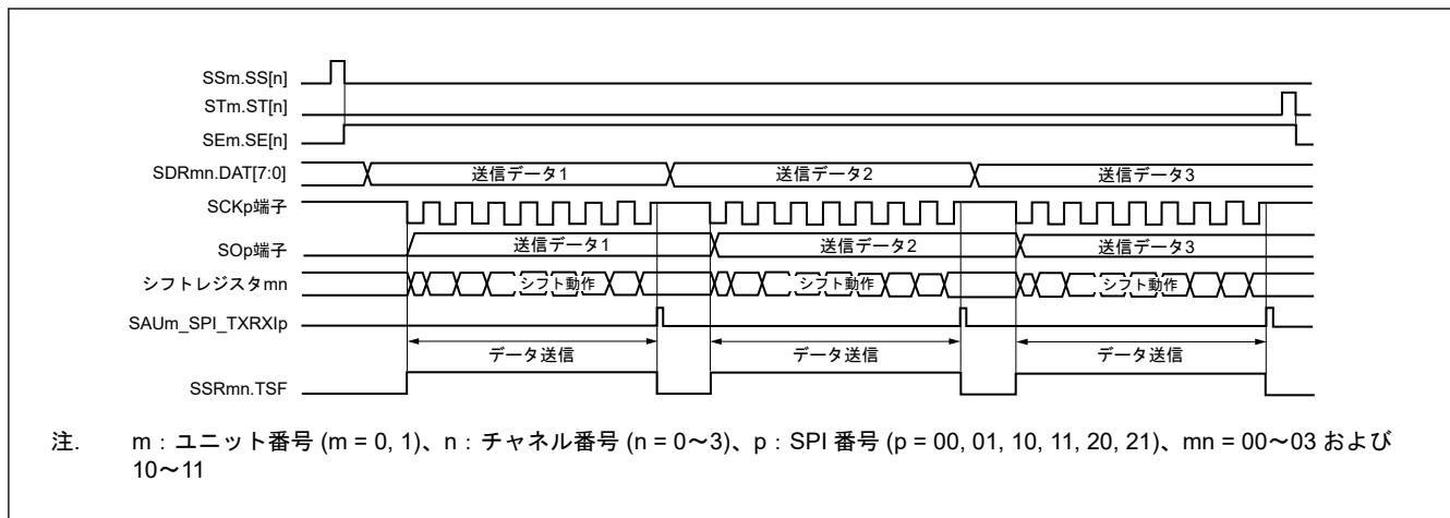
図 21.17 スレープ送信のタイミング (シングル送信モードの場合) (タイプ 1 : SCRmn.DCP[1:0] = 00b)
