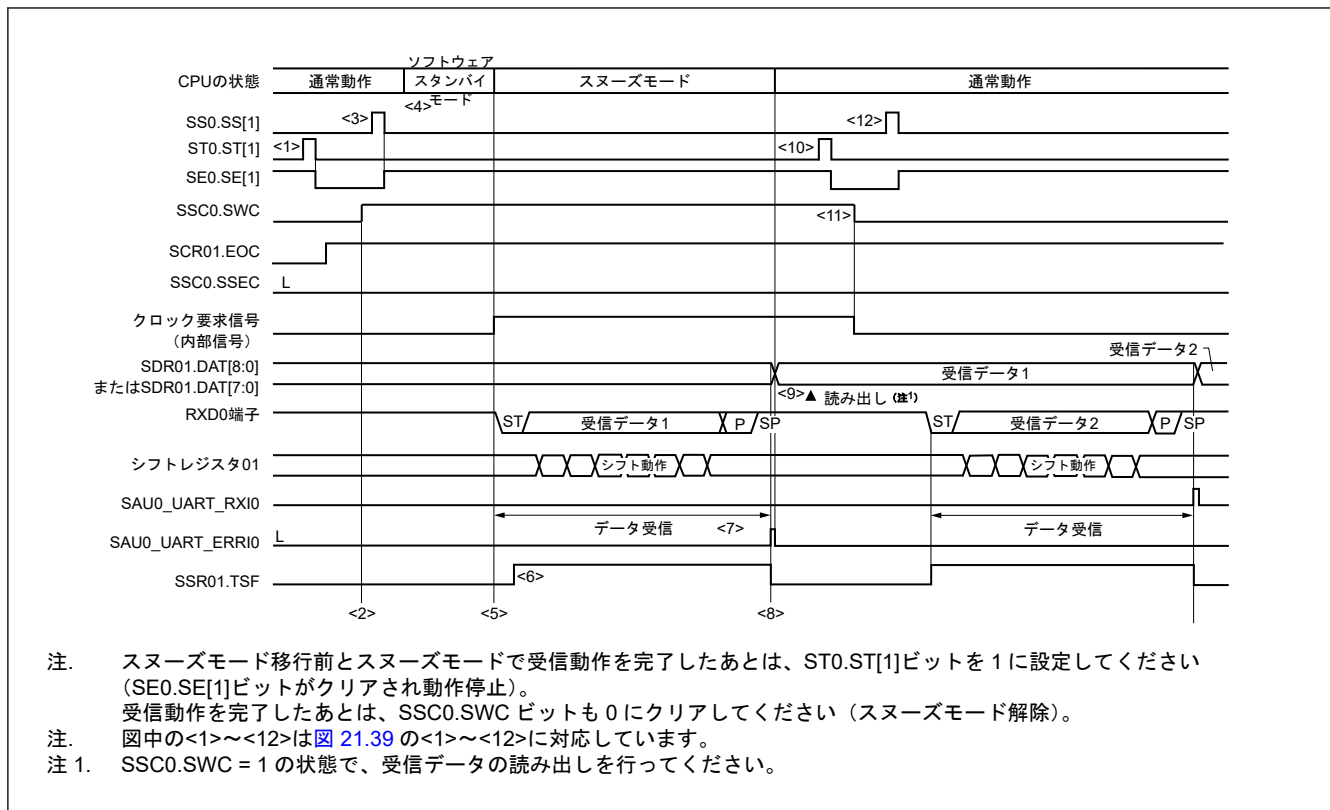
図 21.38 スリープモード動作のタイミング (SCR01.EOC = 1, SSC0.SSEC = 0)
