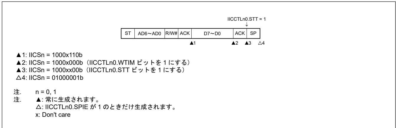
図 22.59 リスタートコンディションの生成を試みた時にストップコンディションによりアービトレーションロストが発生した場合の動作 (IICCTLn0.WTIM = 0)
