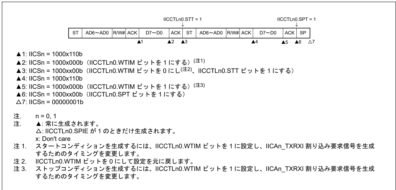
図 22.25 マスタデバイスのリスタート動作 (IICCTLn0.WTIM が 0 の場合)
