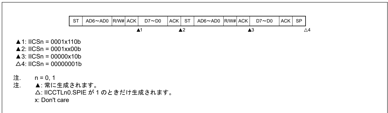
図 22.36 通常アクセスの後のスレーブデバイスの動作、一致しない (IICCTLn0.WTIM = 1)
