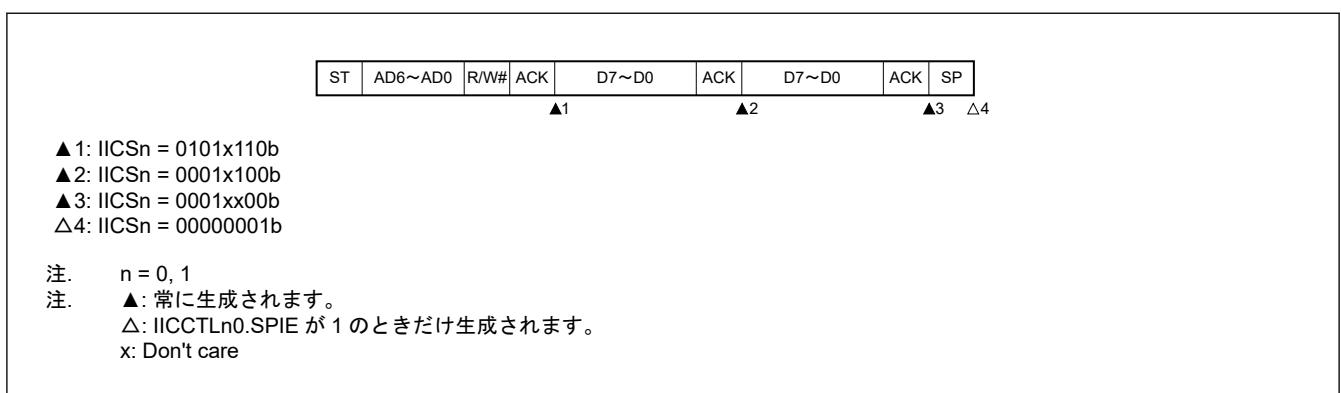
図 22.47 スレーブアドレスデータ送信時のアービトレーションロスト (IICCTLn0.WTIM が 1 の場合)
