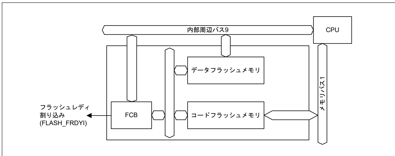
図 28.1 フラッシュメモリ関連モジュールのブロック図
