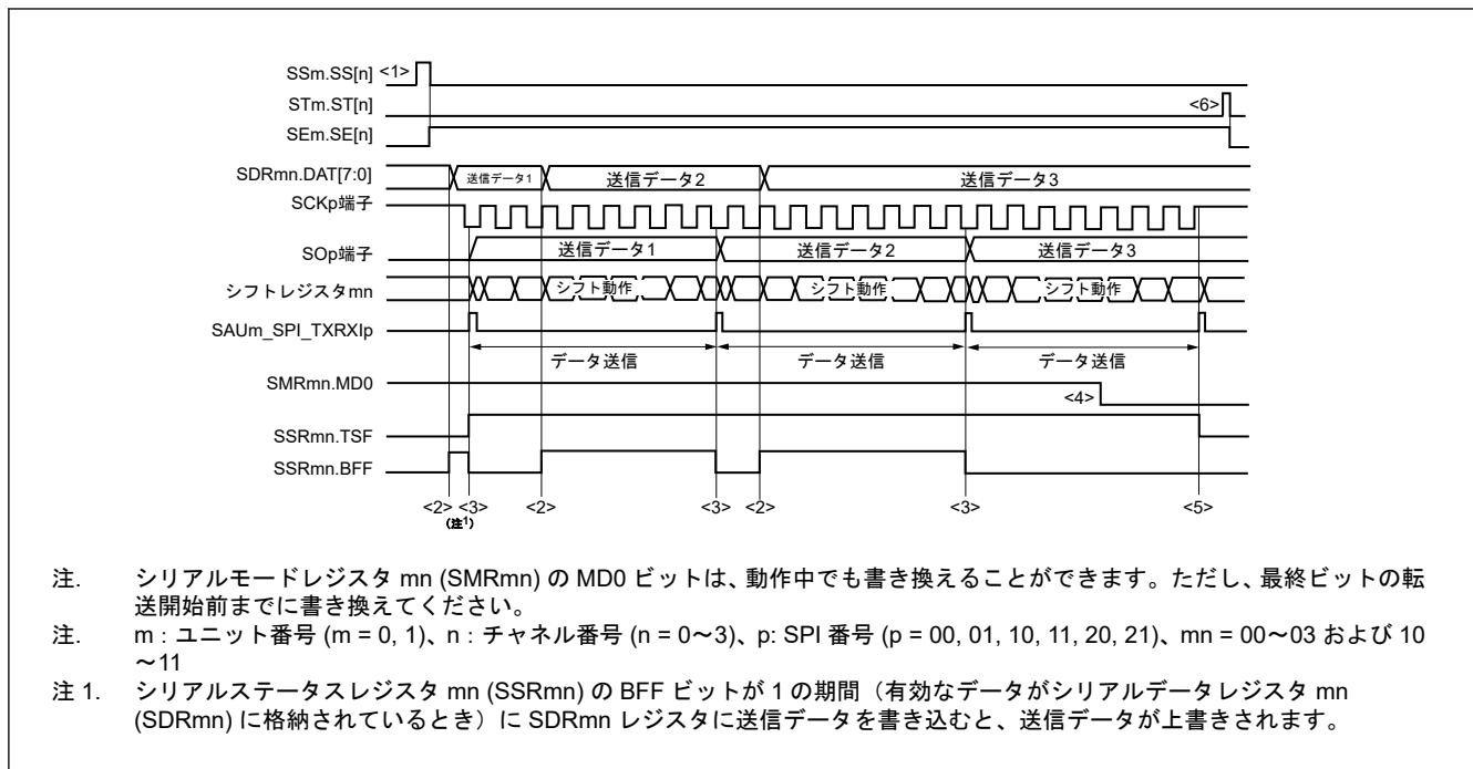
図 21.19 スレーブ送信のタイミング (連続送信モードの場合) (タイプ 1 : SCRmn.DCP[1:0] = 00b)
