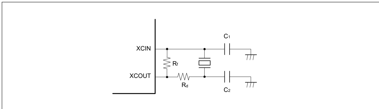
図 8.6 32.768 kHz 水晶振動子の接続例
