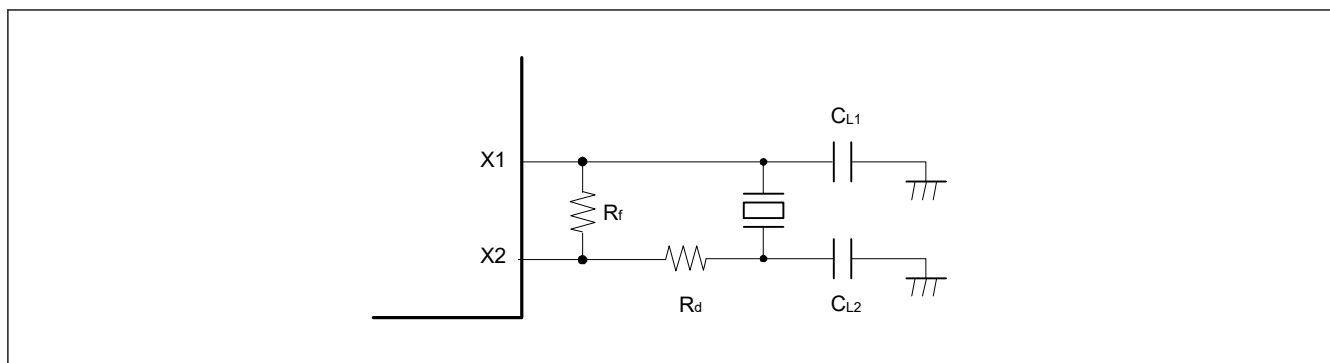
図 8.3 発振子の接続例
