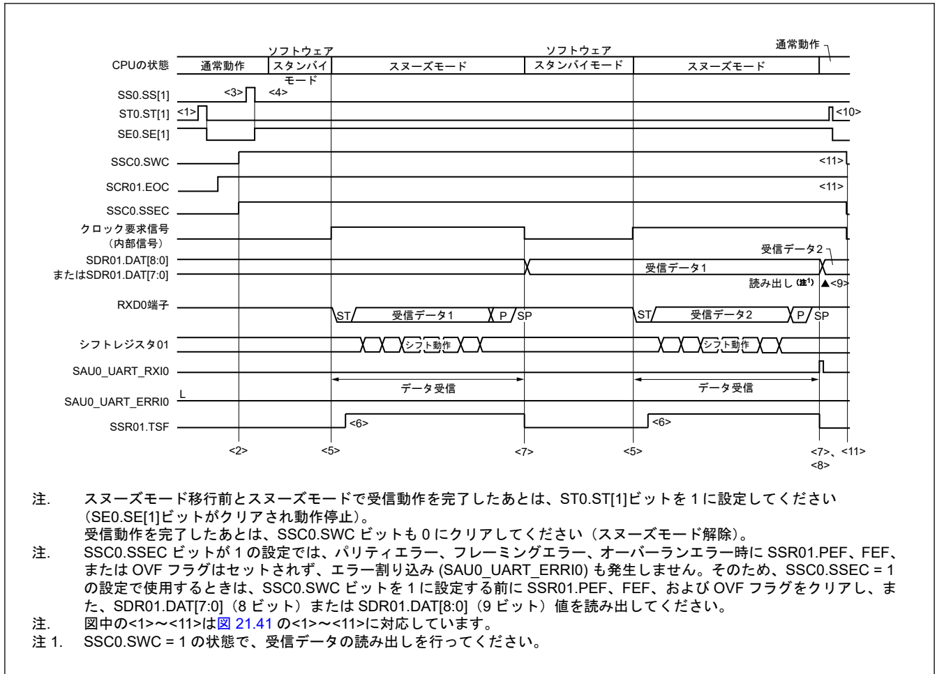
図 21.40 スヌーズモード動作のタイミング (SCR01.EOC = 1, SSC0.SSEC = 1)
