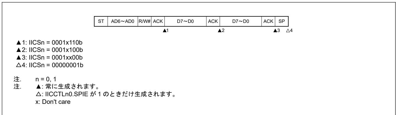
図 22.30 スレーブデバイスのスレーブアドレスデータ受信動作 (IICCTLn0.WTIM が 1 の場合)
