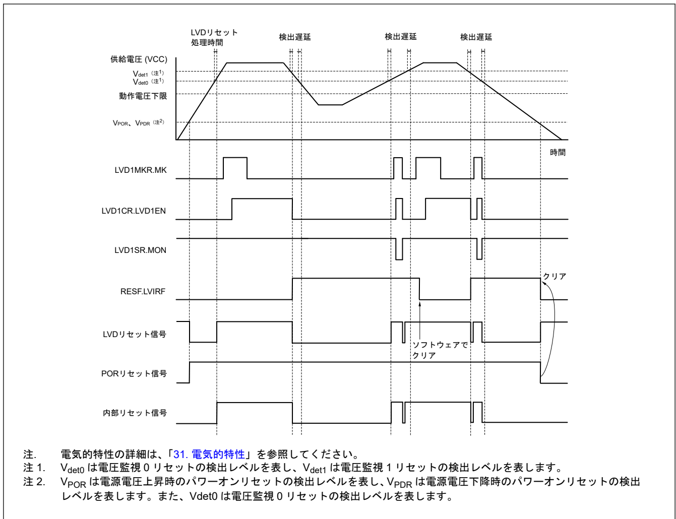
図 5.2 電圧監視 1 リセット時の動作例
