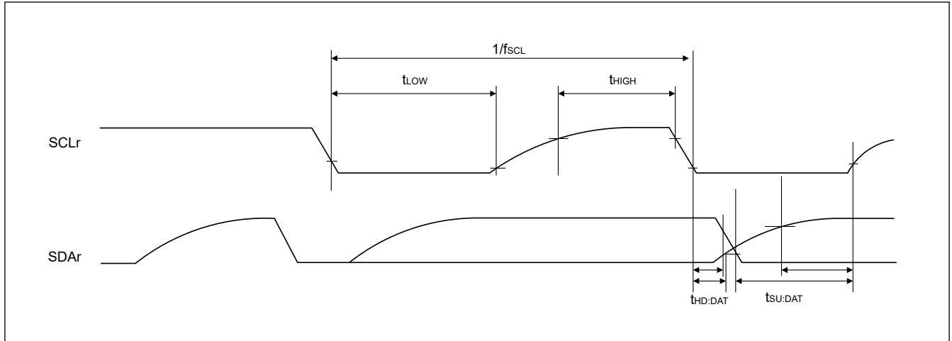
図 31.30 異なる電圧レベルで動作しているデバイスとの簡易 IIC 通信でのシリアル転送のタイミング
