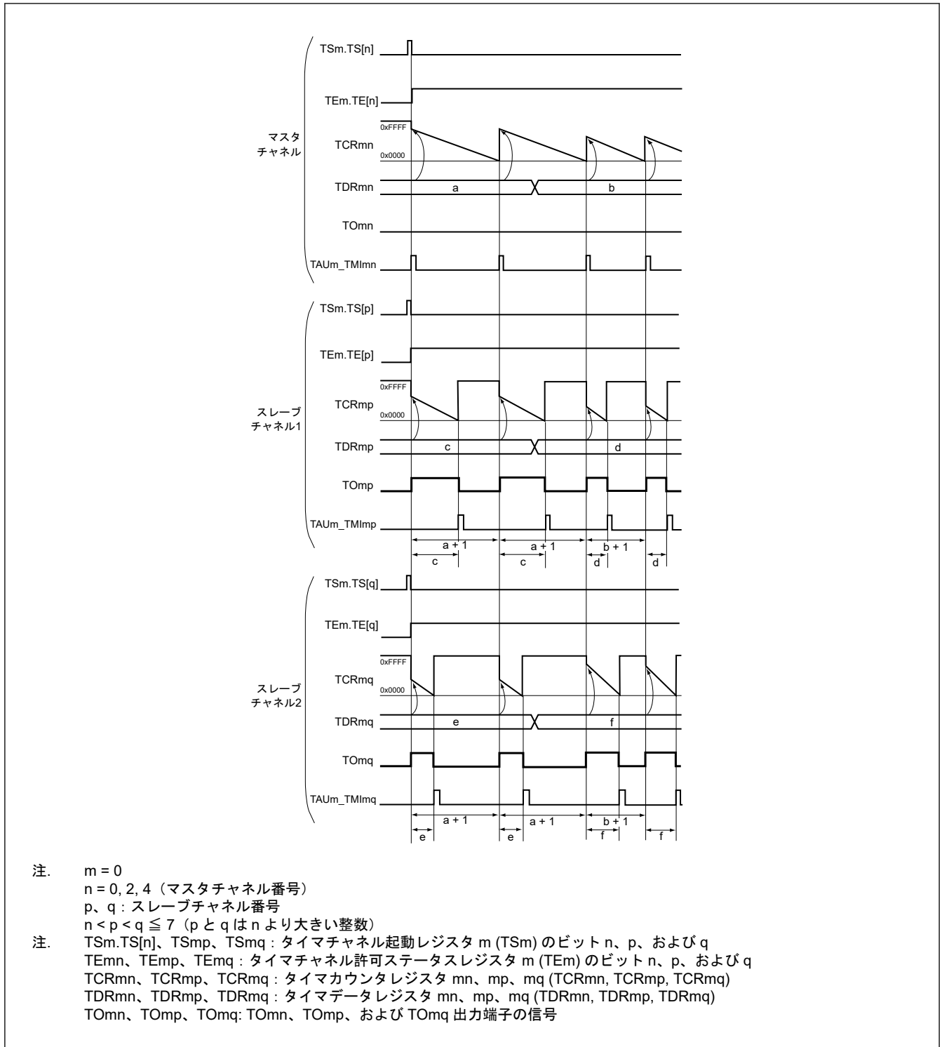
図 17.54 多重 PWM 出力機能として動作する場合の基本タイミング例 (2 種類の PWM 波形を出力する場合)
