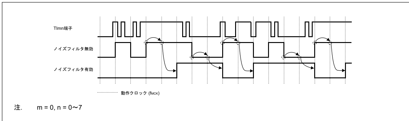
図 17.36 TI0n 入力端子から入力されるサンプリング波形とノイズフィルタが有効な場合と無効な場合の出力波形
