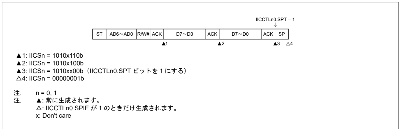
図 22.28 マスタデバイスの拡張コード送信動作 (IICCTLn0.WTIM が 1 の場合)
