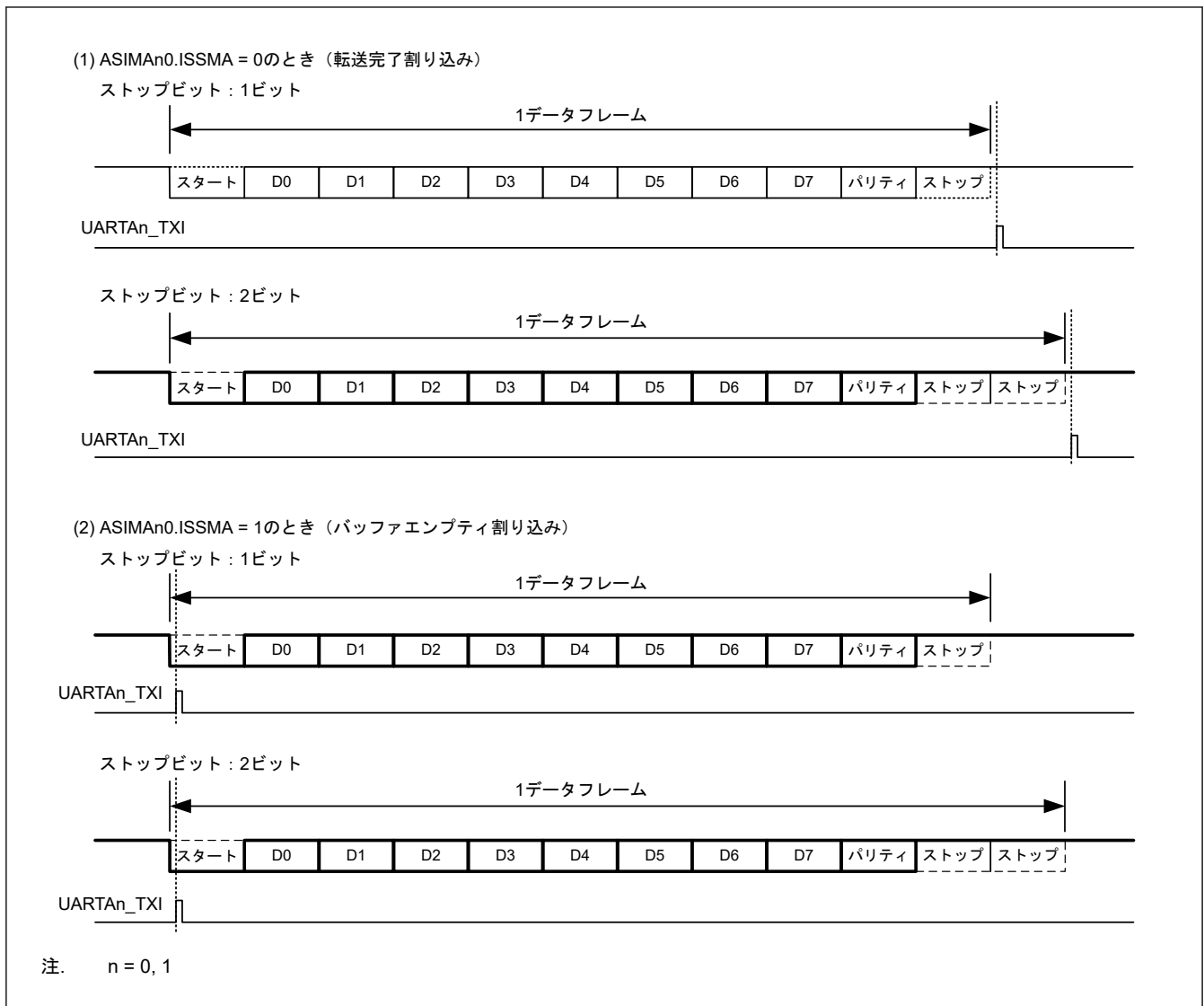
図 23.4 割り込み出力タイミング
