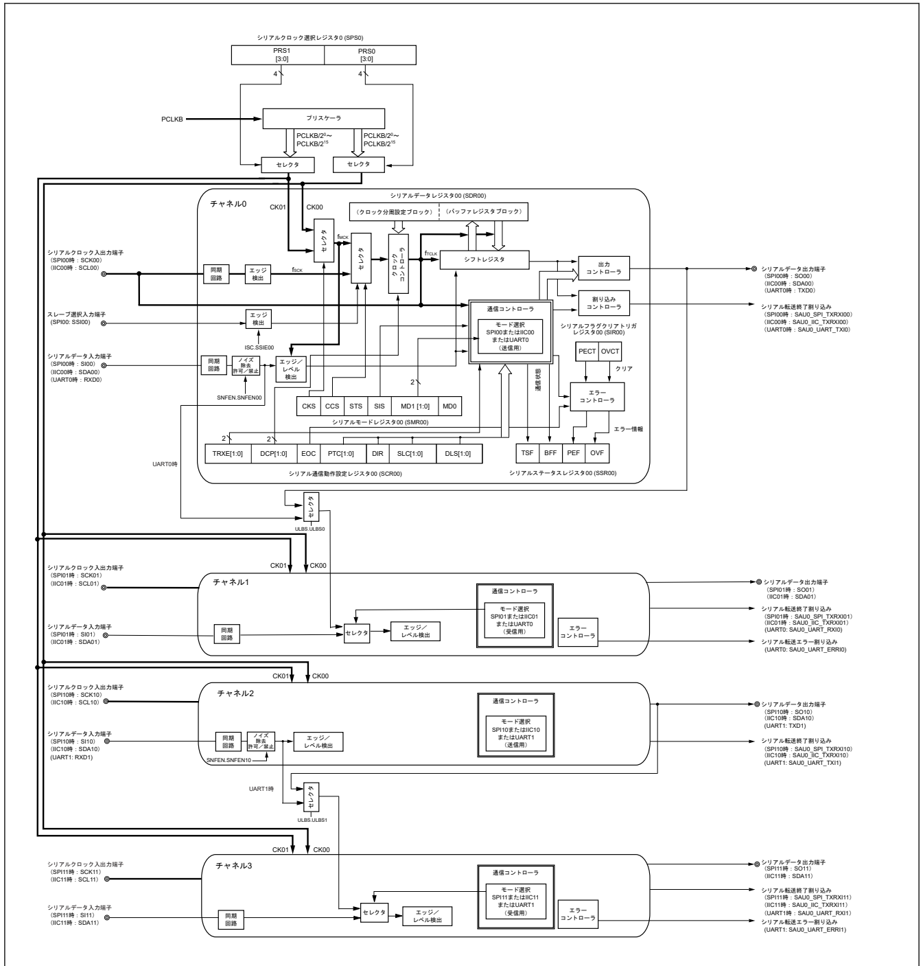
図 21.1 シリアルアレイユニット 0 のブロック図 図 21.2 にシリアルアレイユニット 1 のブロック図を示します。
