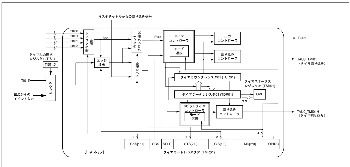
図 17.14 タイマアレユユニット 0 のチャンネル 1 の内部ブロック図
