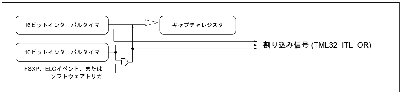
図 18.3 16 ビットインターバルタイマと 16 ビットキャプチャの機能イメージ
