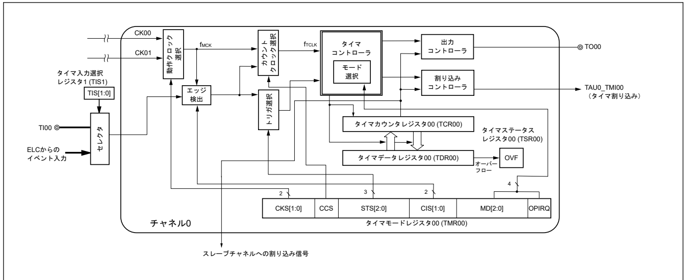
図 17.13 タイマアレユユニット 0 のチャンネル 0 の内部ブロック図
