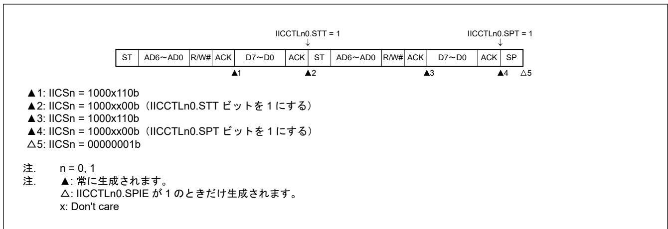
図 22.26 マスタデバイスのリスタート動作 (IICCTLn0.WTIM が 1 の場合)
