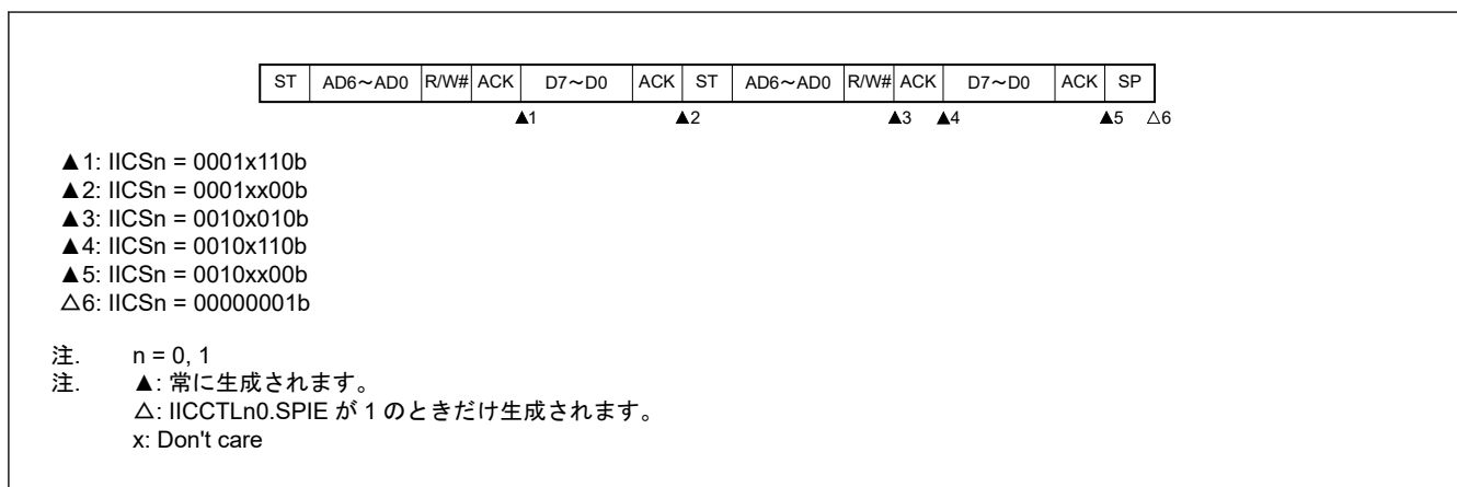
図 22.34 通常アクセス、拡張コードとの一致後のスレーブデバイスの動作 (IICCTLn0.WTIM が 1 の場合)
