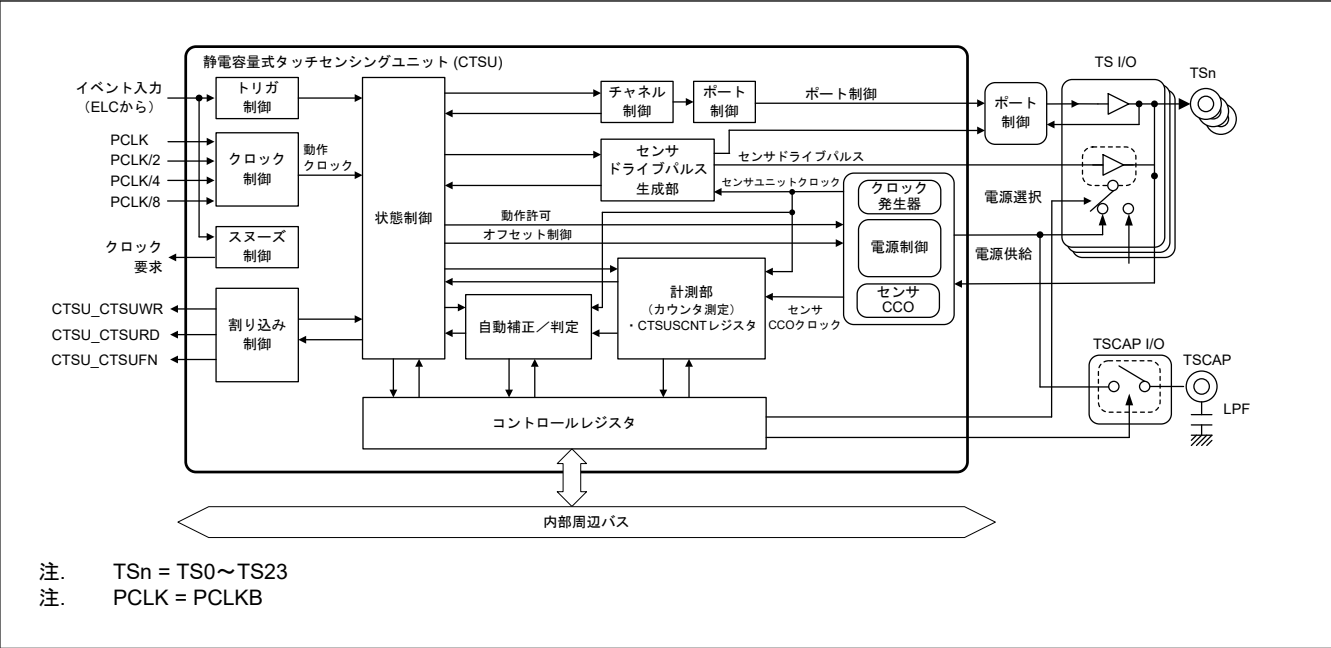
図 27.3 CTSU のブロック図
