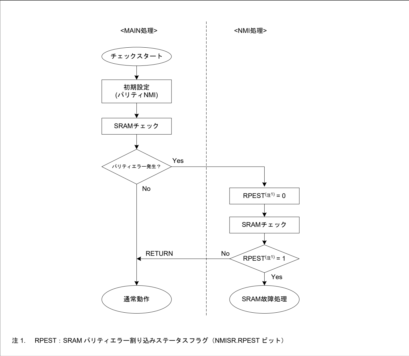
図 28.2 SRAM パリティ割り込み許可の場合の SRAM パリティチェックのフロー
