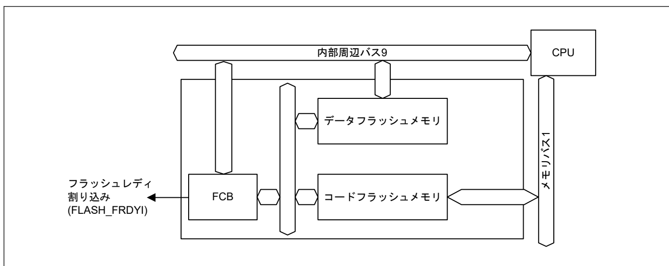
図 29.1 フラッシュメモリ関連モジュールのブロック図
