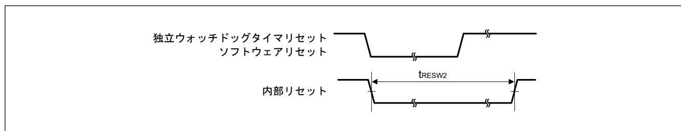
図 32.11 リセット入力タイミング (2)
