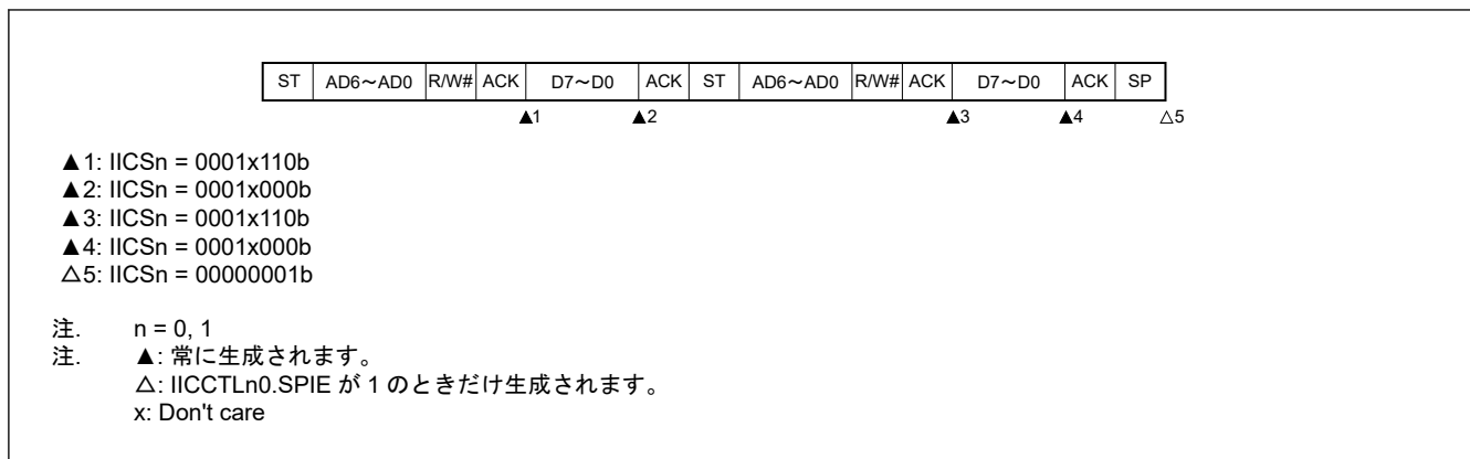
図 22.31 通常アクセス、SVAn との一致後のスレーブデバイスの動作 (IICCTLn0.WTIM が 0 の場合)
