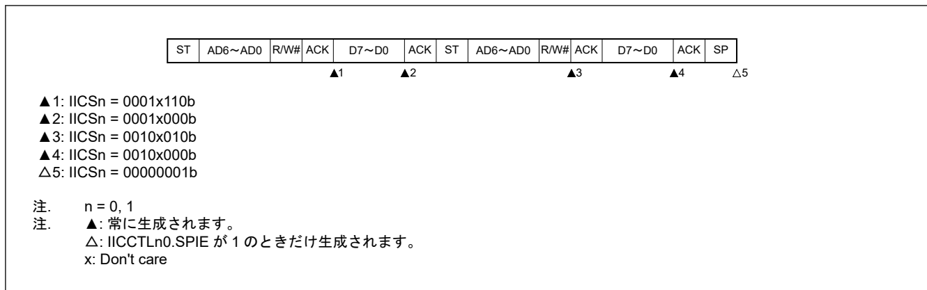
図 22.33 通常アクセス、拡張コードとの一致後のスレーブデバイスの動作 (IICCTLn0.WTIM が 0 の場合)
