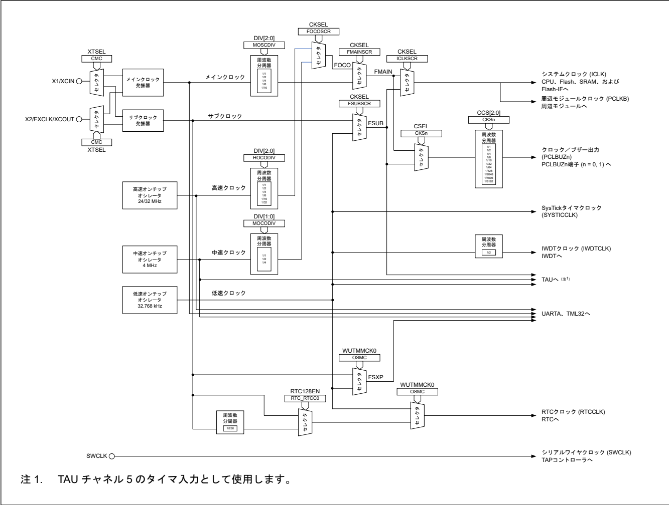
図 8.2 クロック発生回路のブロック図 (24、20 ピン)
