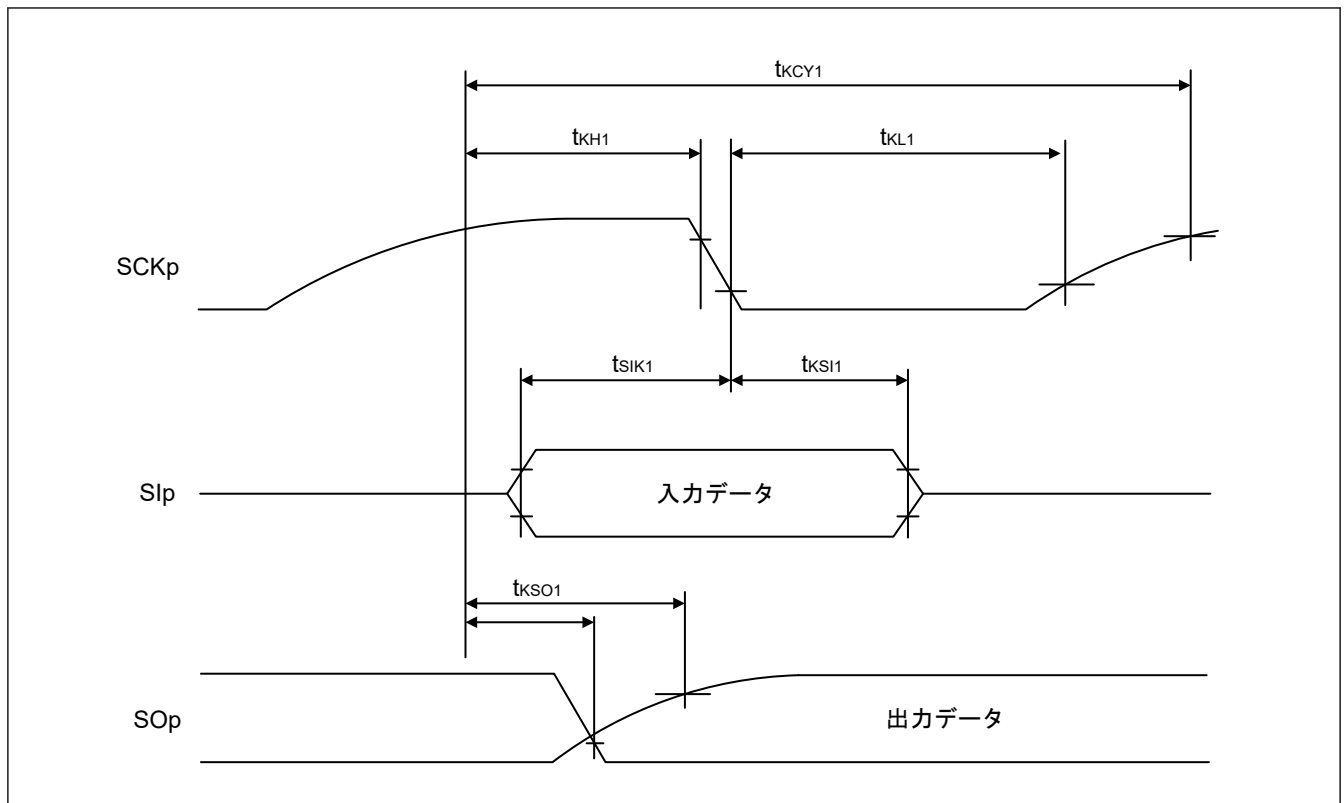
図 32.25 異なる電圧レベルで動作しているデバイスとのマスタモードでの簡易 SPI 通信でのシリアル転送のタイミング (SCRmn.DCP[1:0] = 01b または 10b の場合)
