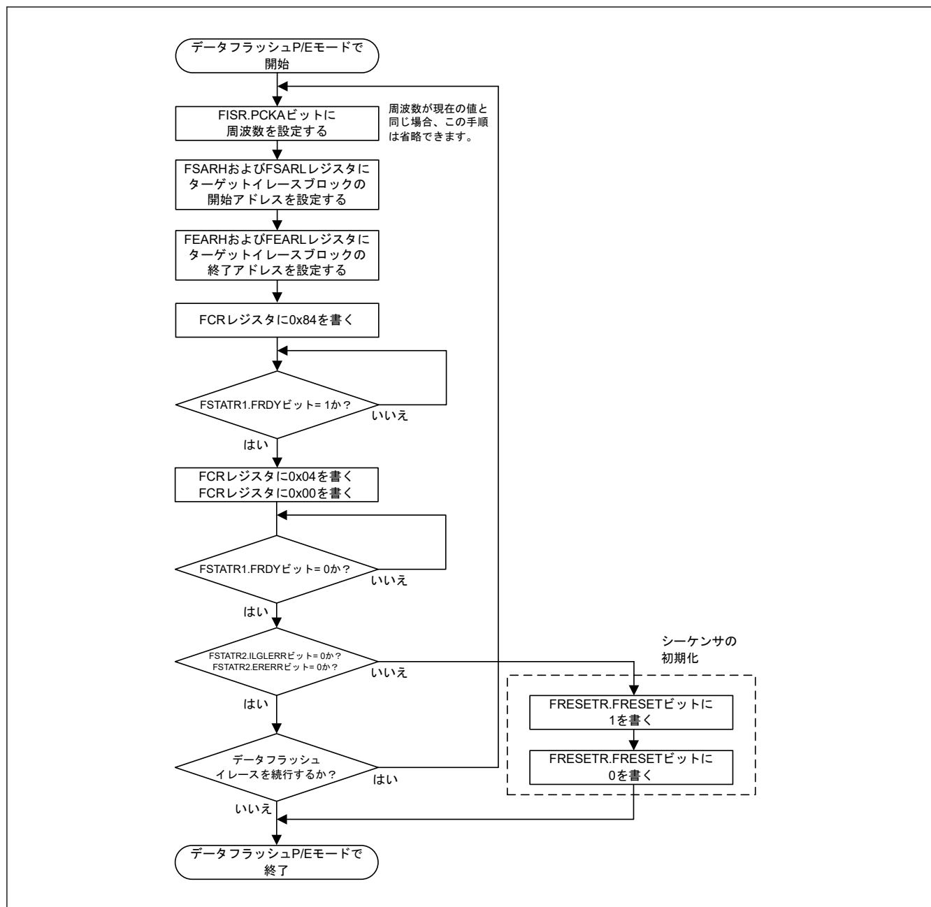
図 29.20 データフラッシュブロックイレース手順のフローチャート
