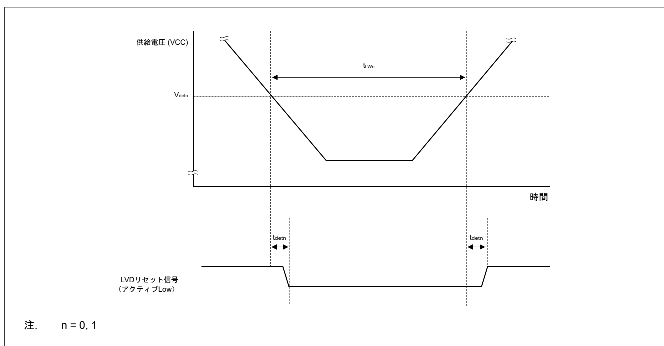
図 32.35 電圧検出回路タイミング
