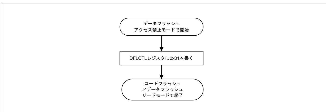
図 29.12 データフラッシュアクセス禁止モードからリードモードへのモード遷移
