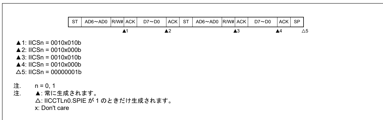
図 22.41 コードアクセス、拡張コードとの一致後のスレーブデバイスの動作 (IICCTLn0.WTIM が 0 の場合)
