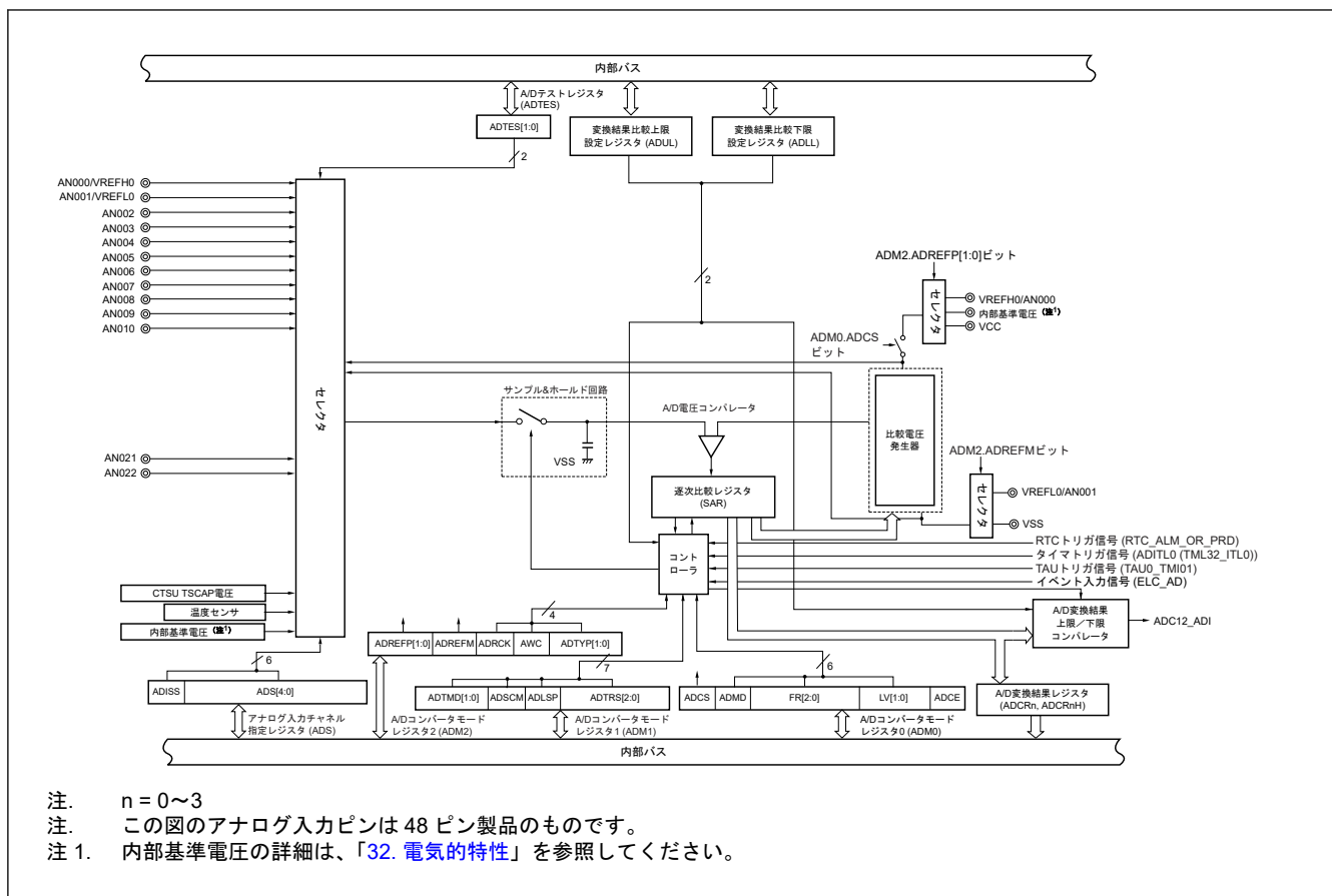
図 25.1 A/D コンバータのブロック図
