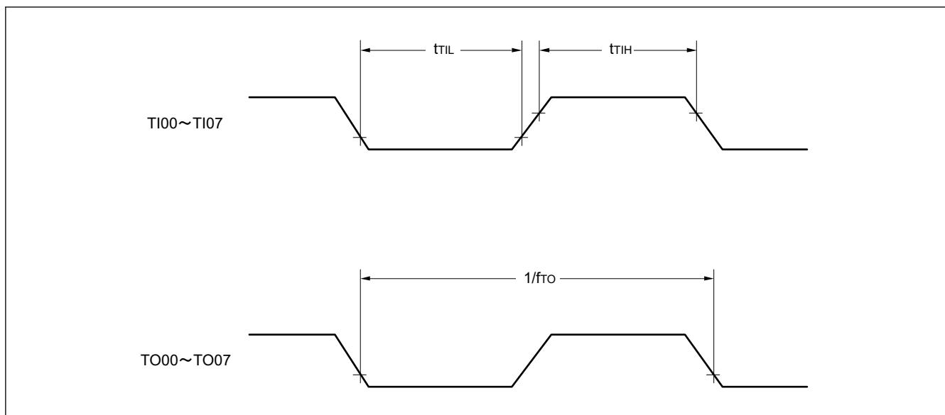
図 32.7 TI/TO タイミング
