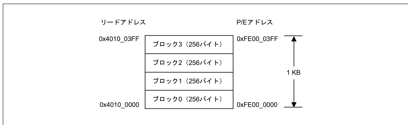
図 29.3 データフラッシュメモリマッピング
