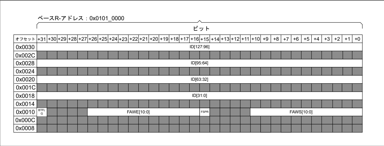
図 29.5 構成領域ビットマップ
