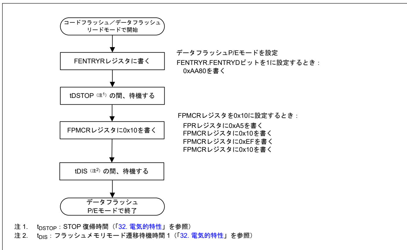
図 29.14 リードモードからデータフラッシュ P/E モードに切り替える手順
