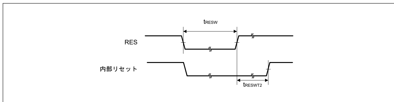
図 32.10 リセット入力タイミング (1)
