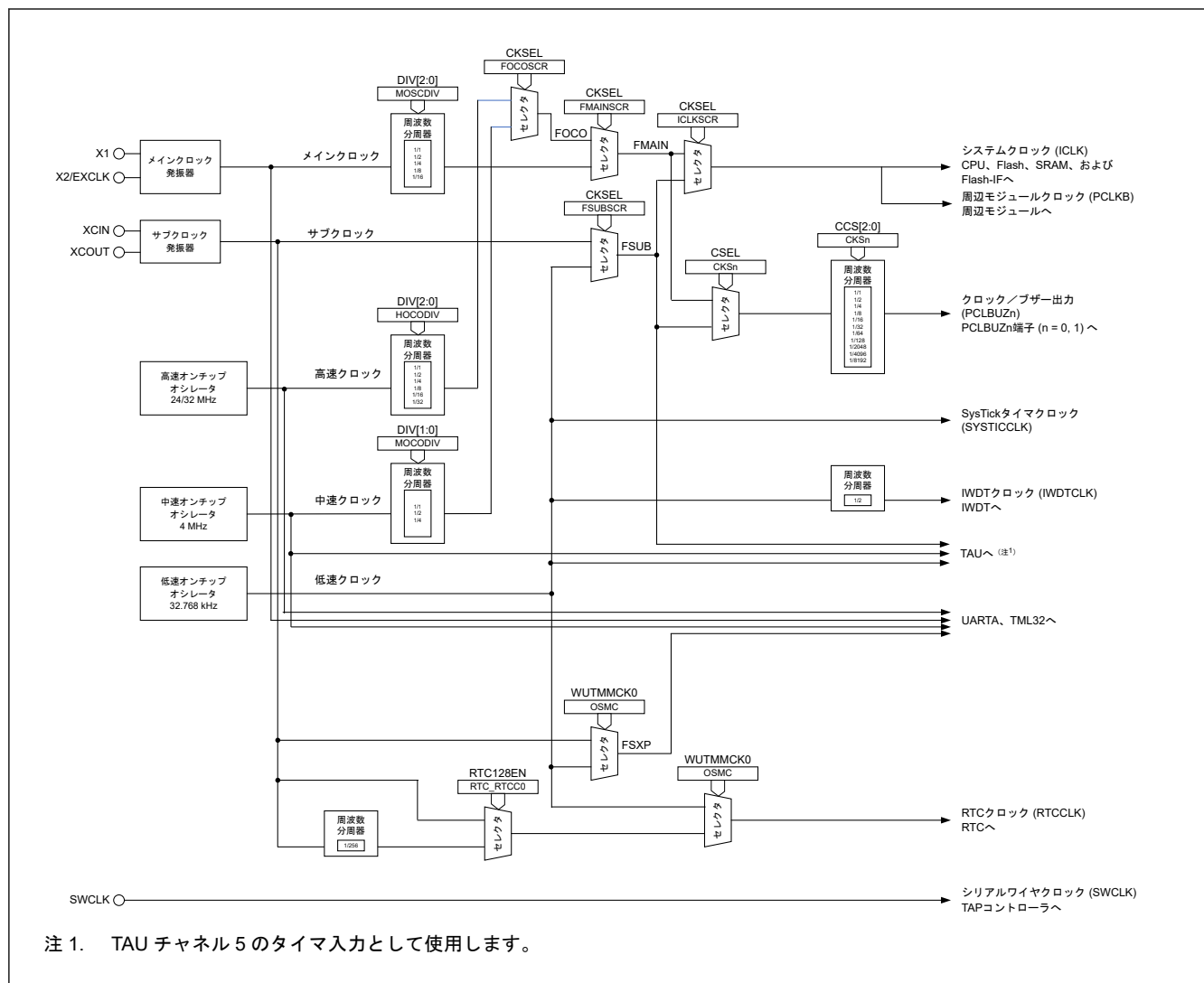
図 8.1 クロック発生回路のブロック図 (48、32 ピン)
