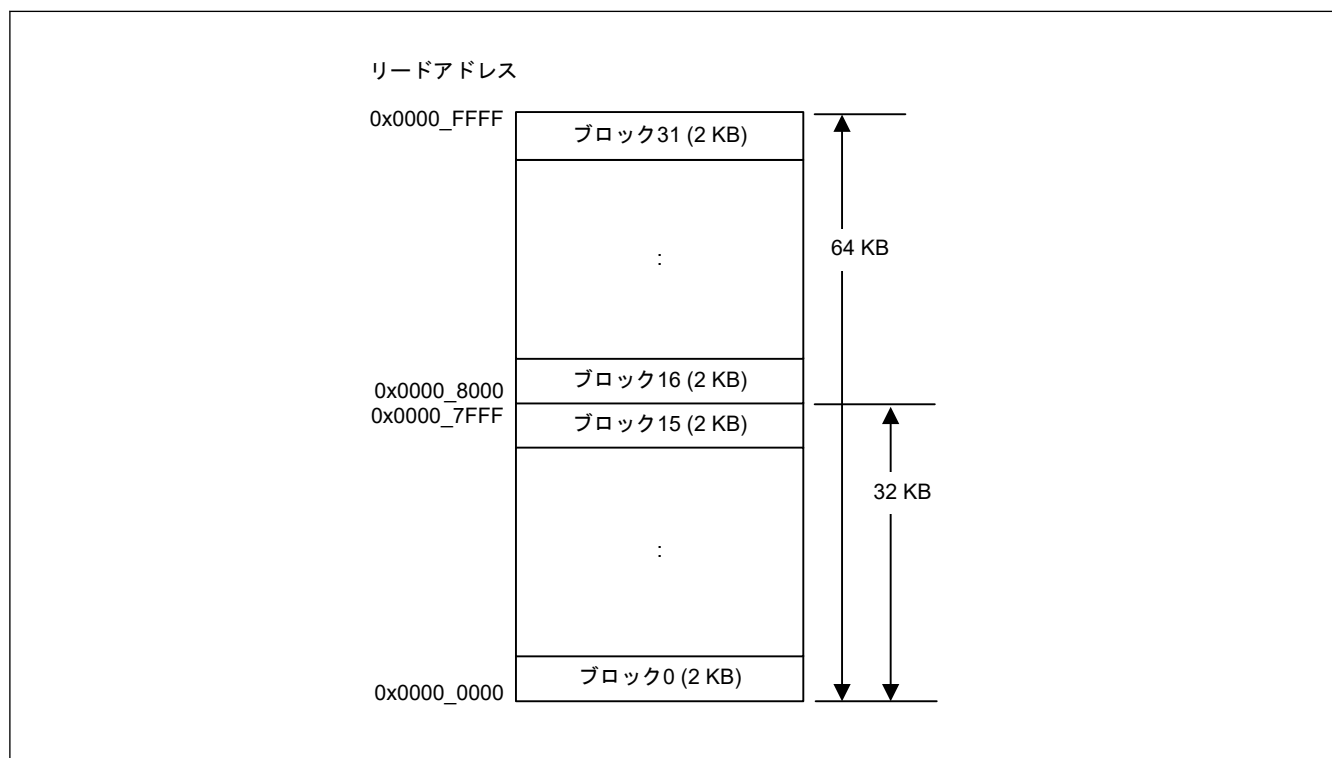
図 29.2 コードフラッシュメモリマッピング
