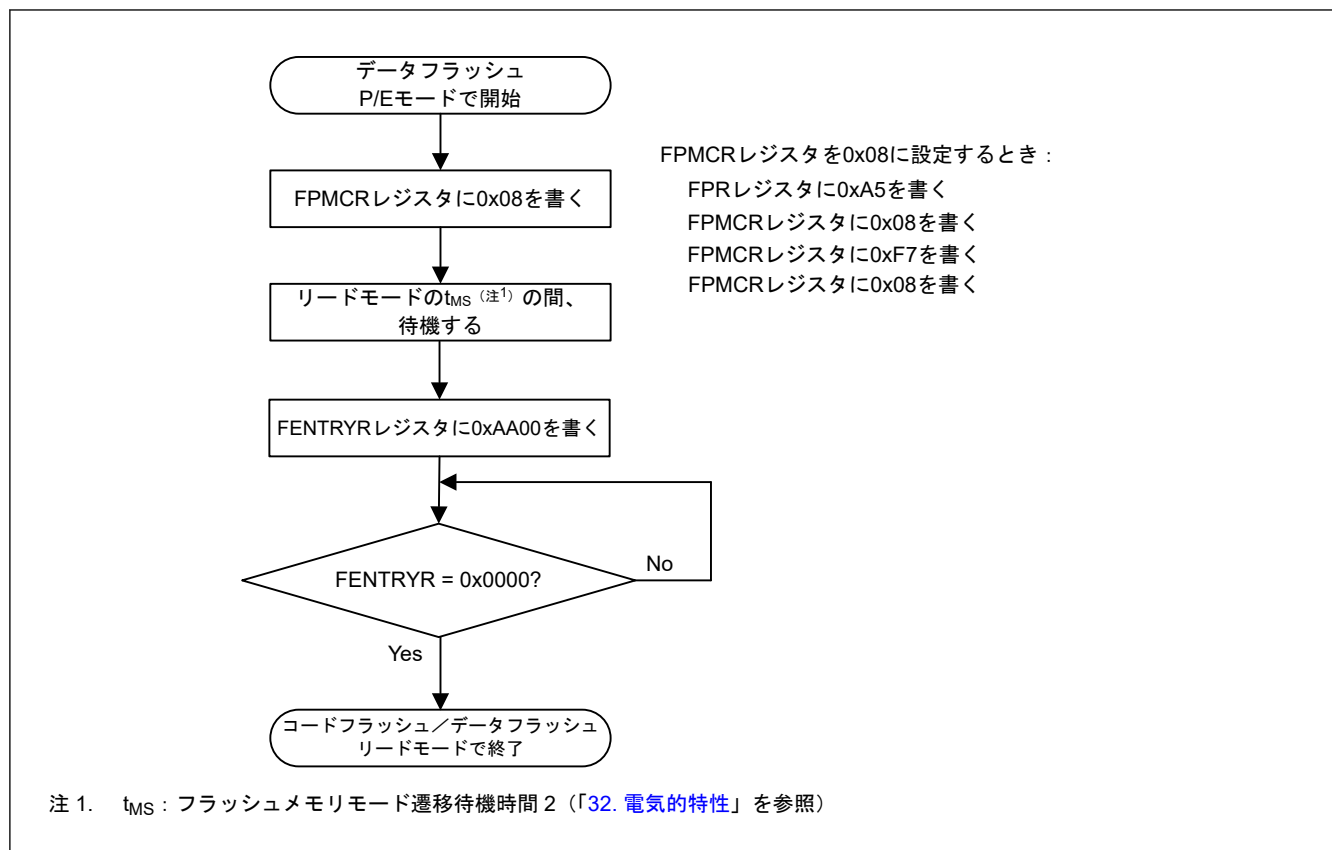
図 29.16 データフラッシュ P/E モードからリードモードへの変更手順
