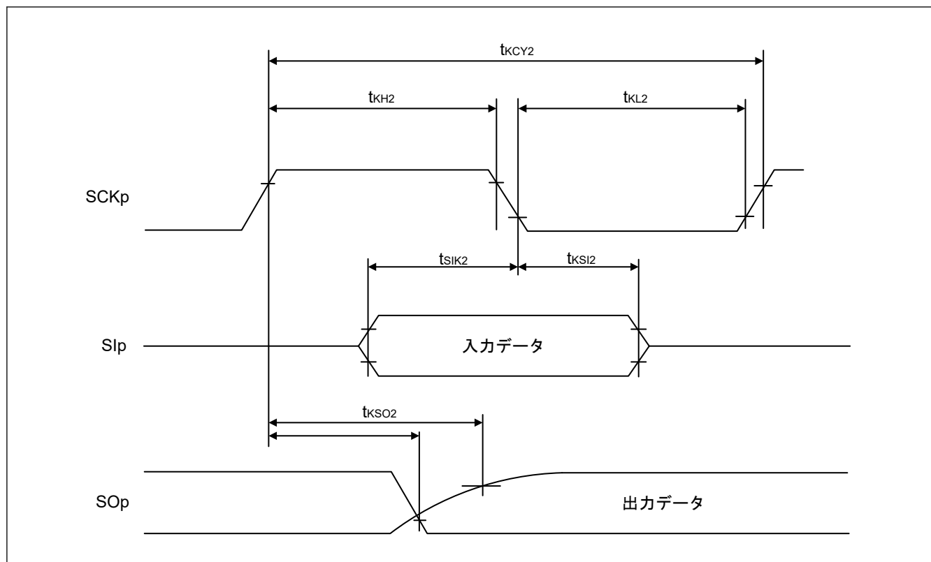
図 32.28 異なる電圧レベルで動作しているデバイスとのスレープモードでの簡易 SPI 通信でのシリアル転送のタイミング (SCRmn.DCP[1:0] = 01b または 10b の場合)
