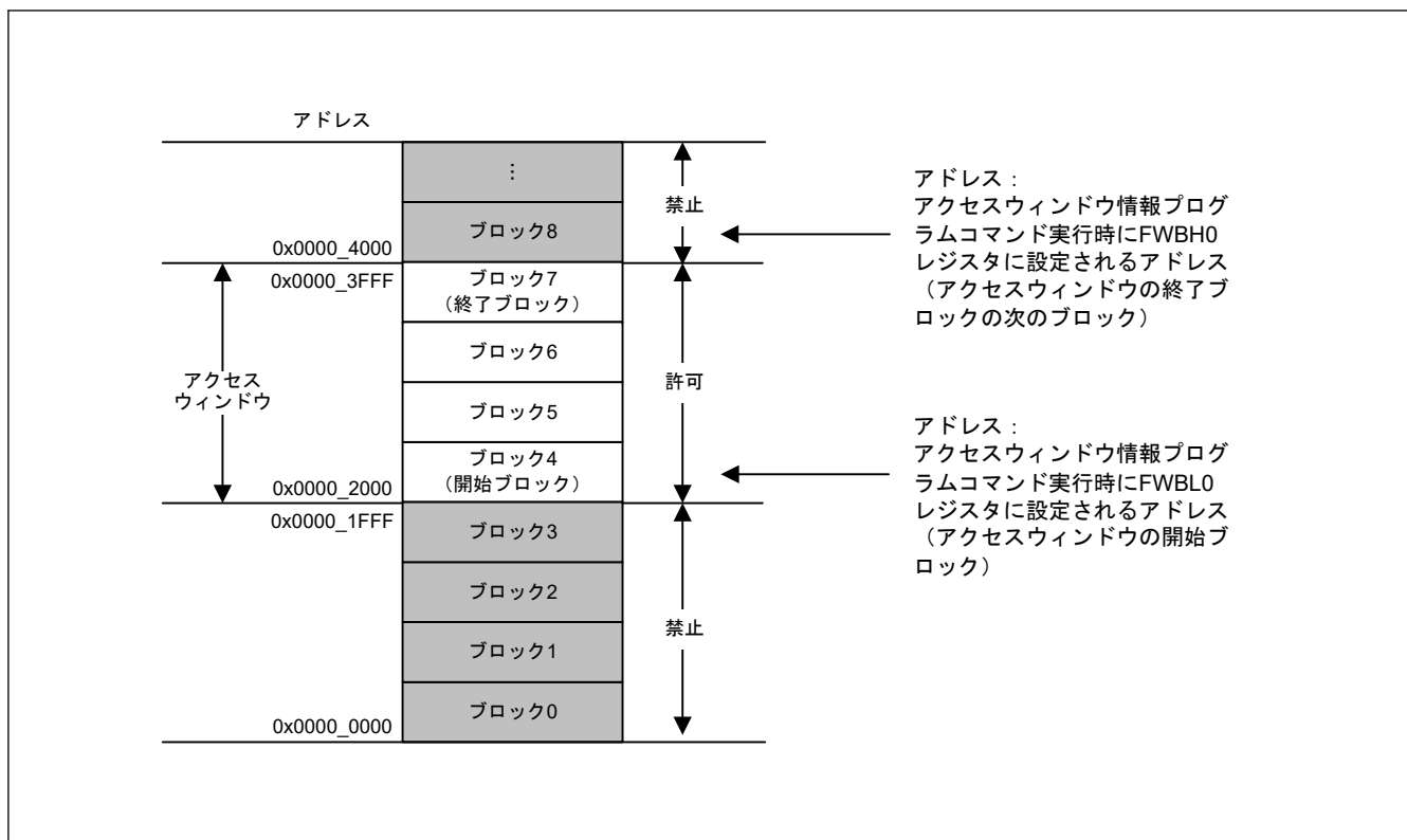
図 29.9 領域プロテクションの概要
