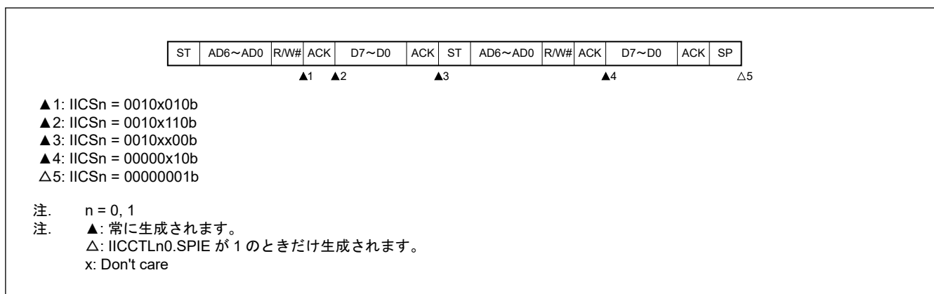
図 22.44 コードアクセス、不一致後のスレーブデバイスの動作（IICCTLn0.WTIM が 1 の場合）
