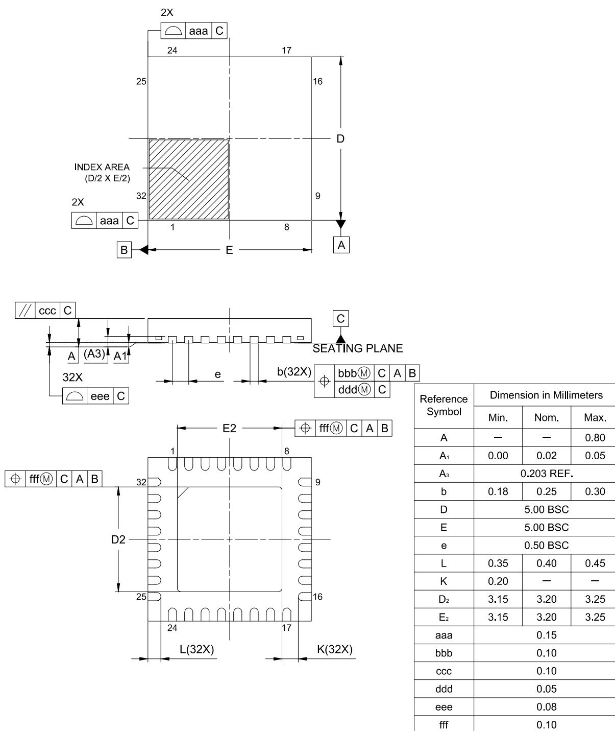
図 A2.4 HWQFN 32 ピン
