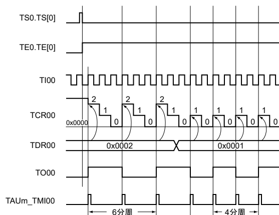
図 17.42 周波数分周器として動作する場合 (TMR00.OPIRQ = 1) の基本タイミング例
