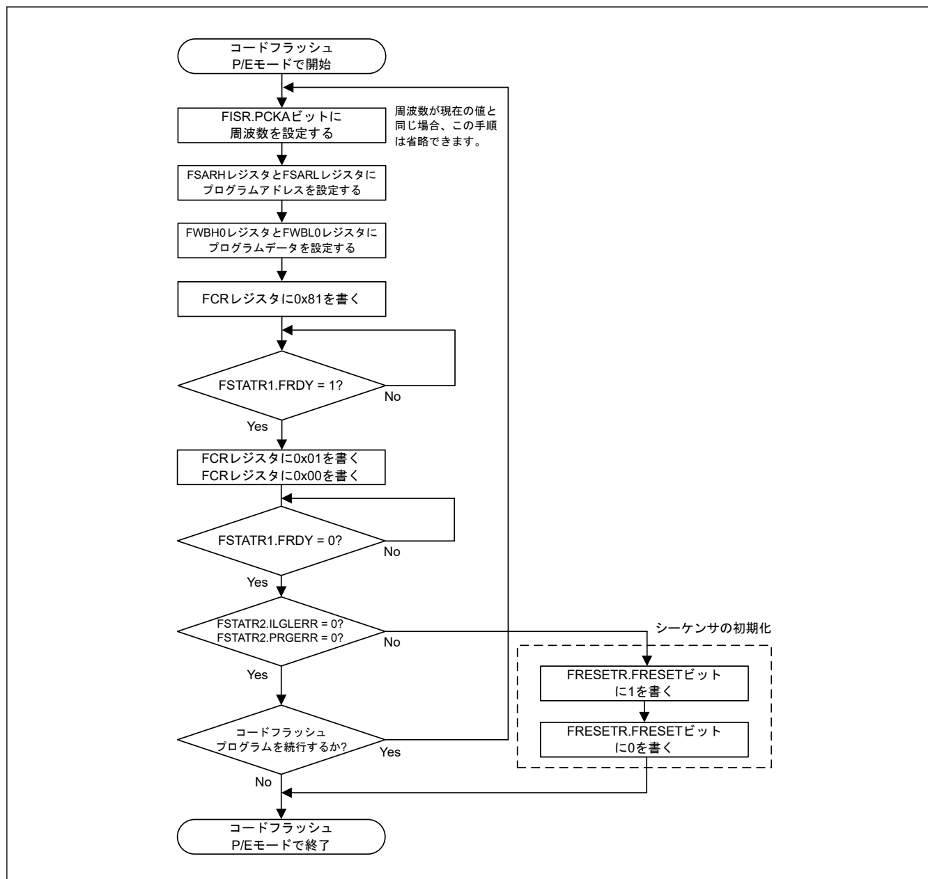
図 29.17 コードフラッシュのプログラム時のフローチャート
