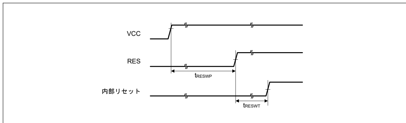
図 32.9 電源投入時リセット入力タイミング
