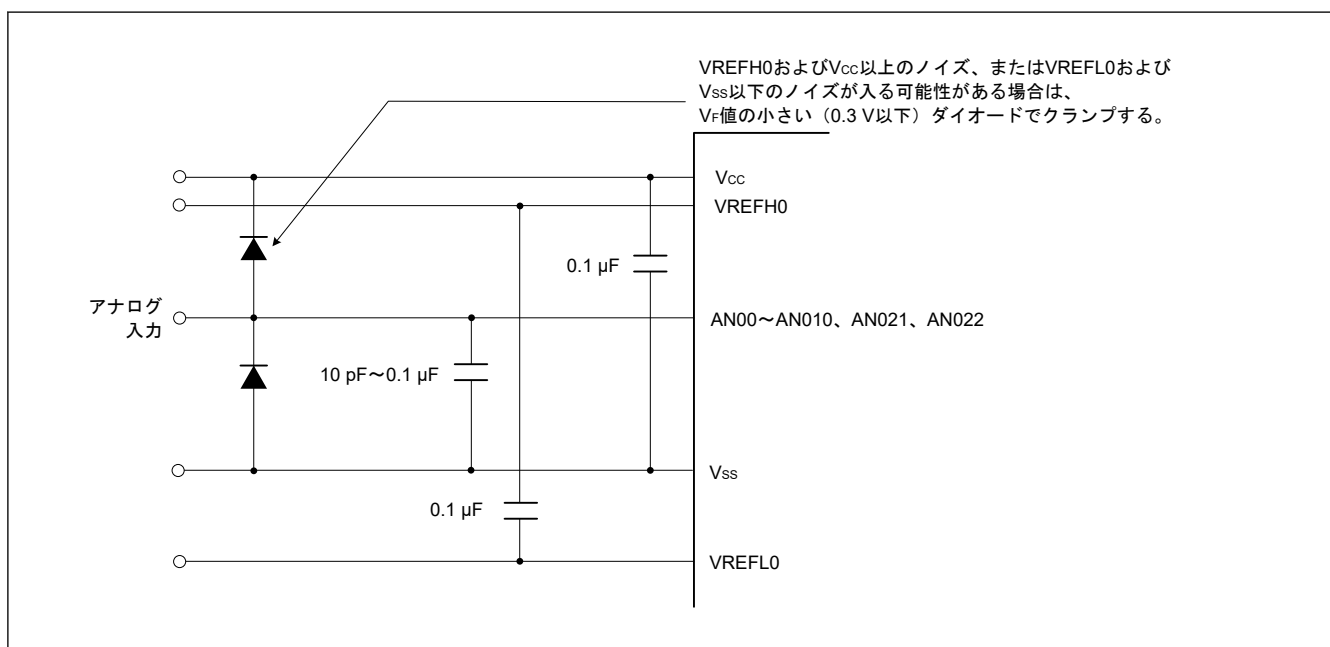
図 25.35 VCC 端子、VREFH0 端子、アナログ入力端子の接続
