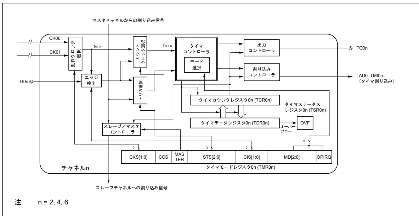
図 17.15 タイマアレユユニット 0 のチャンネル 2、4、6 の内部ブロック図
