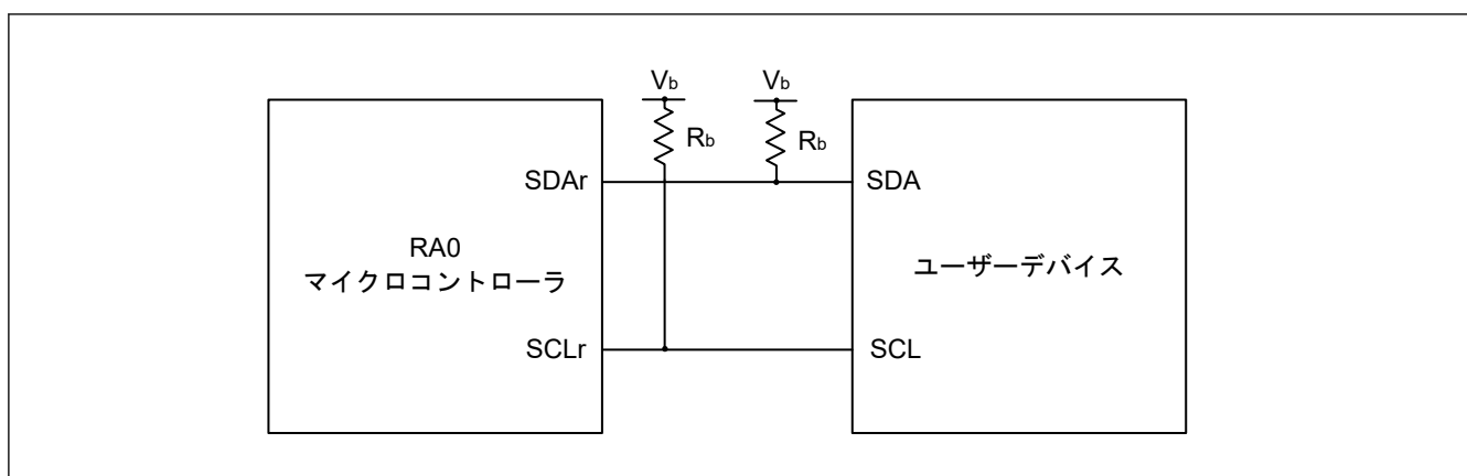
図 32.29 異なる電圧レベルで動作しているデバイスとの IIC 通信での接続
