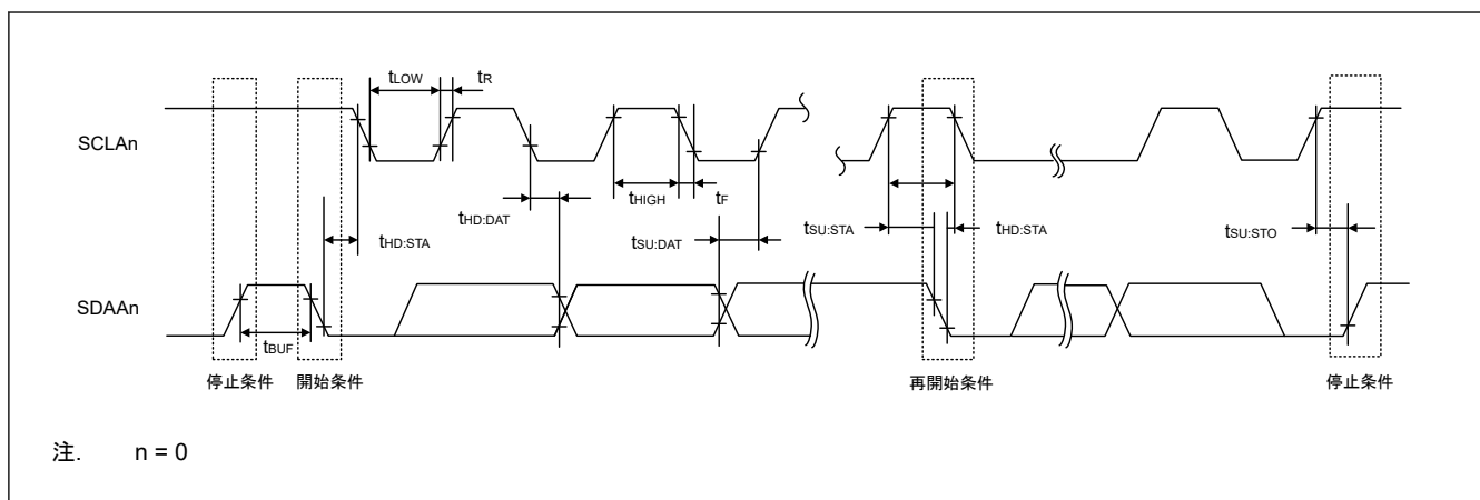
図 32.31 I 2 C シリアル転送タイミング
