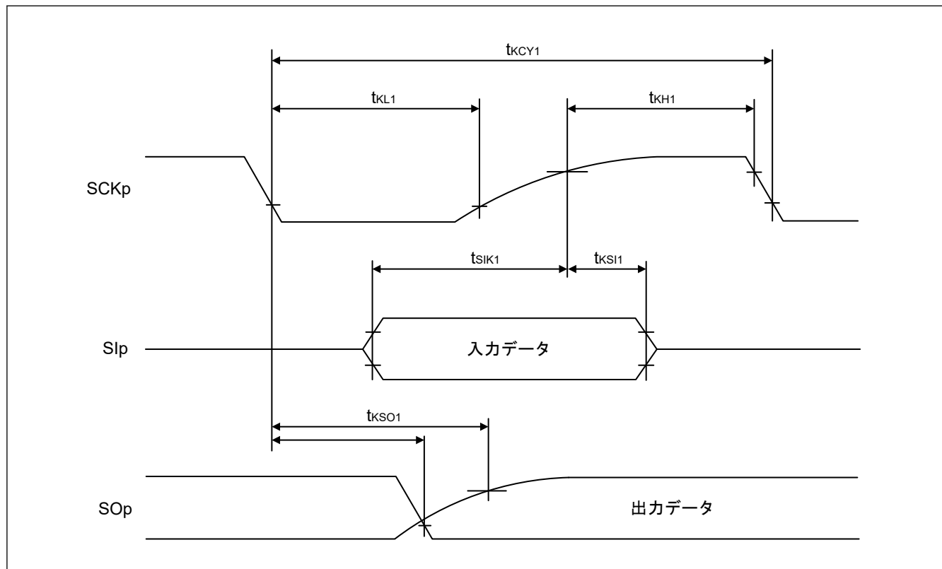
図 32.24 異なる電圧レベルで動作しているデバイスとのマスタモードでの簡易 SPI 通信でのシリアル転送のタイミング (SCRmn.DCP[1:0] = 00b または 11b の場合)
