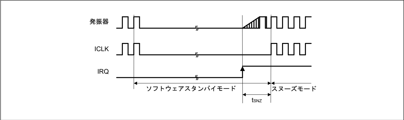
図 32.13 ソフトウェアスタンバイモードからスリープモードへの復帰タイミング
