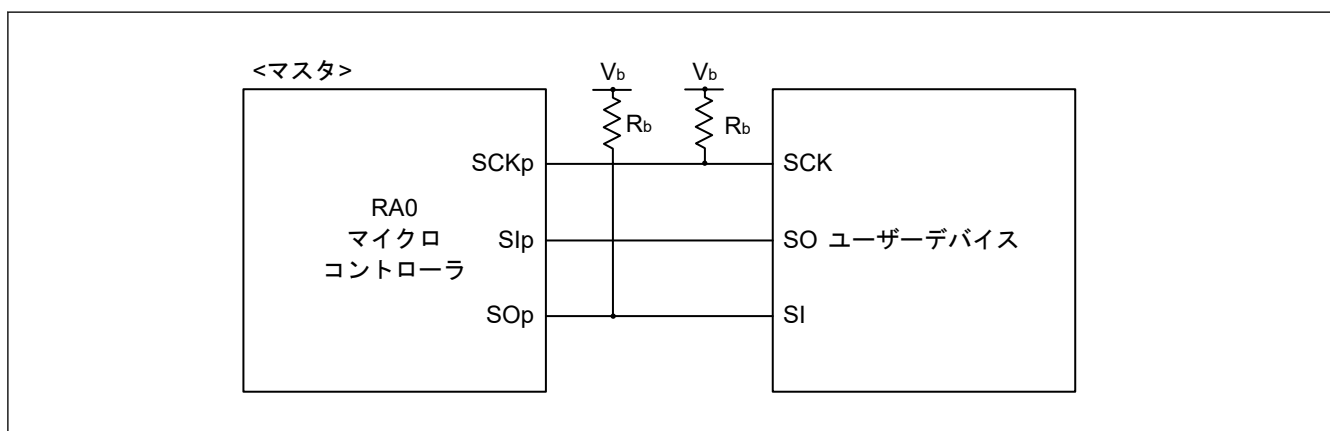
図 32.23 異なる電圧レベルで動作しているデバイスとの簡易 SPI 通信での接続
