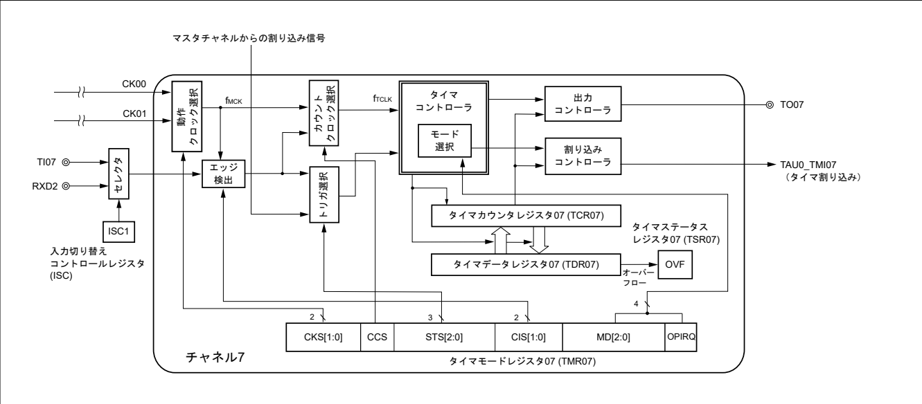
図 17.18 タイマアレユニツ 0 のチャンネル 7 の内部ブロック図
