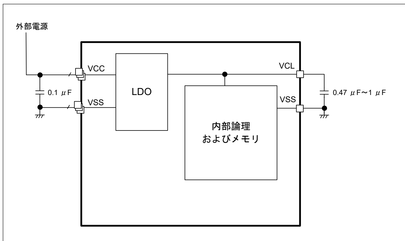
図 31.1 LDO モード設定
