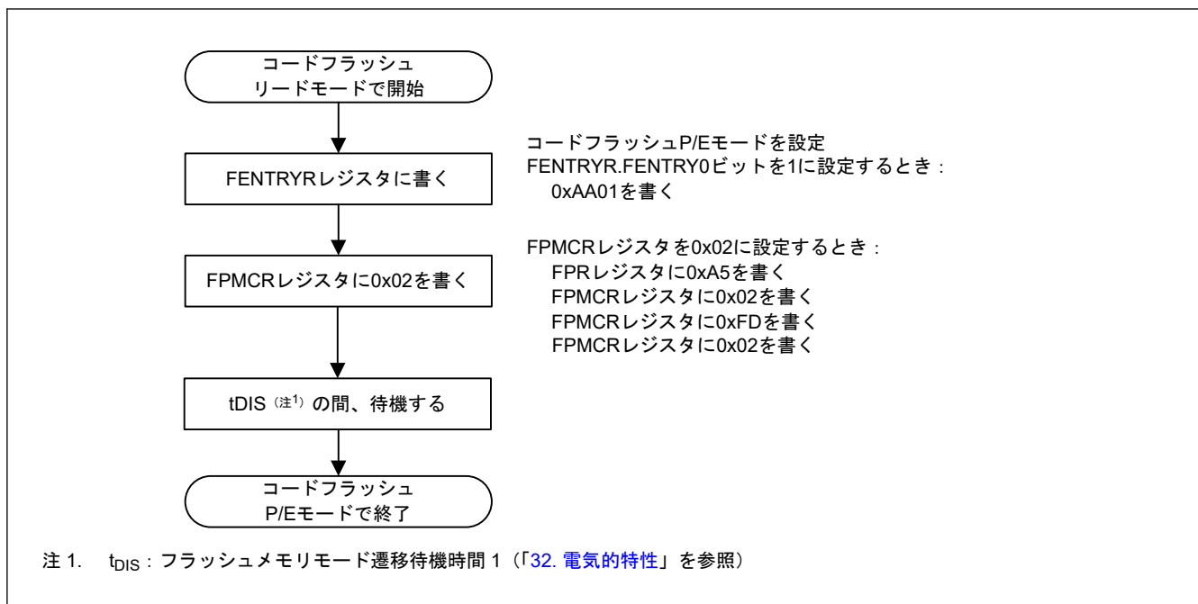
図 29.13 リードモードからコードフラッシュ P/E モードへの変更手順
