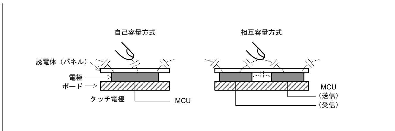
図 27.2 自己容量方式と相互容量方式
