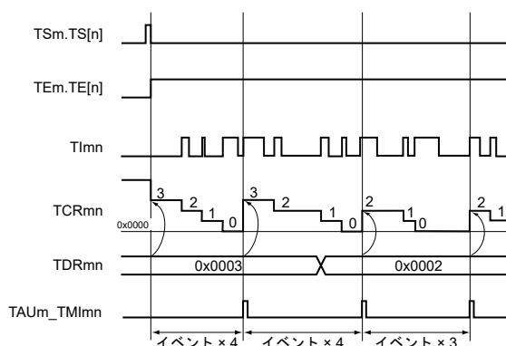
図 17.40 外部イベントカウンタとして動作する場合の基本タイミング例
