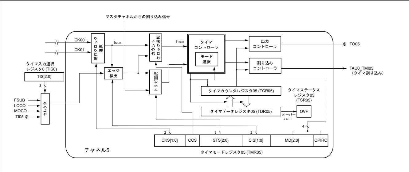
図 17.17 タイマアレユニツ 0 のチャンネル 5 の内部ブロック図
