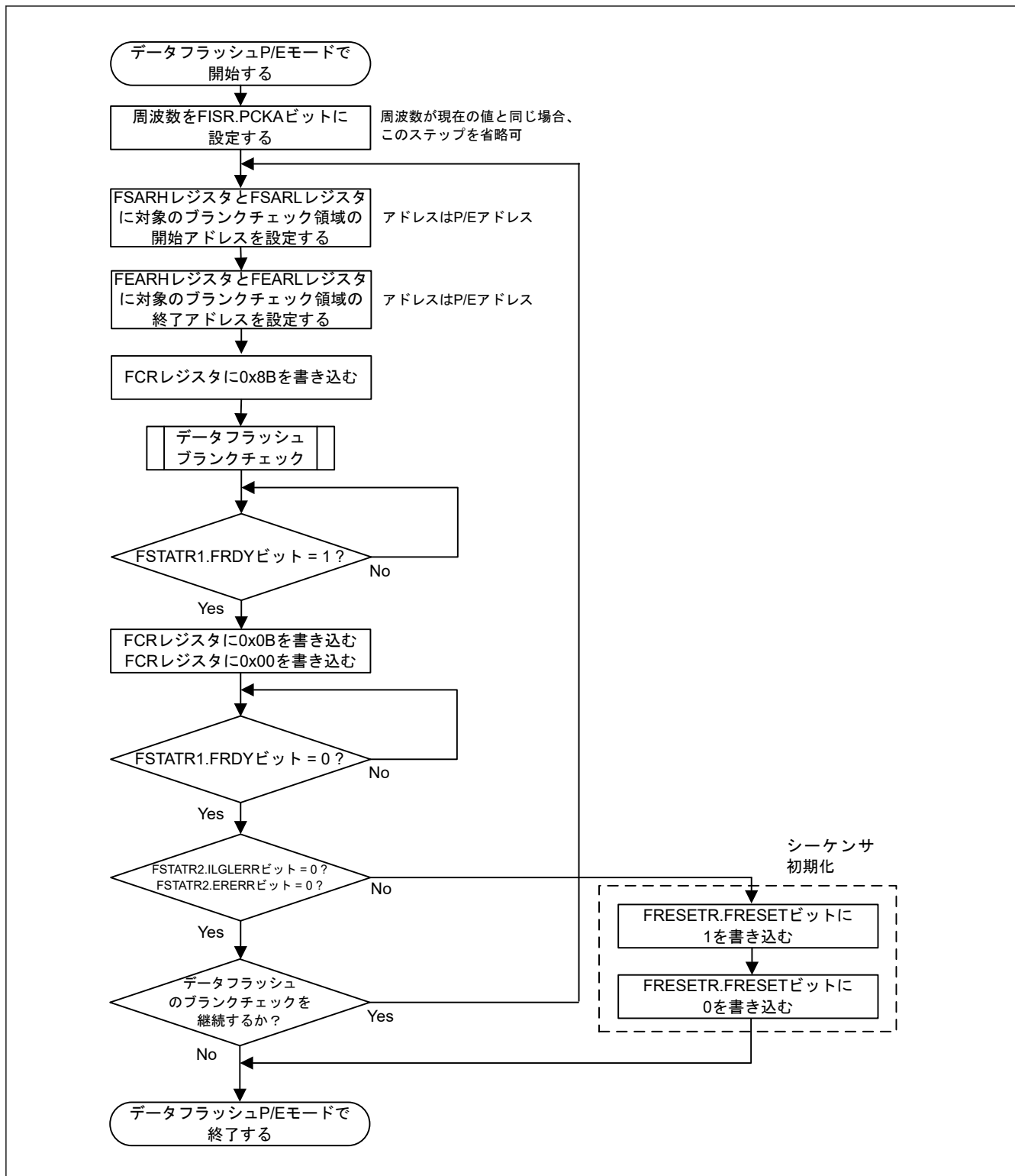
図 29.22 データフラッシュブランクチェック手順のフローチャート
