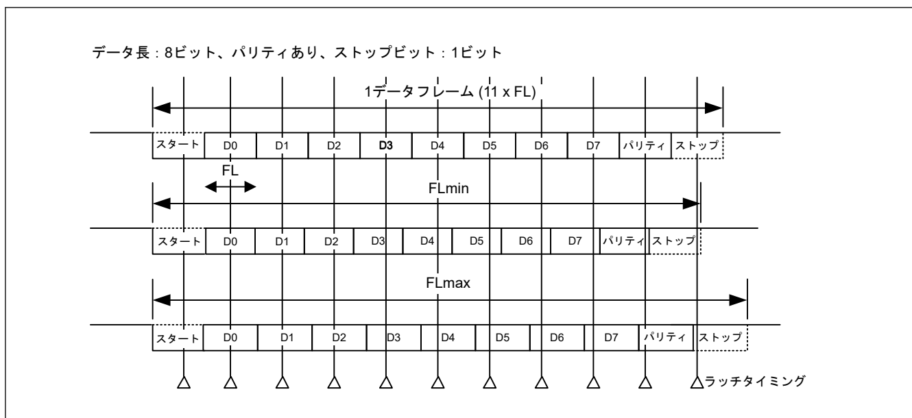
図 23.11 受信時の許容ポーレート範囲
