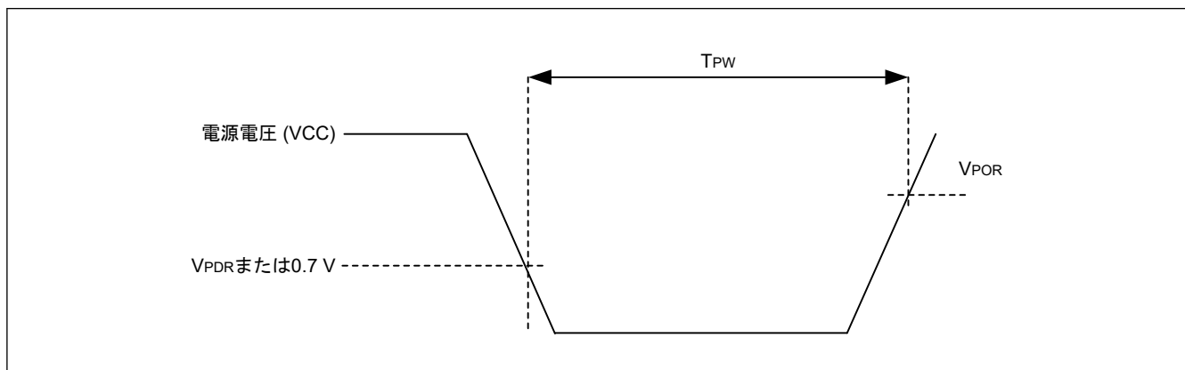
図 32.34 最小 VCC パルス幅
