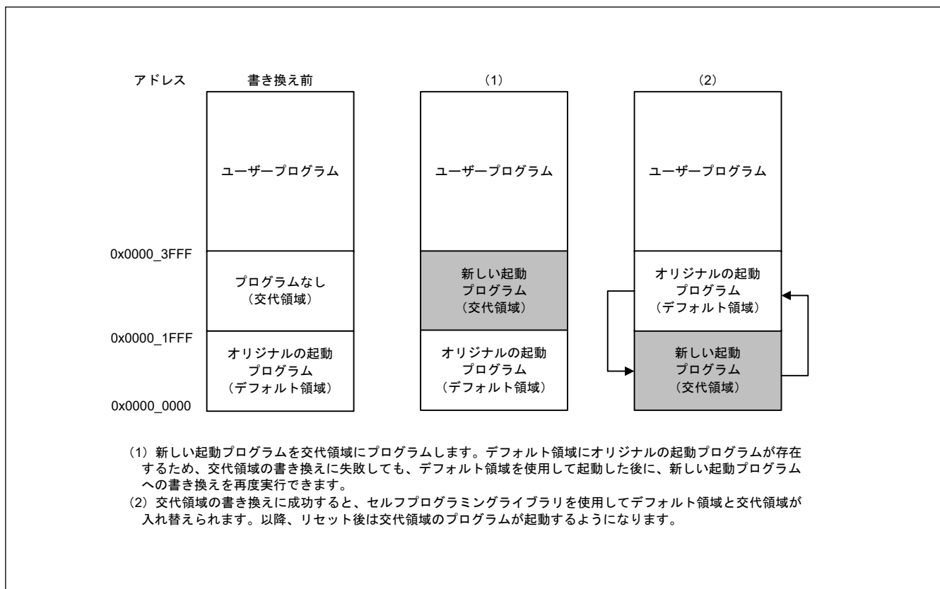
図 29.6 スタートアッププログラムプロテクションの概要
