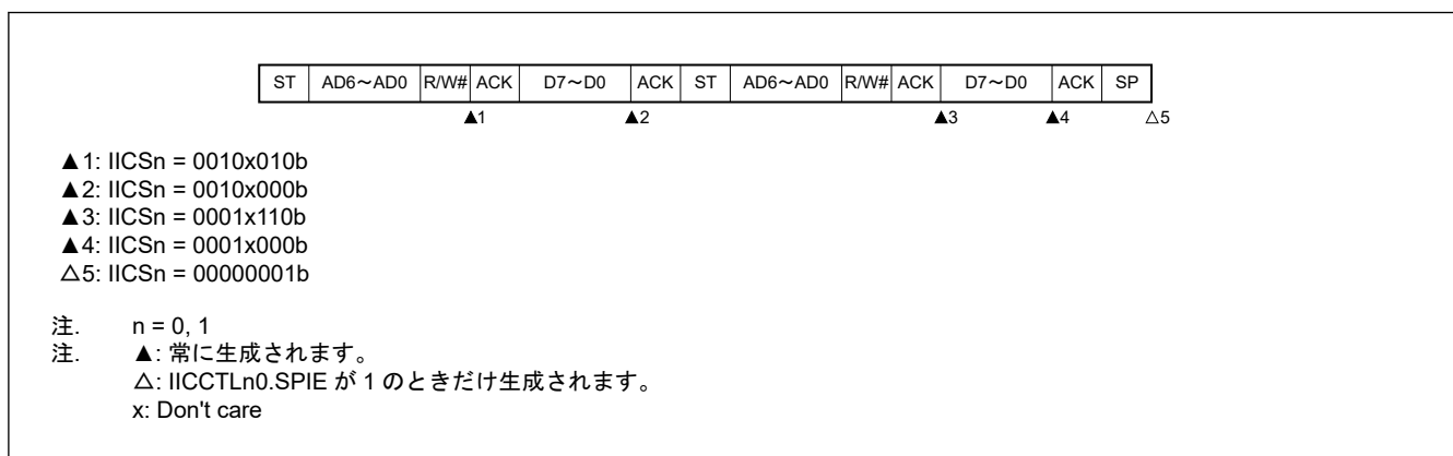
図 22.39 コードアクセス、SVAn との一致後のスレーブデバイスの動作 (IICCTLn0.WTIM が 0 の場合)
