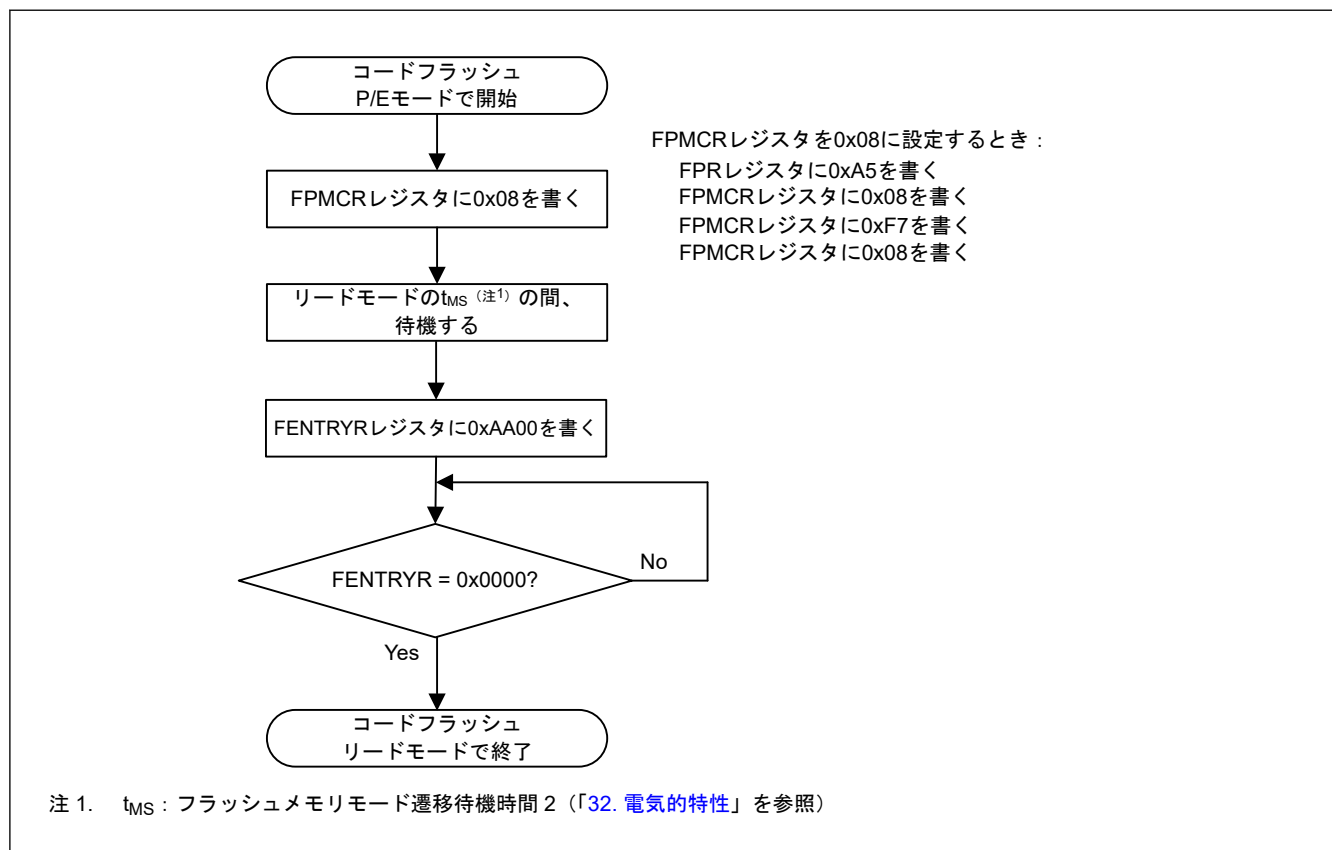
図 29.15 コードフラッシュ P/E モードからリードモードへの変更手順
