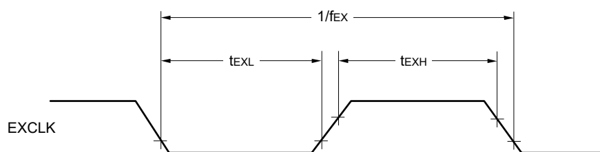
図 32.6 外部システムクロックタイミング
