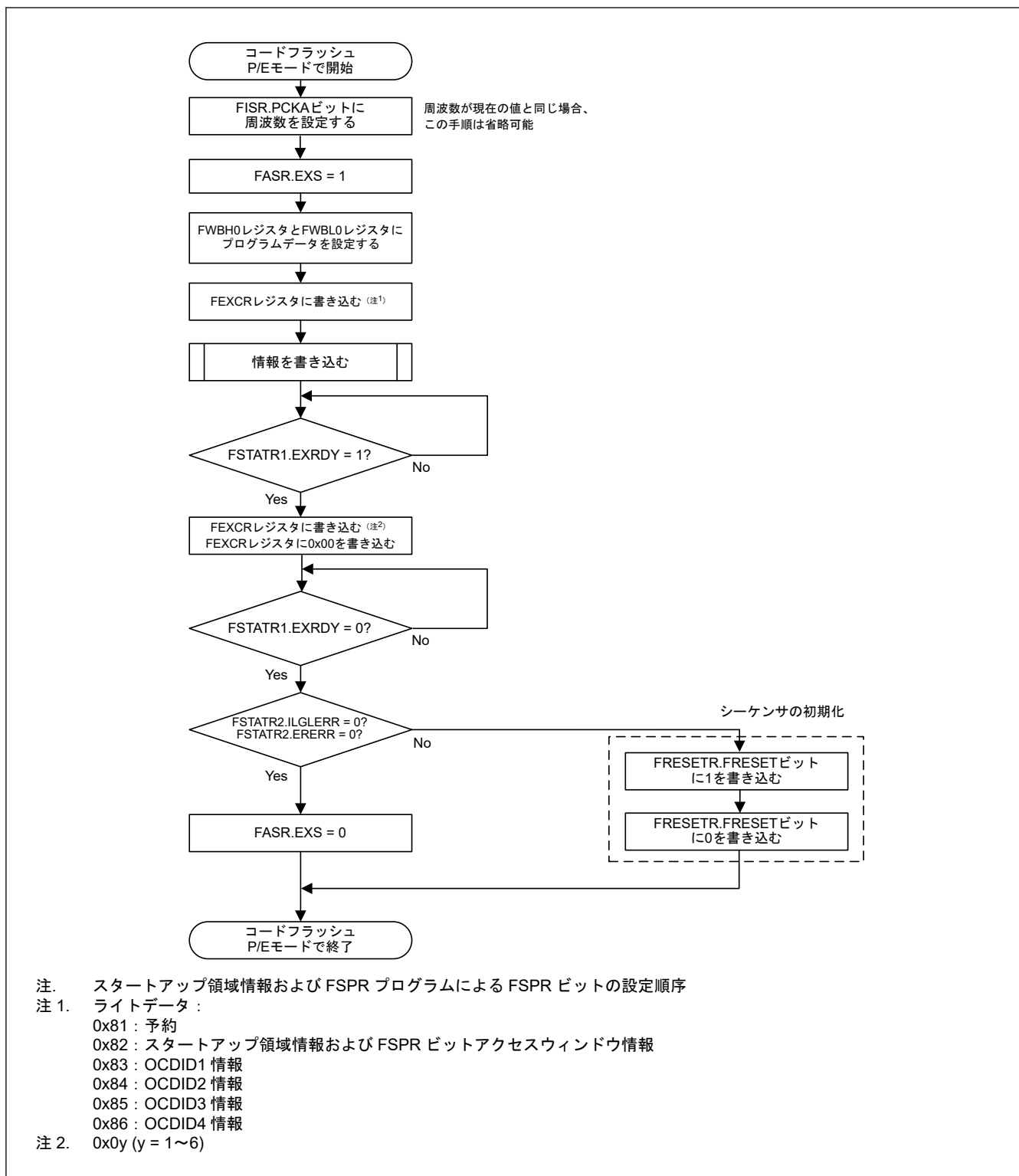
図 29.23 スタートアップ領域情報および FSPR プログラム/アクセスウィンドウ情報プログラム/OCDID 情報プログラムの手順を示す簡易フローチャート
