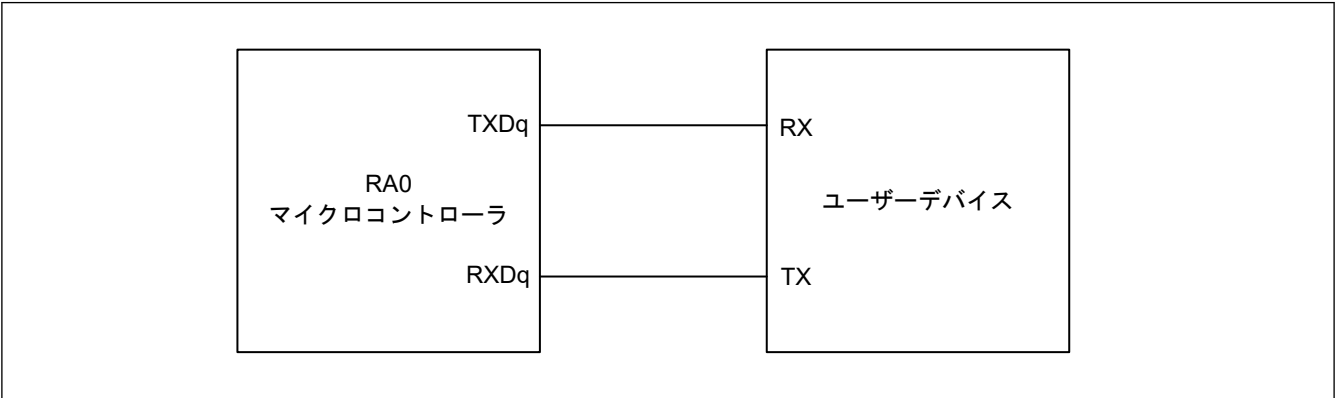
図 32.14 同じ電圧レベルで動作しているデバイスとの UART 通信での接続
