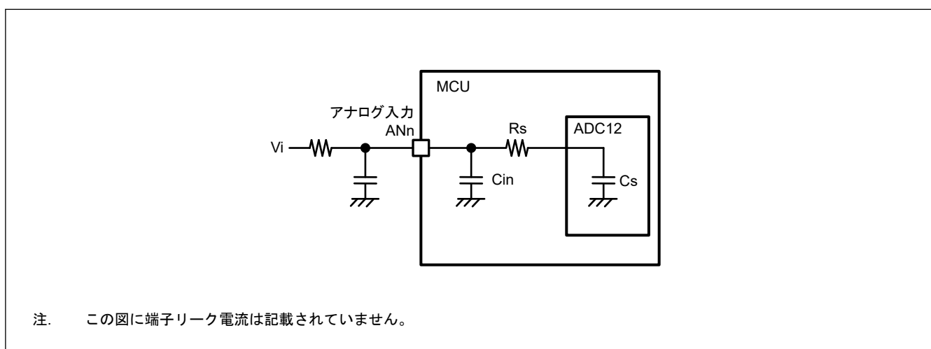
図 32.32 アナログ入力の等価回路
