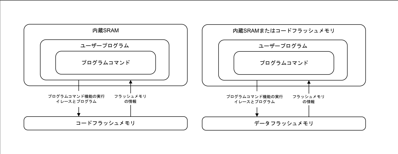
図 29.10 セルフプログラミングの概念
