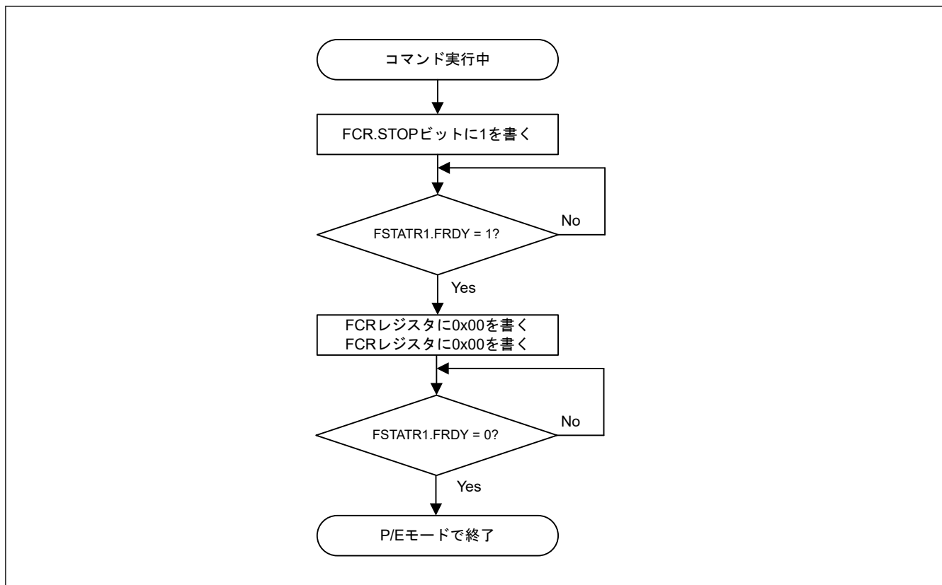
図 29.24 強制停止手順の簡易フローチャート
