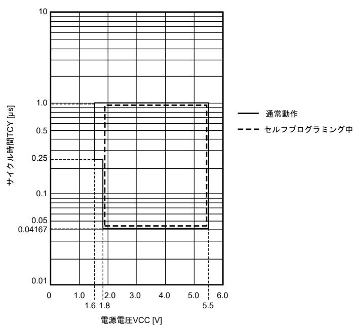
図 32.3 T_{CY} vs V_{CC} (Middle-speed モード)
