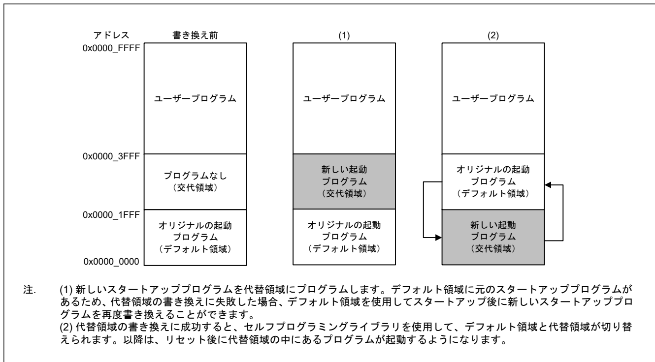
図 29.8 スタートアッププログラムプロテクションの概要
