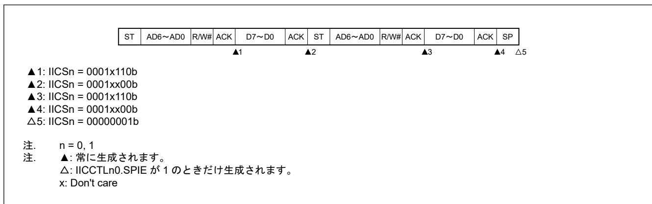
図 22.32 通常アクセス、SVAn との一致後のスレーブデバイスの動作 (IICCTLn0.WTIM が 1 の場合)
