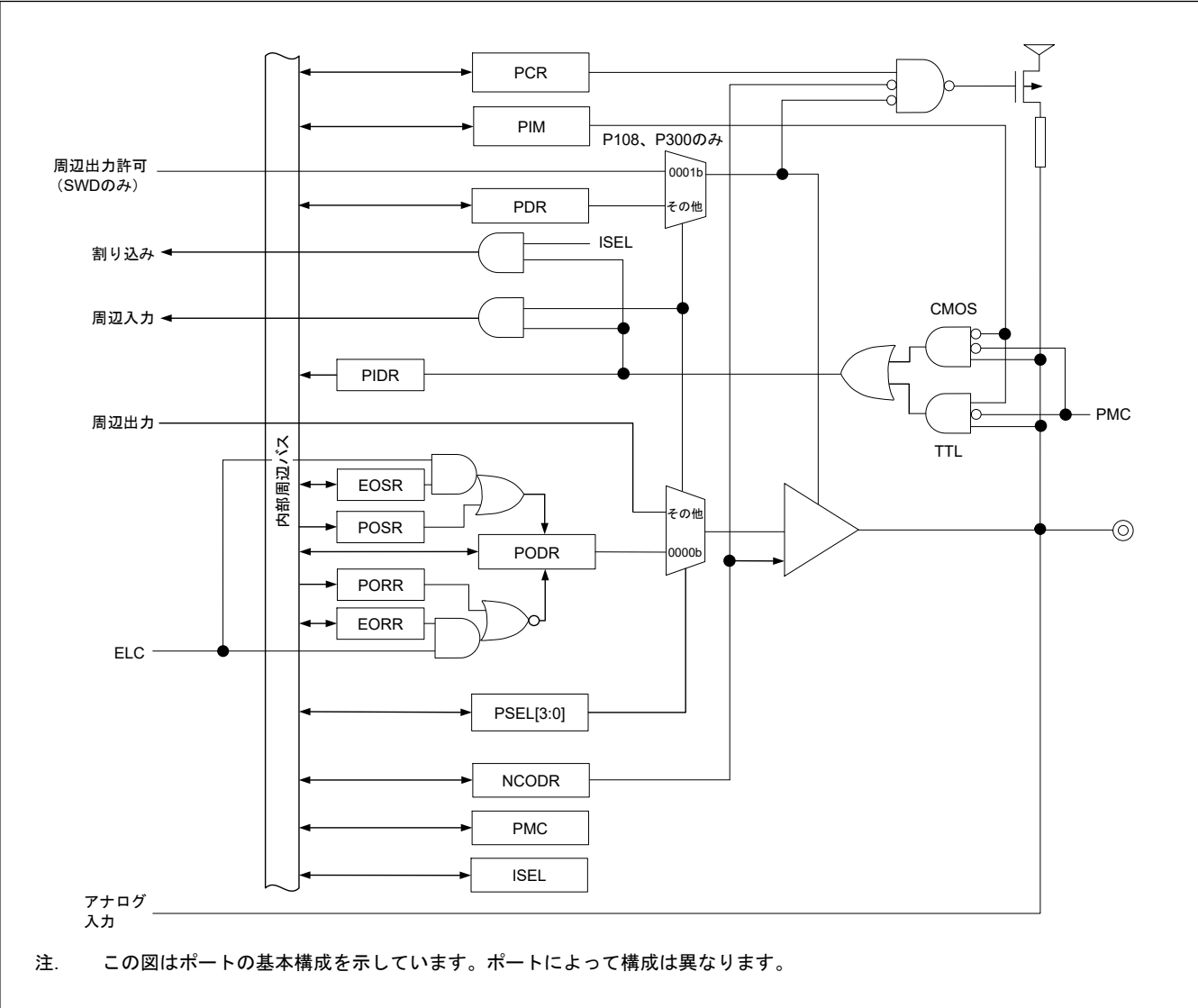
図 16.1 I/O ポートレジスタの接続図
