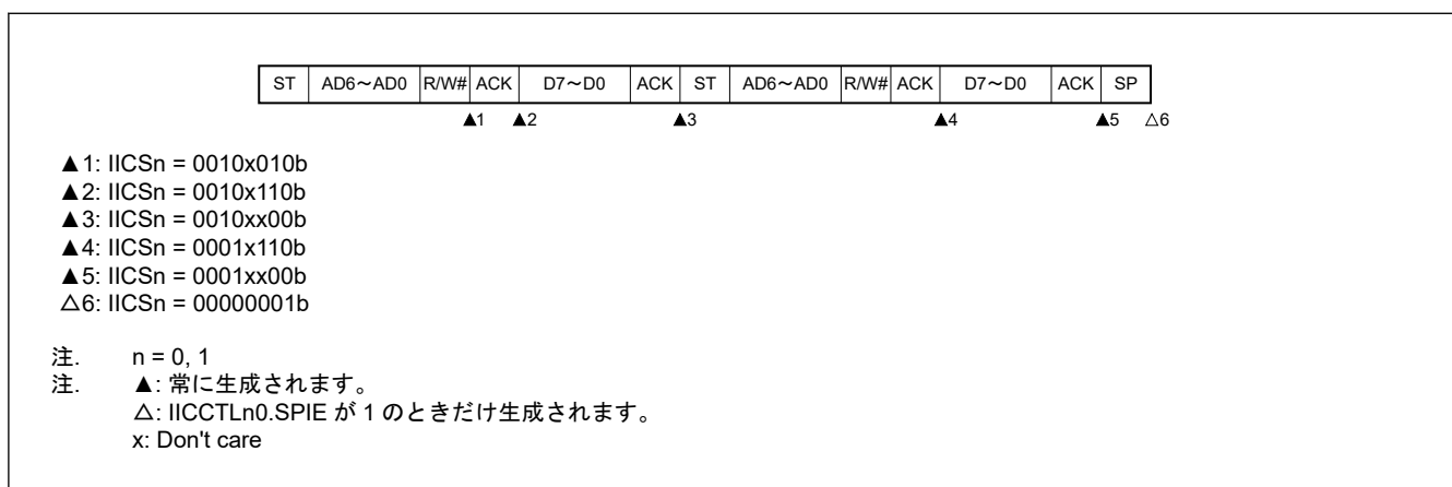
図 22.40 コードアクセス、SVAn との一致後のスレーブデバイスの動作 (IICCTLn0.WTIM が 1 の場合)
