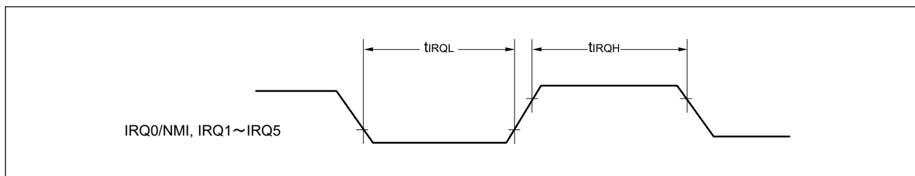
図 32.8 IRQ 割り込み入力タイミング
