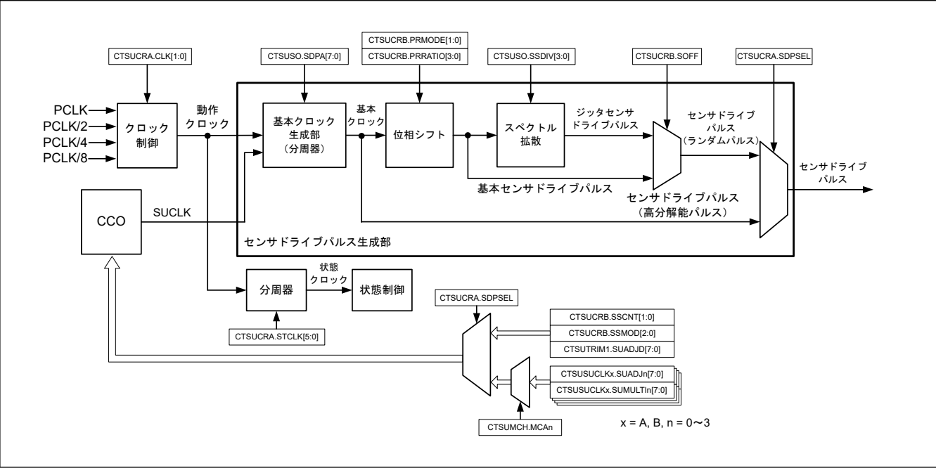
図 27.4 センサドライバパルスの生成
