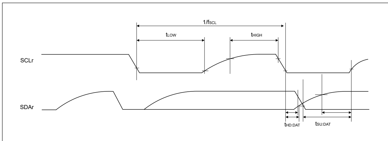
図 32.30 異なる電圧レベルで動作しているデバイスとの簡易 IIC 通信でのシリアル転送のタイミング
