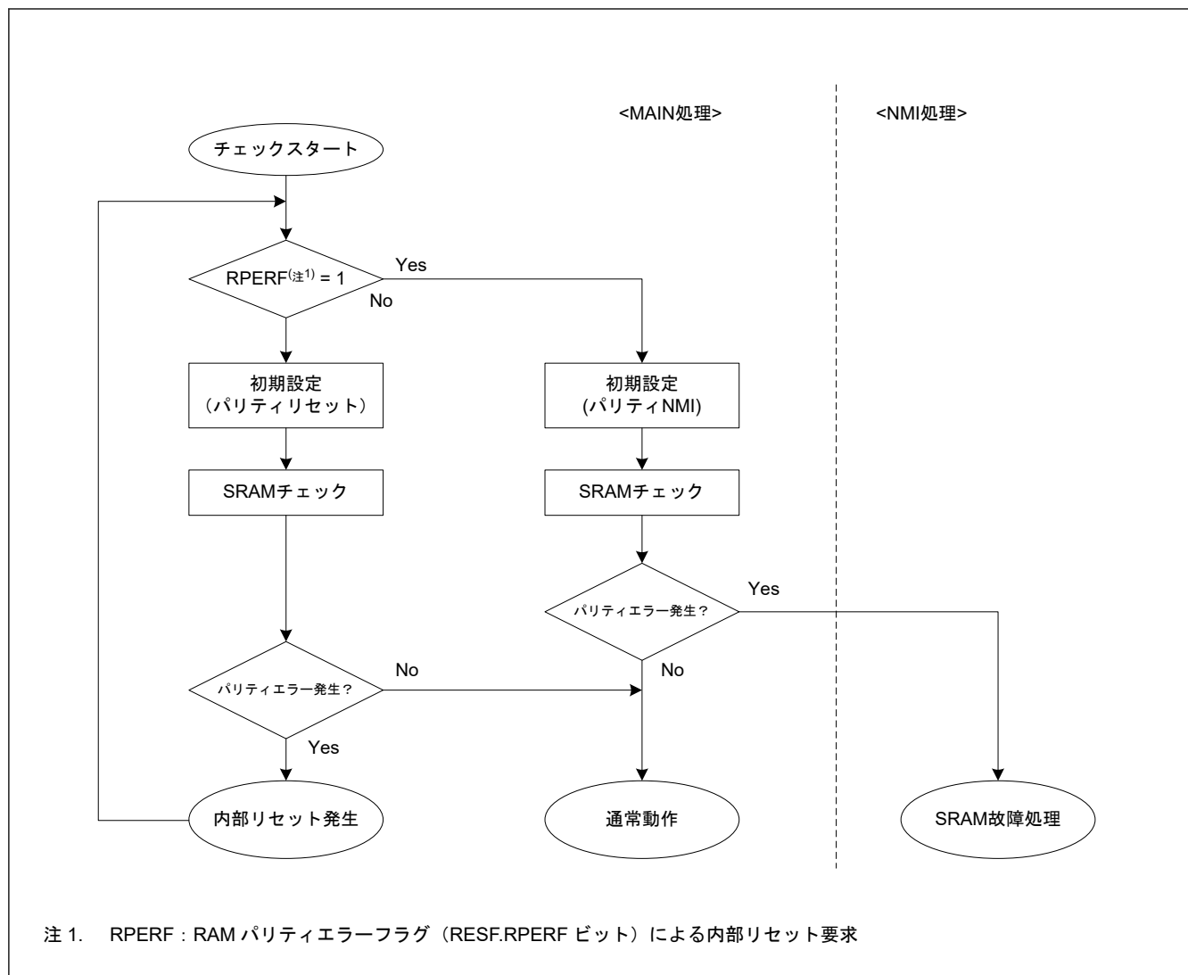
図 28.1 SRAM パリティリセット許可の場合の SRAM パリティチェックのフロー
