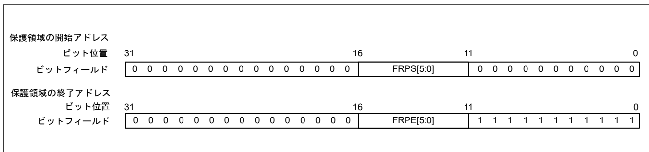
図 6.2 保護領域の開始アドレスと終了アドレス
