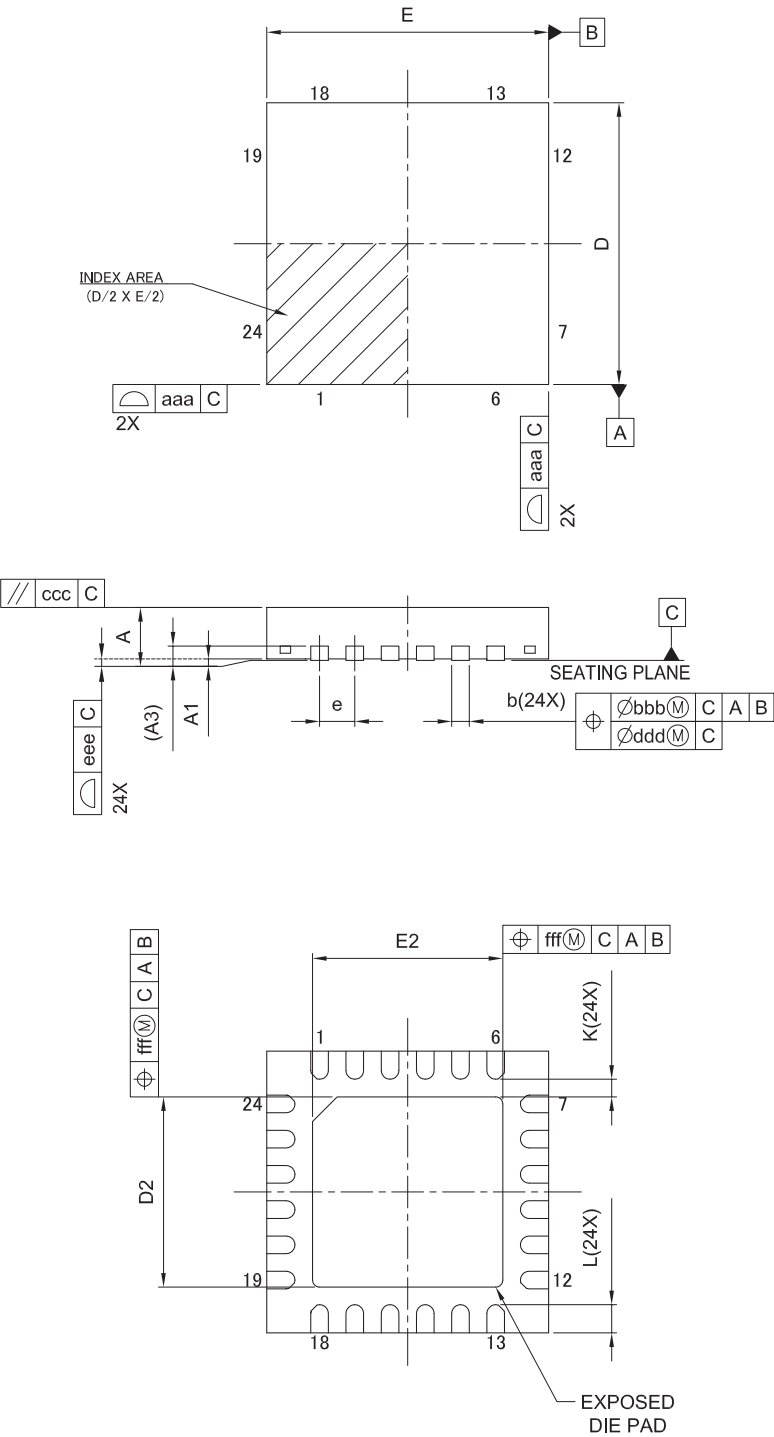
図 A2.5 HWQFN 24 ピン
