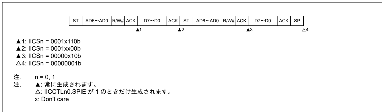
図 22.36 通常アクセス、不一致後のスレーブデバイスの動作 (IICCTLn0.WTIM が 1 の場合)
