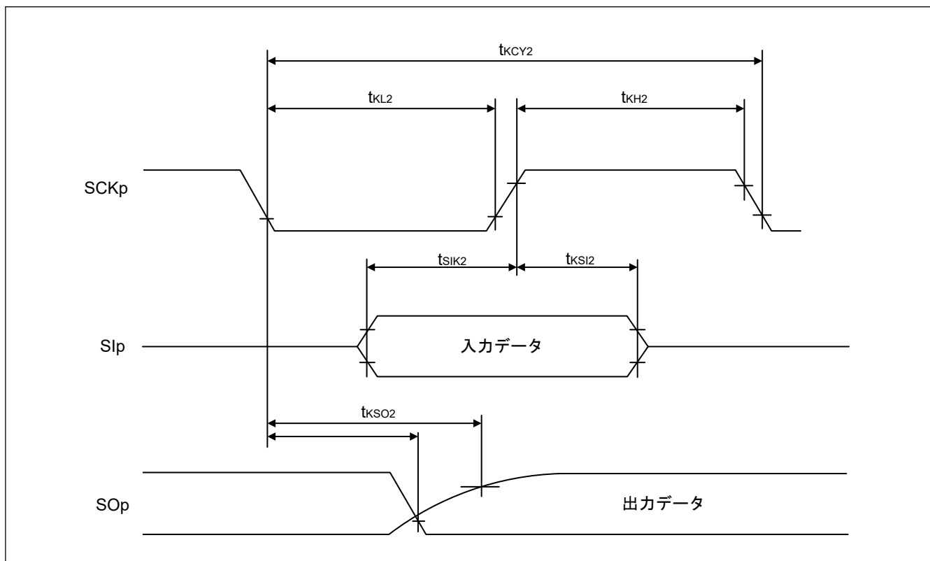
図 32.27 異なる電圧レベルで動作しているデバイスとのスレープモードでの簡易 SPI 通信でのシリアル転送のタイミング (SCRmn.DCP[1:0] = 00b または 11b の場合)
