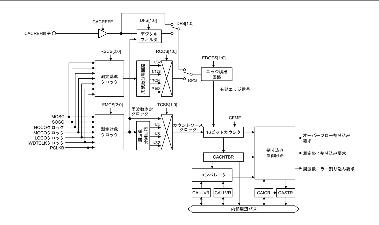
図 10.1 CAC のブロック図
