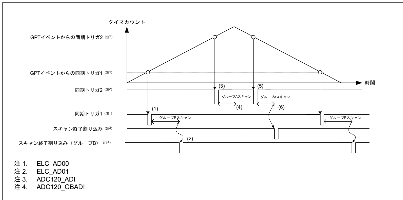
図 30.15 グループスキャンモードでダブルトリガモードを使用する場合の基本動作例 (ELC からの同期トリガ使用時)
