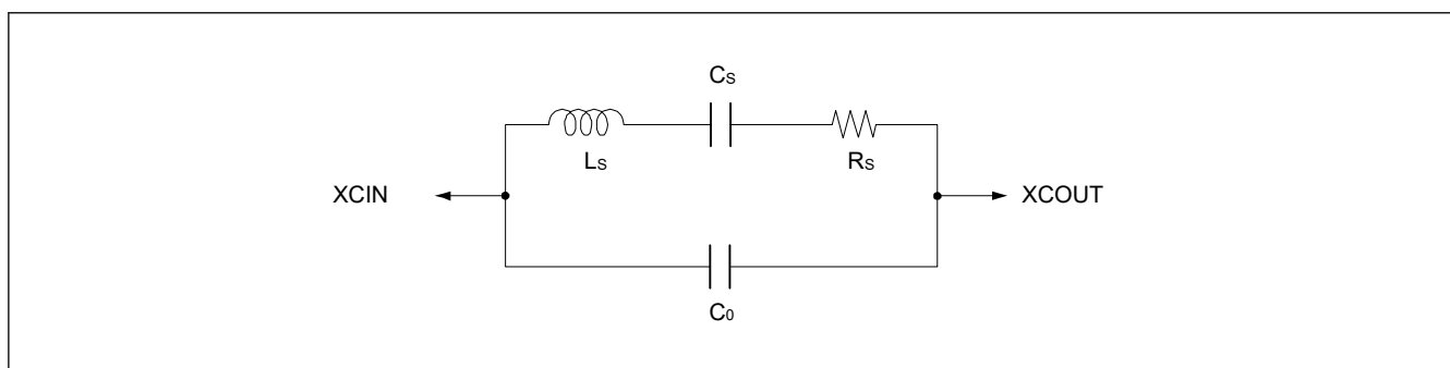
図 9.9 32.768 kHz 水晶振動子の等価回路
