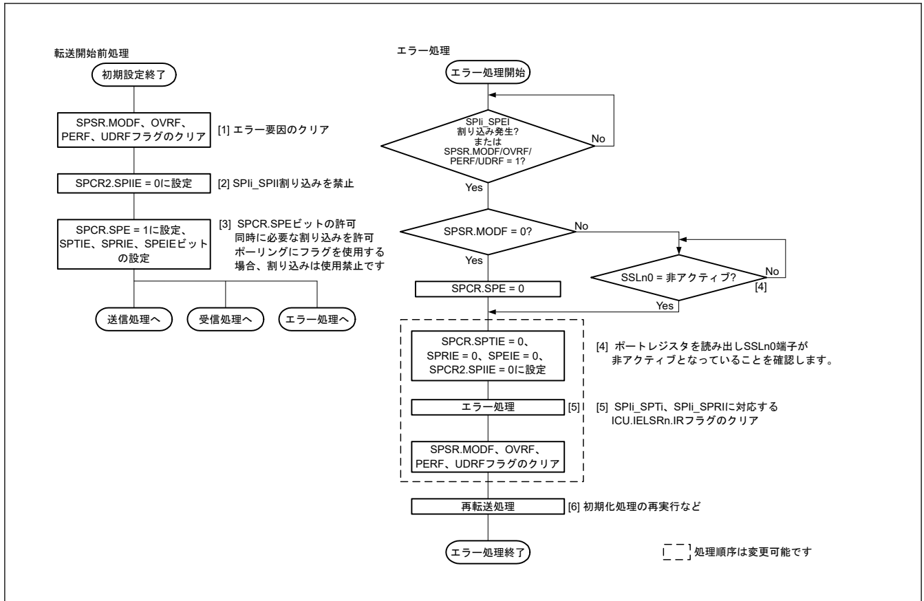
図 28.35 マスタモードでのエラー処理フロー
