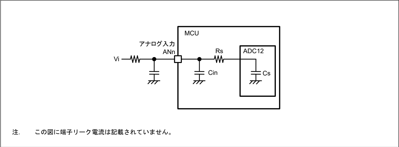
図 41.38 アナログ入力の等価回路
