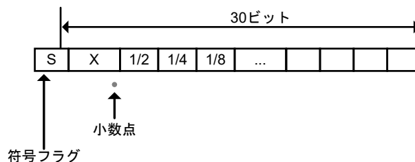
図 37.2 固定小数点モードでの Q フォーマットの例
