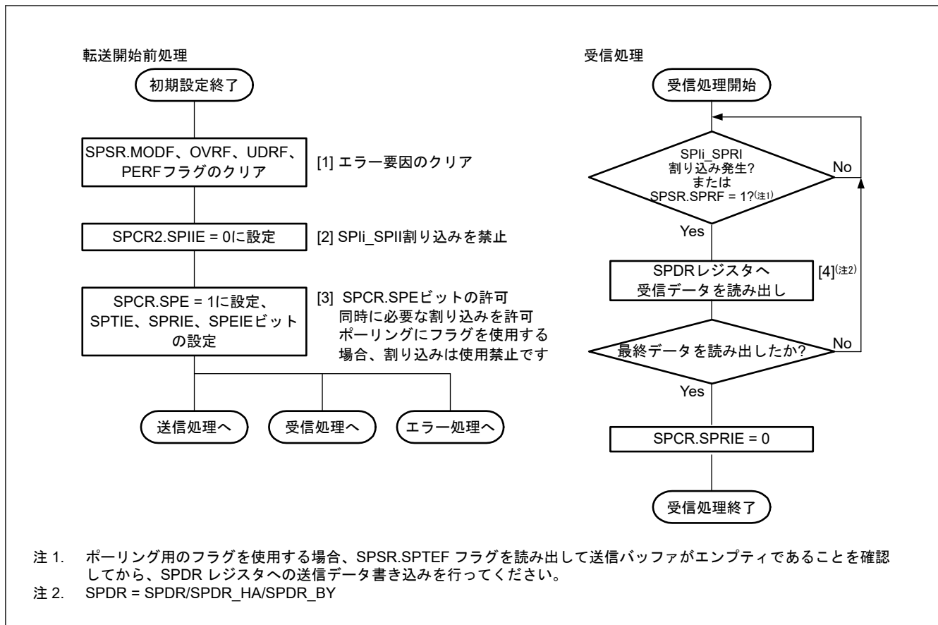
図 28.38 スレープモードでの受信手順
