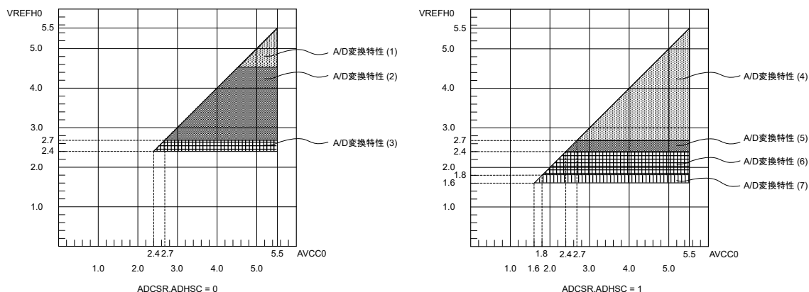
図 41.37 AVCC~VREFH0 電圧範囲
