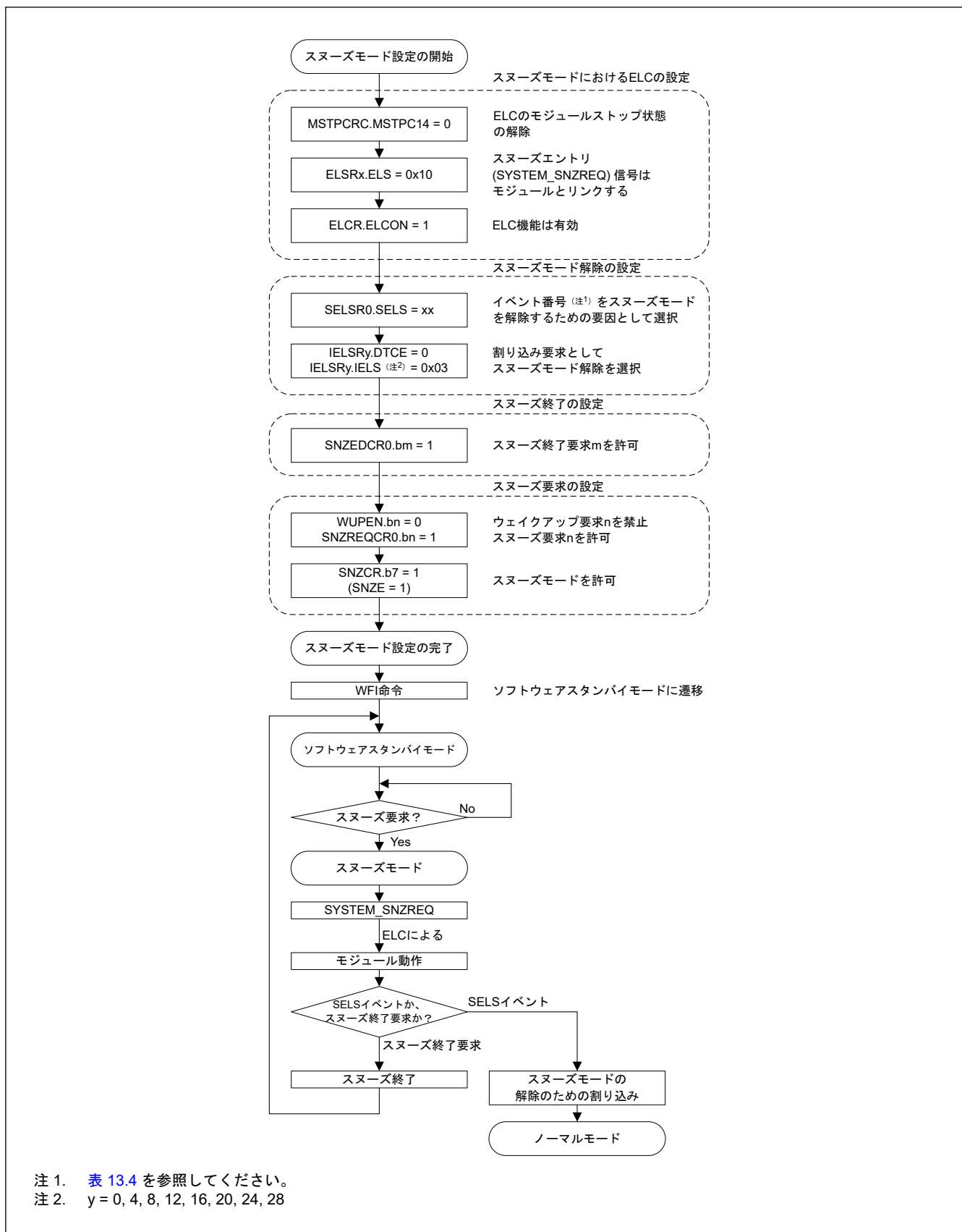
図 11.10 スリープモードで ELC を使用するための設定例
