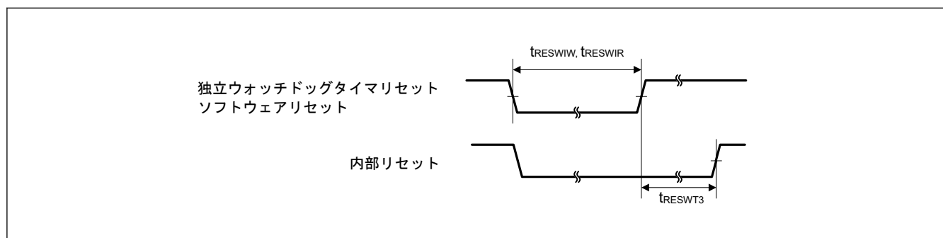
図 41.10 リセット入力タイミング (2)
