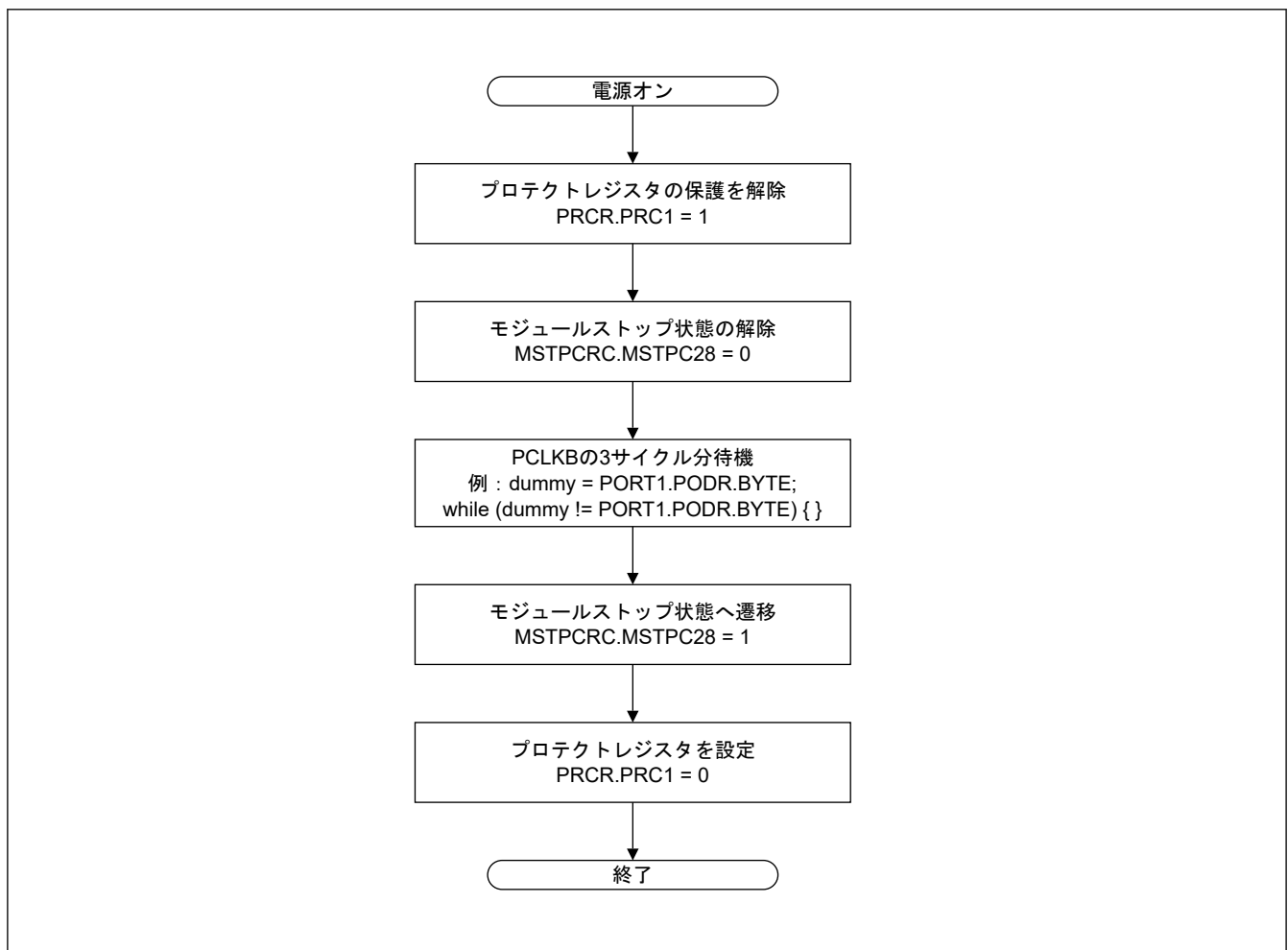
図 11.12 未使用回路の初期設定フロー例
