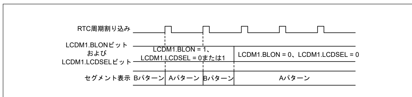
図 36.4 点滅表示から A パターン表示への切り替え動作
