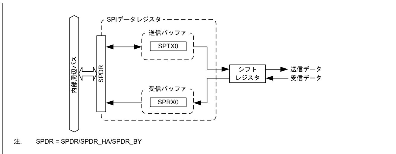
図 28.2 SPDR/SPDR_HA/SPDR_BY の構成
