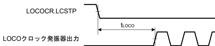
図 41.4 LOCO クロック発振開始タイミング
