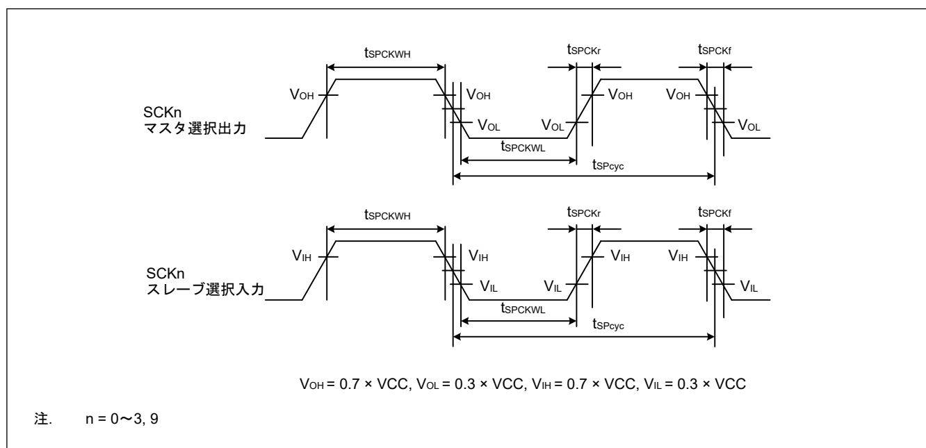
図 41.22 SCI 簡易 SPI モードクロックタイミング
