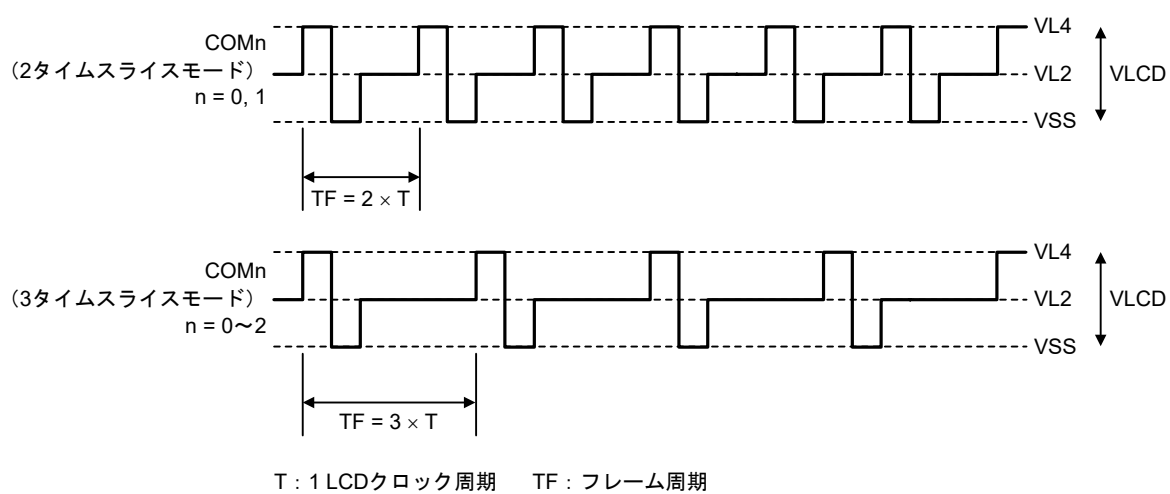
図 36.17 共通信号波形 (1/2)
