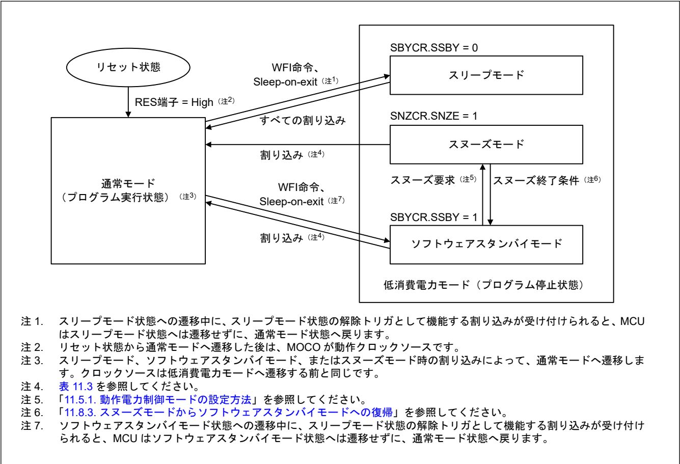
図 11.1 低消費電力モードの遷移
