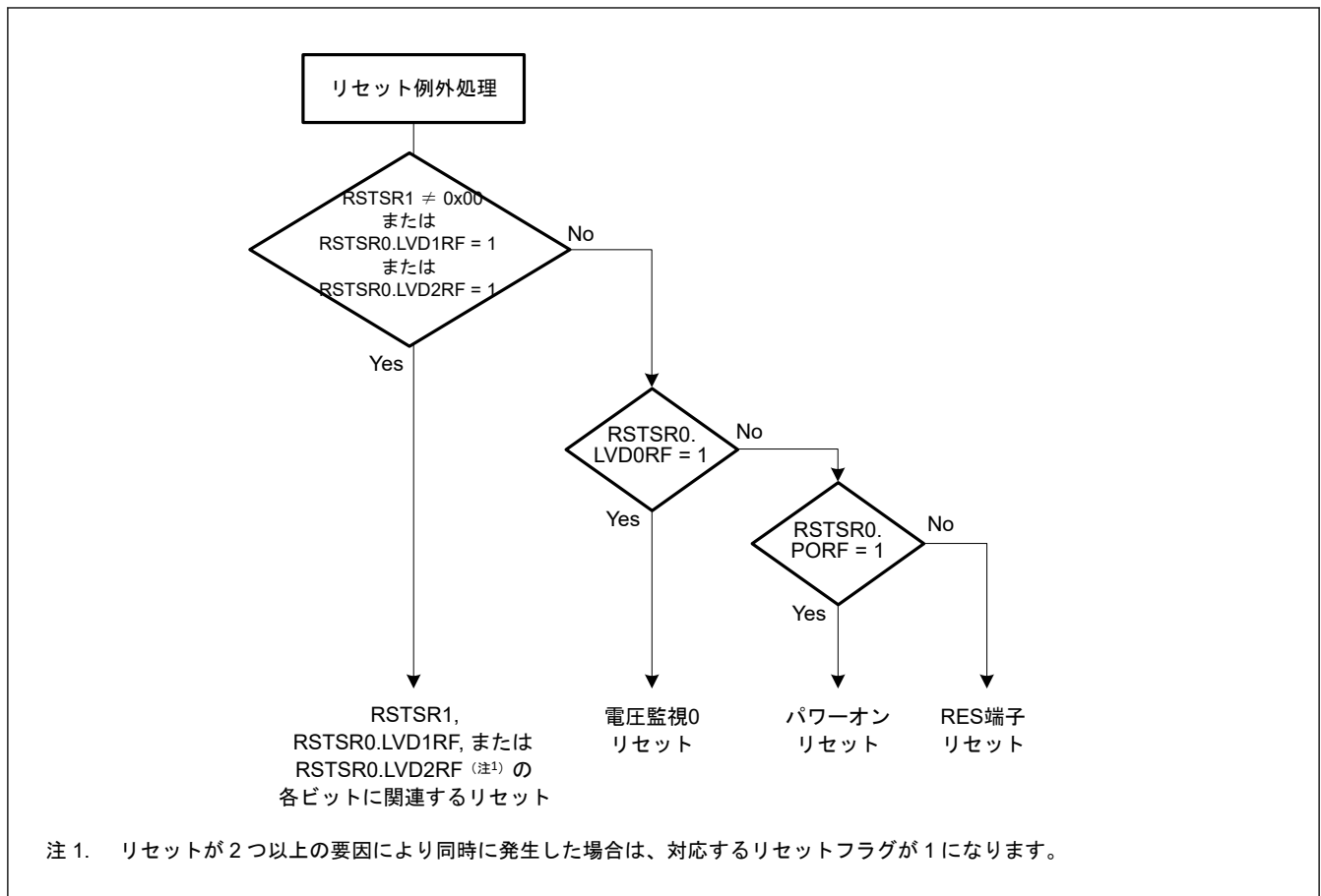
図 6.4 リセット発生要因の判定フロー例
