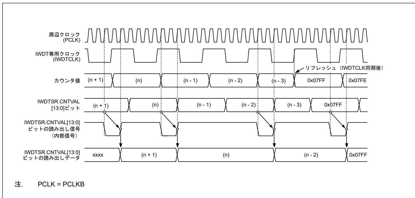
図 25.5 IWDT ダウンカウンタ値の読み出し処理 (OFS0.IWDTCKS[3:0] = 0000b、OFS0.IWDTTOS[1:0] = 11b の場合)
