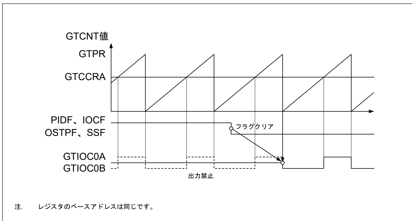
図 19.3 GPT 端子出力の出力禁止状態の解除タイミング
