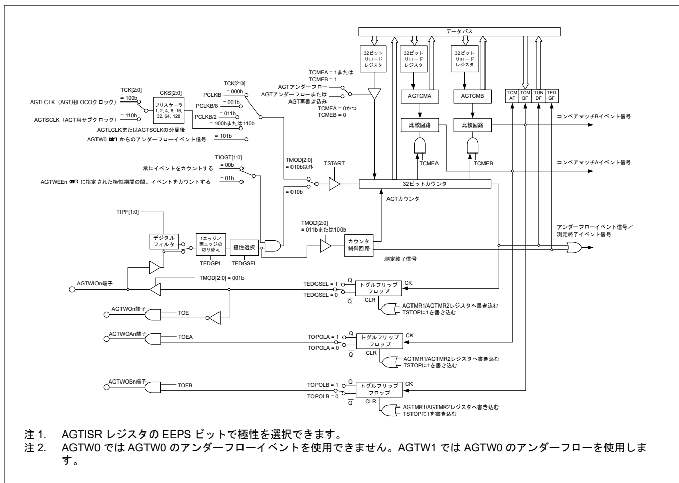
図 22.1 AGTW のブロック図
