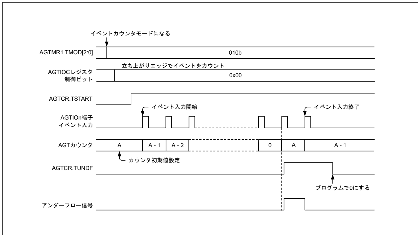
図 21.8 イベントカウンタモードでの動作例 1
