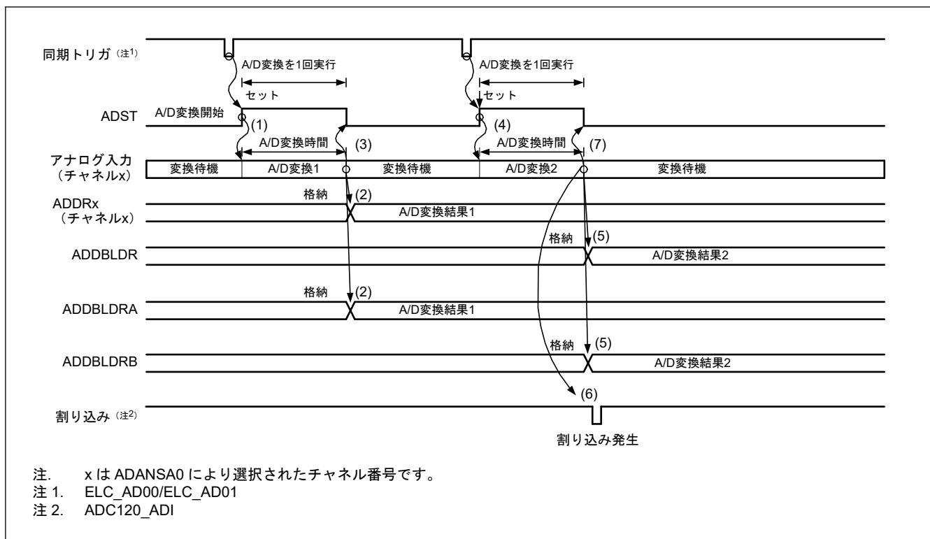
図 30.11 アナログ入力 (チャンネル x) と ELC_AD00/ELC_AD01 の重複選択時のダブルトリガモード拡張動作例
