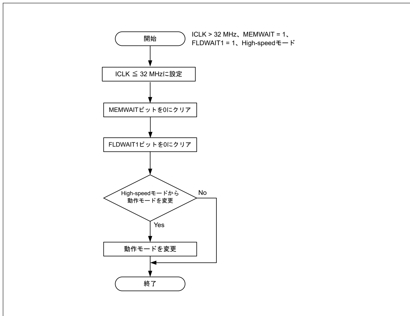
図 9.4 ICLK &gt; 32 MHz から ICLK ≤ 32 MHz に設定する場合
