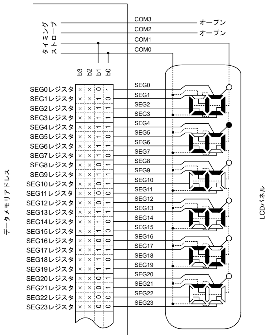
図 36.26 2 タイムスライス LCD パネルの接続例
