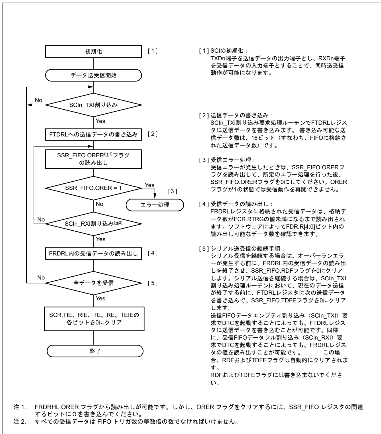
図 26.46 クロック同期式モードにおけるシリアル同時送受信動作のフローチャート例（FIFO 選択時）
