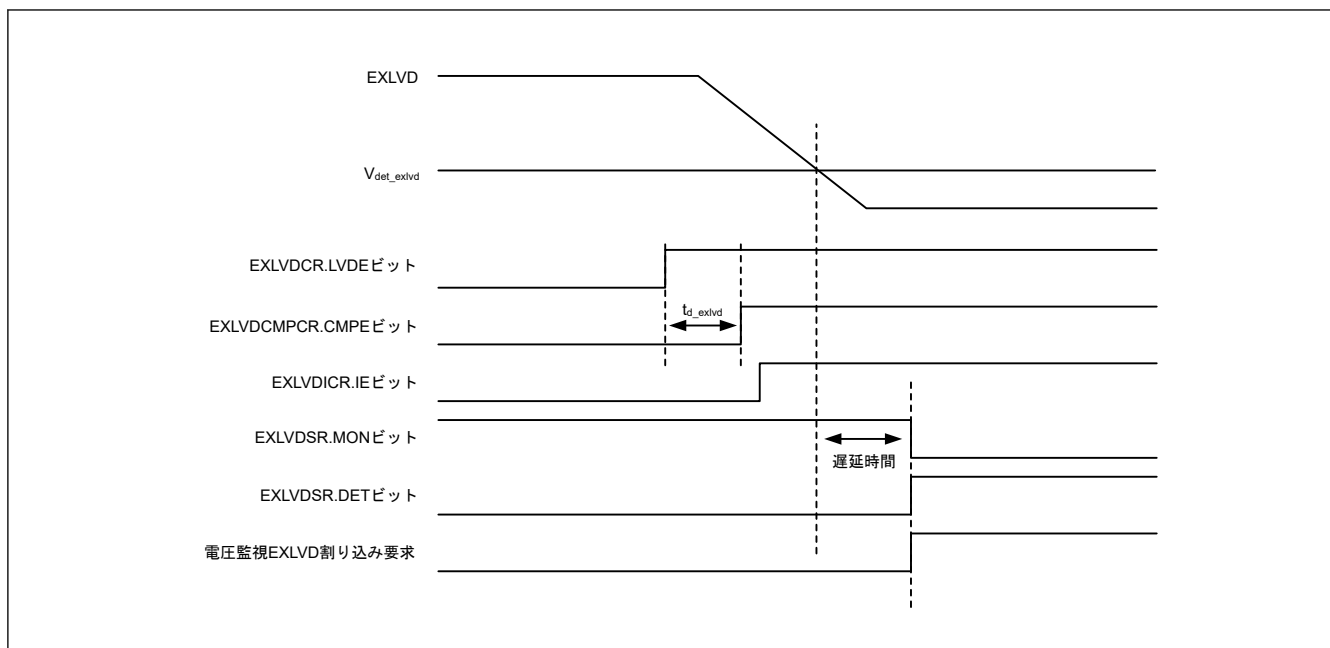
図 8.14 EXLVD 端子の低電圧検出 ON の基本動作
