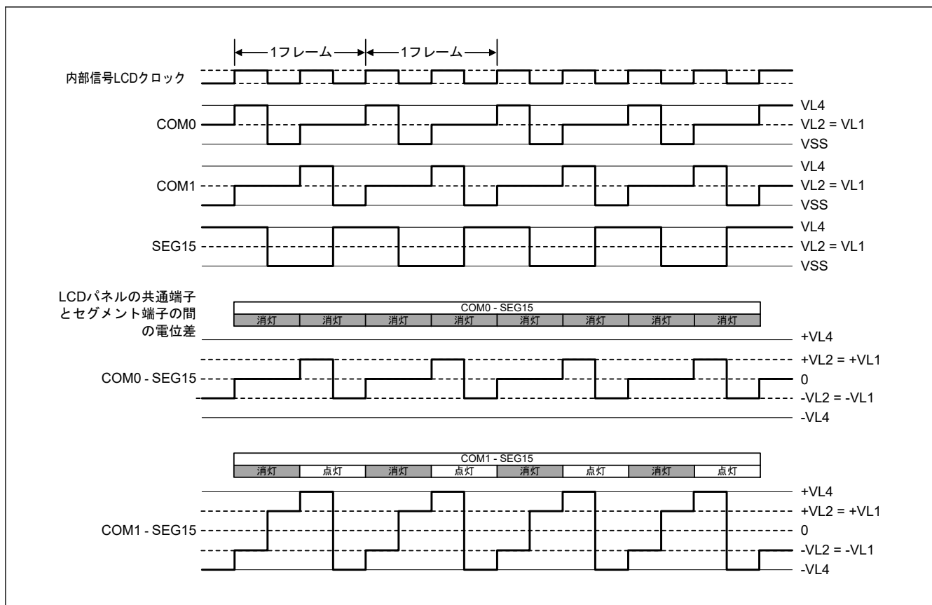
図 36.27 1/2 バias方式を使用時の SEG15 と各共通信号の間の 2 タイムスライス LCD 駆動波形の例
