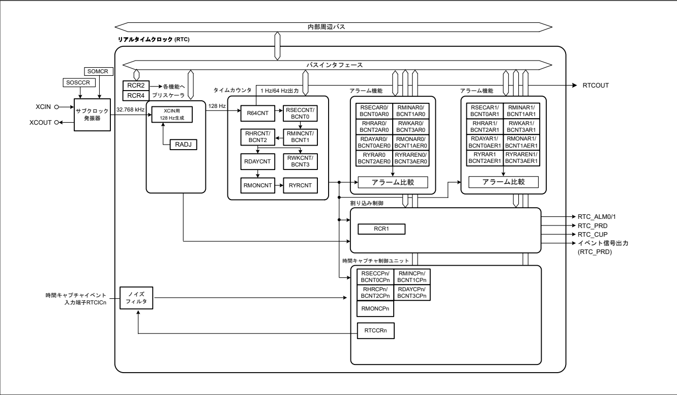
図 23.1 RTC のブロック図
