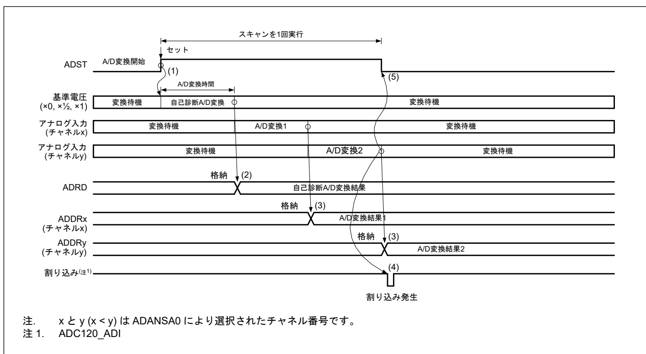
図 30.8 シングルスキャンモードの基本動作例 (アナログ入力 (チャネル x と y) 選択+自己診断)
