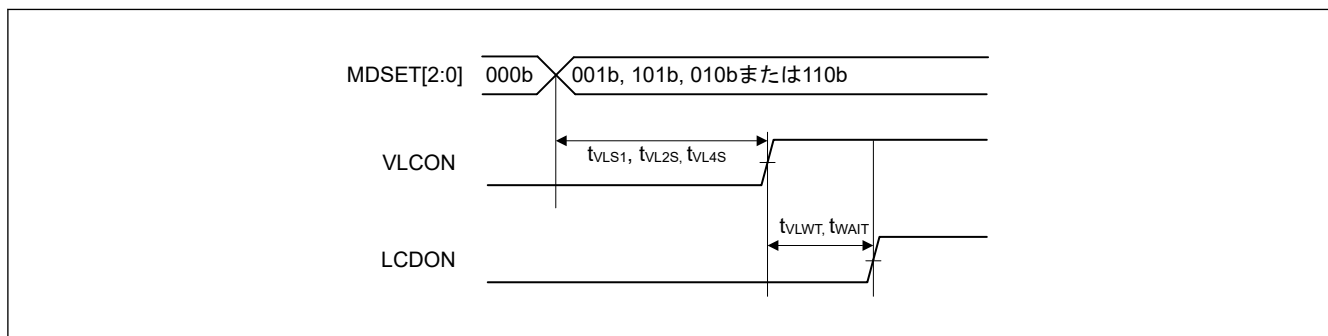
図 41.51 LCD リファレンス電圧起動時間、電圧昇圧待機時間、容量分割待機時間
