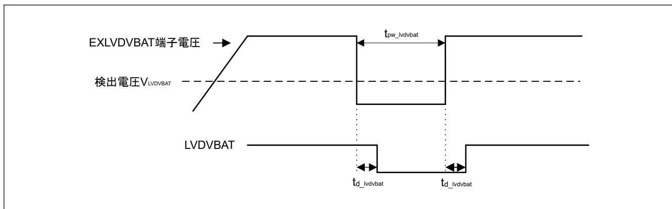
図 41.48 EXLVDVAT 端子電圧検出回路のタイミング
