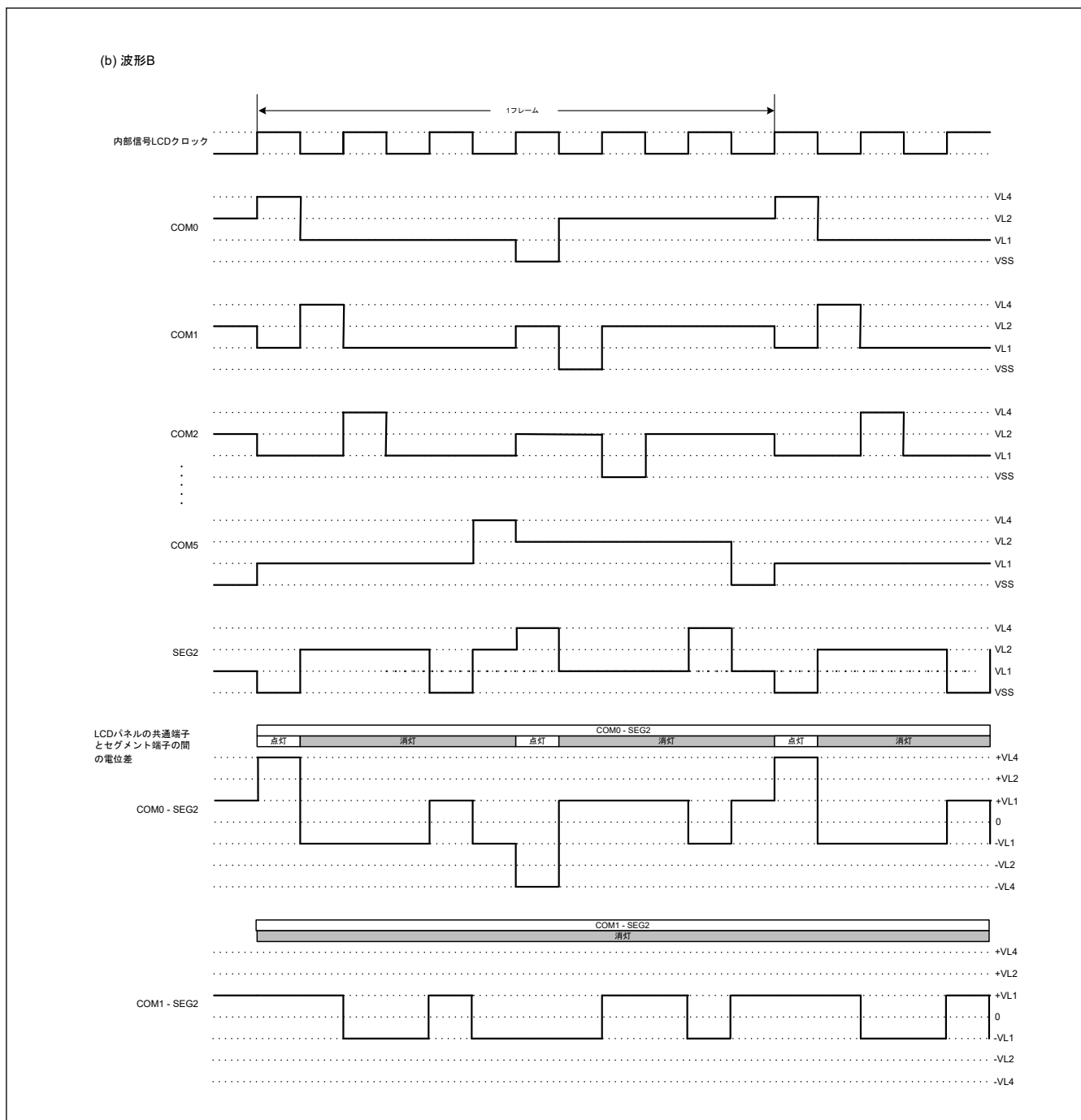
図 36.39 1/3 バias方式を使用時の SEG2 と各共通信号の間の 6 タイムスライス LCD 駆動波形の例
