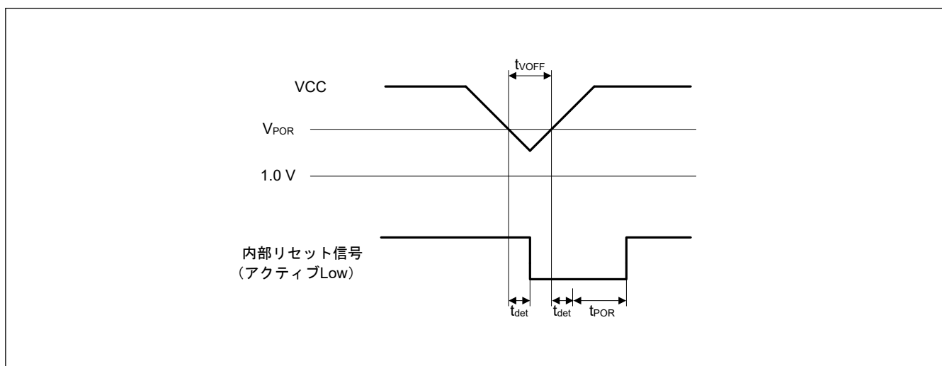
図 41.42 電圧検出しリセットタイミング
