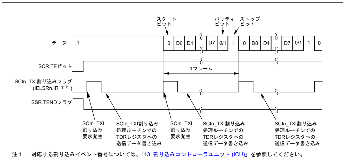
図 26.7 調歩同期式モードにおけるシリアル送信の動作例 (1) (8 ビットデータ/パリティあり/1ストップビット/CTS 機能不使用/送信開始時)
