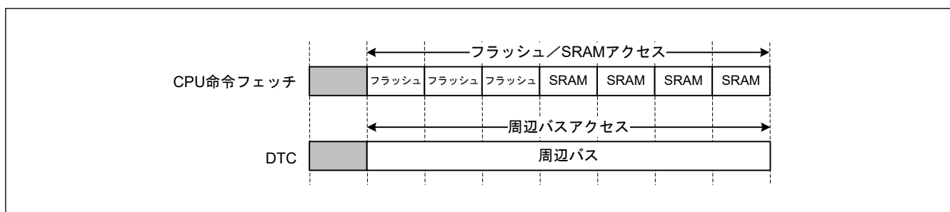
図 14.2 並列動作の例
