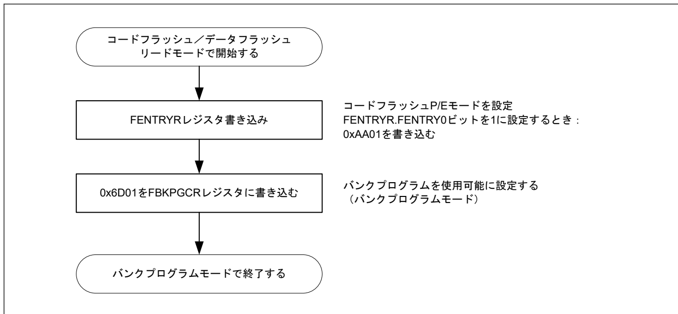
図 35.10 バンクプログラムモードに移移する手順
