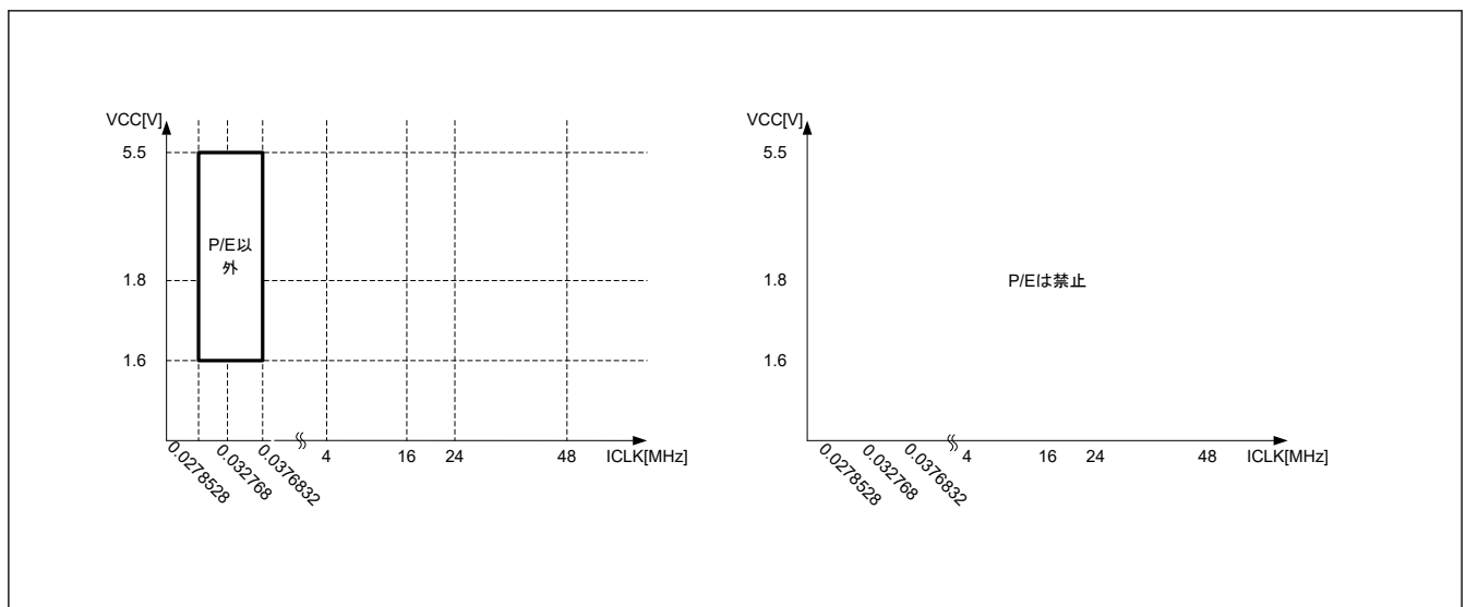
図 11.5 Subosc-speed モードにおける動作電圧と動作周波数
