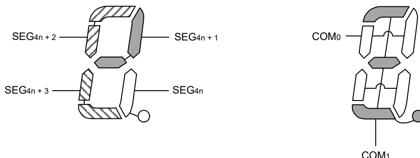
図 36.25 2 タイムスライス LCD 表示パターンと電極接続
