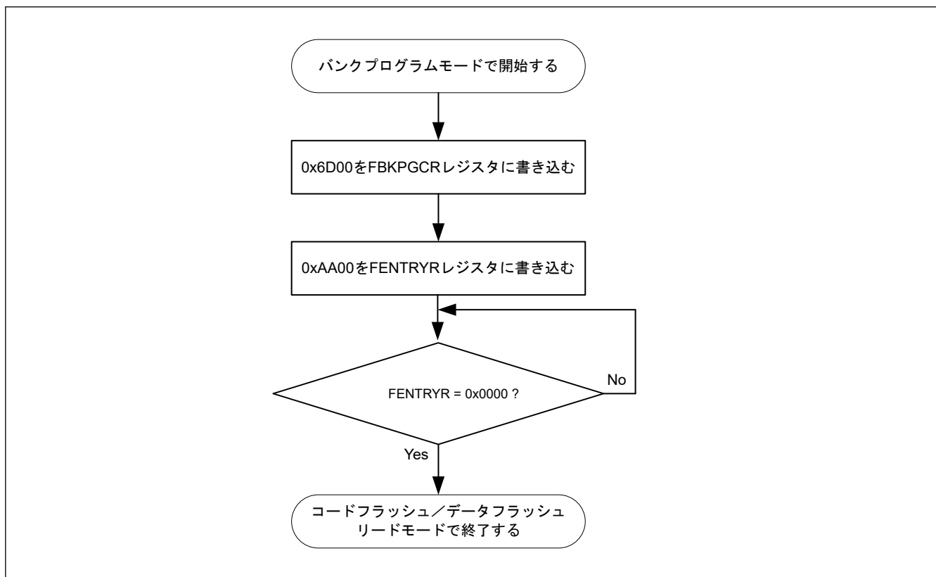
図 35.11 バンクプログラムモードからコードフラッシュリードモードに移移する手順
