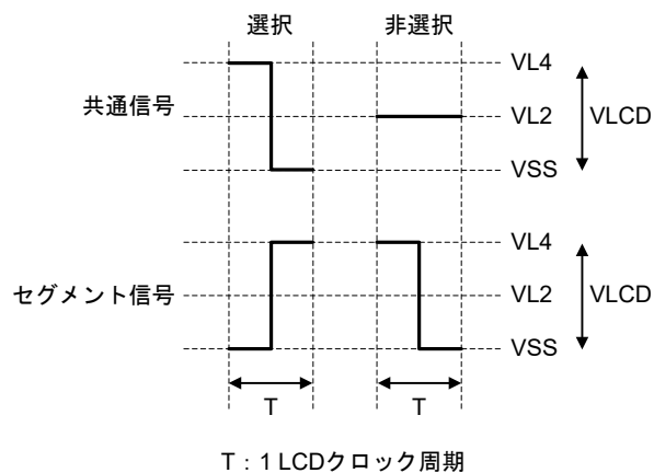
図 36.19 共通信号とセグメント信号の電圧と位相 (1/3)
