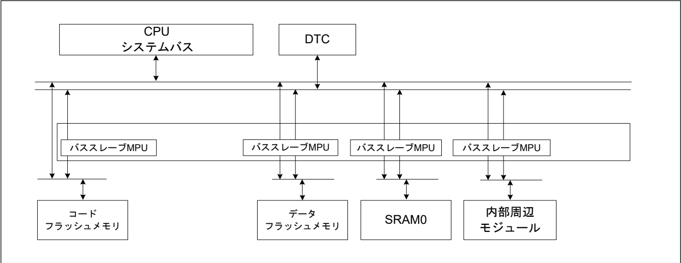
図 15.9 バススレーブ MPU のブロック図
