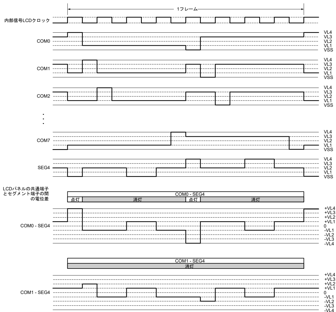
図 36.43 1/4 バias方式を使用時の SEG4 と各共通信号の間の 8 タイムスライス LCD 駆動波形の例 (2/2)
