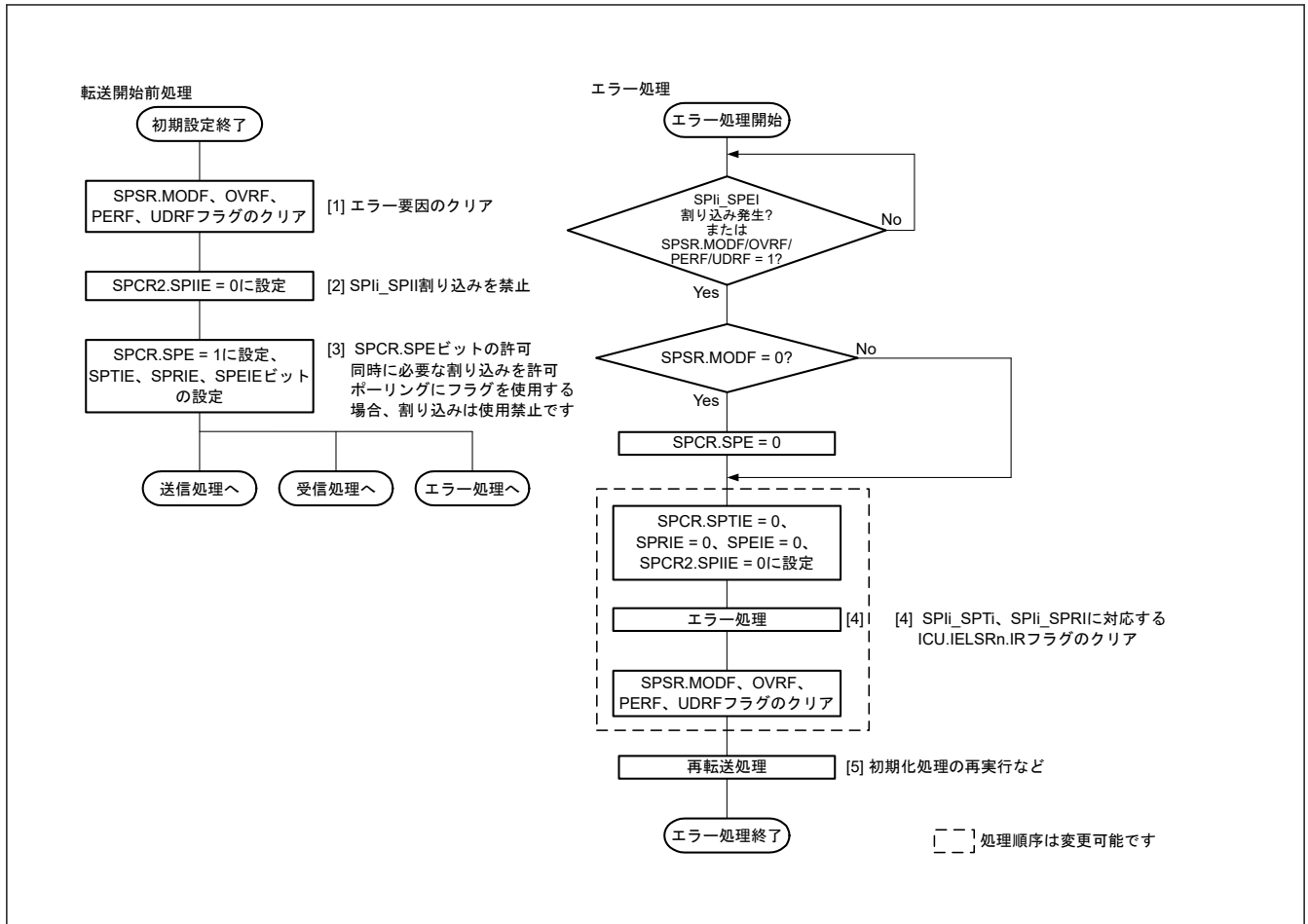
図 28.39 スレープモードでのエラー処理フロー
