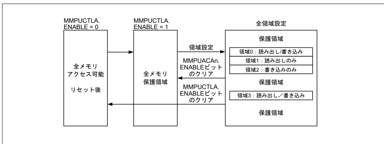
図 15.5 バスマスタ MPU の使用例
