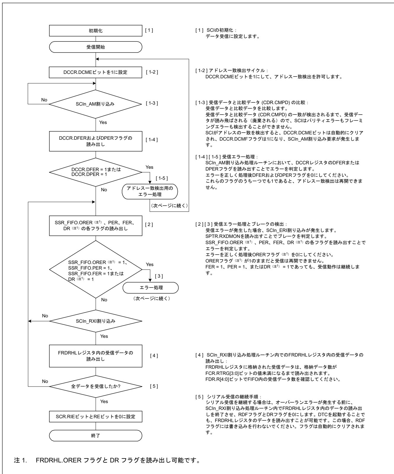
図 26.23 調歩同期式モードにおけるシリアル受信のフローチャート例 (FIFO 選択、アドレス一致検出有効時) (1)
