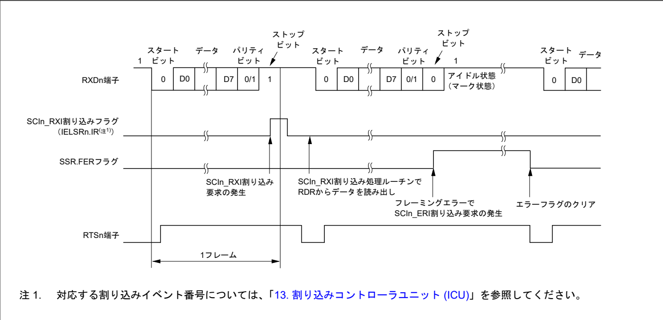
図 26.14 調歩同期式モードにおけるシリアル受信の動作例 (2) (RTS 機能を使用する場合) (8 ビットデータ/パリティあり/1 ストップビットの場合)
