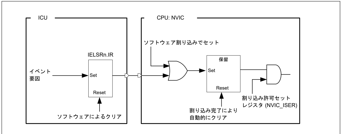
図 13.3 ICU および CPU の割り込み経路 (NVIC) (IELSRn で設定 (n = 32~67))
