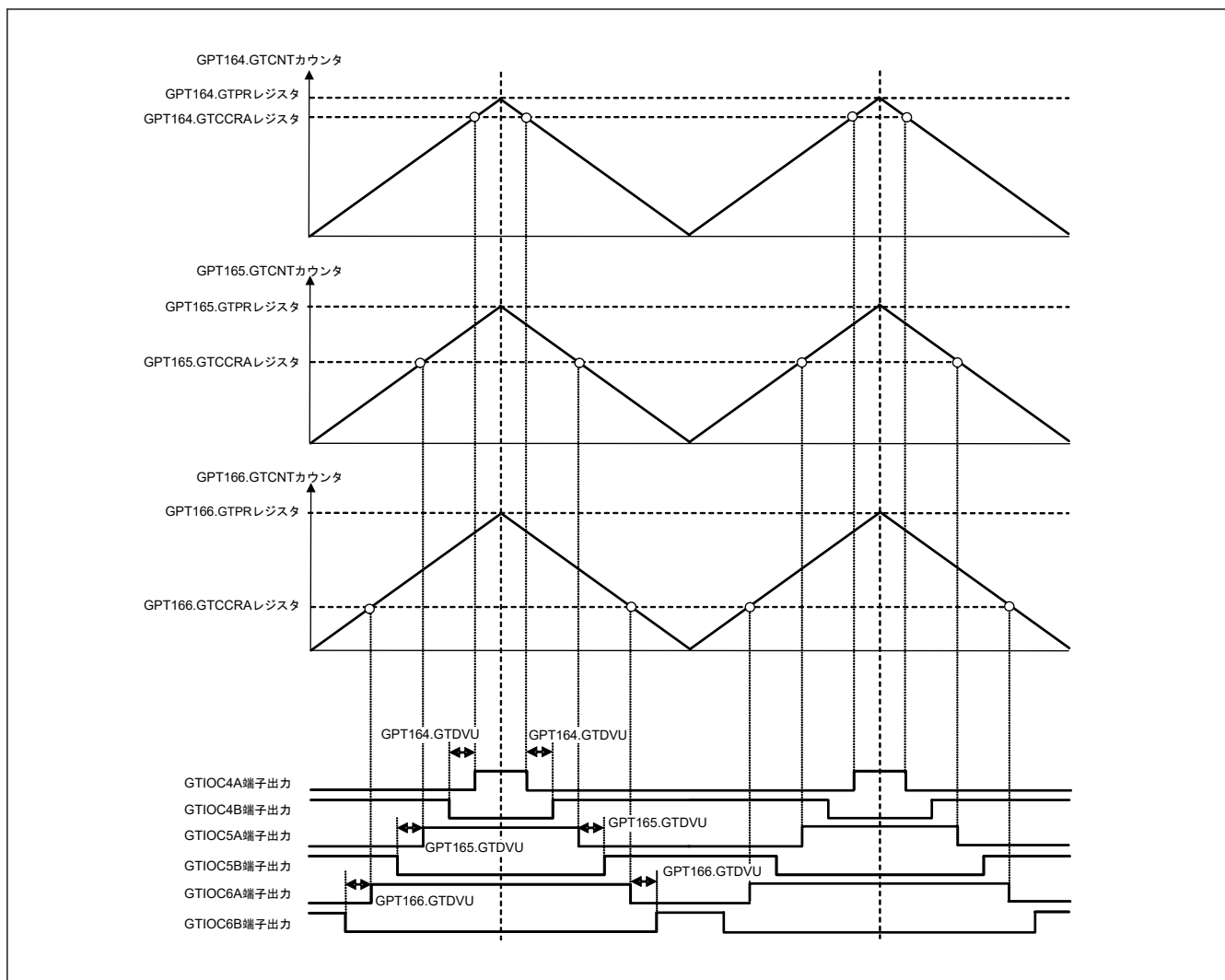
図 20.43 三角波 3 相相補 PWM 出力例 (デッドタイム自動設定)
