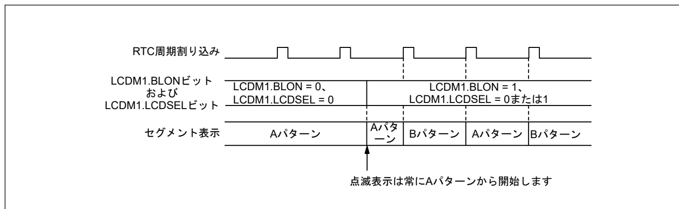
図 36.3 A パターン表示から点滅表示への切り替え動作
