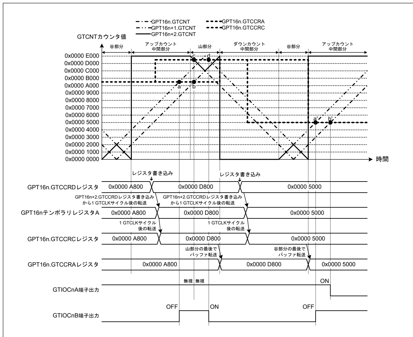
図 20.56 相補 PWM モードでのコンペアマッチ発生シーケンス動作例 (相補 PWM モード 3 シングルバッファ動作、アップカウントの GTCCRA レジスタコンペアマッチ時: GTIOCN A 端子 = Low/GTIOCN B 端子 = High、ダウンカウントの GTCCRA レジスタコンペアマッチ時: GTIOCN A 端子 = High/GTIOCN B 端子 = Low、デッドタイム値: 0x0000 2000、コンペアマッチ発生順序: a → (b, c) → d) (n = 0)
