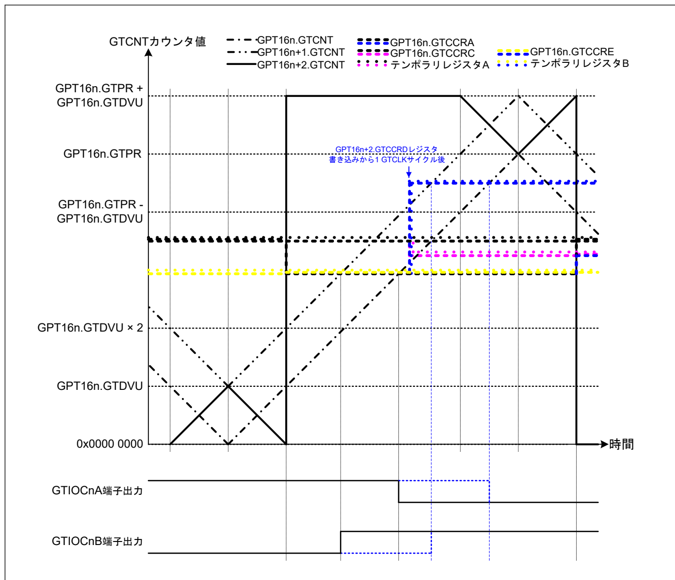
図 20.76 相補 PWM モード 4 のダブルバッファ動作例（アップカウント中間部分）（相補 PWM モード 4 ダブルバッファ動作、アップカウントの GTCCRA レジスタコンペアマッチ時：GTIOcNA 端子 = Low / GTIOcNB 端子 = High、ダウンカウントの GTCCRA レジスタコンペアマッチ時：GTIOcNA 端子 = High / GTIOcNB 端子 = Low、アップカウントコンペアマッチ後に値が GTCCRF レジスタに書き込まれた場合）（ n = 0 ）
