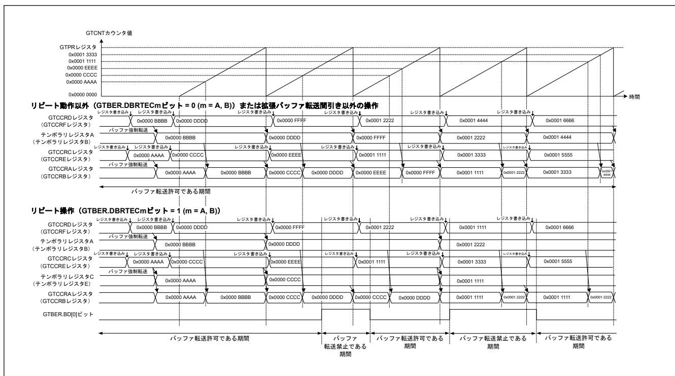
図 20.167 GTCCR バッファ転送が禁止されているときのリピートダブルバッファ動作例 (のこぎり波ワンショットパルスモード、GTBER.BD[0]ビットを更新)
