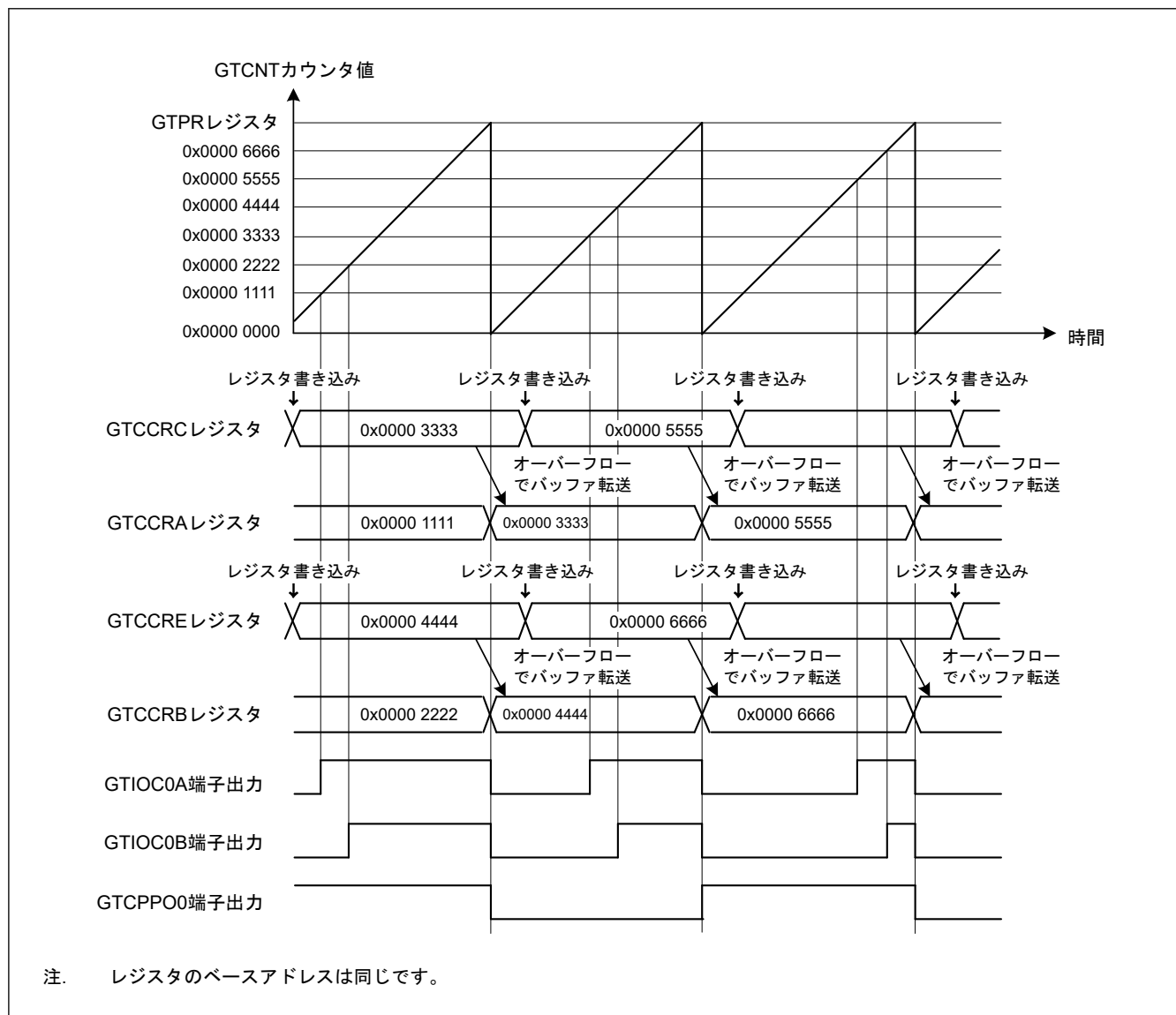
図 20.38 のこぎり波 PWM モード 1 の動作例 (アップカウント、バッファ動作、GTCCRA/GTCCRB レジスタのコンペアマッチで High 出力、周期の終わりで Low 出力、GTIOR.PSYE = 1 の場合)
