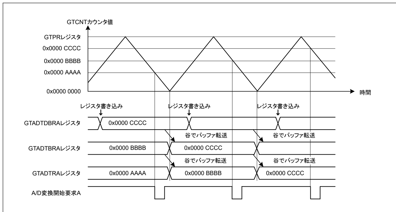
図 20.32 GTADTRA および GTADTRB レジスタのダブルバッファ動作例（三角波、谷でバッファ転送、ダウンカウントで A/D 変換開始要求発生の場合）
