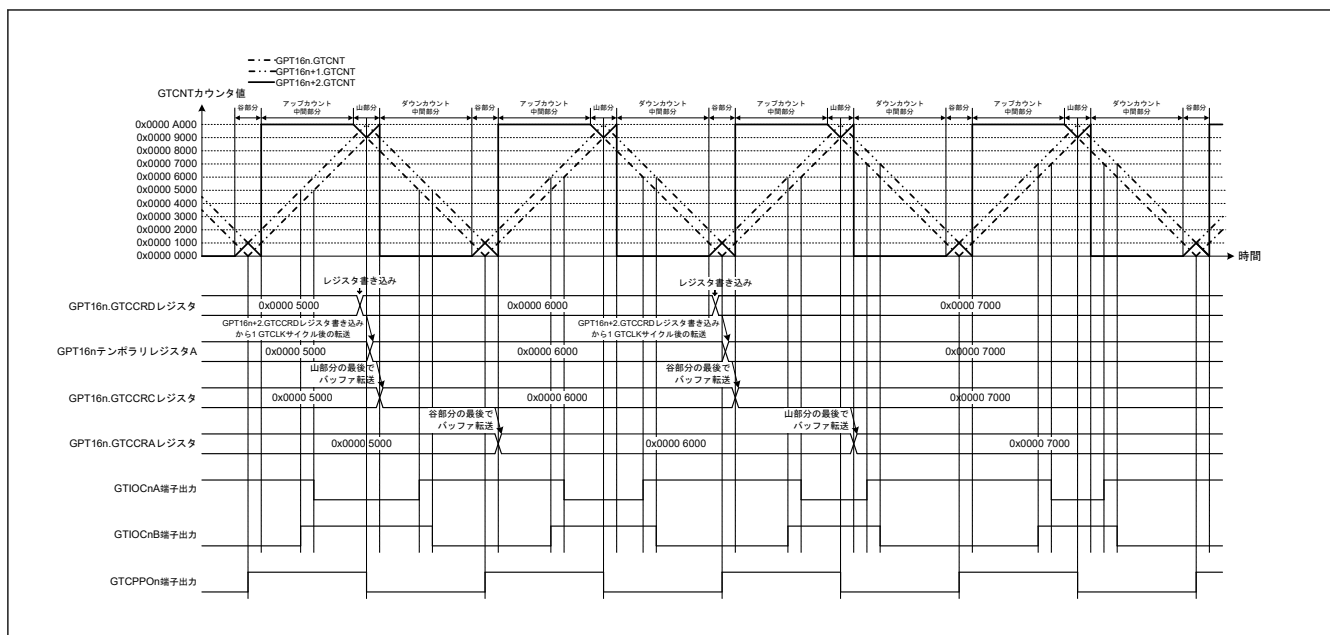
図 20.52 相補 PWM モード 3 動作例 (シングルバッファ動作、アップカウントの GTCCRA レジスタコンペアマッチ時: GTIOCnA 端子 = Low/GTIOCnB 端子 = High、ダウンカウントの GTCCRA レジスタコンペアマッチ時: GTIOCnA 端子 = High/GTIOCnB 端子 = Low、デッドタイム値: 0x0000 1000、GTCCRD レジスタを山部分と谷部分で更新) (n = 0)
