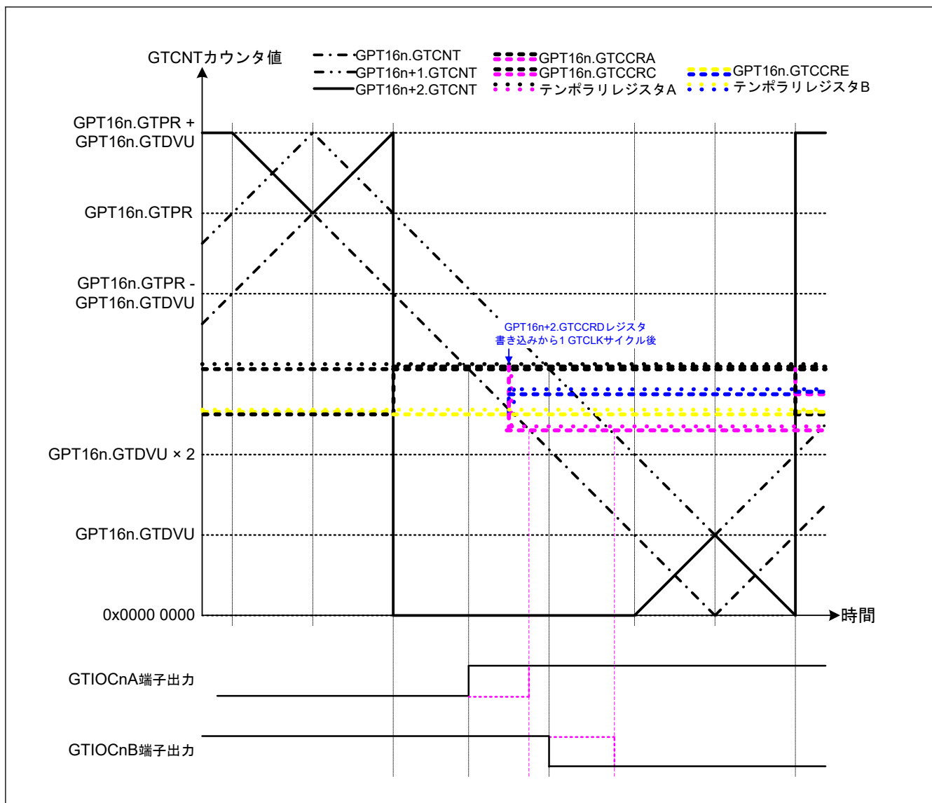
図 20.78 相補 PWM モード 4 のダブルバッファ動作例 (ダウンカウント中間部分) (相補 PWM モード 4 ダブルバッファ動作、アップカウントの GTCCRA レジスタコンペアマッチ時: GTIOCN A 端子 = Low/GTIOCN B 端子 = High、ダウンカウントの GTCCRA レジスタコンペアマッチ時: GTIOCN A 端子 = High/GTIOCN B 端子 = Low、ダウンカウントデッドタイム時に値が GTCCRD レジスタに書き込まれた場合) (n = 0)
