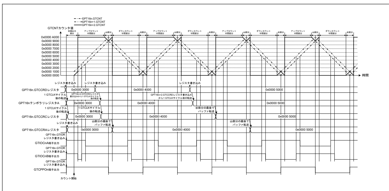
図 20.47 相補 PWM モード 1 動作例（初期出力時：GTIOCA 端子 = High/GTIOCB 端子 = High、アップカウンタの GTCCRA レジスタコンペアマッチ時：GTIOCA 端子 = Low/GTIOCB 端子 = High、ダウンカウンタの GTCCRA レジスタコンペアマッチ時：GTIOCA 端子 = High/GTIOCB 端子 = Low、デッドタイム値：0x0000 1000、GTCCRD レジスタを中間部分で更新）(n = 0)
