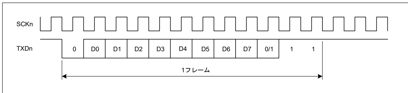
図 24.4 調歩同期式モードにおける出力クロックと送信データの位相関係 (SMR.CHR = 0、PE = 1、MP = 0、および STOP = 1 の場合)
