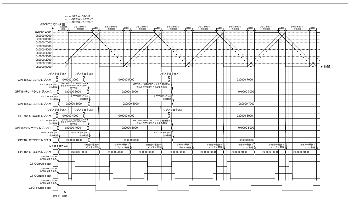
図 20.53 相補 PWM モード 3 動作例 (ダブルバッファ動作、初期出力時: GTIOCnA 端子 = High/GTIOCnB 端子 = High、アップカウントの GTCCRA レジスタコンペアマッチ時: GTIOCnA 端子 = Low/GTIOCnB 端子 = High、ダウンカウントの GTCCRA レジスタコンペアマッチ時: GTIOCnA 端子 = High/GTIOCnB 端子 = Low、デッドタイム値: 0x0000 1000、GTCCRD レジスタを中間部分で更新) (n = 0)
