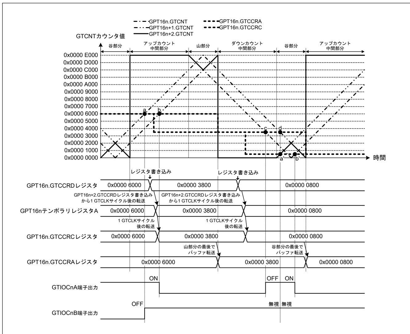
図 20.63 相補 PWM モードでのコンペアマッチ発生シーケンス動作例 (相補 PWM モード 3 シングルバッファ動作、アップカウントの GTCCRA レジスタコンペアマッチ時: GTIOcNA 端子 = Low/GTIOcNB 端子 = High、ダウンカウントの GTCCRA レジスタコンペアマッチ時: GTIOcNA 端子 = High/GTIOcNB 端子 = Low、デッドタイム値: 0x0000 2000、コンペアマッチ発生順序: c → a' → d → b') (n = 0)
