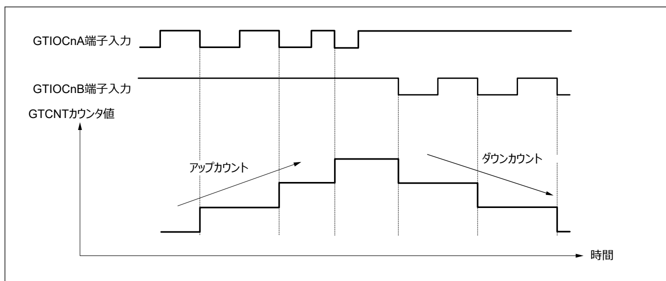
図 20.127 位相計数モード3の動作例 (A)
