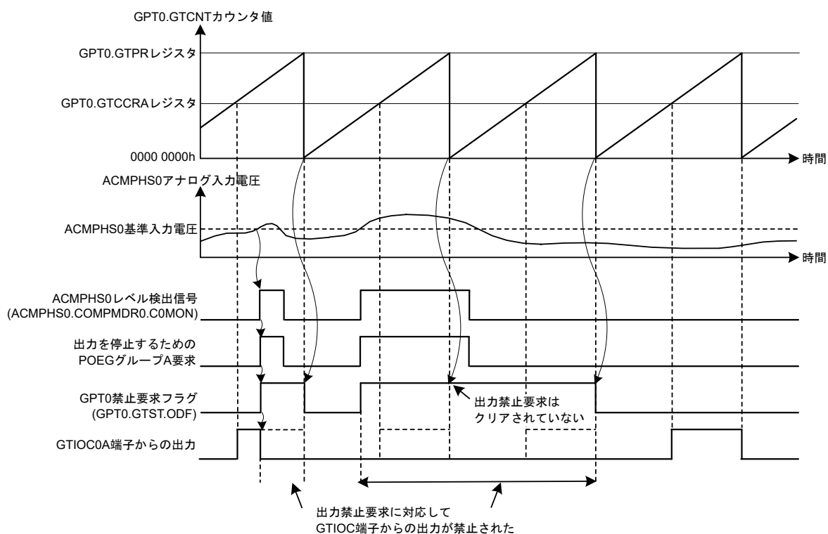
図 19.4 コンパレータによるレベル検出に対応して GTIOC 端子からの出力を停止する動作の例
