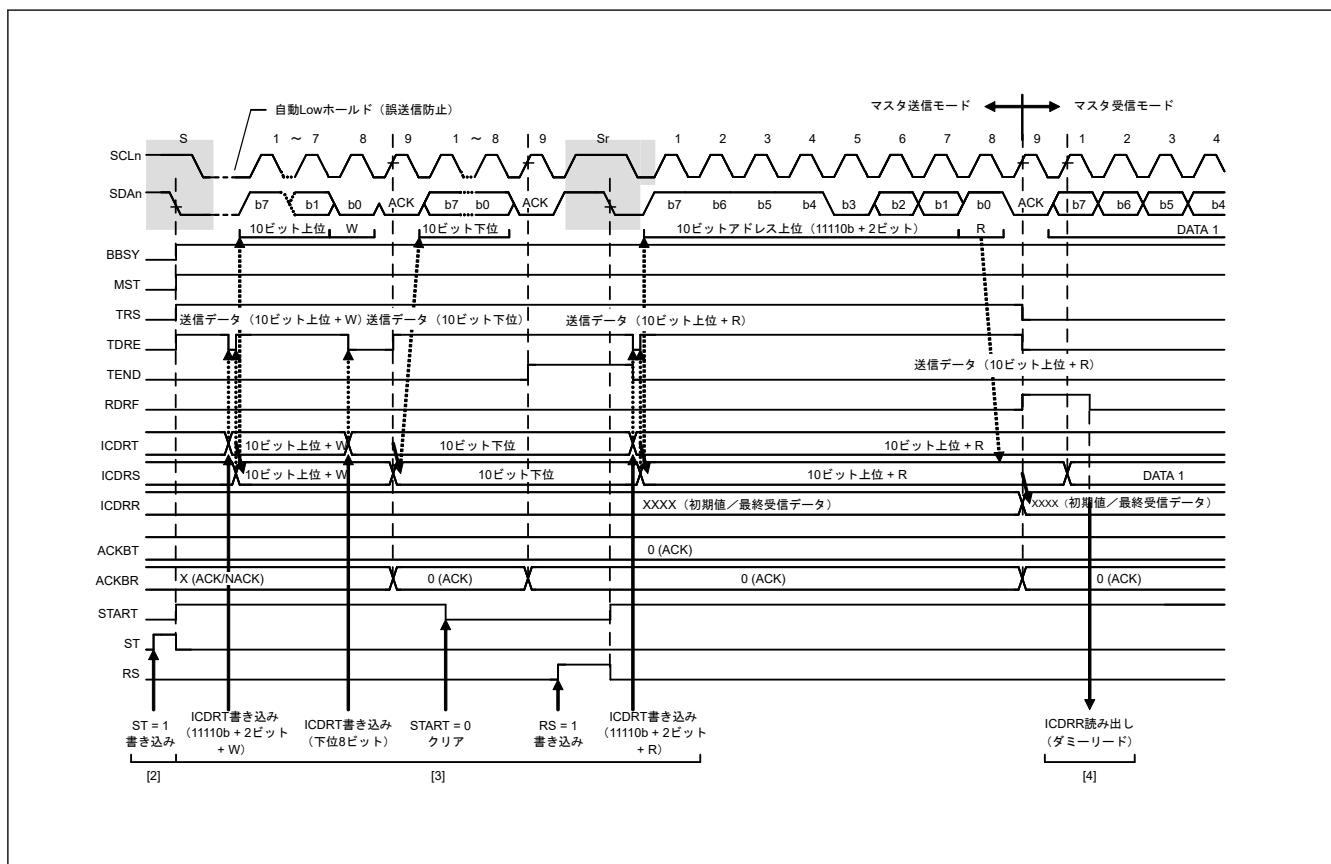
図 25.13 マスタ受信の動作タイミング (2) (10 ビットアドレスフォーマットで RDRFS = 0 の場合)
