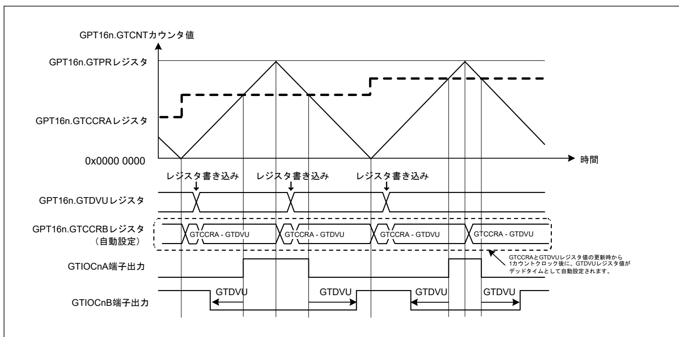
図 20.84 デッドタイム付きコンペアマッチ値の自動設定機能の動作例 (三角波 PWM モード 1、GPT163 でアクティブ High の場合)
