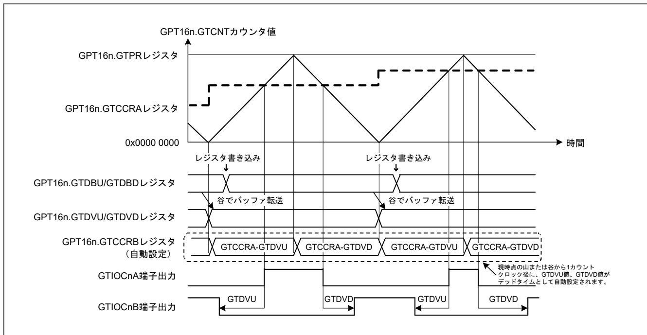
図 20.83 デッドタイム付きコンペアマッチ値の自動設定機能の動作例 (三角波 PWM モード 1、GTDVU と GTDVD はバッファ動作に設定、GPT160~GPT162 でアクティブ High の場合)
