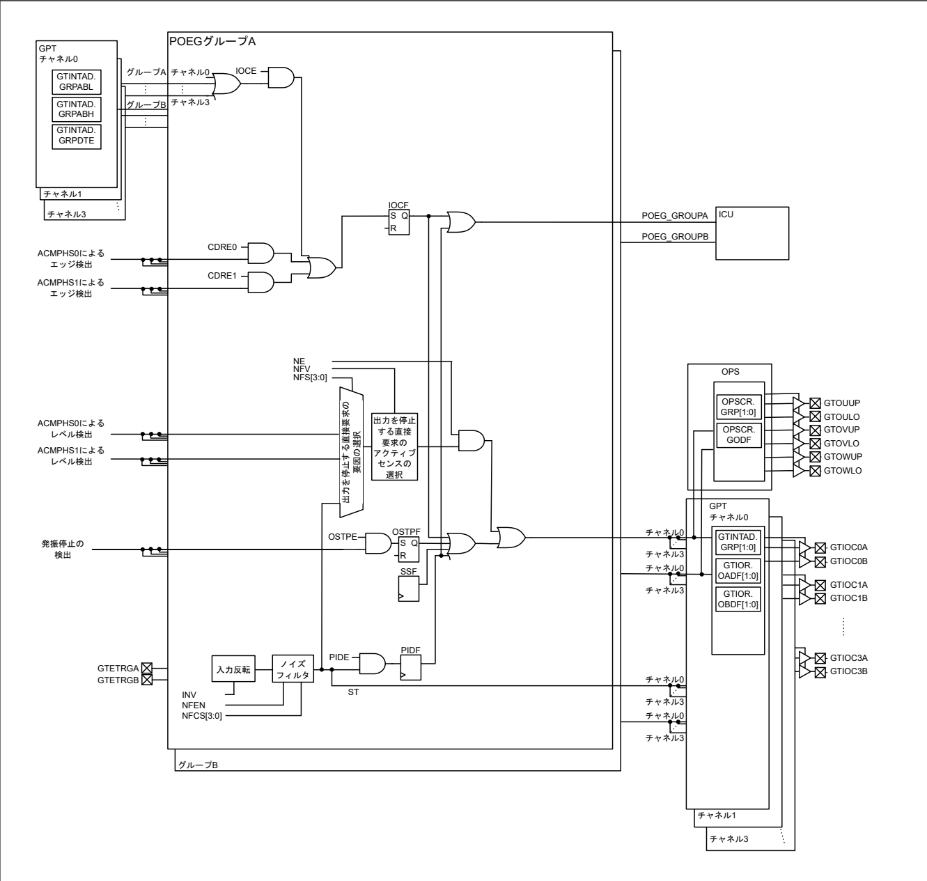
図 19.1 POEG ブロック図
