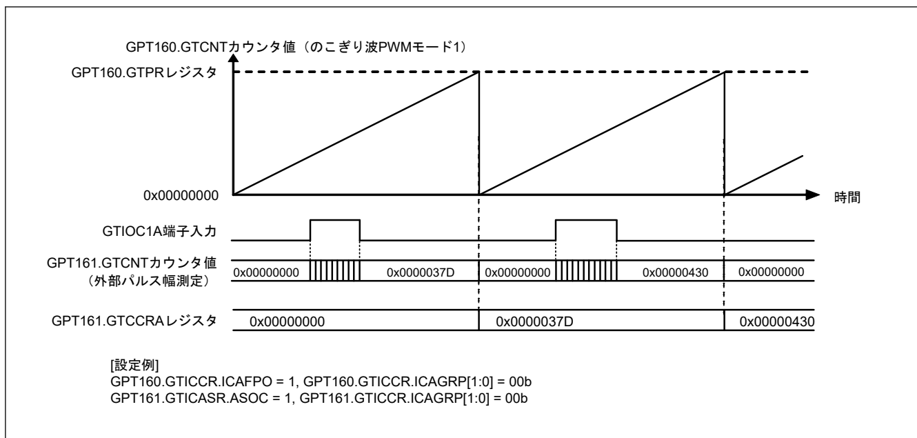
図 20.114 チャンネル間連携によるインプットキャプチャ動作の例 (チャンネル1はチャンネル0のオーバーフローによりキャプチャ)
