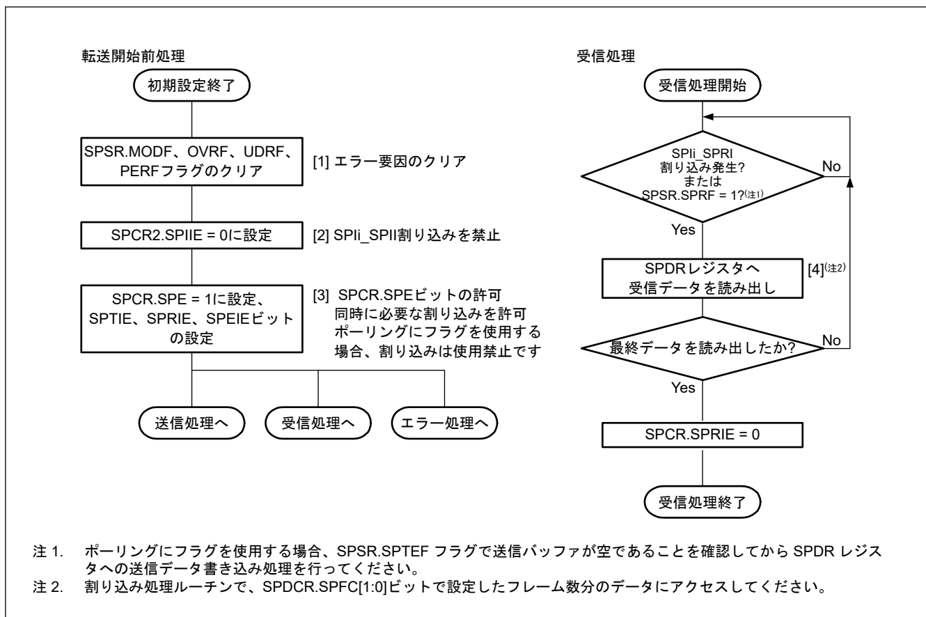
図 26.37 スレーブモードでの受信フロー
