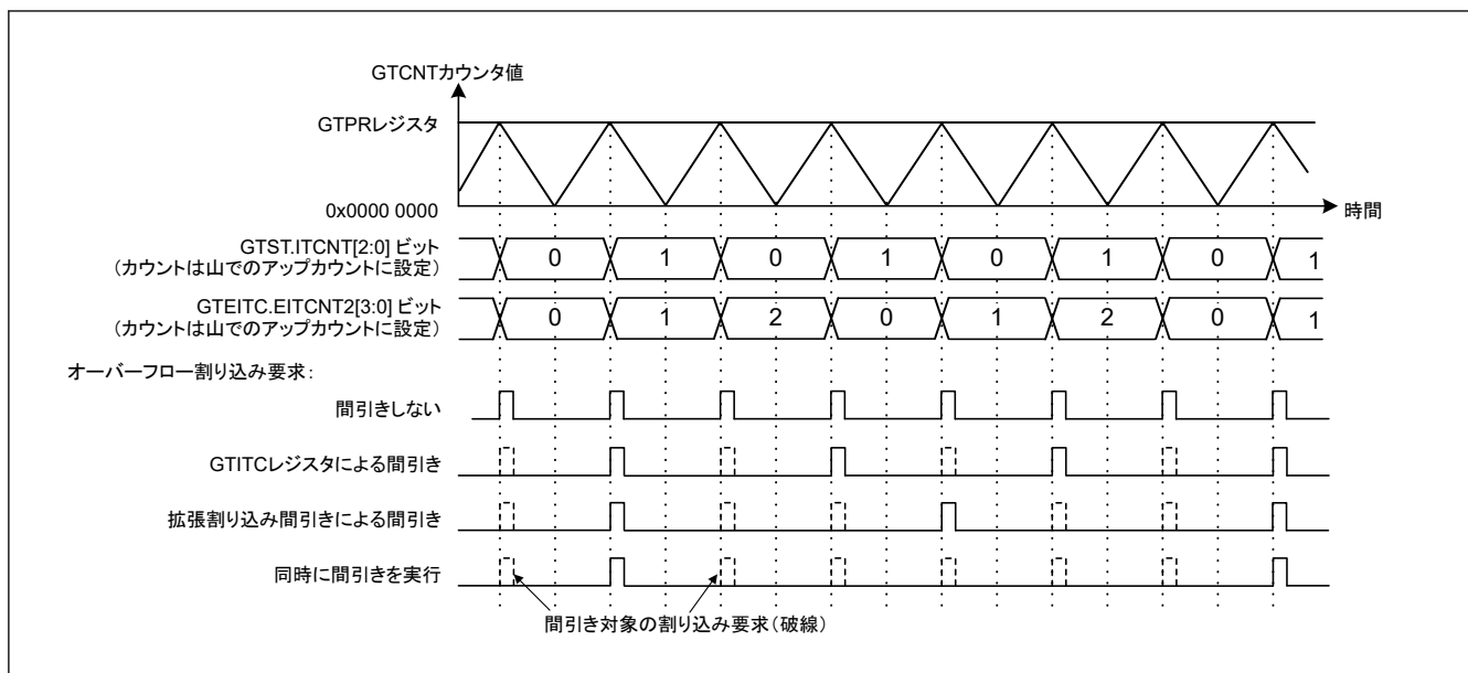
図 20.146 割り込み間引き動作の例 (GTITC レジスタによる間引き : 山でカウント、拡張割り込み間引き : EIVTC1[1:0] = 00b、EIVTC2[1:0] = 01b、EITLV[2:0] = 010b)
