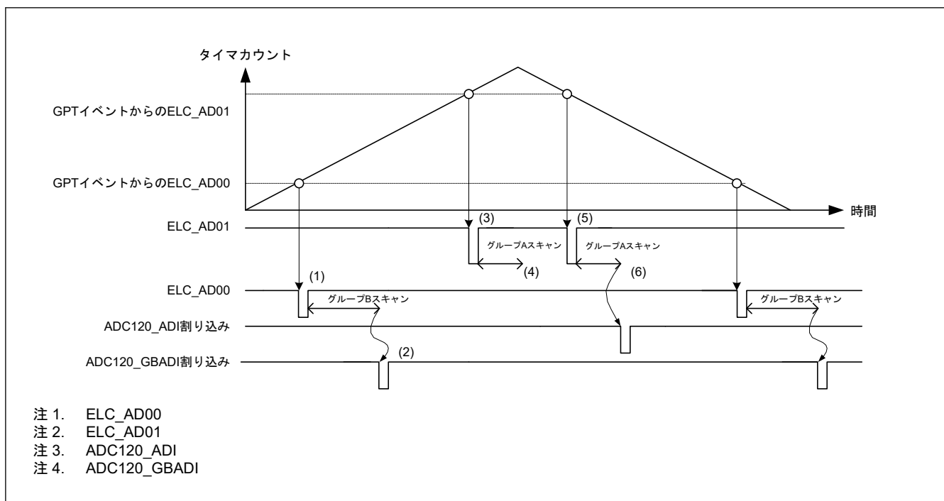
図 29.19 グループスキャンモードでダブルトリガモードを使用する場合の基本動作例 (ELC からの同期トリガ使用時)
