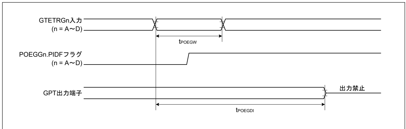
図 35.15 GTETRn 端子の入力レベル検出に対応した検出フラグによる POEG の出力禁止時間
