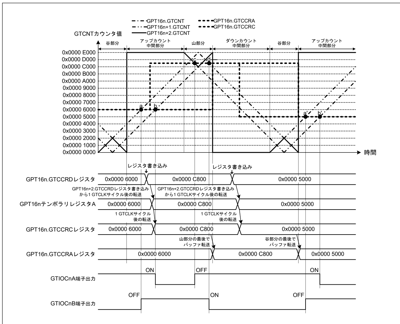
図 20.55 相補 PWM モードでのコンペアマッチ発生シーケンス動作例 (相補 PWM モード 3 シングルバッファ動作、アップカウントの GTCCRA レジスタコンペアマッチ時: GTIOCnA 端子 = Low/GTIOCnB 端子 = High、ダウンカウントの GTCCRA レジスタコンペアマッチ時: GTIOCnA 端子 = High/GTIOCnB 端子 = Low、デッドタイム値: 0x0000 2000、コンペアマッチ発生順序: a → b → c → d) (n = 0)
