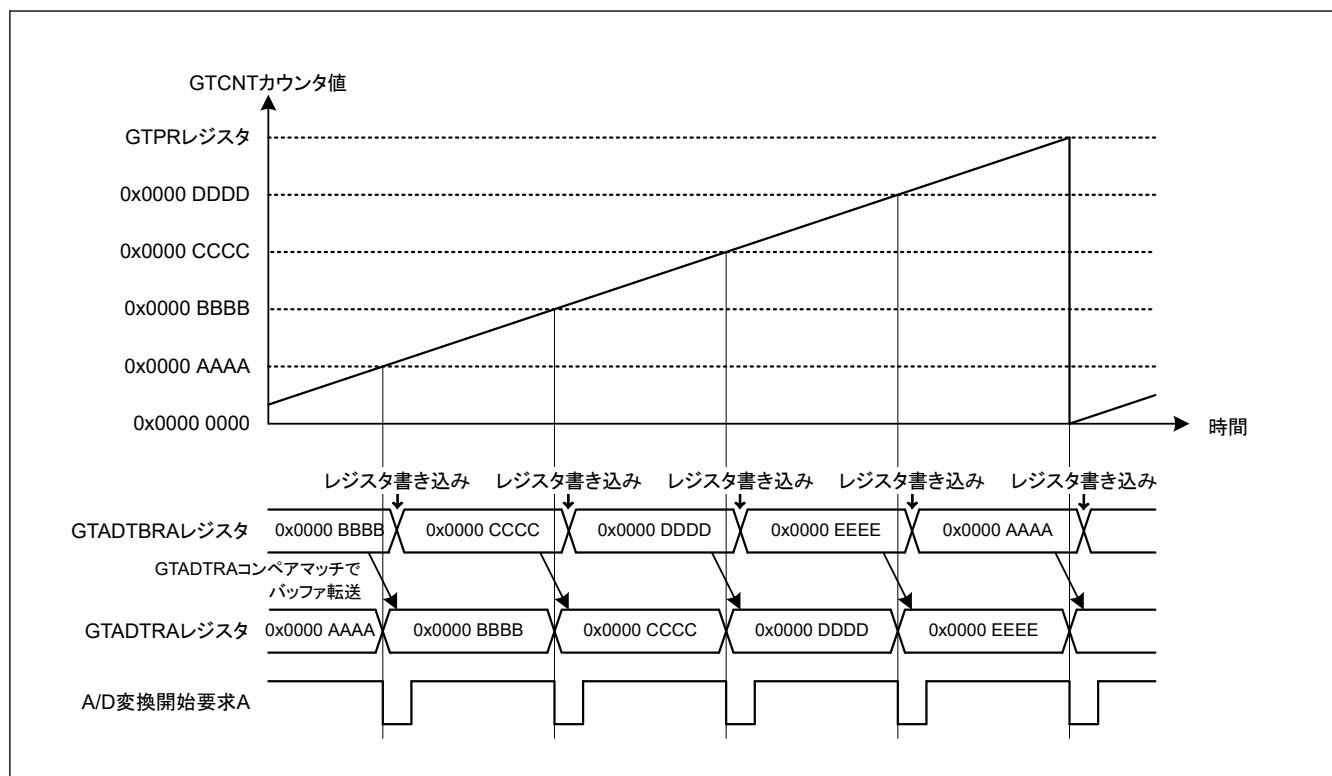
図 20.31 GTADTRA および GTADTRB レジスタのパッファ動作例 (のこぎり波でアップカウント、GTADTRA コンペアマッチでパッファ転送、アップカウントで A/D 変換開始要求発生の場合)
