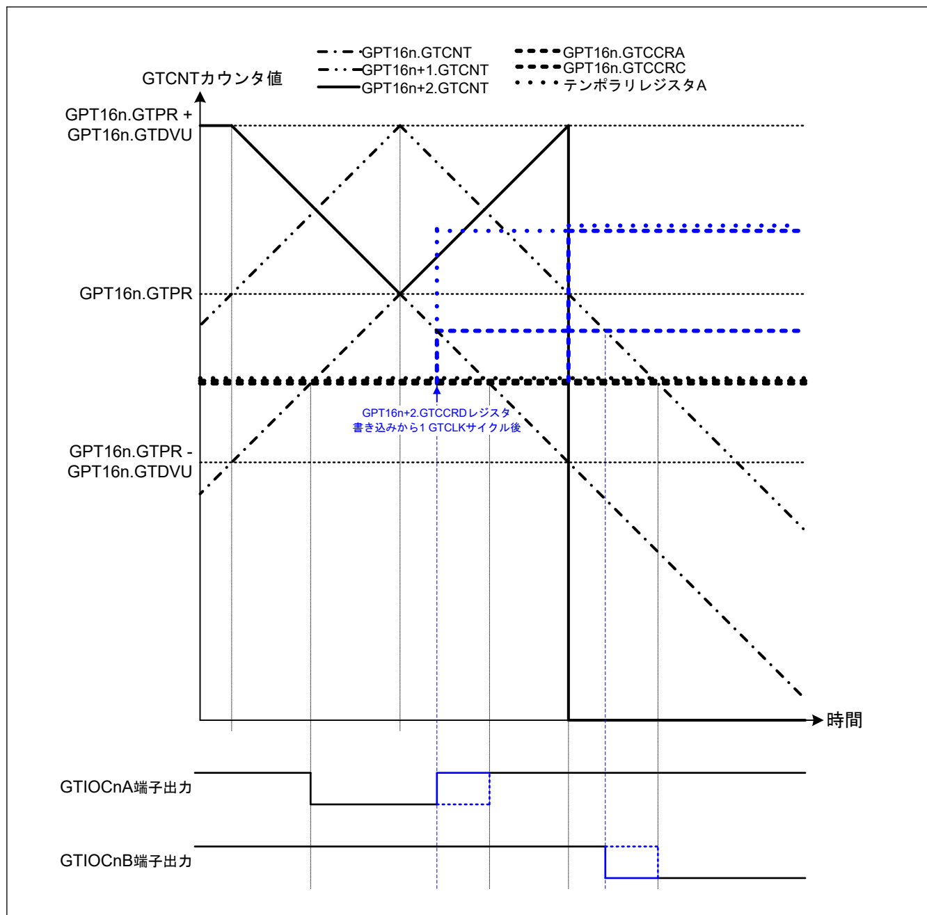
図 20.72 相補 PWM モード 4 のシングルバッファ動作例（ダウンカウント山部分）（相補 PWM モード 4 のシングルバッファ動作、アップカウントの GTCCRA レジスタコンペアマッチ時：GTIOCnA 端子 = Low / GTIOCnB 端子 = High、ダウンカウントの GTCCRA レジスタコンペアマッチ時：GTIOCnA 端子 = High / GTIOCnB 端子 = Low、アップカウントのコンペアマッチ後ダウンカウントのコンペアマッチ前に GPT16n.GTCNT 値以上の値が GTCCRD レジスタに書き込まれた場合）（n = 0）
