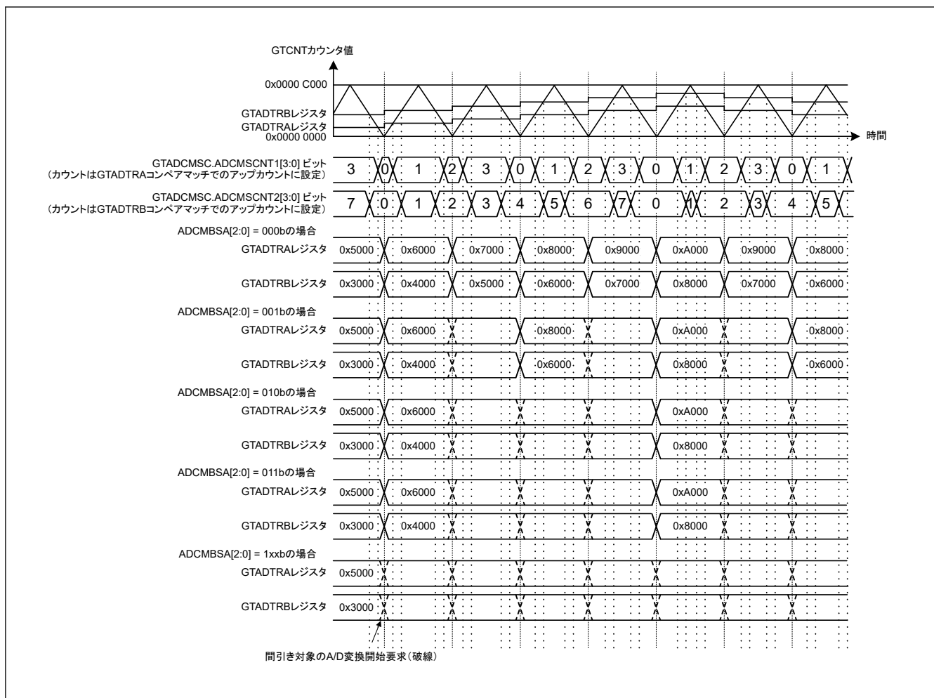
図 20.159 A/D 変換開始要求コンペアマッチ間引き機能の動作例（三角波、A/D 変換開始要求コンペアマッチ間引き 1 間引きカウント：3 カウント GTADTRA コンペアマッチ、A/D 変換開始要求コンペアマッチ間引き 2 間引きカウント：7 カウント GTADTRB コンペアマッチ、GTADTRA および GTADTRB の谷でのバッファ転送）
