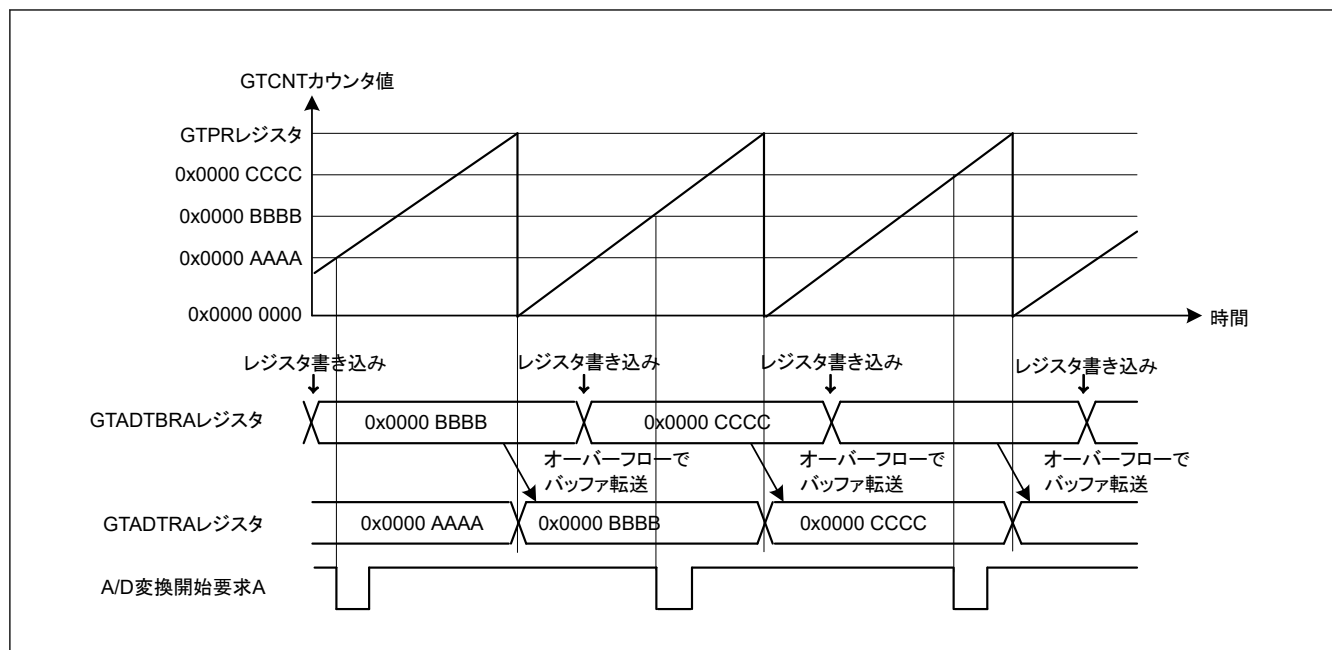
図 20.30 GTADTRA および GTADTRB レジスタのパッファ動作例 (のこぎり波でアップカウント、アップカウントで A/D 変換開始要求発生の場合)
