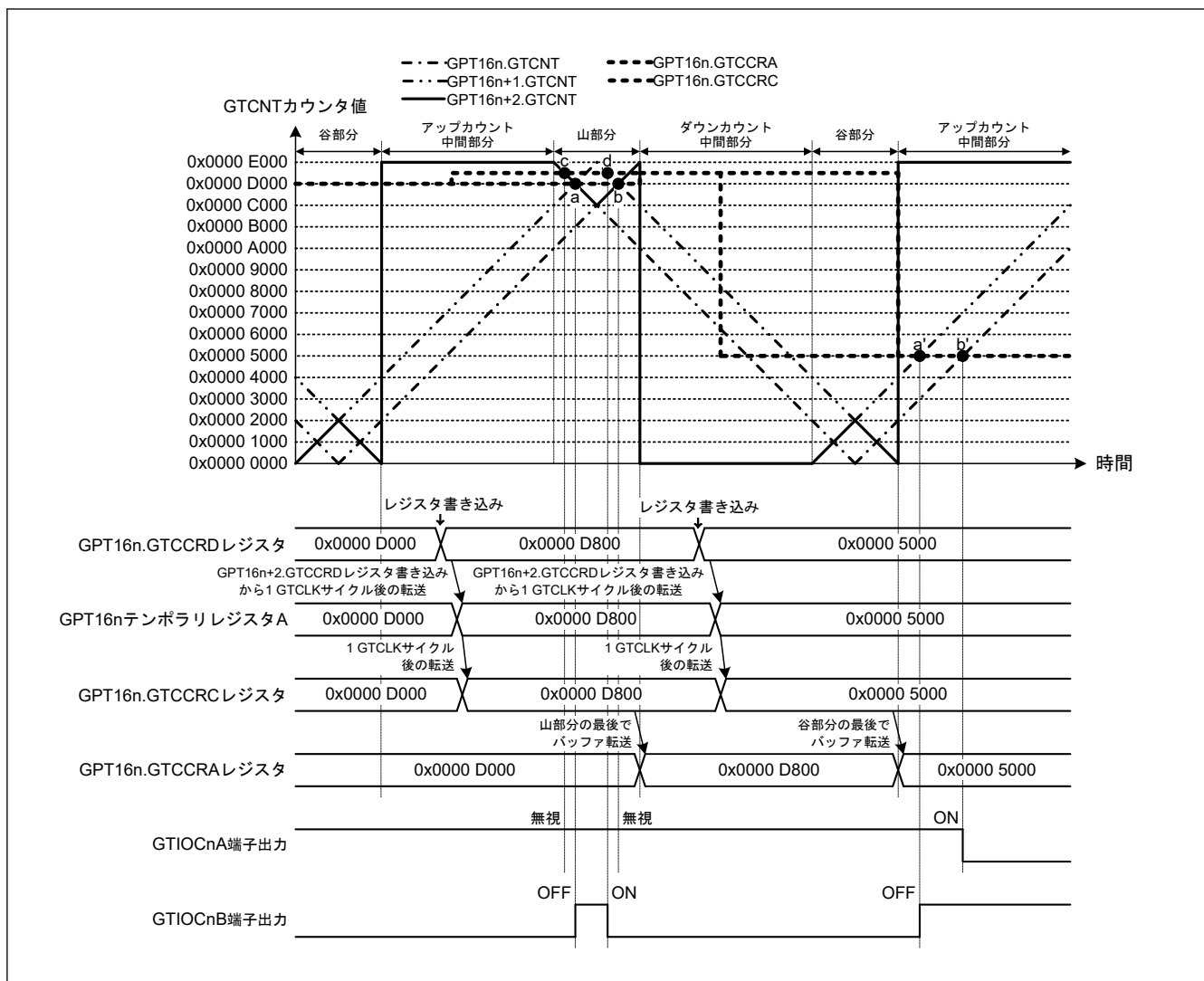
図 20.59 相補 PWM モードでのコンペアマッチ発生シーケンス動作例 (相補 PWM モード 3 シングルバッファ動作、アップカウントの GTCCRA レジスタコンペアマッチ時: GTIOcNA 端子 = Low/GTIOcNB 端子 = High、ダウンカウントの GTCCRA レジスタコンペアマッチ時: GTIOcNA 端子 = High/GTIOcNB 端子 = Low、デッドタイム値: 0x0000 2000、コンペアマッチ発生順序: c → a → d → b) (n = 0)
