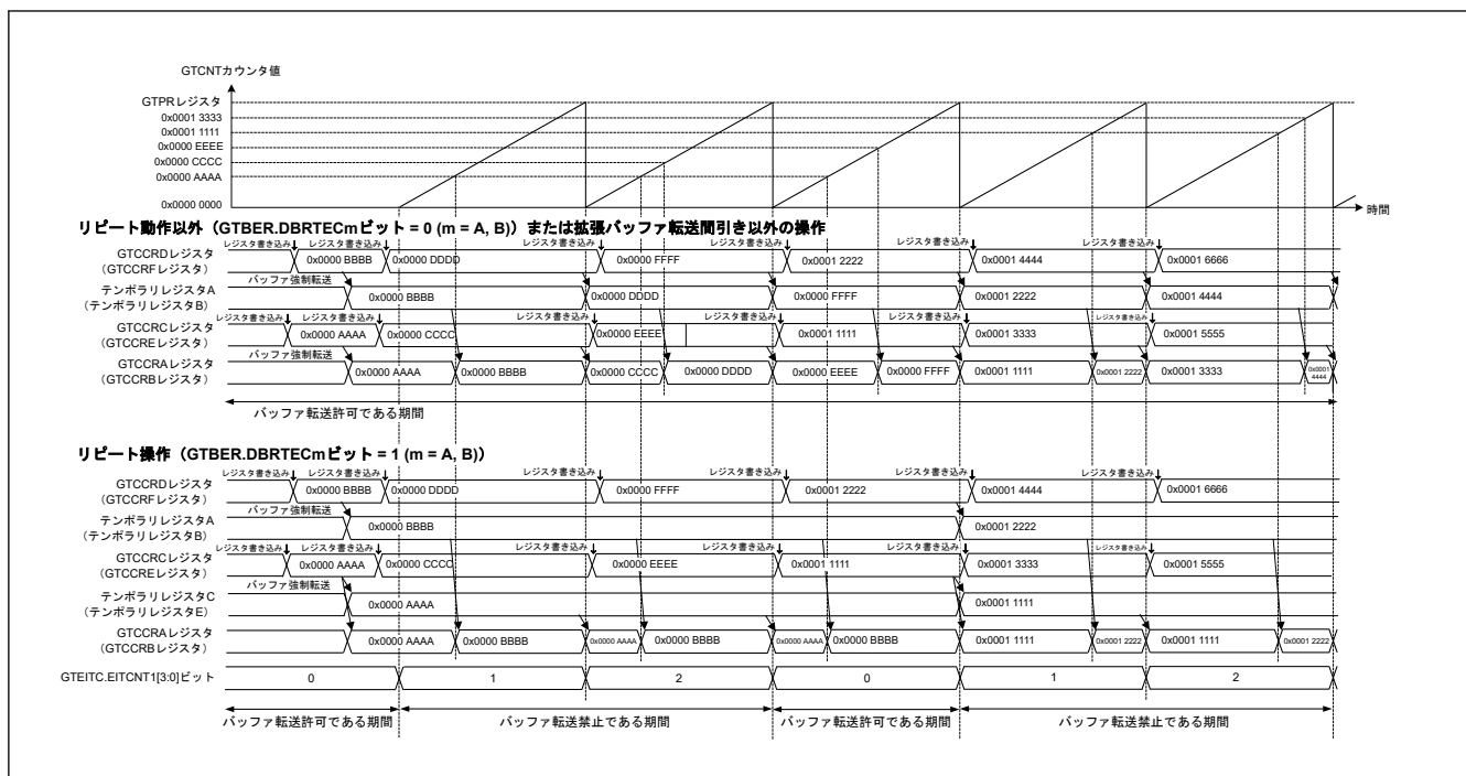
図 20.166 GTCCR バッファ転送が禁止されているときのリピートダブルバッファ動作例 (のこぎり波ワンショットパルスモード、拡張バッファ転送間引きを使用、GTBER.BD[0]は常に 0 の場合)
