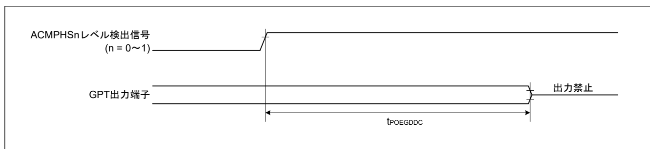
図 35.21 ACMPHS からレベル検出信号に対応した POEG の出力禁止時間
