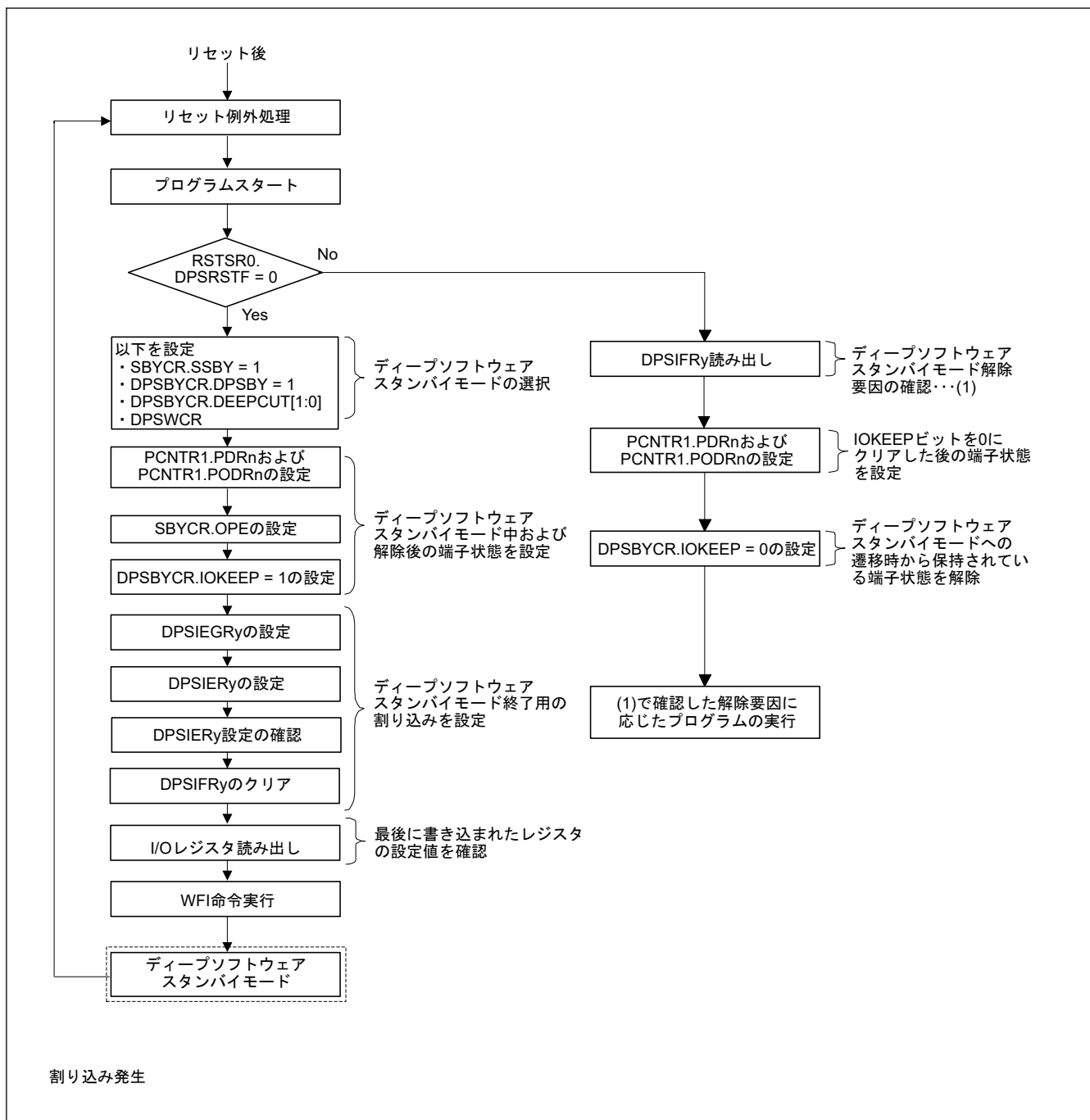
図 10.9 ディープソフトウェアスタンバイモード使用時のフローチャート例
