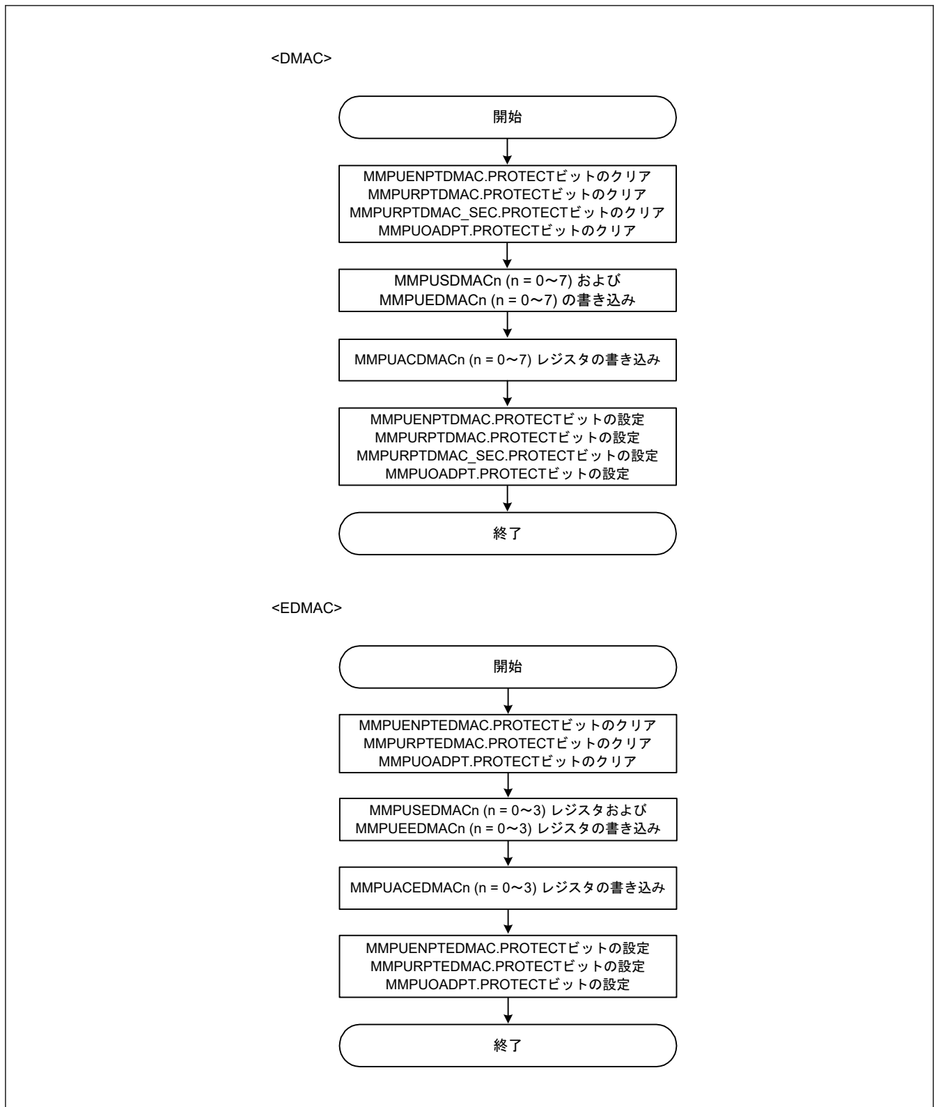
図 15.4 領域追加のレジスタ設定フロー
