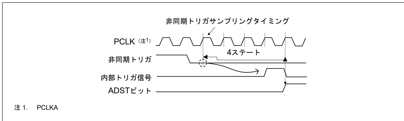
図 39.31 非同期トリガ入力タイミング
