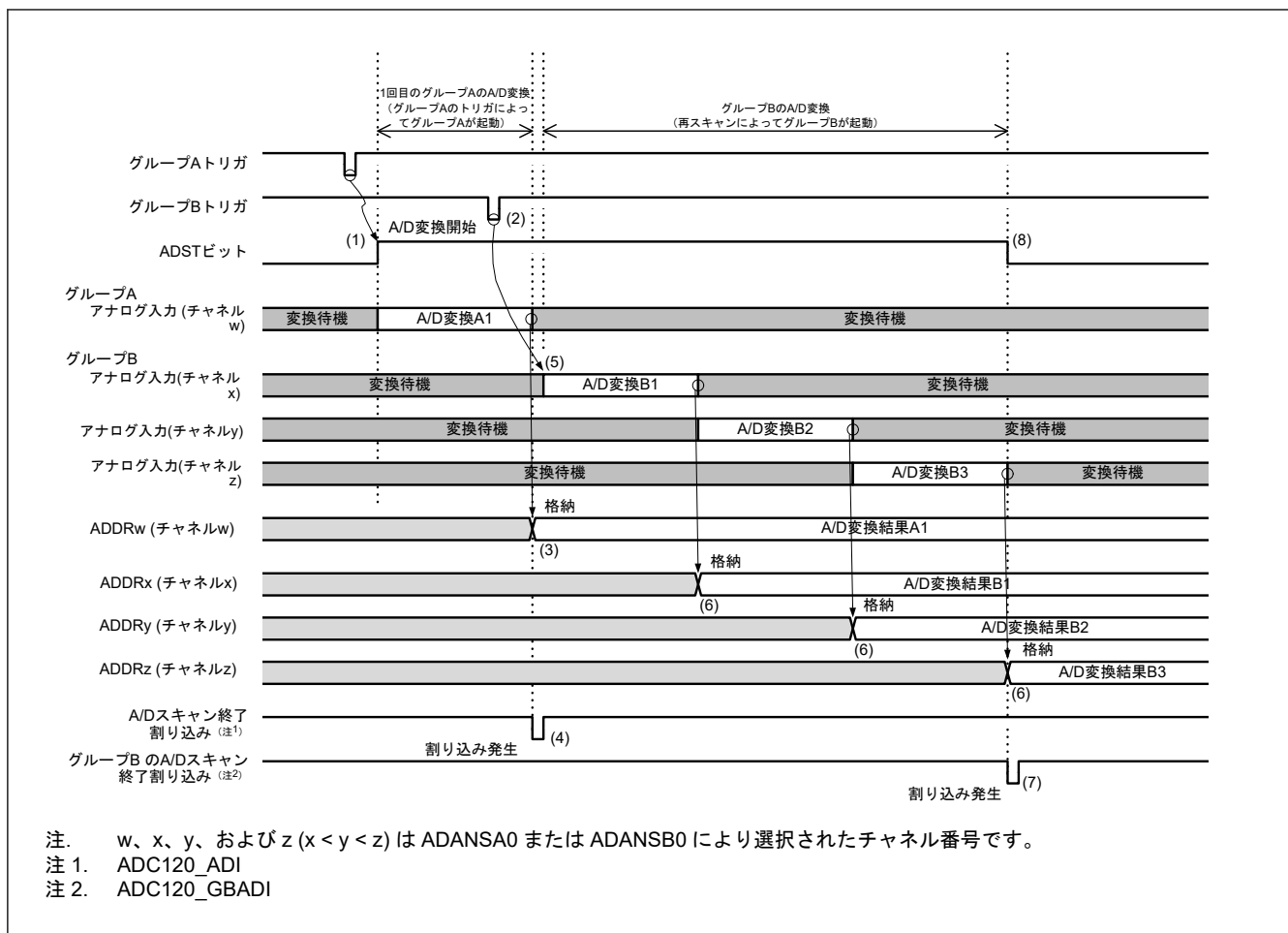
図 39.20 グループ優先動作の例 1-3: グループ A スキャン中のグループ B トリガ入力、再スキャンあり (ADGSPCR.GBRSCN = 1, ADGSPCR.GBRP = 0, および ADGSPCR.LGRRS = 0 の場合)
