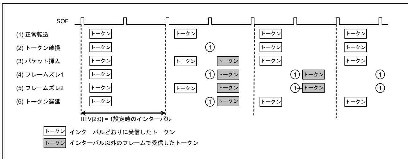
図 28.23 IITV[2:0] = 1 の場合のインターバルエラー発生例
