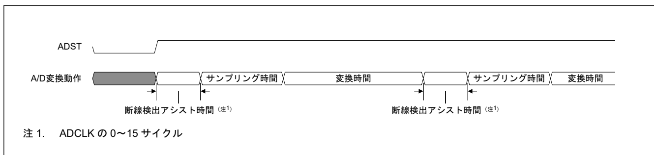
図 39.28 断線検出アシスト機能を使用した場合の A/D 変換動作図
