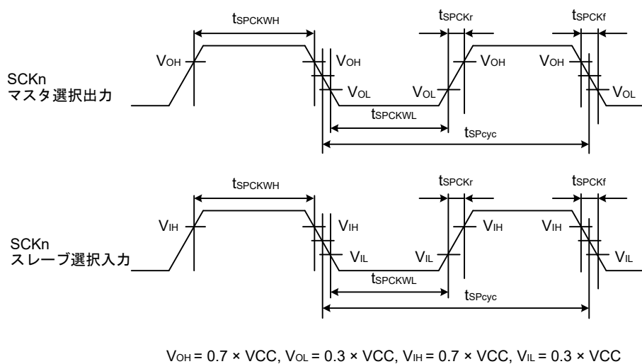
図 47.27 SCI 簡易 SPI モードクロックタイミング
