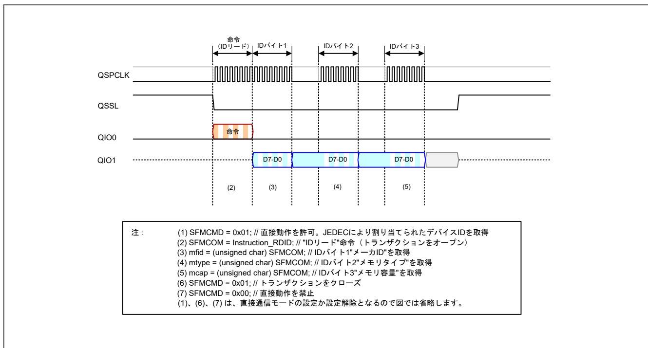
図 33.41 ID リードの直接通信タイミング例
