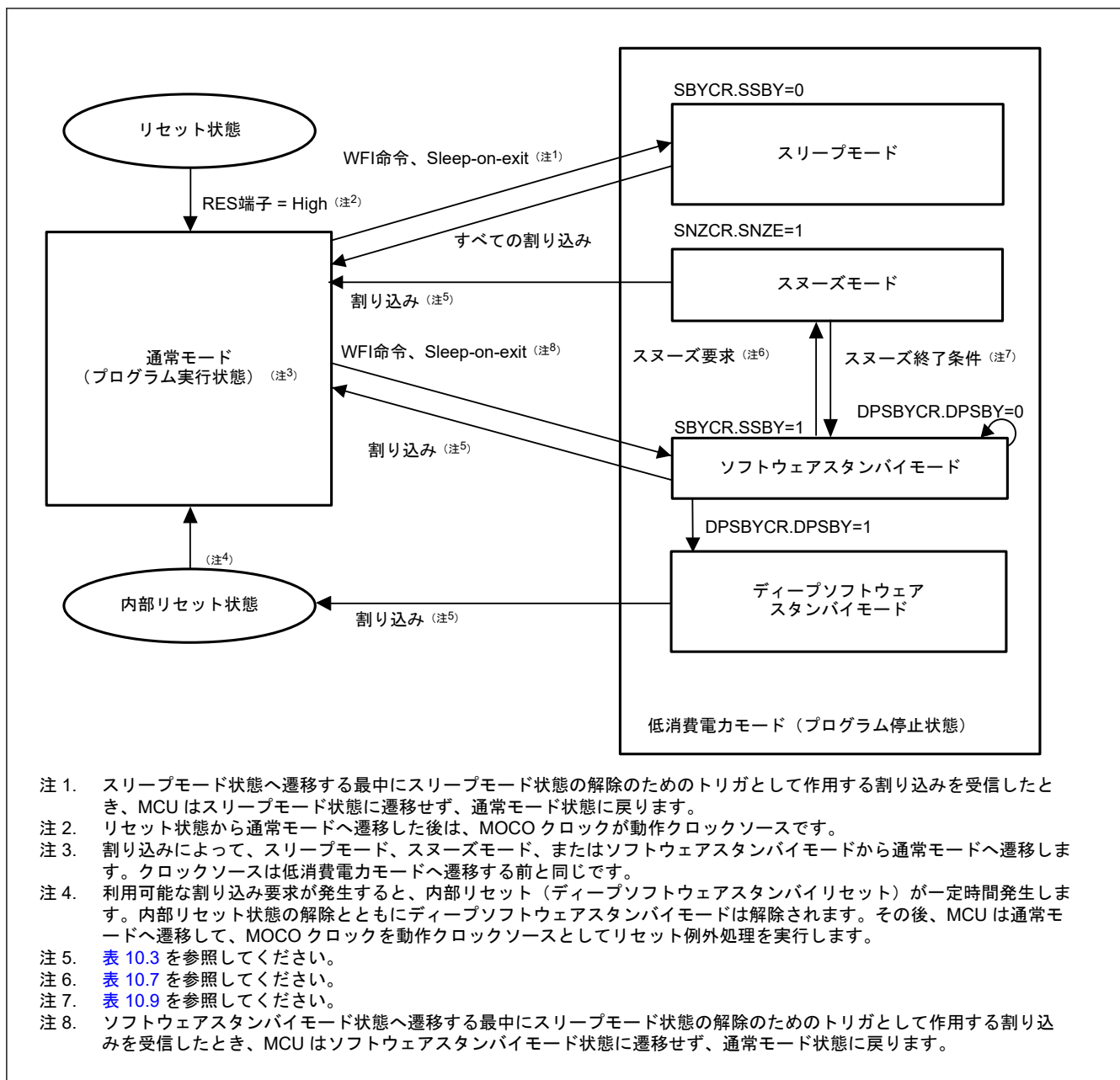
図 10.1 モード遷移
