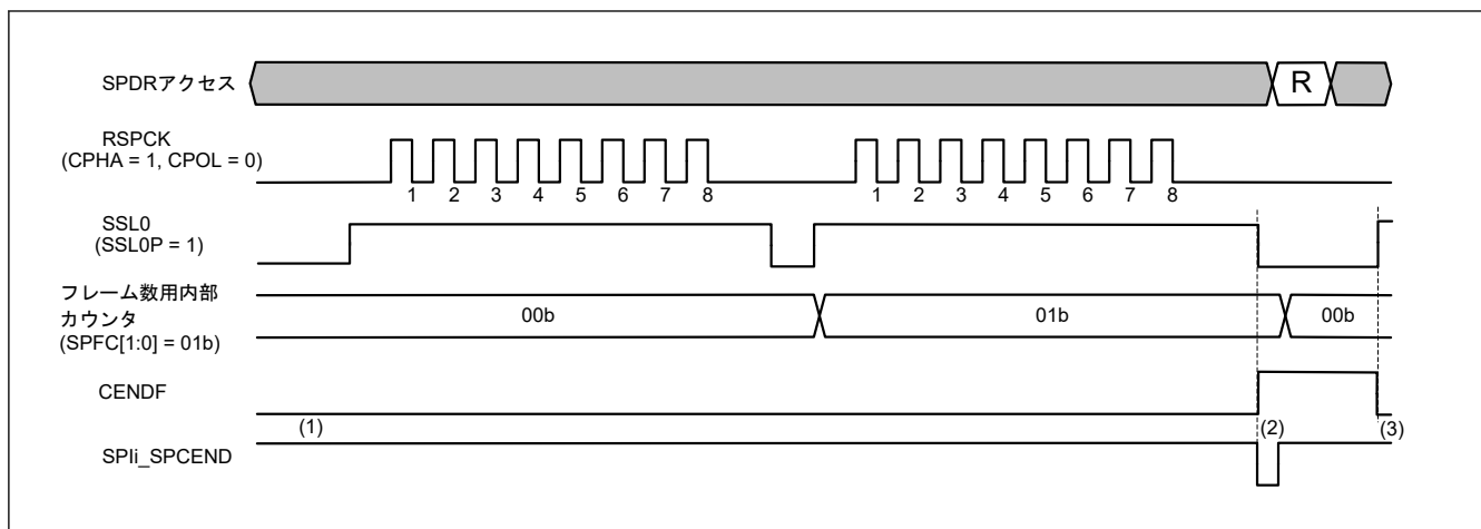
図 32.33 通信終了割り込み動作例 (SPI 動作時の受信専用スレーブモード)
