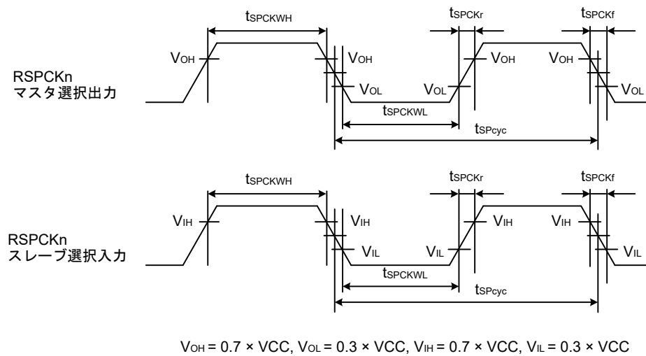
図 47.33 SPI クロックタイミング
