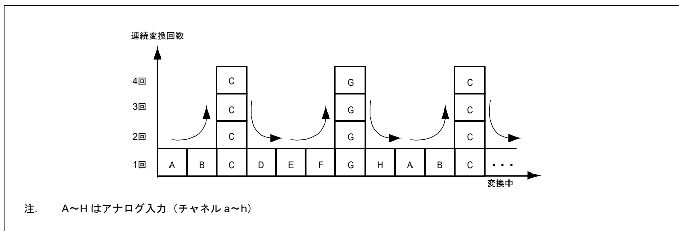
図 39.2 ADADC.ADC[2:0] = 011b および ADADS0 によるアナログ入力 C と G を 1 に選択時のスキャン変換シーケンス
