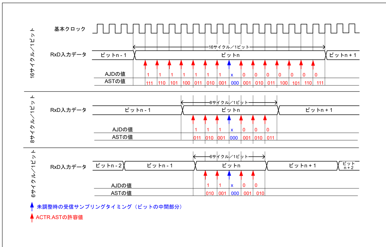
図 29.34 受信サンプリングタイミングの調整動作の概要 (内部クロックを使用した調歩同期式モード)
