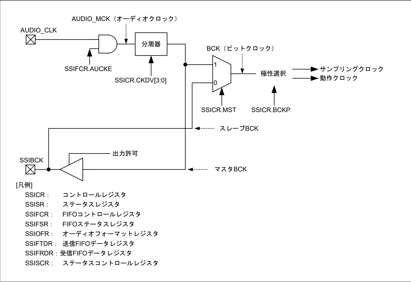
図 34.4 SSIE クロック構成
