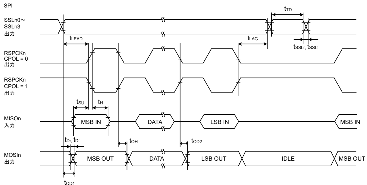
図 47.34 CPHA = 0 の場合におけるマスタの SPI タイミング
