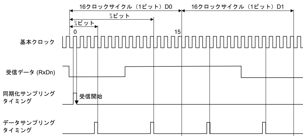
図 29.59 マンチェスタモードでのデータ受信サンプリングタイミング
