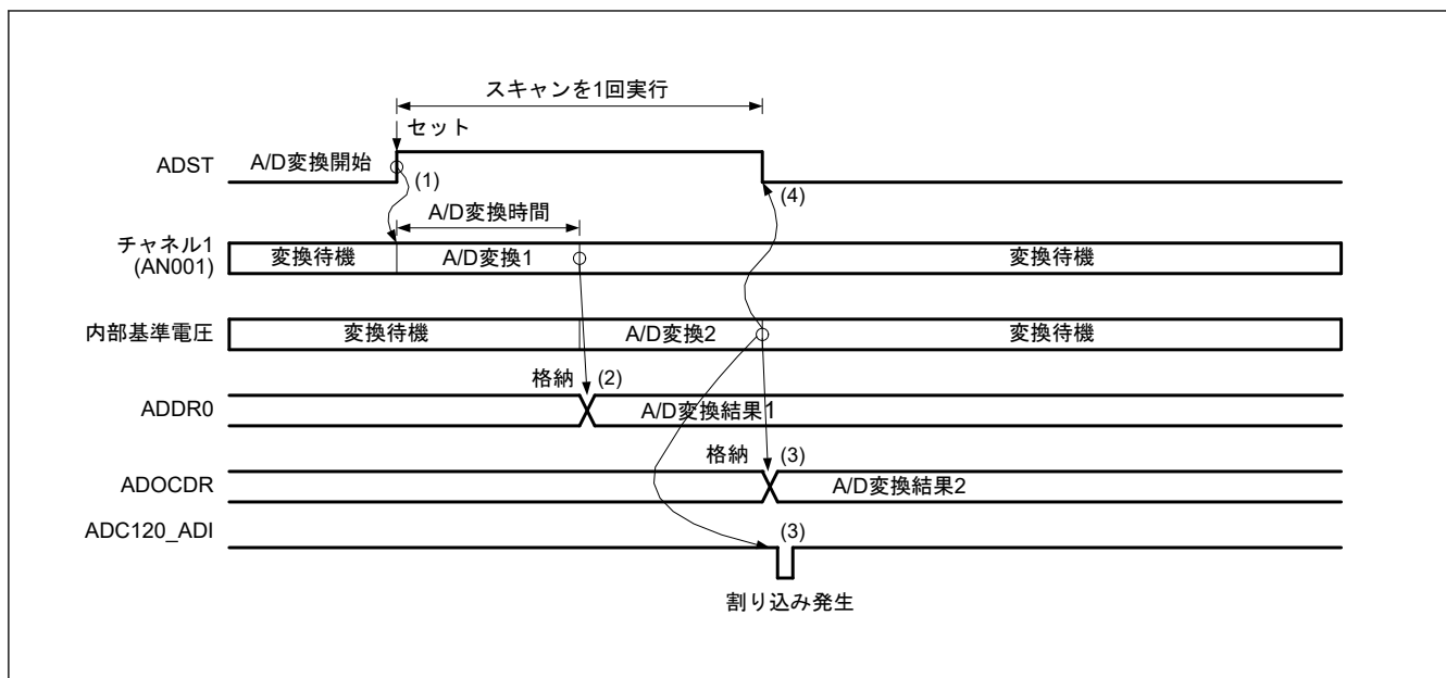
図 39.9 シングルスキャンモードの基本動作例 (AN000、内部基準電圧選択時)
