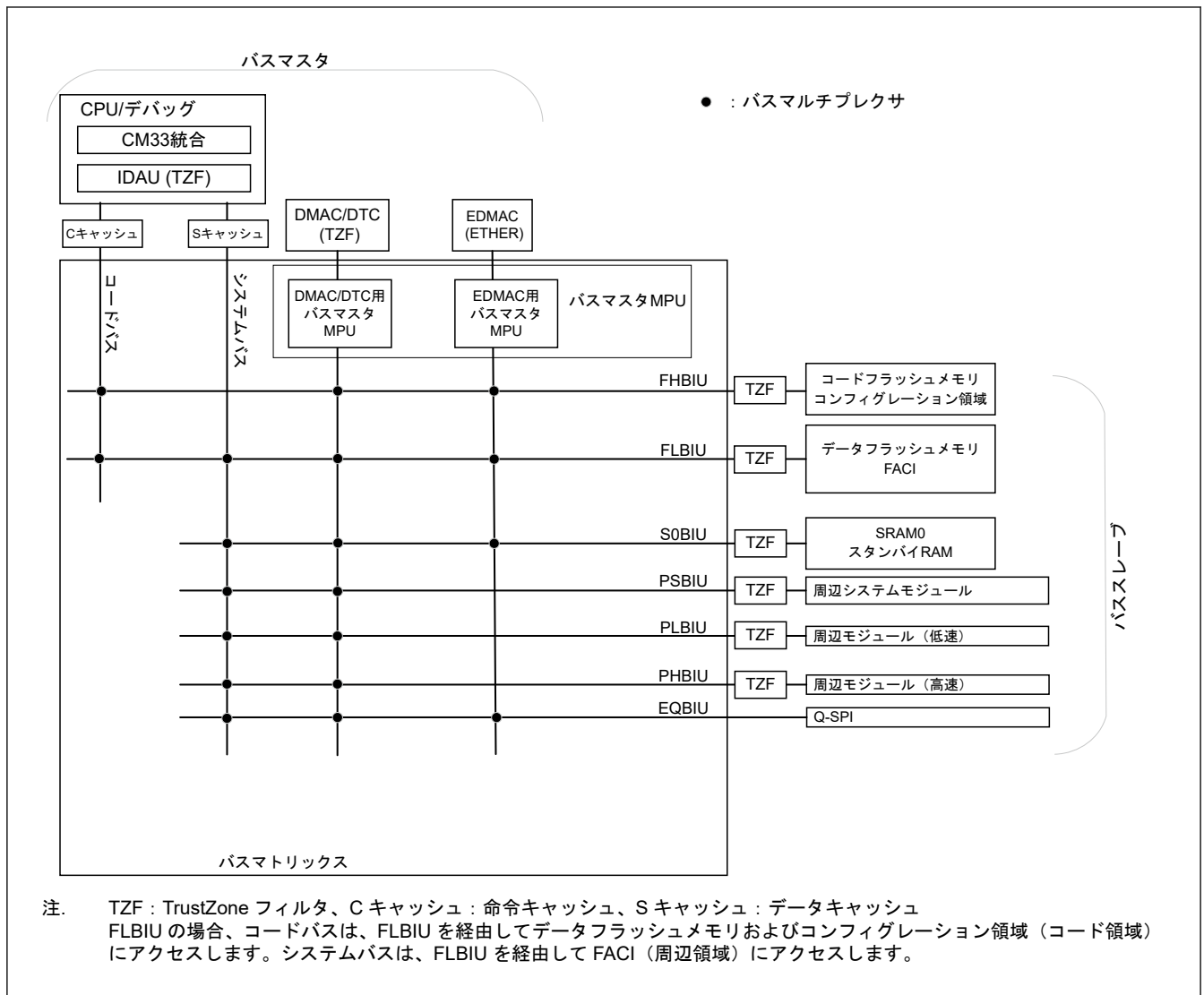
図 14.1 バス接続
