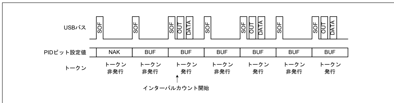
図 28.18 IITV[2:0] = 1 の場合のトークン発行の有無
