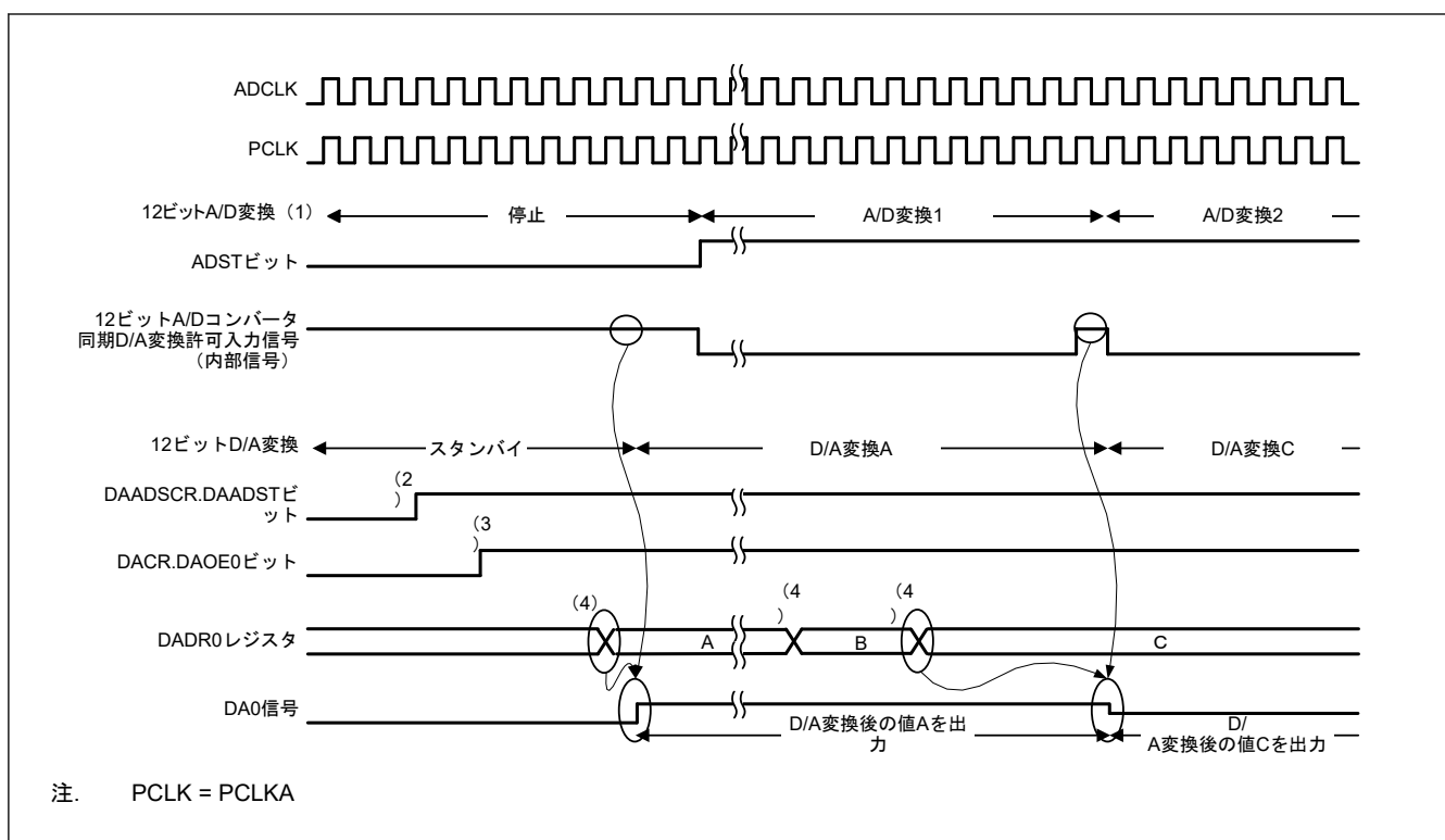
図 40.3 DAC12 を ADC12 に同期して変換する例
