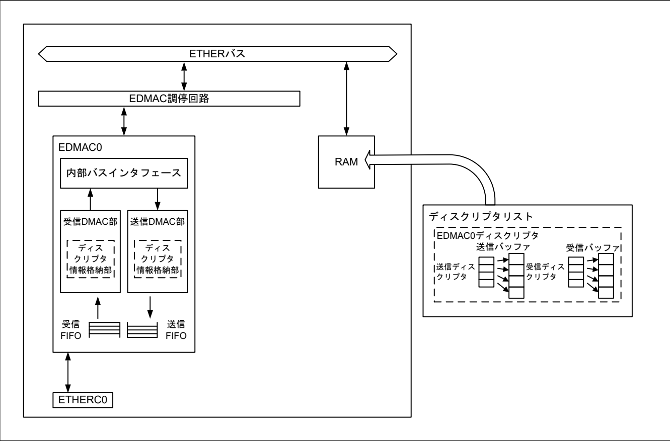
図 27.2 メモリ内のディスクリプタおよび送受信バッファの構成
