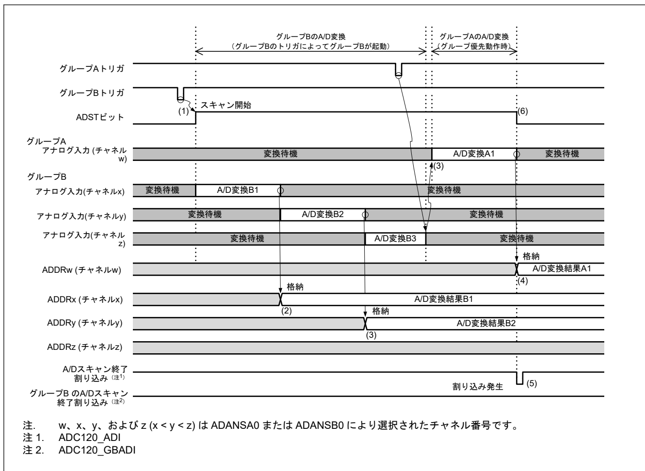
図 39.21 グループ優先動作の例 1-4 : グループ B スキャン中のグループ A トリガ入力、再スキャンなし (ADGSPCR.GBRSCN = 0、ADGSPCR.GBRP = 0、および ADGSPCR.LGRRS = 0 の場合)
