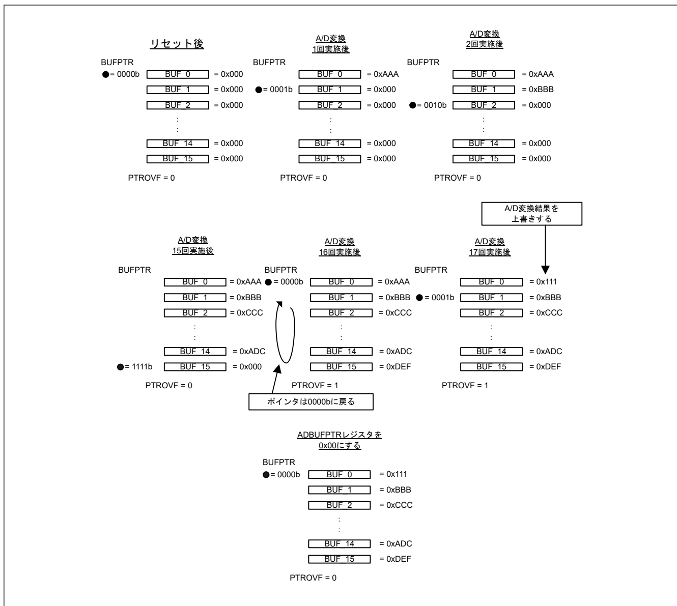
図 39.32 データバッファ、ポインタ、およびオーバーフローフラグの動作概略図
