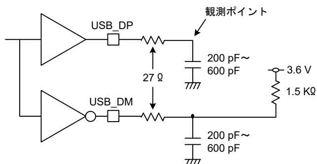
図 47.55 Low-speed モードにおける測定回路
