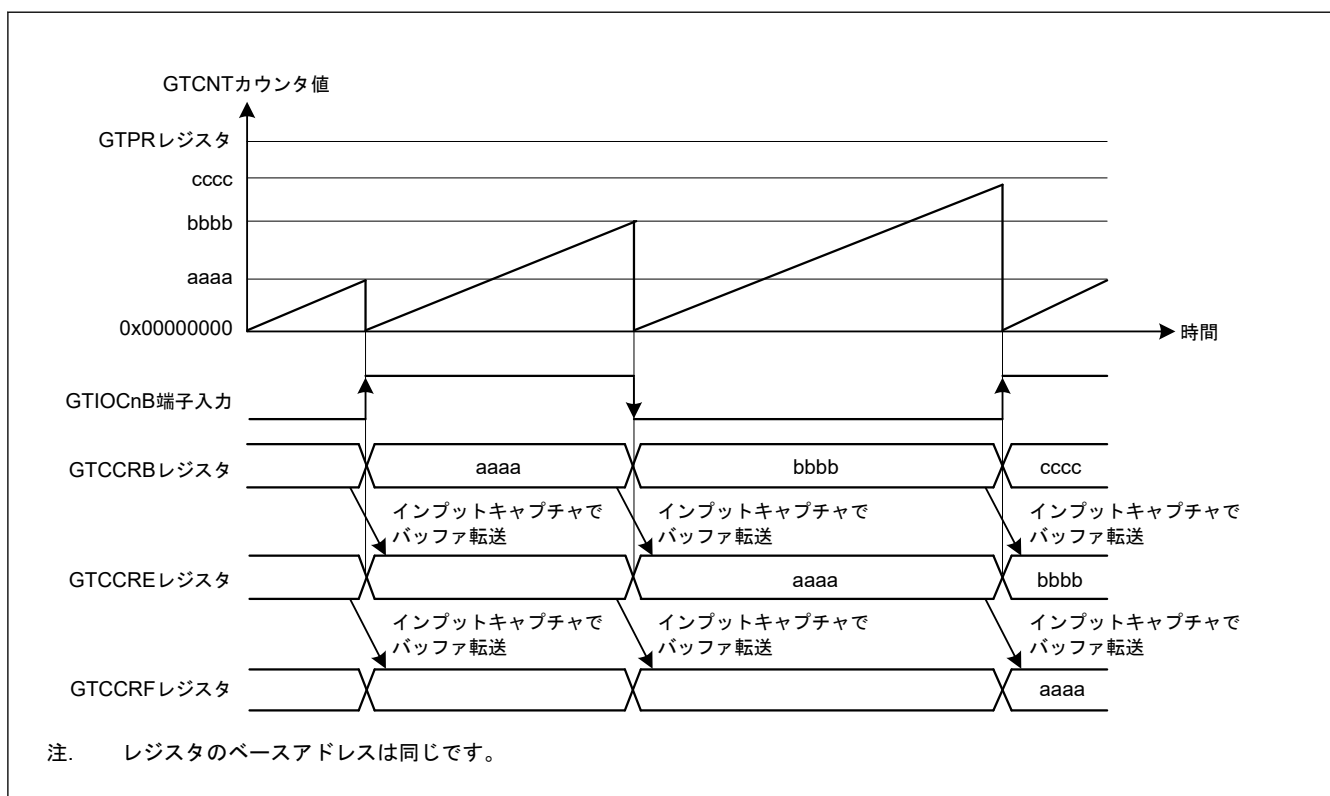
図 21.18 GTCRB レジスタのダブルバッファ動作例 (GTIOCnB 端子入力の両エッジでインプットキャプチャ、のこぎり波でアップカウント、GTIOCnB 端子入力の両エッジで GTCNT カウンタクリアの場合)
