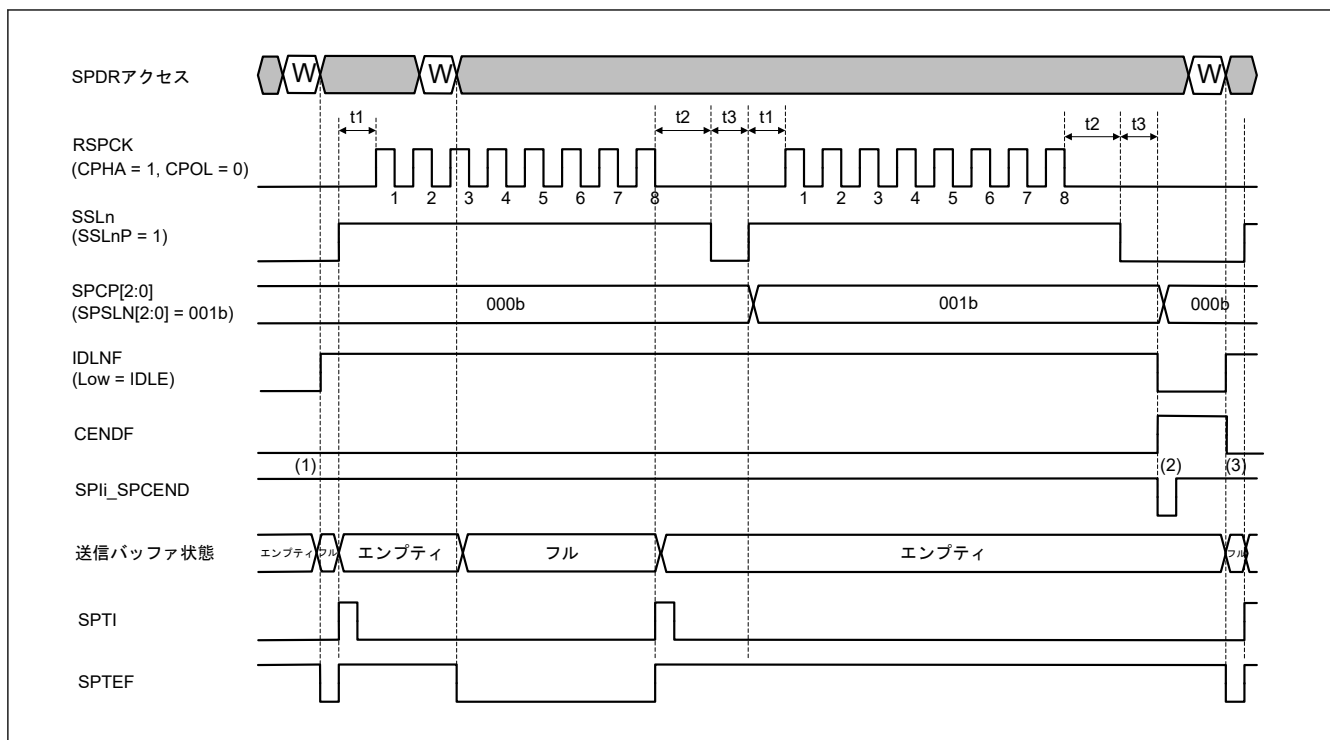
図 32.31 通信終了割り込み動作例（送受信／送信マスターモード）
