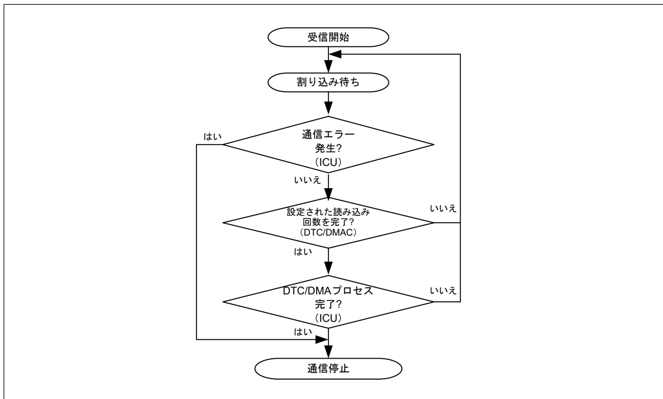
図 34.55 受信手順
