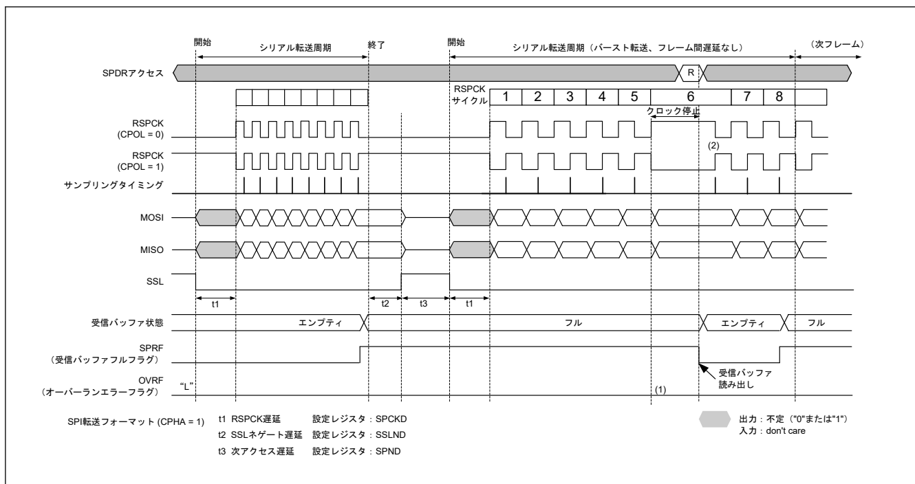
図 32.40 マスタモードの受信バッファフル状態でシリアル転送が継続する場合のクロック停止波形(バースト転送でフレーム間遅延なし、CPHA = 1)
