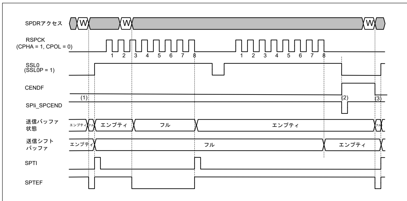
図 32.32 通信終了割り込み動作例 (SPI 動作時の送受信/送信スレーブモード)
