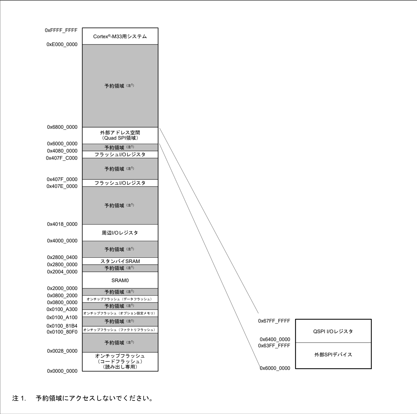
図 4.2 外部アドレス空間の対応関係
