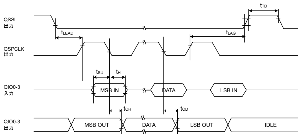
図 47.41 送受信タイミング
