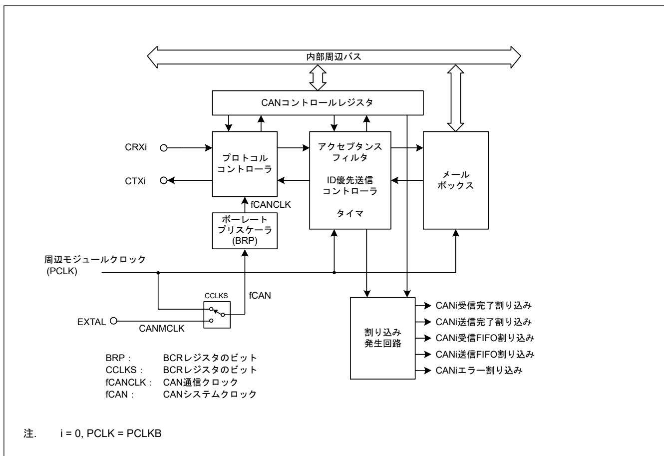
図 31.1 CAN モジュールブロック図
