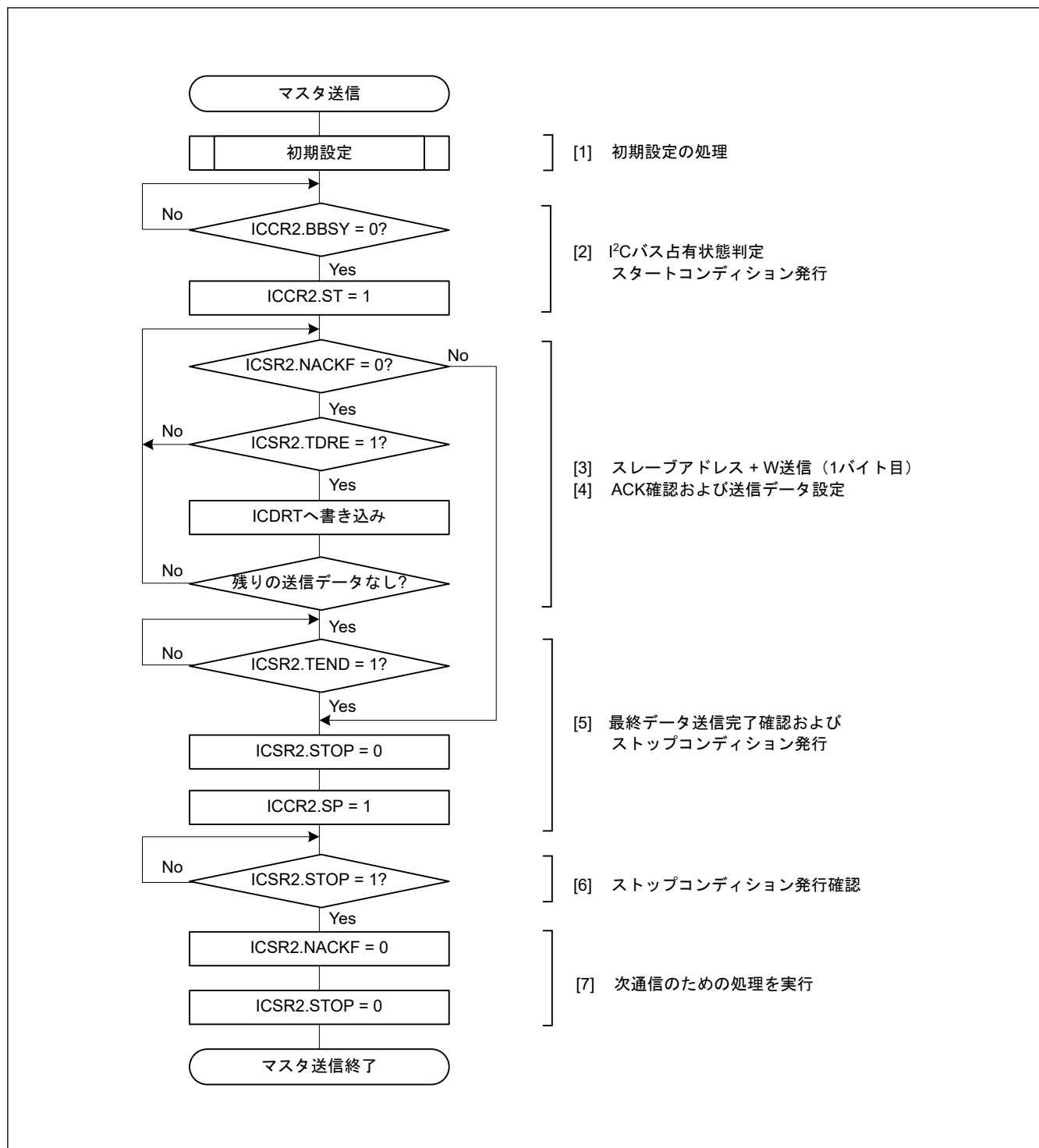
図 30.6 マスタ送信のフローチャート例
