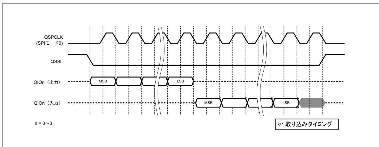
図 33.8 シリアルインタフェースの基本タイミング (SPI モード 0)
