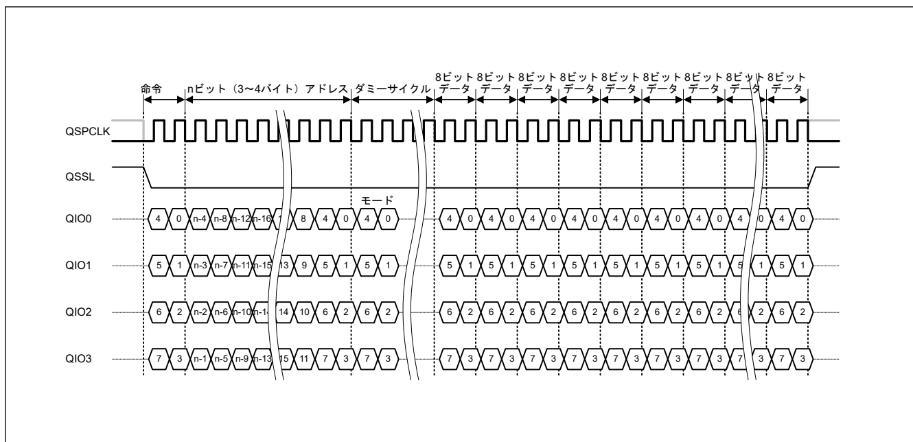
図 33.7 Quad-SPI プロトコル例 (ファストリード Quad I/O)
