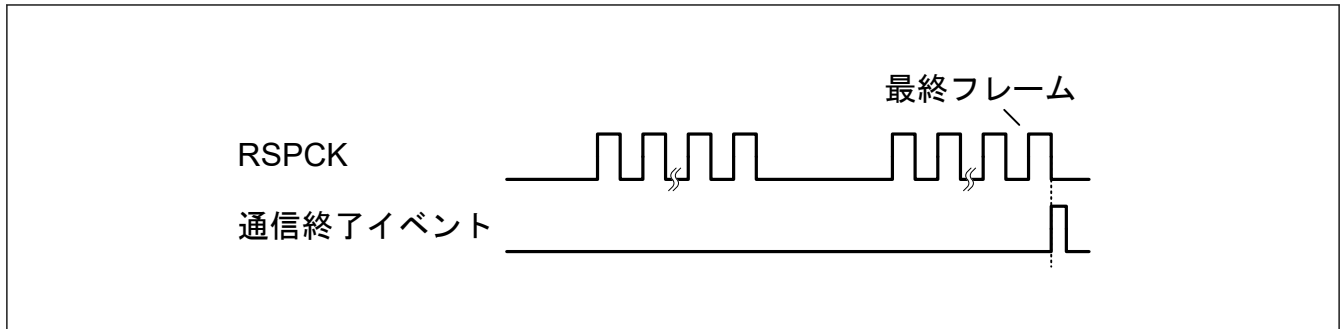
図 32.66 通信終了イベント出力タイミング (受信専用スレーブモード、クロック同期式動作)
