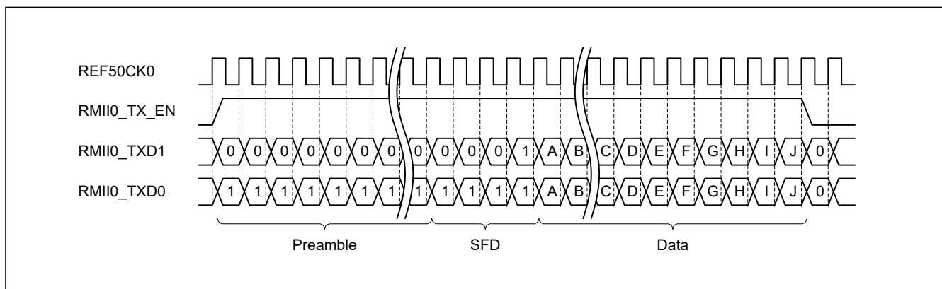
図 26.5 RMII フレーム送信タイミング (正常送信時)
