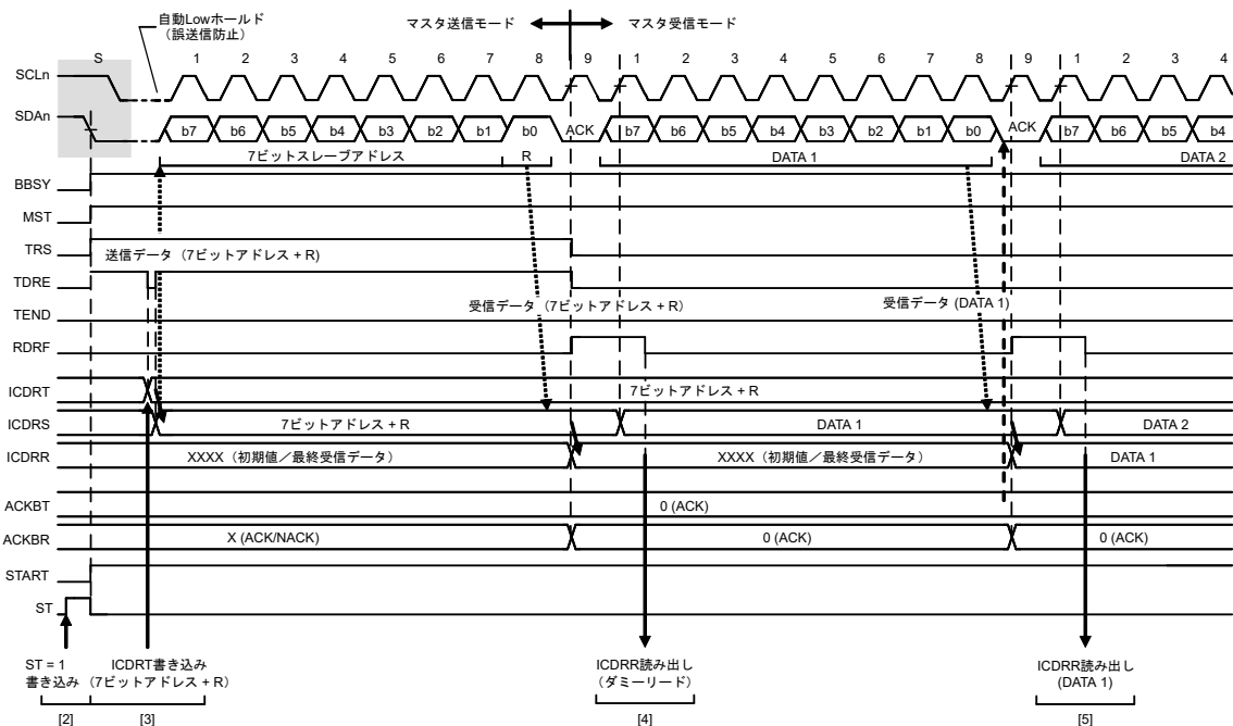
図 30.12 マスタ受信の動作タイミング (1) (7 ビットアドレスフォーマットで RDRFS = 0 の場合)
