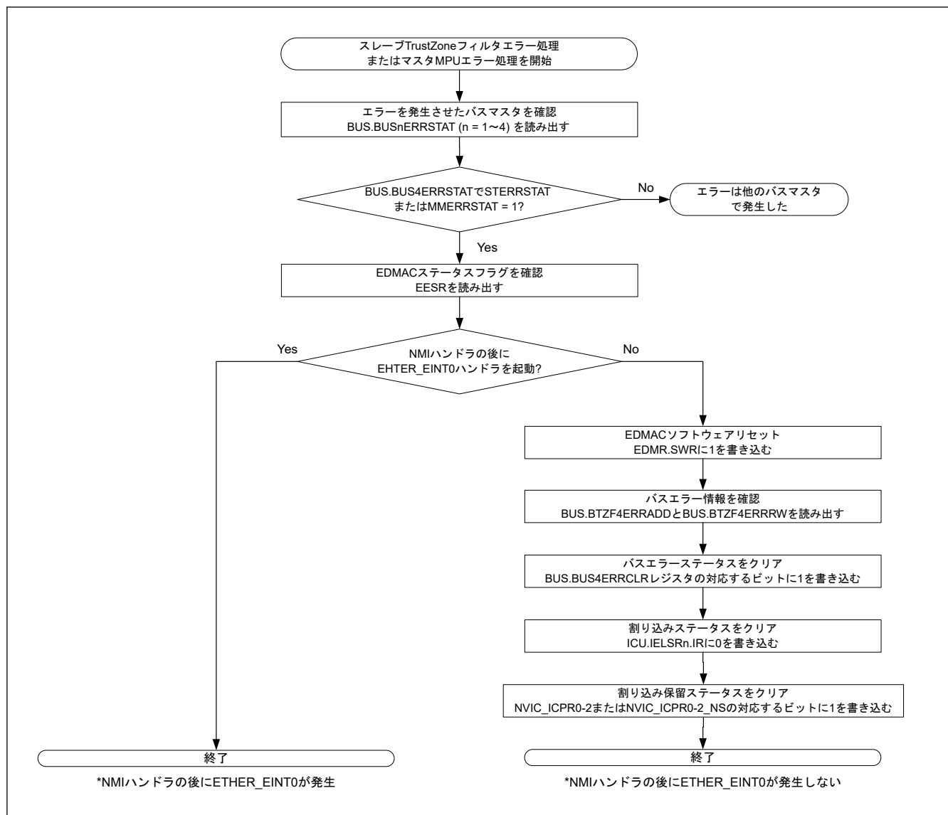
図 27.9 NMI ハンドラにおけるバス転送エラーの処理
