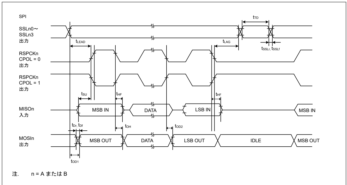
図 47.35 CPHA = 0 で、PCLKA/2 にビットレートが設定されている場合におけるマスタの SPI タイミング
