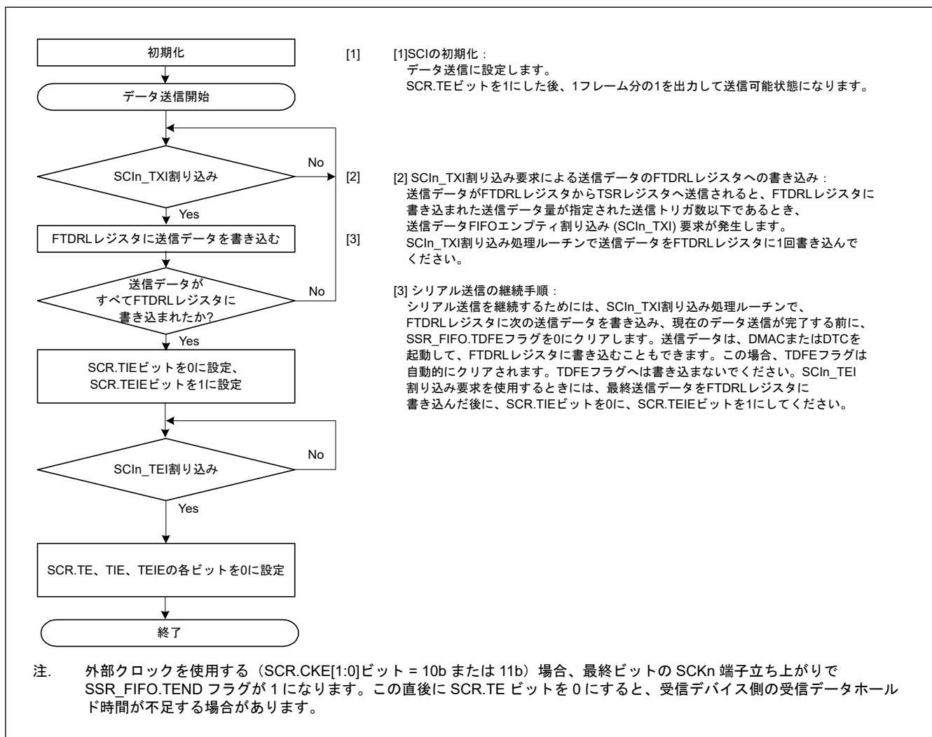
図 29.70 クロック同期式モードにおけるシリアル送信のフローチャート例 (FIFO 選択時)
