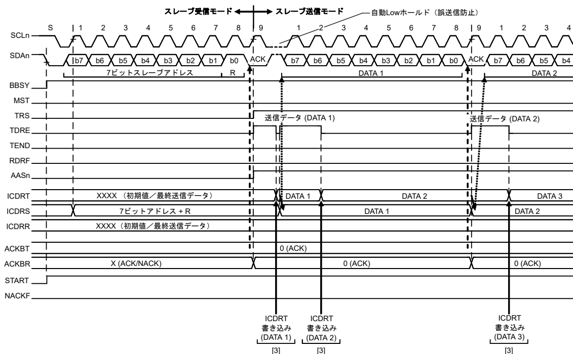
図 30.16 スレーブ送信の動作タイミング (1) (7 ビットアドレスフォーマット)
