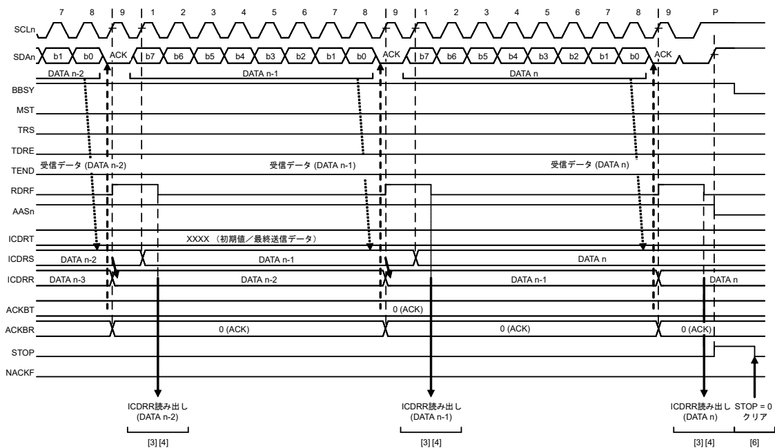
図 30.20 スレープ受信の動作タイミング (2) ( RDRFS = 0 の場合)
