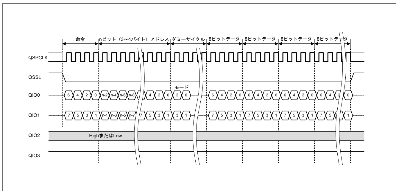
図 33.6 Dual-SPI プロトコル例（ファストリード Dual I/O）
