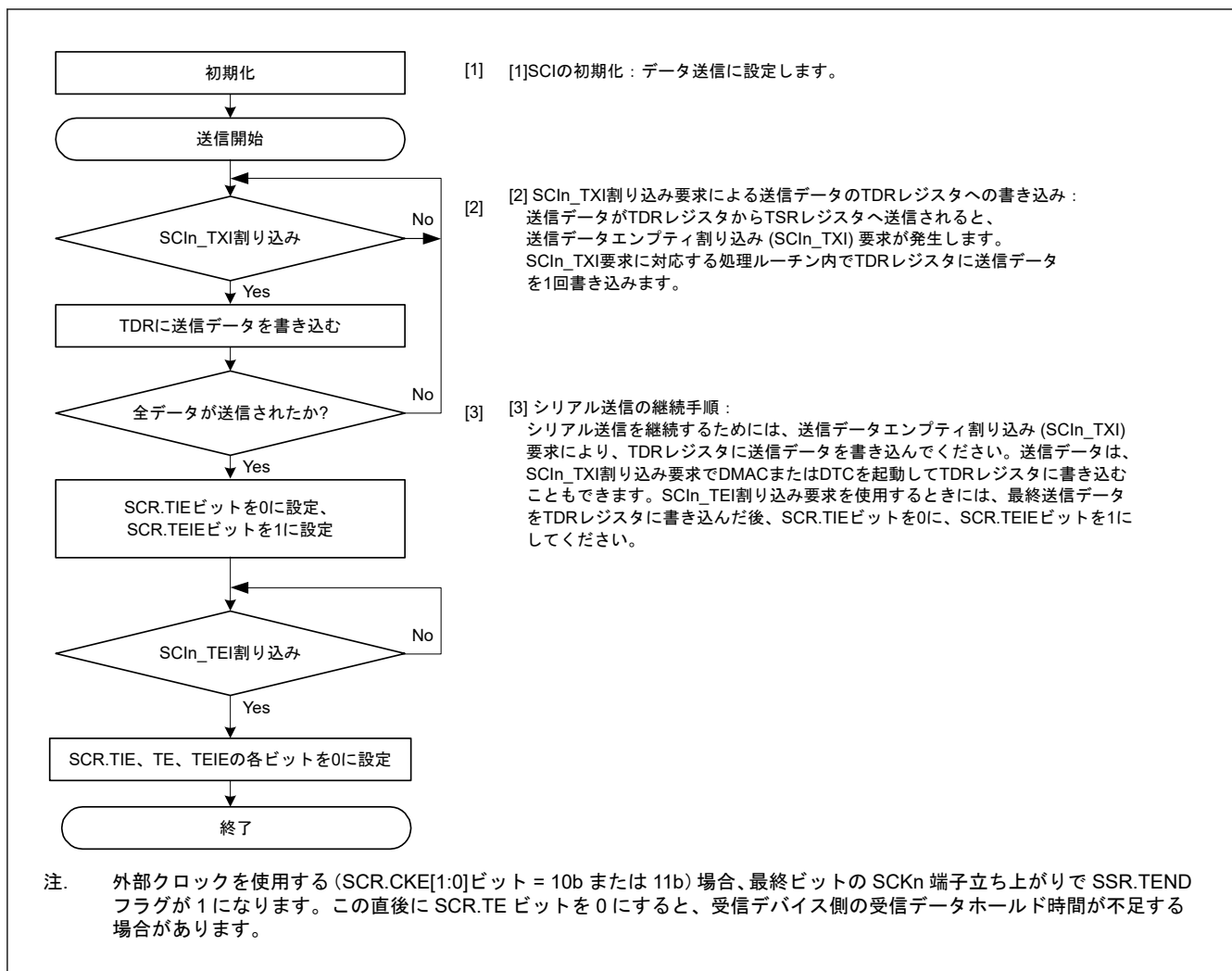
図 29.69 クロック同期式モードにおけるシリアル送信のフローチャート例 (非 FIFO 選択時)
