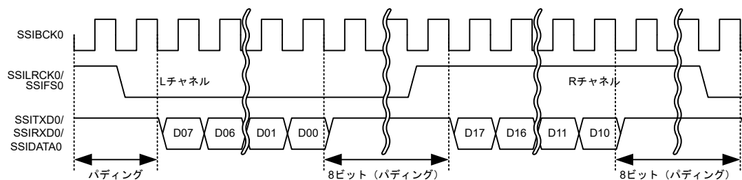
図 34.11 パディングビットの極性
