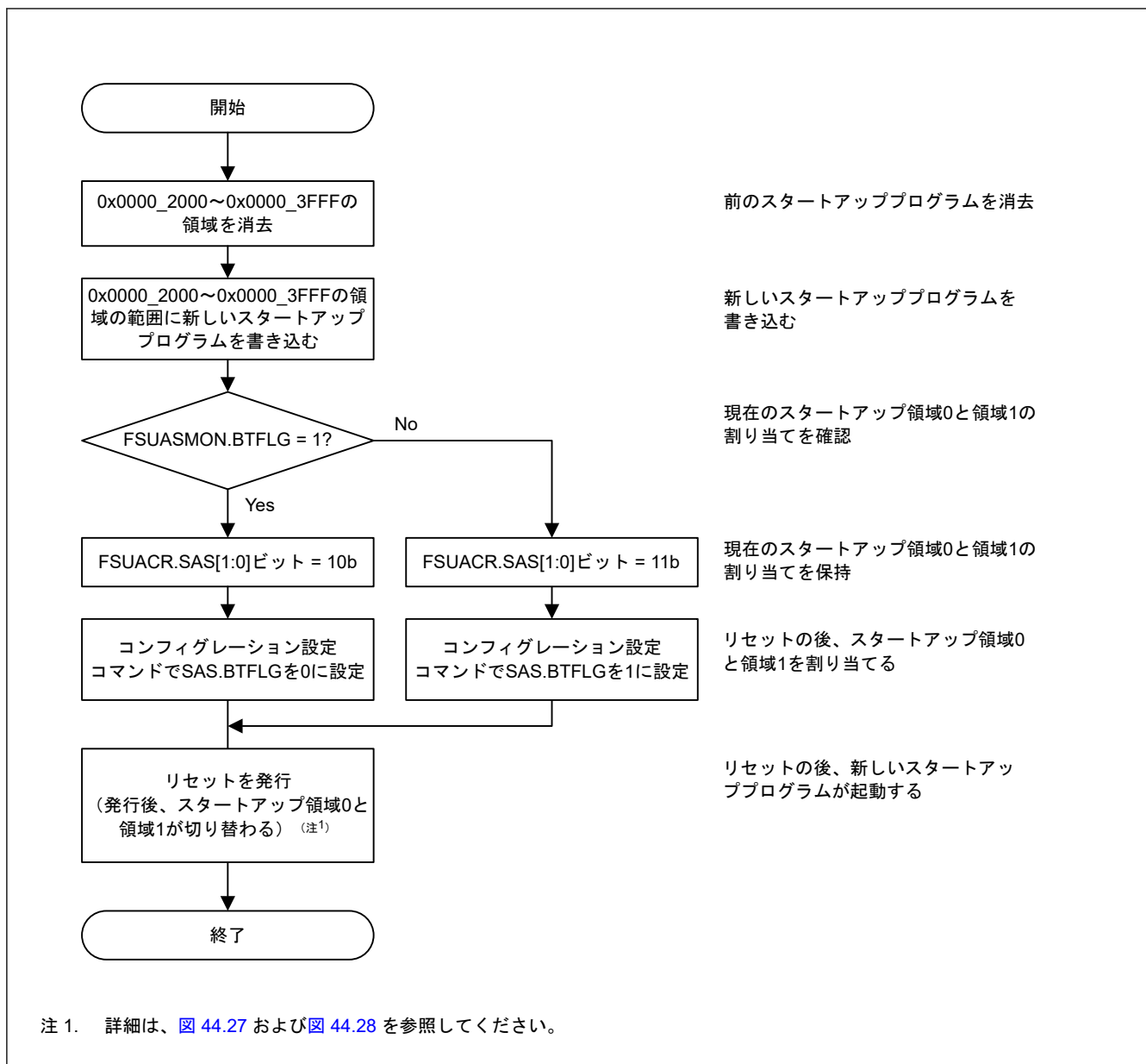
図 44.29 スタートアッププログラムプロテクションの概念
