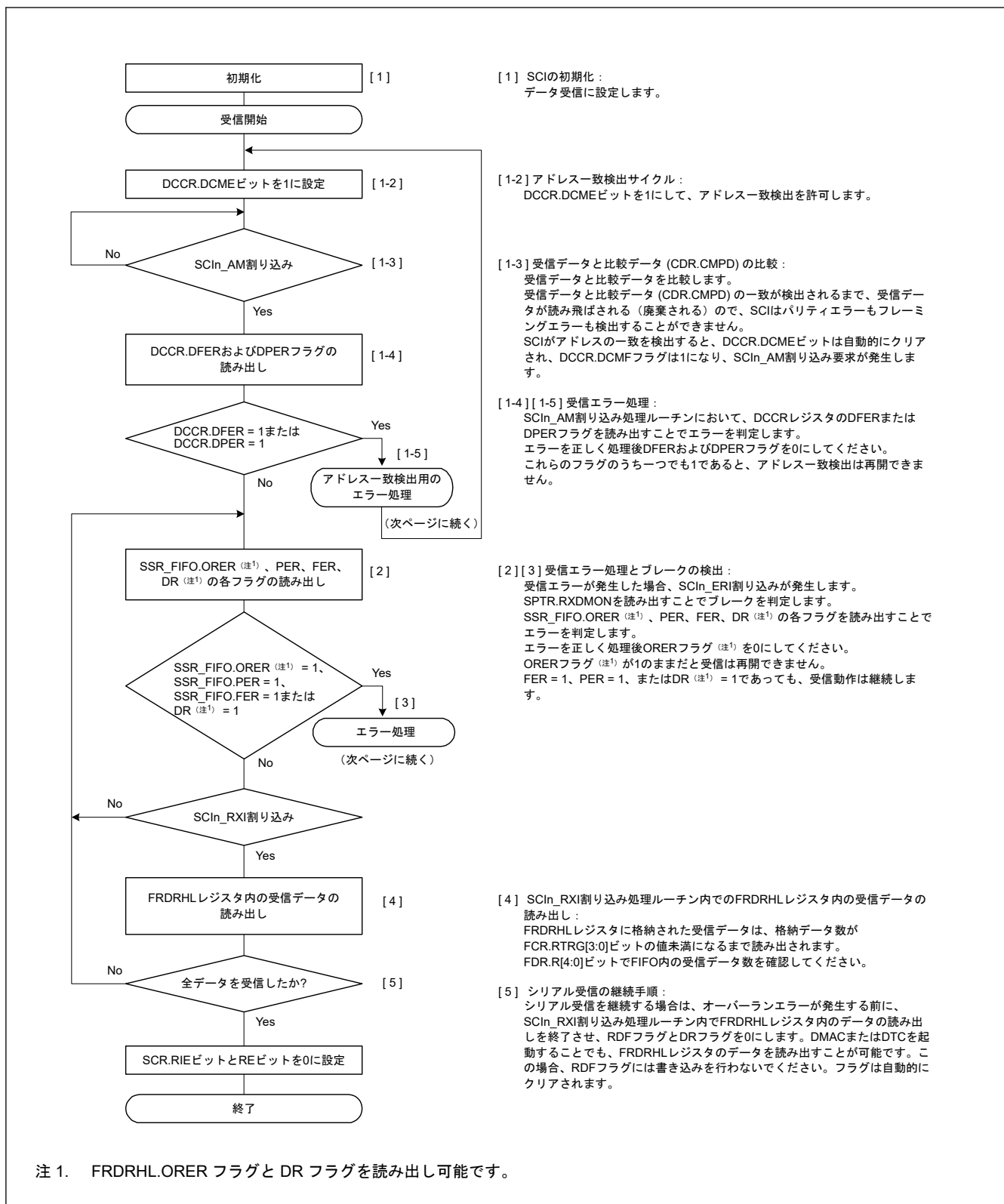
図 29.28 調歩同期式モードにおけるシリアル受信のフローチャート例 (FIFO 選択、アドレス一致検出有効時) (1)
