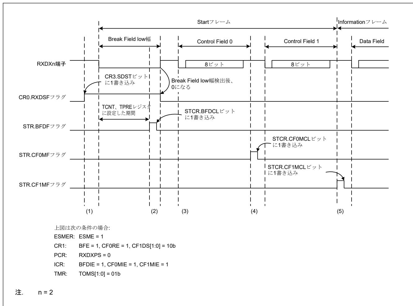
図 29.106 Start Frame 受信時の動作例
