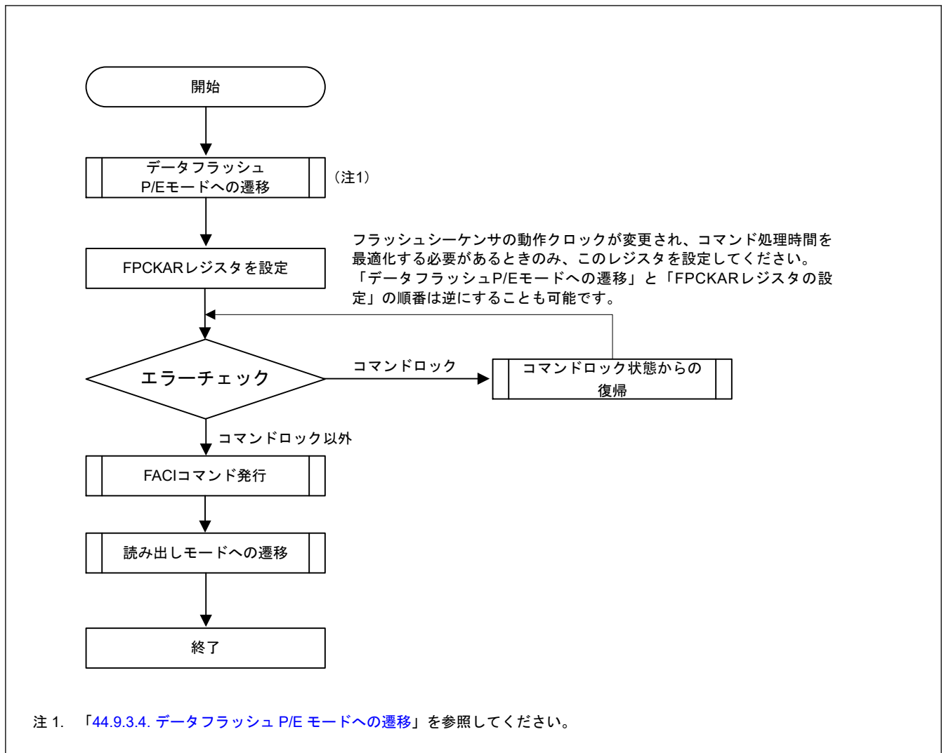
図 44.9 データフラッシュ P/E モードでのコマンド使用概要
