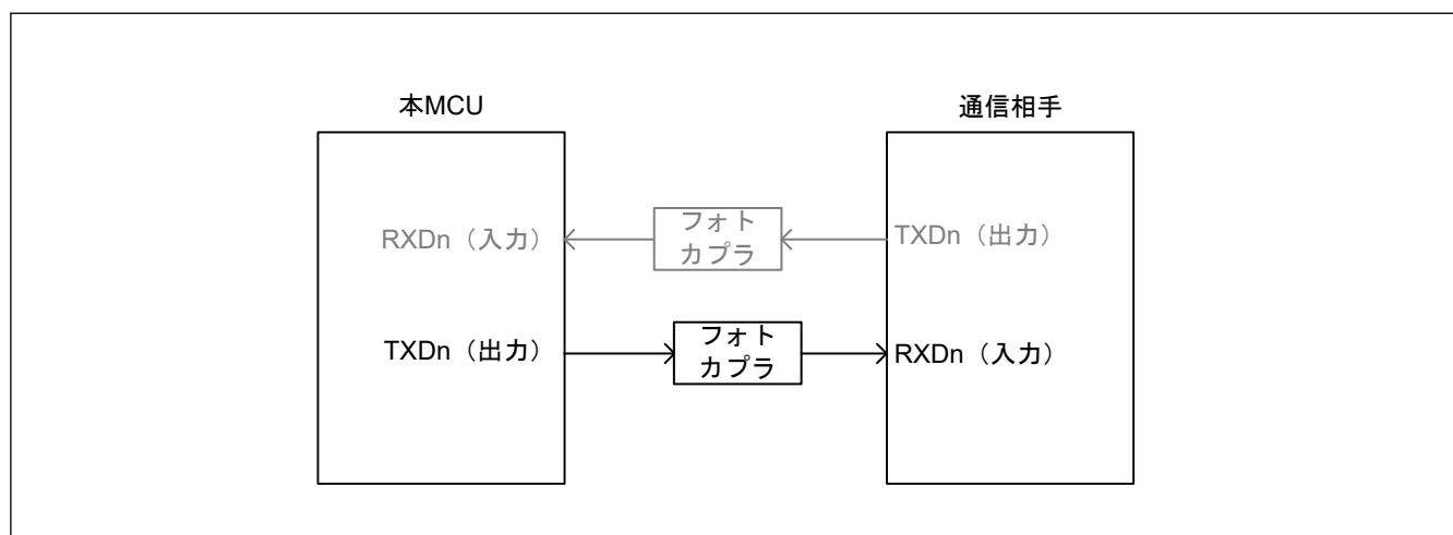
図 29.35 フォトカプラを通過する送信イメージのブロック図
