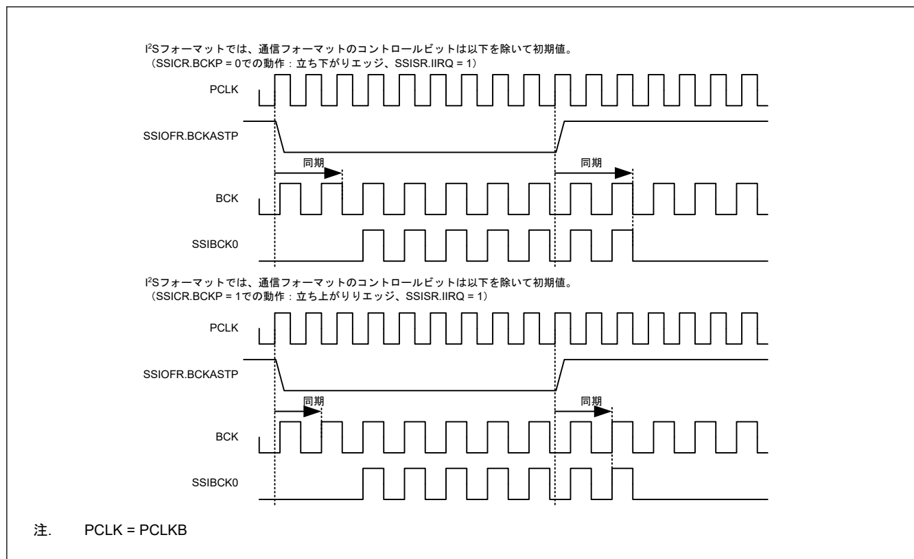
図 34.45 SSIOFR.BCKASTP による SSIBCK0 停止の例
