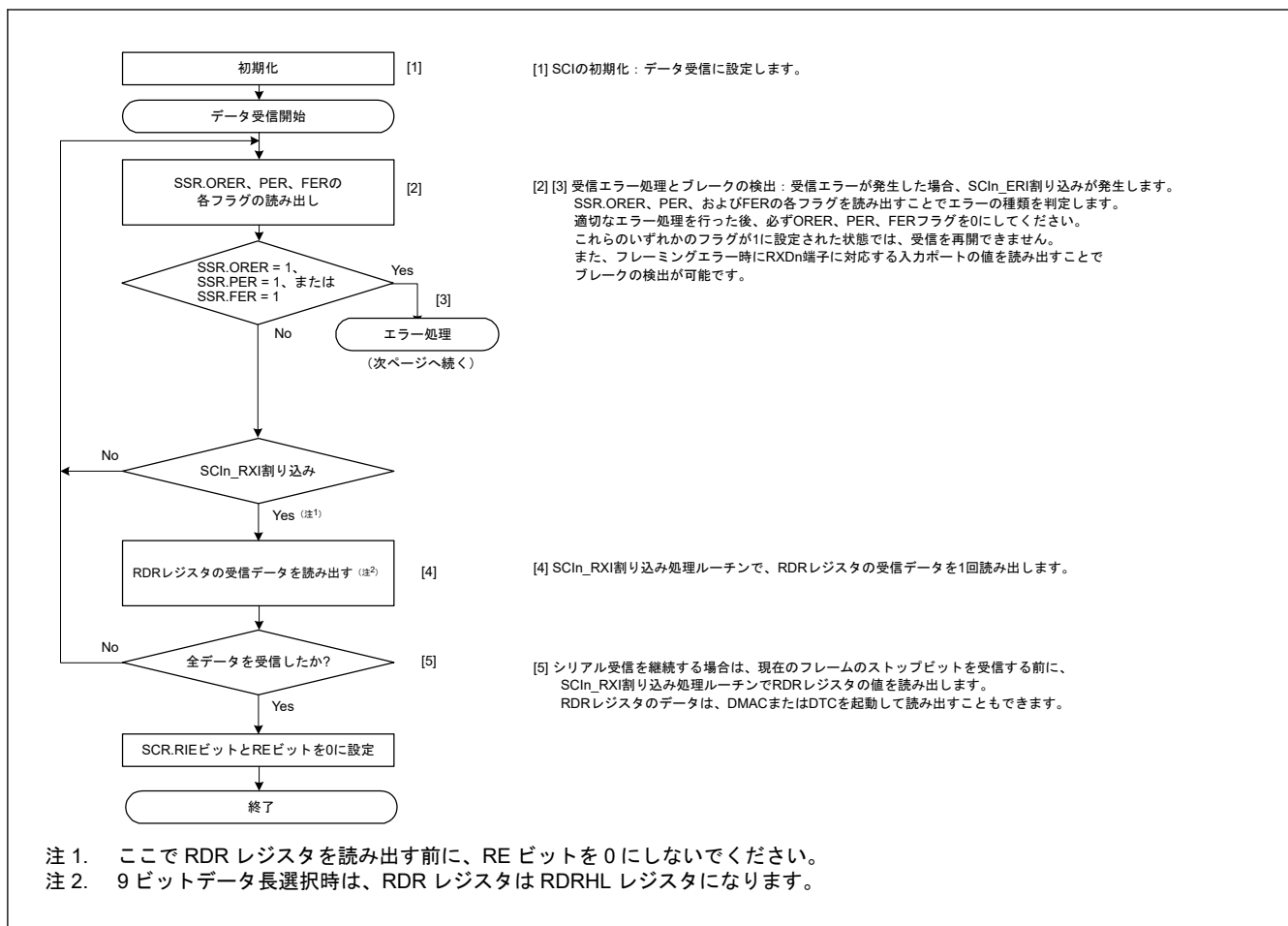
図 29.20 調歩同期式モードにおけるシリアル受信のフローチャート例（非 FIFO 選択、アドレス一致検出無効時） (1)
