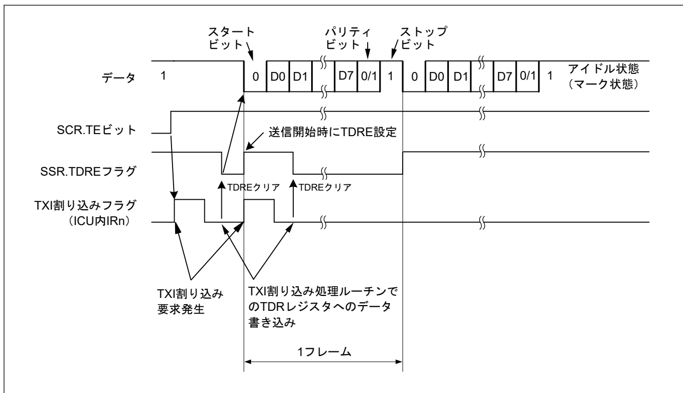
図 29.14 調歩同期式モードにおけるシリアル送信の動作例 (4) (8 ビットデータ/パリティあり/1 ストップビット/CTS 機能不使用/送信中～送信完了時、プリアンプル停止)
