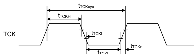
図 47.67 バウンダリスキャン TCK タイミング
