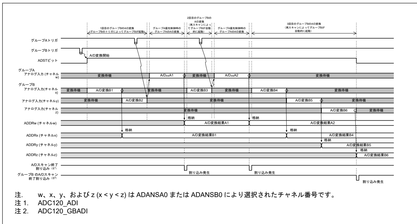
図 39.19 グループ優先動作の例 1-2: グループ B 再スキャン中のグループ A トリガ入力、再スキャンあり (ADGSPCR.GBRSCN = 1、ADGSPCR.GBRP = 0、および ADGSPCR.LGRRS = 0 の場合)
