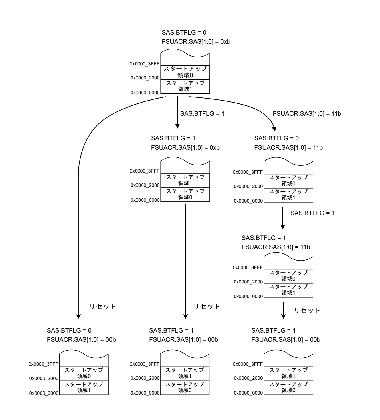
図 44.28 スタートアッププログラムプロテクション設定の遷移例 2
