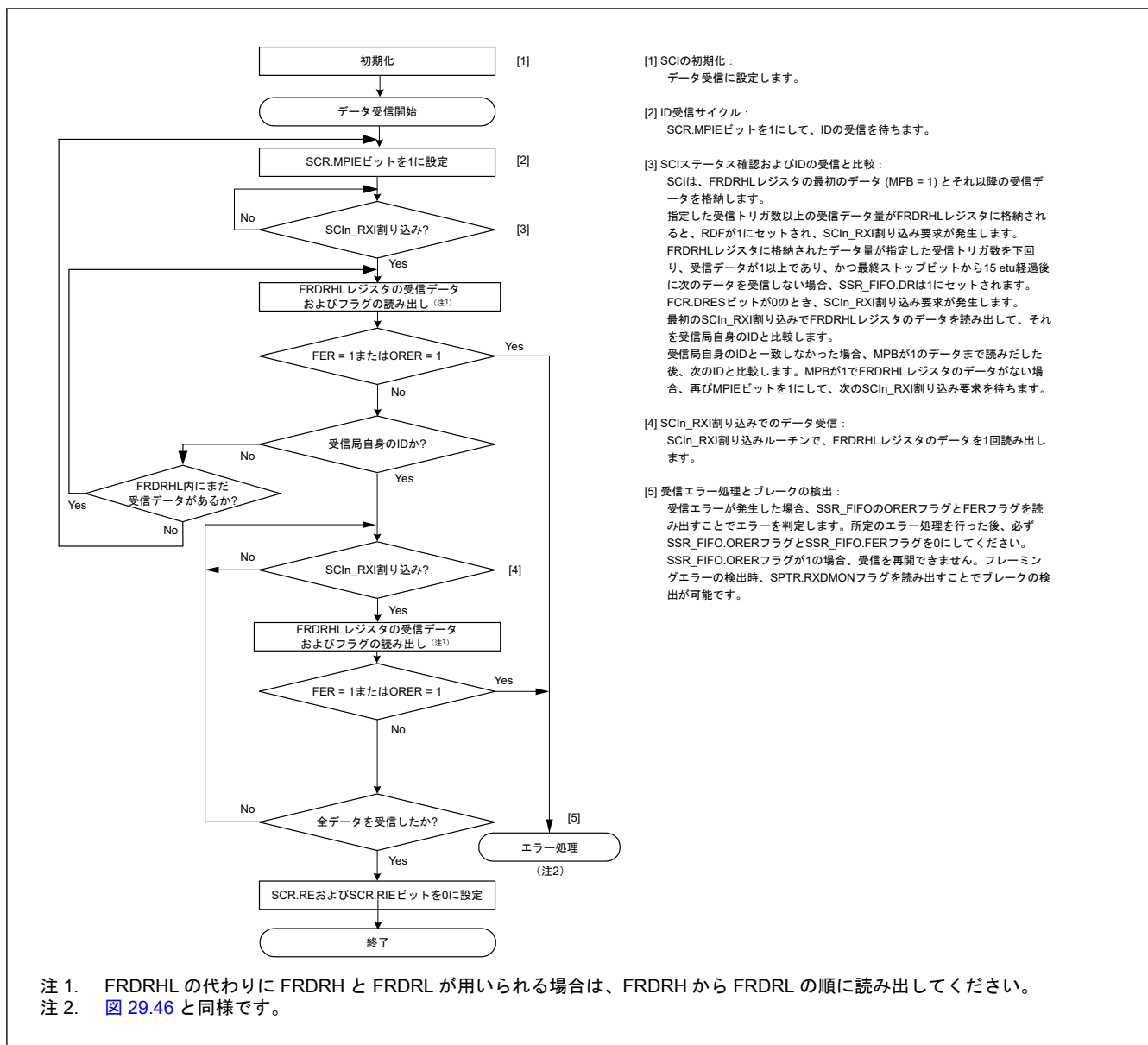
図 29.48 マルチプロセッサモードにおけるシリアル受信のフローチャート例 (FIFO 選択時)
