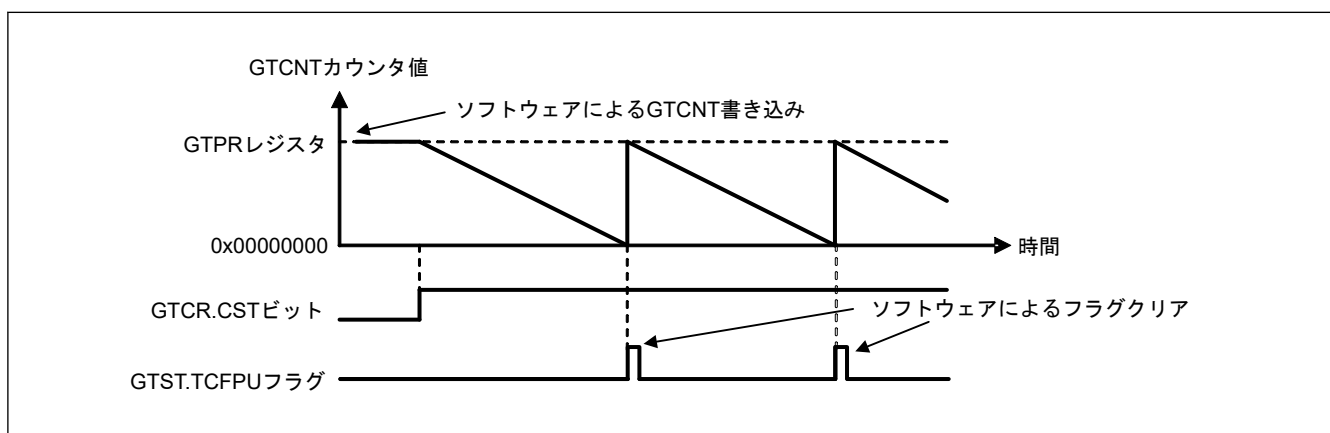
図 21.4 カウントクロックによるダウンカウント時の周期カウント動作例
