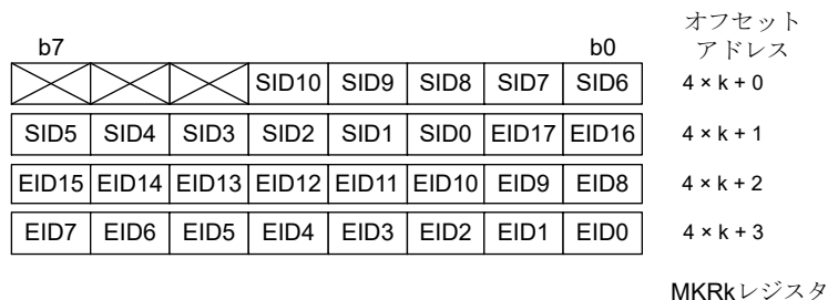
図 31.14 マスクレジスタの構造 ( j = 0 \sim 7 )
