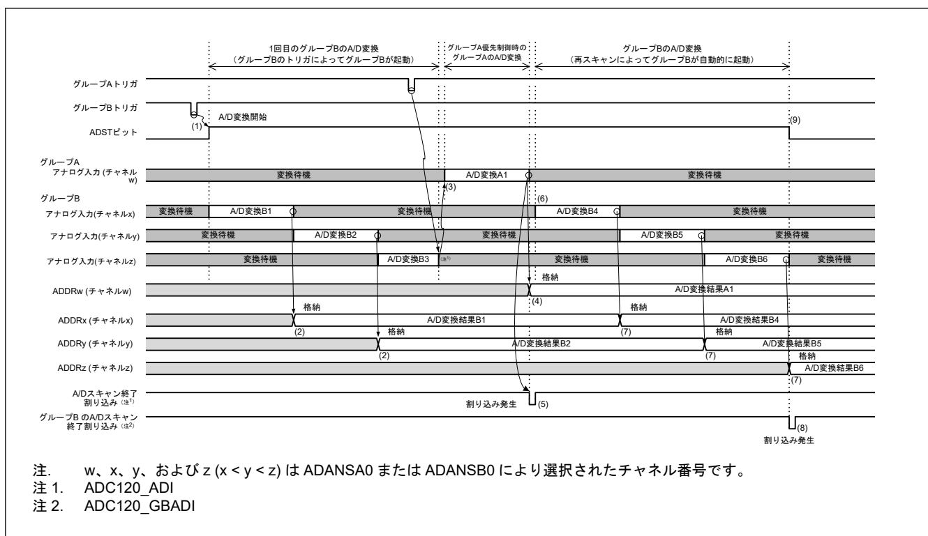
図 39.18 グループ優先動作の例 1-1: グループ B スキャン中のグループ A トリガ入力、再スキャンあり (ADGSPCR.GBRSCN = 1、ADGSPCR.GBRP = 0、および ADGSPCR.LGRRS = 0 の場合)
