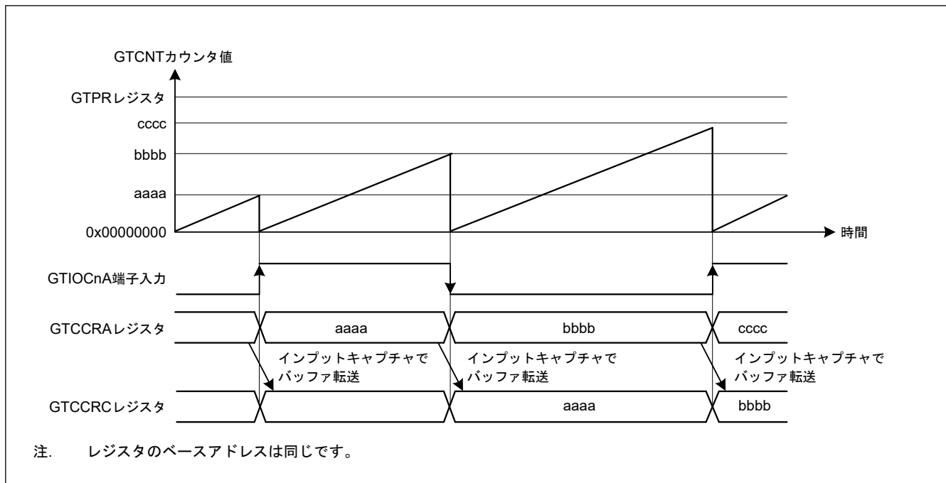
図 21.17 GTCRA レジスタのバッファ動作例 (GTIOCnA 端子入力の両エッジでインプットキャプチャ、のこぎり波でアップカウント、GTIOCnA 端子入力の両エッジで GTCNT カウンタクリアの場合)
