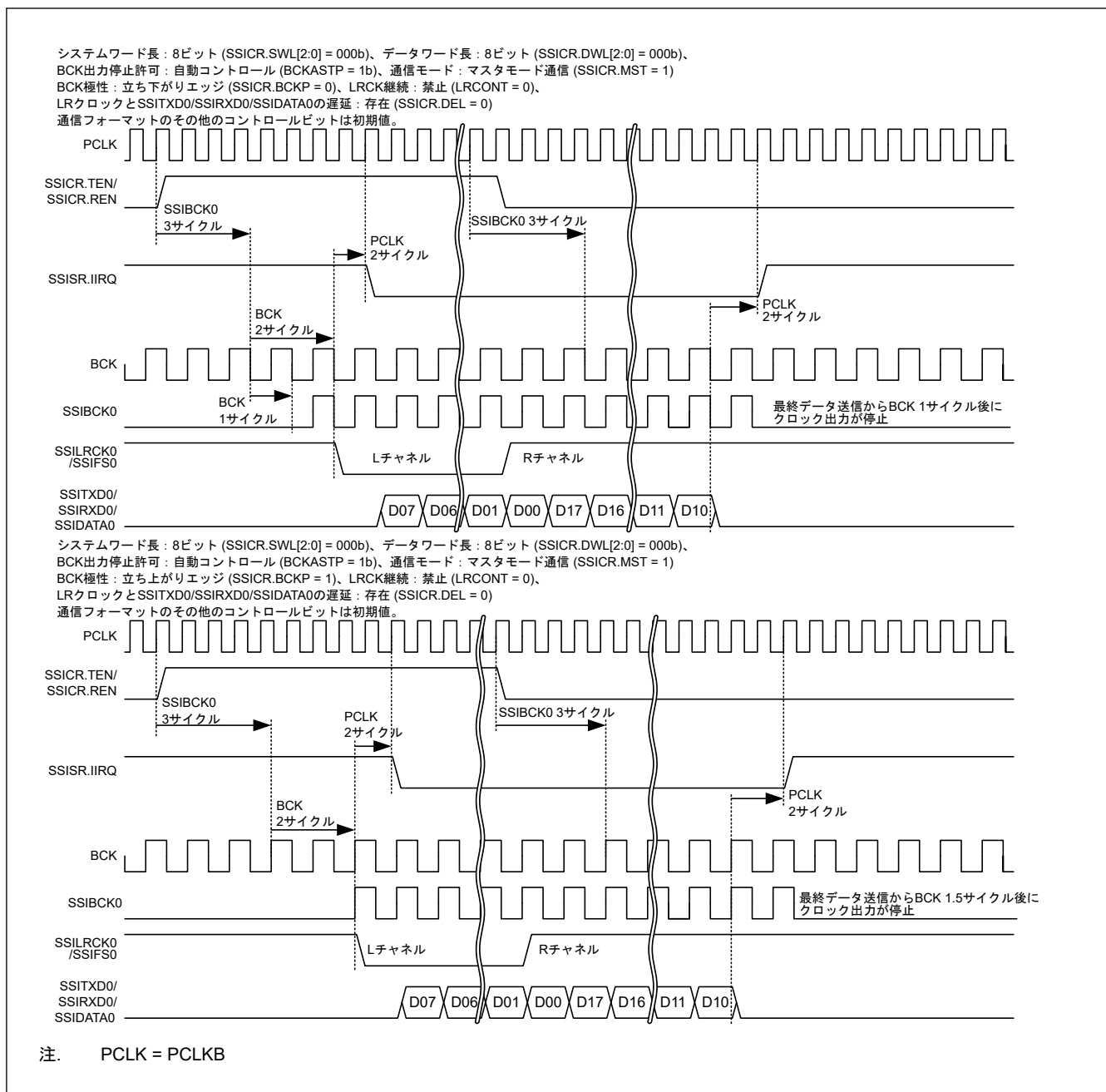
図 34.35 BCKASTP ビットの動作例 (BCKASTP = 1 での通信動作の場合)
