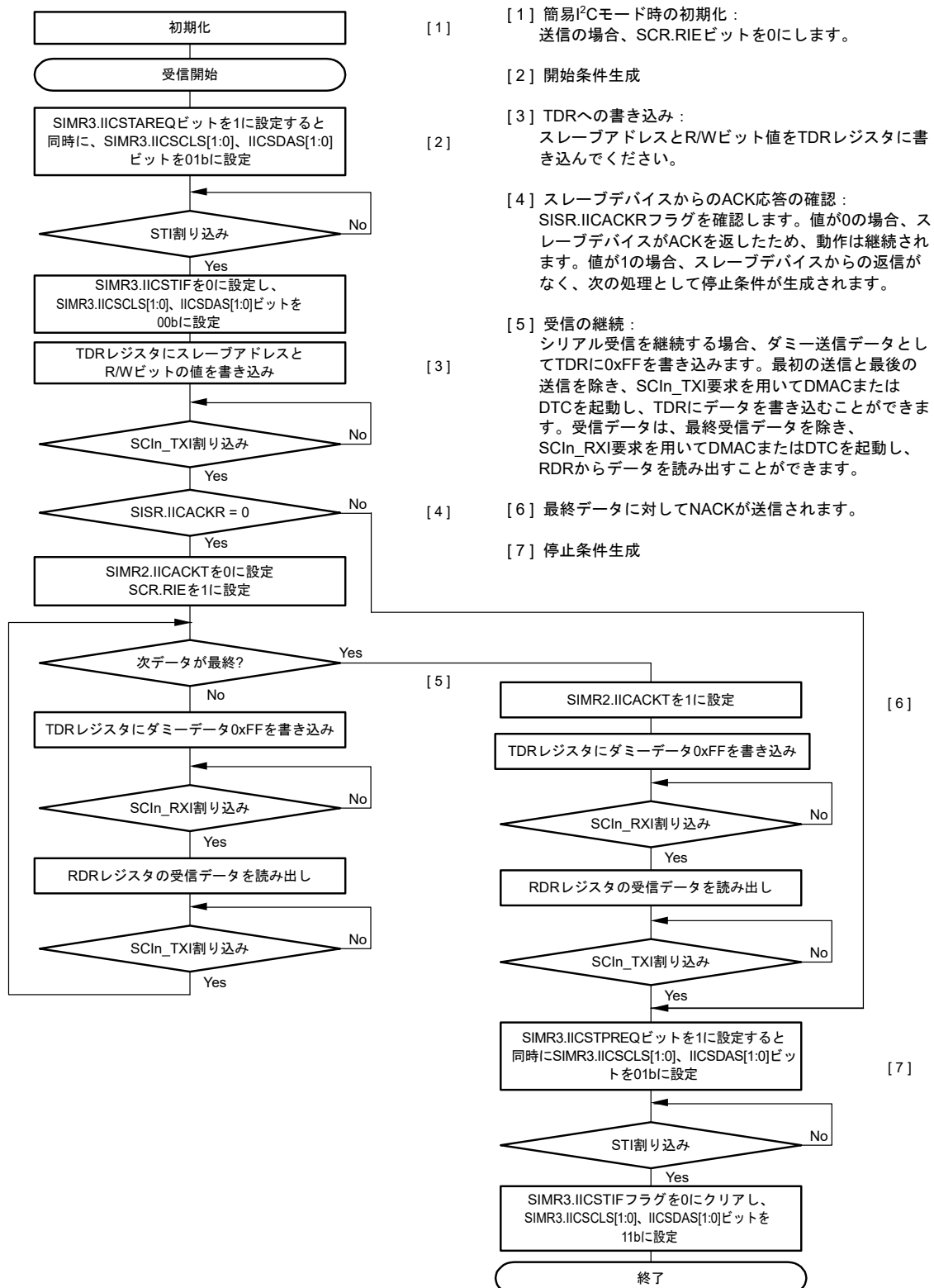
図 29.97 簡易 IIC モードにおけるマスタ受信のフローチャート例（送信割り込み、受信割り込み使用時）
