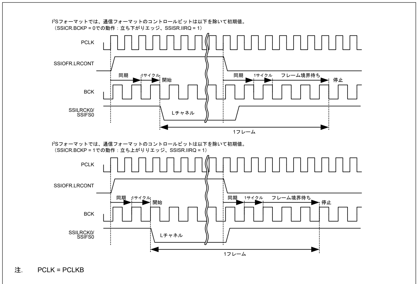
図 34.44 SSIOFR.LRCONT による LR クロック/フレーム同期継続禁止の例
