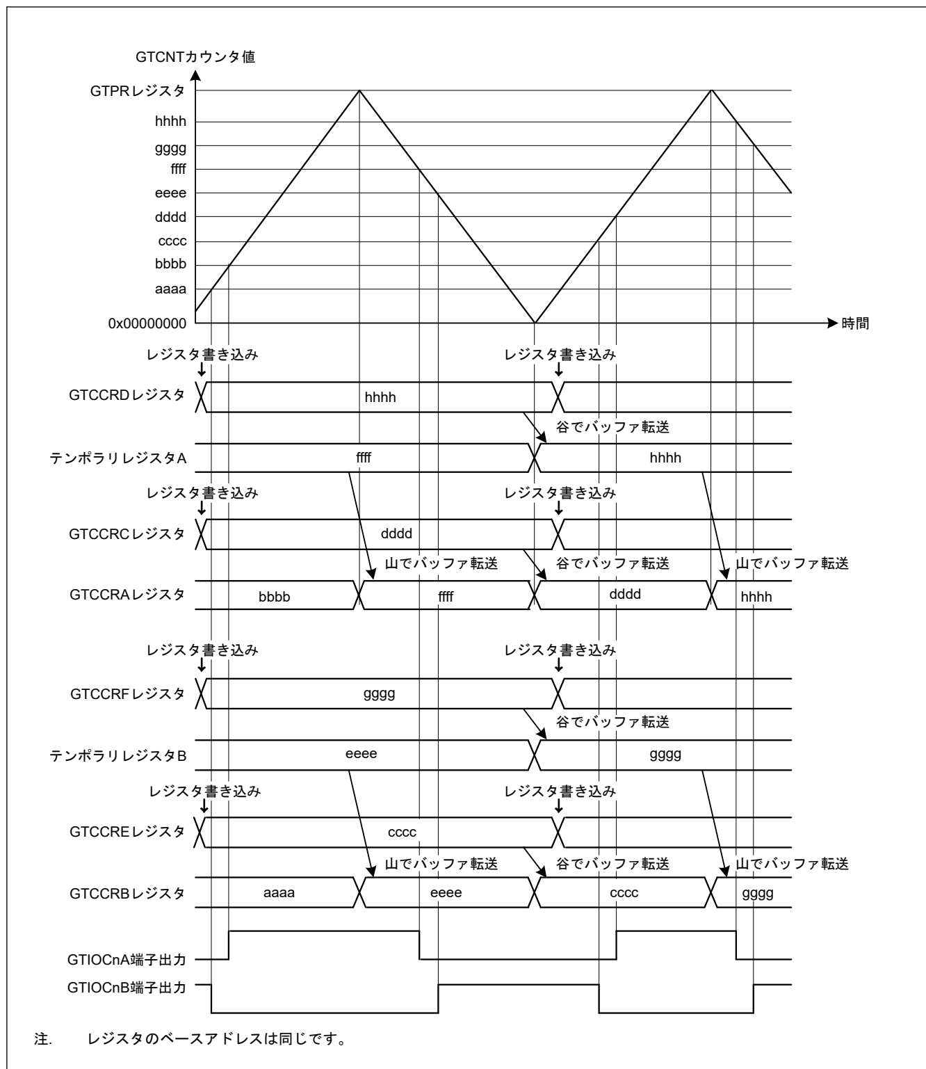
図 21.23 三角波 PWM モード 3 の動作例 (カウントスタート時に GTIOCN A 端子= Low 出力、および GTIOCN B 端子= High 出力、GTCCRA/GTCCRB レジスタのコンペアマッチ時にトグル出力、周期の終わりで出力保持の場合)
