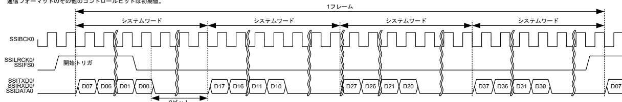
図 34.42 TDM フォーマット（パディングあり、システムワード長 > データワード長）
