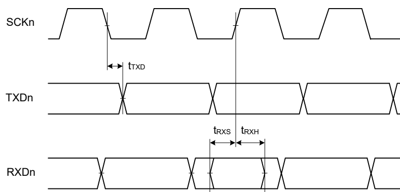
図 47.26 クロック同期式モードにおける SCI 入出力タイミング
