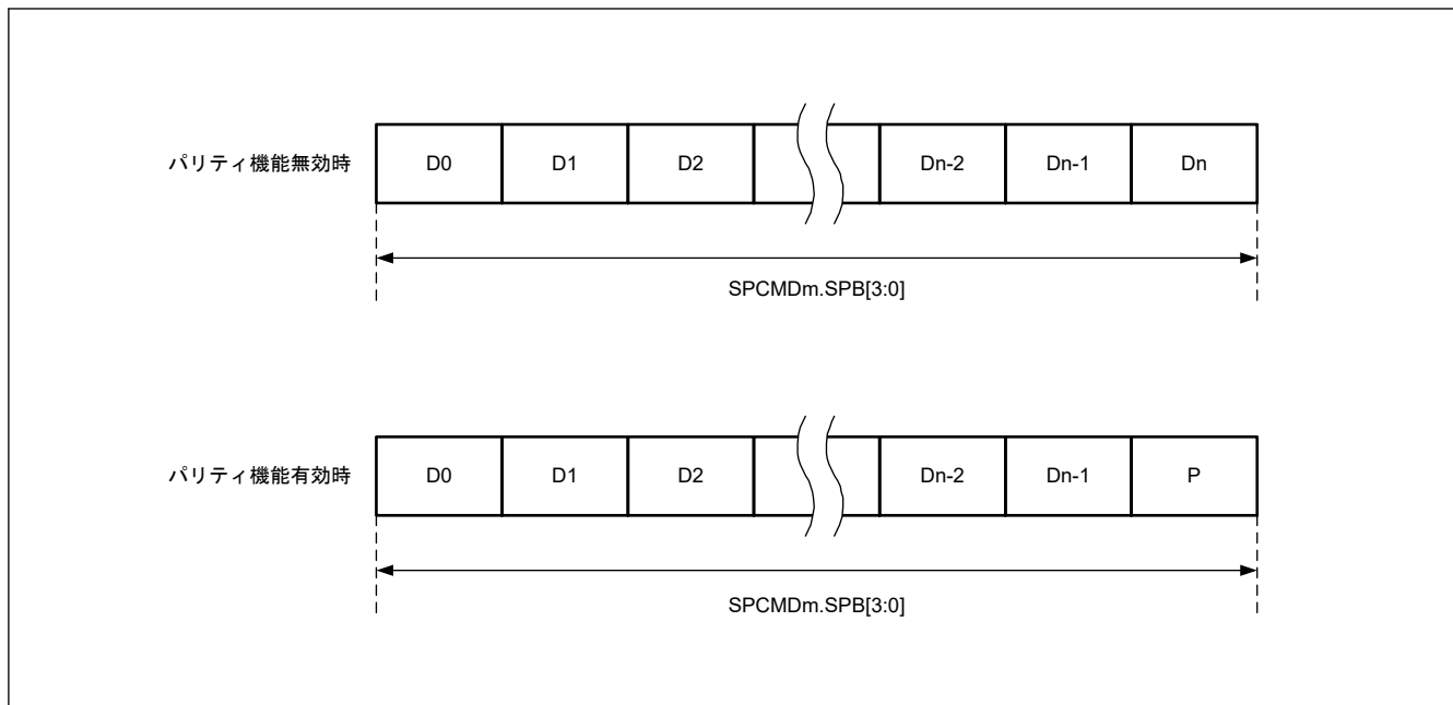
図 32.13 パリティ機能無効時と有効時のデータフォーマット
