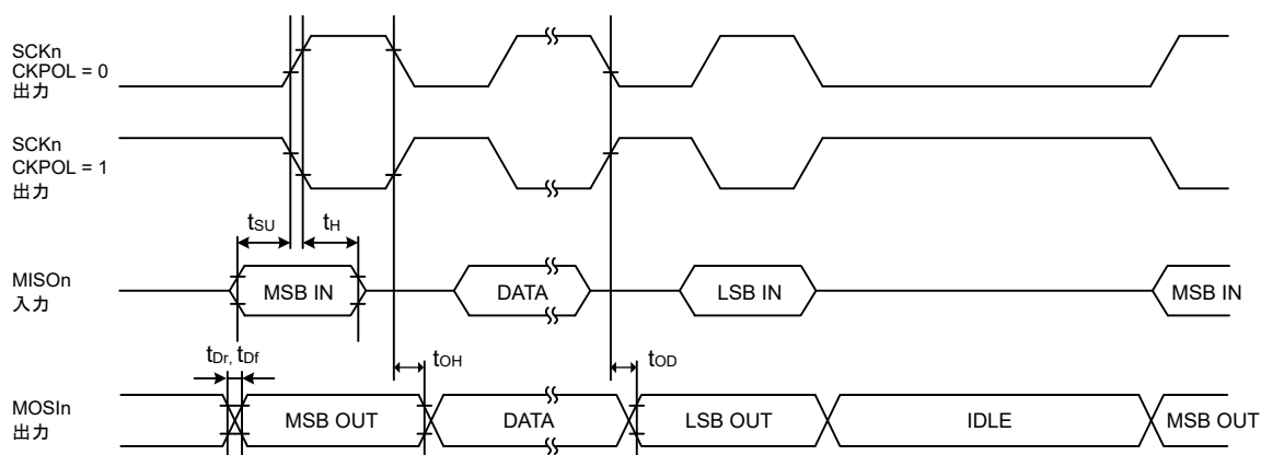
図 47.28 CKPH = 1 の場合におけるマスタの SCI 簡易 SPI モードタイミング
