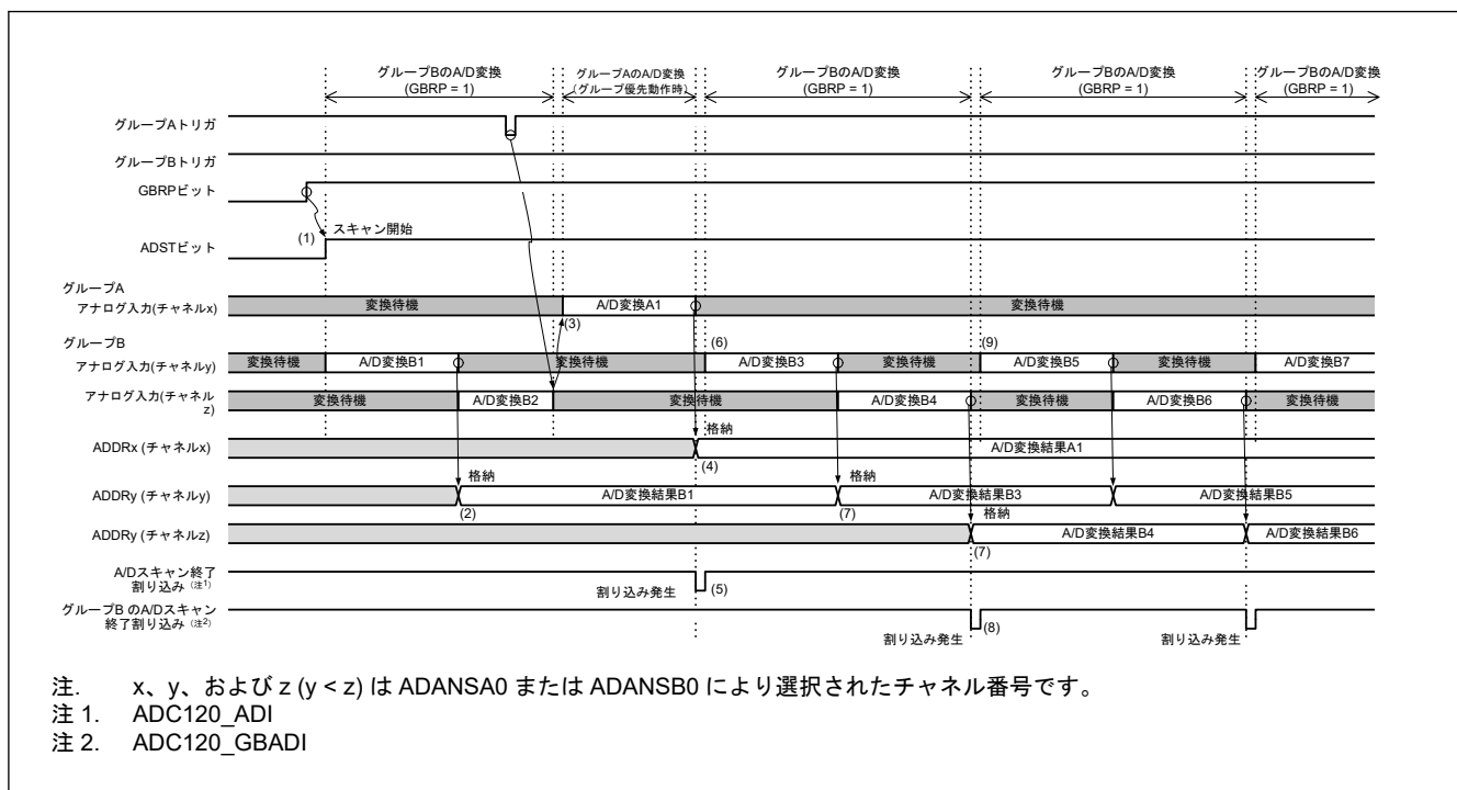
図 39.22 グループ優先動作の例 1-5 : グループ B のシングルスキャン連続動作 (ADGSPCR.GBRP = 1、ADGSPCR.LGRRS = 0 の場合)
