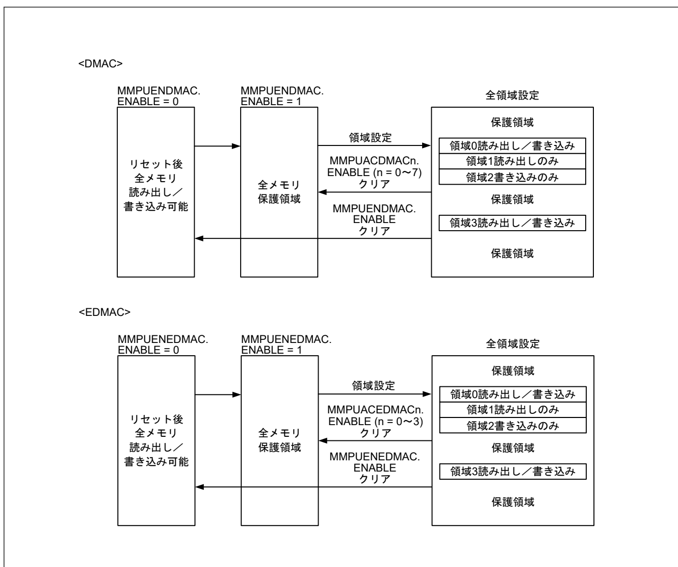
図 15.1 バスマスタ MPU の使用例
