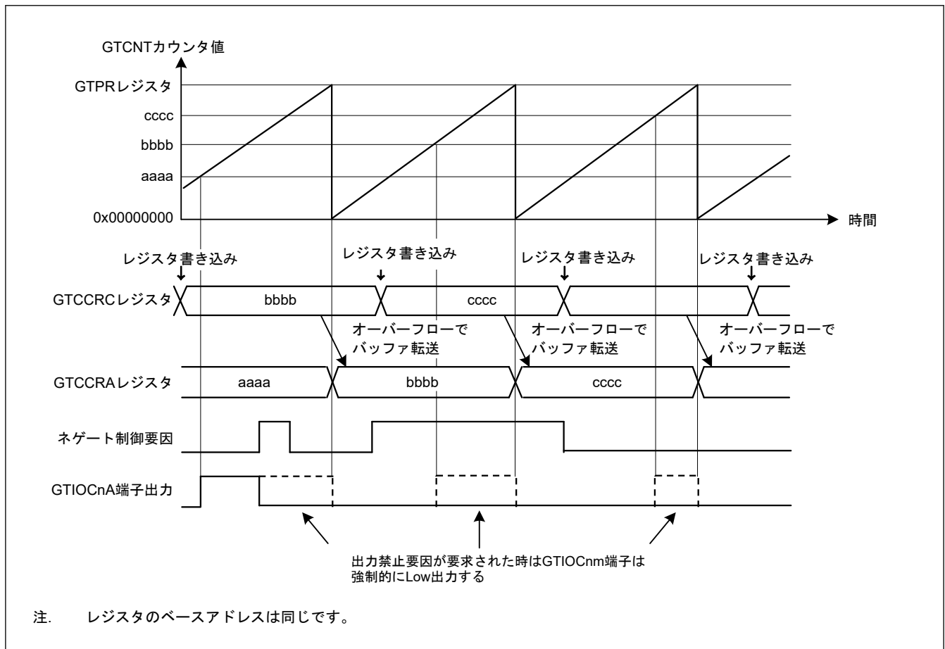
図 21.62 GTIOCnm 端子出力禁止制御動作例 (のこぎり波でアップカウント、バッファ動作、アクティブレベル 1、GTCCRA レジスタのコンペアマッチで High 出力、周期の終わりで Low 出力、および出力禁止で Low 出力の場合) (n = 1、2、4~7, m = A, B)
