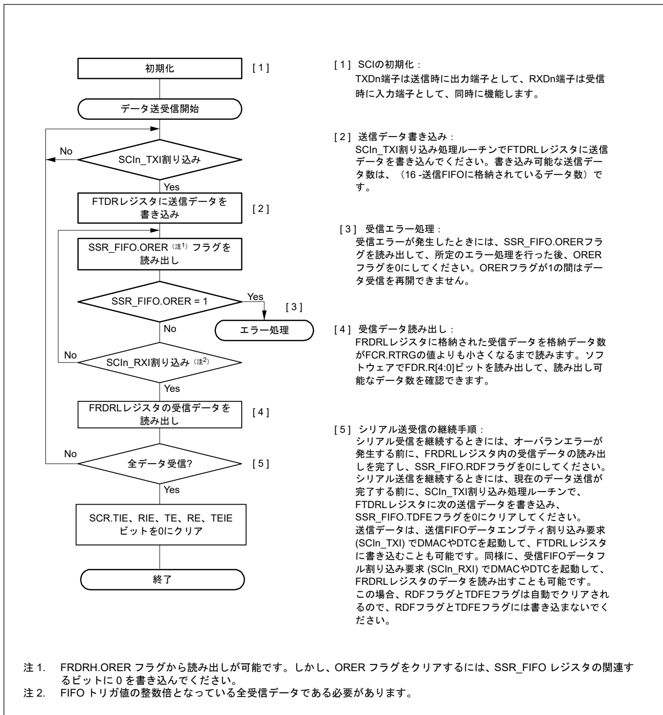
図 29.76 クロック同期式モードにおけるシリアル同時送受信動作のフローチャート例 (FIFO 選択時)
