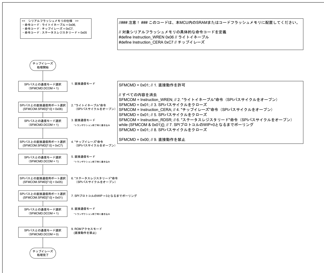
図 33.40 チップイレーズのフローチャート
