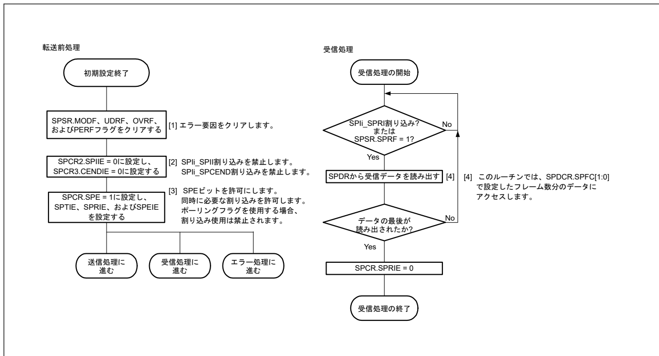
図 32.54 スレーブモードでの受信フロー
