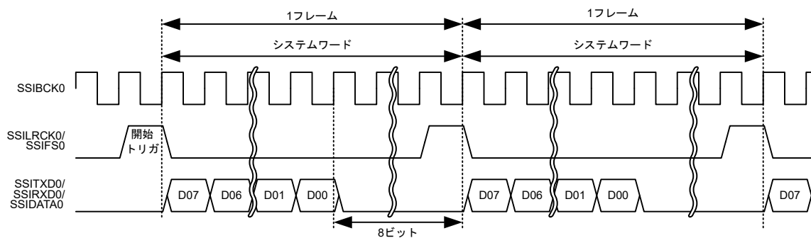
図 34.39 モノラルフォーマットにおけるショートフレーム（パディングあり、システムワード長 > データワード長）
