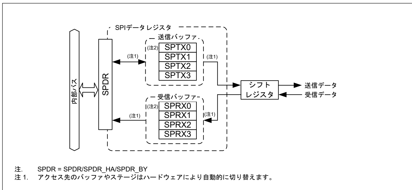
図 32.2 SPDR/SPDR_HA/SPDR_BY レジスタの構成図
