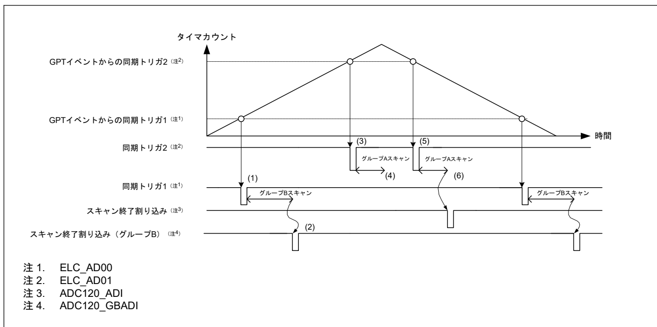
図 39.16 グループスキャンモードでダブルトリガモードを使用する場合の基本動作例 (ELC からの同期トリガ使用時)
