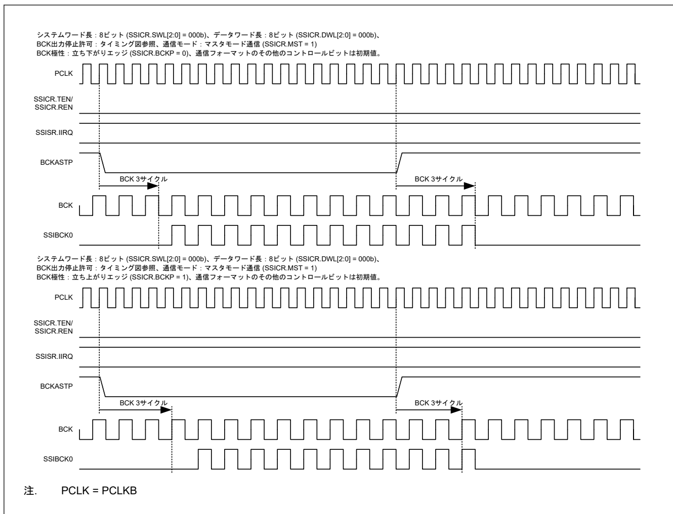
図 34.34 BCKASTP ビットの動作例（アイドル状態の場合）
