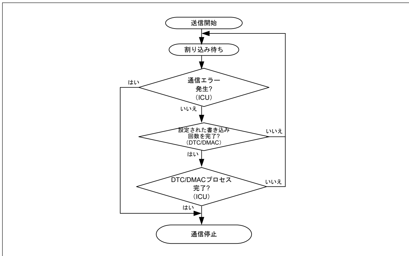
図 34.54 送信手順
