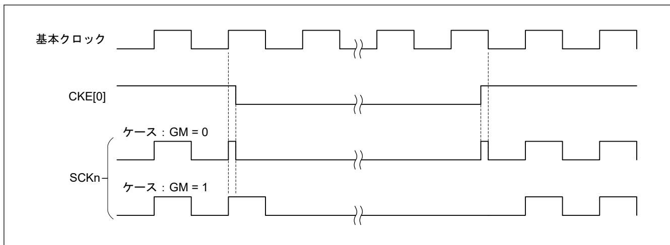
図 29.87 クロック出力タイミング
