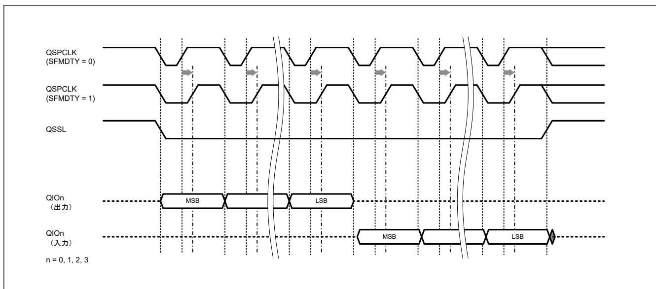
図 33.10 PCLKA を 3 通倍した場合の SFMDTY ビットを使用した QSPCLK 信号デューティ比補正例
