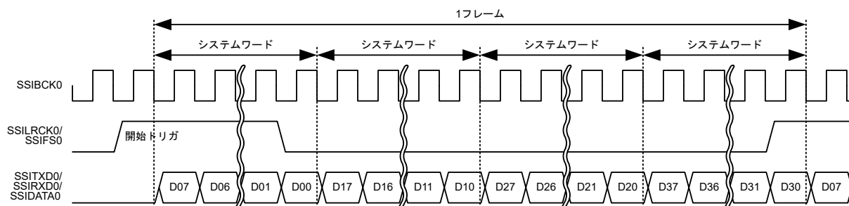
図 34.41 TDM フォーマット（パディングなし、システムワード長 = データワード長）
