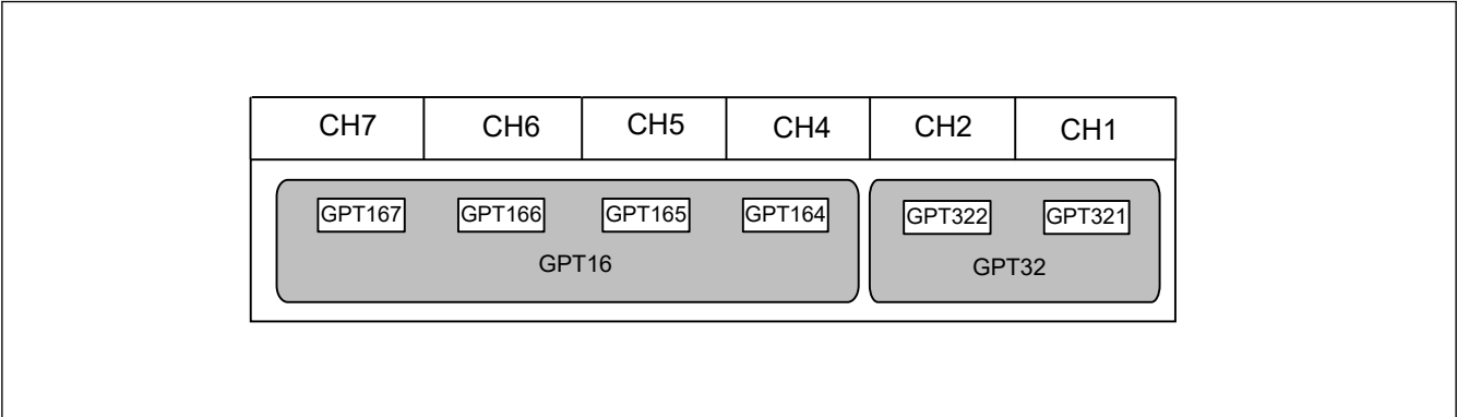
図 21.2 GPT チャネルとモジュール名の関係
