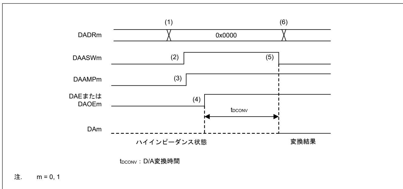
図 40.5 出力アンプを使用した DAC12 の初期化フロー例
