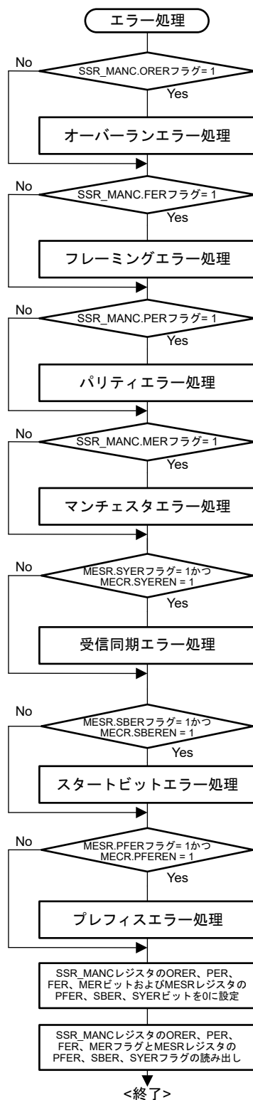
図 29.62 マンチェスタモードにおけるシリアル受信フローチャート例（エラー処理）
