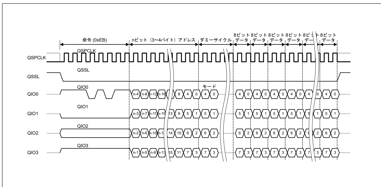
図 33.27 ファストリード Quad I/O バスサイクル
