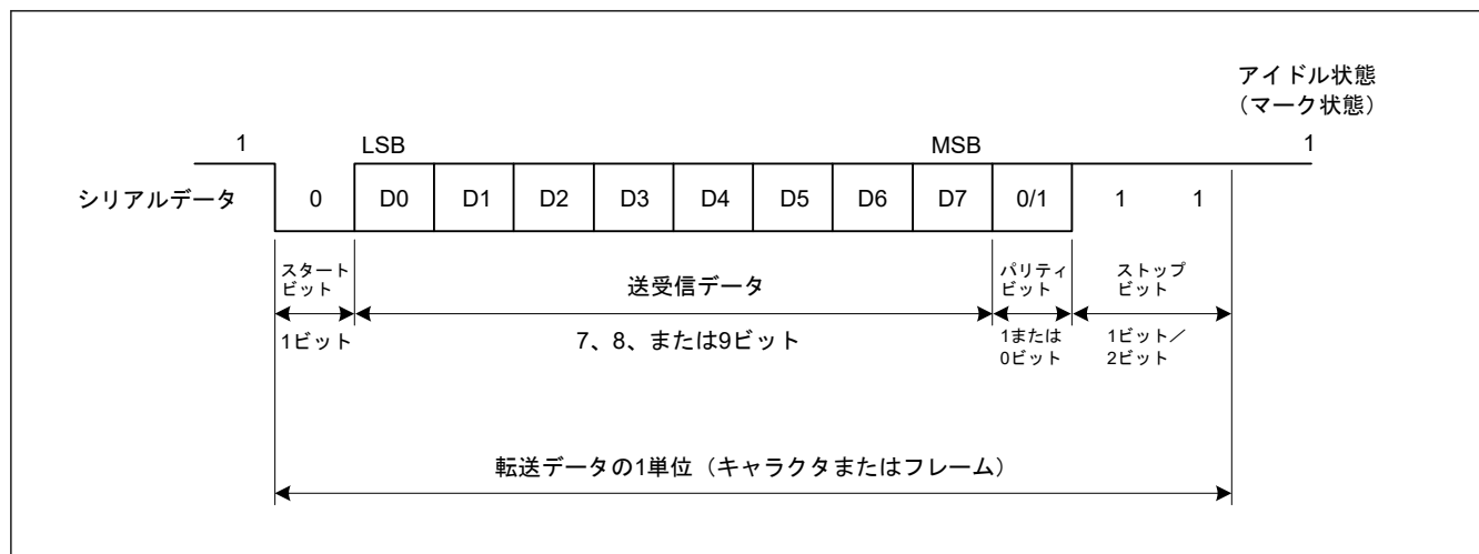
図 29.6 調歩同期式シリアル通信のデータフォーマット (8 ビットデータ／パリティあり／2 ストップビットの場合)
