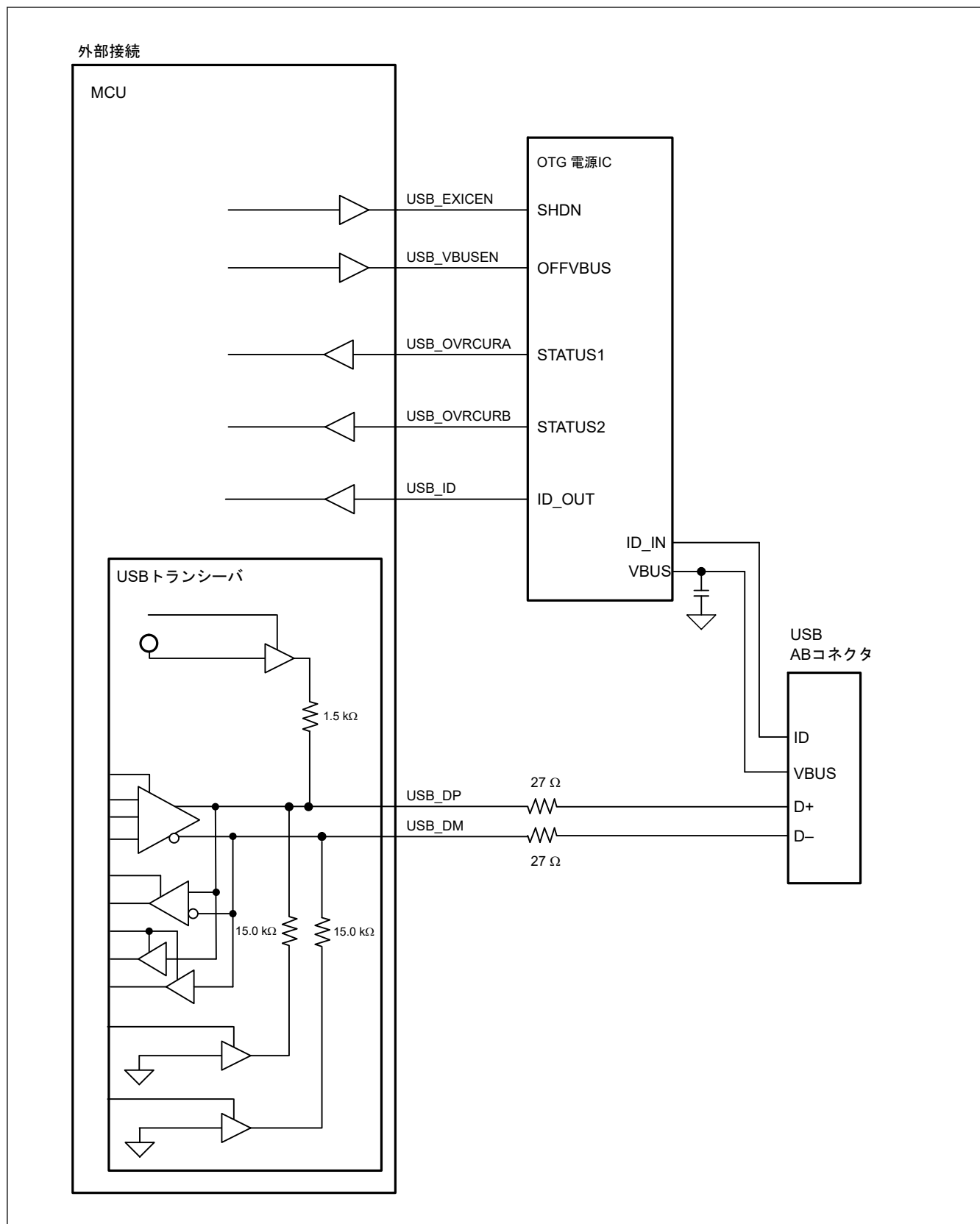
図 28.2 セルフパワードシステムでの OTG 接続例
