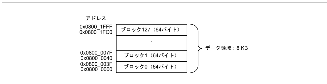
図 44.4 データフラッシュメモリのマップ
