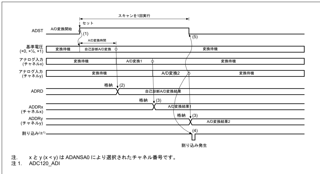
図 39.8 シングルスキャンモードの基本動作例（アナログ入力（チャンネル x と y）選択+自己診断）
