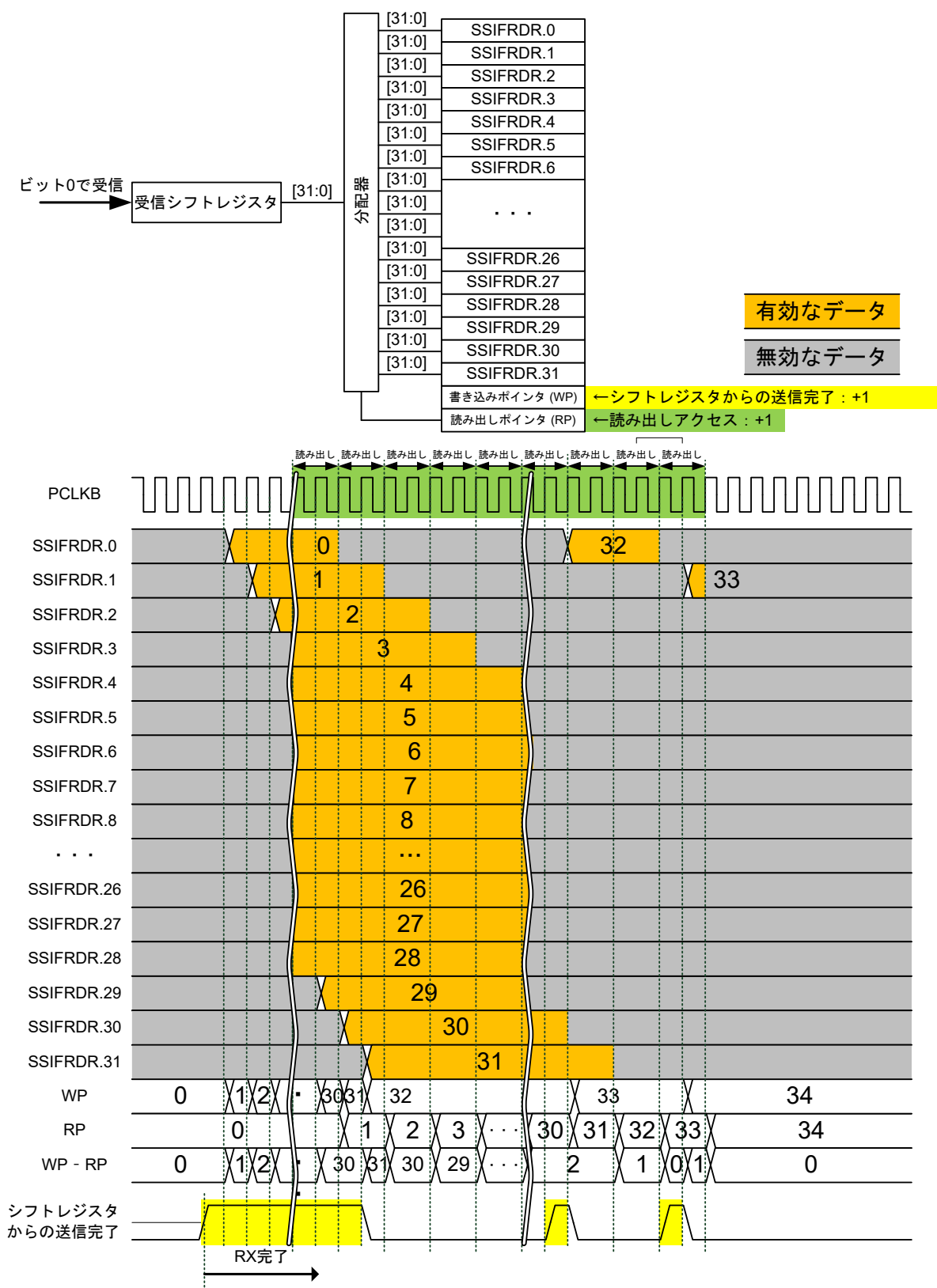
図 34.32 受信 FIFO データレジスタと受信シフトレジスタの構成、および FIFO の動作例
