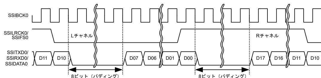
図 34.10 パディングビットを伴うシリアルデータのアライメント設定
