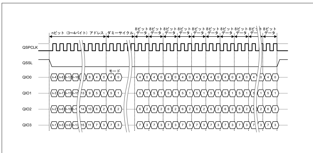
図 33.28 XIP モード時のファストリード Quad I/O バスサイクル
