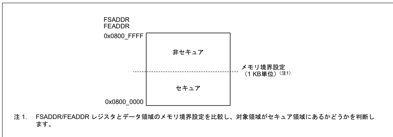
図 44.37 データ領域のセキュア／非セキュア領域
