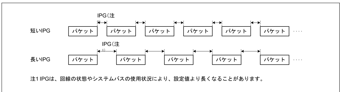
図 26.12 IPG の変化による伝送効率の違い
