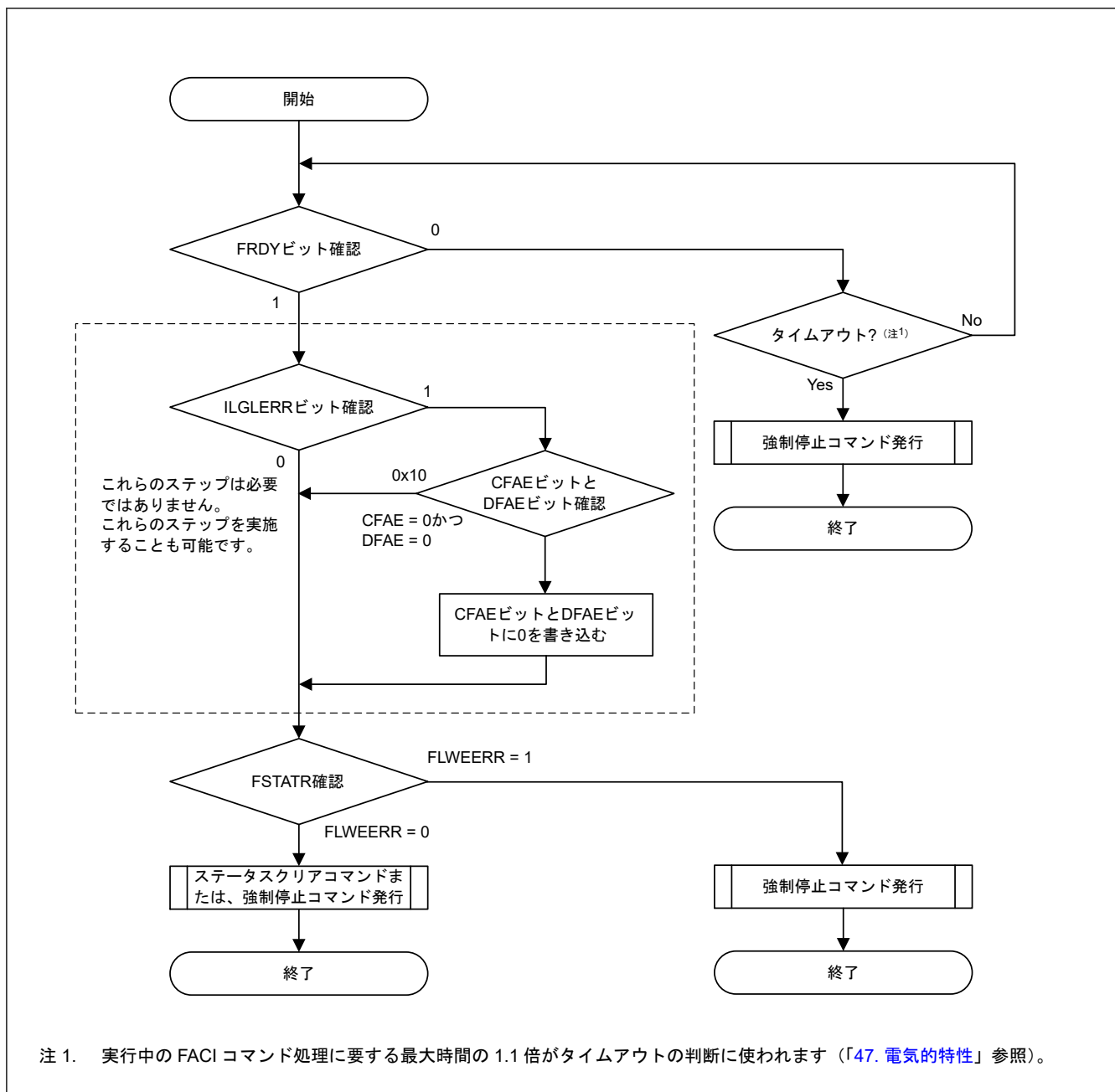
図 44.13 コマンドロック状態からの復帰フロー
