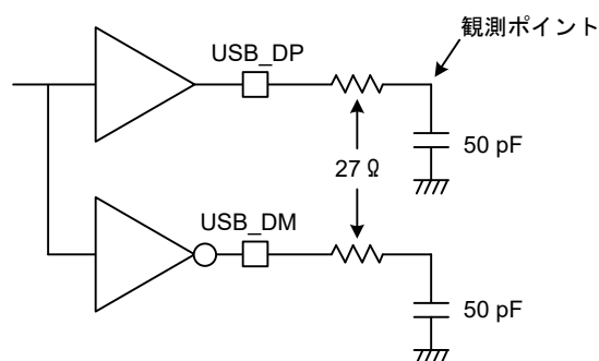
図 47.57 フルスピードモードにおける測定回路
