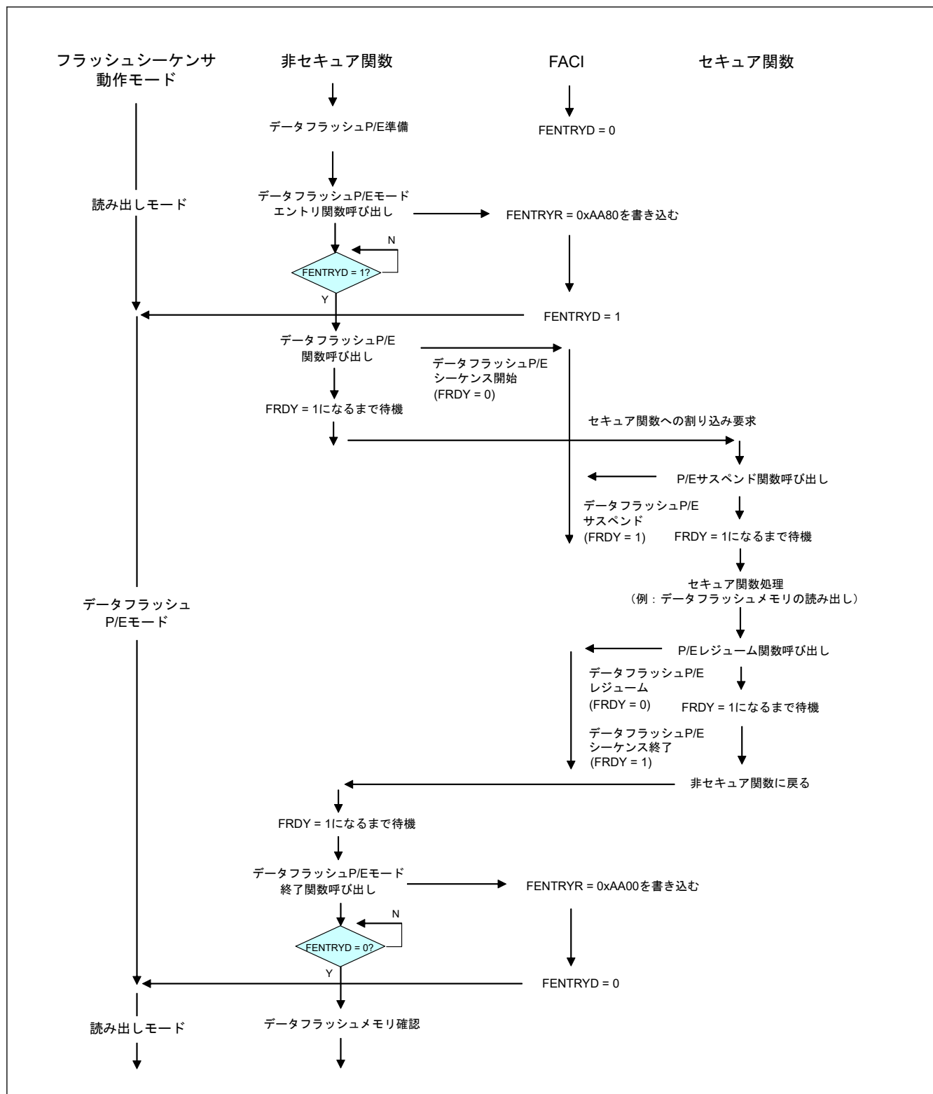
図 44.40 セキュア関数のデータフラッシュ P/E サスペンド例 (P/E 終了を検出するには FRDY ビットを確認)
