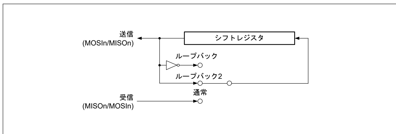
図 32.61 ループバックモード時のシフトレジスタ入出力経路の構成（マスタモード）
