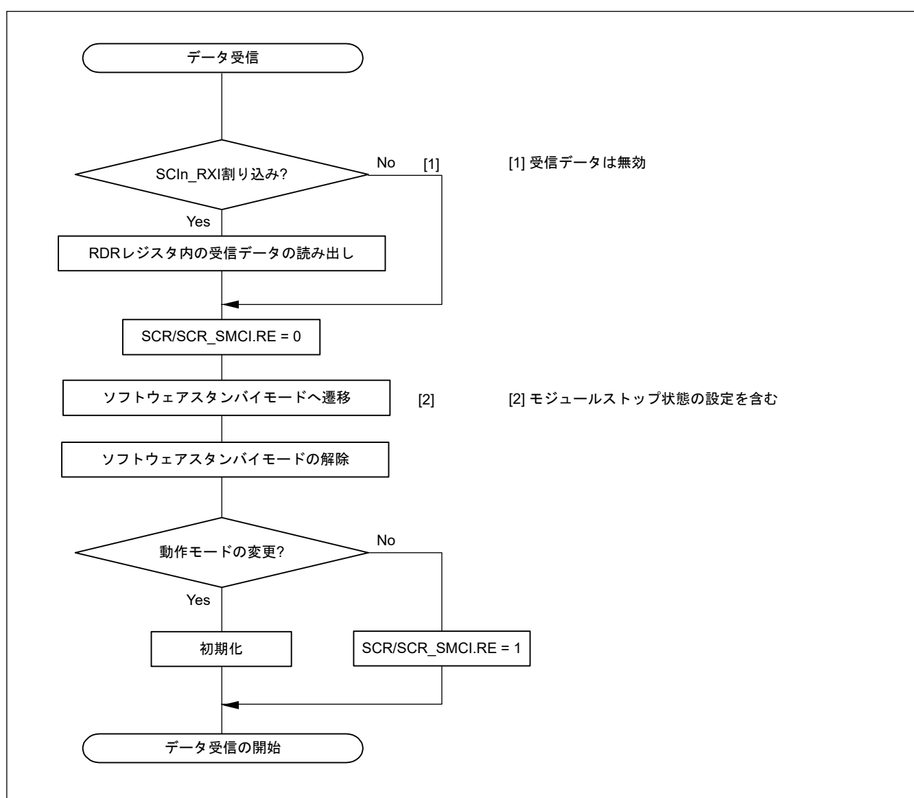
図 29.121 受信中にソフトウェアスタンバイモードへ遷移する場合のフローチャート例
