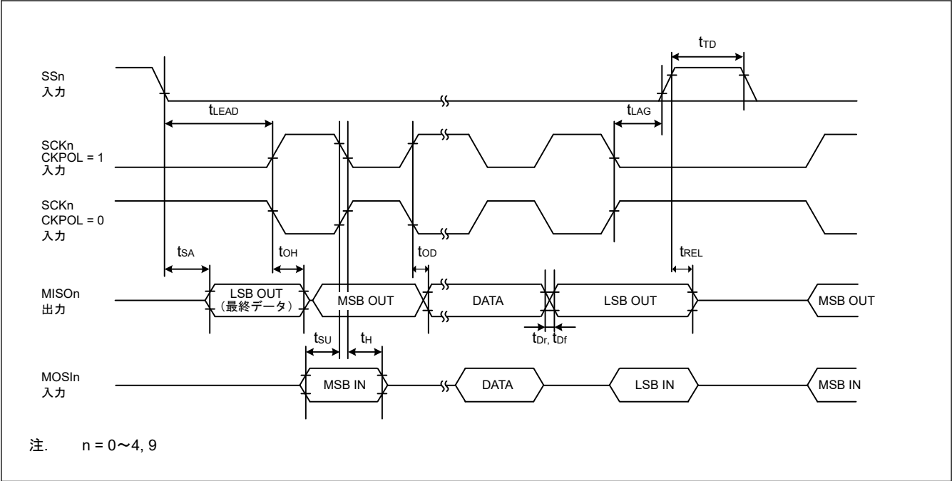
図 47.31 CKPH = 0 の場合におけるスレーブの SCI 簡易 SPI モードタイミング
