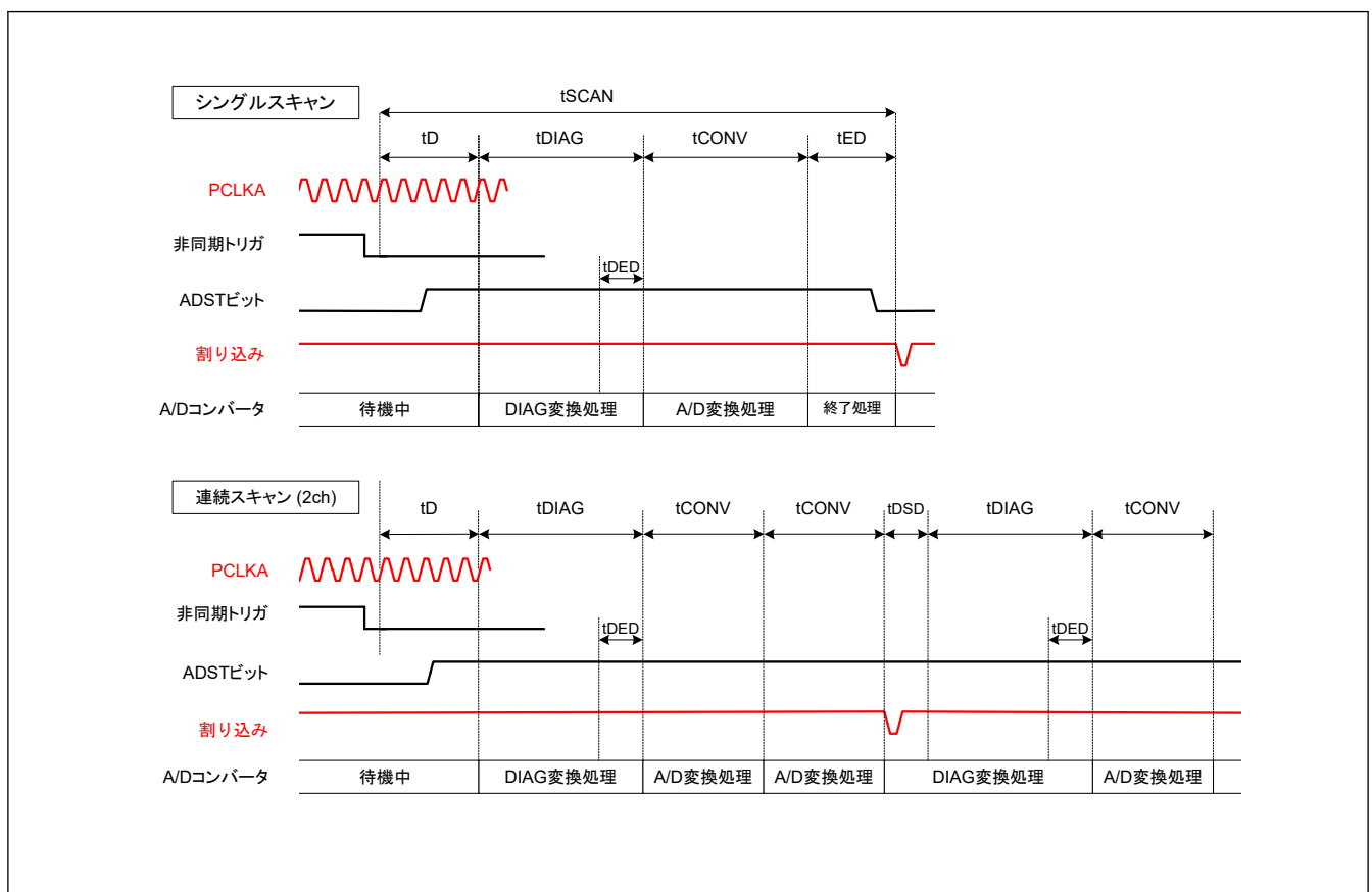
図 39.27 スキャン変換のタイミング (非同期トリガ入力 (ADTRG0) 起動の場合)
