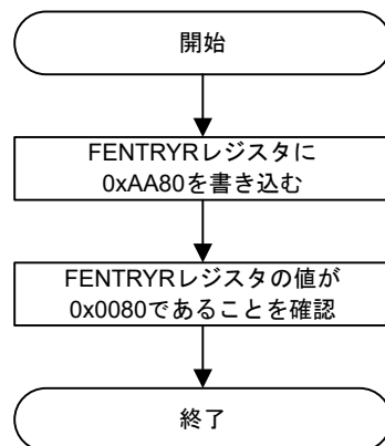
図 44.11 データフラッシュ P/E モードへの遷移手順
