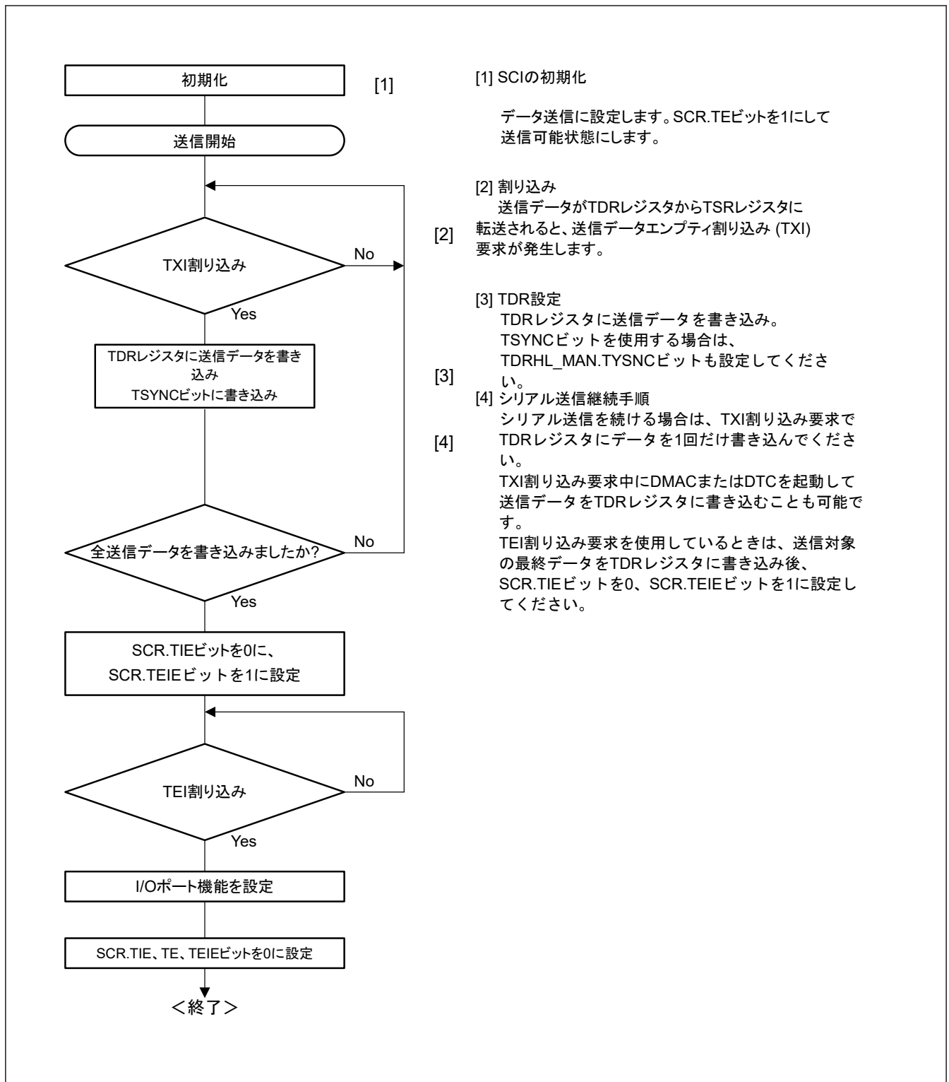
図 29.55 マンチェスタモードにおけるシリアル送信のフローチャート例
