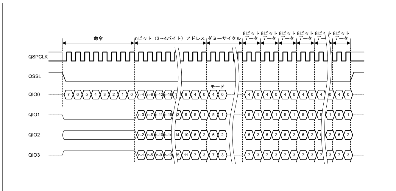
図 33.5 拡張 SPI プロトコル例（ファストリード Quad I/O）
