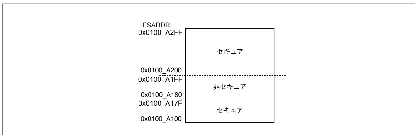
図 44.38 オプション設定メモリのセキュア／非セキュア領域
