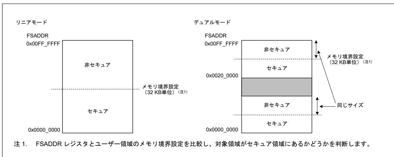
図 44.36 ユーザー領域のセキュア／非セキュア領域
