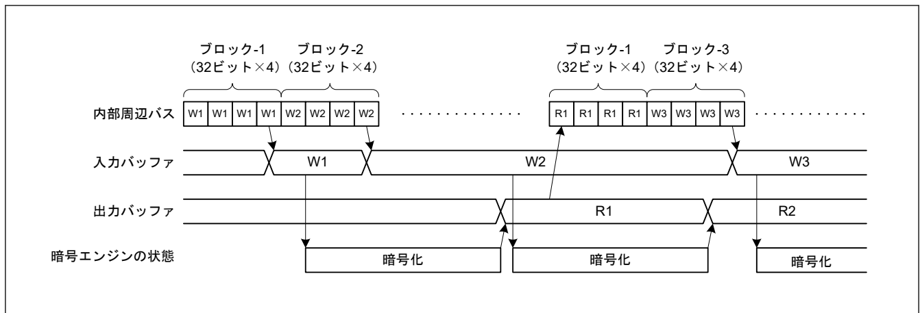
図 38.3 暗号／復号処理タイミング (AES)
