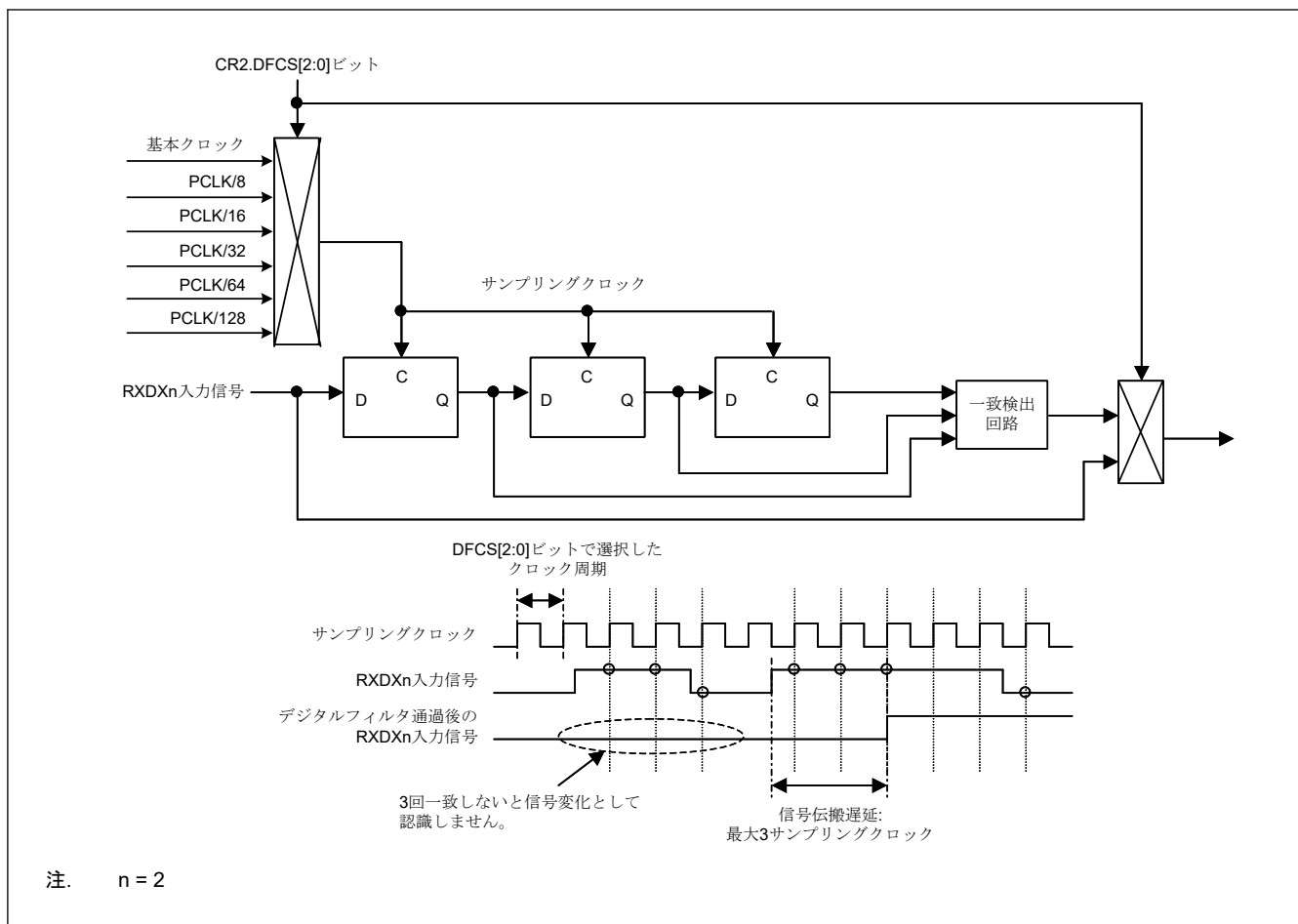
図 29.112 デジタルフィルタ機能の動作例
