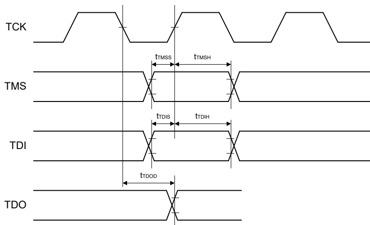
図 47.68 バウンダリスキャン入出力タイミング
