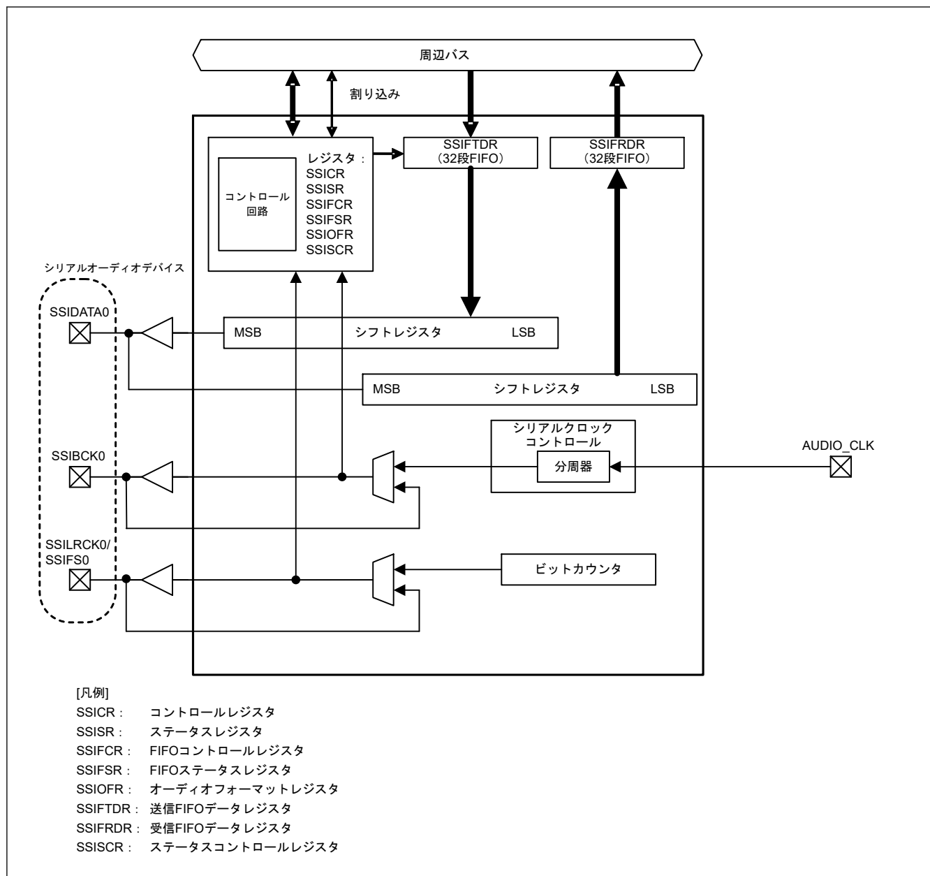
図 34.3 半二重通信の SSIE ブロック図
