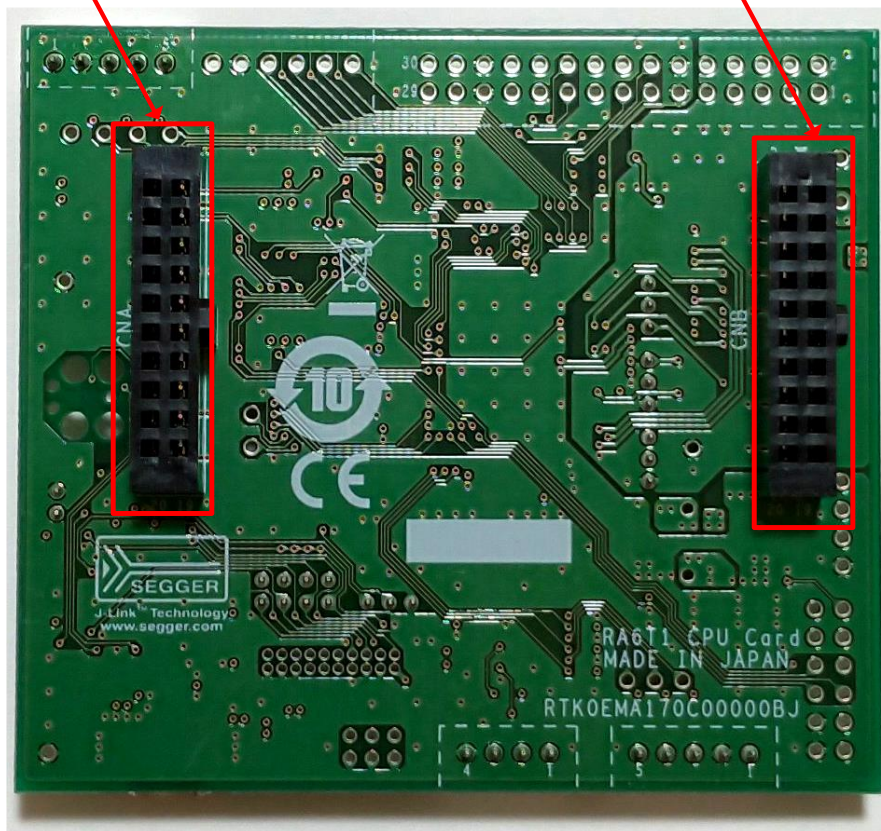
図 1-2 RA6T1 CPU Card (裏面)
