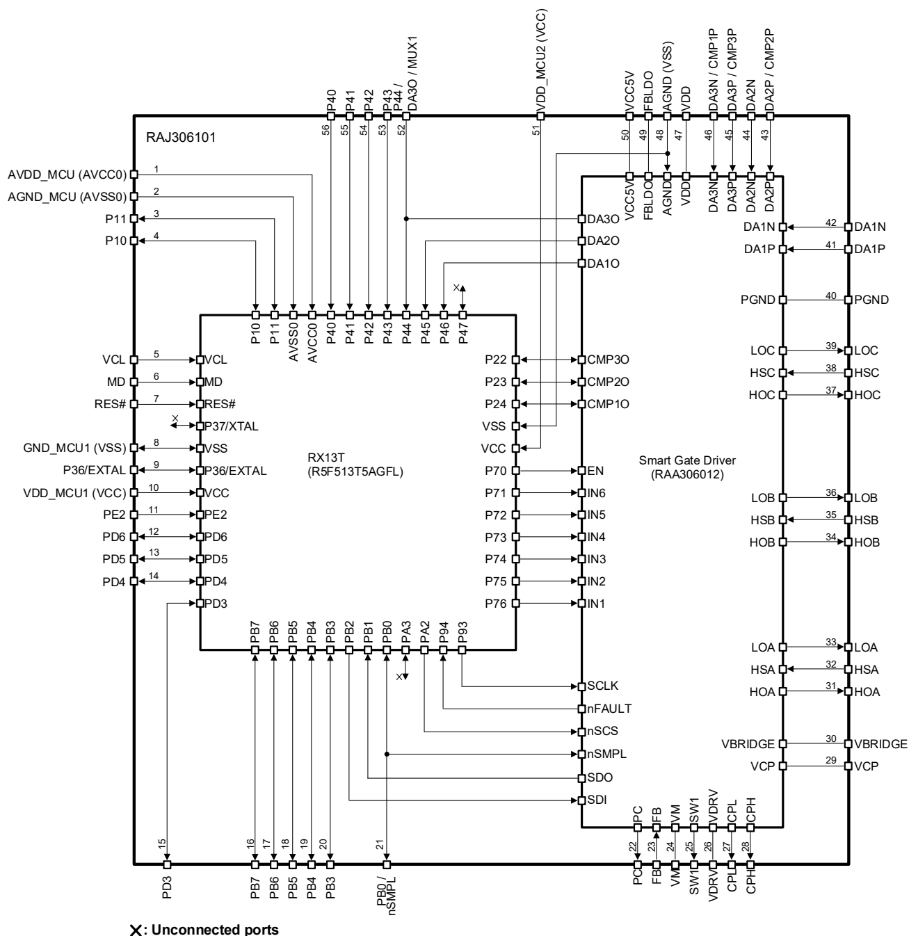
図 1-5 内部接続図
