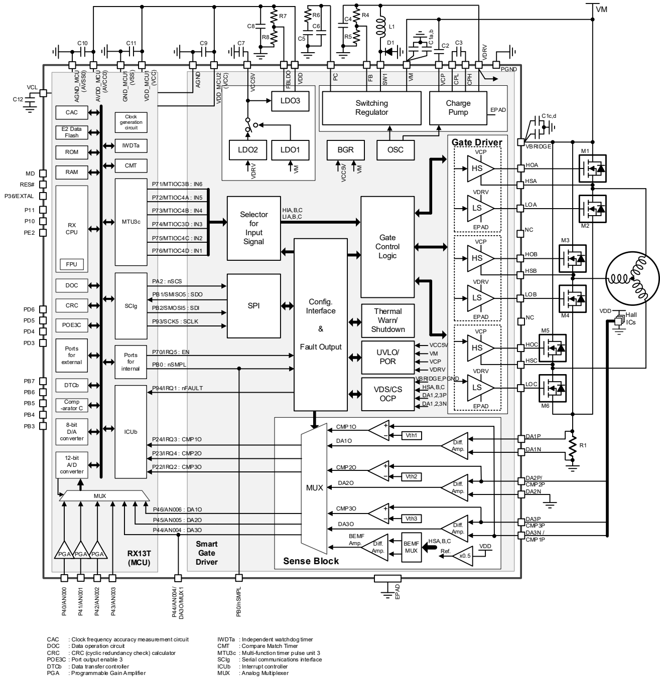
図 1-6 アプリケーション簡易ブロック図: ホールセンサモータ制御 (3 コンパレータ)
