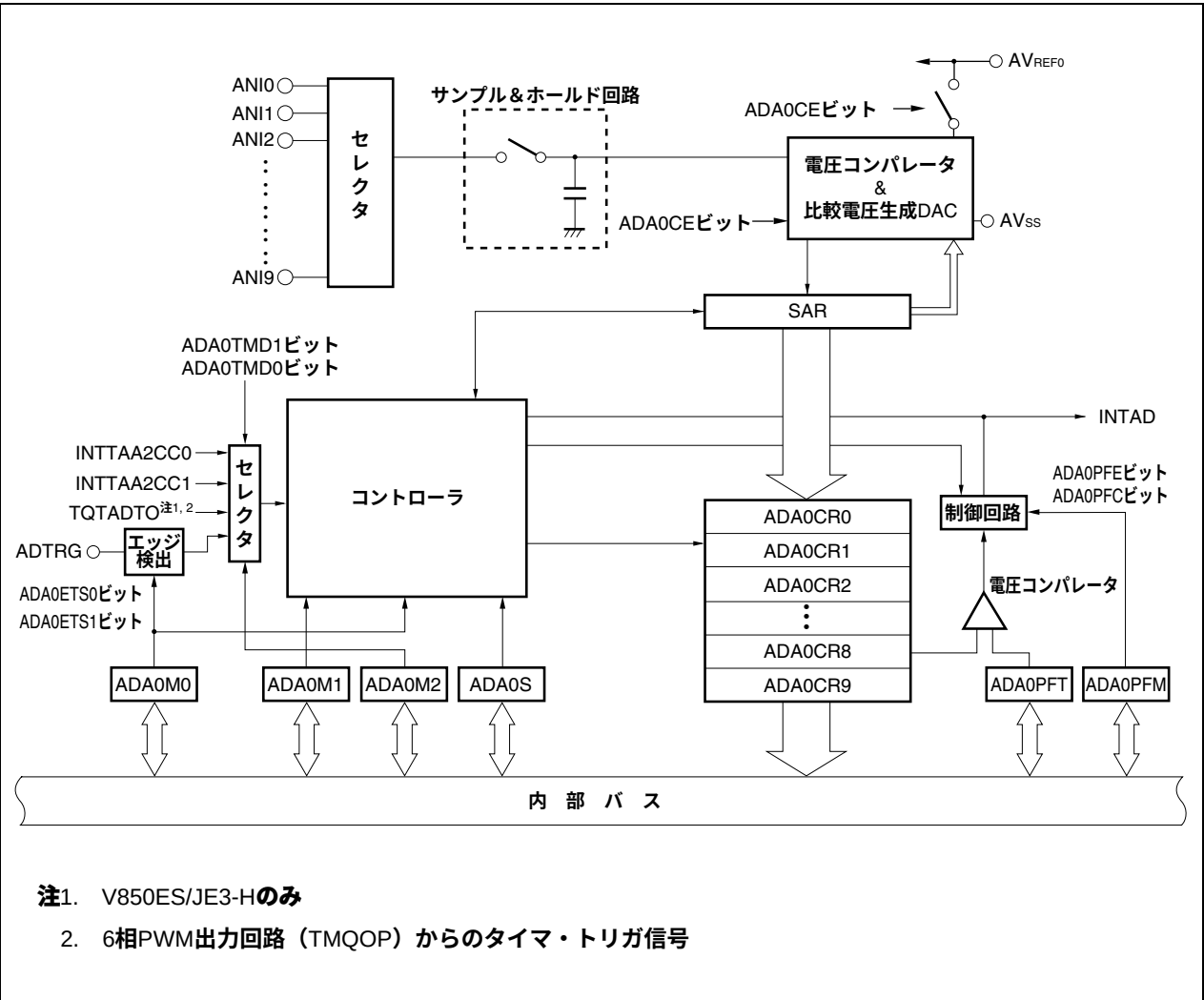
図14-1 A/Dコンバータのブロック図
