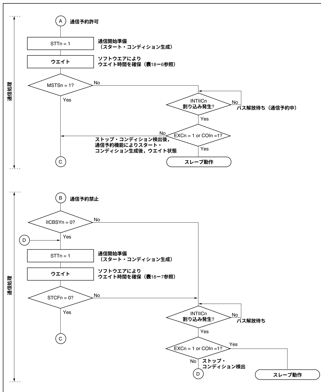
図18-19 マルチマスタ・システムでのマスタ動作 (2/3)
