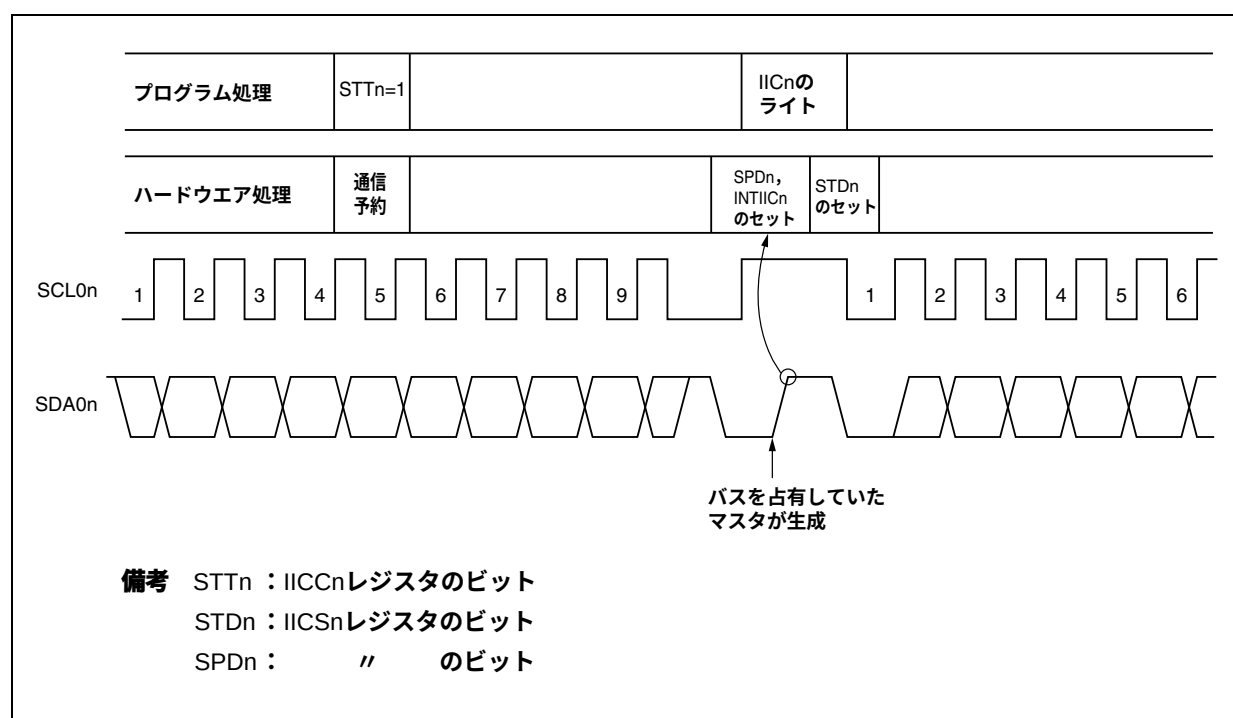
図18-15 通信予約のタイミング
