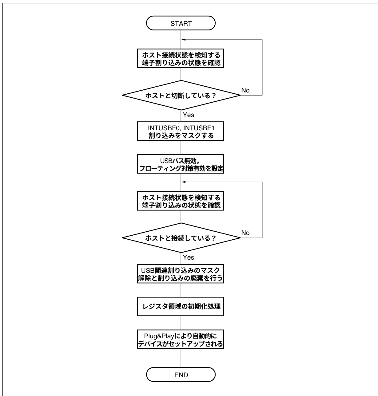
図20-12 ホスト切断／ホスト再接続時のプログラムのフロー・チャート
