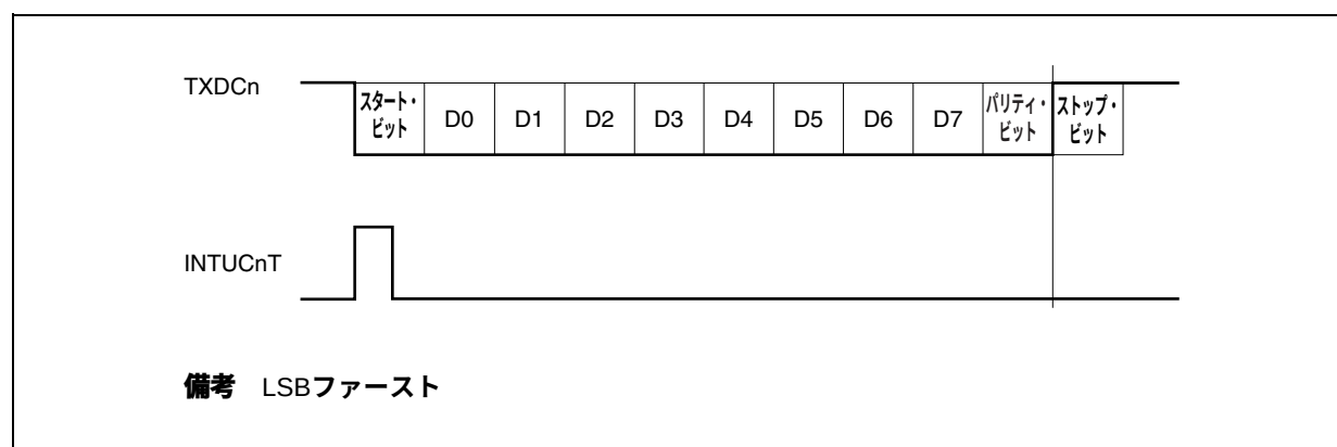
図16-11 UART送信
