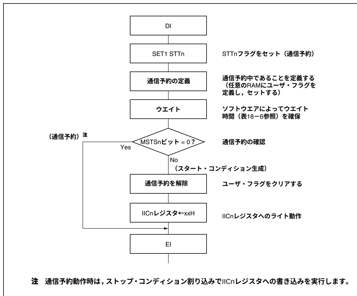
図18-17 通信予約の手順
