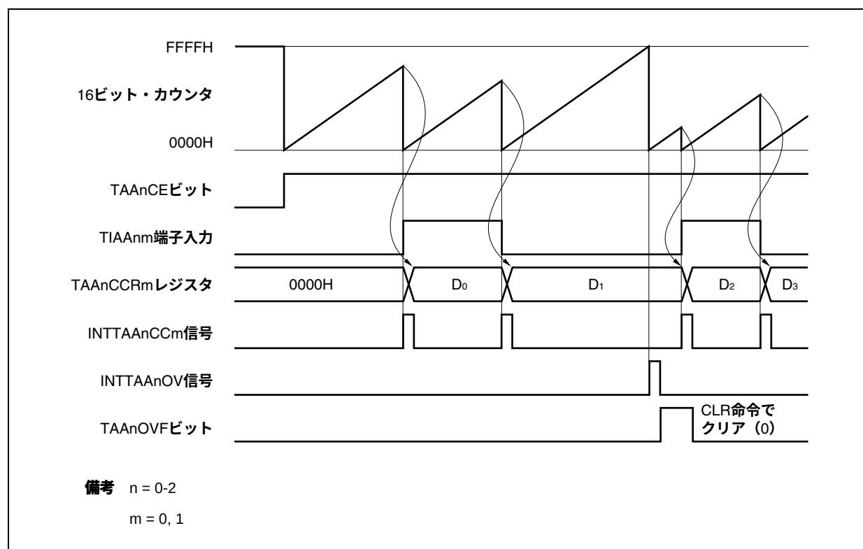
図6-40 パルス幅測定モードの基本タイミング
