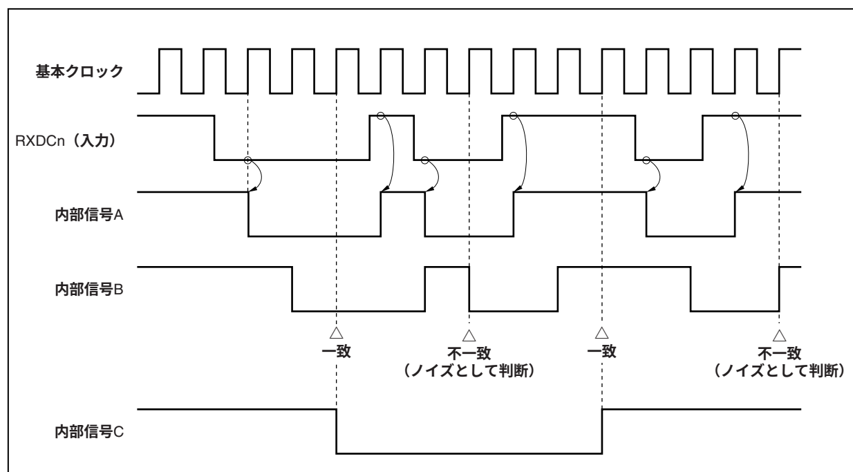
図16-17 ノイズとして判断されるRXDCn信号のタイミング
