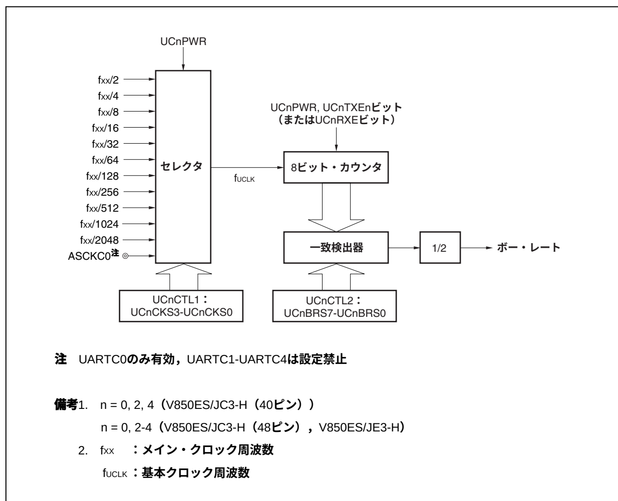
図16-18 ボー・レート・ジェネレータの構成
