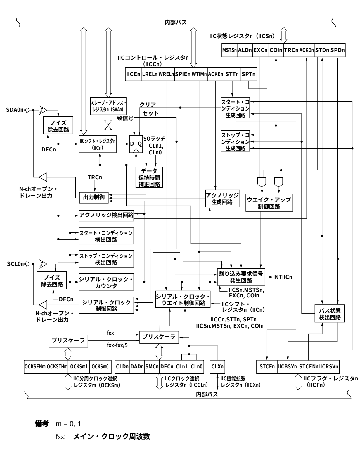
図18-4 I 2 C0nのブロック図
