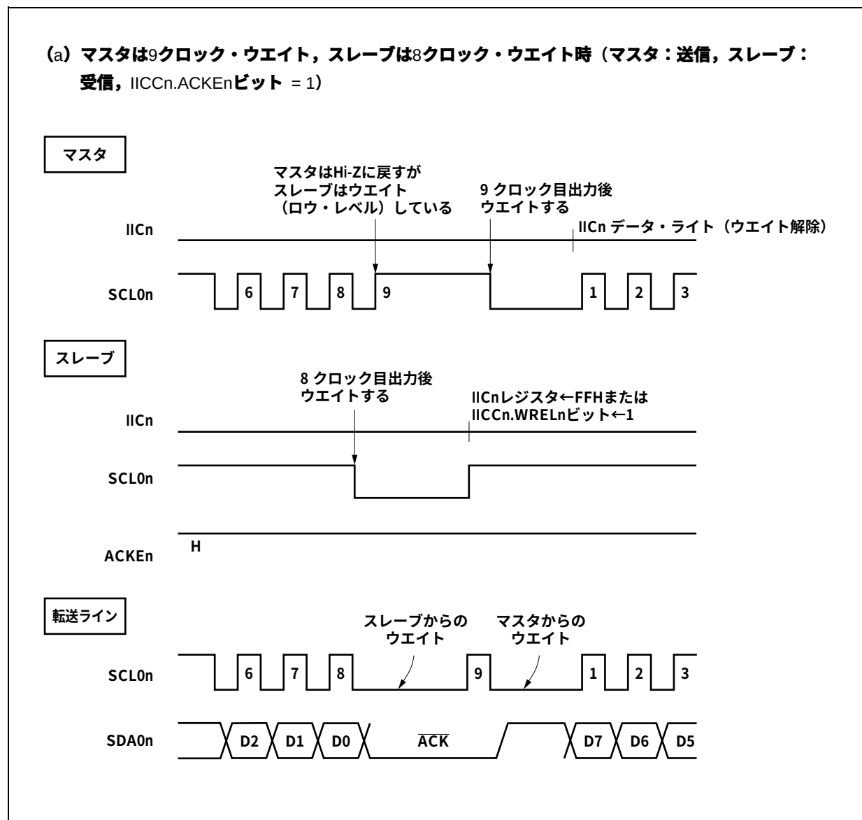
図18-13 ウェイト (1/2)
