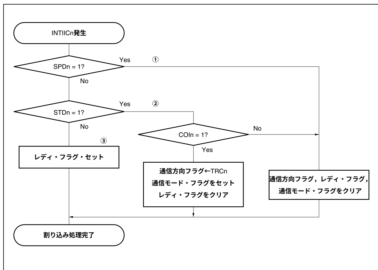
図18-22 スレーブ動作手順（2）
