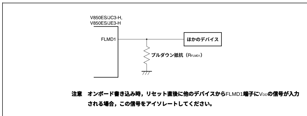
図30-13 FLMD1端子の接続例
