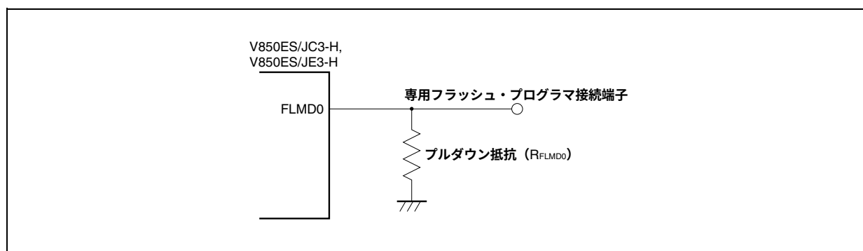
図30-12 FLMD0端子の接続例
