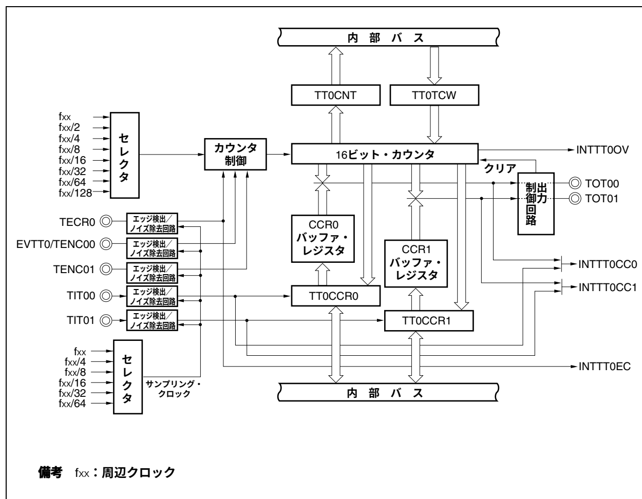
図8-1 TMT0のブロック図
