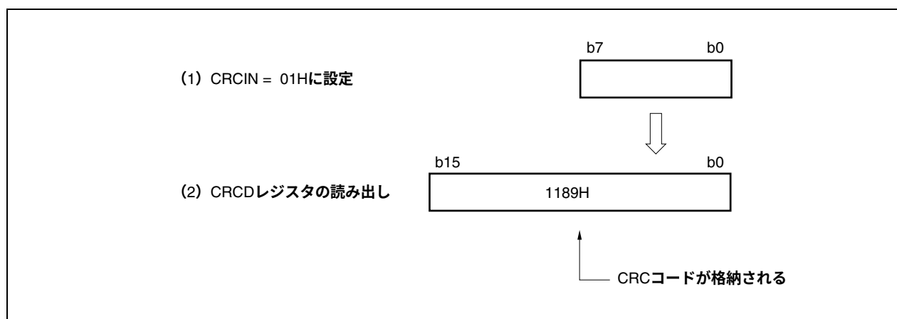
図28-2 CRC演算回路の演算例 (LSBファースト)
