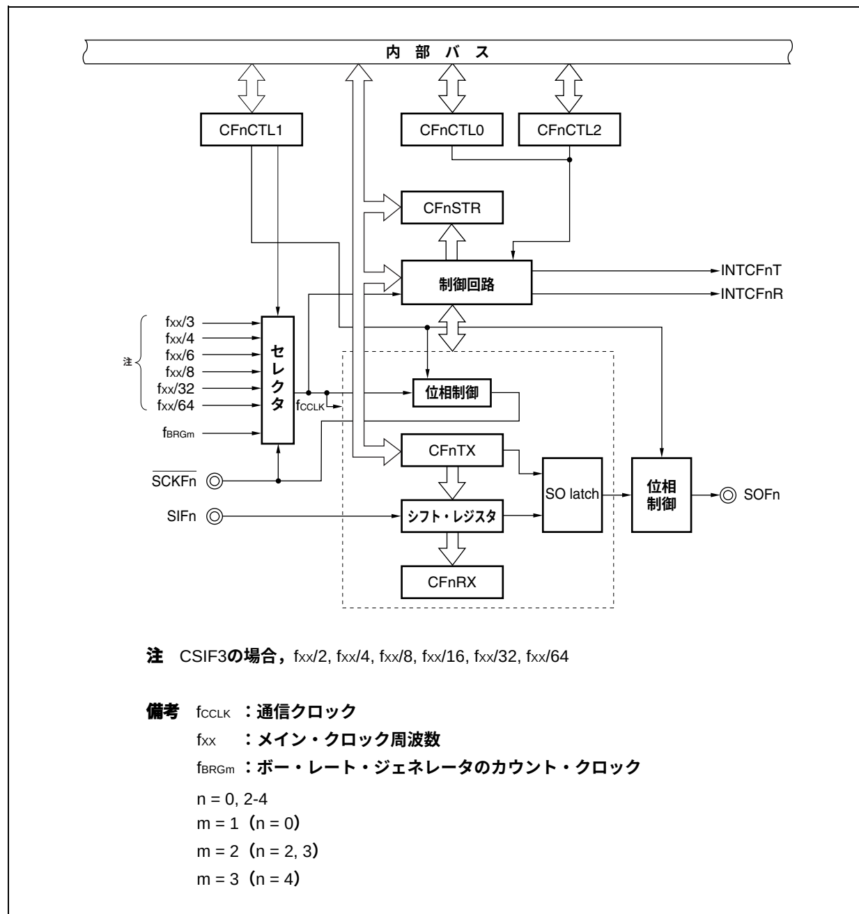
図17-4 CSIFnのブロック図
