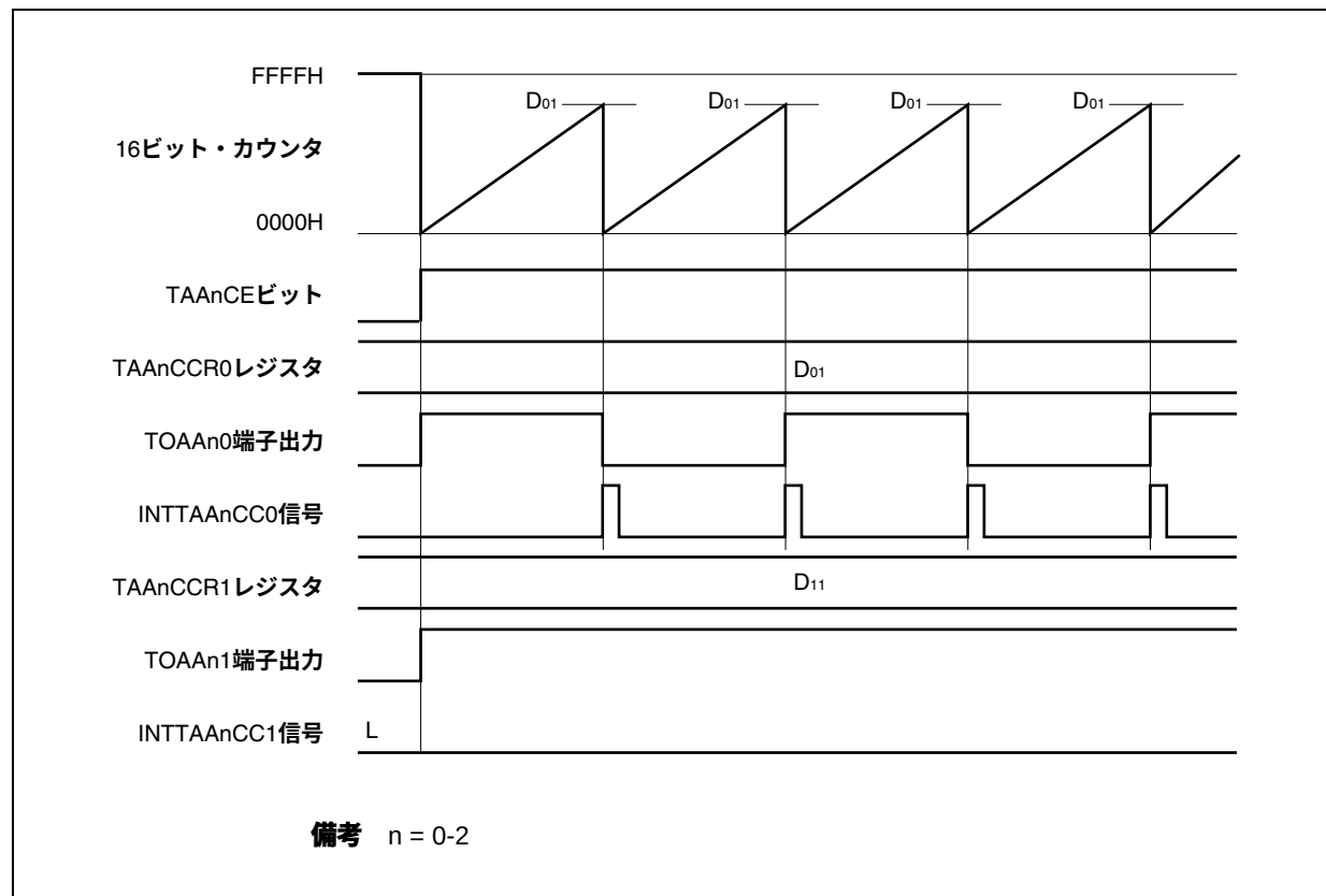
図6-13 D 01 <D 11 の場合のタイミング図
