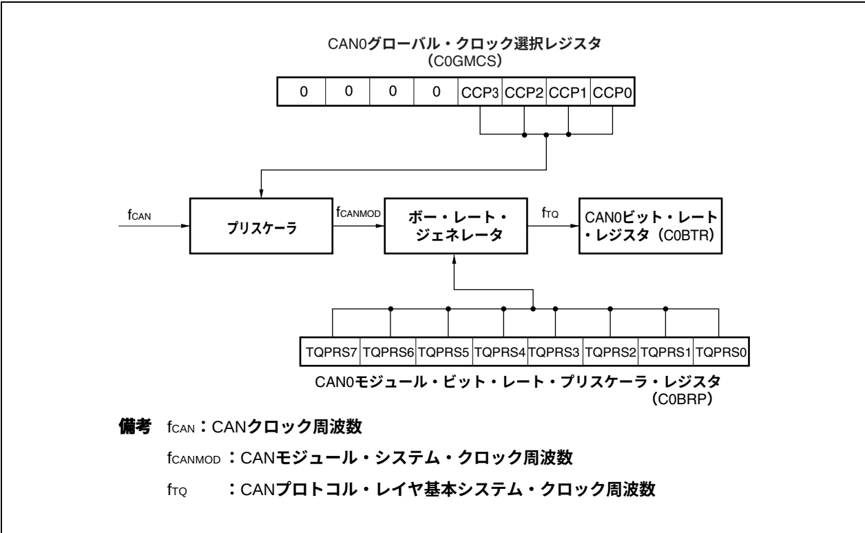
図19-23 CANモジュールのクロック
