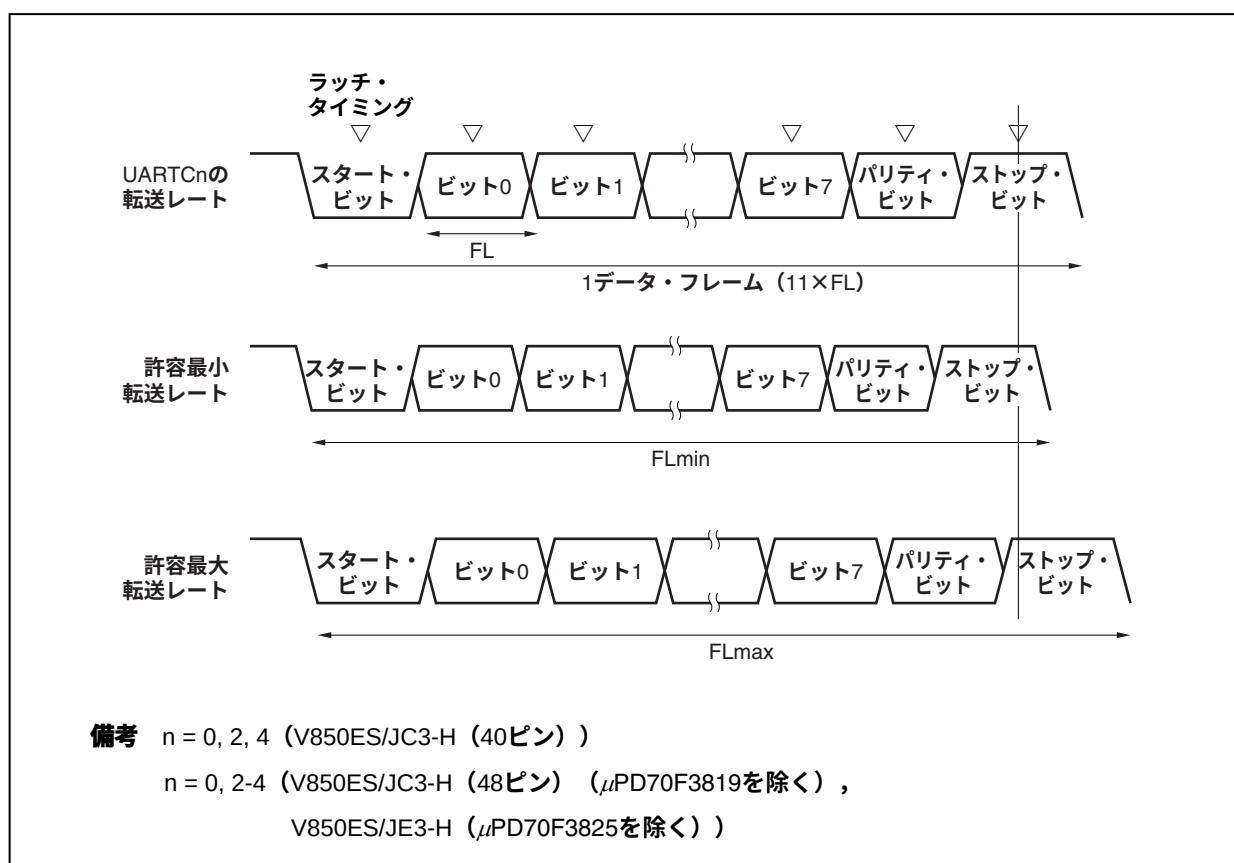
図16-19 受信時の許容ボー・レート範囲
