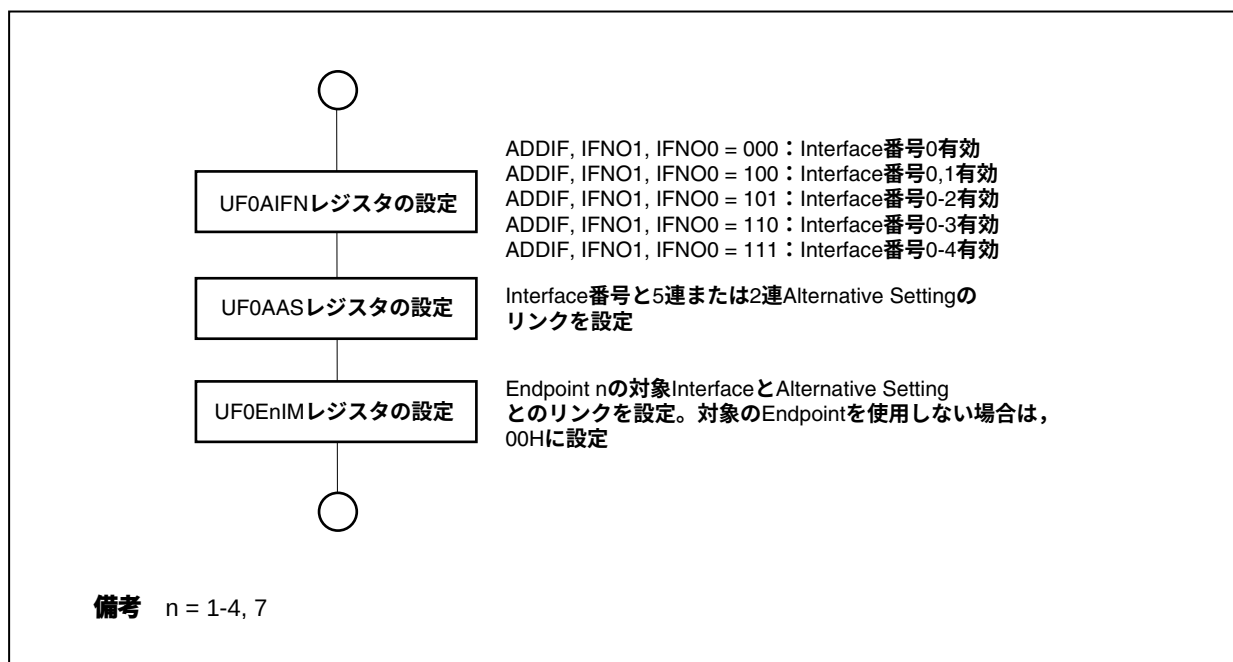
図20-16 InterfaceとEndpointの設定
