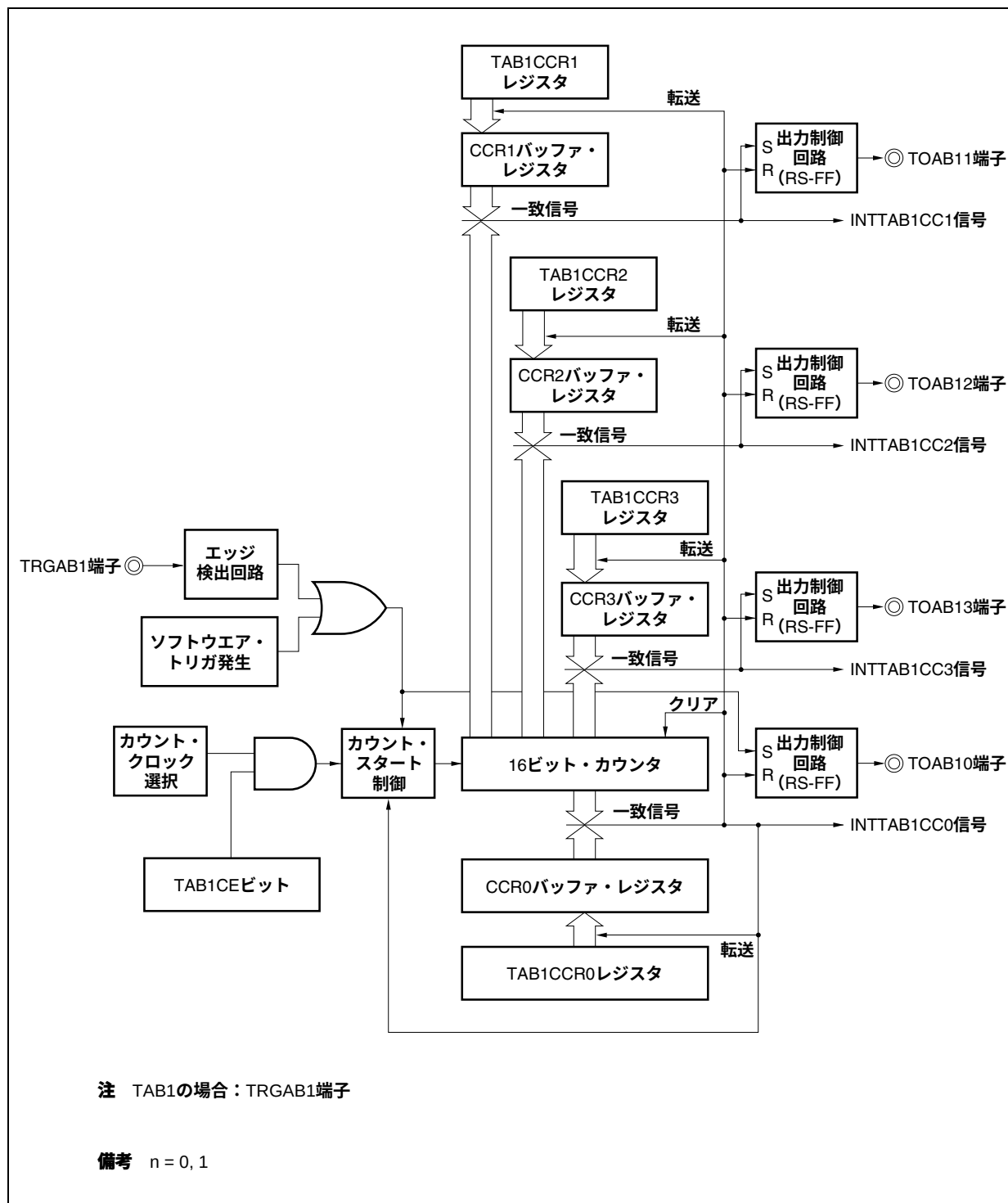
図7-20 ワンショット・パルス出力モードの構成図
