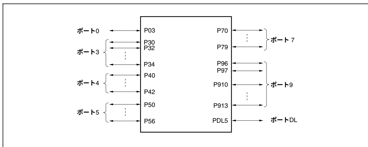
図4-2 ポートの構成図 (V850ES/JC3-H (40ピン))
