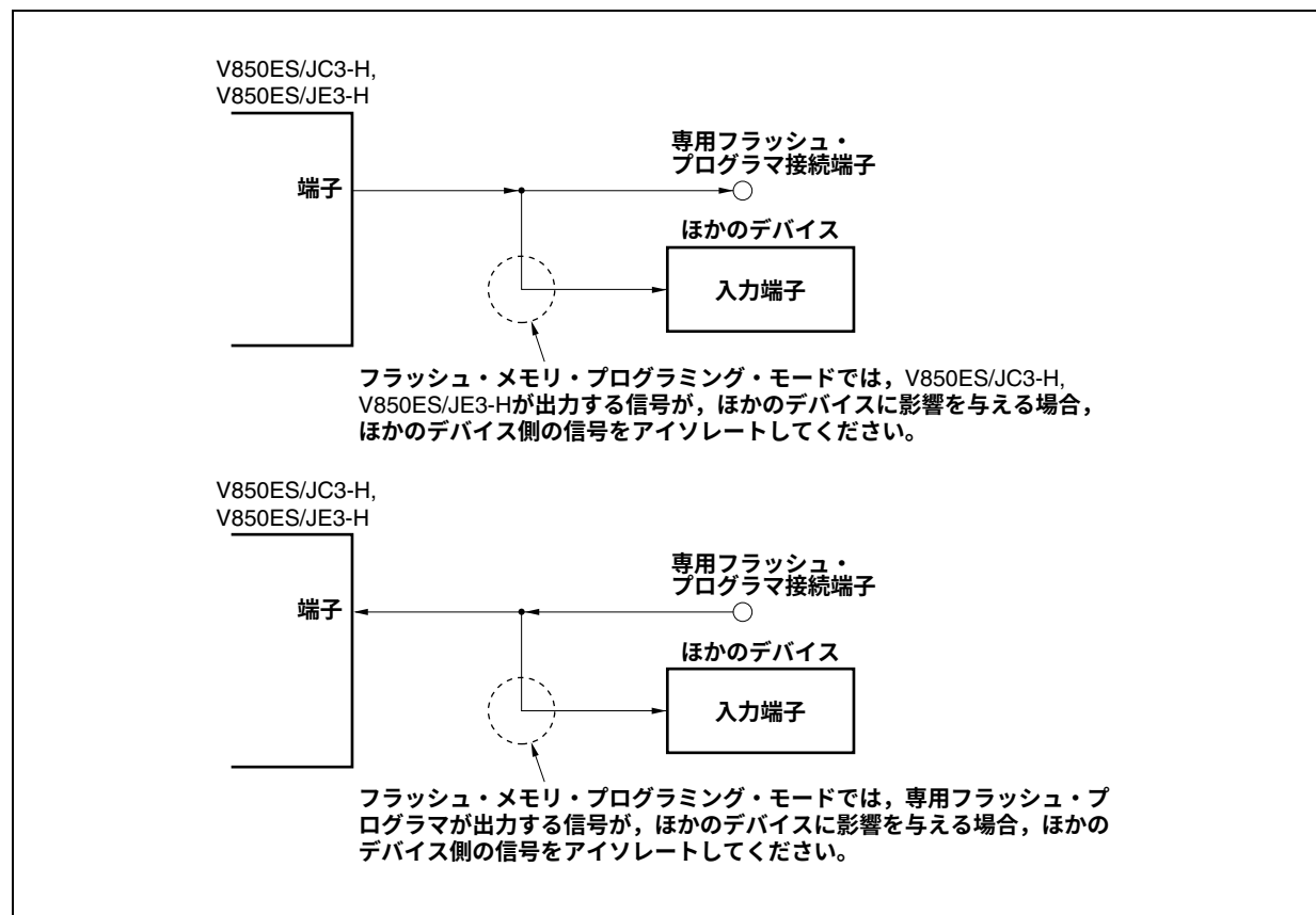
図30-15 ほかのデバイスの異常動作
