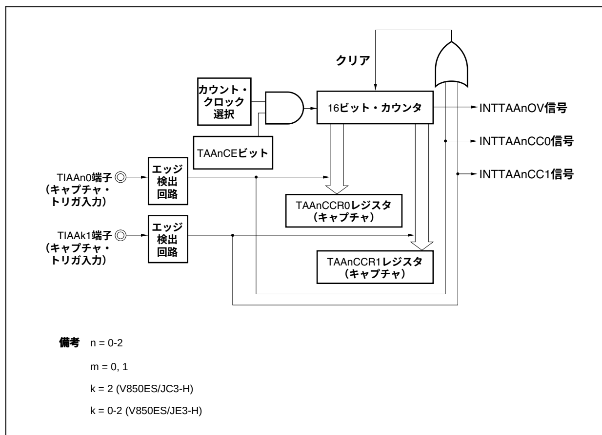
図6-39 パルス幅測定モードの構成図
