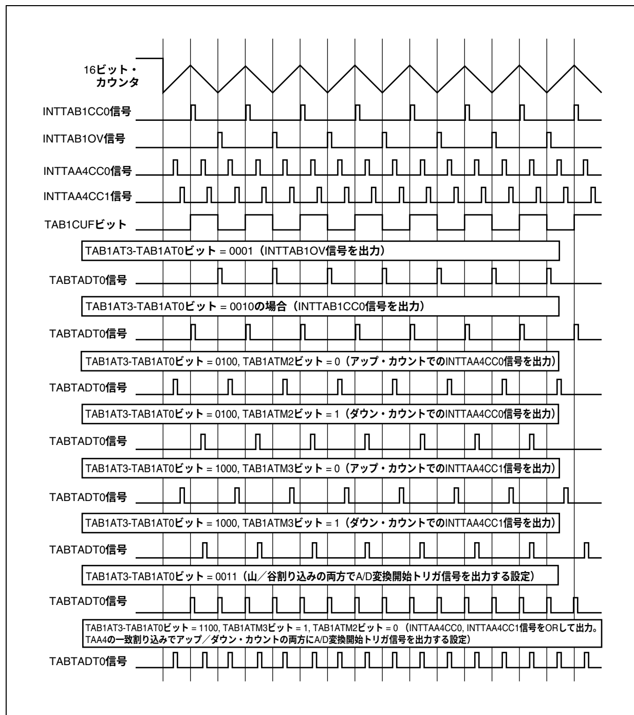
図10-38 A/D変換開始トリガ (TABTADT0) 信号出力例 (TAB1OPT1.TAB1ICEビット = 1, TAB1IOEビット = 1, TAB1ID4-TAB1ID0ビット = 00000 : 割り込み間引きなし)
