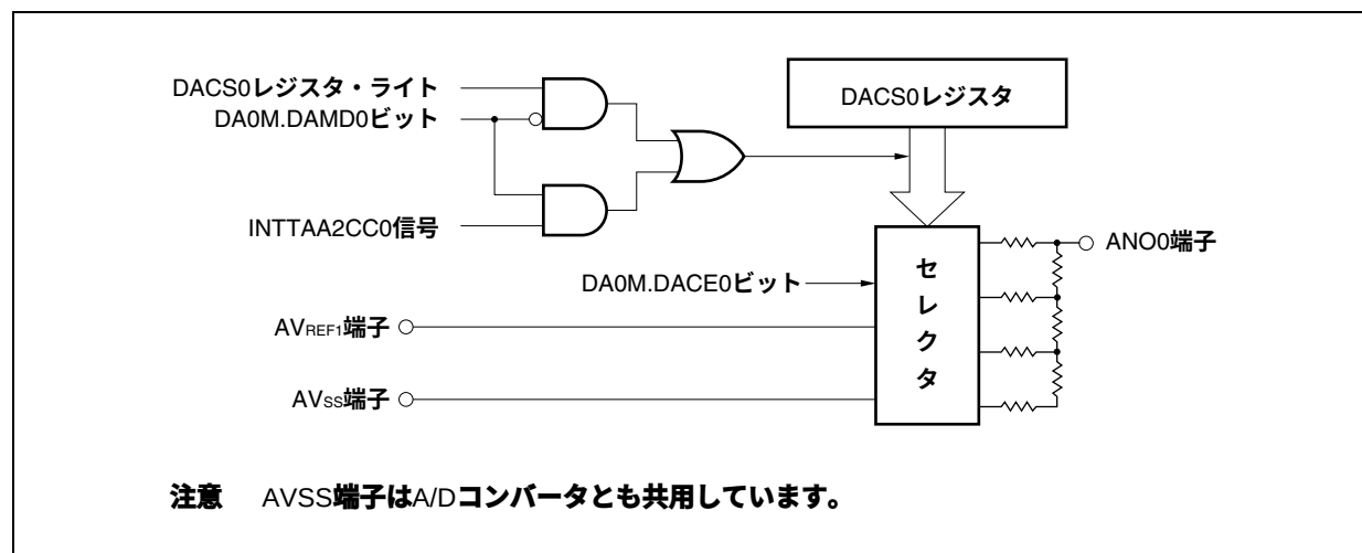
図15-1 D/Aコンバータのブロック図
