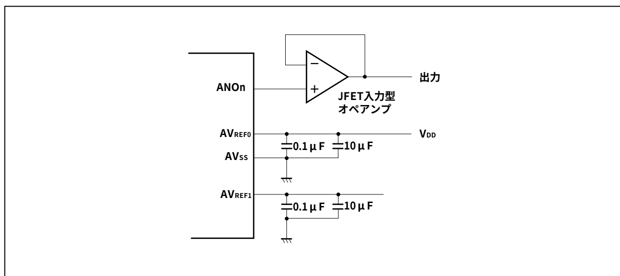
図15-2 外部端子の接続例
