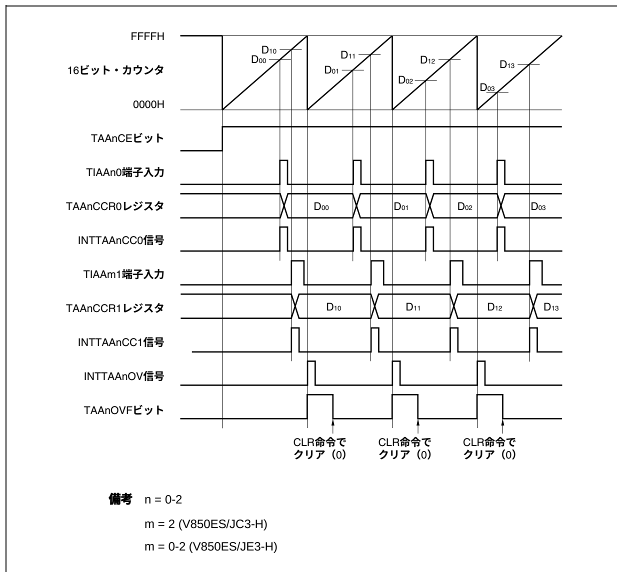
図6-35 フリー・ランニング・タイマ・モードの基本タイミング (キャプチャ機能)
