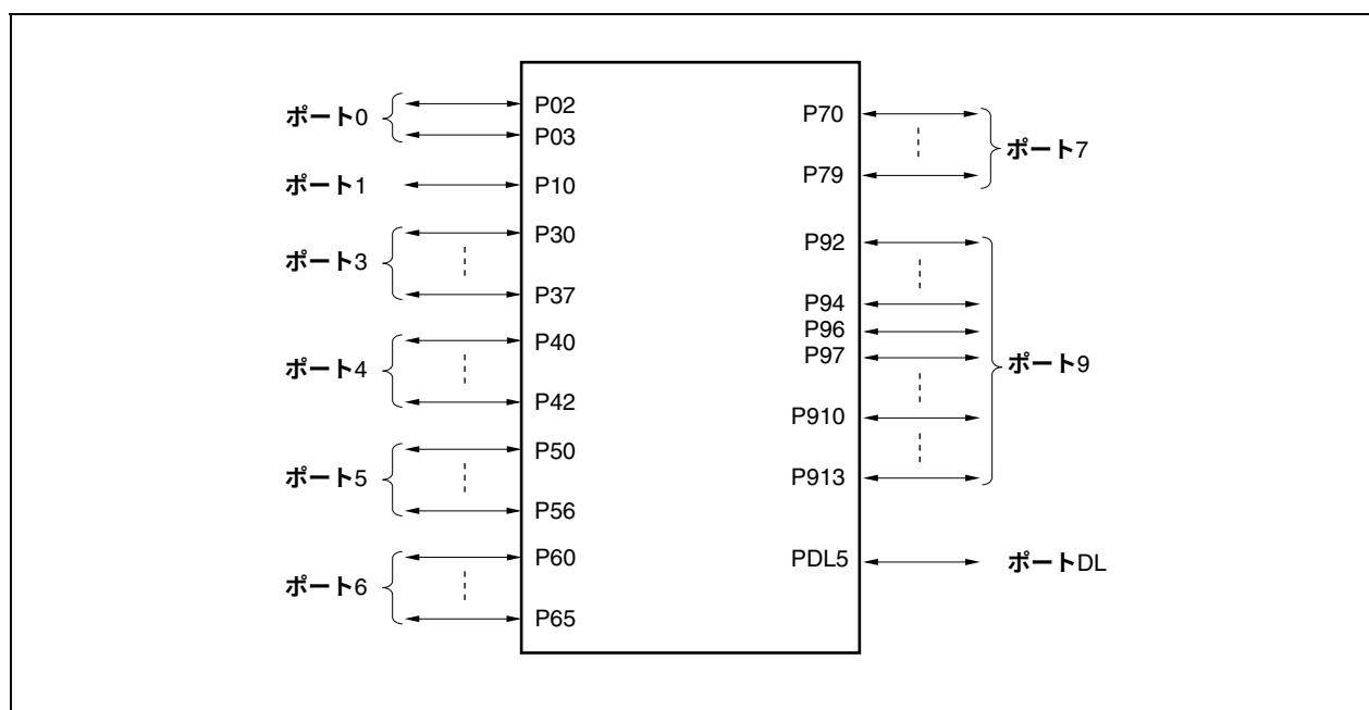
図4-3 ポートの構成図 (V850ES/JE3-H)
