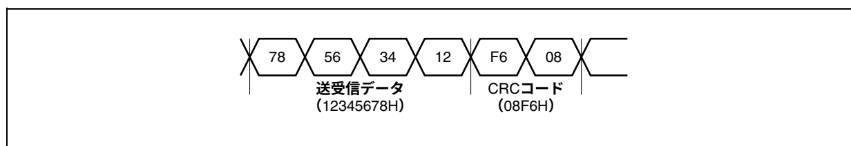
図28-4 CRC送信例
