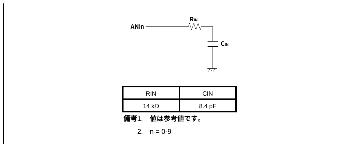
図14-14 ANIn端子内部等価回路
