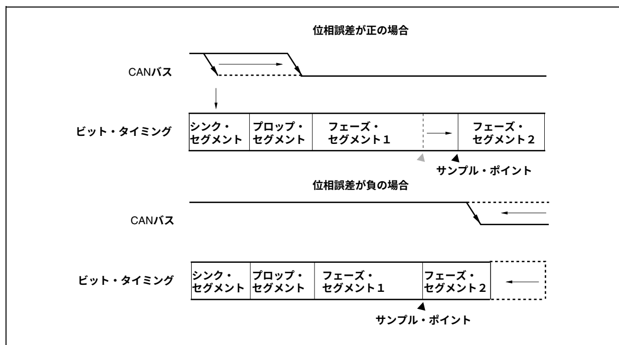
図19-21 再同期
