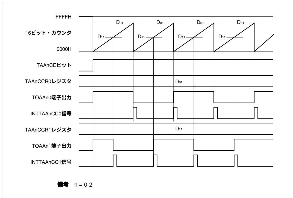
図6-12 D_{01} \geq D_{11} の場合のタイミング図
