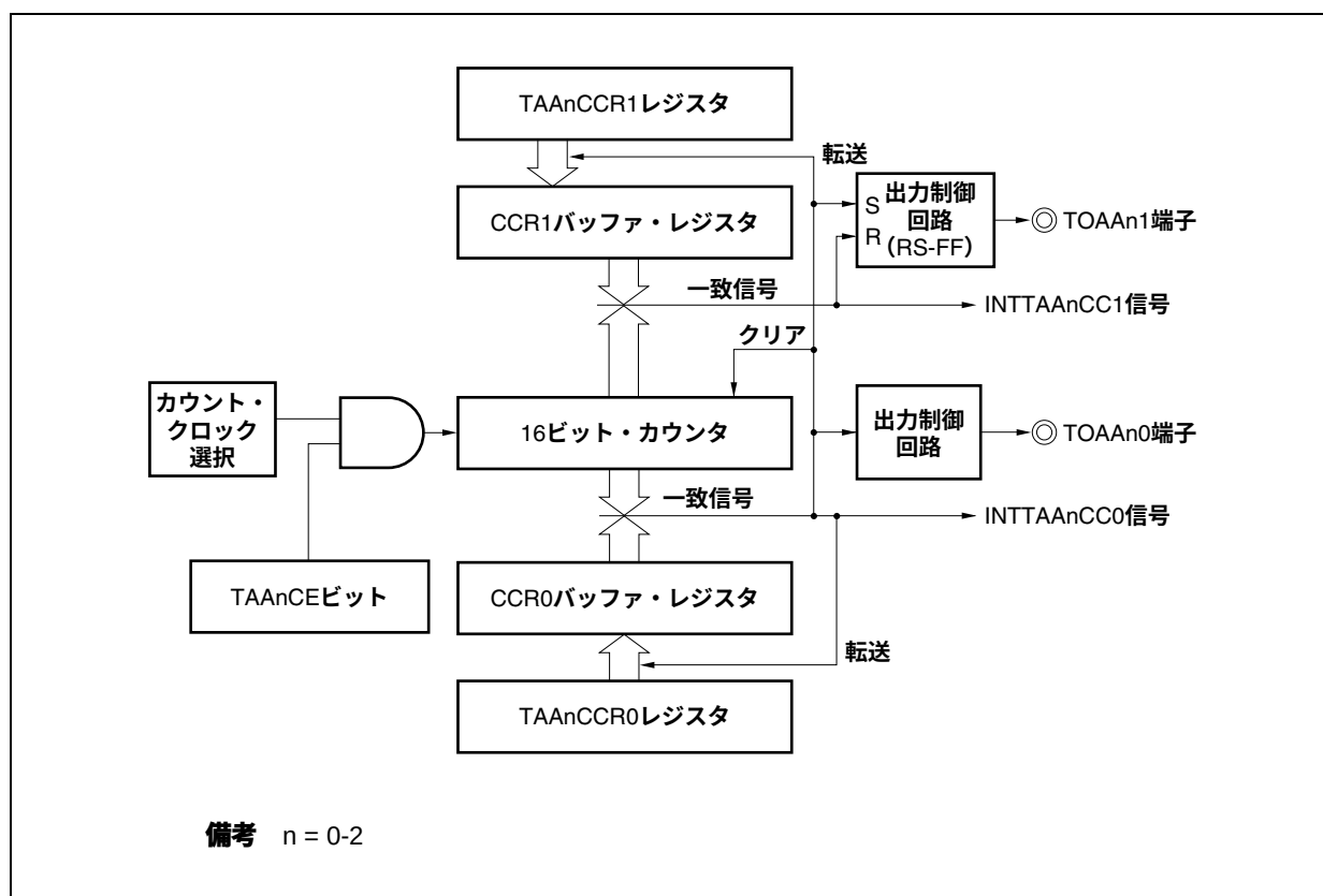
図6-29 PWM出力モードの構成図
