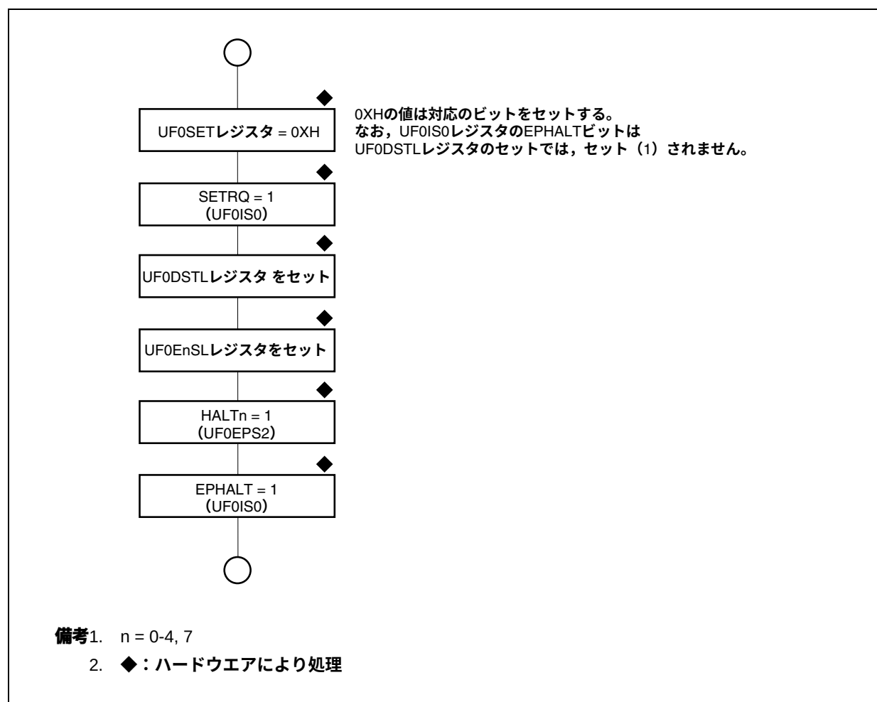
図20-22 SET_CONFIGURATION処理
