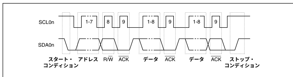
図18-7 I 2 Cバスのシリアル・データ転送タイミング
