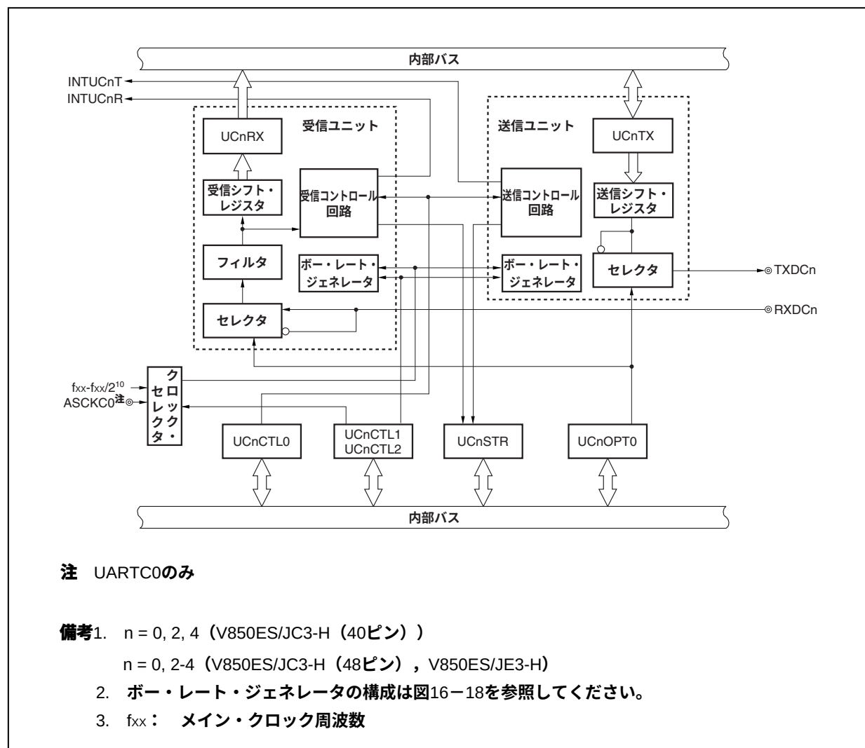
図16-1 アシクロナス・シリアル・インタフェースCnのブロック図
