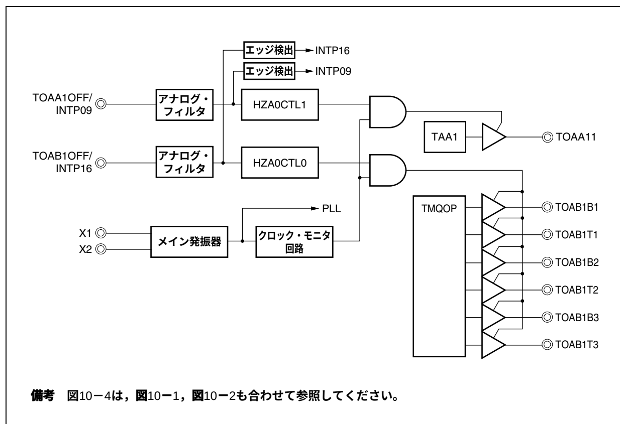
図10-4 ハイ・インピーダンス出力制御回路構成
