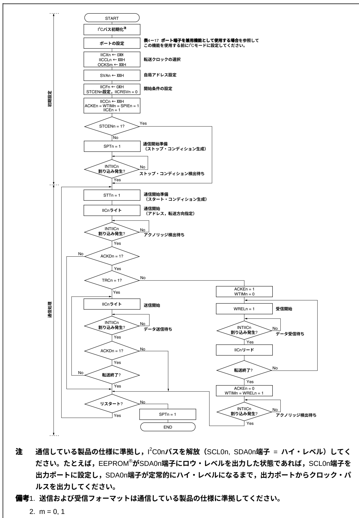
図18-18 シングルマスタ・システムでのマスタ動作
