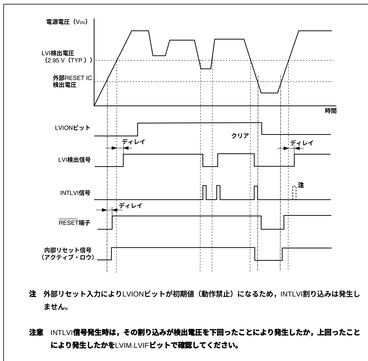
図27-3 低電圧検出回路の動作タイミング (LVIMDビット = 0)
