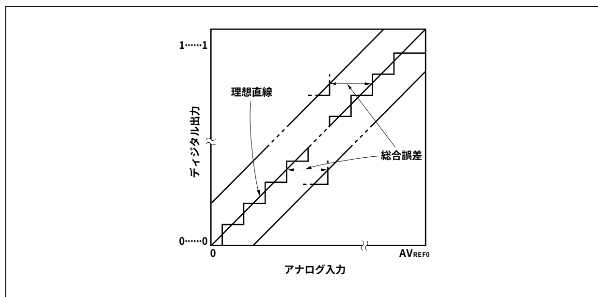
図14-16 総合誤差
