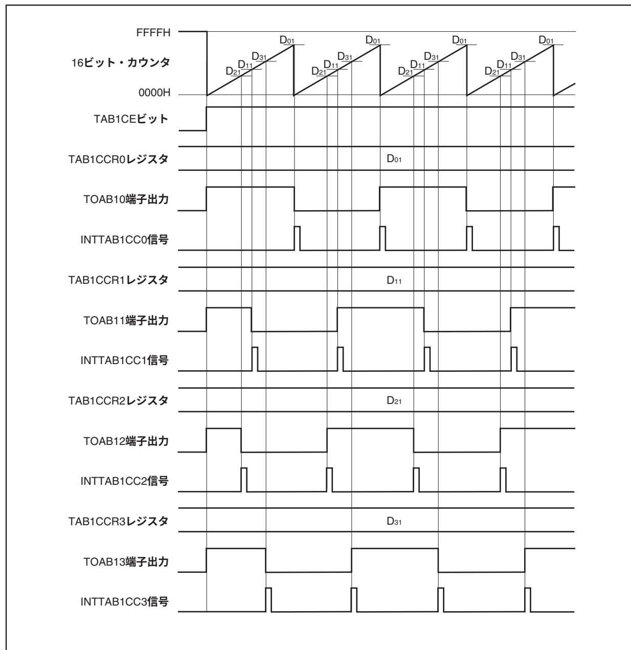
図7-7 D_{01} \geq D_{k1} の場合のタイミング図
