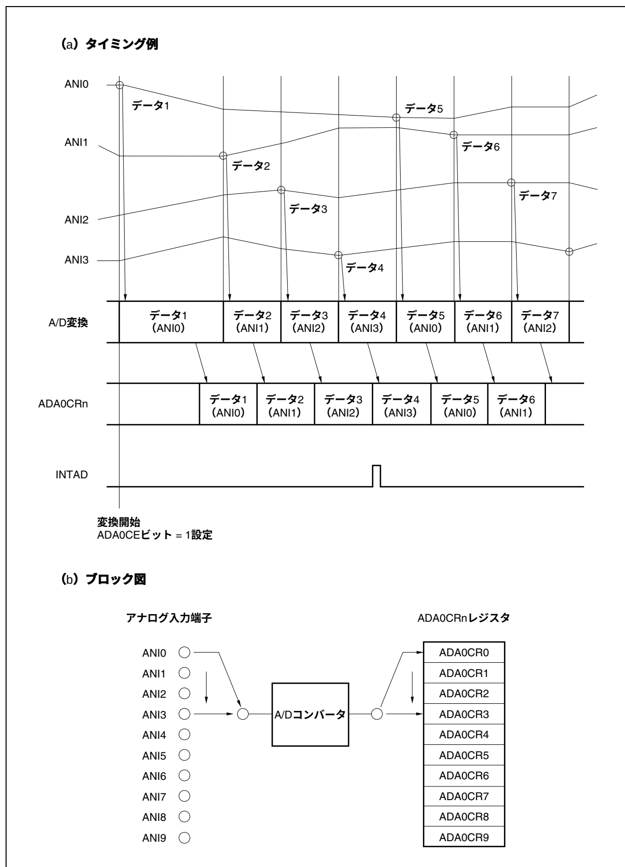
図14-5 連続スキャン・モード動作タイミング例 (ADA0Sレジスタ = 03H)
