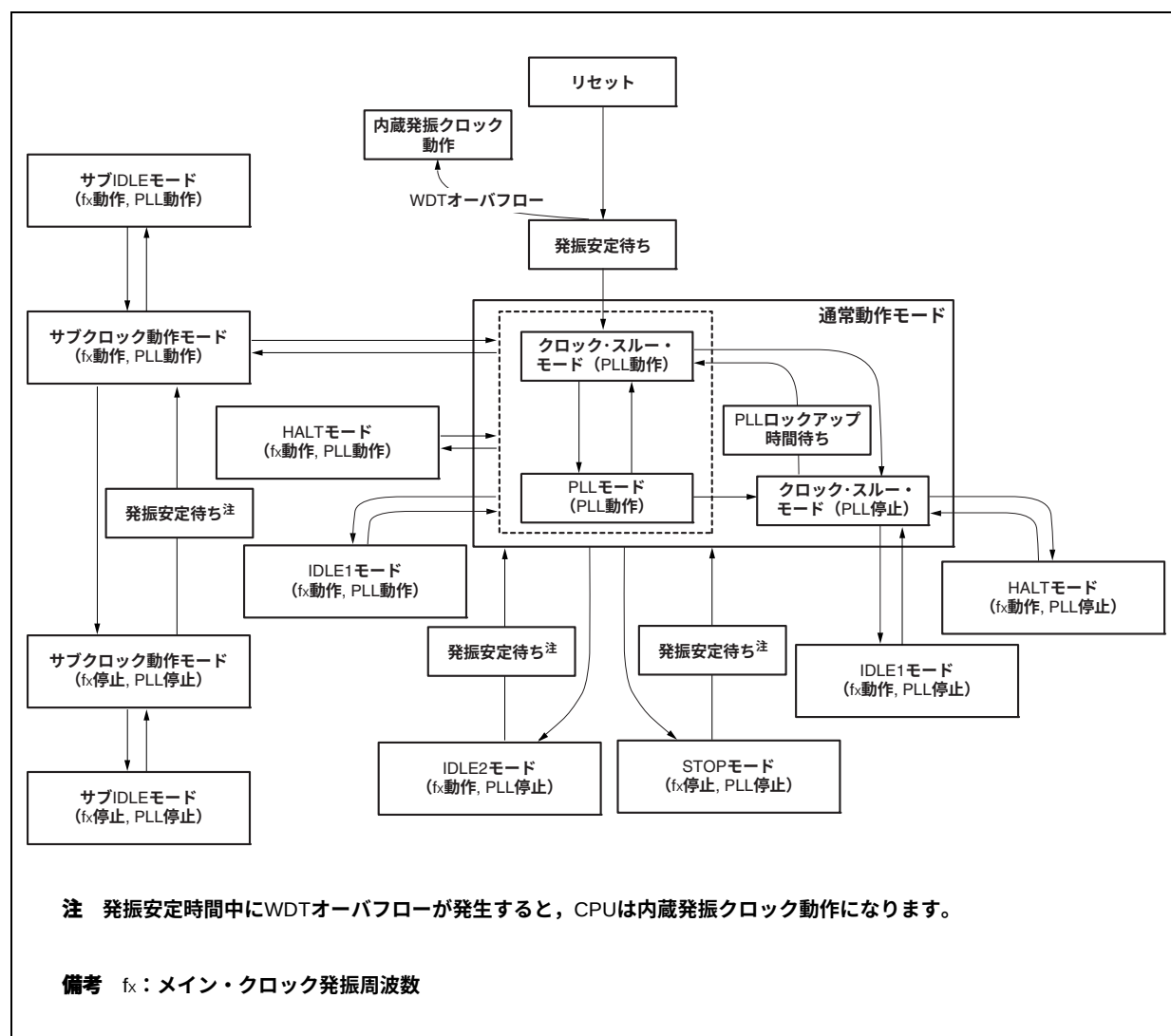
図24-1 状態遷移図
