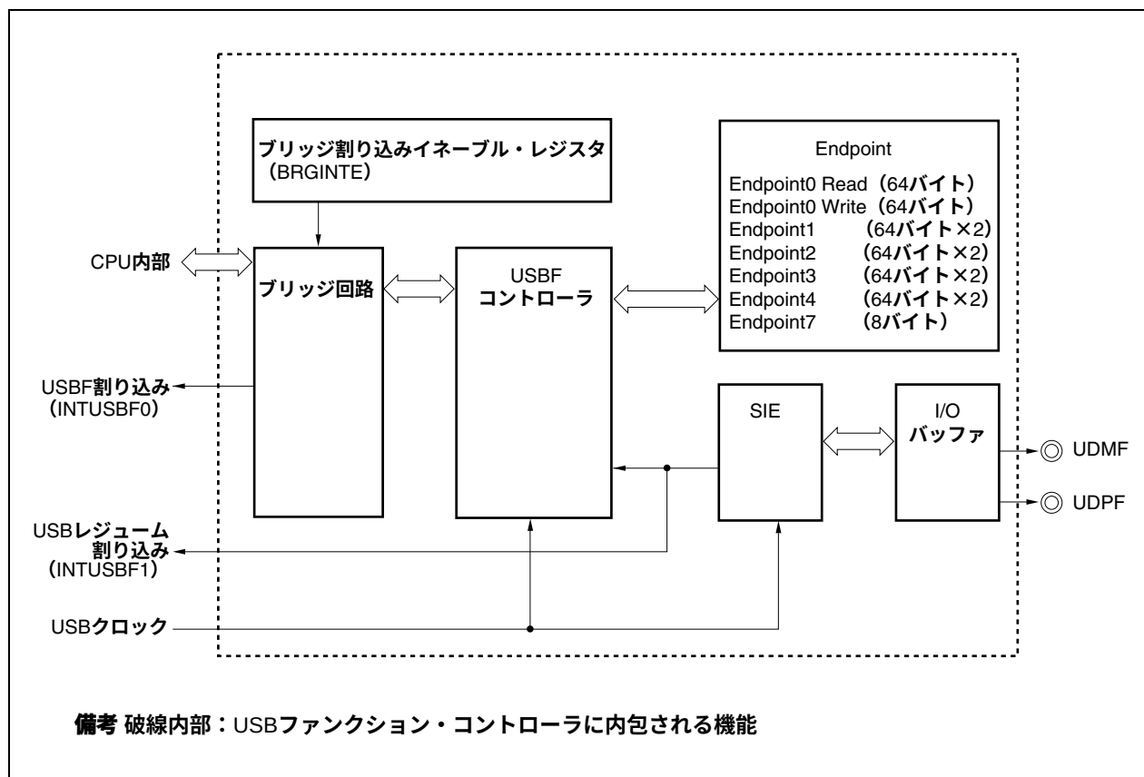
図20-1 USBファンクション・コントローラのブロック図
