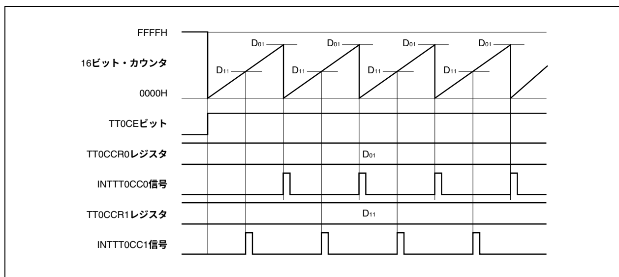
図8-19 D_{01} \geq D_{11} の場合のタイミング図
