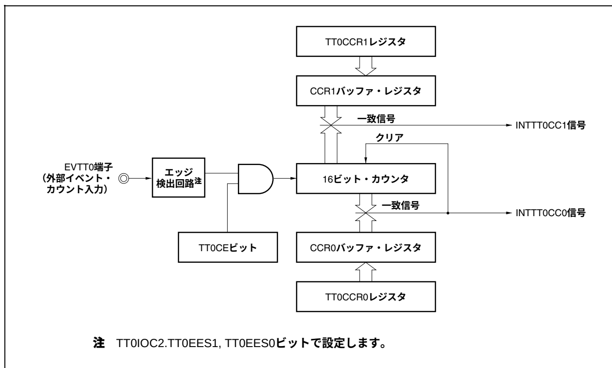
図8-18 TT0CCR1レジスタ1の構成図
