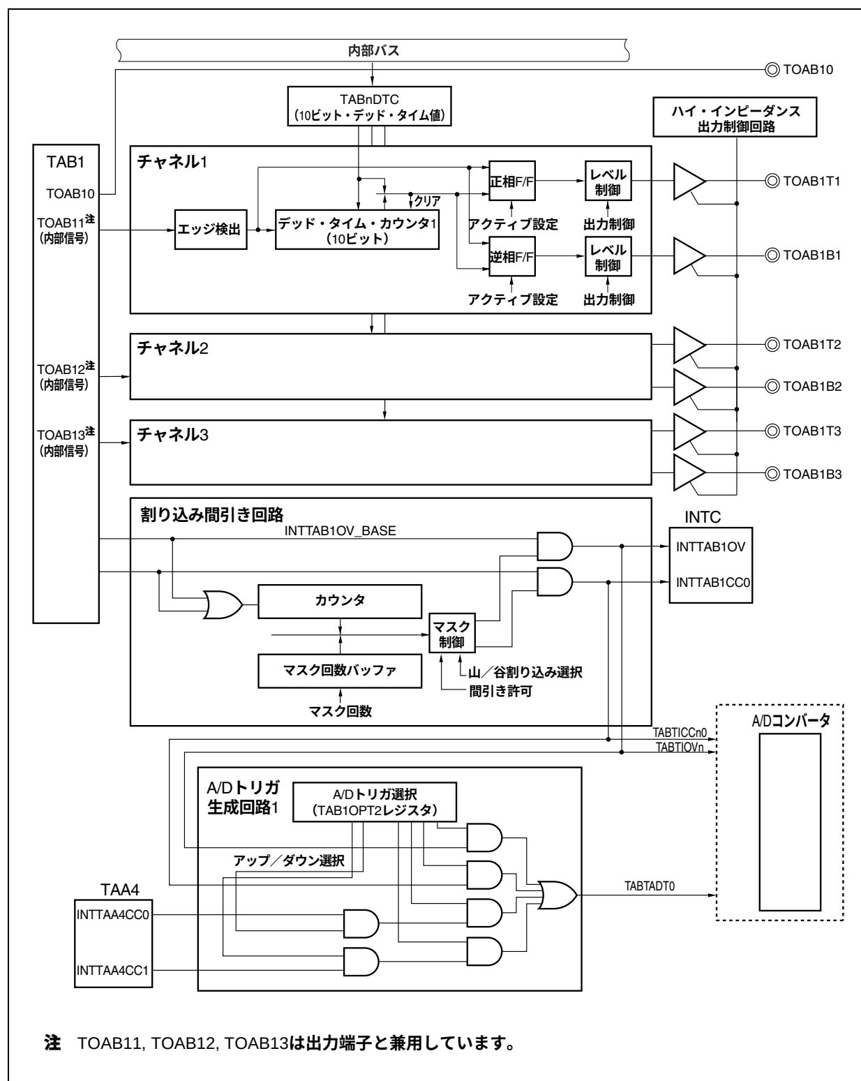
図10-2 TMQ1オプション
