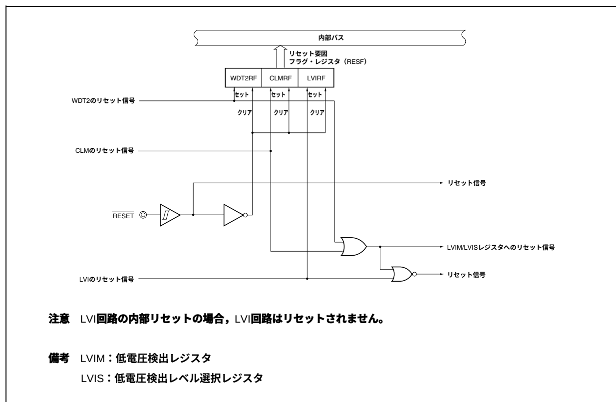
図25-1 リセット機能のブロック図
