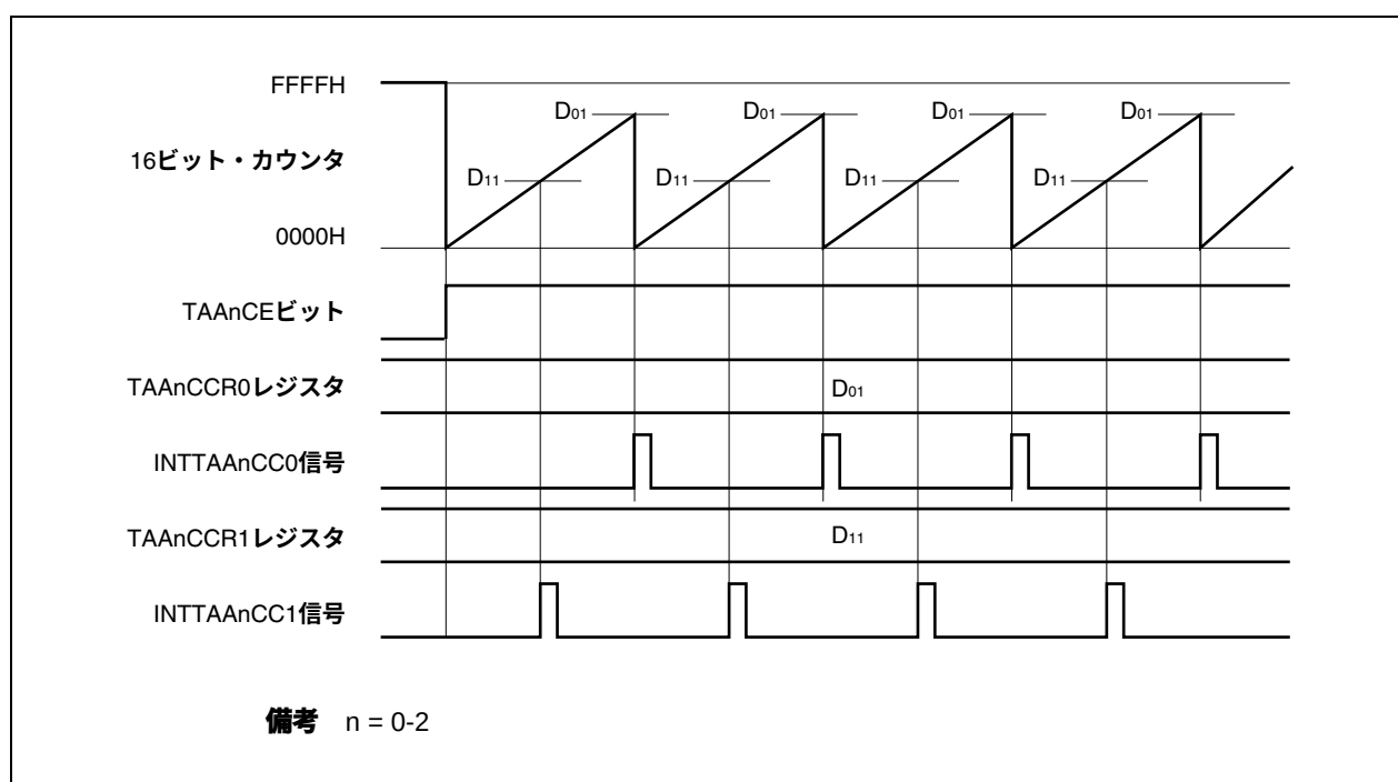
図6-19 D_{01} \geq D_{11} の場合のタイミング図
