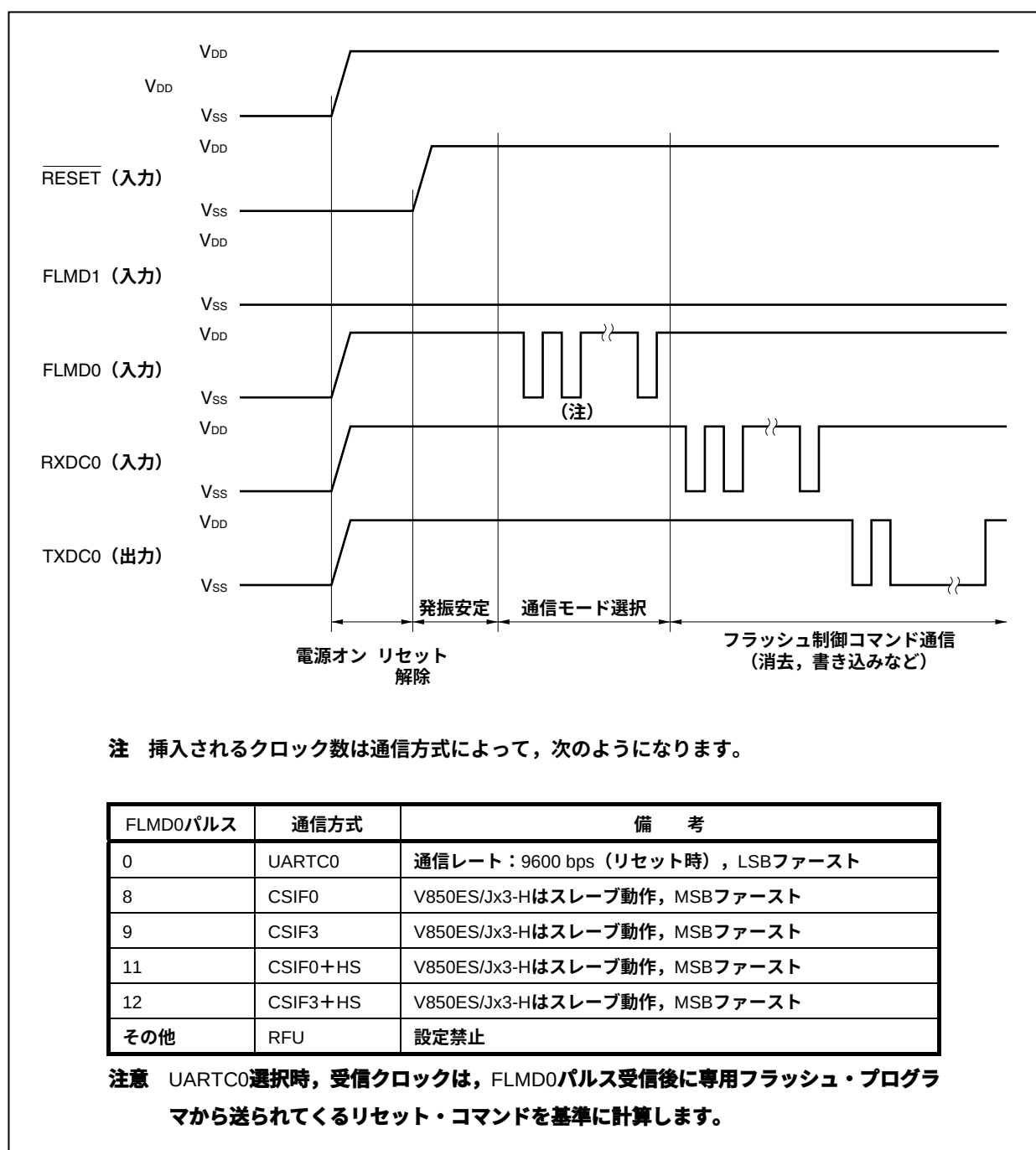
図30-10 通信方式の選択
