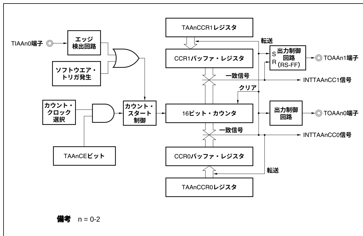
図6-21 外部トリガ・パルス出力モードの構成図
