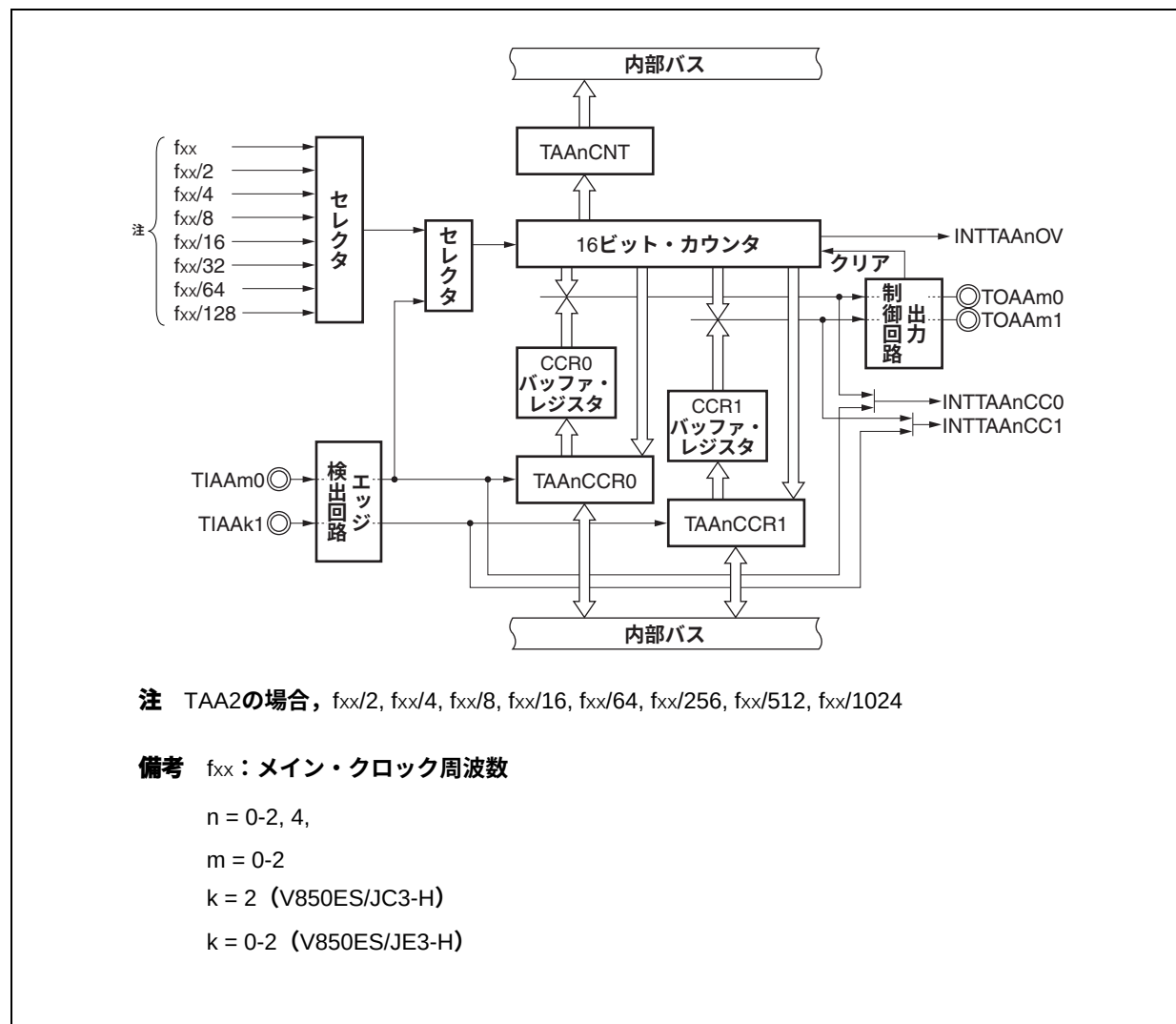
図6-1 TAA n のブロック図
