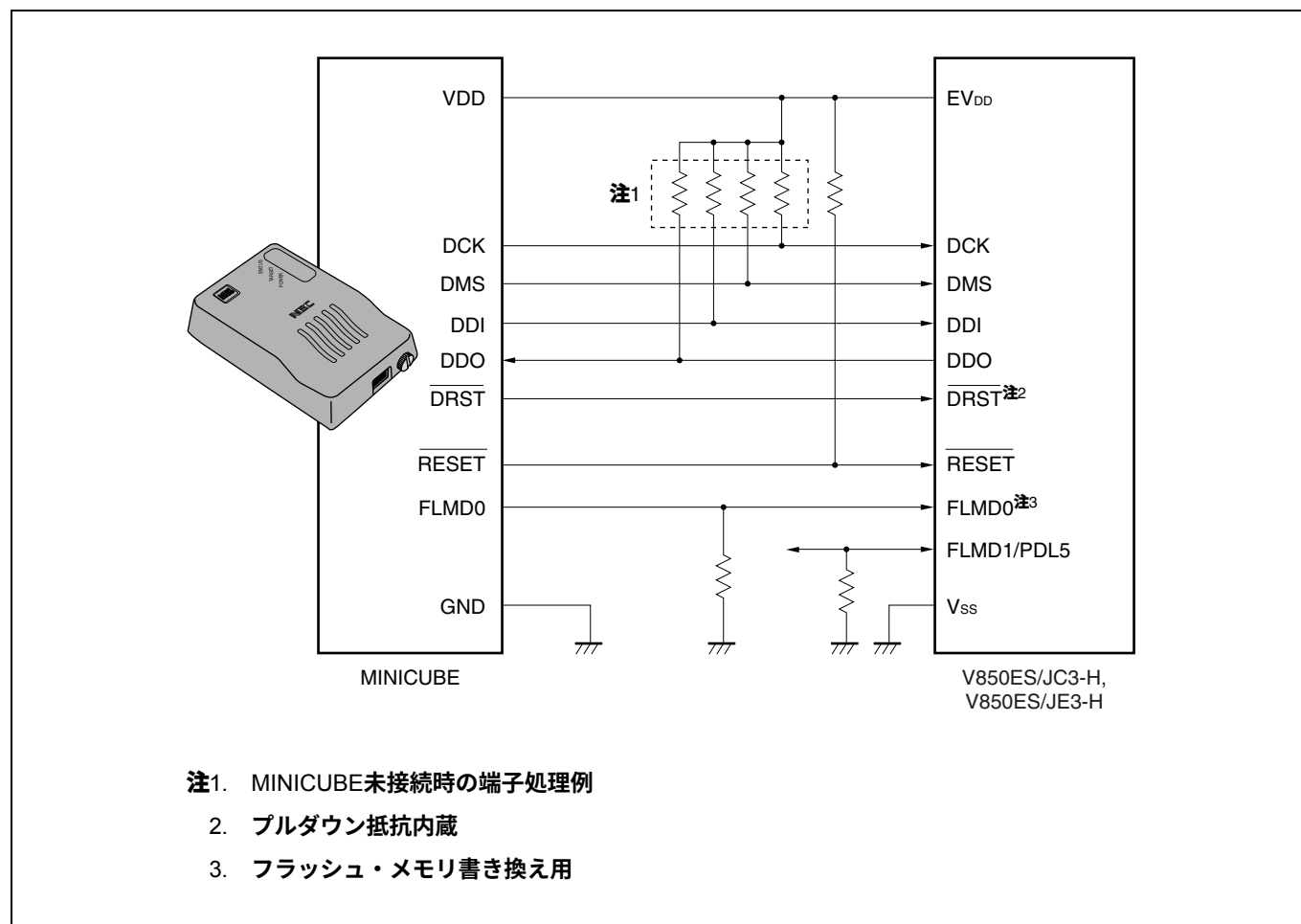
図31-1 デバッグ・インタフェース端子を通信インタフェースとして使用する場合の回路接続例
