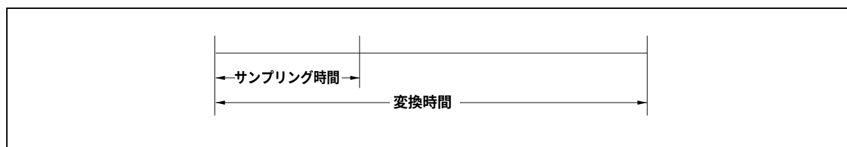
図14-22 サンプリング時間
