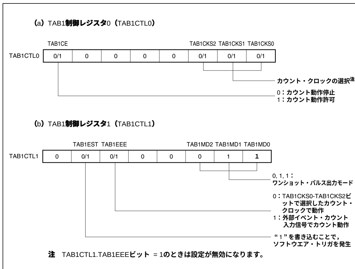
図7-22 ワンショット・パルス出力モード動作時のレジスタ設定内容 (1/3)
