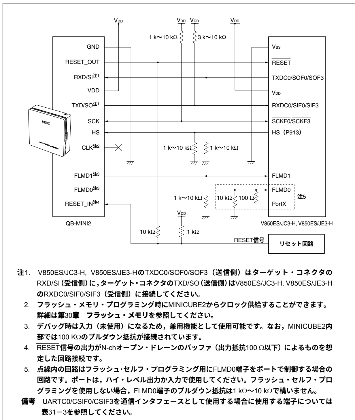
図31-3 UARTC0/CSIF0/CSIF3を通信インタフェースとして使用する場合の回路接続例
