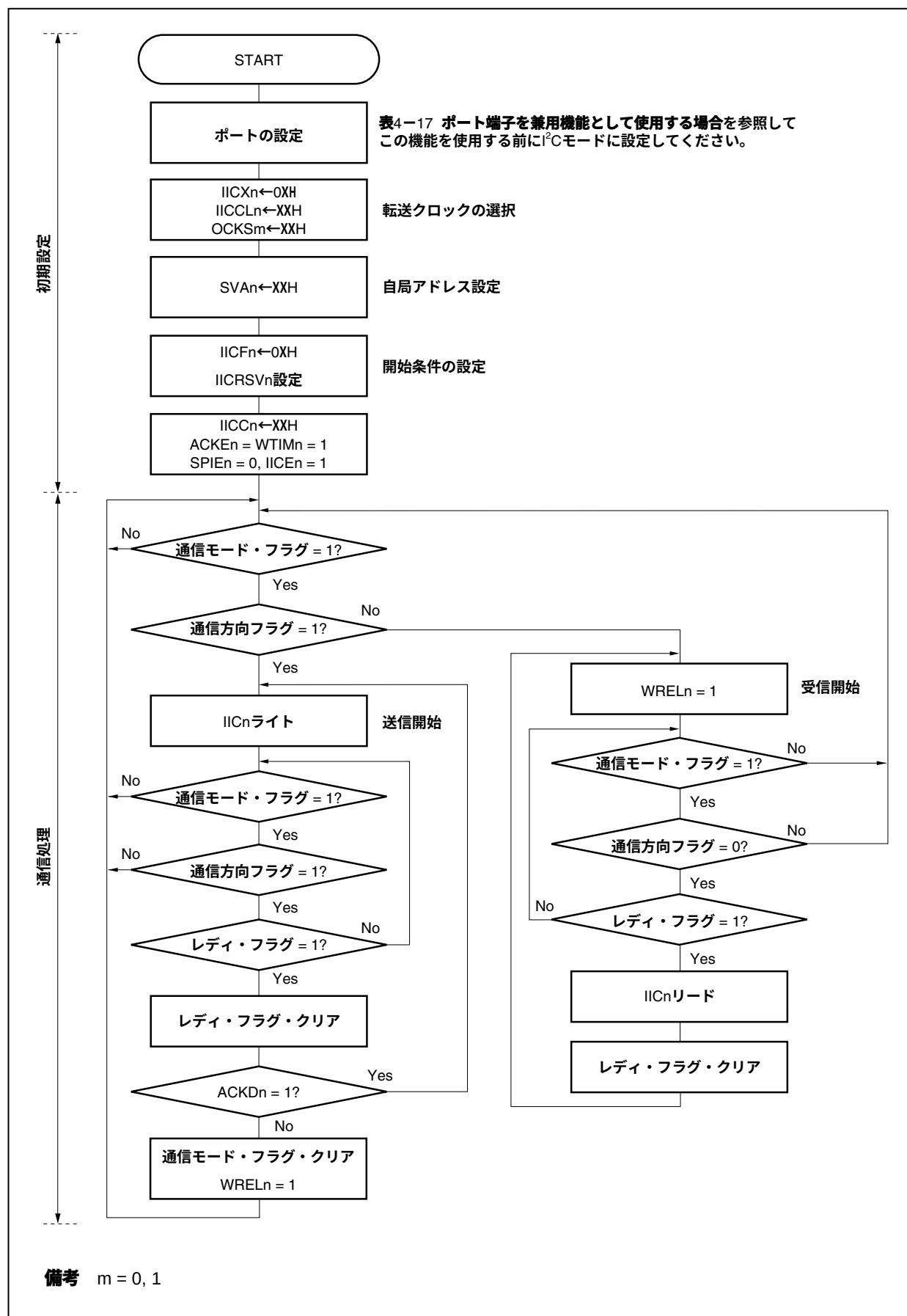
図18-21 スレーブ動作手順 (1)
