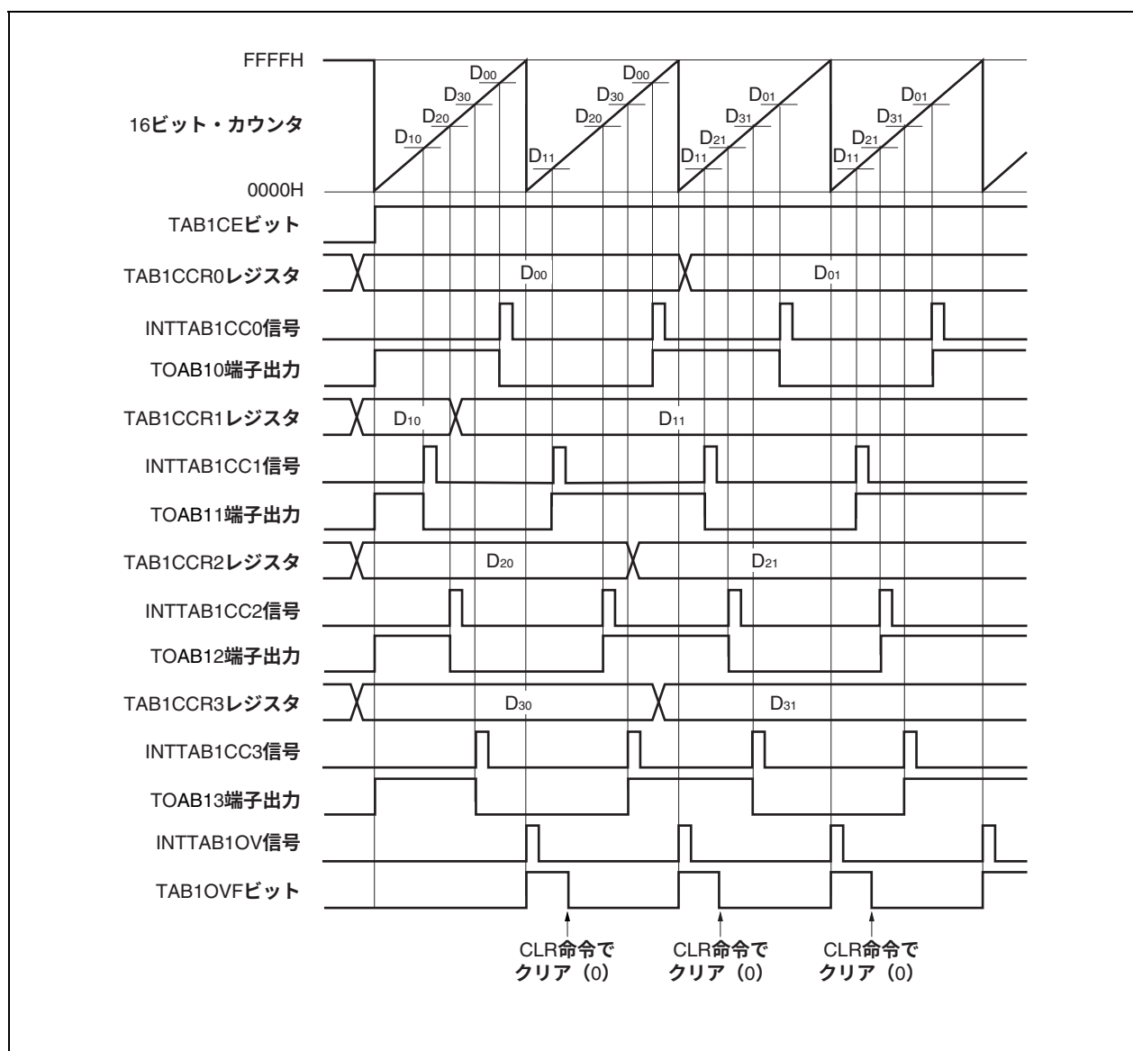
図7-29 フリー・ランニング・タイマ・モードの基本タイミング (コンパレー機能)
