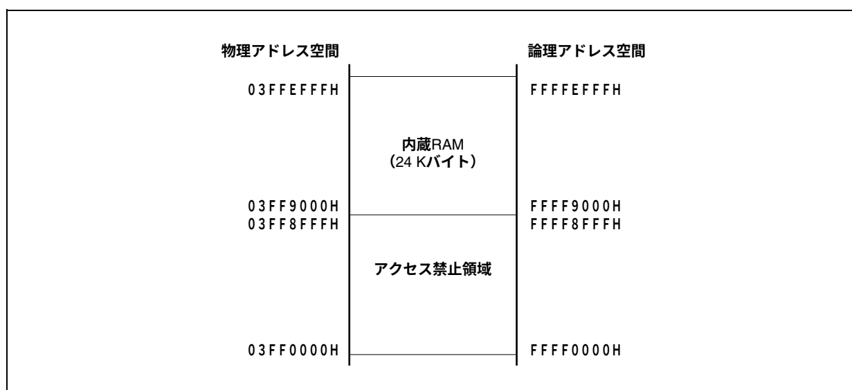
図3-11 内蔵RAM領域 (24 Kバイト)
