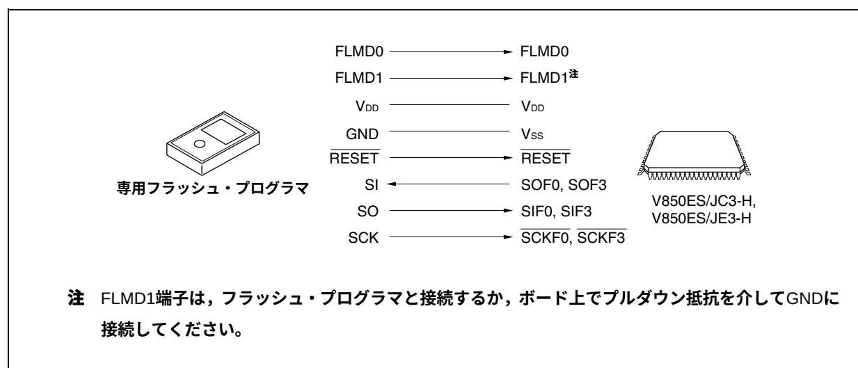
図30-4 専用フラッシュ・プログラマとの通信 (CSIF0, CSIF3)
