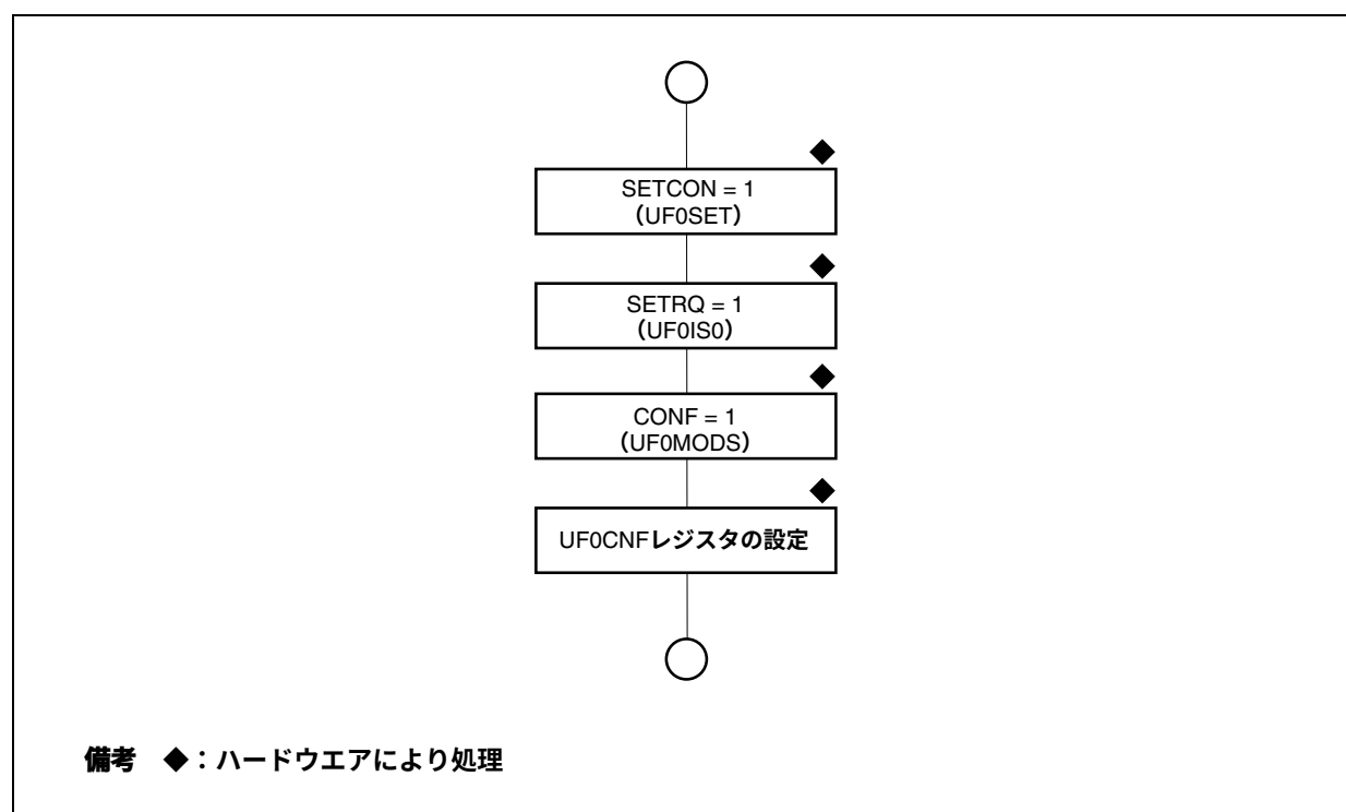
図20-22 SET_CONFIGURATION処理
