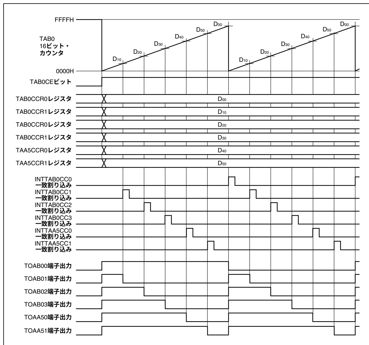
図6-47 同調PWM機能のタイミング例 (TAB0, TAA5)
