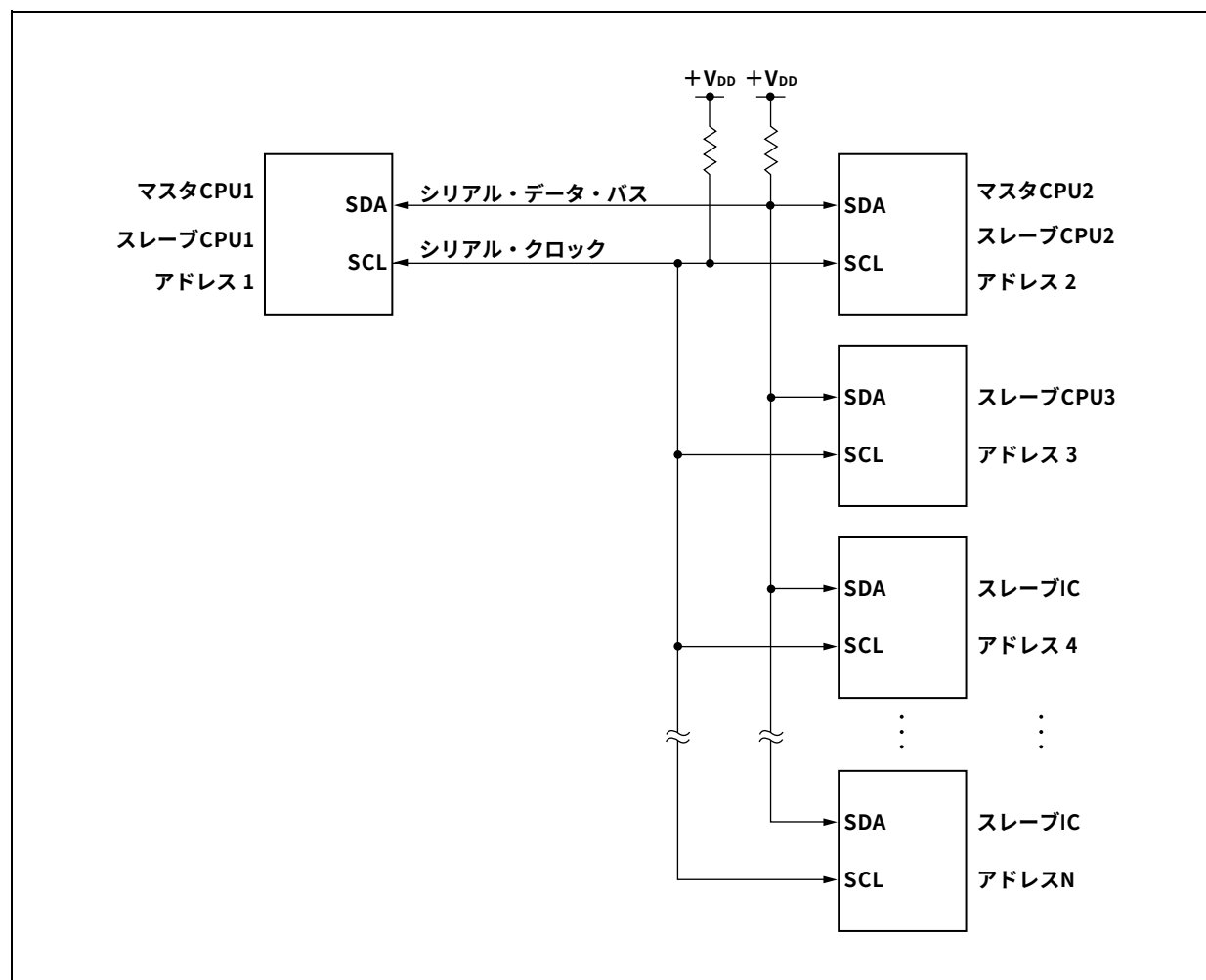
図18-5 I 2 Cバスによるシリアル・バス構成例
