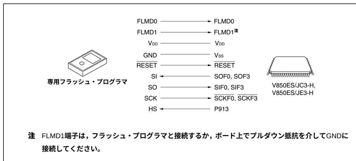
図30-5 専用フラッシュ・プログラマとの通信（CSIF0+HS, CSIF3+HS）
