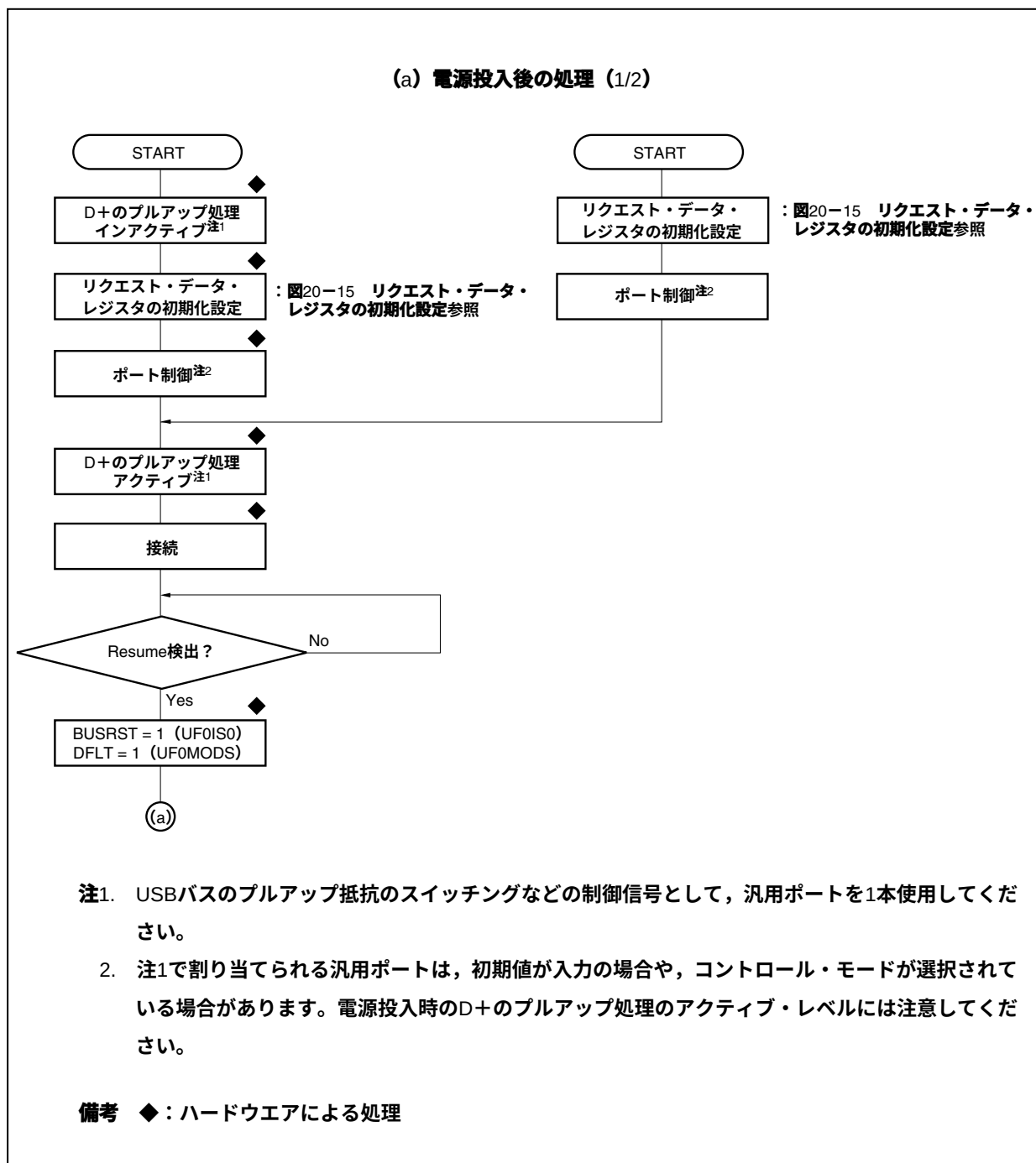
図20-31 電源投入後の処理／電源切断の処理例 (1/3)
