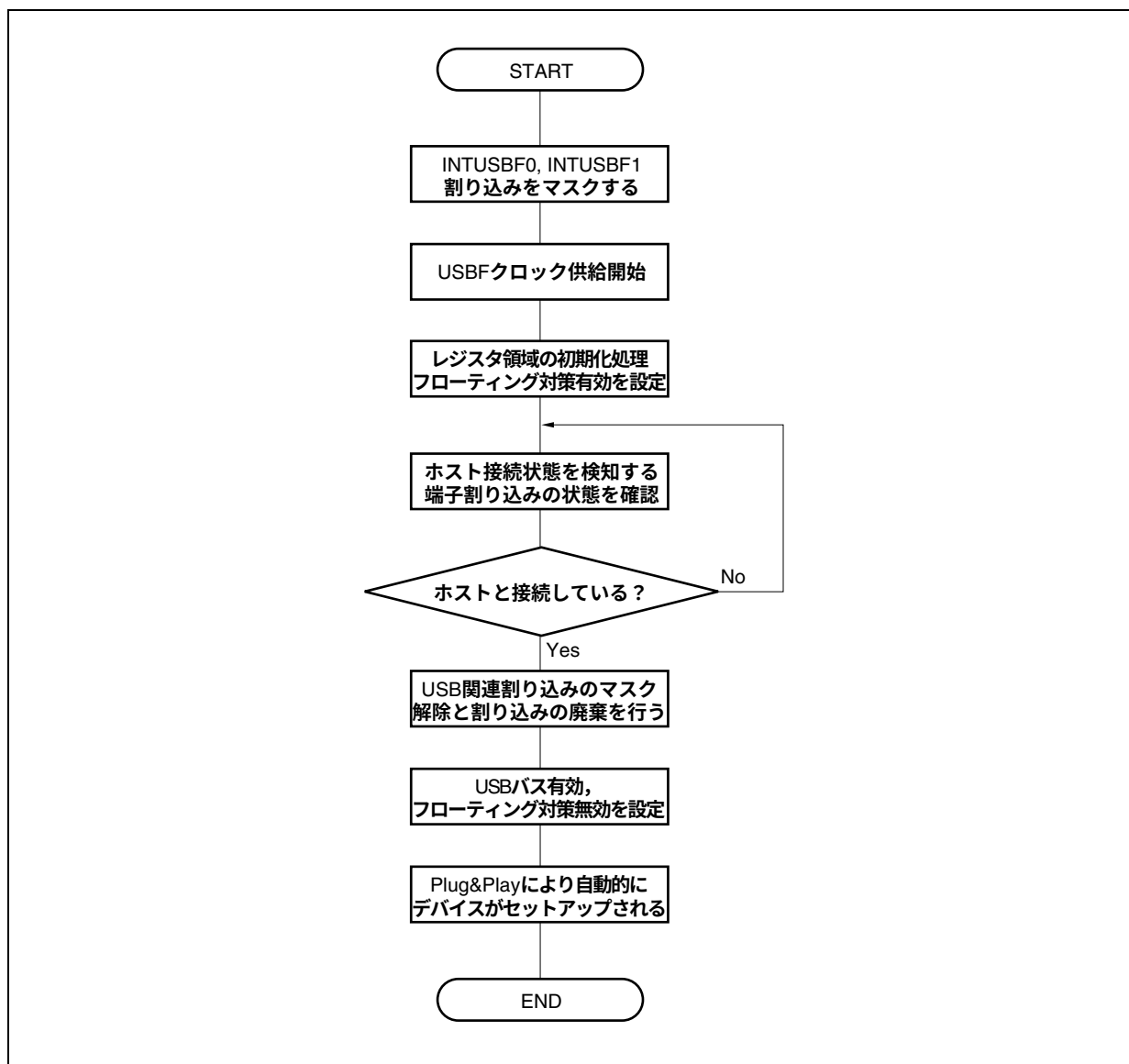
図20-13 電源投入時のプログラムのフロー・チャート
