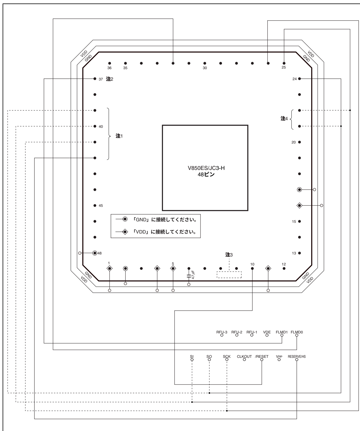
図30-7 V850ES/JC3-H (48ピン) フラッシュ書き込み用アダプタの配線例 (CSIF0+HSモード時) (1/2)
