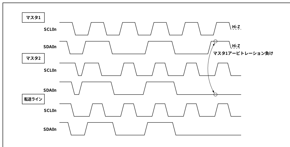
図18-14 アービトレーション・タイミング例
