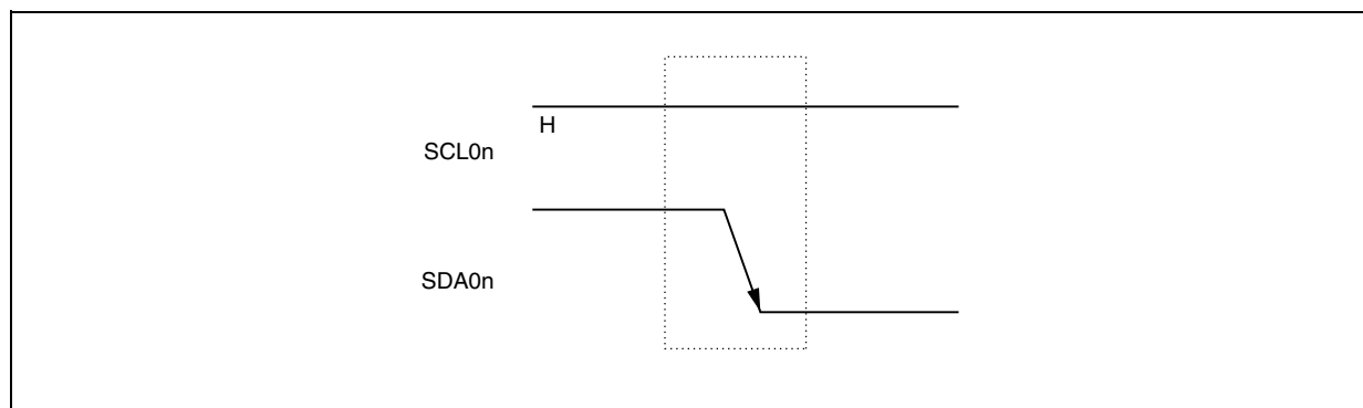
図18-8 スタート・コンディション
