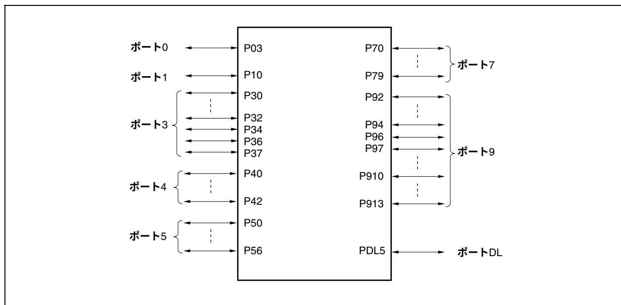
図4-2 ポートの構成図 (V850ES/JC3-H (40ピン))
