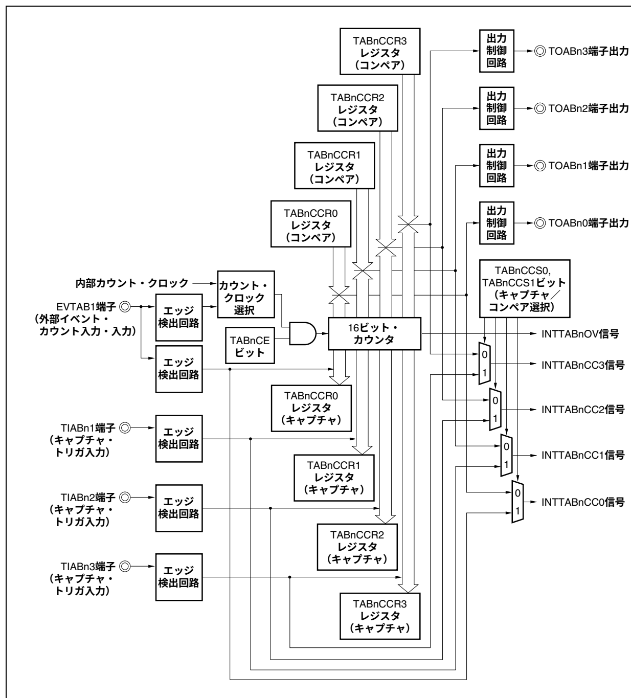
図7-28 フリー・ランニング・タイマ・モードの構成図
