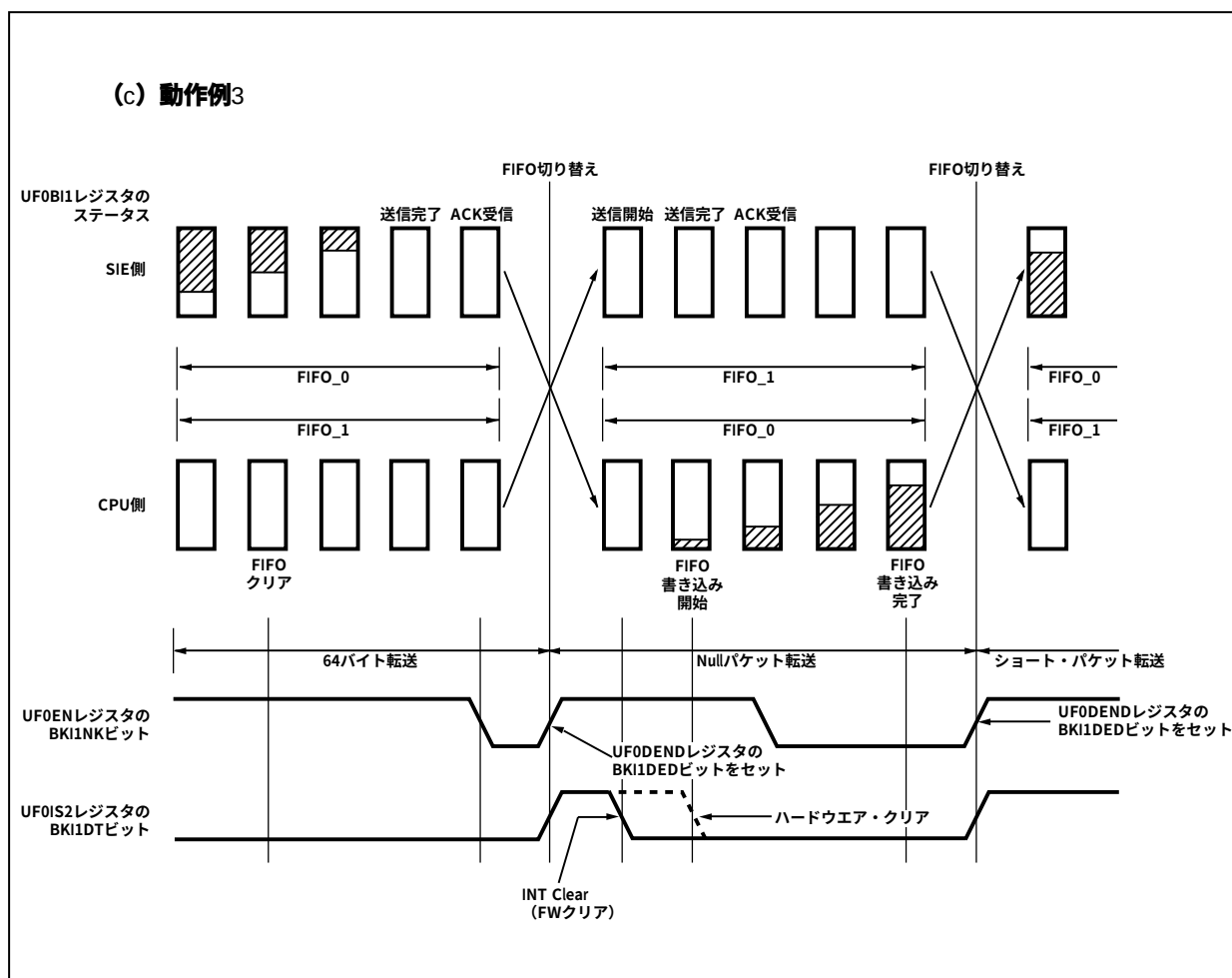
図20-9 UF0BI1レジスタの動作 (3/3)
