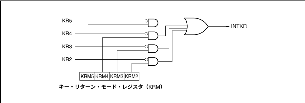
図23-1 キー・リターンのブロック図
