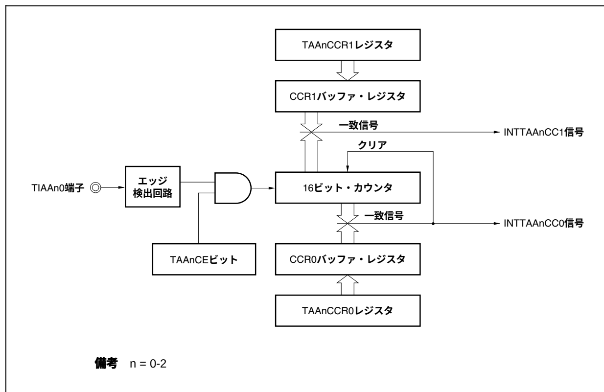
図6-18 TAAAnCCR1レジスタの構成図
