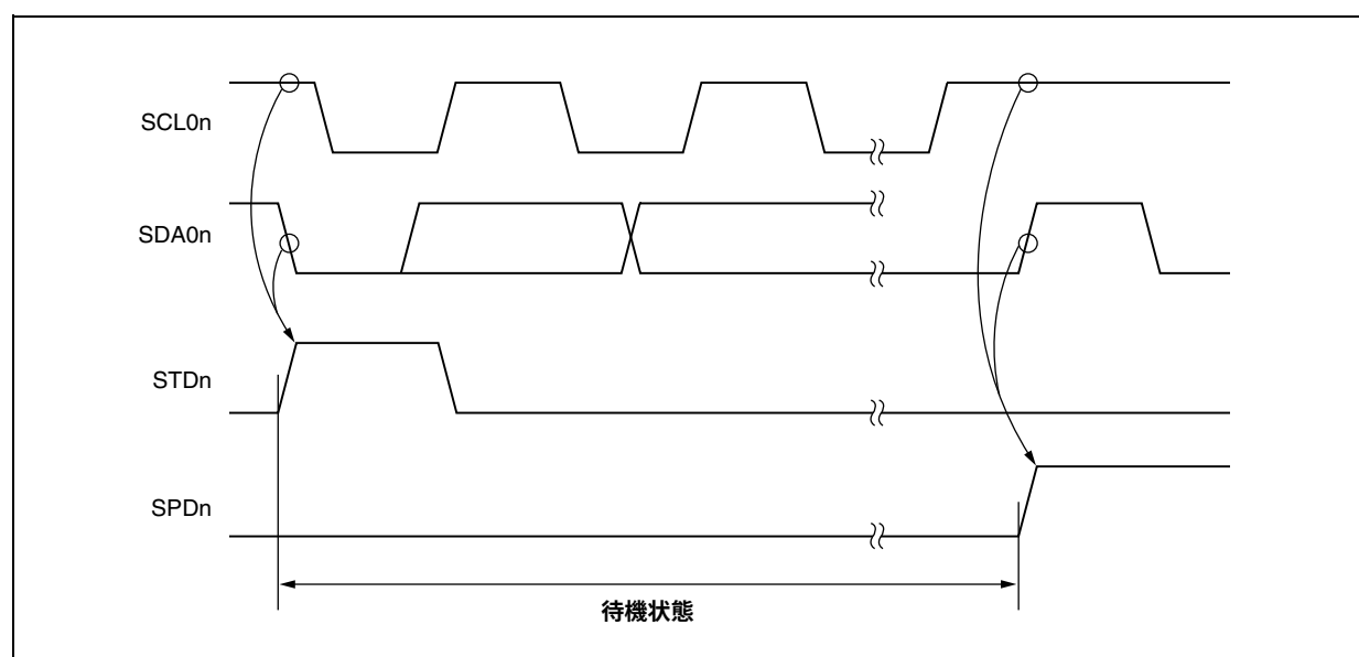
図18-16 通信予約受け付けタイミング
