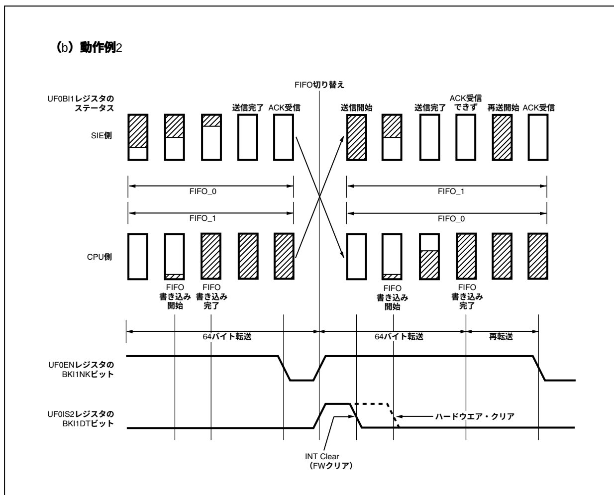
図20-9 UF0BI1レジスタの動作 (2/3)
