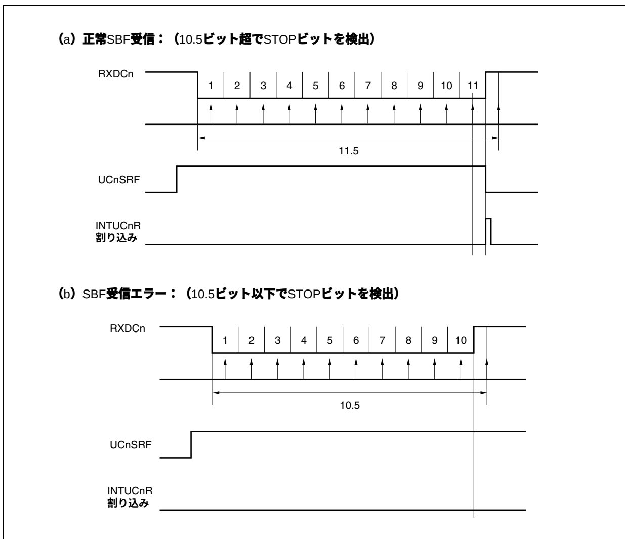
図16-10 SBF受信
