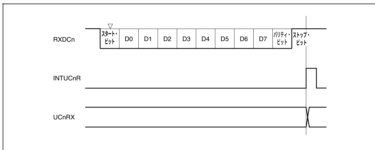
図16-14 UART受信
