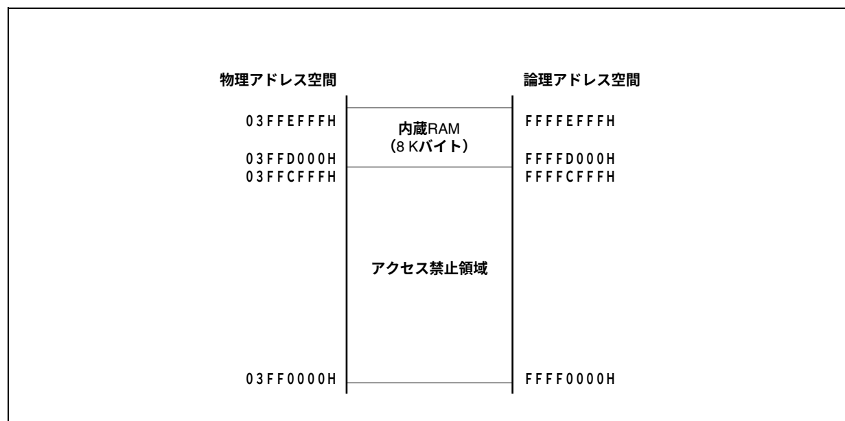
図3-9 内蔵RAM領域 (8 Kバイト)
