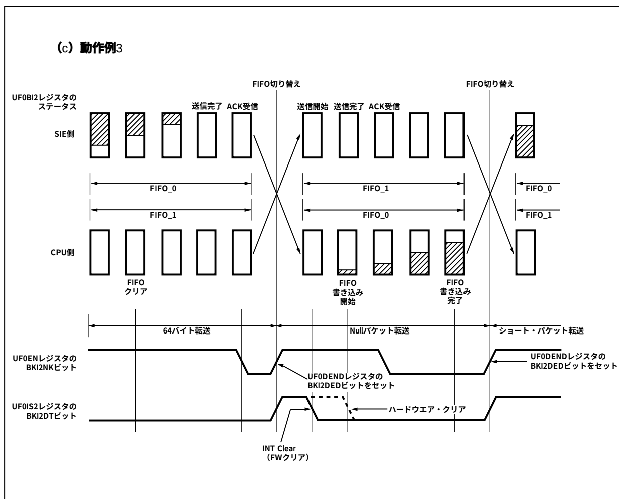
図20-10 UF0BI2レジスタの動作 (3/3)
