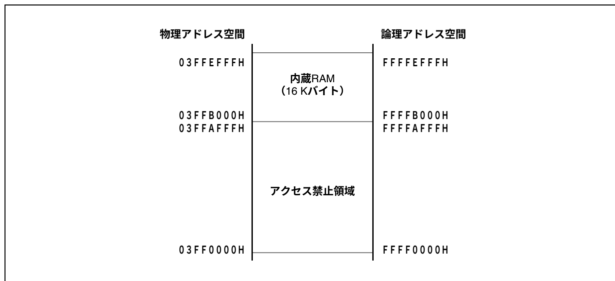
図3-10 内蔵RAM領域 (16 Kバイト)
