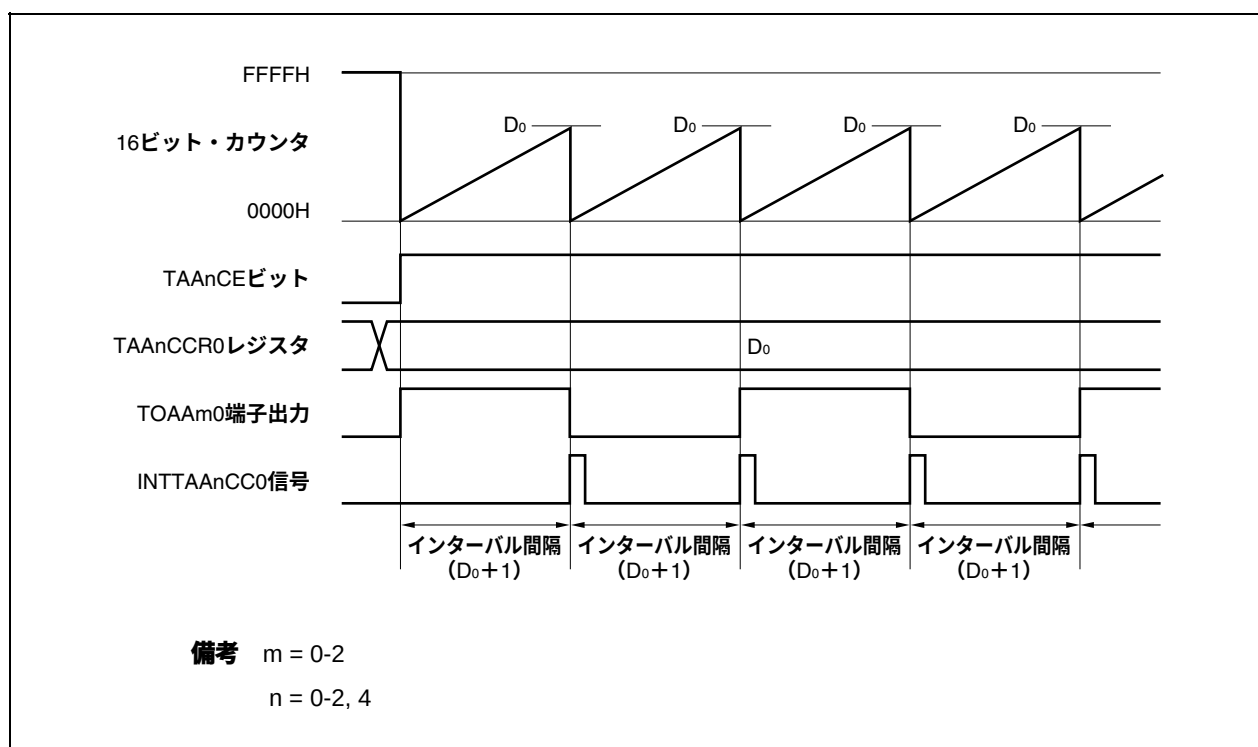
図6-8 インターバル・タイマ・モード動作の基本タイミング
