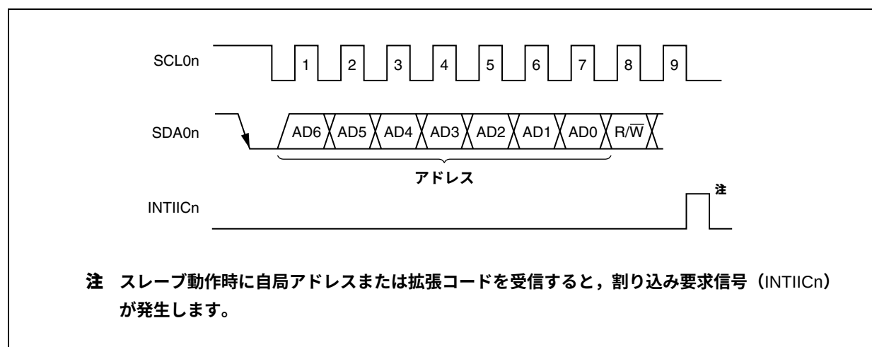
図18-9 アドレス
