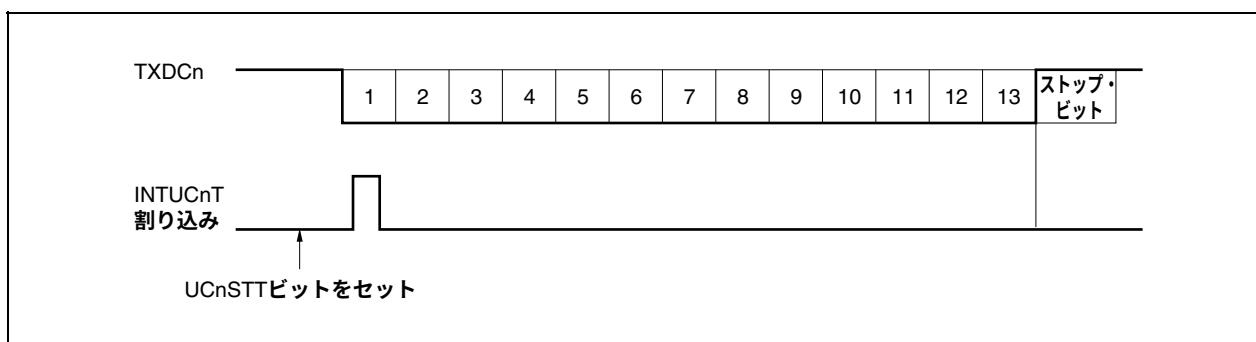
図16-9 SBF送信
