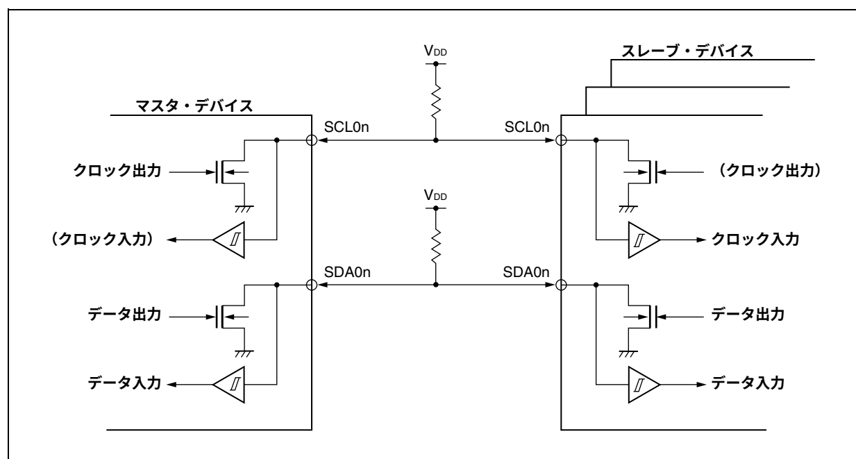
図18-6 端子構成図
