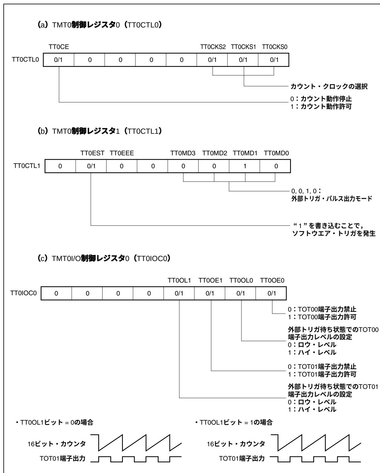
図8-23 外部トリガ・パルス出力モード動作時のレジスタ設定内容 (1/2)
