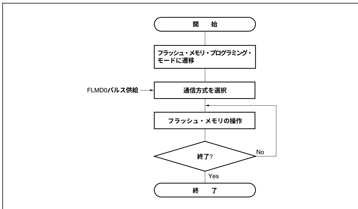
図30－9 フラッシュ・メモリの操作手順
