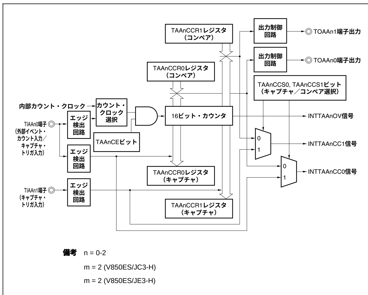
図6-33 フリー・ランニング・タイマ・モードの構成図
