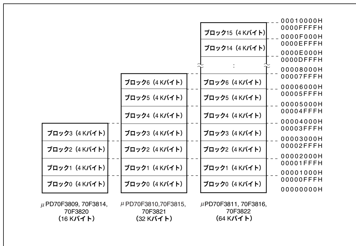
図30-1 フラッシュ・メモリ・マッピング (1/2)
