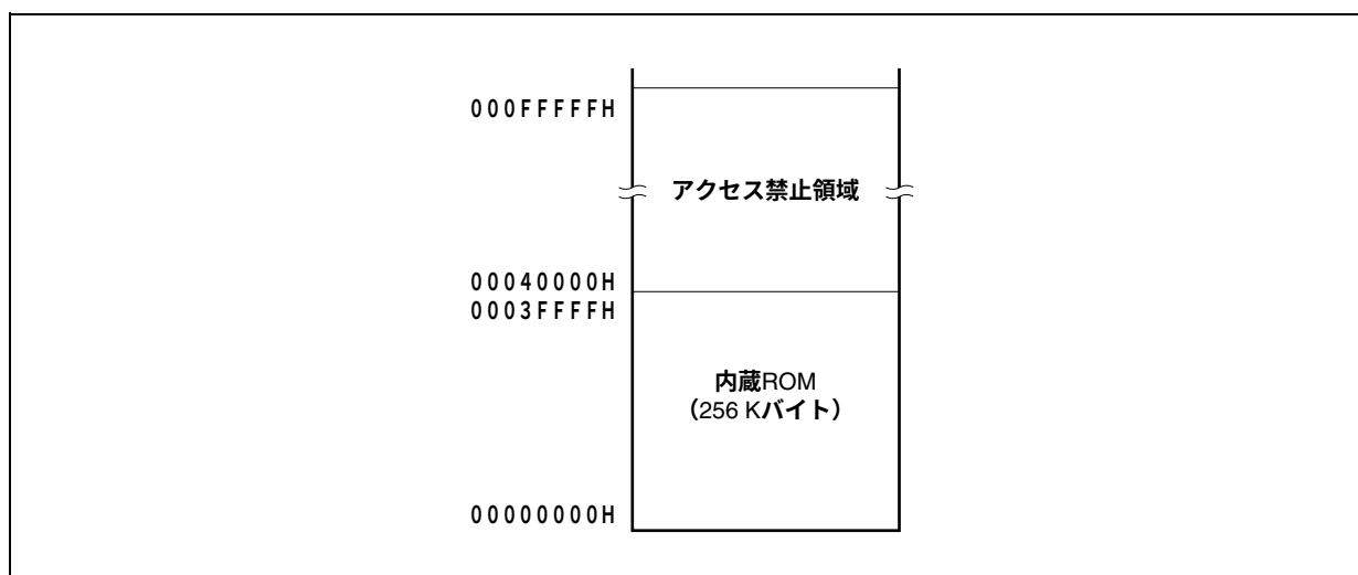
図3-8 内蔵ROM領域 (256 Kバイト)
