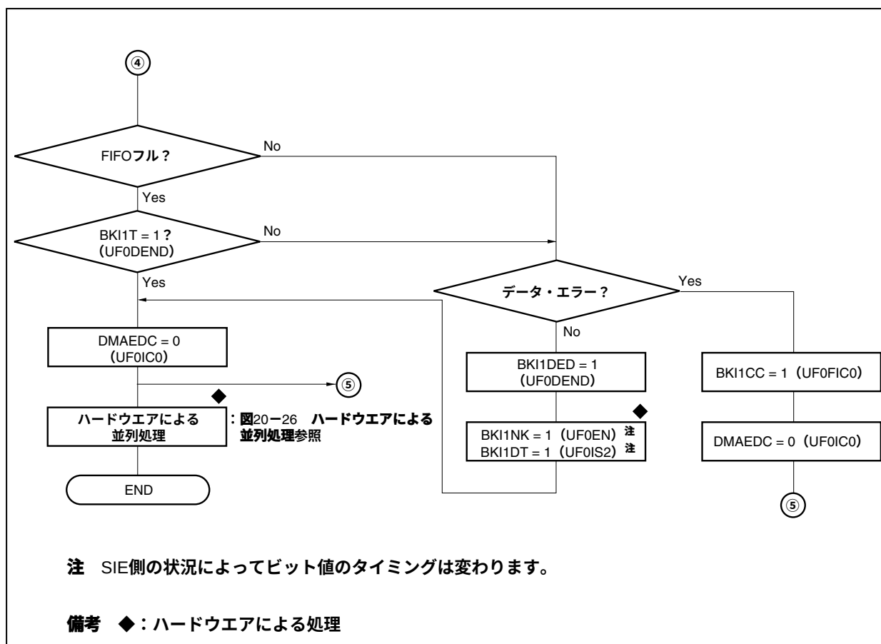
図20-33 バルク転送 (IN) によるDMA処理 (4/4)
