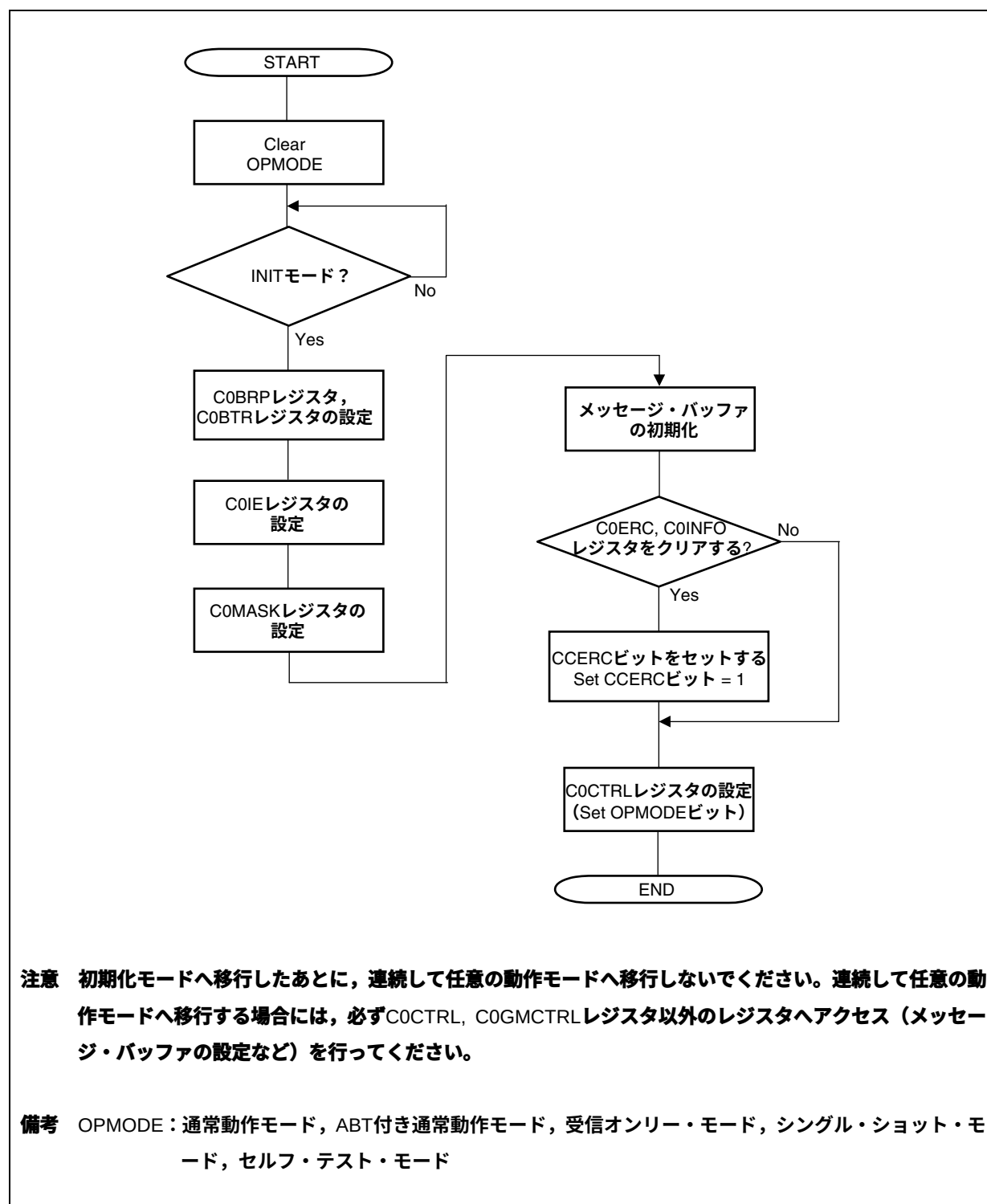
図19-37 再初期化
