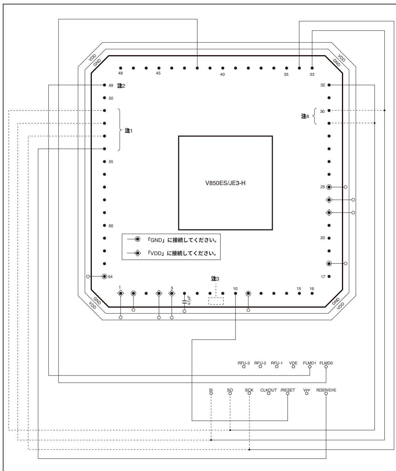
図30-8 V850ES/JE3-Hフラッシュ書き込み用アダプタの配線例 (CSIF0+HSモード時) (1/2)
