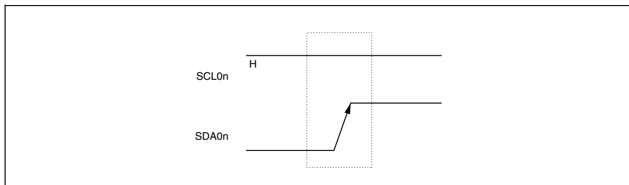
図18-12 ストップ・コンディション
