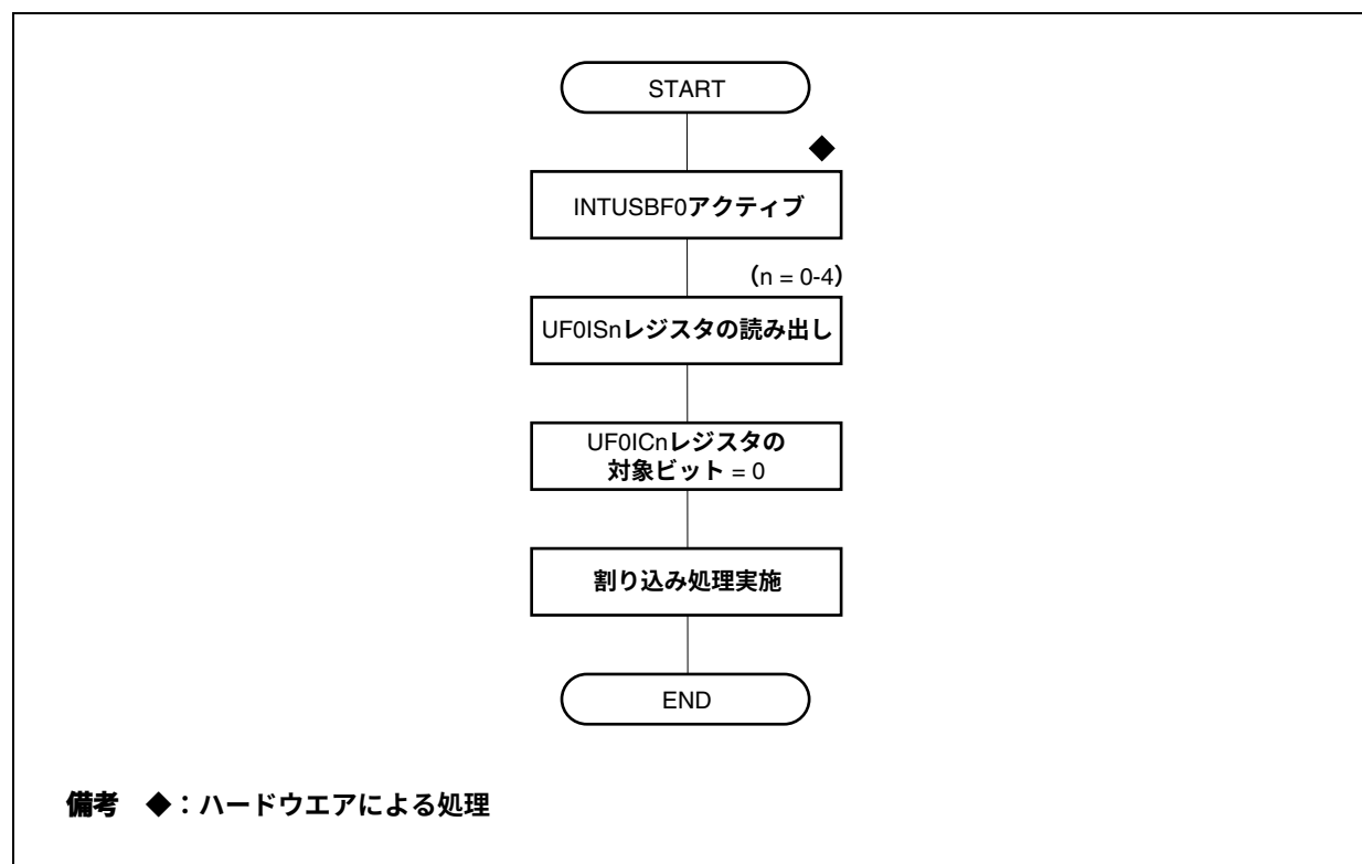
図20-18 割り込み処理
