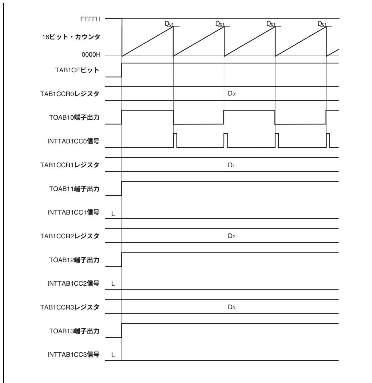
図7-8 D_{01} < D_{k1} の場合のタイミング図
