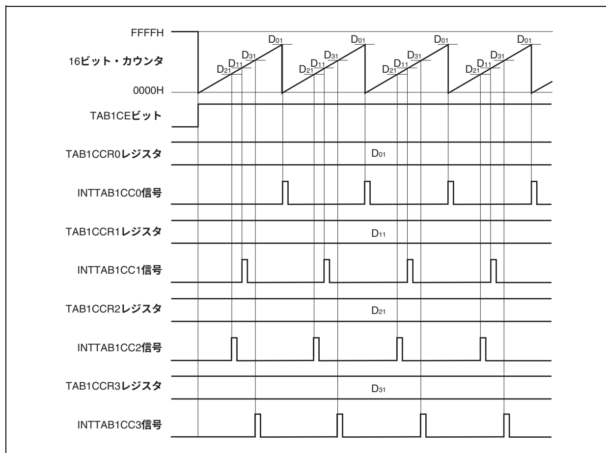
図7-14 D_{01} \geq D_{k1} の場合のタイミング図
