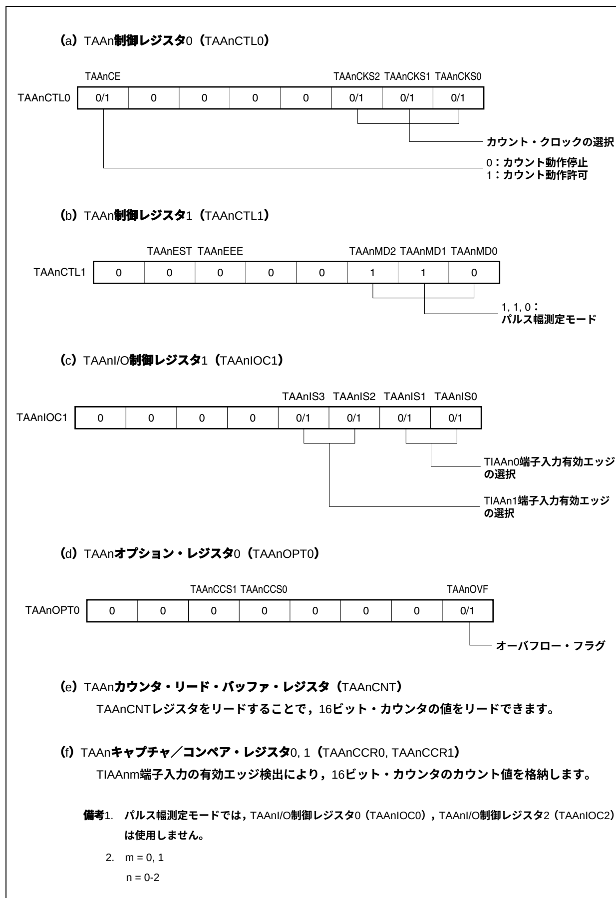
図6-41 パルス幅測定モード動作時のレジスタ設定内容
