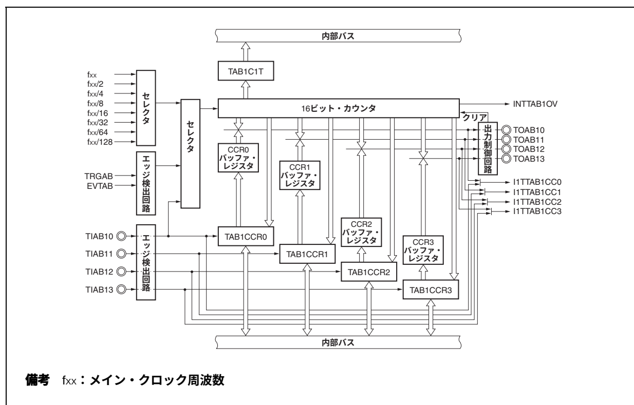
図7-1 TAB1のブロック図
