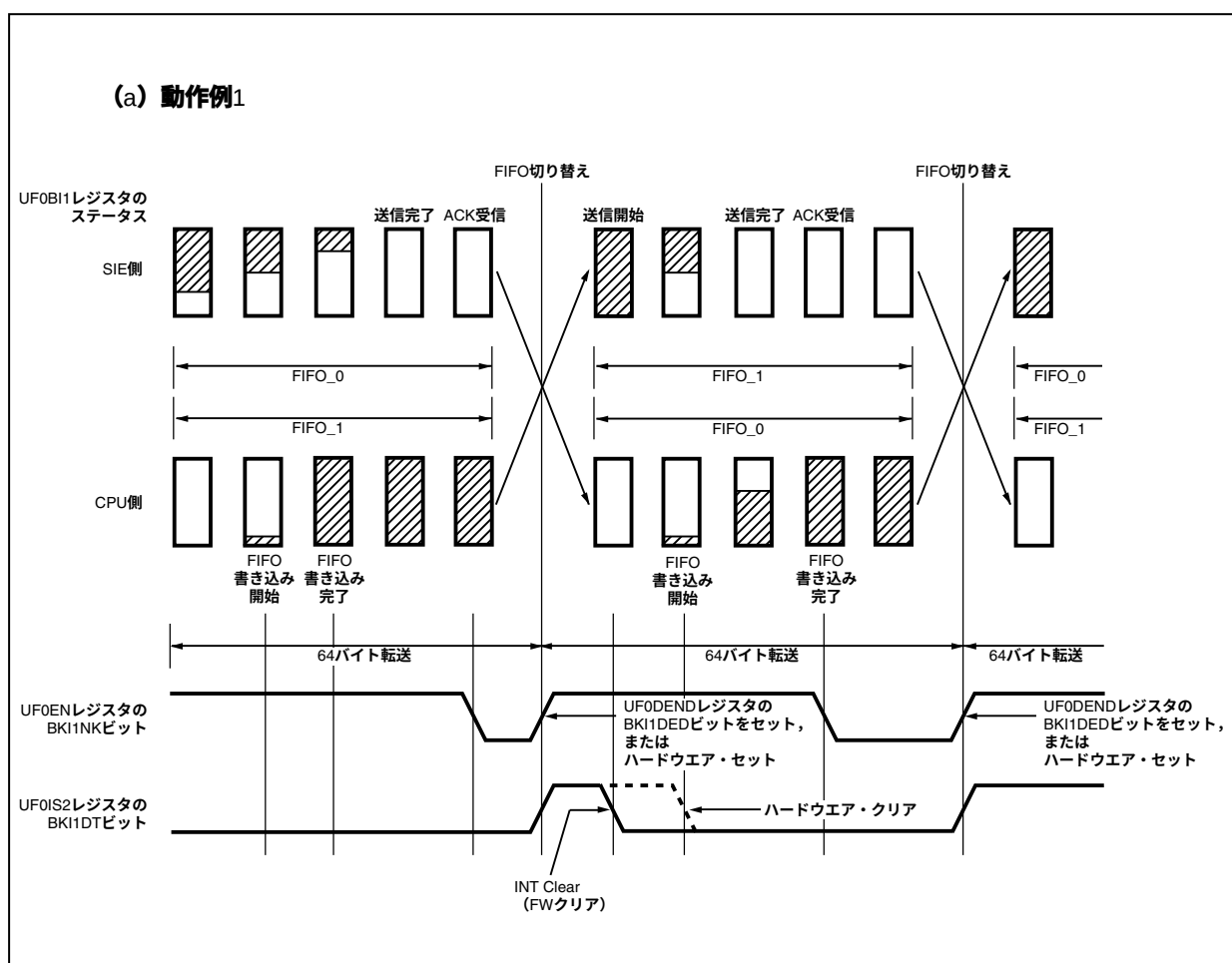
図20-9 UF0BI1レジスタの動作 (1/3)
