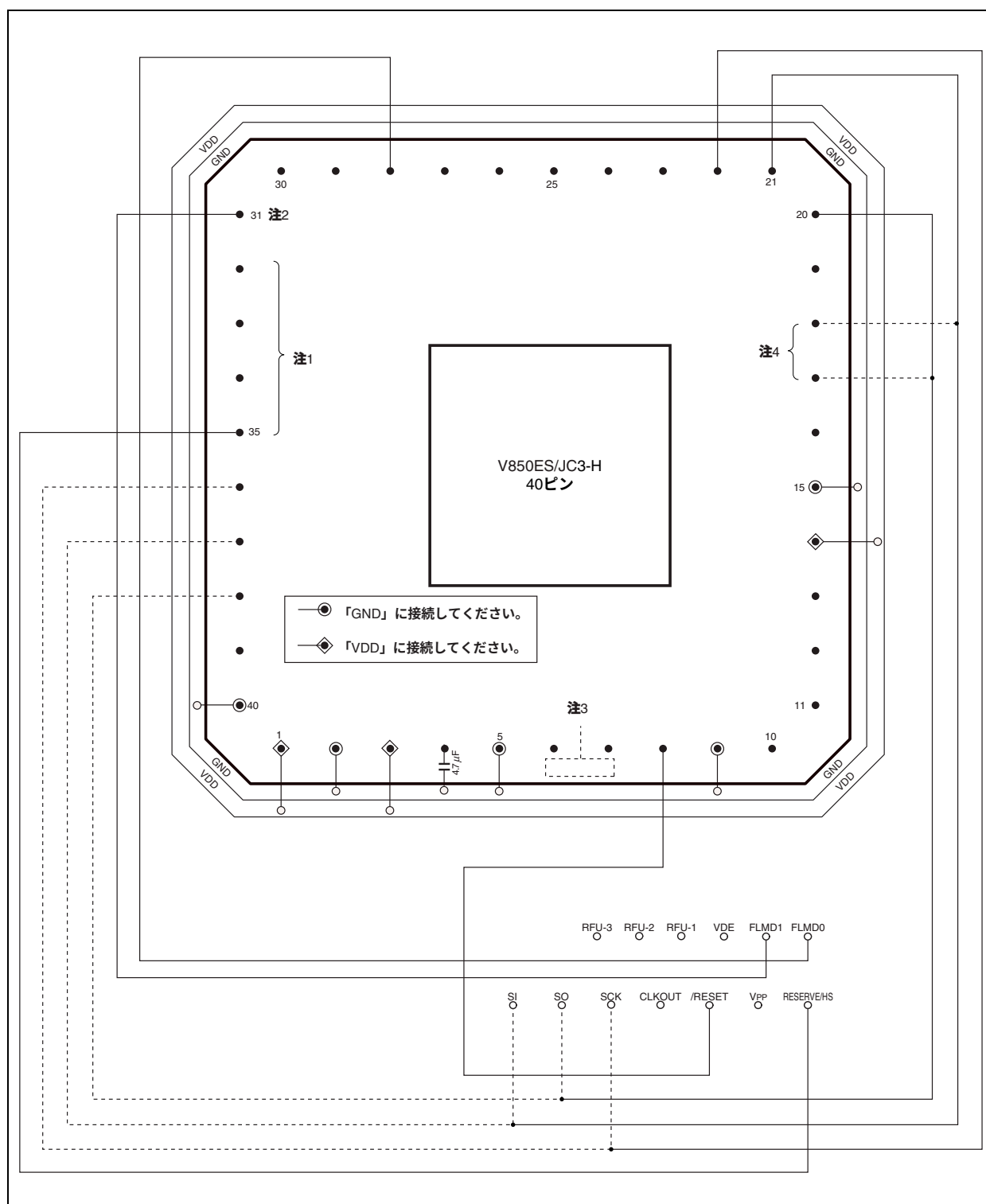
図30-6 V850ES/JC3-H (40ピン) フラッシュ書き込み用アダプタの配線例 (CSIF0+HSモード時) (1/2)
