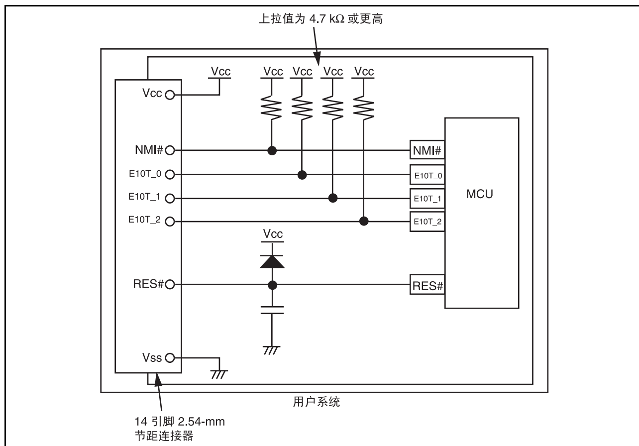
图 4.1 仿真器连接示例
