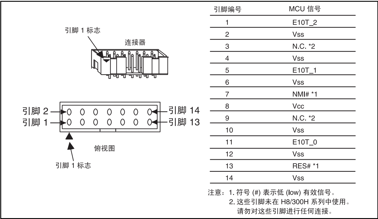
图 3.1 连接器的引脚分配
