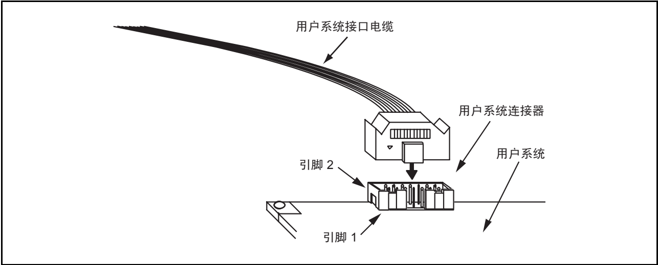
图 2.1 将用户系统接口电缆连接到用户系统
