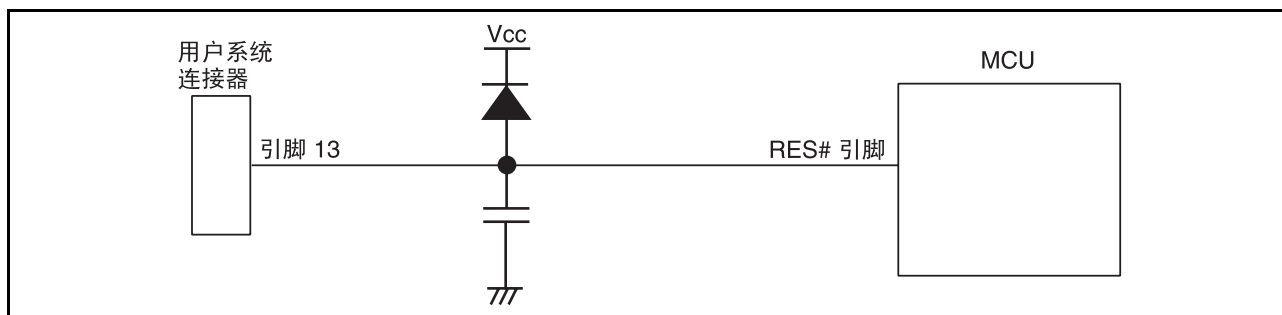
图 4.4 复位电路示例
