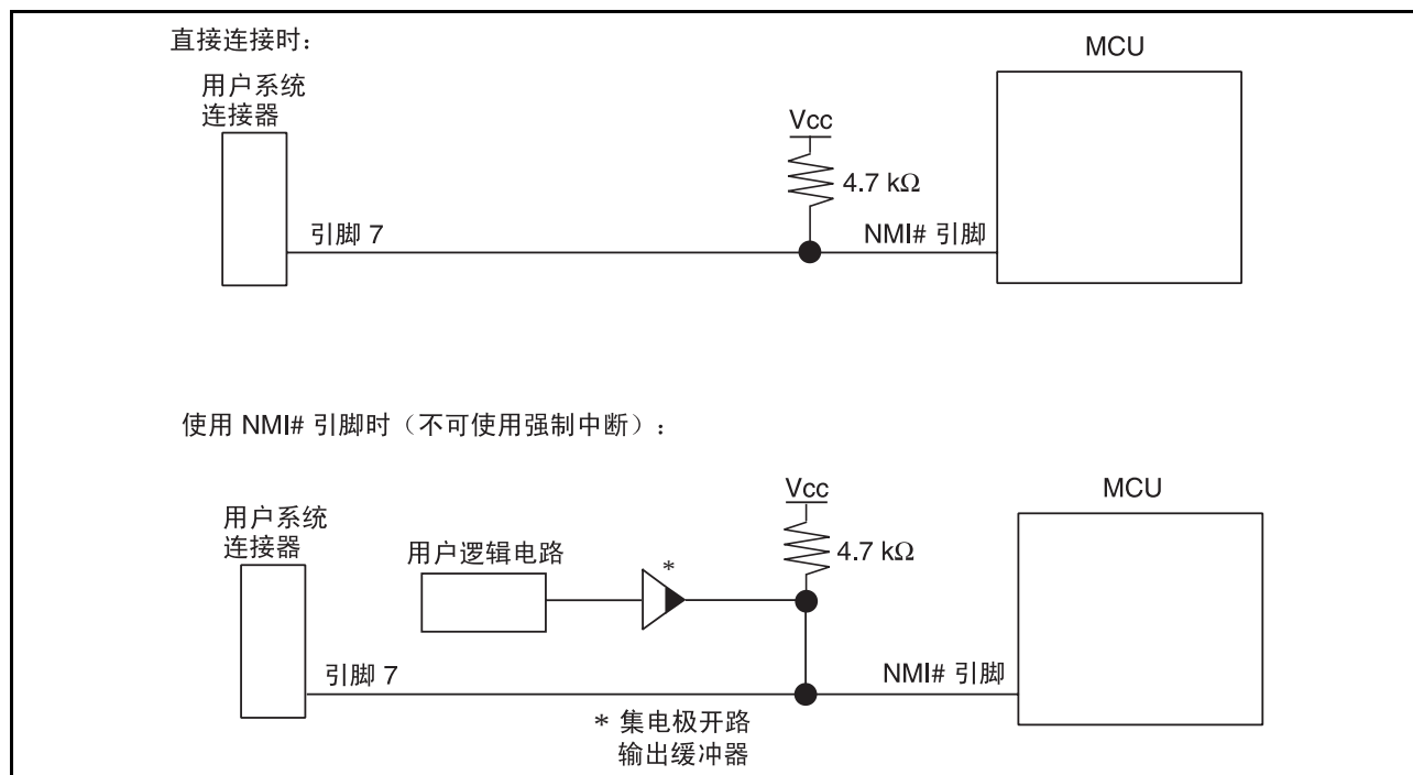
图 4.3 仿真器和 NMI# 引脚的连接
