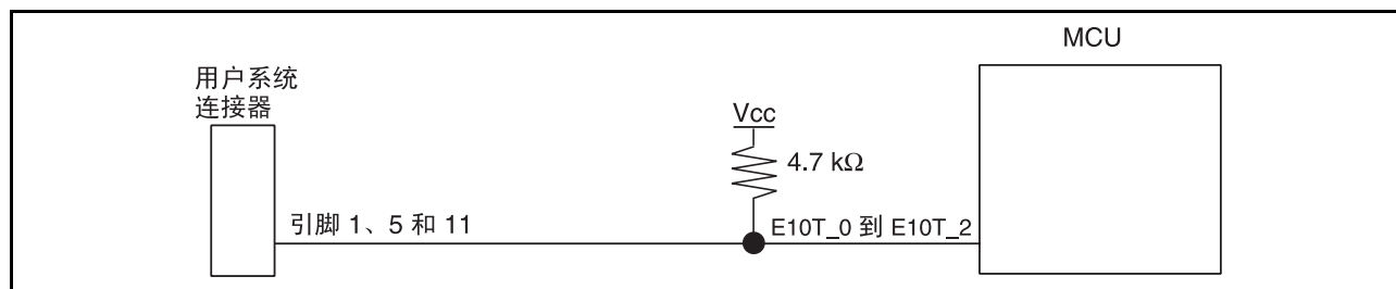
图 4.2 仿真器和 E10T_0 到 E10T_2 引脚的连接
