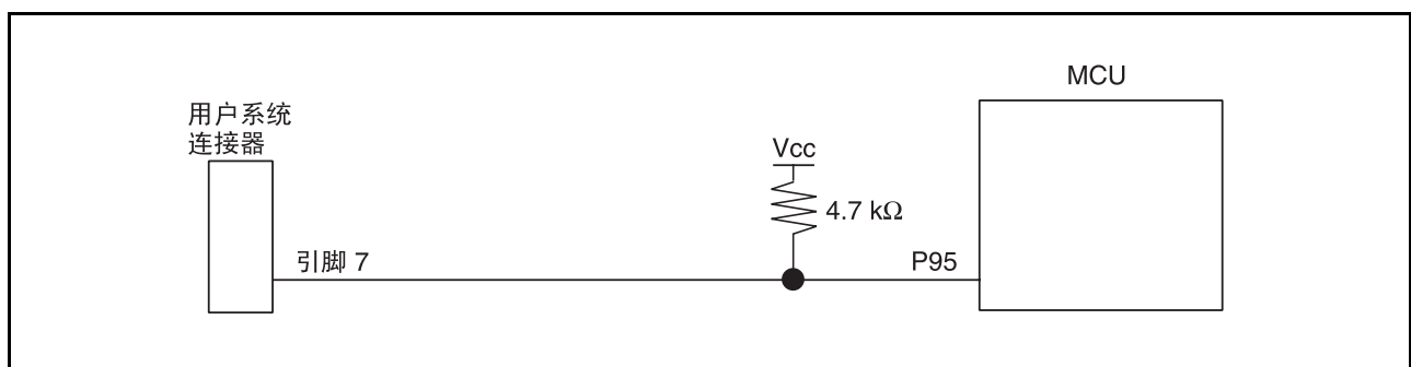
图 4.3 仿真器和 P95 引脚的连接
