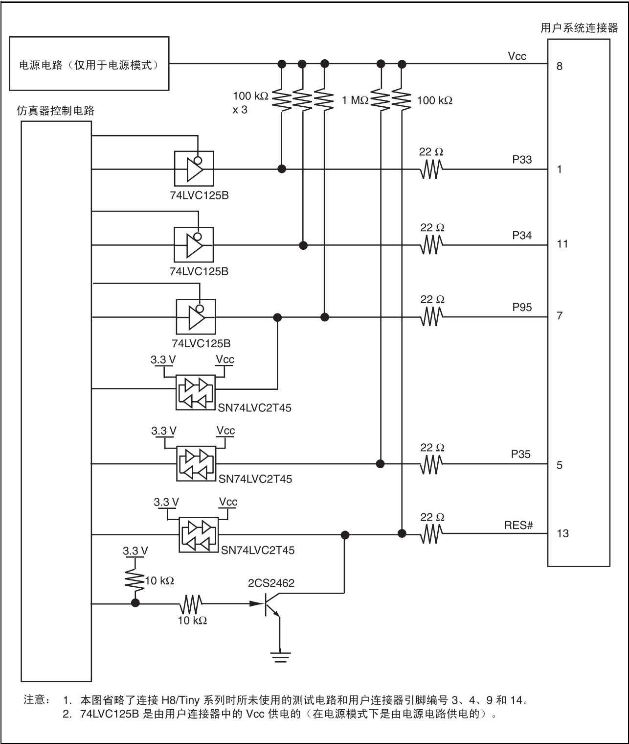
图 4.6 E8a 仿真器中的接口电路（参考）
