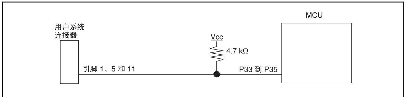
图 4.2 仿真器和 P33 到 P35 引脚的连接
