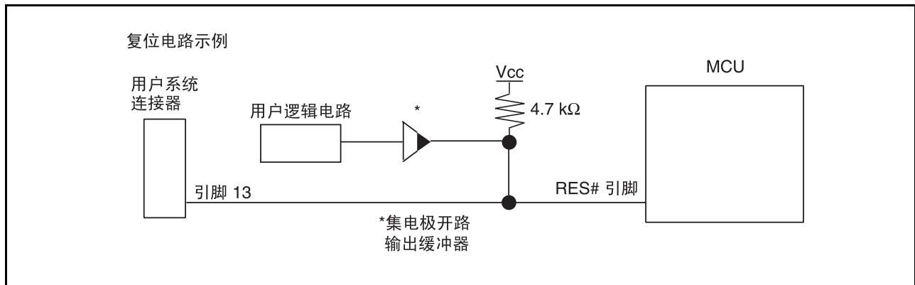
图 4.4 复位电路示例
