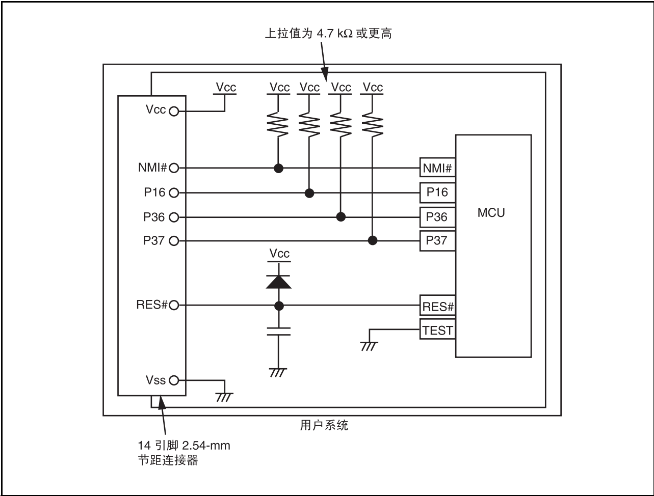
图 4.1 仿真器连接示例
