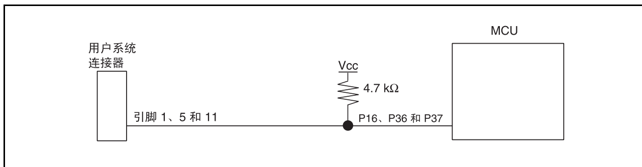
图 4.2 仿真器与 P16、P36 和 P37 引脚的连接
