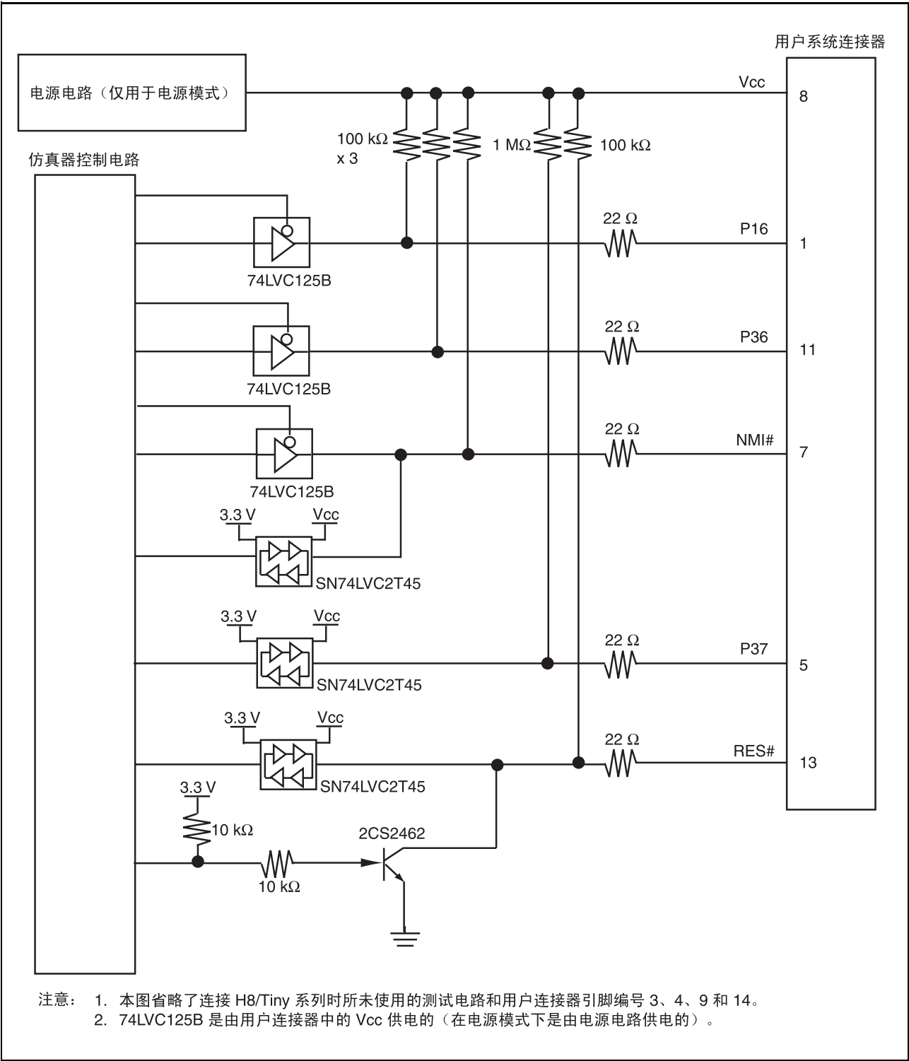
图 4.7 E8a 仿真器中的接口电路（参考）
