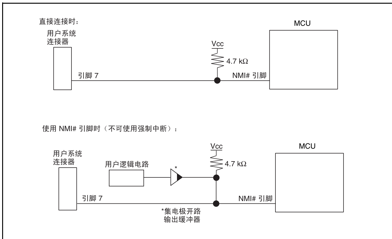
图 4.3 仿真器和 NMI# 引脚的连接
