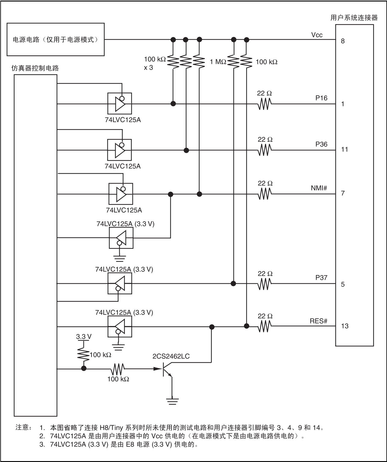
图 4.6 E8 仿真器中的接口电路（参考）
