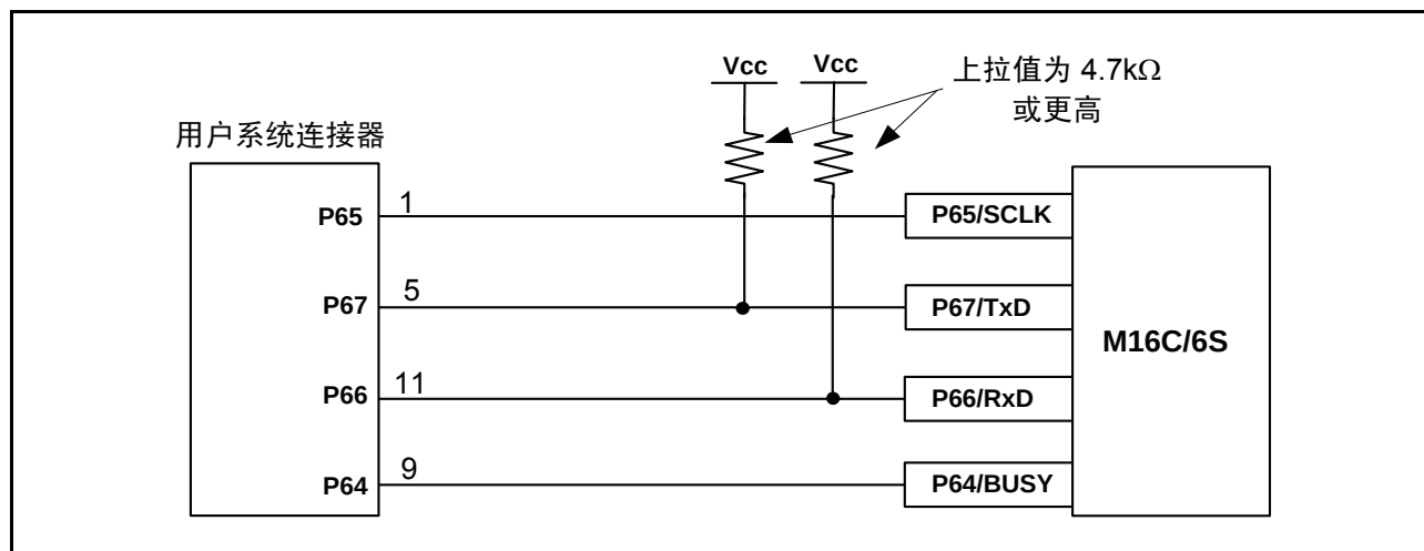
图 5.2 E8a 仿真器和 MCU 连接
