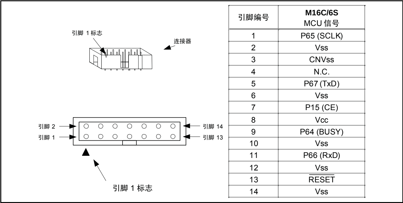
图 4.1 E8a 连接器引脚分配
