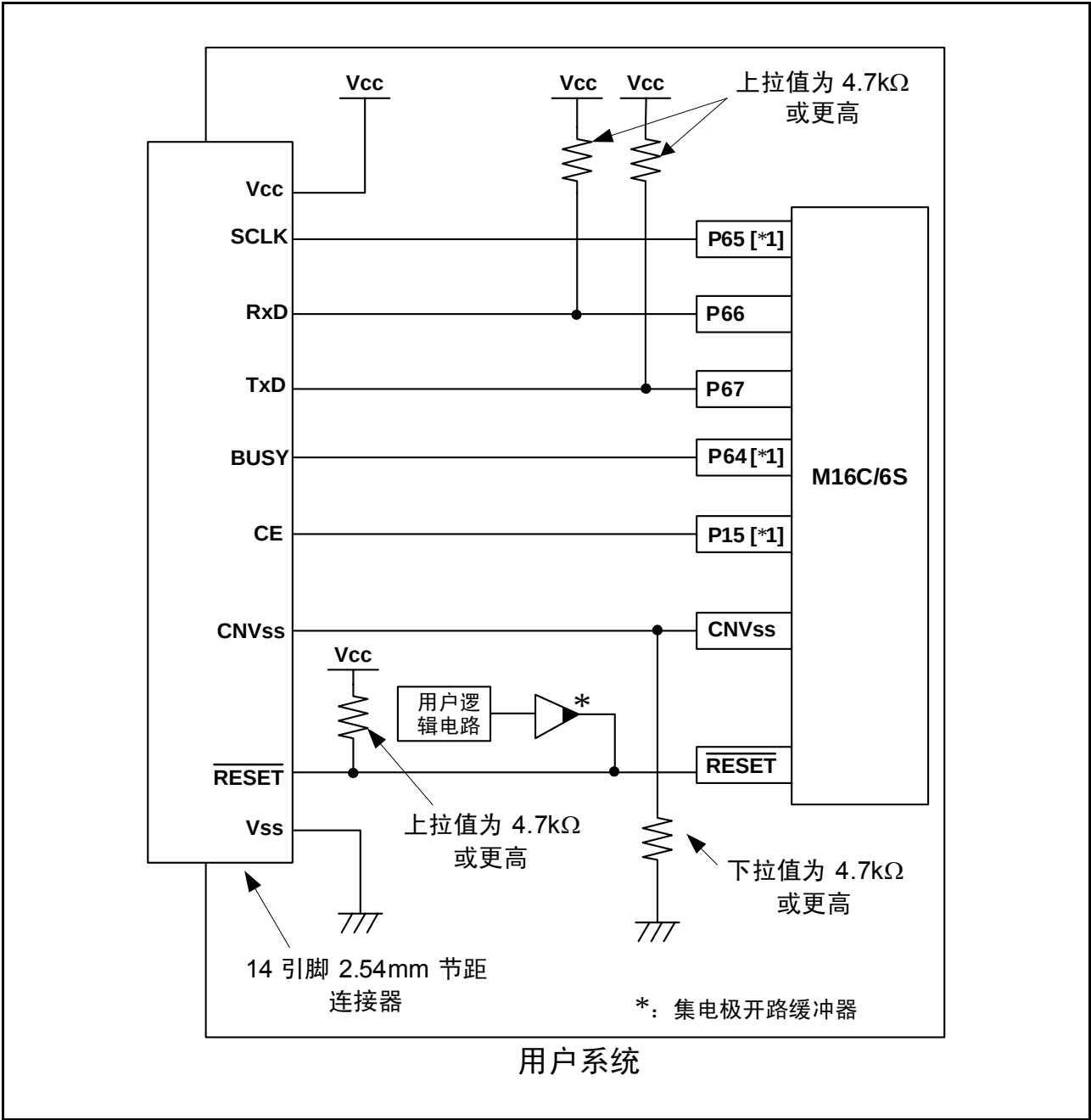
图 5.1 E8a 连接示例
