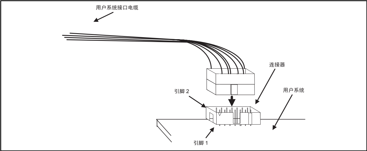
图 3.1 将用户系统接口电缆连接到 E8a 连接器
