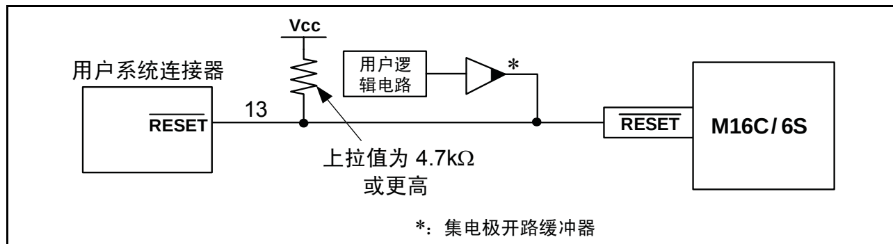
图 5.5 复位电路示例
