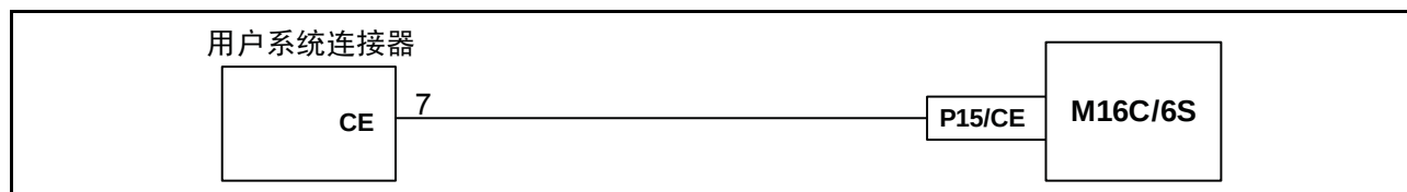
图 5.3 E8a 仿真器与 P15 引脚的连接
