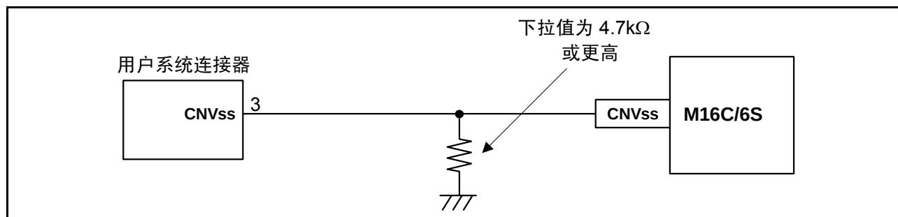
图 5.4 E8a 仿真器和 CNVss 引脚的连接
