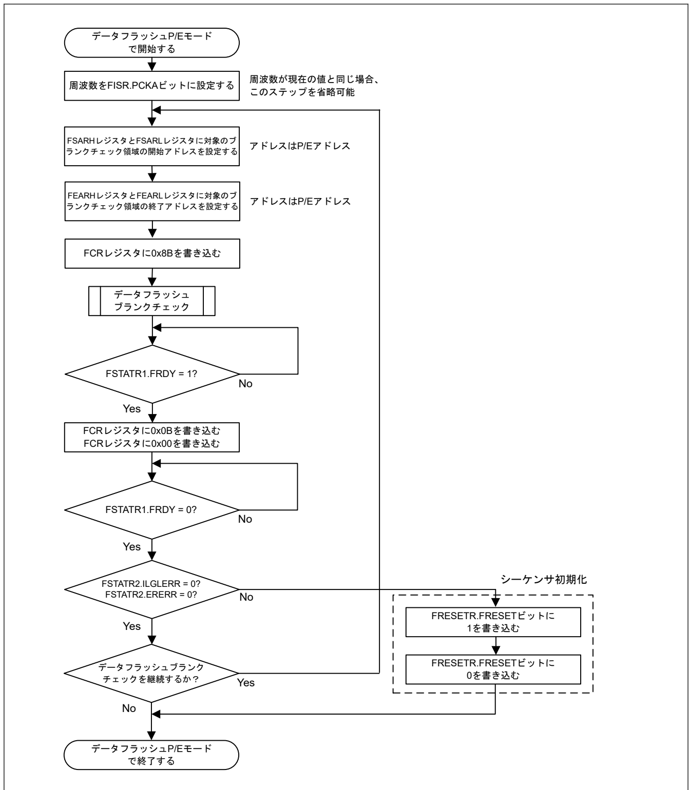
図 35.28 データフラッシュブランクチェック手順のフローチャート
