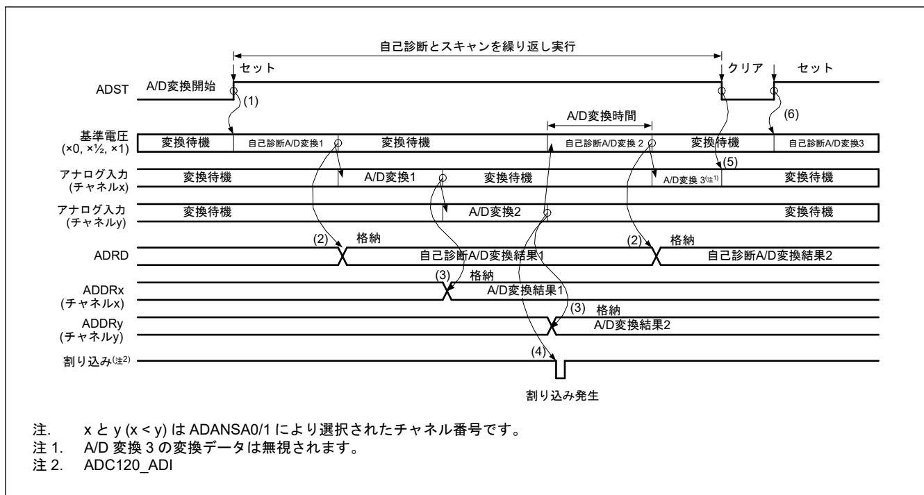
図 29.13 連続スキャンモードの基本動作例（アナログ入力（チャネル x、y）選択+自己診断）
