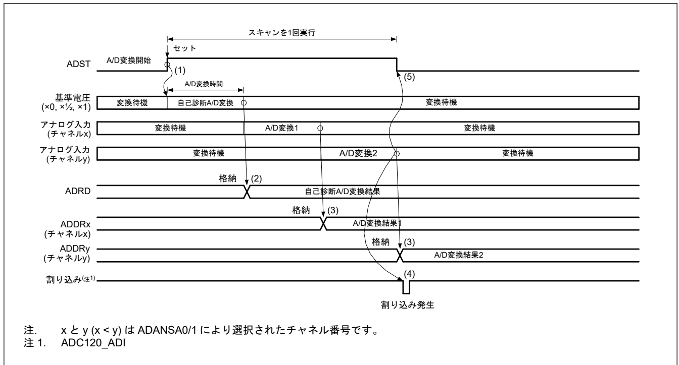
図 29.8 シングルスキャンモードの基本動作例（アナログ入力（チャネル x と y）選択+自己診断）
