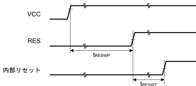
図 39.7 電源投入時リセット入力タイミング
