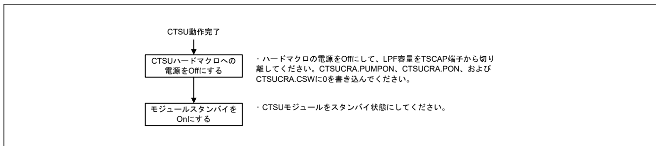
図 32.9 CTSU 停止のフロー
