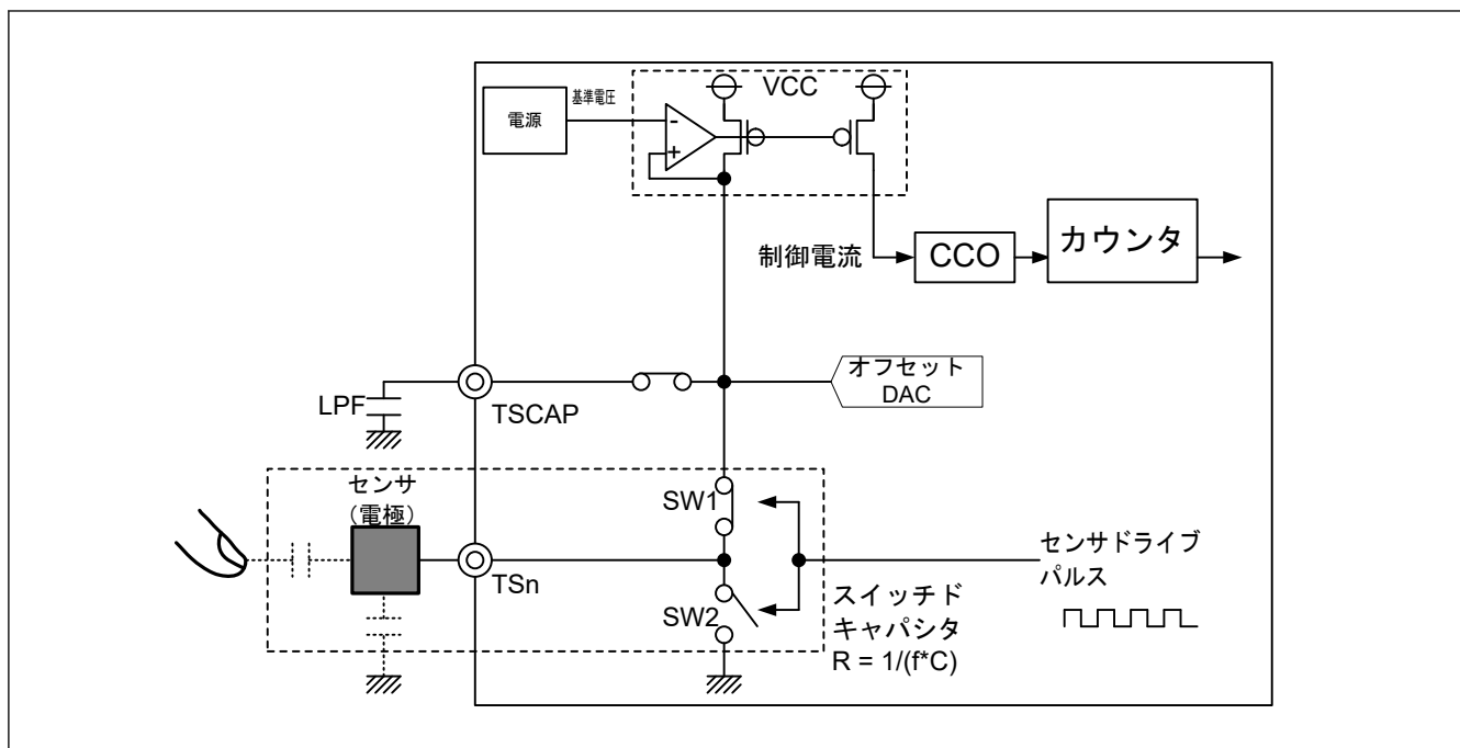
図 32.4 自己容量方式計測部回路
