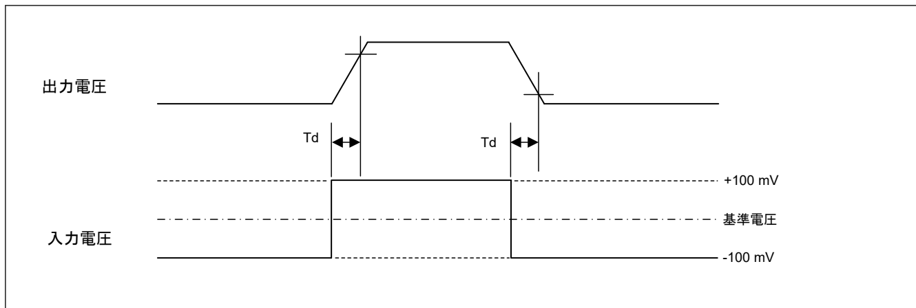
図 39.47 出力遅延時間
