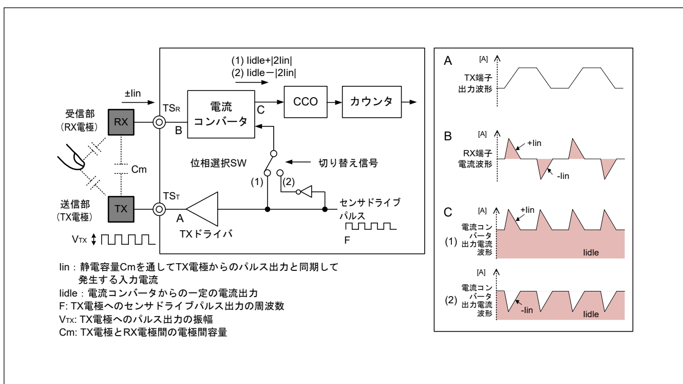
図 32.14 高速計測のための計測部回路
