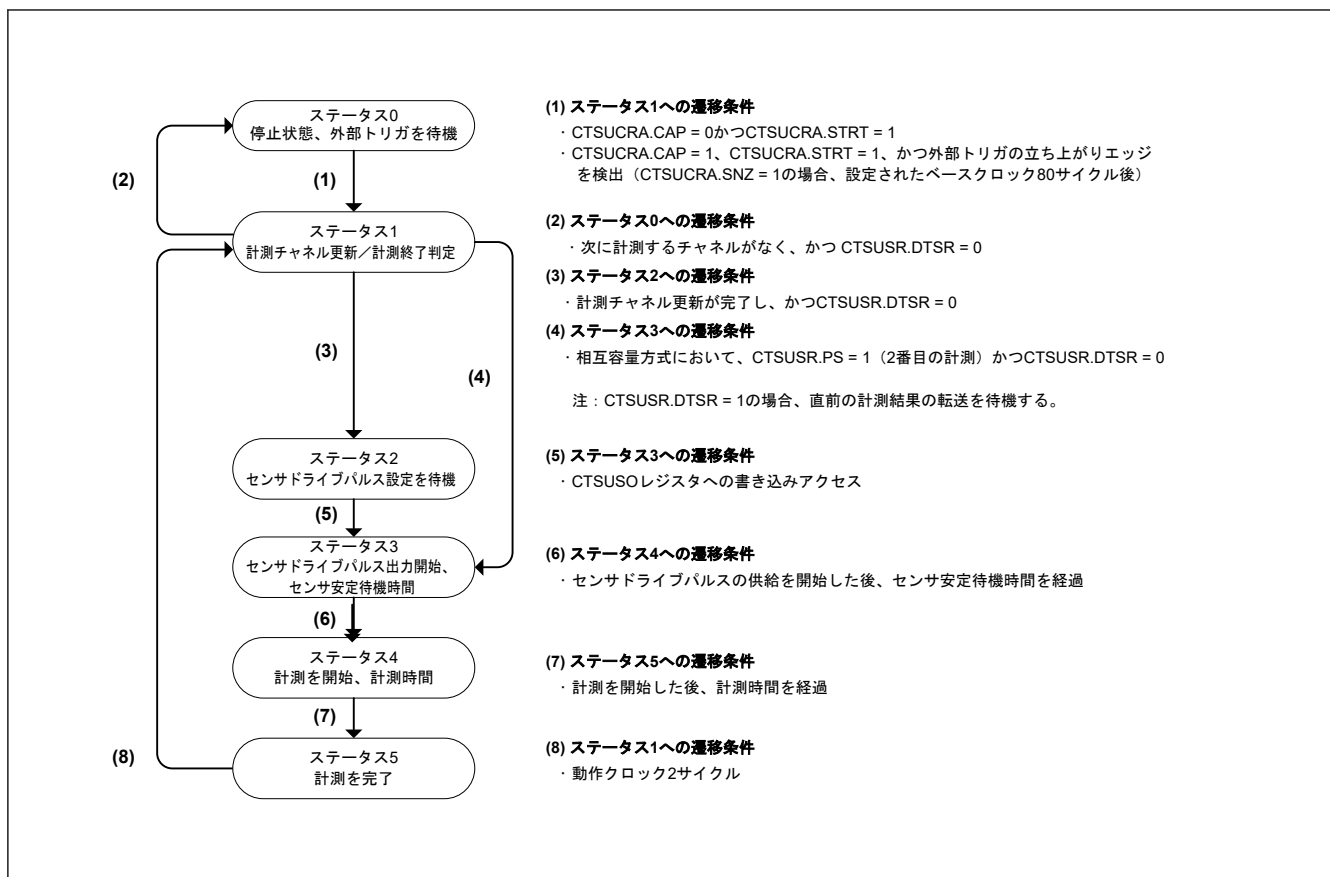
図 32.10 ステータス動作遷移図
