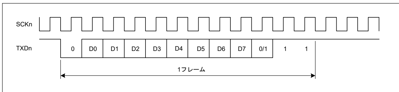
図 25.4 調歩同期式モードにおける出力クロックと送信データの位相関係 (SEMR.CHR = 0、PE = 1、MP = 0、および STOP = 1 の場合)
