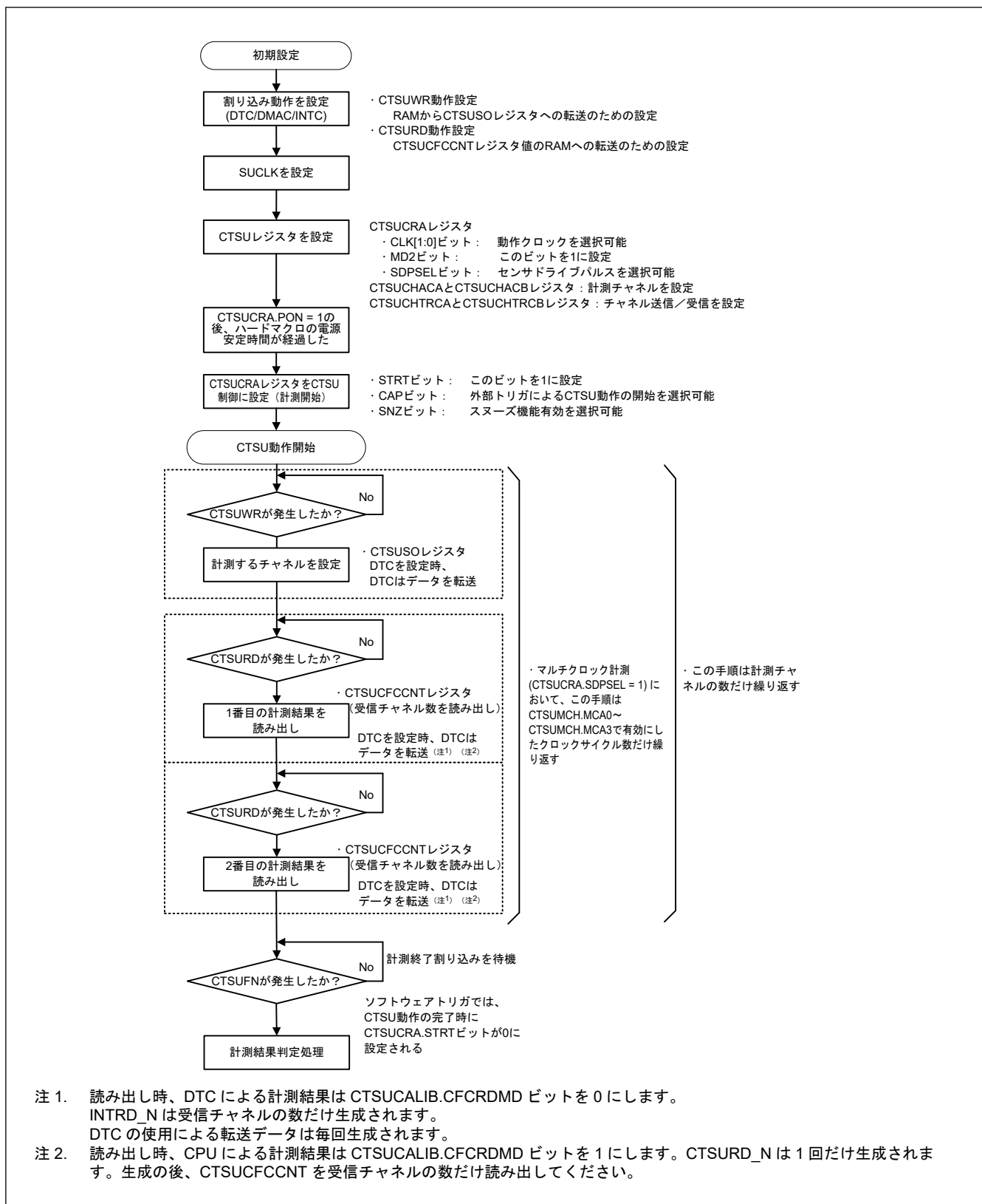
図 32.15 高速計測方式のソフトウェアフローと動作例
