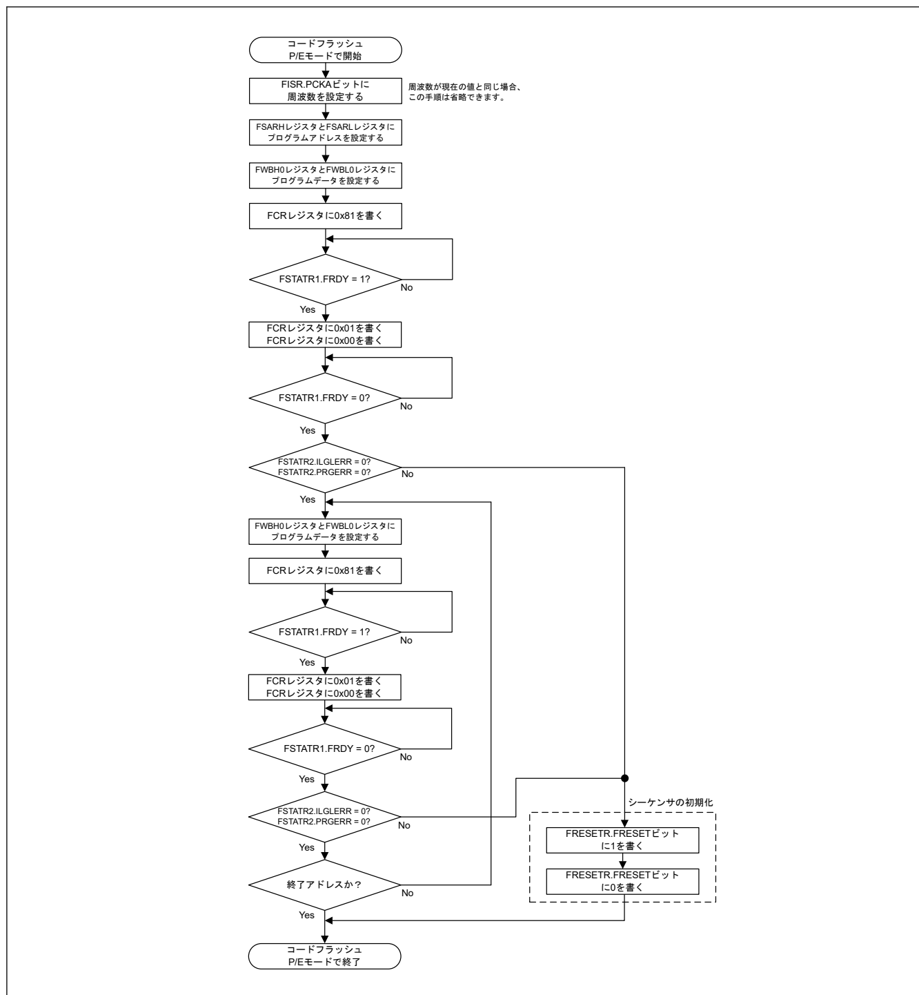
図 35.21 コードフラッシュの連続プログラム時のフローチャート
