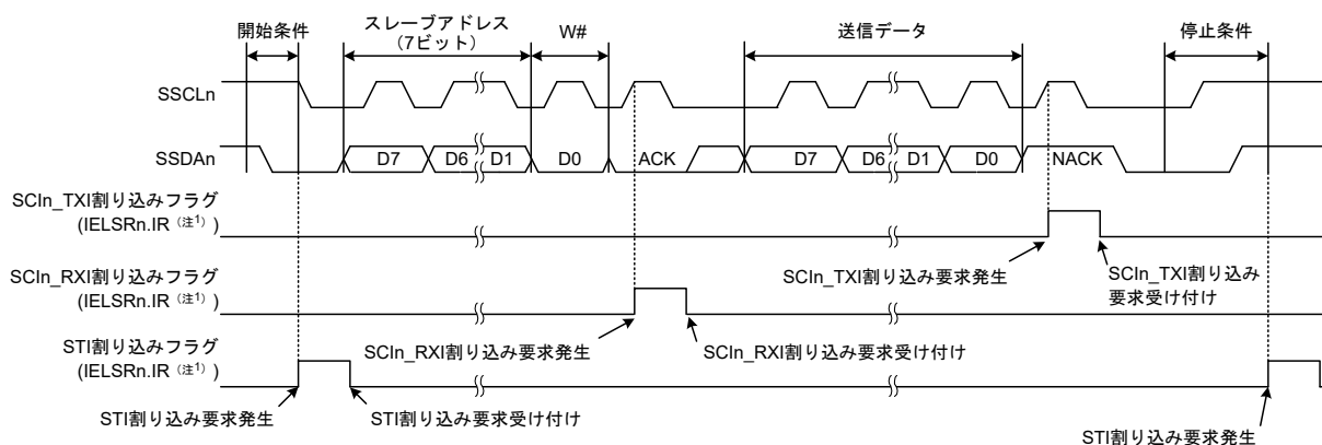
図 25.64 簡易 IIC モードにおけるマスタ送信の動作例 2(7 ビットスレーブアドレス、ACK 割り込み、および NACK 割り込み使用時)
