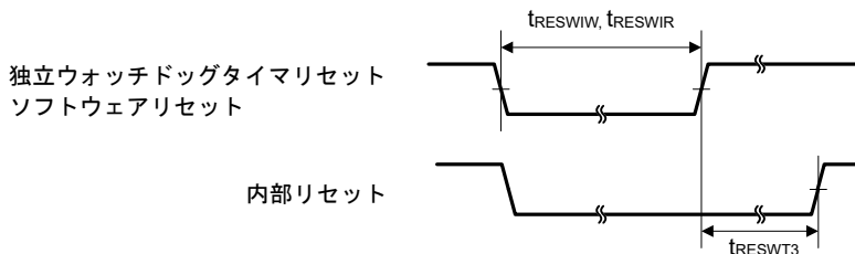
図 39.9 リセット入力タイミング (2)
