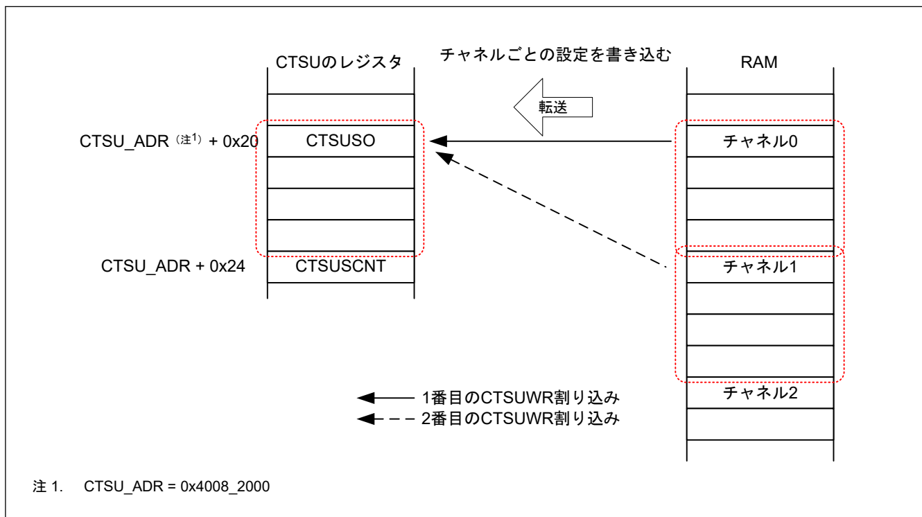
図 32.16 CTSUWR 割り込みを用いた DTC 転送動作例
