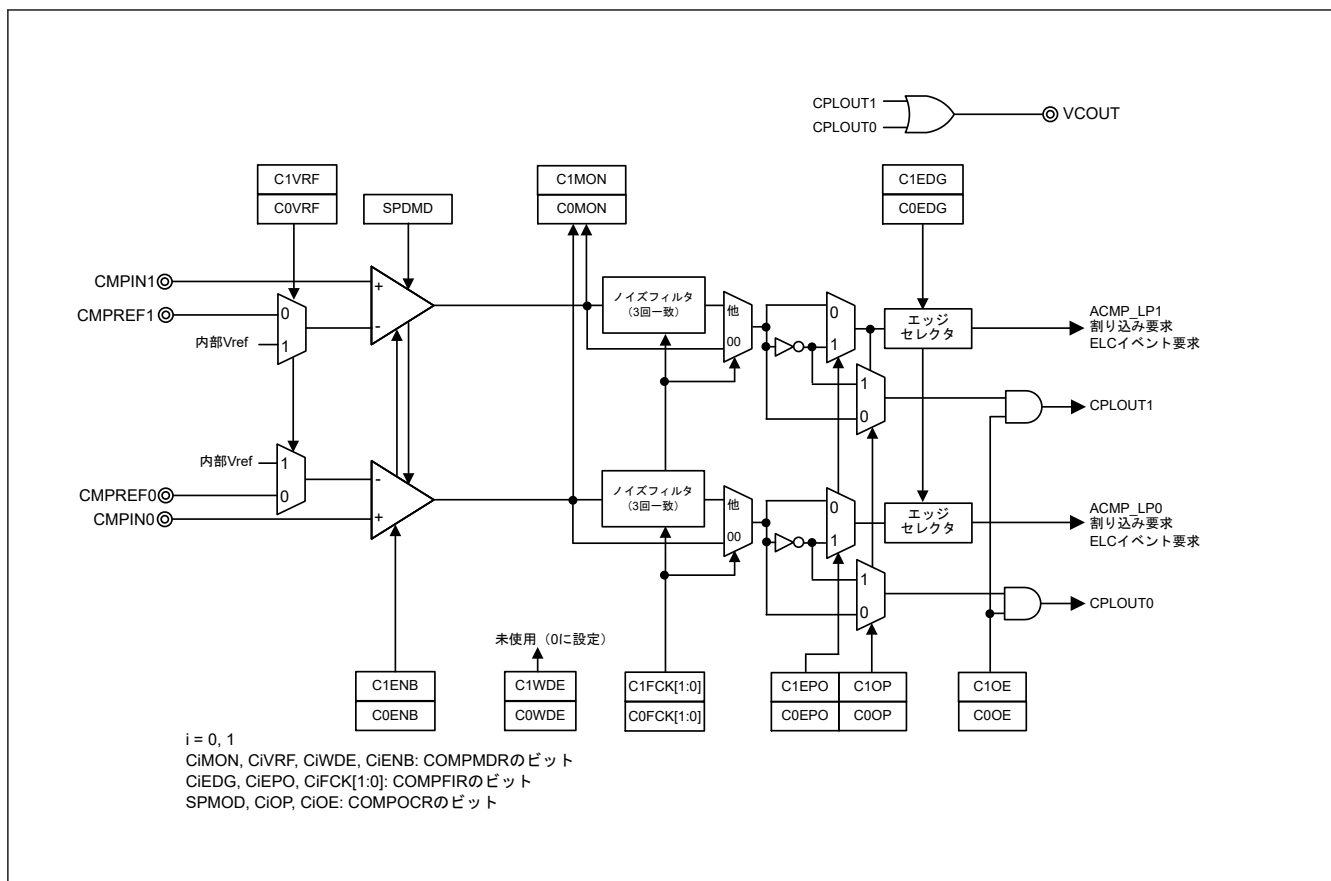
図 31.1 ウィンドウ機能無効時の ACMPLP ブロック図
