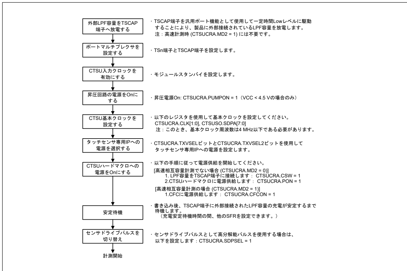
図 32.8 CTSU の初期設定フロー
