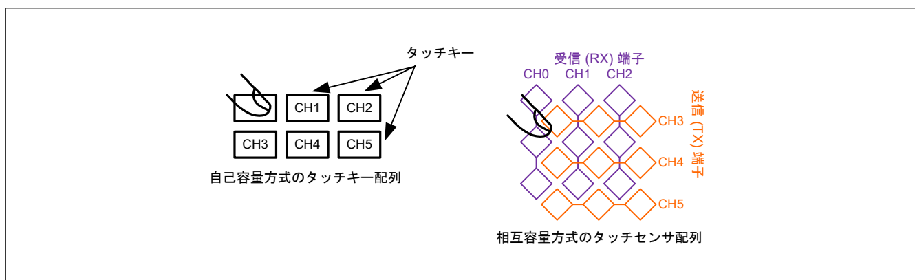
図 32.11 自己容量方式と相互容量方式の概要
