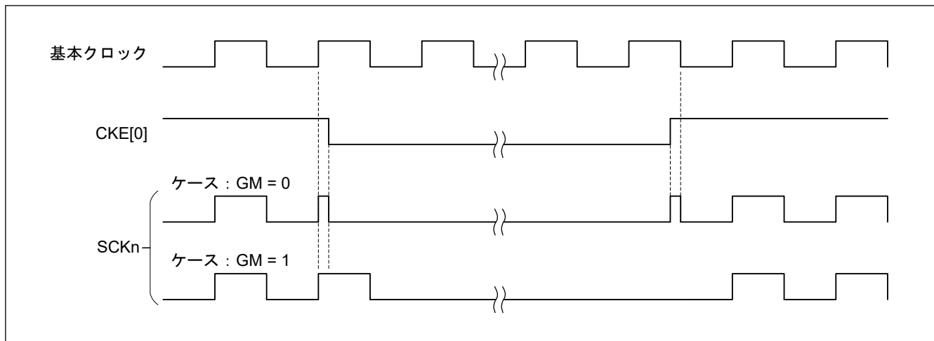
図 25.57 クロック出力タイミング
