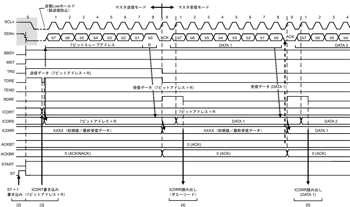
図 26.12 マスタ受信の動作タイミング (1) (7 ビットアドレスフォーマットで RDRFS = 0 の場合)
