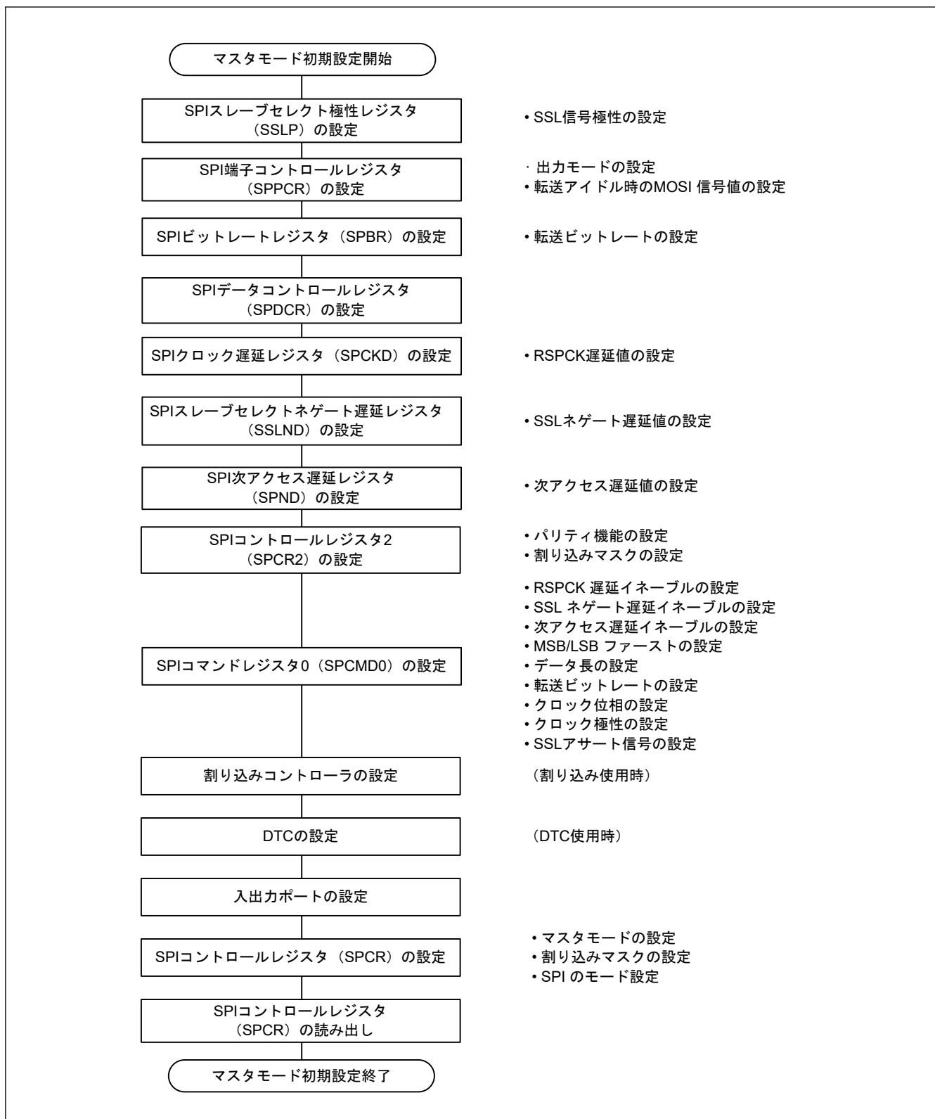
図 27.32 マスタモード時の SPI 動作の初期化フロー例
