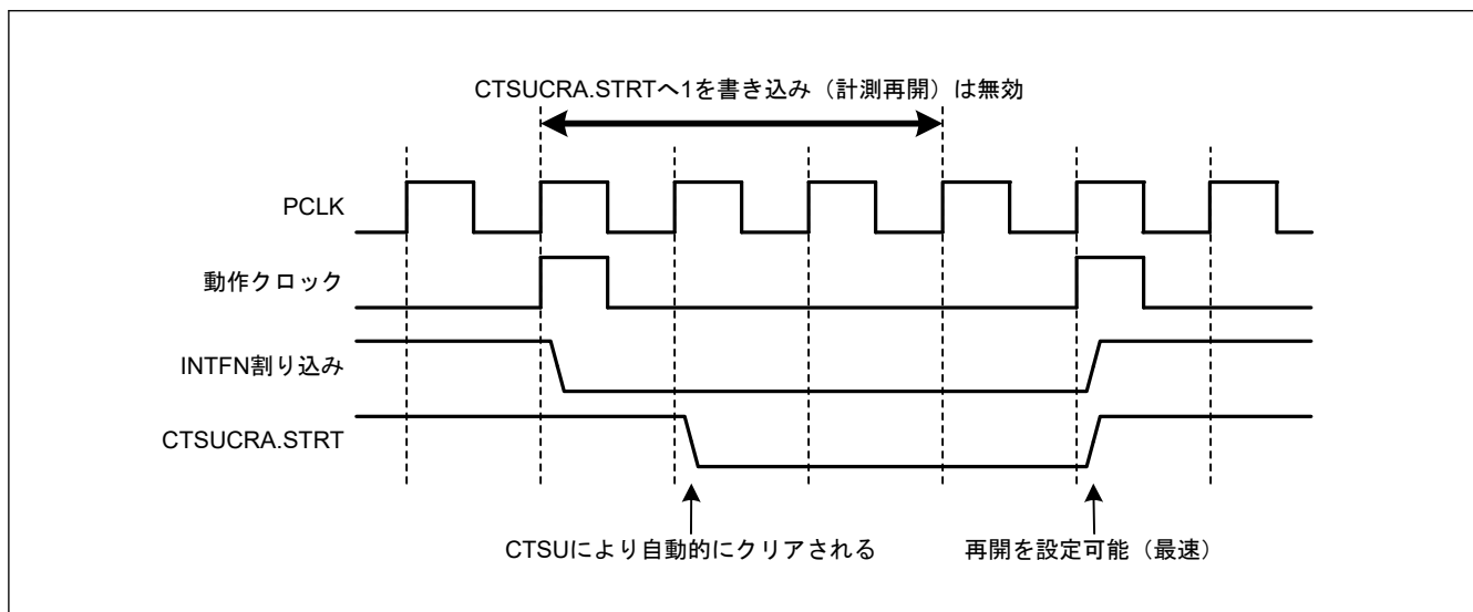
図 32.18 計測再開時の注意事項
