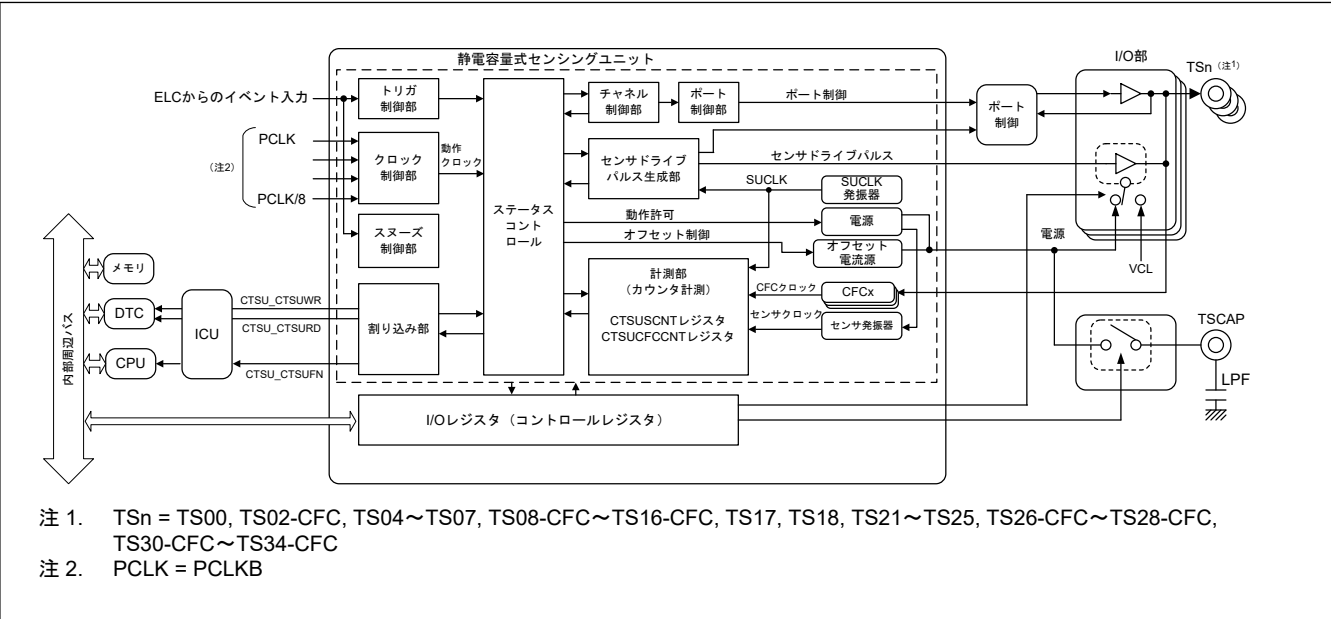
図 32.3 CTSU2 のブロック図
