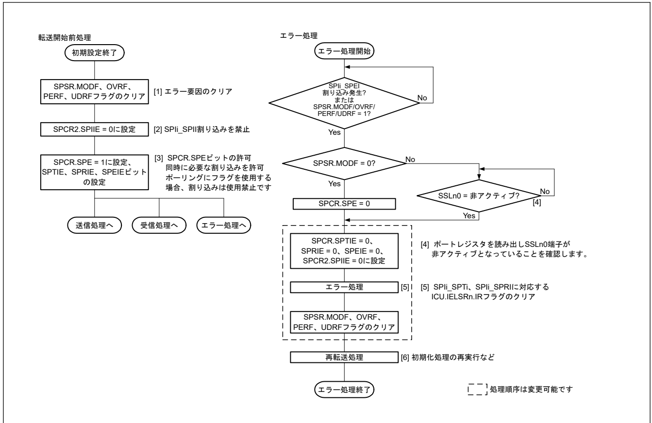
図 27.35 マスタモードでのエラー処理フロー
