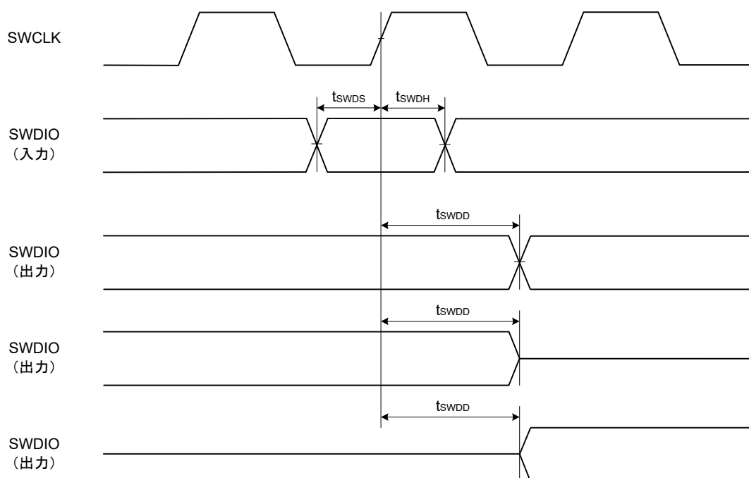
図 39.49 SWD 入出力タイミング
