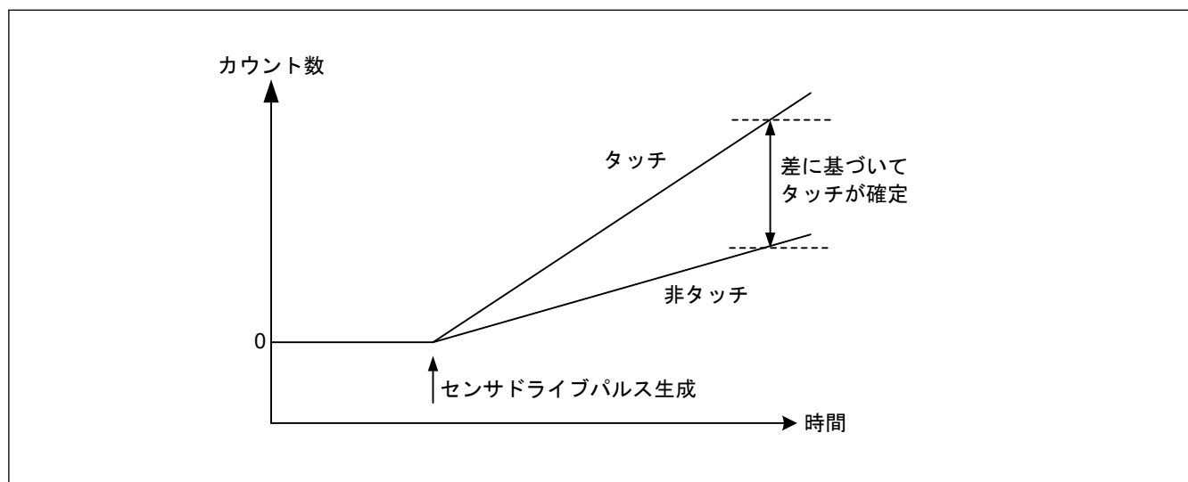
図 32.7 指の接触／非接触による計測値の変化
