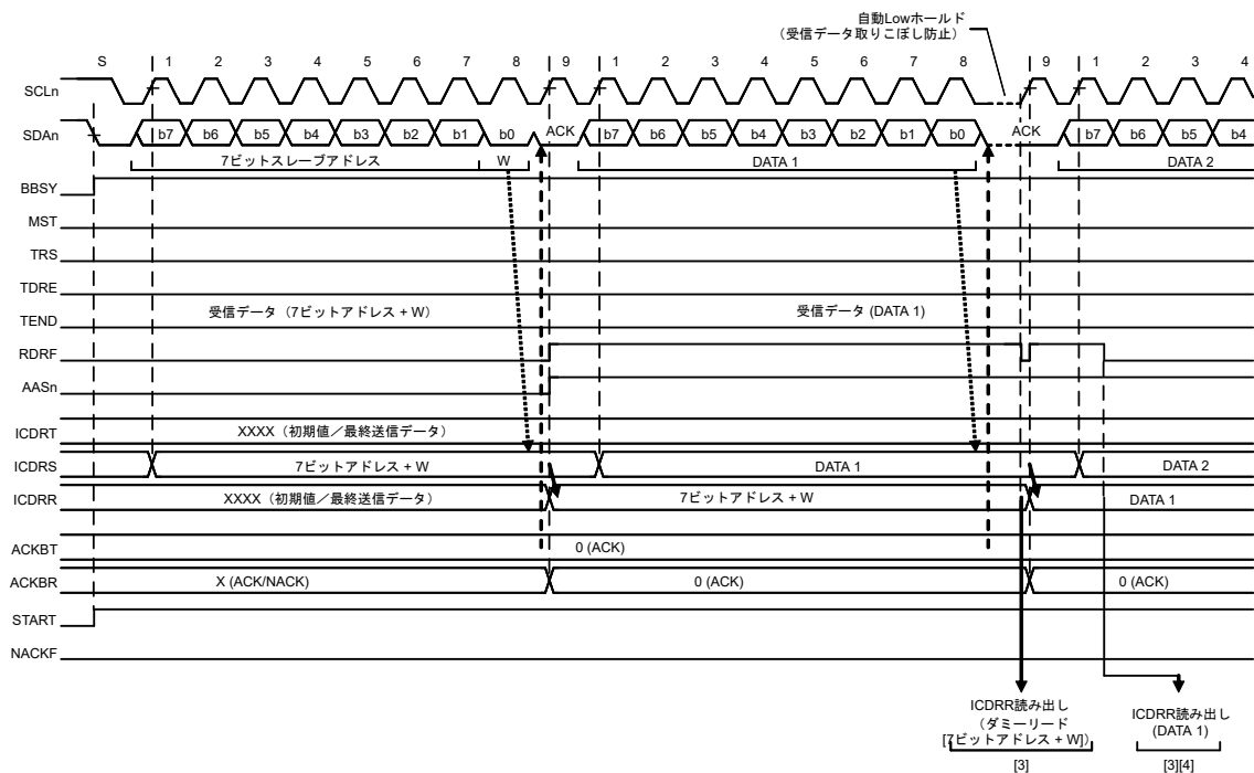
図 26.19 スレープ受信の動作タイミング (1) (7 ビットアドレスフォーマットで RDRFS = 0 の場合)
