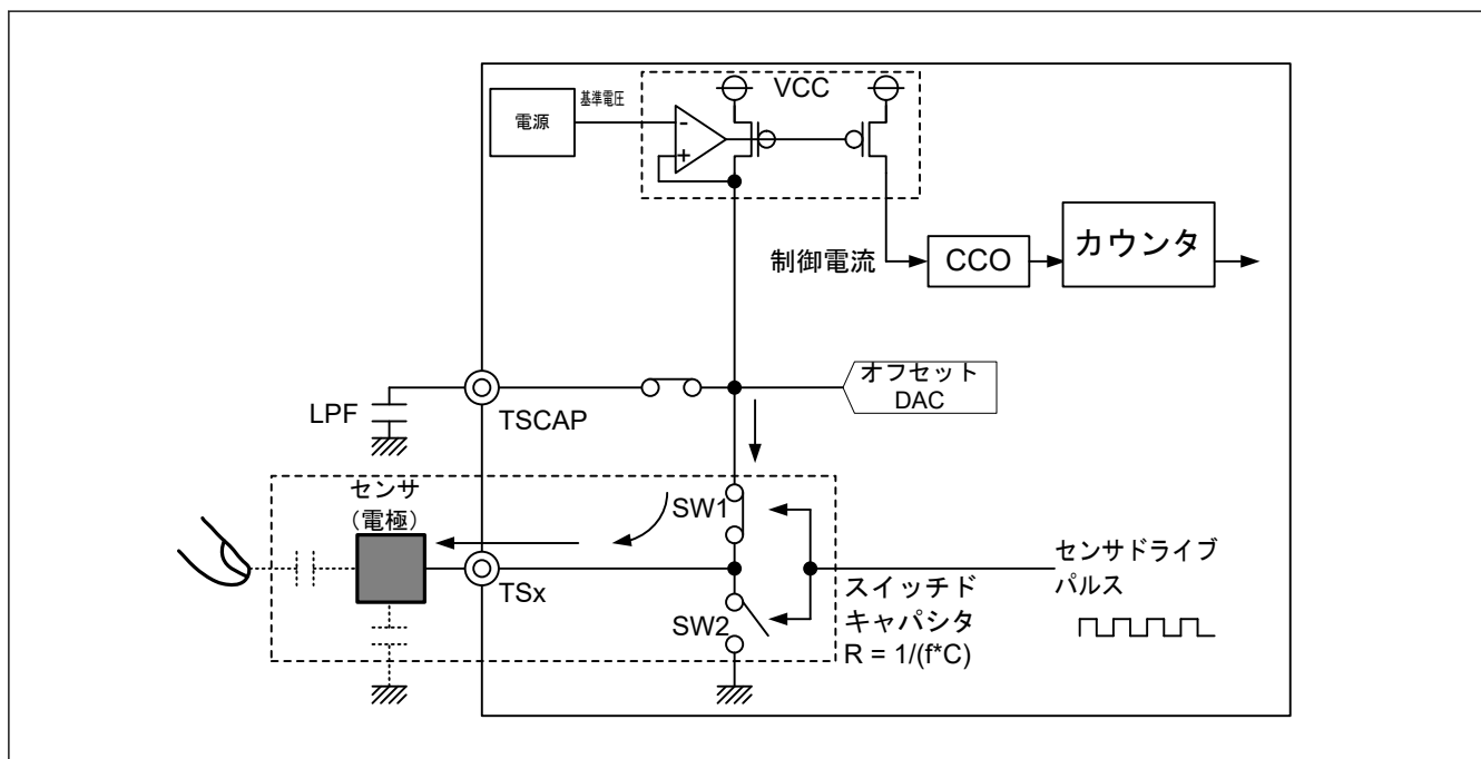
図 32.5 自己容量充電動作
