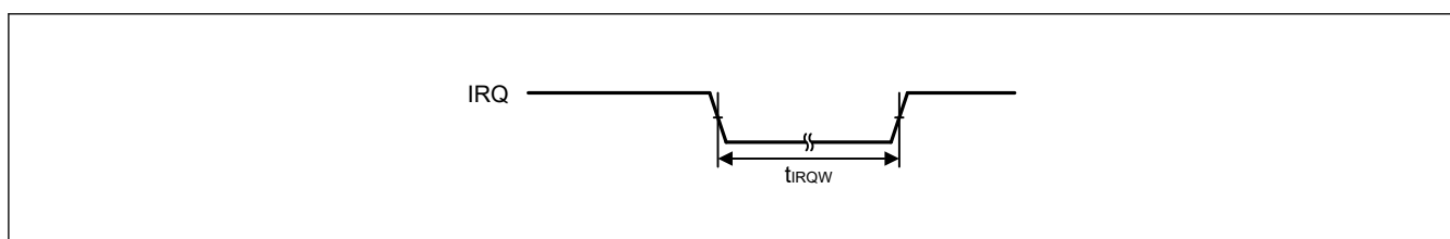
図 39.13 IRQ 割り込み入力タイミング
