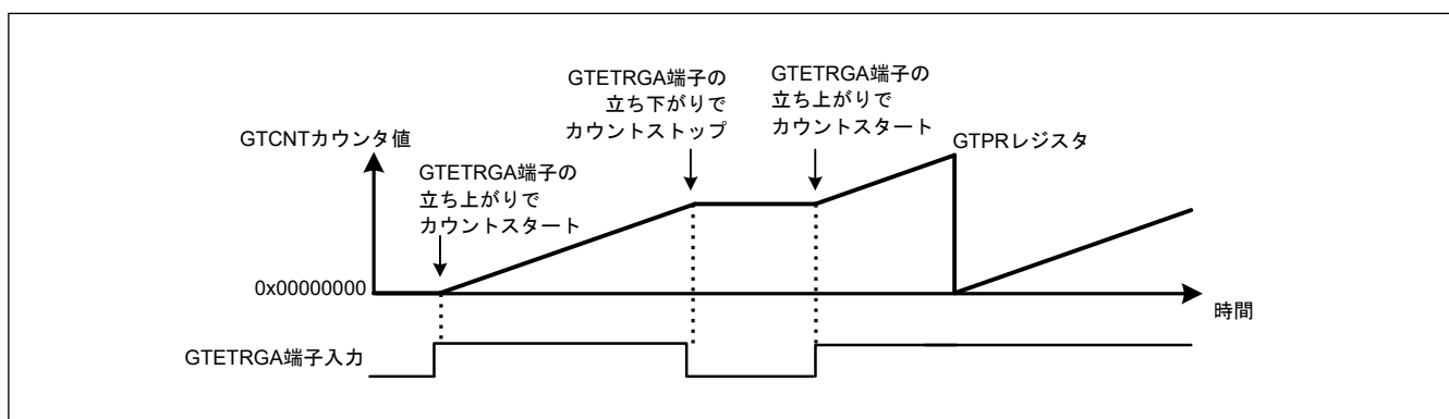
図 20.32 ハードウェア要因によるカウンタスタート/ストップ動作例 (GTETRGA 端子入力の立ち上がりエッジでスタート、GTETRGA 端子入力の立ち下がりエッジでストップの場合)
