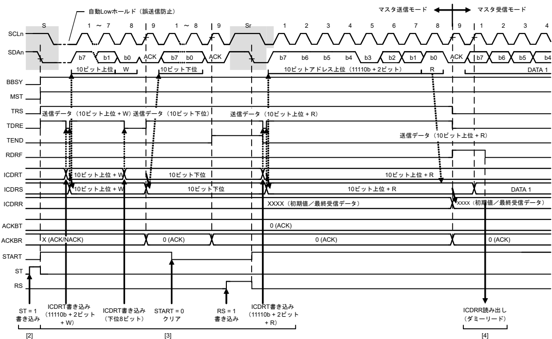
図 26.13 マスタ受信の動作タイミング (2) (10 ビットアドレスフォーマットで RDRFS = 0 の場合)
