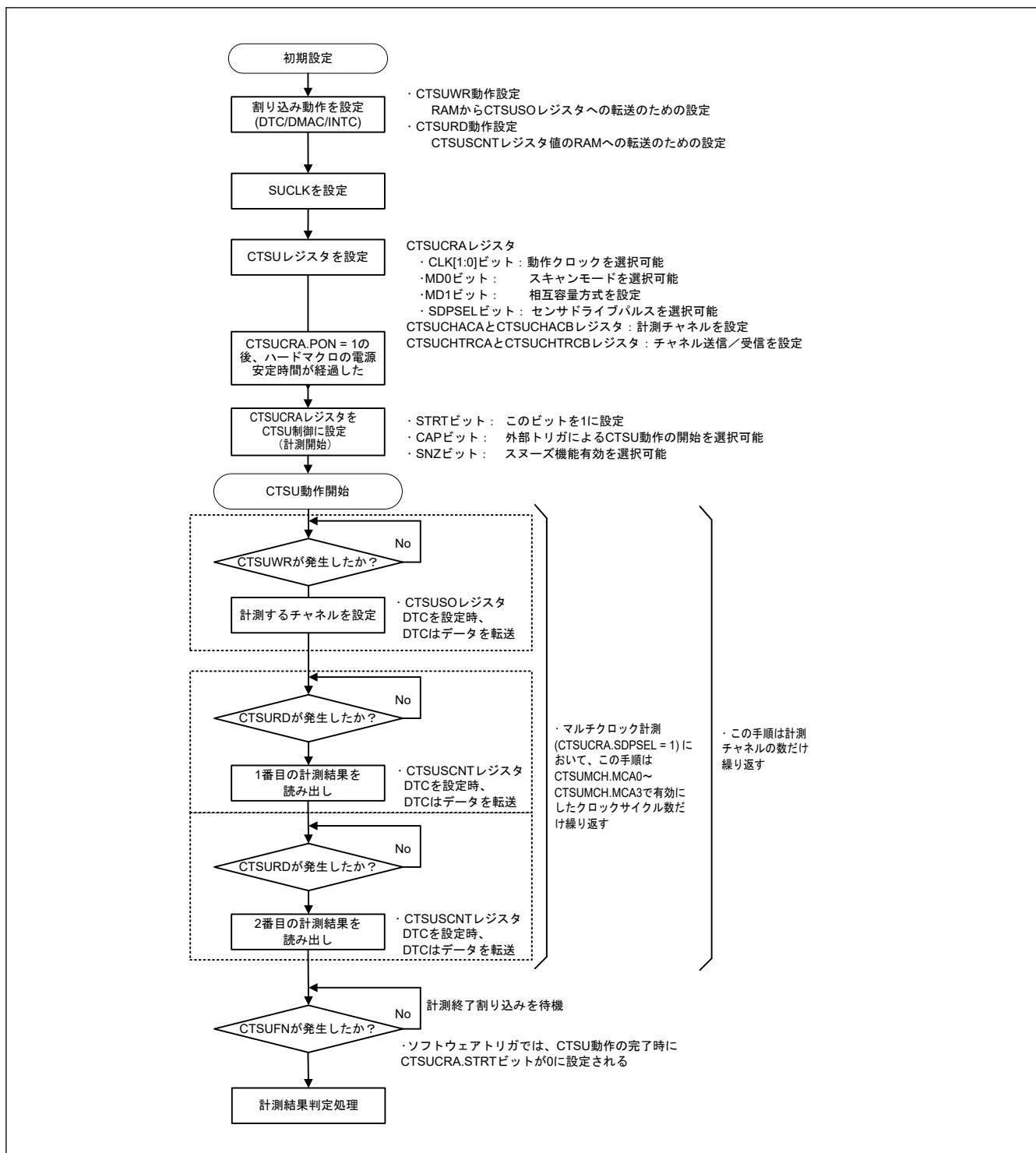
図 32.13 相互容量方式のソフトウェアフローと動作例
