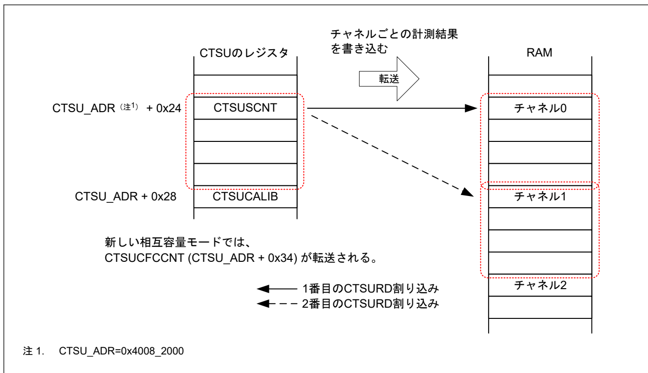
図 32.17 CTSURD 割り込みを用いた DTC 転送動作例
