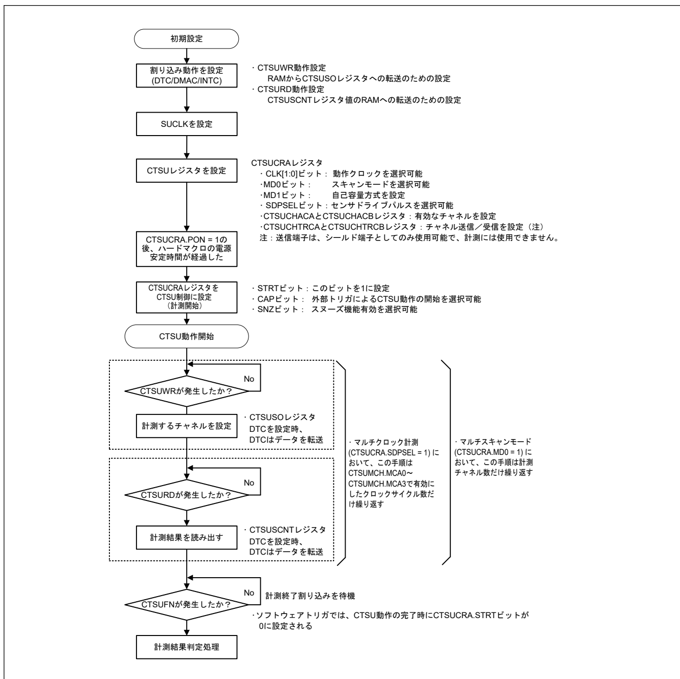
図 32.12 自己容量方式のソフトウェアフローと動作例
