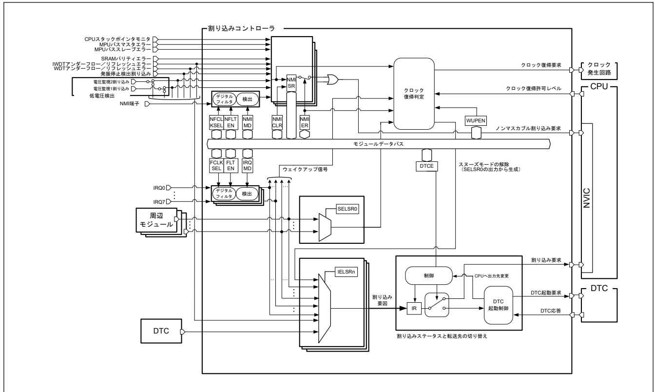
図 12.1 ICU のブロック図
