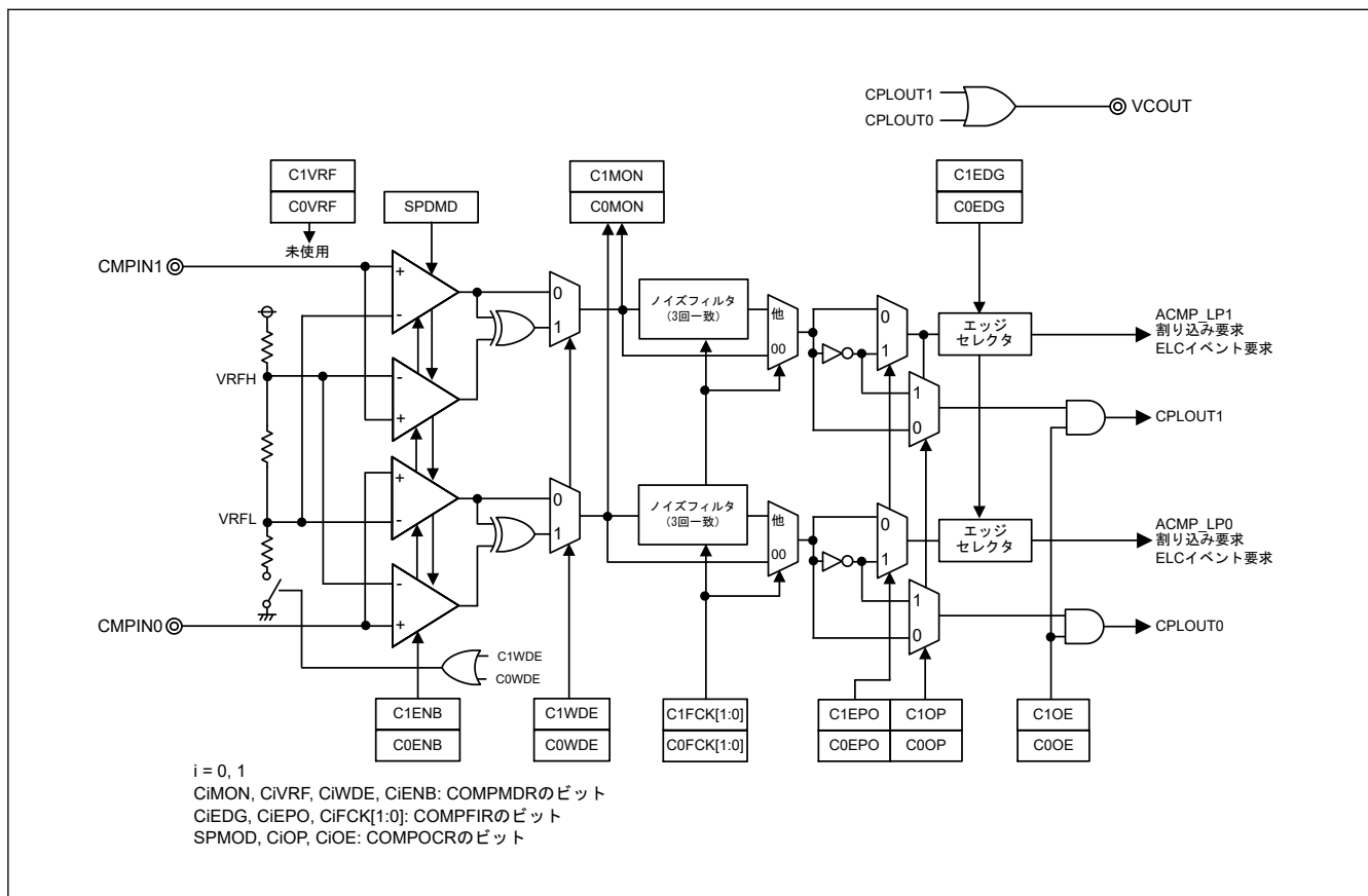
図 31.2 ウィンドウ機能有効時の ACMPLP ブロック図
