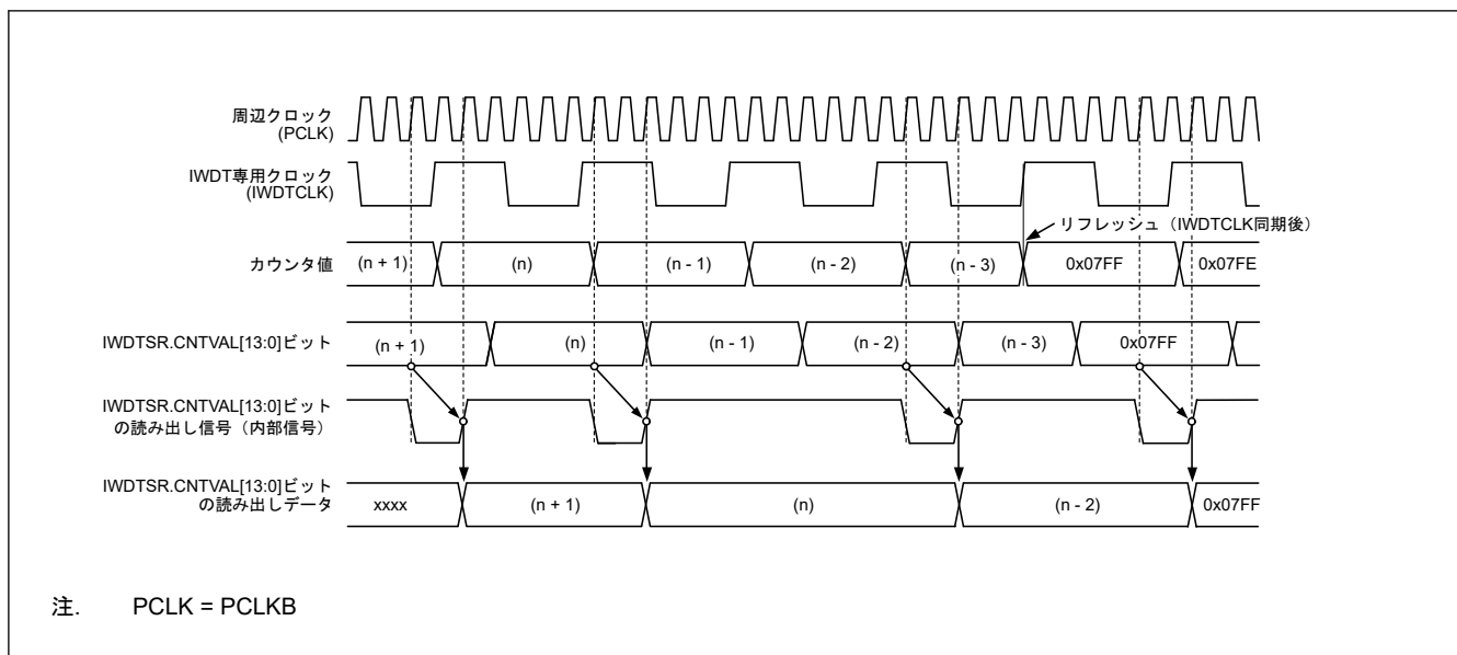
図 25.5 IWDТ ダウンカウンタ値の読み出し処理 (OFS0.IWDTCCKS[3:0] = 0000b、OFS0.IWDТТОPS[1:0] = 11b の場合)
