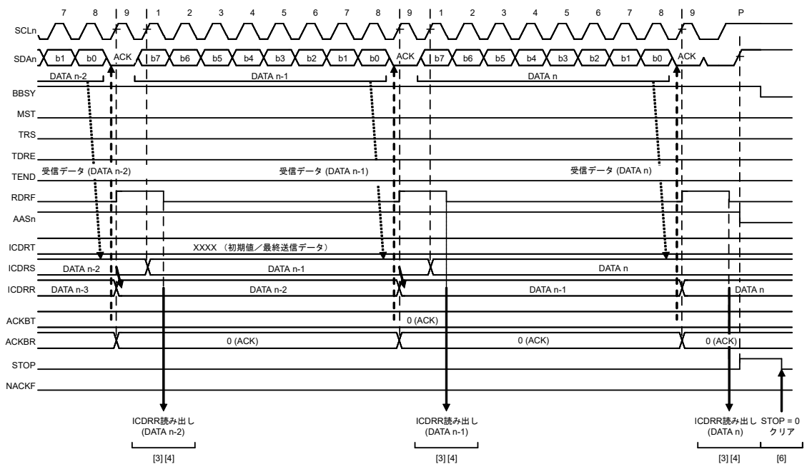
図 28.20 スレープ受信の動作タイミング (2) ( RDRFS = 0 の場合)
