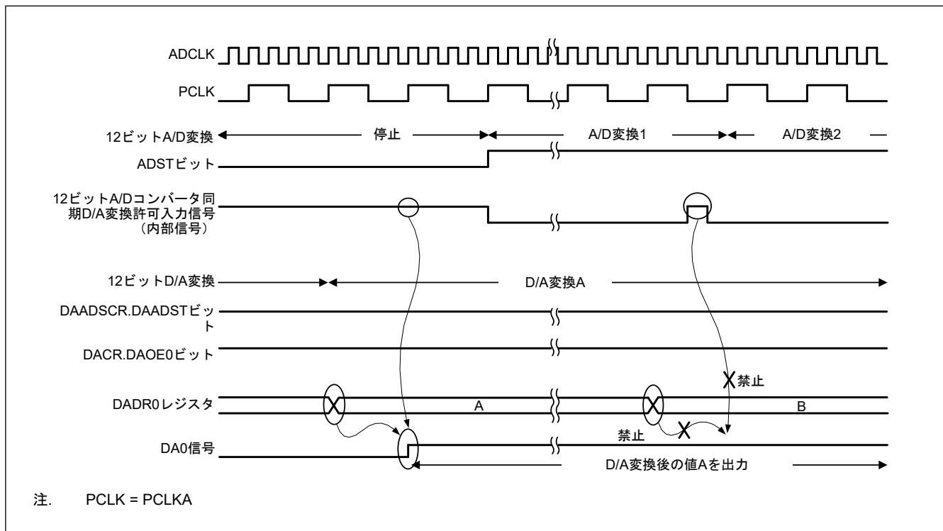
図 38.4 DAC12 が次からの同期 D/A 変換許可入力信号を取り込めない場合の例 : ADC12
