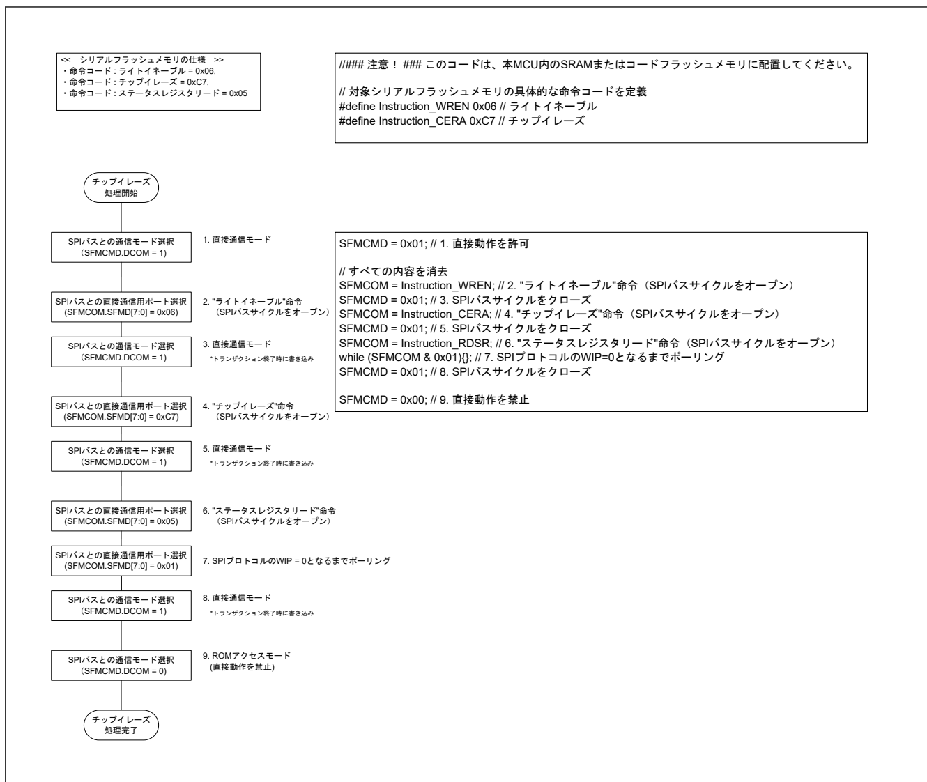
図 31.40 チップイレーズのフローチャート
