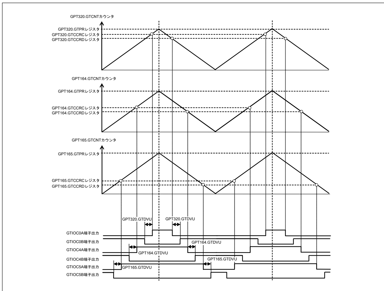
図 21.44 非対称三角波 3 相補 PWM 出力例 (デッドタイム自動設定)
