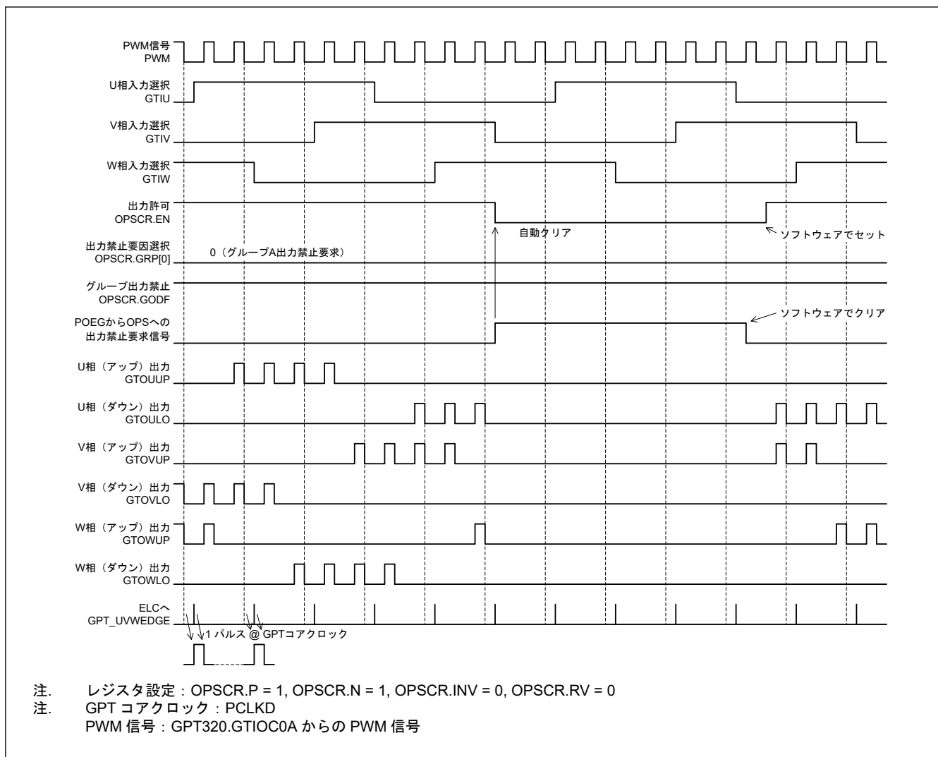
図 21.60 グループ出力禁止制御動作例
