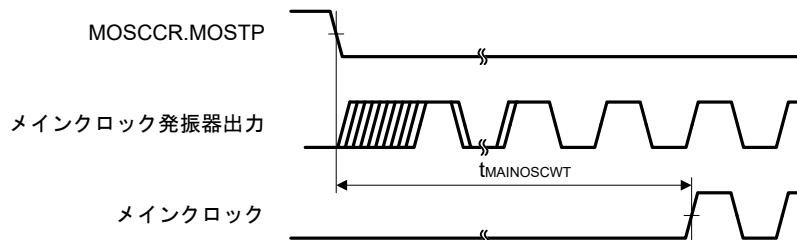
図 47.8 メインクロック発振開始タイミング
