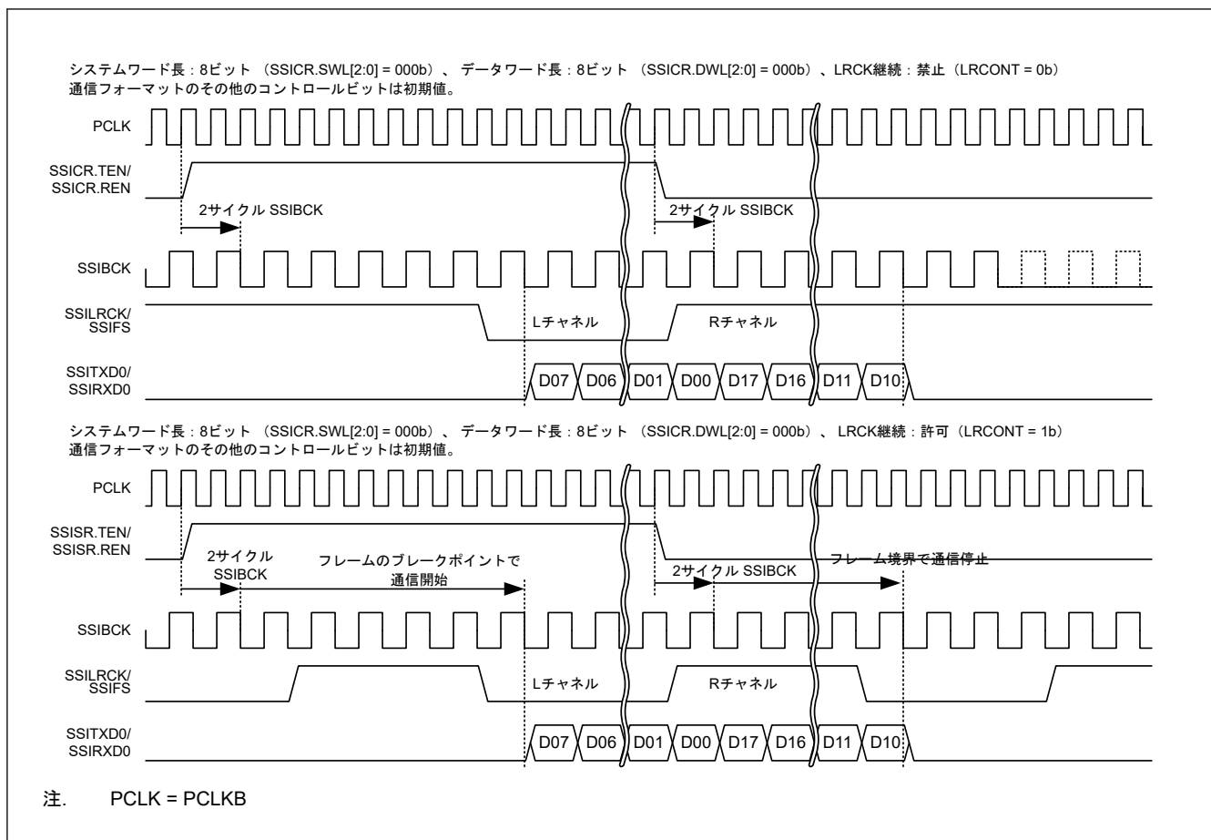
図 32.32 LR クロック/フレーム同期継続の動作例
