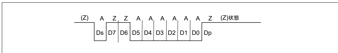
図 27.80 インバースコンペンション (SCMR.SDIR ビット = 1、SCMR.SINV ビット = 1、SMR_SMCI.PM ビット = 1)
