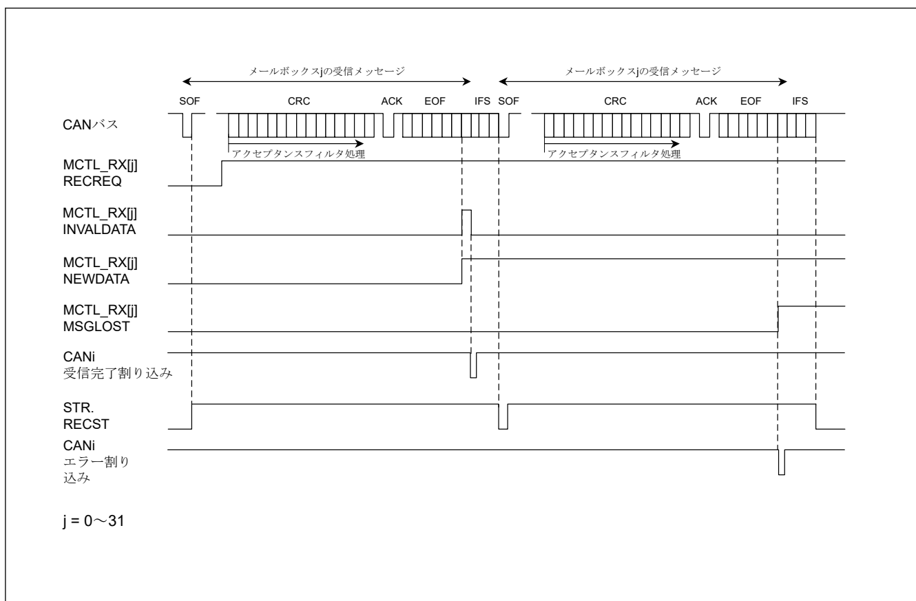
図 29.19 オーバーランモードでのデータフレーム受信の動作例
