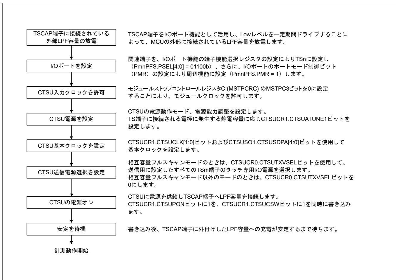
図 40.9 CTSU 初期設定フロー
