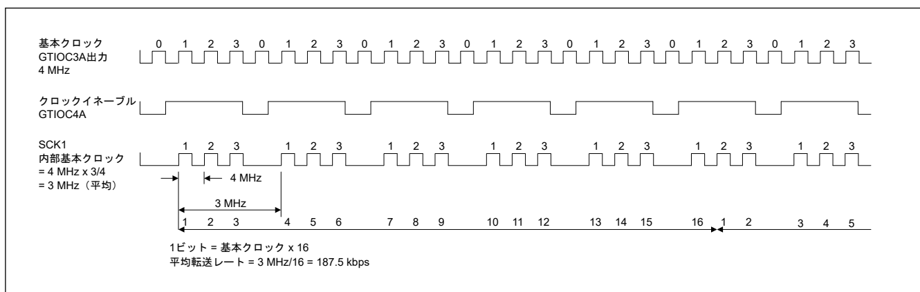
図 27.4 GPT クロック入力時の平均転送レート設定例
