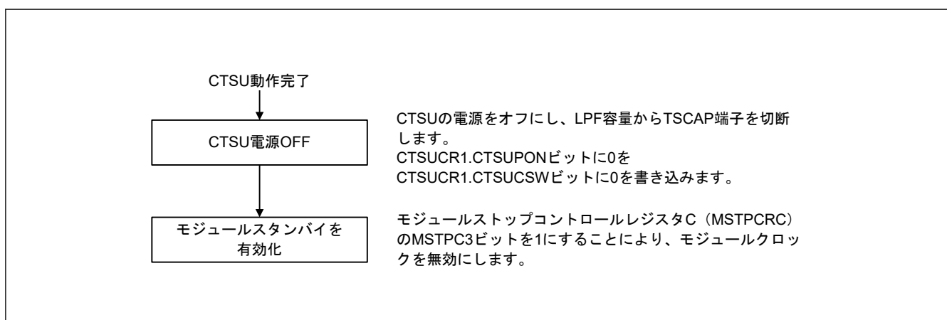
図 40.10 CTSU 停止フロー
