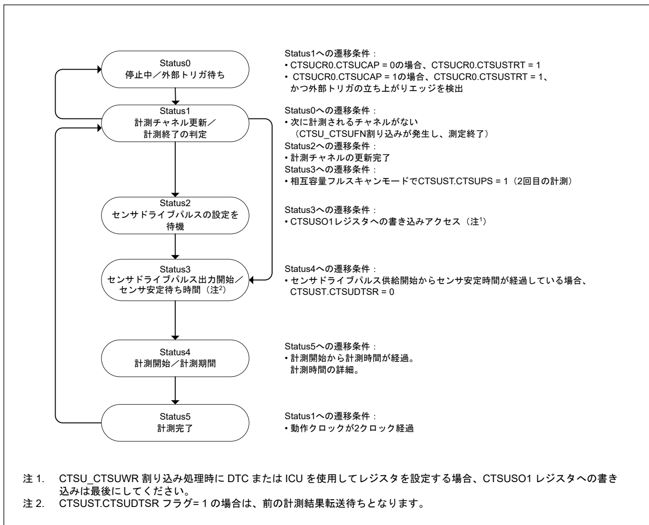
図 40.11 ステータス動作遷移図
