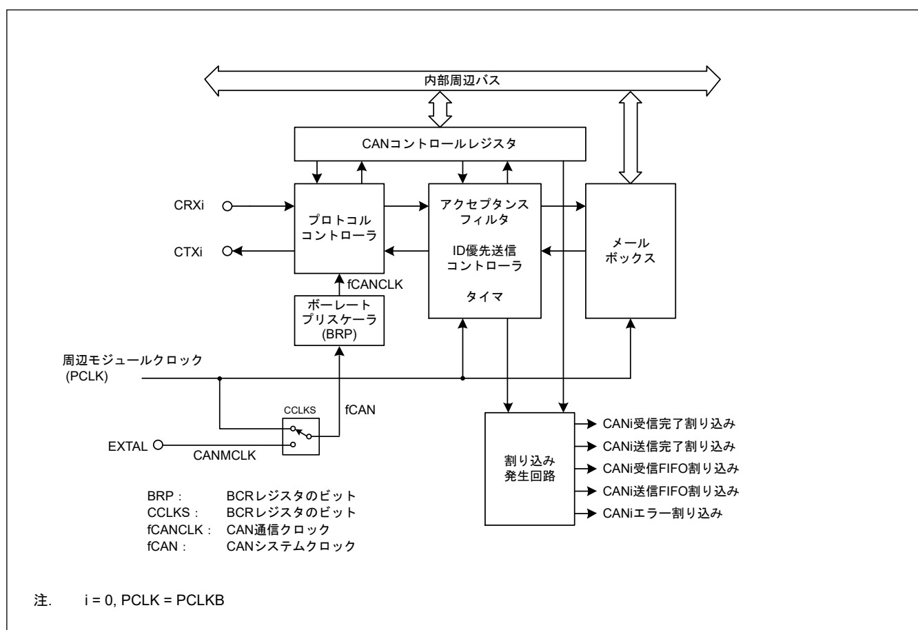
図 29.1 CAN モジュールブロック図
