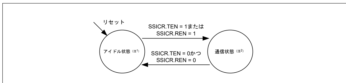
図 32.42 SSIE の状態遷移
