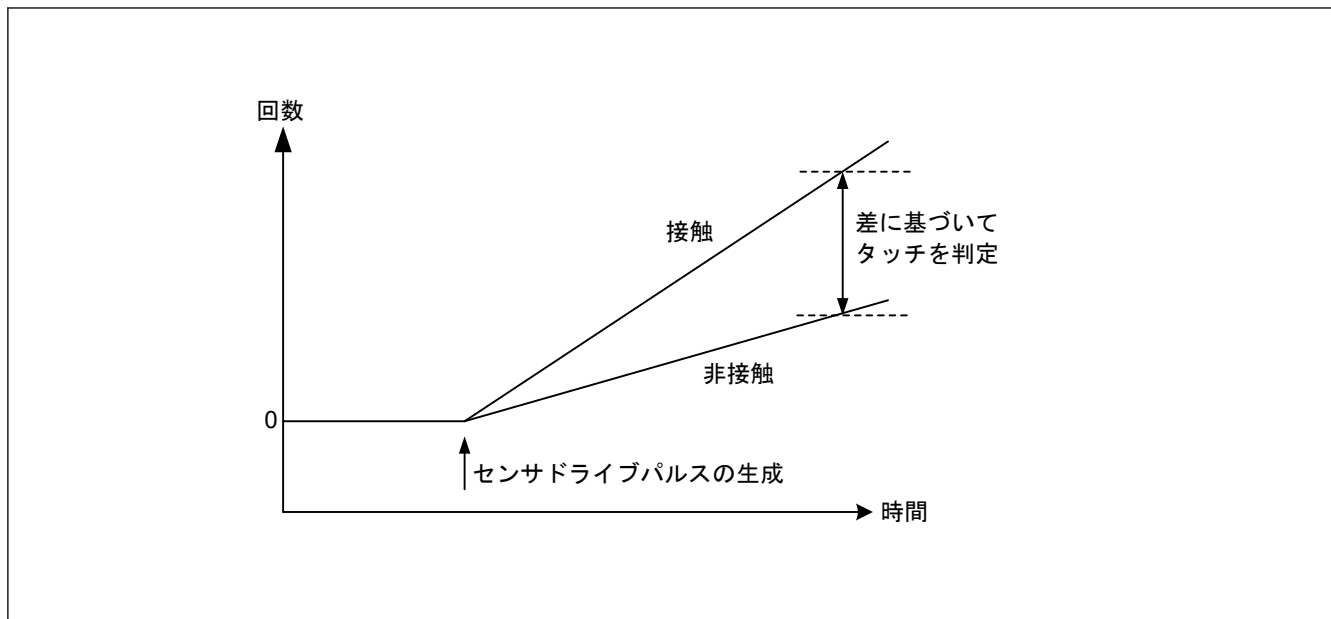
図 40.7 接触／非接触による計測値の変化
