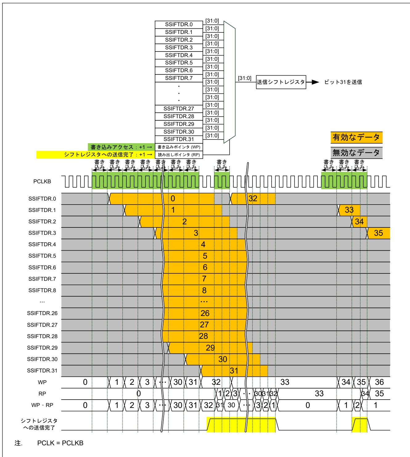
図 32.30 送信 FIFO データレジスタと送信シフトレジスタの構成、および FIFO の動作例
