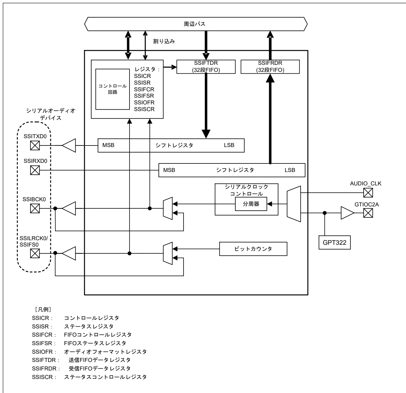
図 32.2 SSIE ブロック図
