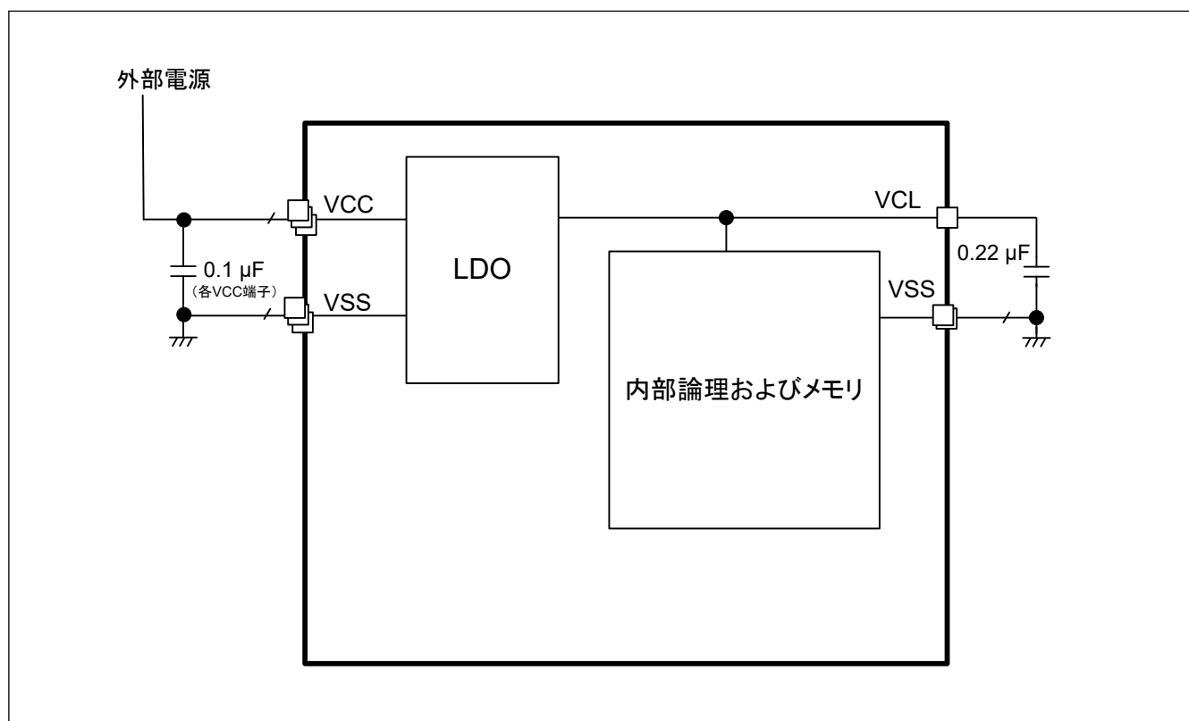
図 45.1 LDO モード設定
