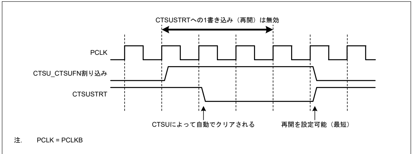
図 40.21 再開時の注意事項
