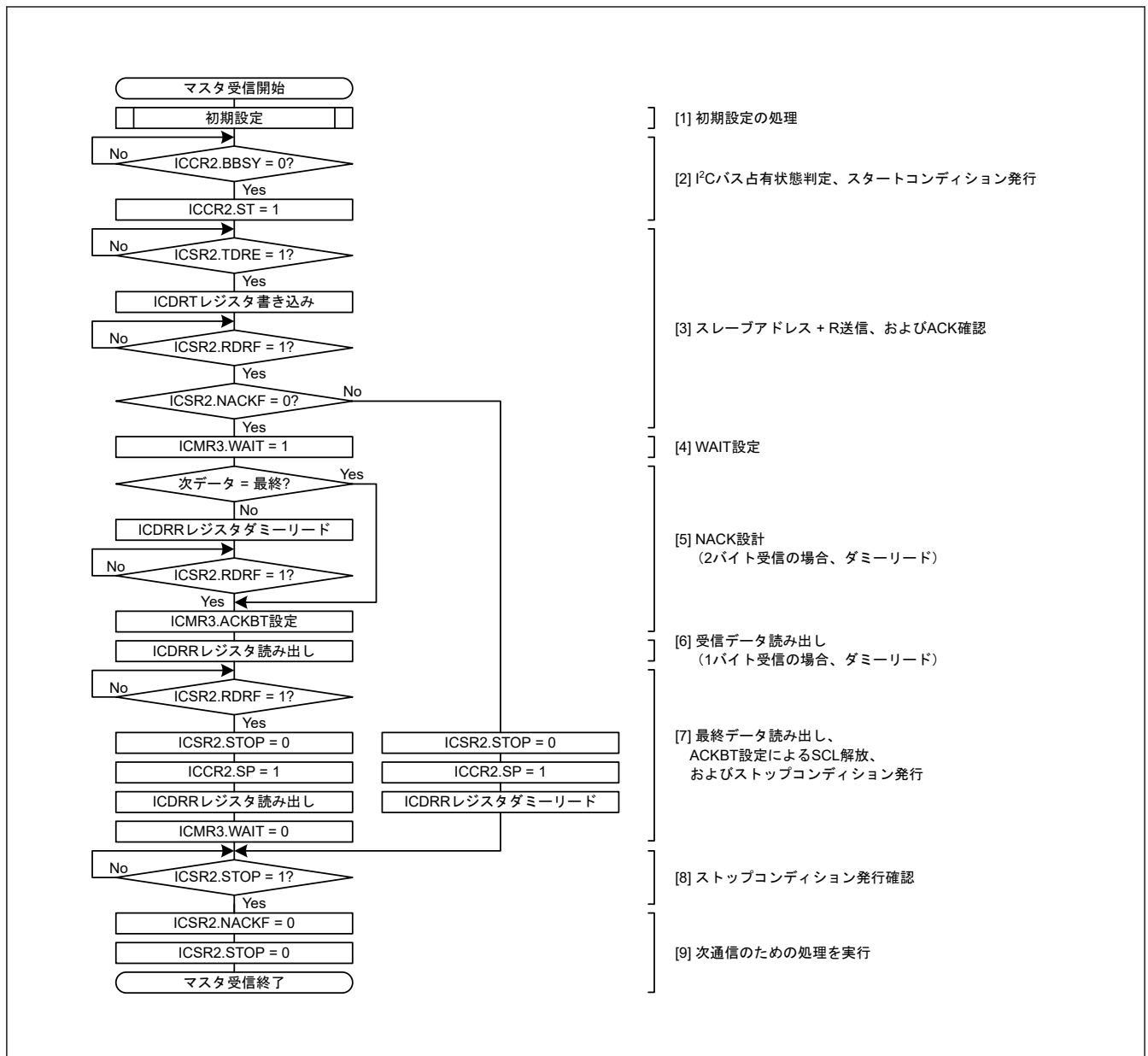
図 28.10 マスタ受信の例 (7 ビットアドレスフォーマットで 1 または 2 バイト受信の場合)
