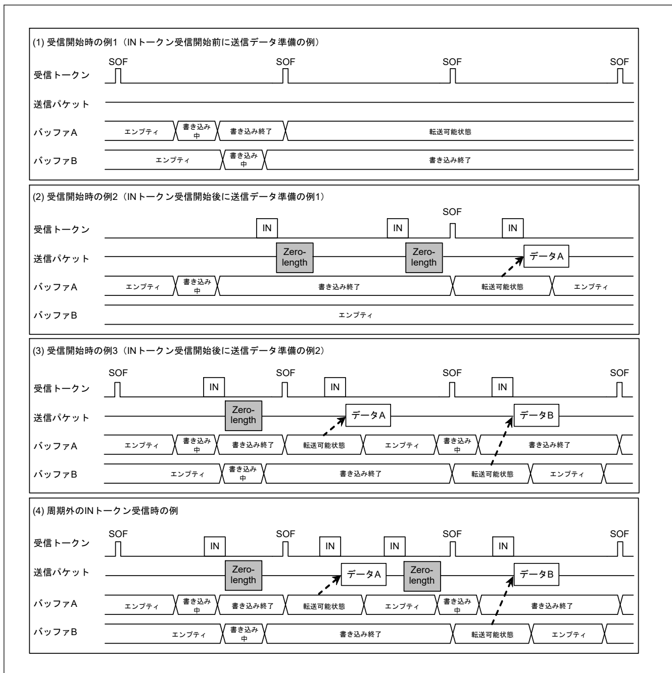
図 26.21 データセットアップ動作例
