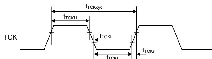
図 47.63 バウンダリスキャン TCK タイミング
