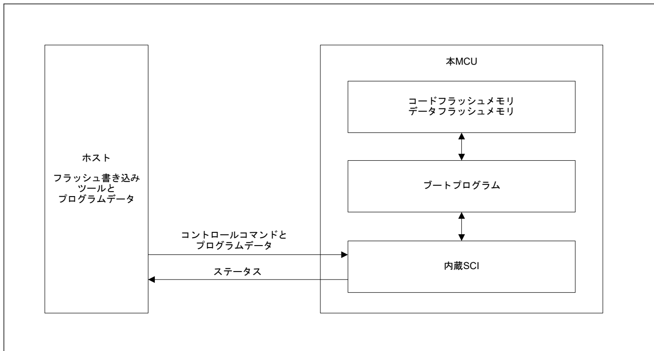
図 44.38 ブートモード（SCI インタフェース）時のシステム構成
