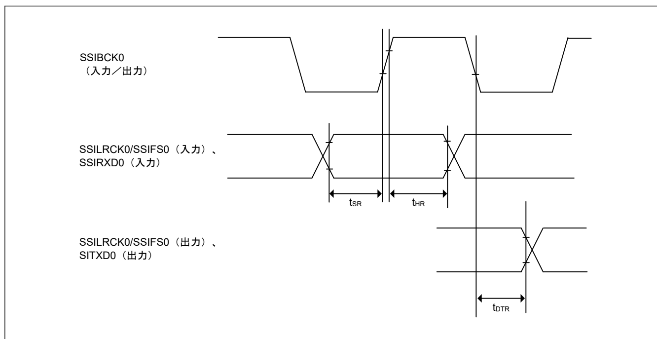
図 47.46 SSICR.BCKP = 0 の場合の SSIE データ送受信タイミング
