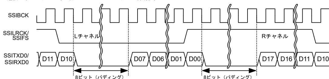
図 32.9 パディングビットを伴うシリアルデータのアライメント設定
