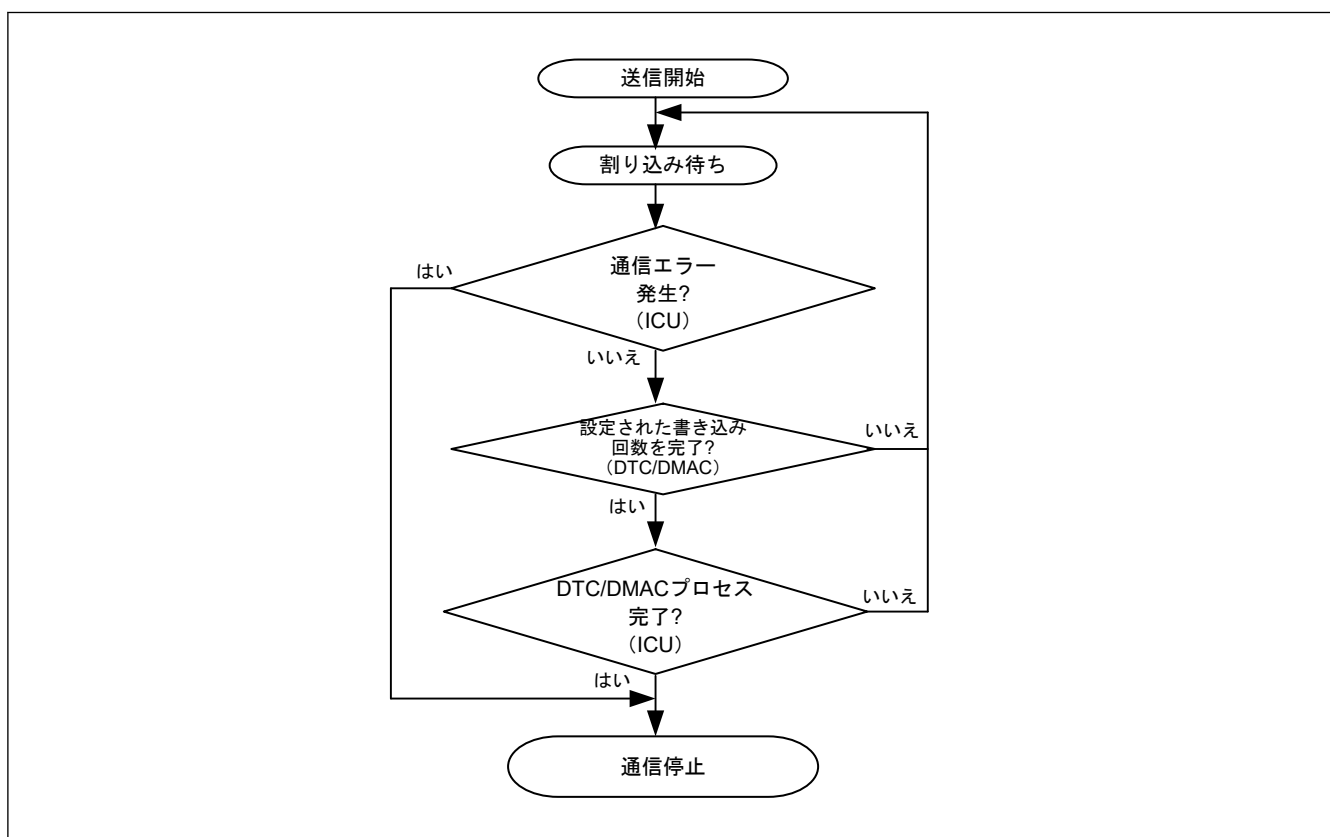
図 32.53 送信手順
