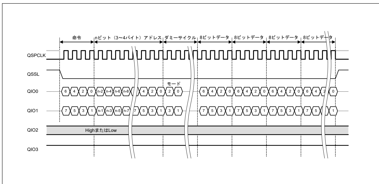
図 31.6 Dual-SPI プロトコル例（ファストリード Dual I/O）
