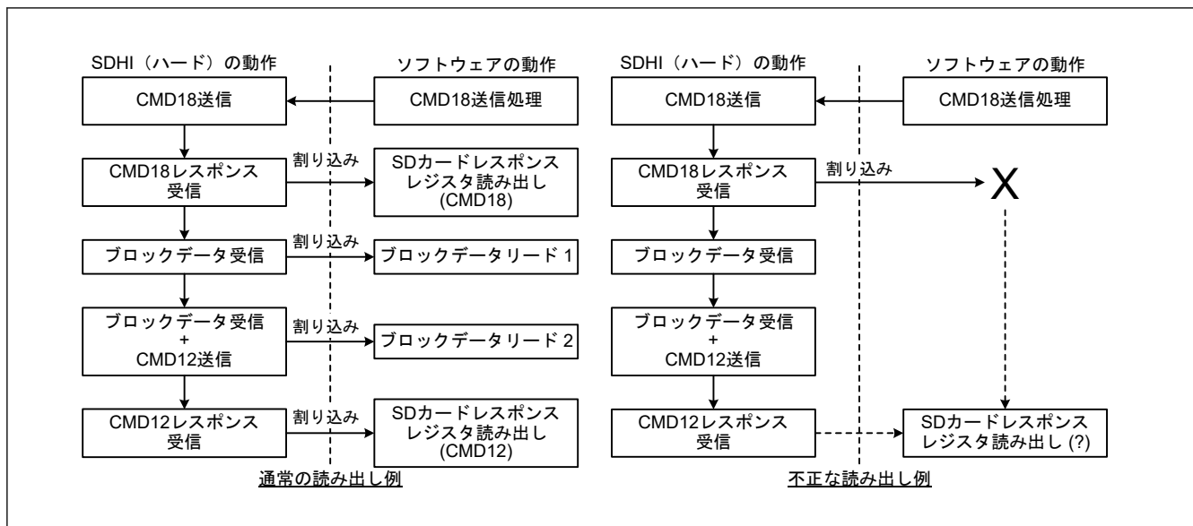
図 33.24 マルチブロックリード動作のフローチャート (2 ブロック)
