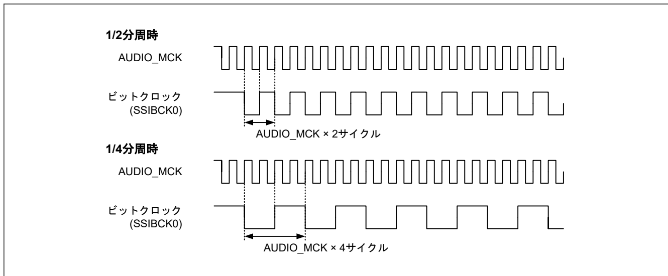
図 32.5 マスタモード通信時のサンプリング周波数
