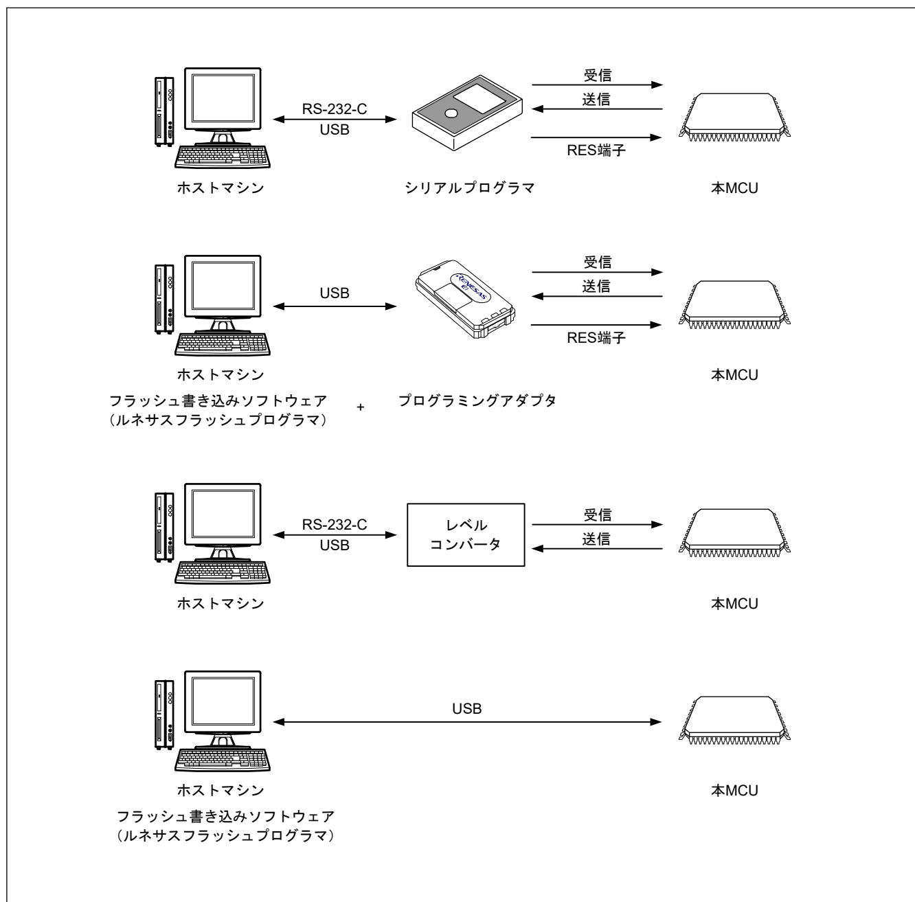
図 44.40 フラッシュメモリを書き換えるための環境
