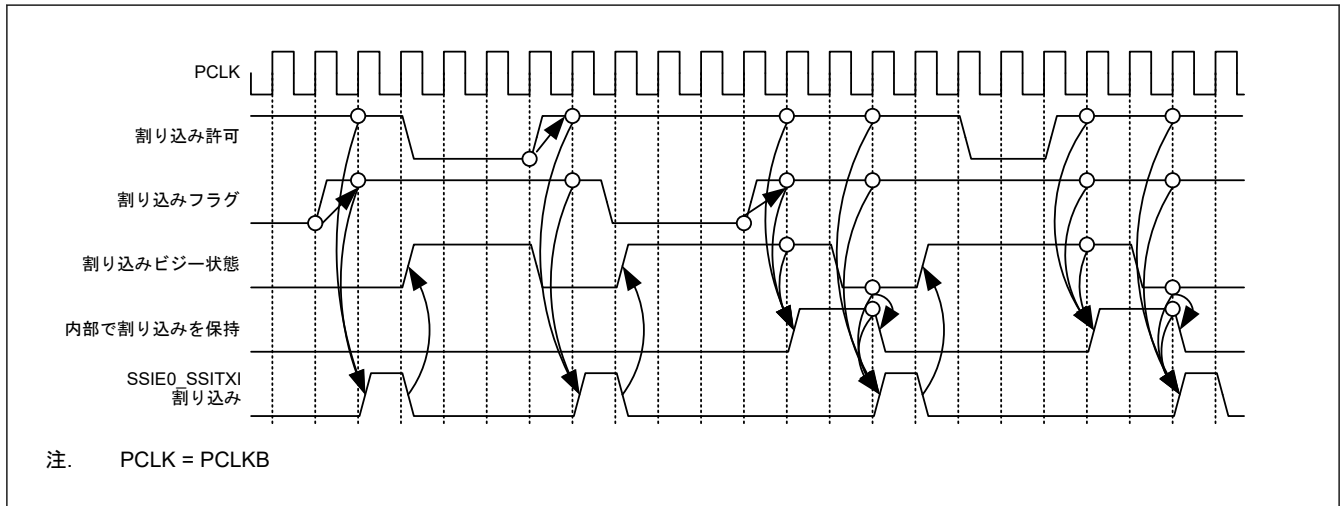
図 32.59 SSIE0_SSITXI 割り込みタイミング図
