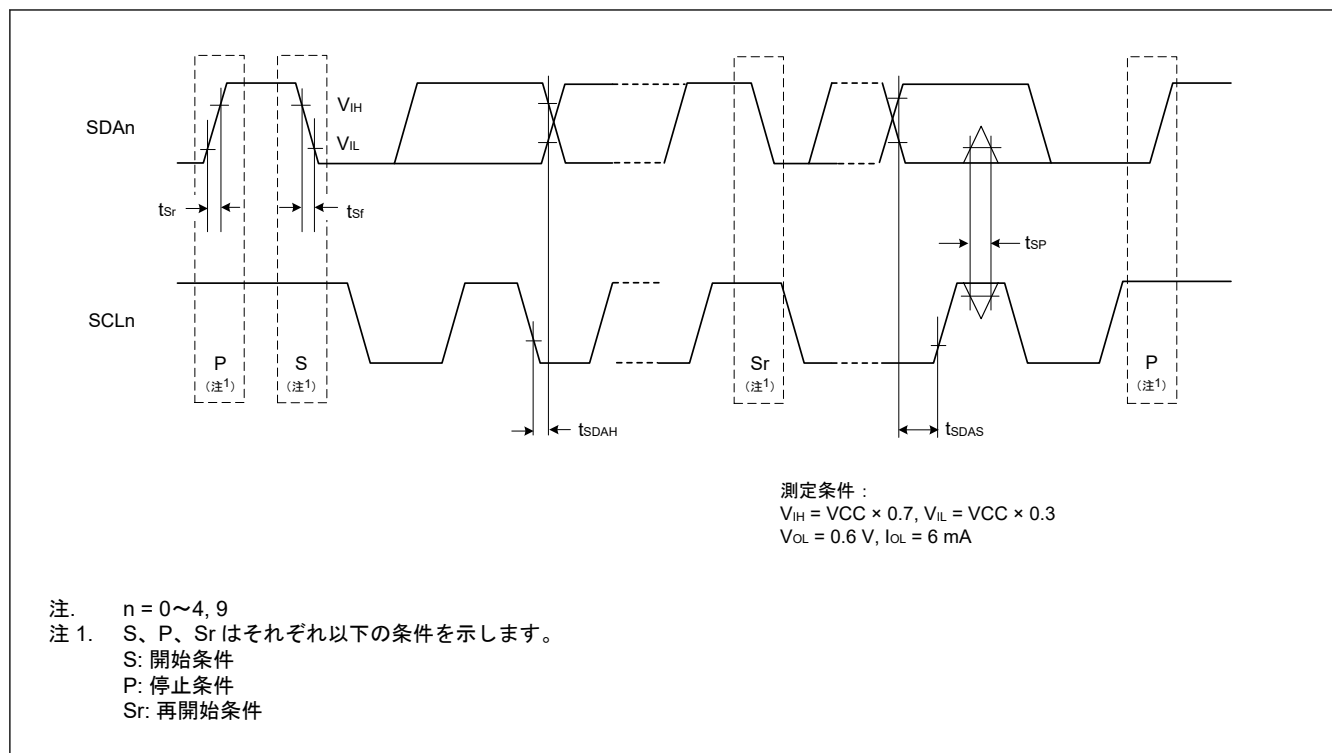
図 47.33 SCI 簡易 IIC モードタイミング
