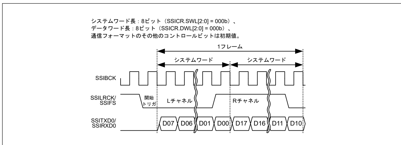
図 32.36 I 2 S フォーマット (パディングなし、システムワード長 = データワード長)
