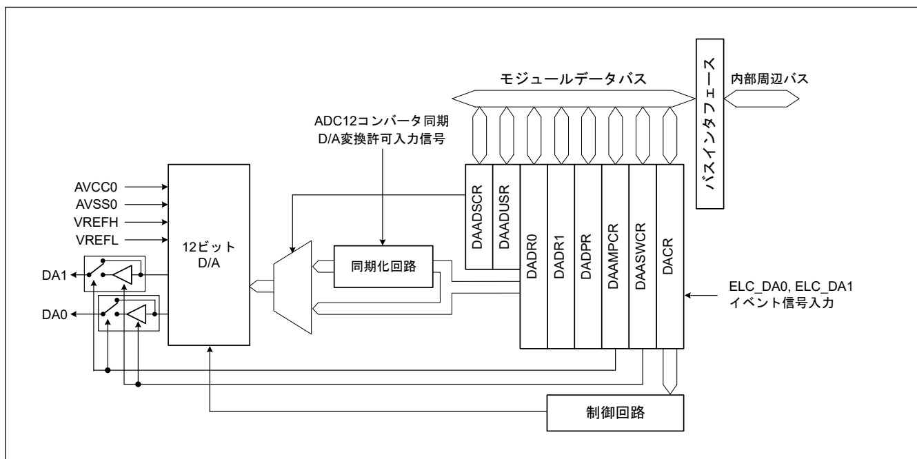
図 38.1 DAC12 のブロック図
