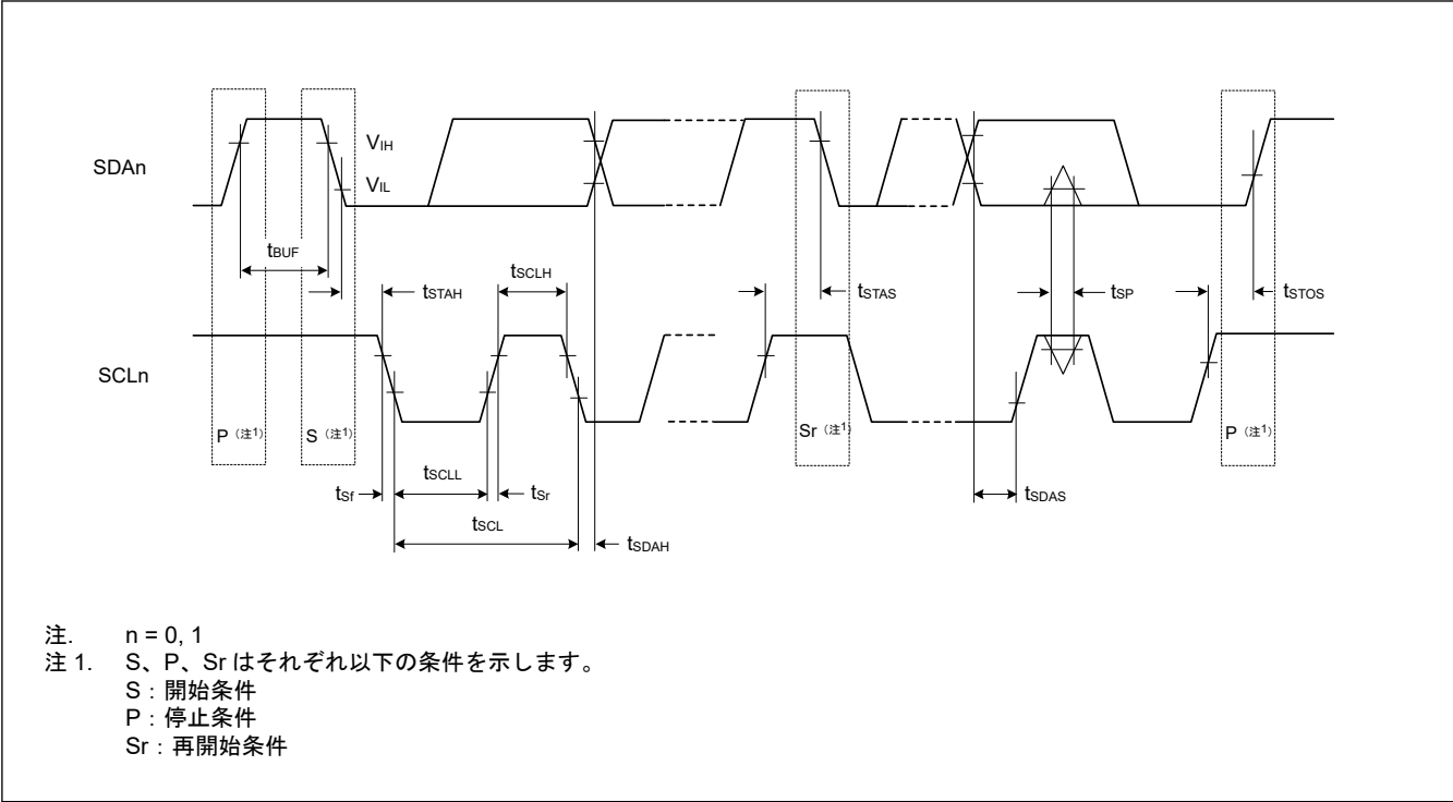
図 47.43 I 2 C バスインタフェース入出力タイミング
