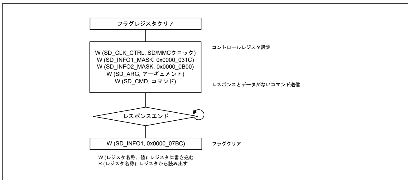
図 33.8 レスポンスまたはデータがないコマンドのフロー例
