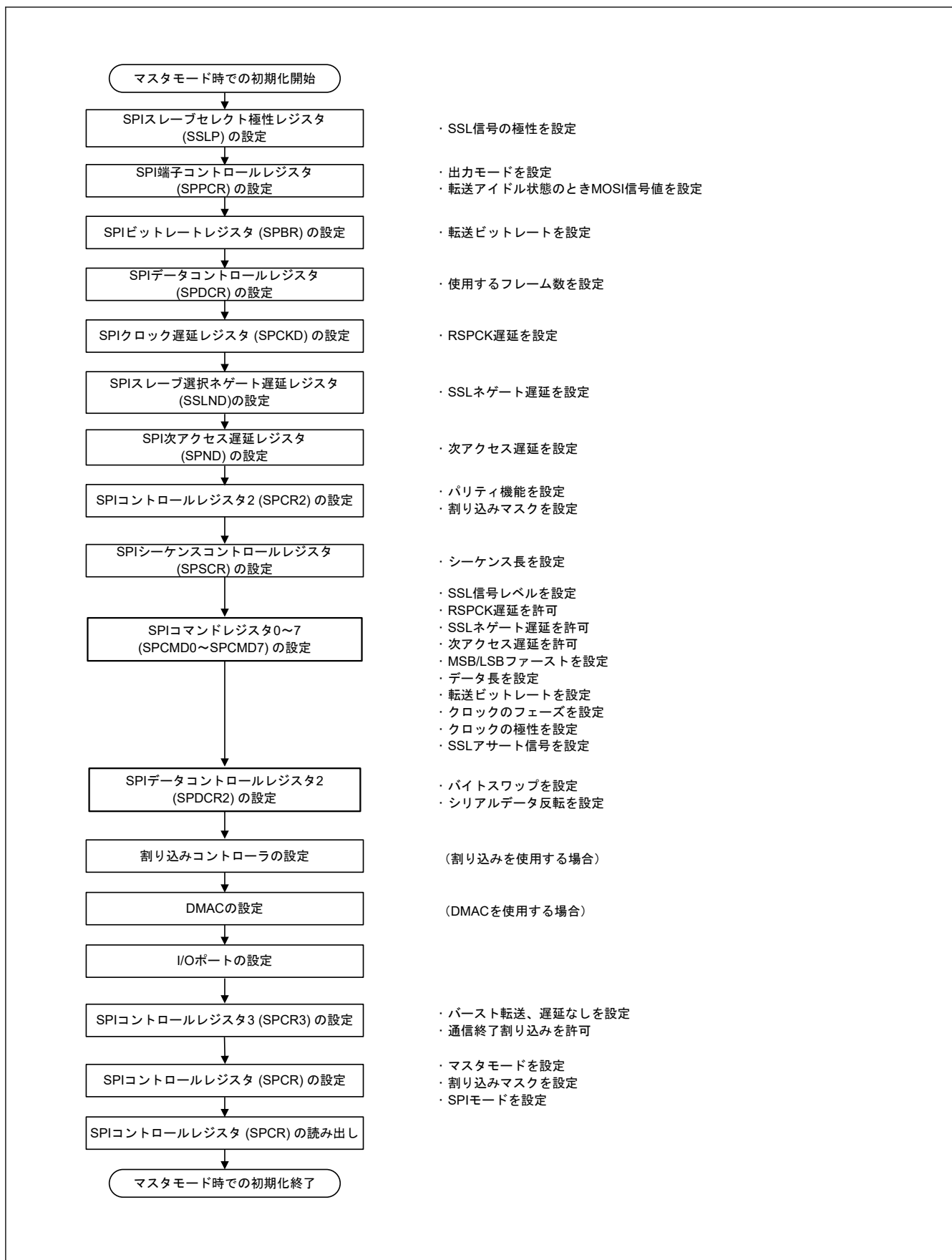
図 30.48 マスタモード時の SPI 動作の初期化フロー例
