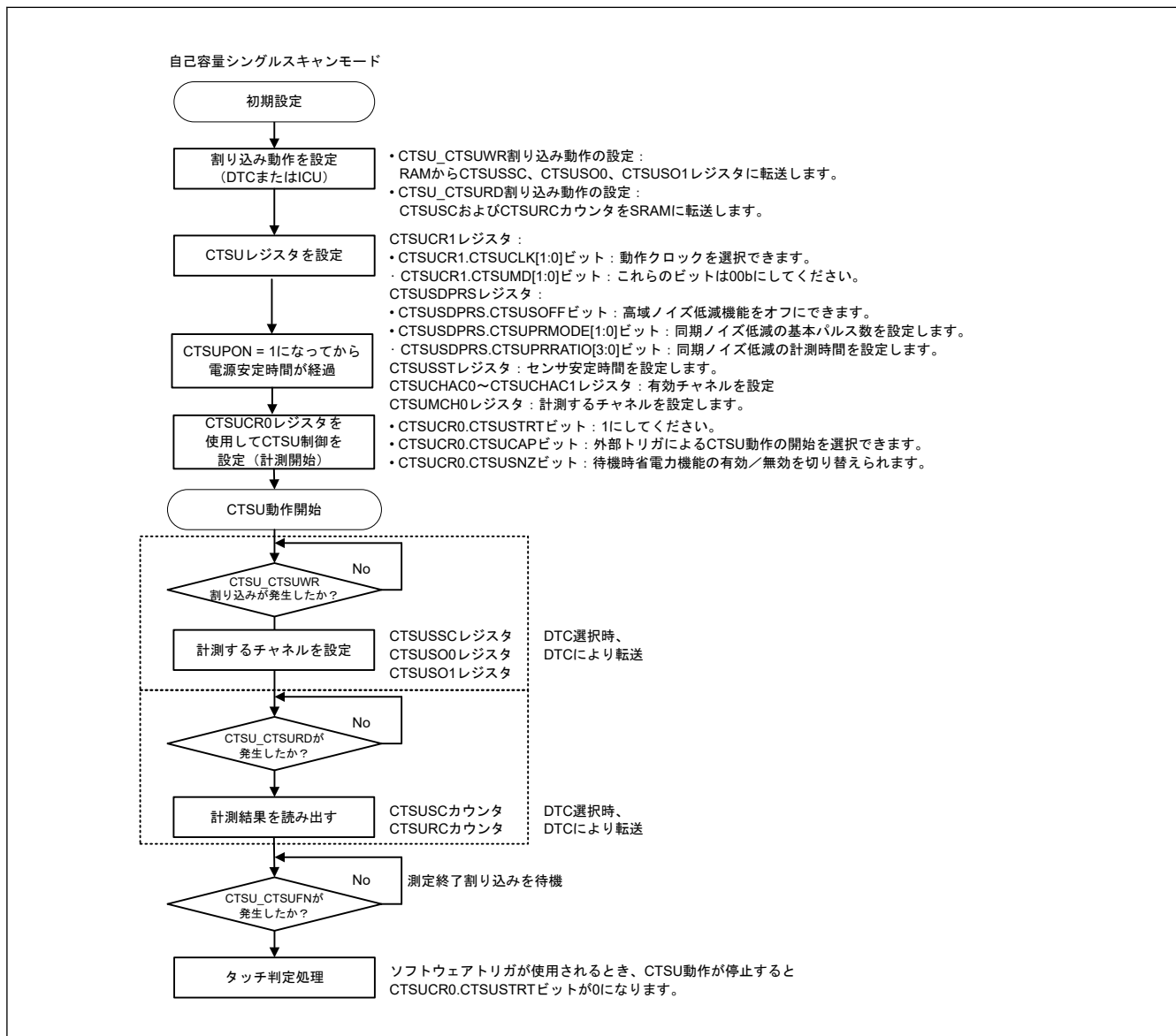
図 40.12 自己容量シングルスキャンモードのソフトウェアフローと動作例
