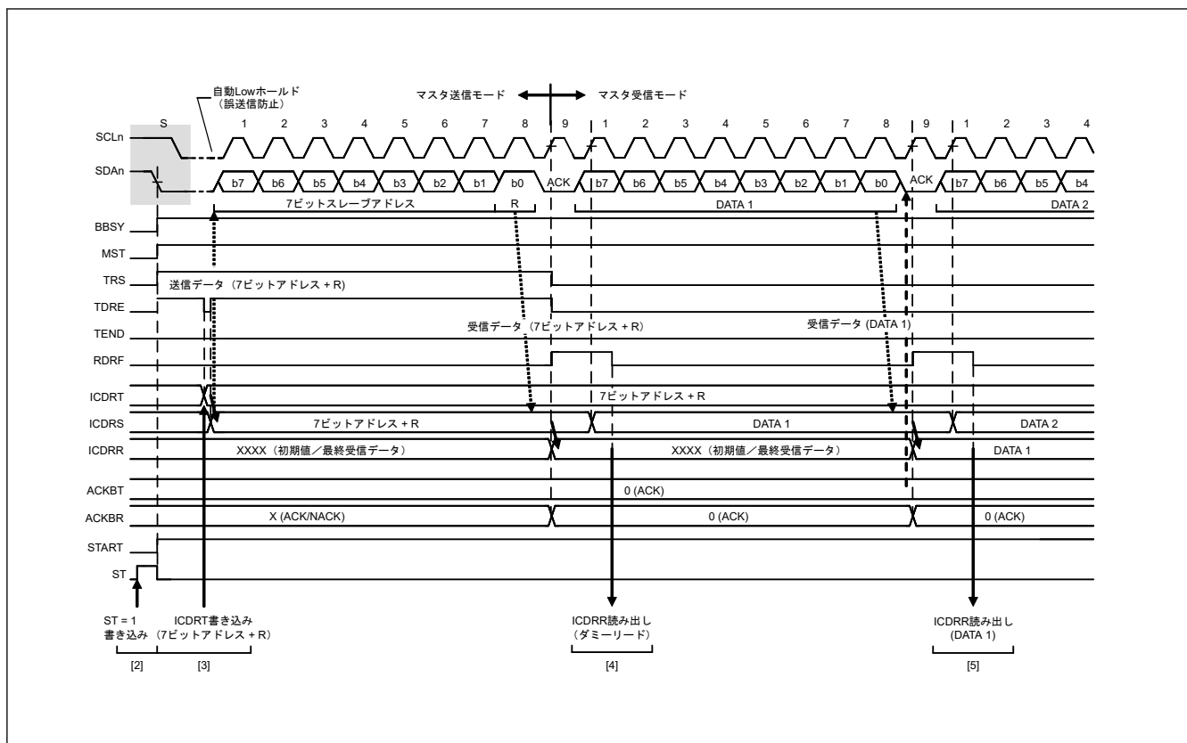
図 28.12 マスタ受信の動作タイミング (1) (7 ビットアドレスフォーマットで RDRFS = 0 の場合)
