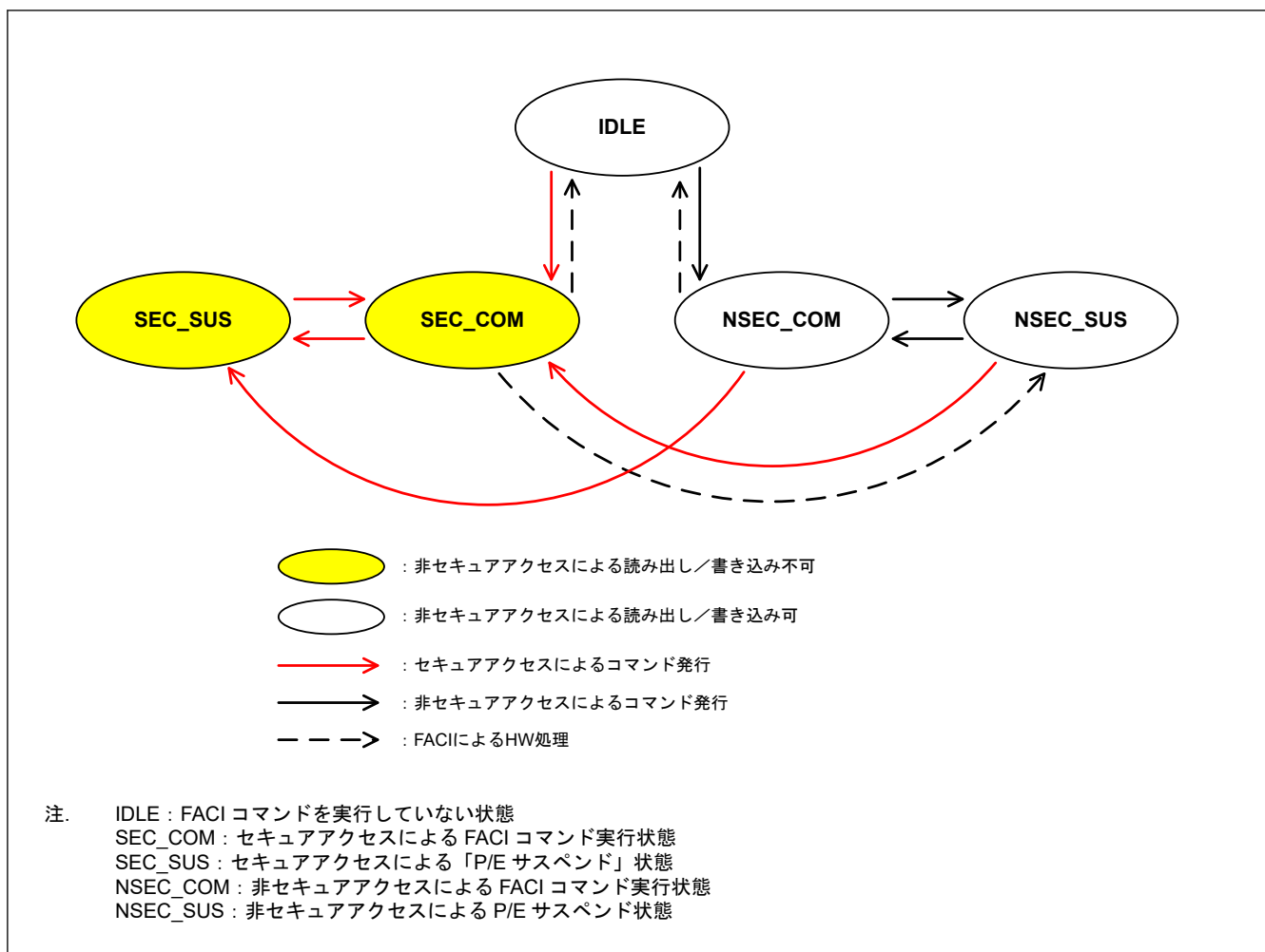
図 44.34 FACI コマンド動作中の保護状態
