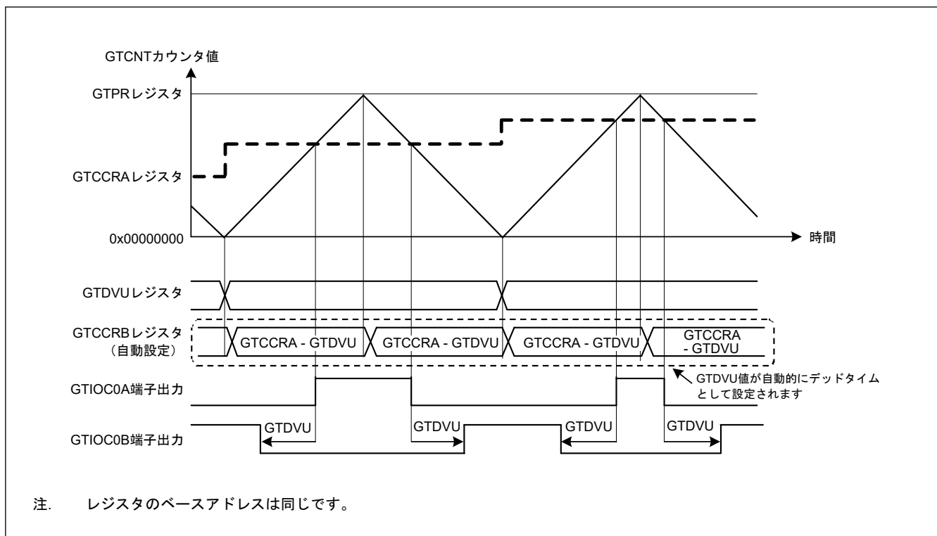
図 21.26 デッドタイム付きコンペアマッチ値の自動設定機能の動作例（三角波 PWM モード 1、アクティブ High の場合）
