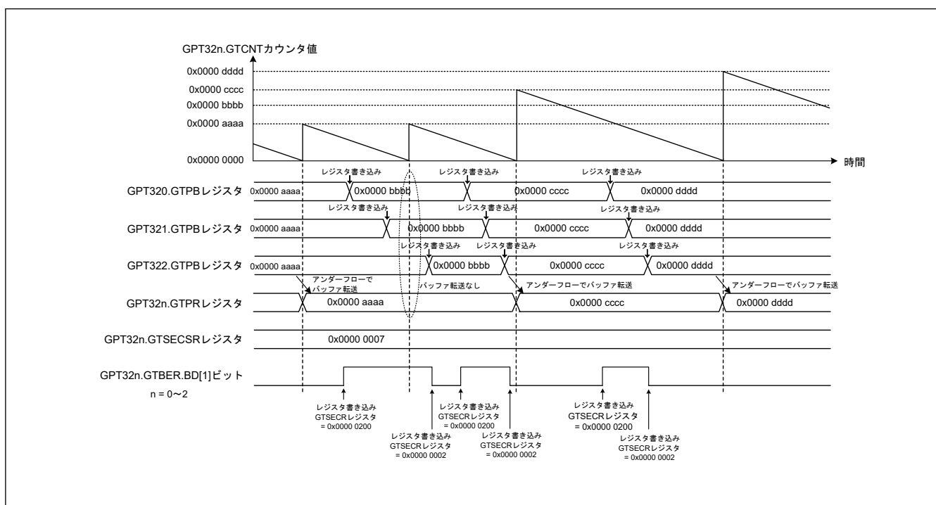
図 21.65 バッファ動作禁止の複数チャンネルの動作例（のこぎり波、シングルバッファ動作）
