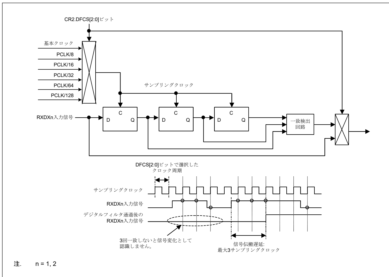
図 27.112 デジタルフィルタ機能の動作例
