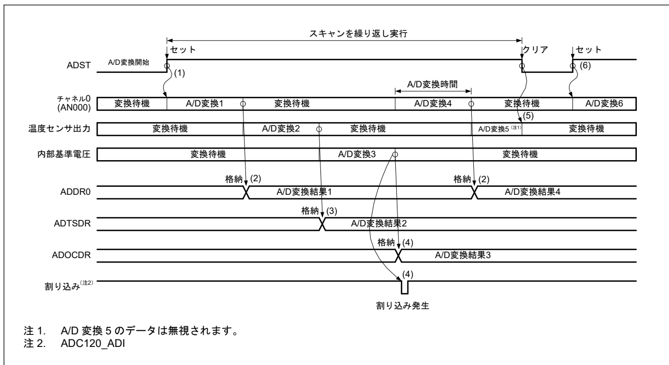
図 37.14 連続スキャンモードの基本動作例 (AN000、温度センサ出力または内部基準電圧選択)
