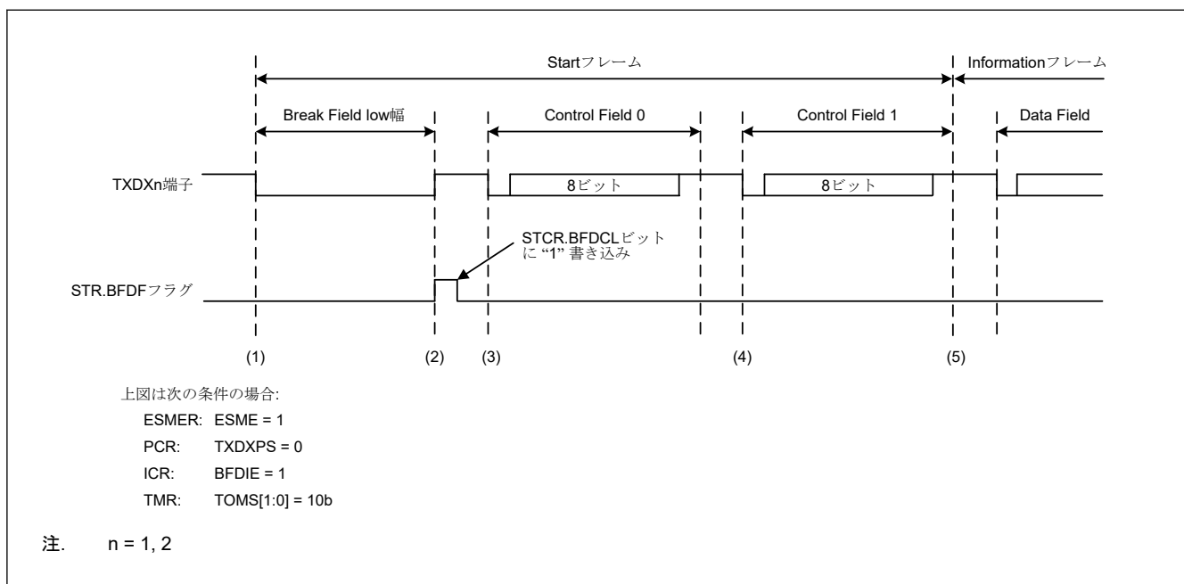
図 27.102 Start Frame 送信時の動作例
