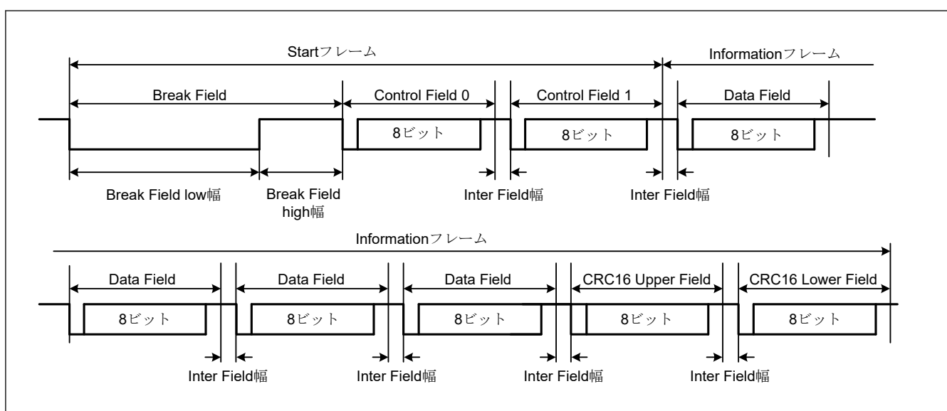
図 27.101 拡張シリアルモード制御部シリアル通信プロトコル
