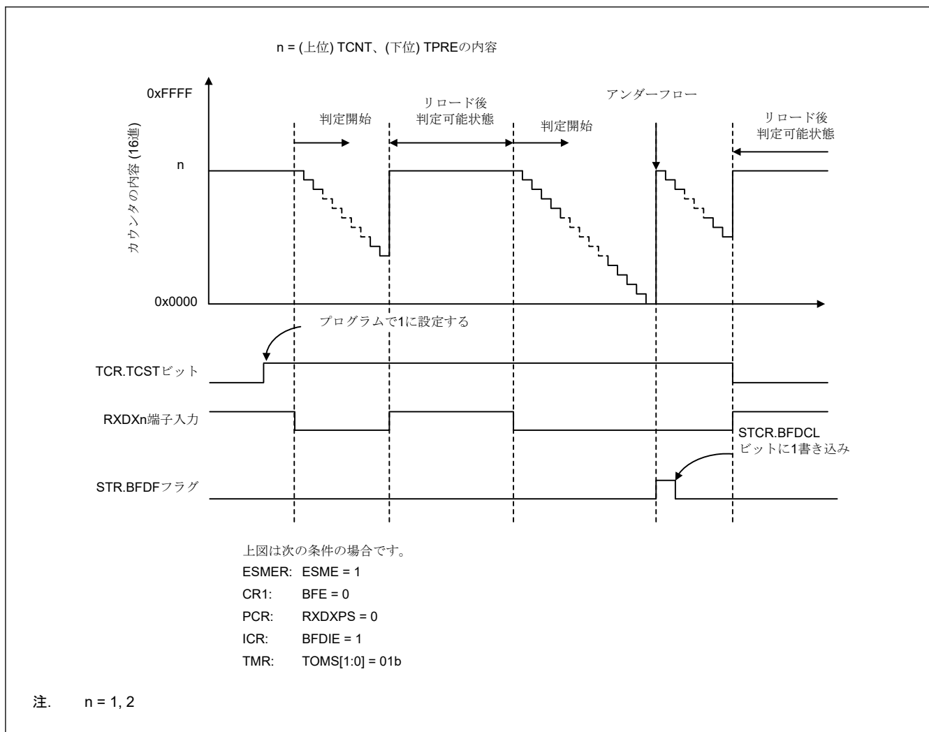
図 27.116 Break Field Low width 判定モードの動作例
