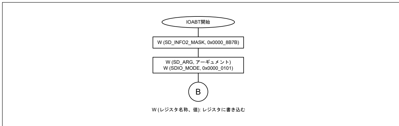
図 33.17 CMD53 マルチブロックリード時に CMD52 (SDIO abort) が送信される場合のフロー
