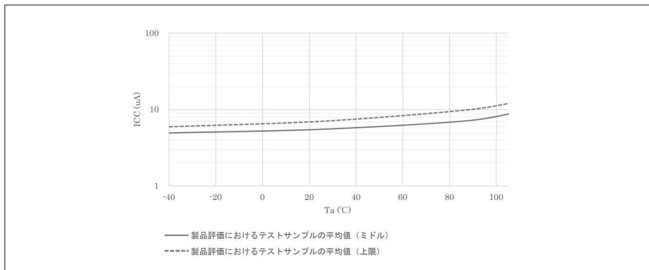
図 47.5 ディープソフトウェアスタンバイモード時の温度依存性、SRAM および USB レジューム検出部への電源供給なし、パワーオンリセット回路、低消費電力機能有効（参考データ）
