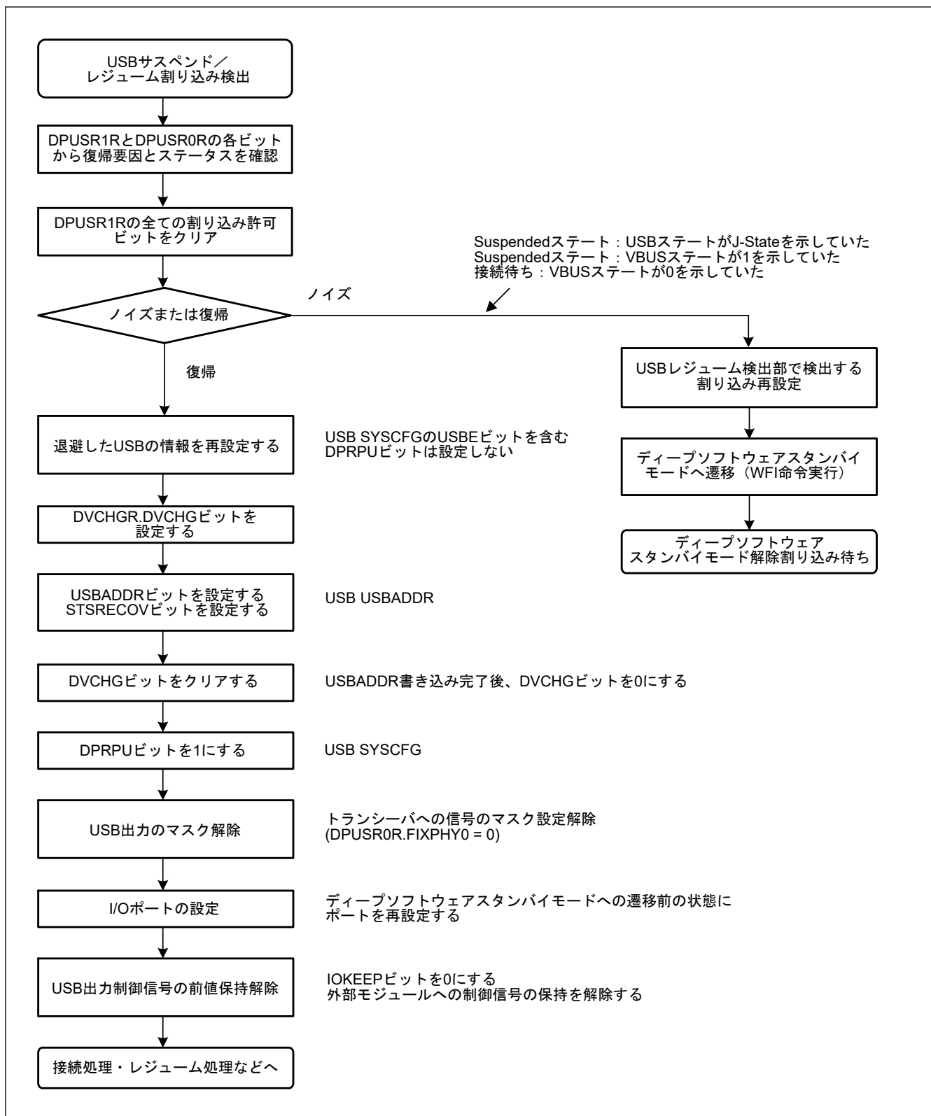
図 26.10 デバイスコントローラ機能選択時におけるディープソフトウェアスタンバイモード解除時のUSBFS 設定フロー
