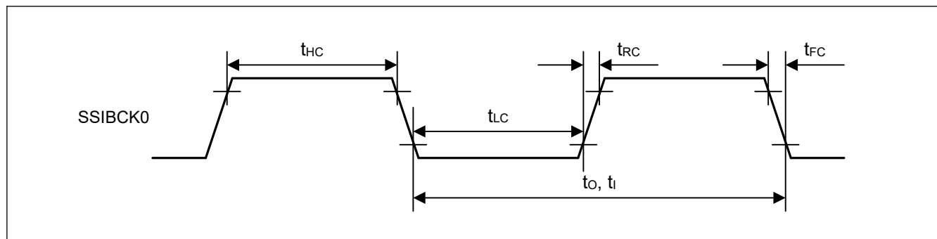
図 47.44 SSIE クロック入出力タイミング
