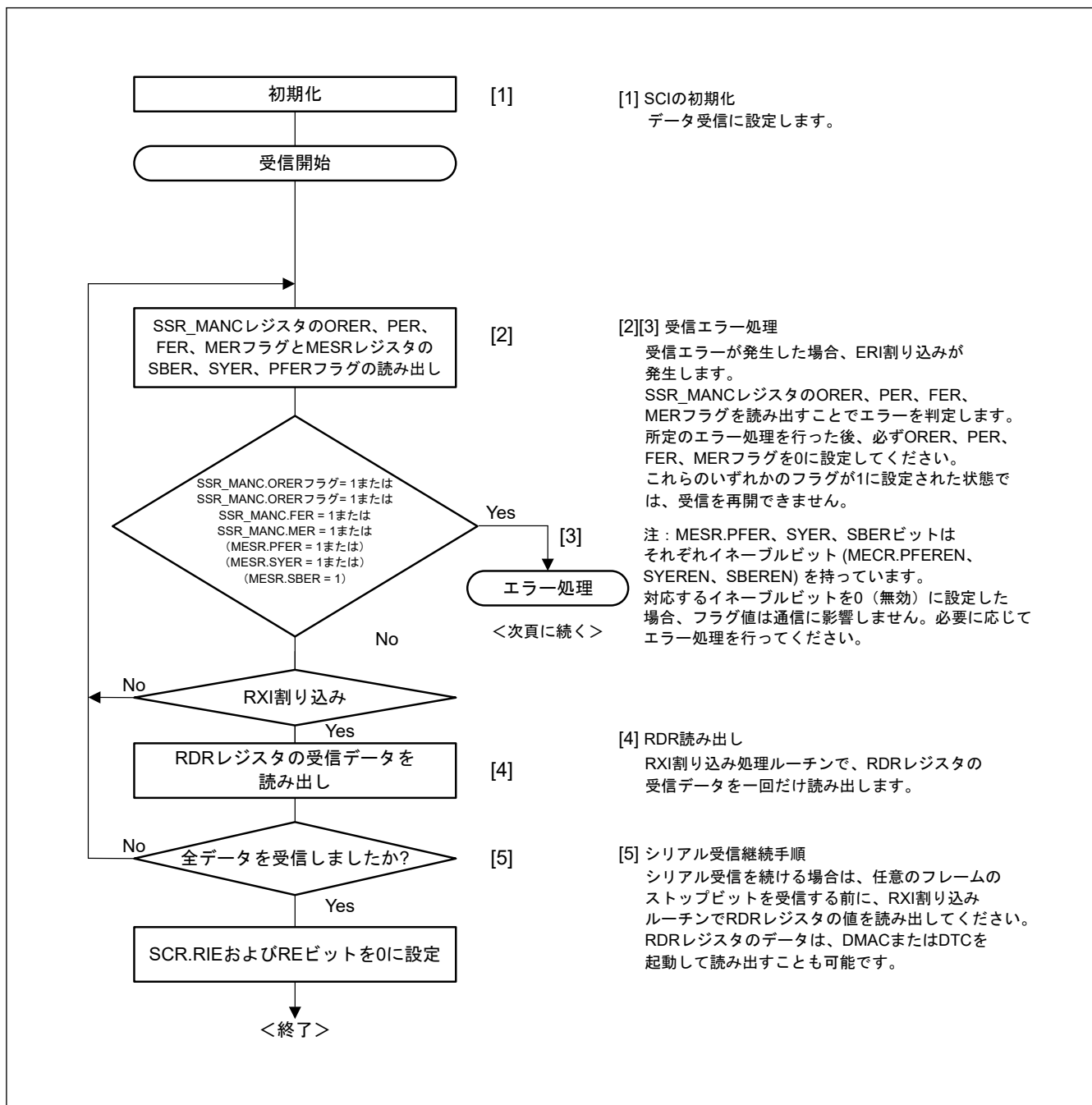
図 27.61 マンチェスタモードにおけるシリアルデータ受信フローチャートの例（正常受信）
