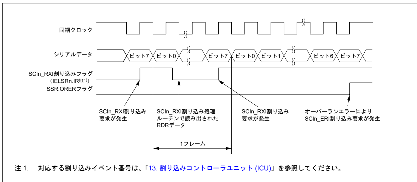
図 27.71 クロック同期式モードにおけるシリアル受信の動作例 (1) (RTS 機能を使用しない場合)
