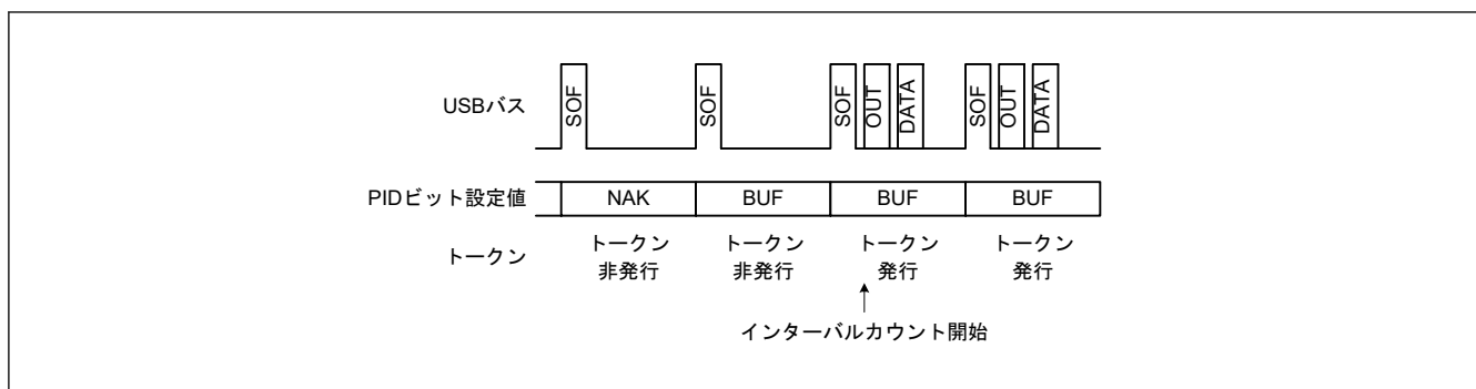
図 26.17 IITV[2:0] = 0 の場合のトークン発行の有無
