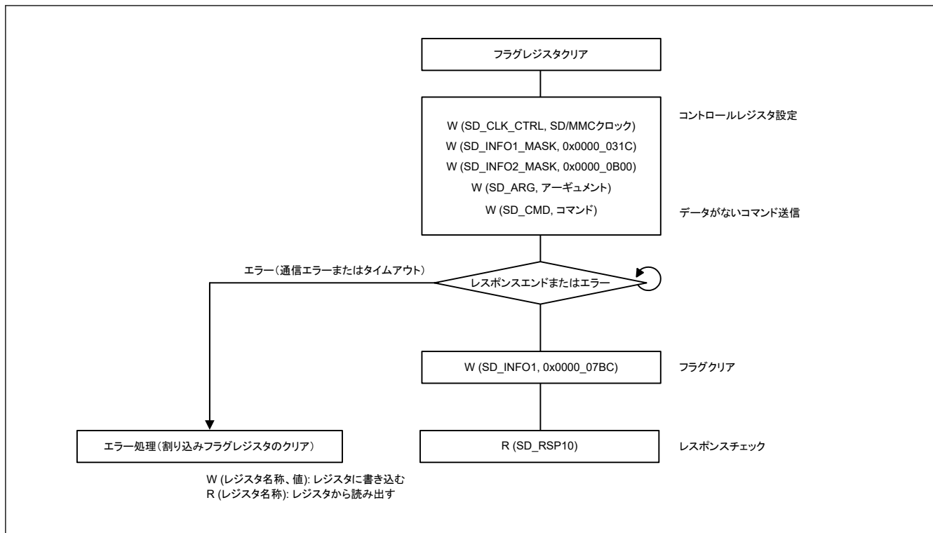
図 33.9 データがないコマンドのフロー例
