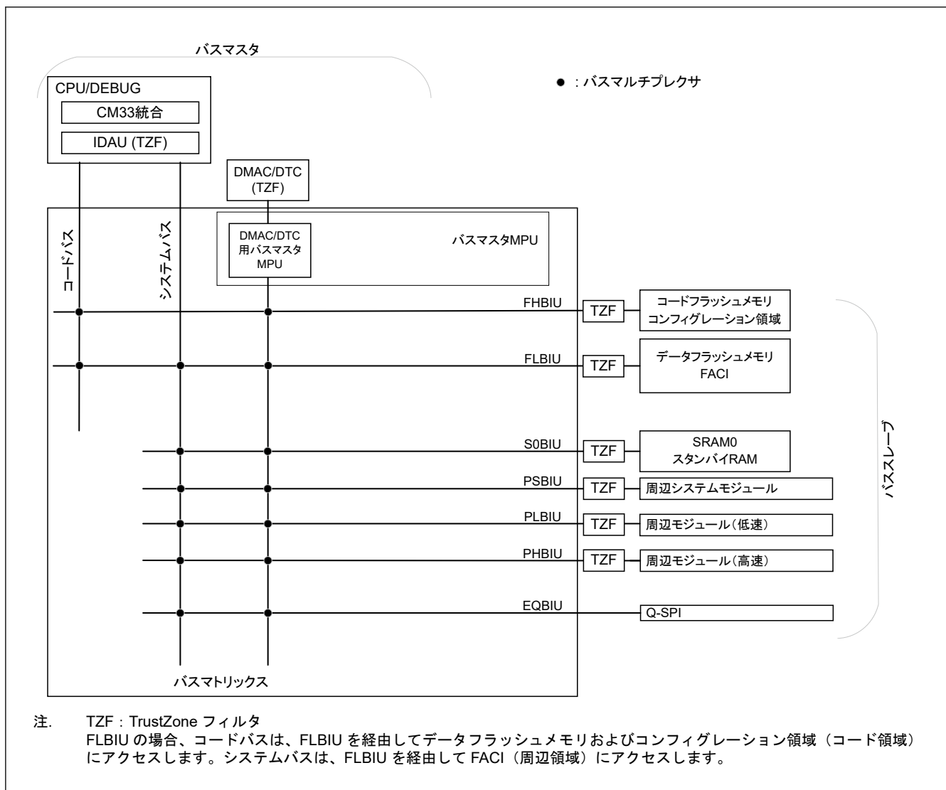
図 14.1 バス接続
