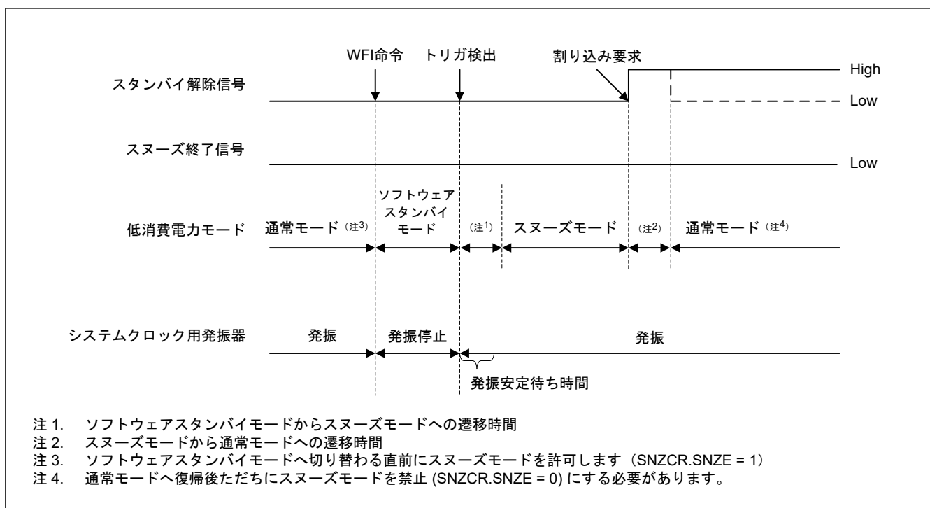
図 10.7 割り込み要求信号が発生する場合のスヌーズモードの解除
