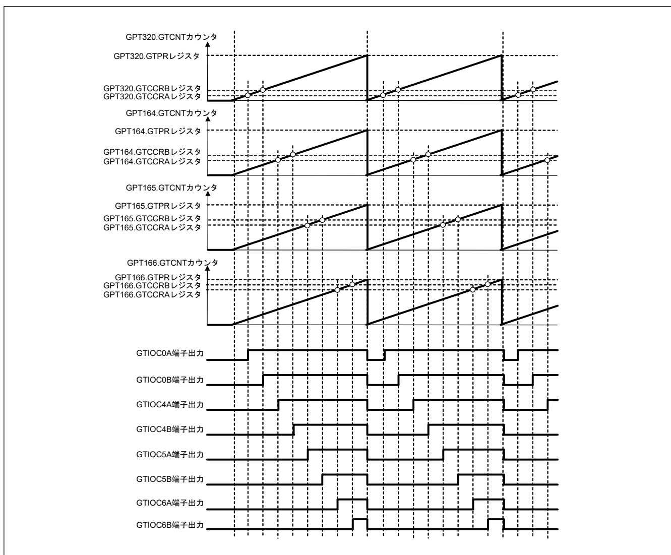
図 21.39 同期 PWM 出力例
