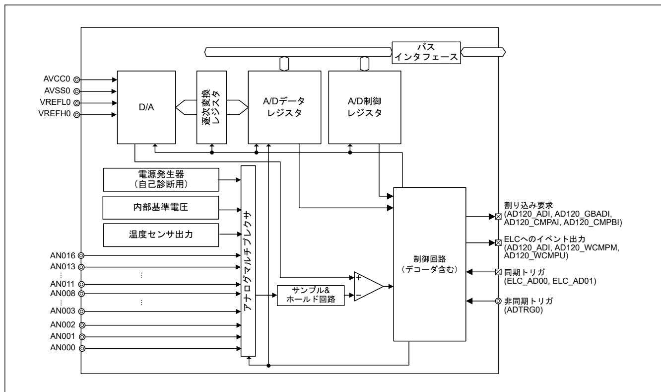
図 37.1 ADC12 のブロック図
