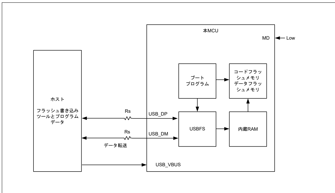
図 44.39 ブートモード（USB インタフェース）のシステム構成図
