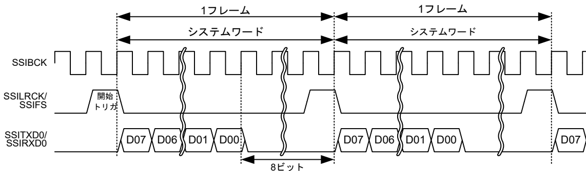
図 32.38 モノラルフォーマットにおけるショートフレーム（パディングあり、システムワード長 > データワード長）
