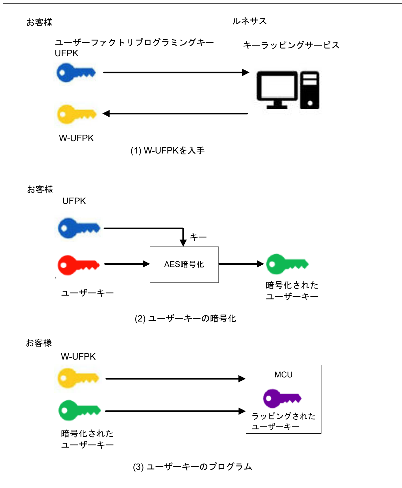
図 46.3 キーインジェクション
