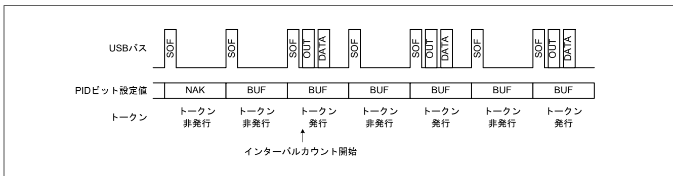
図 26.18 IITV[2:0] = 1 の場合のトークン発行の有無
