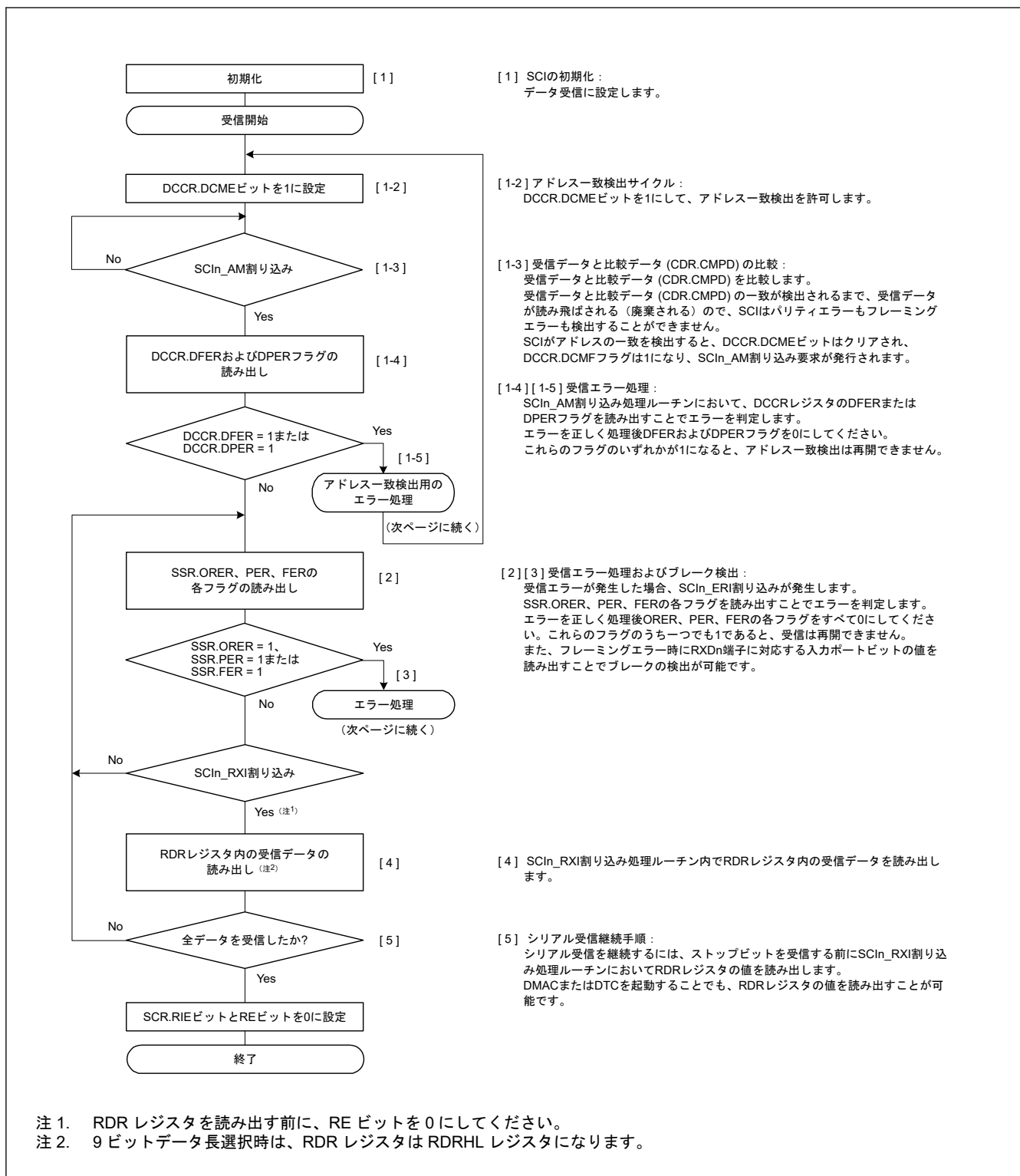
図 27.22 調歩同期式モードにおけるシリアル受信のフローチャート例（非 FIFO 選択、アドレス一致検出有効時） (1)
