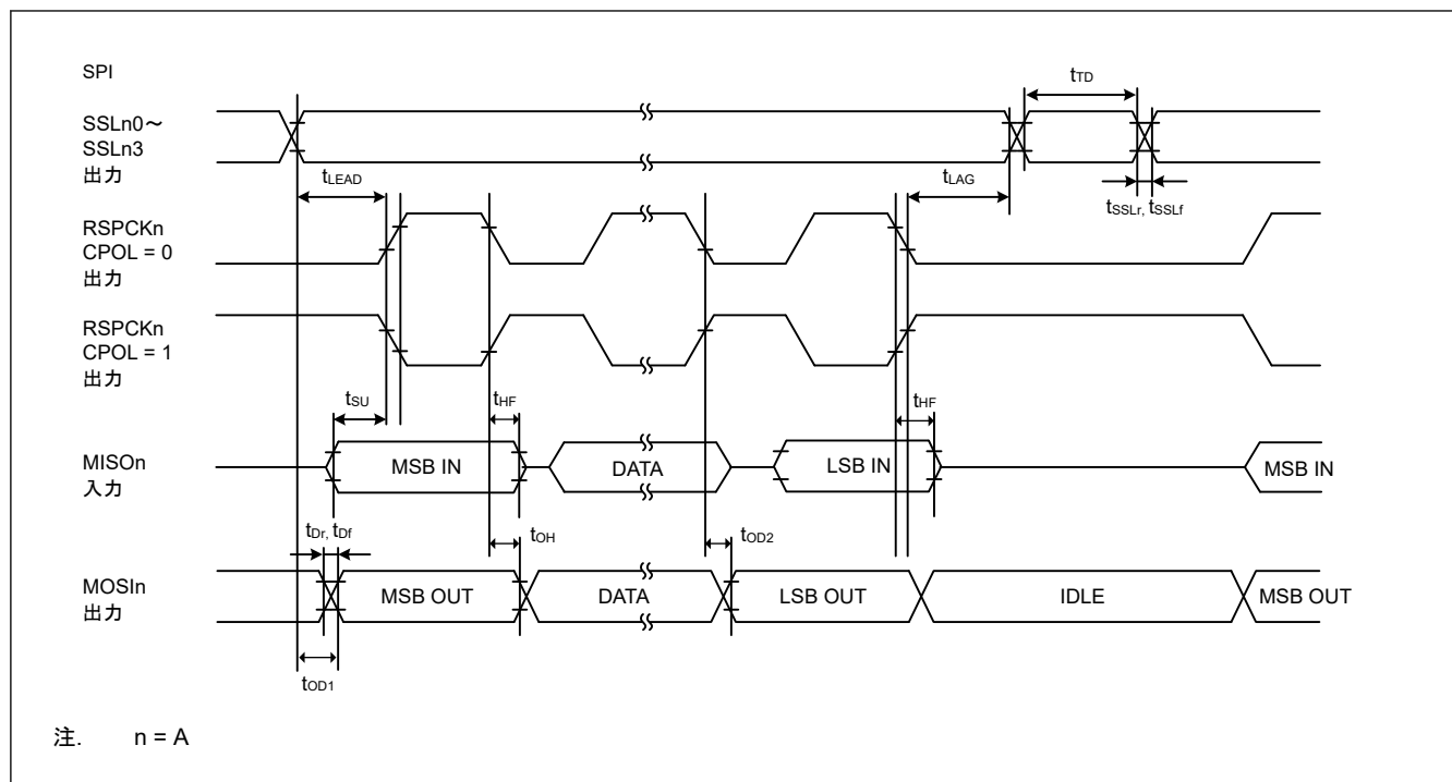
図 47.36 CPHA = 0 でビットレートが PCLKA/2 に設定されている場合におけるマスタの SPI タイミング
