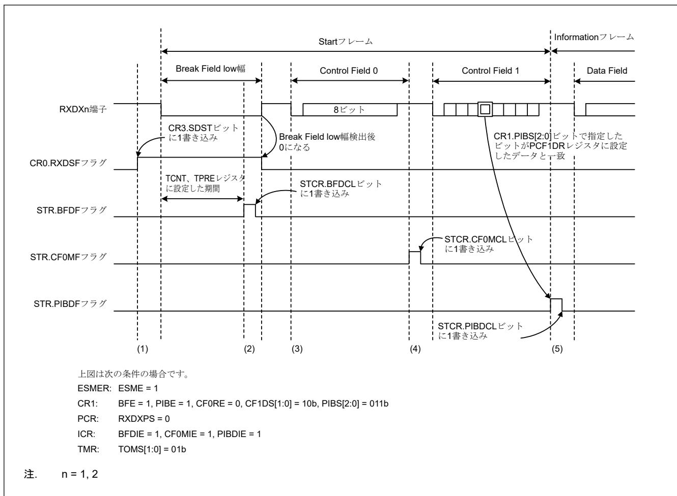
図 27.110 Start Frame の受信時の動作例（プライオリティインタラプトビット使用時）
