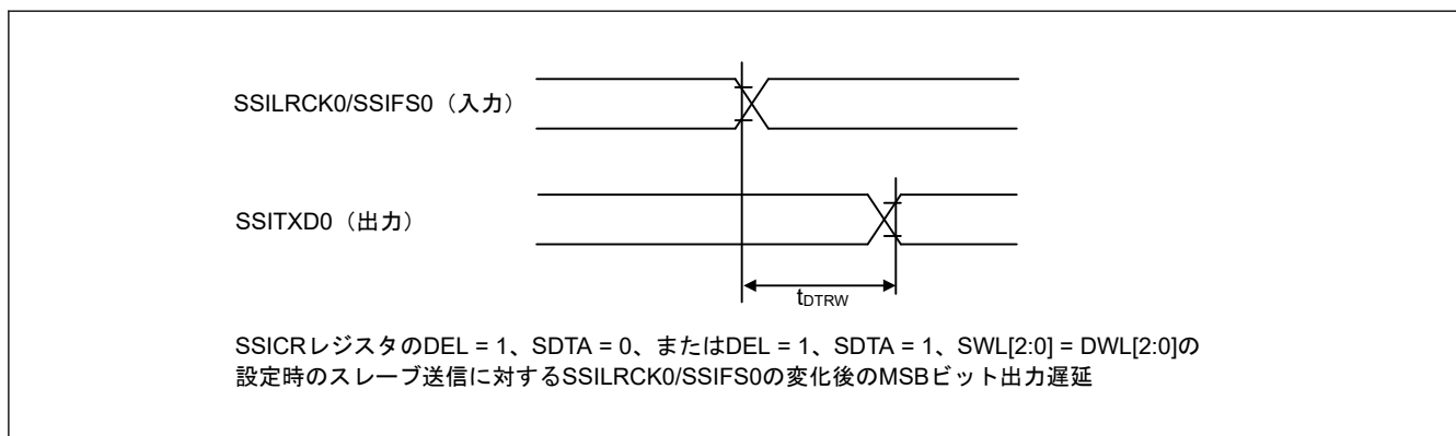
図 47.48 SSILRCK0/SSIFS0 変化時からの SSIE データ出力遅延
