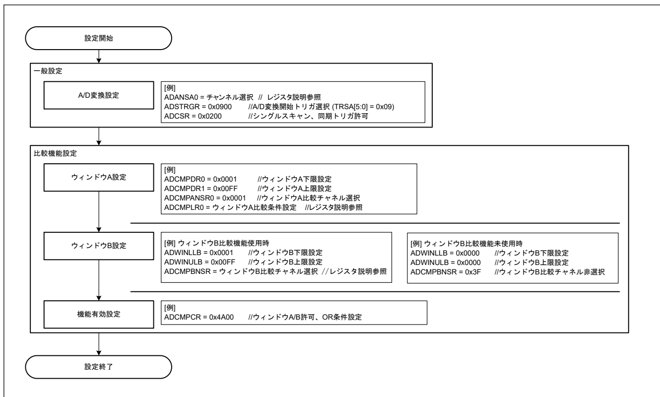
図 37.24 コンペア機能のイベント出力使用時の設定例
