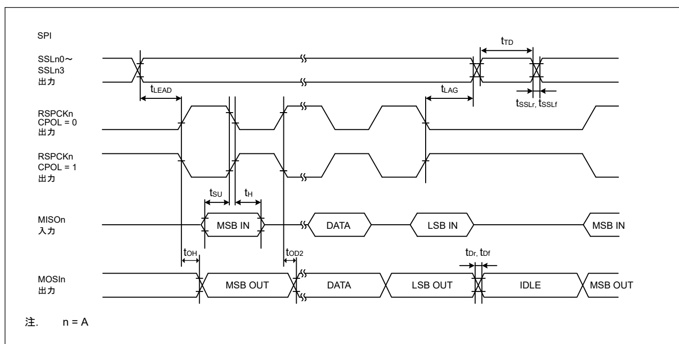
図 47.37 CPHA = 1 の場合におけるマスタの SPI タイミング
