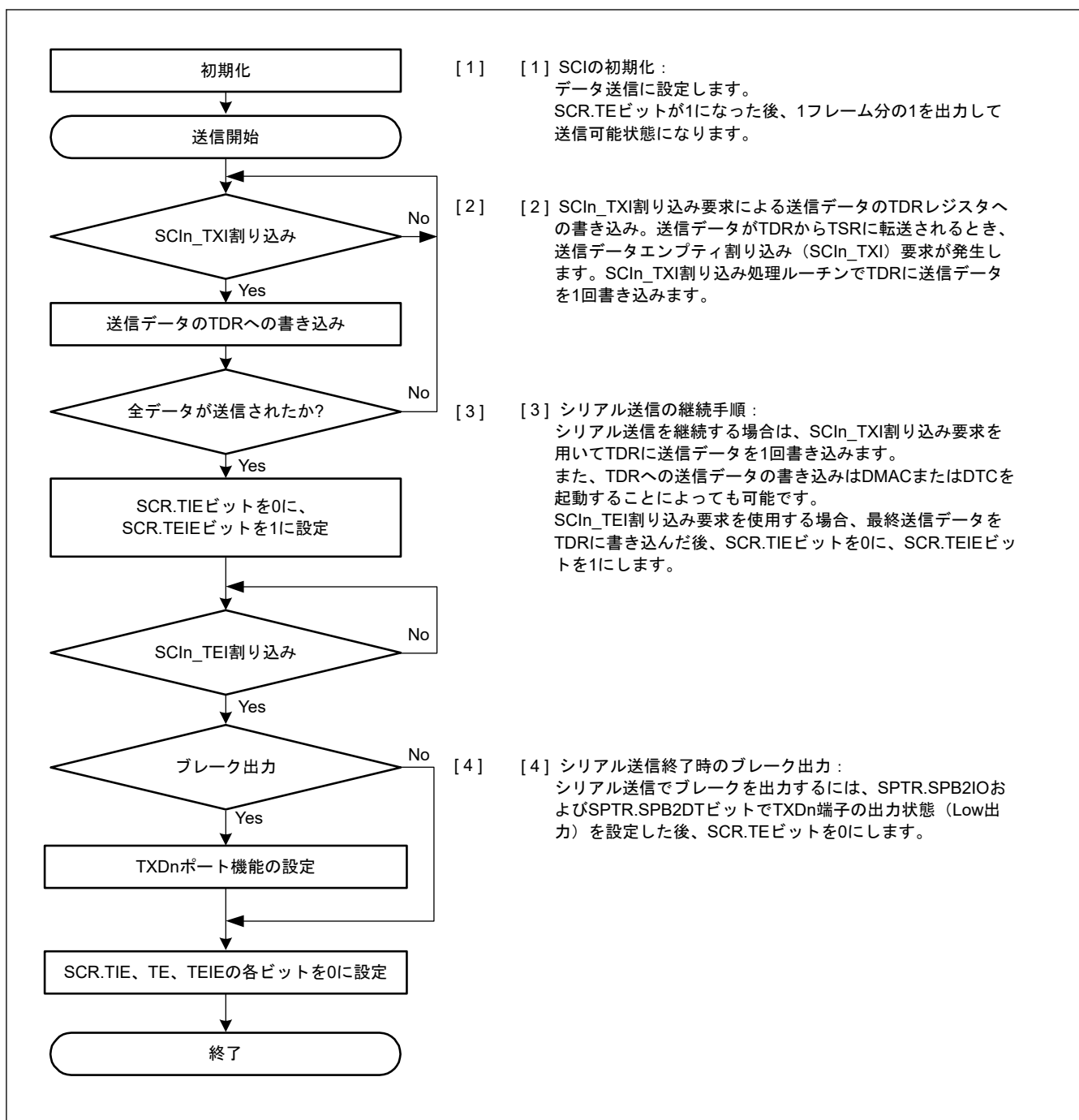
図 27.15 調歩同期式モードにおけるシリアル送信のフローチャート例（非 FIFO 選択時）
