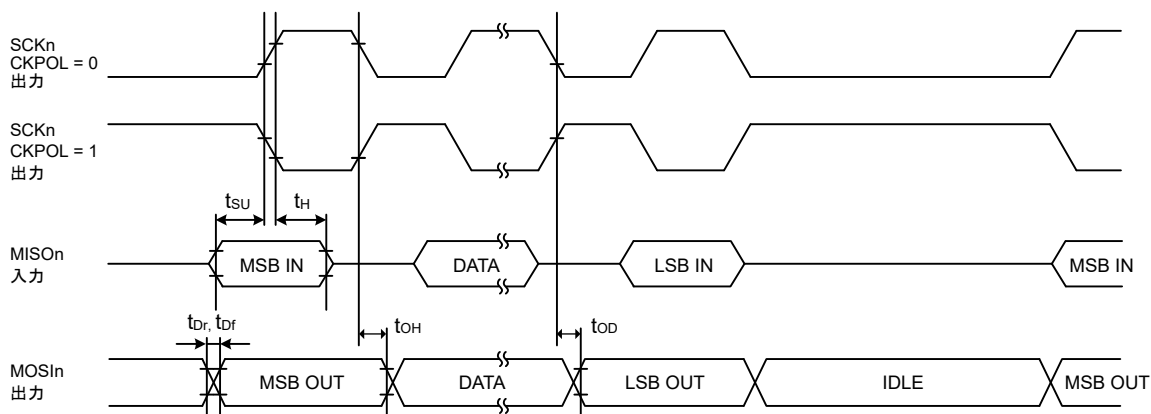
図 47.29 CKPH = 1 の場合におけるマスタの SCI 簡易 SPI モードタイミング
