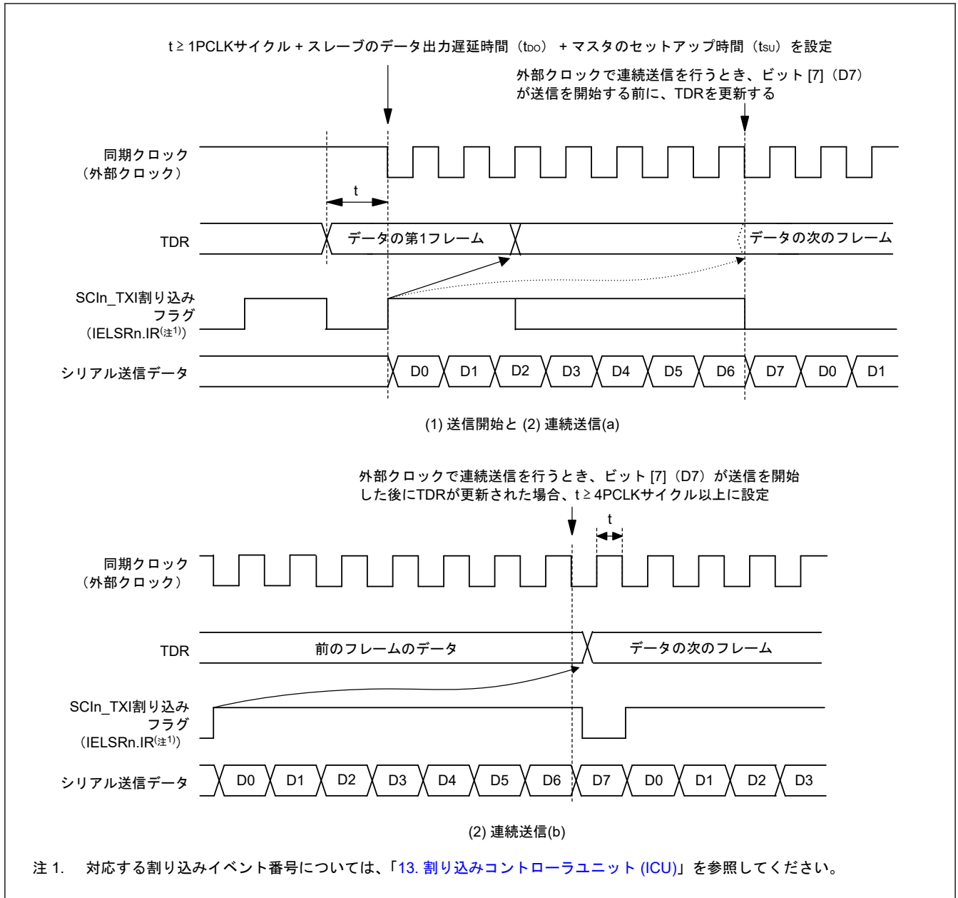
図 27.123 クロック同期式送信時の外部クロック使用に関する制約事項
