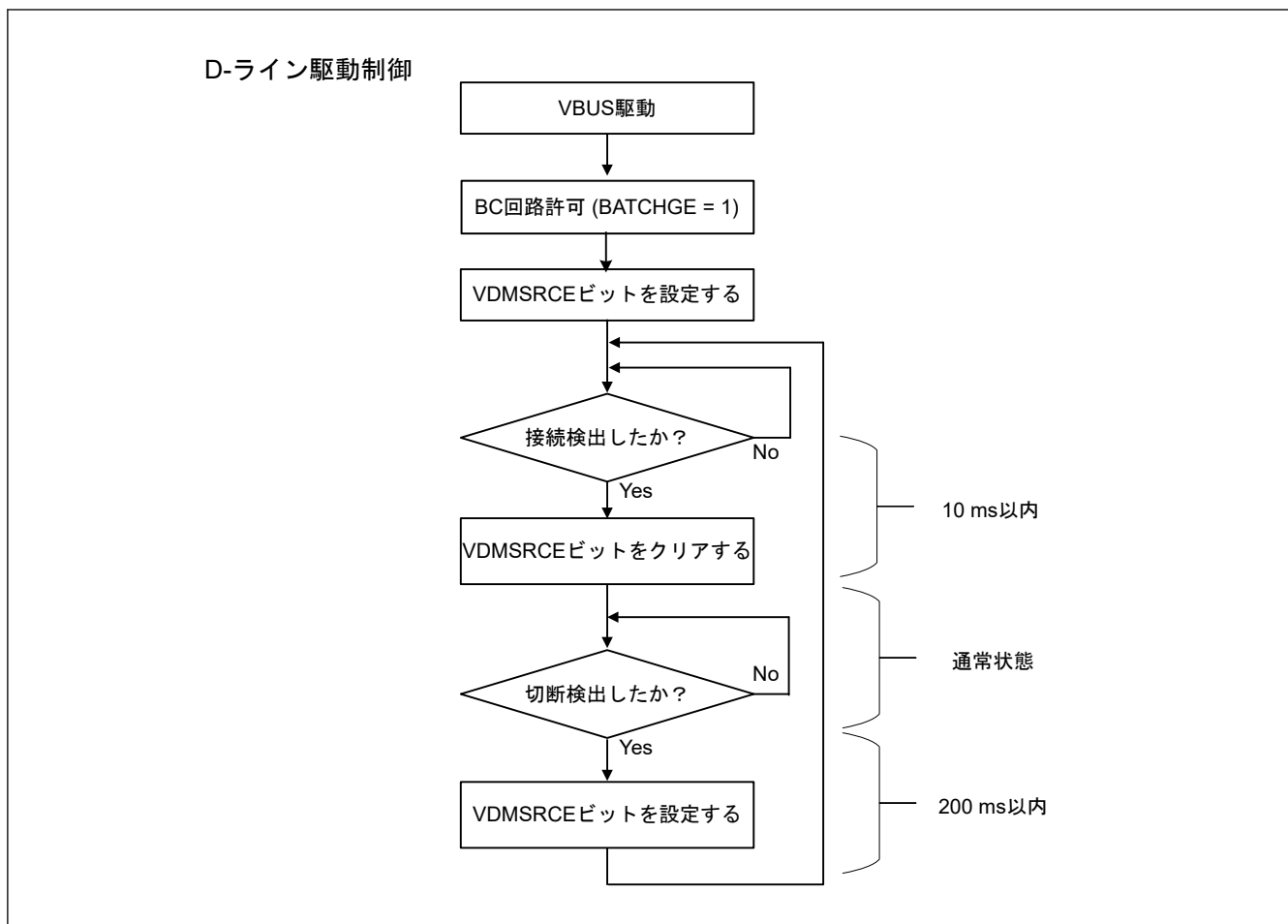
図 26.26 ポータブルデバイス検知機能を使用しない場合の処理フロー（ステップ a、b）
