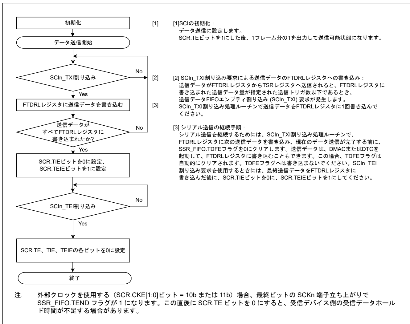
図 27.70 クロック同期式モードにおけるシリアル送信のフローチャート例 (FIFO 選択時)
