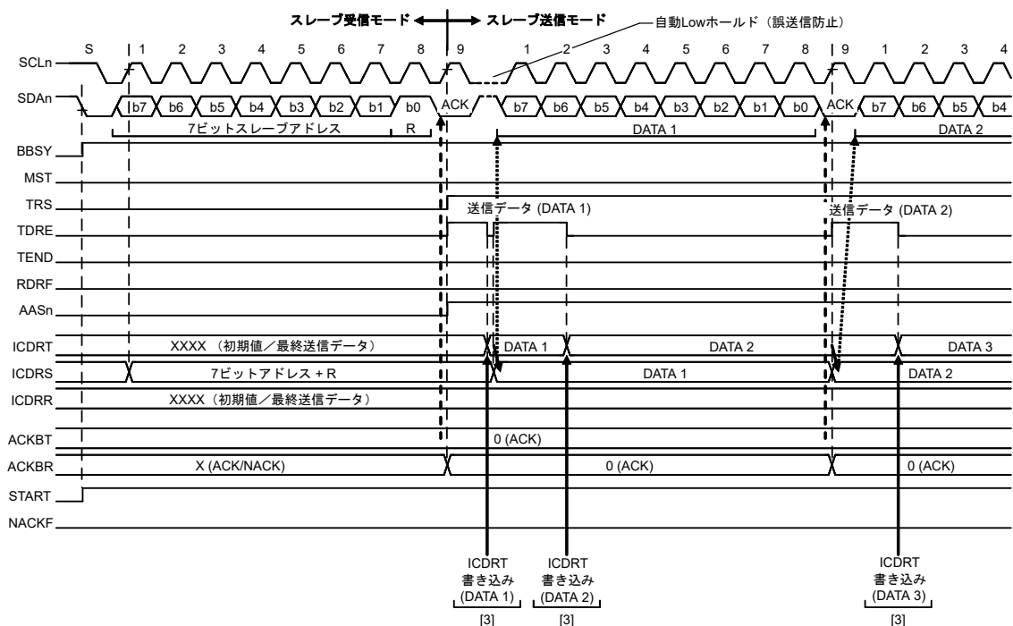
図 28.16 スレープ送信の動作タイミング (1) (7ビットアドレスフォーマット)
