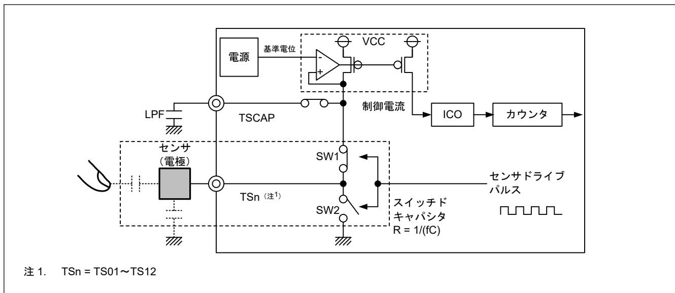
図 40.4 計測部回路
