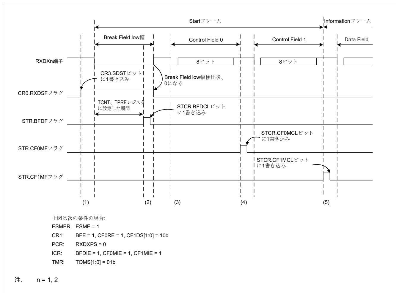
図 27.106 Start Frame 受信時の動作例
