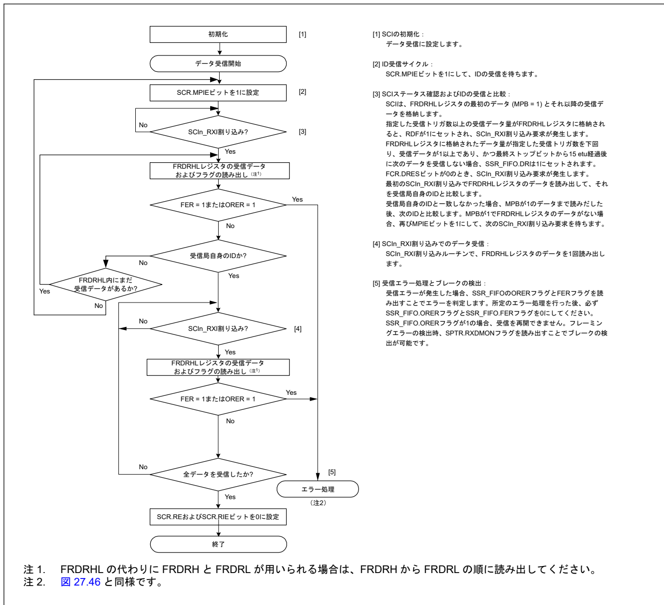
図 27.48 マルチプロセッサモードにおけるシリアル受信のフローチャート例 (FIFO 選択時)
