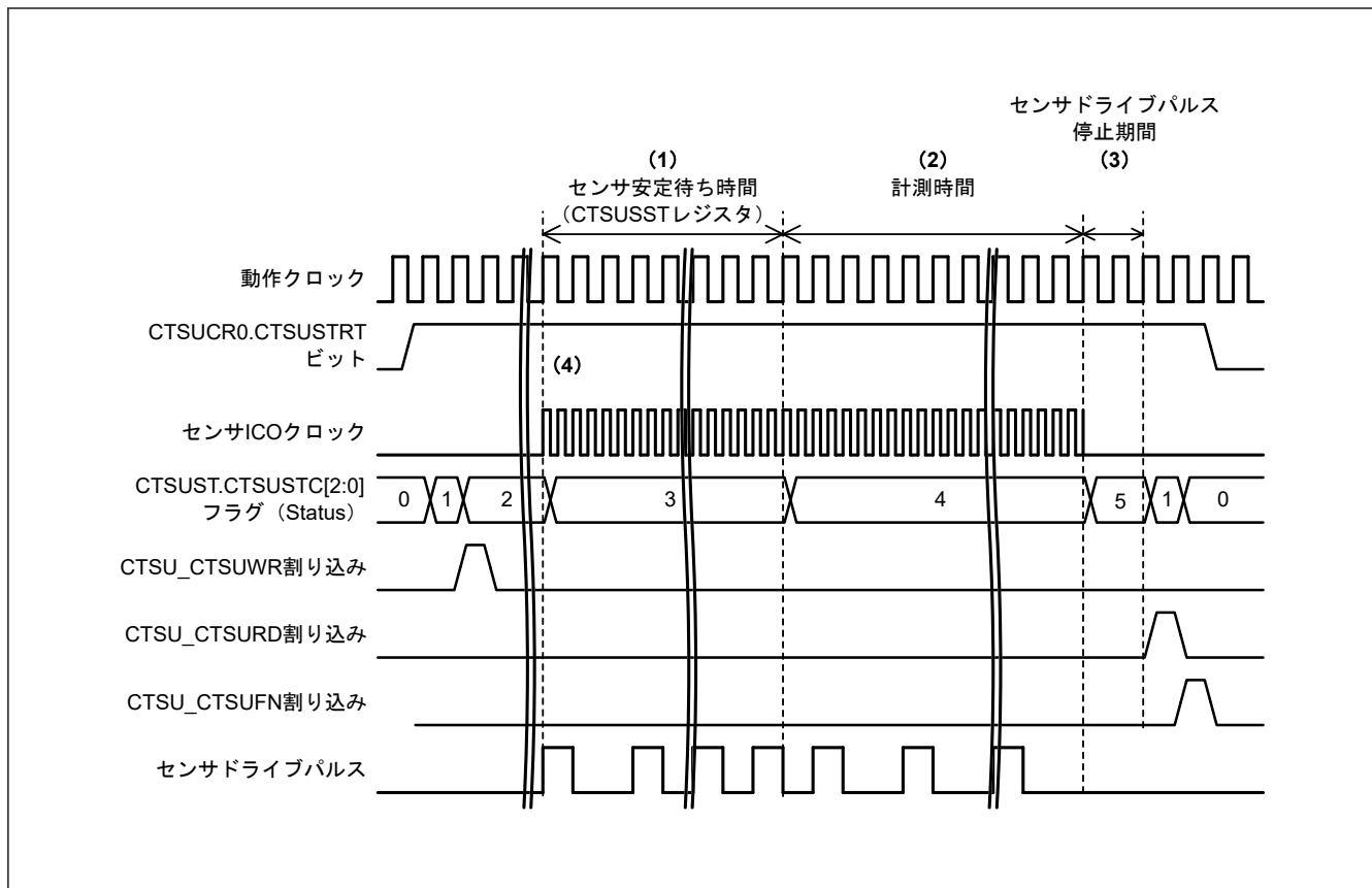
図 40.18 センサ安定待ちと計測のタイミング
