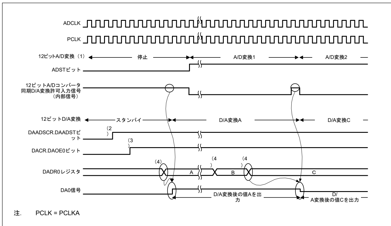
図 38.3 DAC12 を次に同期して変換する例 : ADC12
