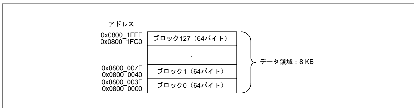
図 44.3 データフラッシュメモリのマップ
