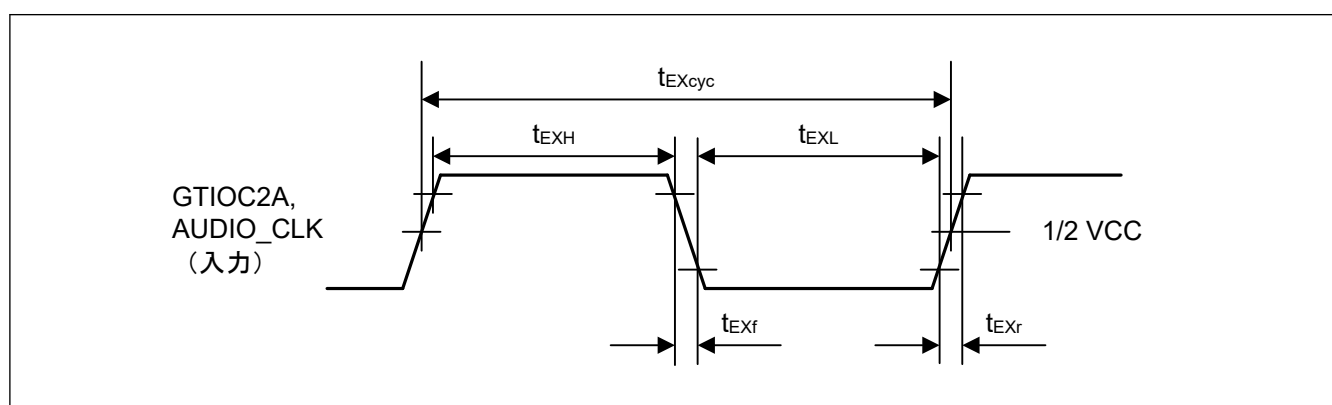
図 47.45 クロック入力タイミング
