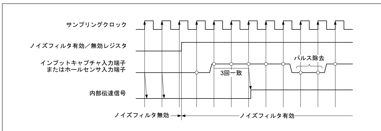
図 21.63 ノイズフィルタのタイミング
