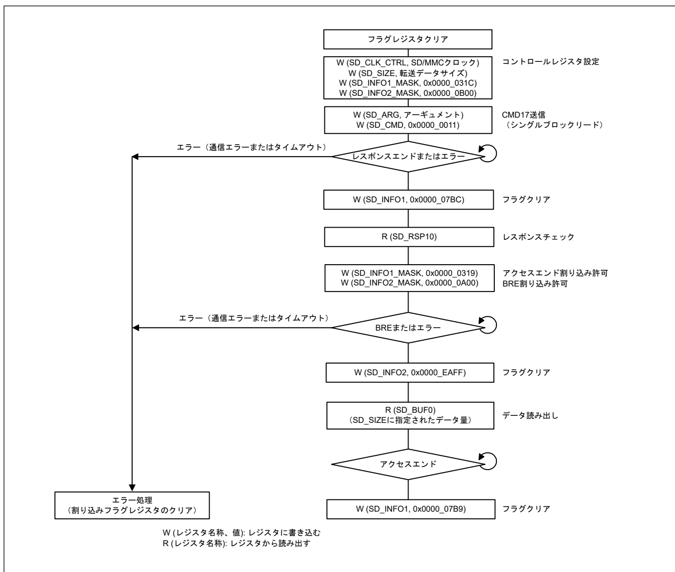
図 33.10 シングルブロックリード動作のフロー例
