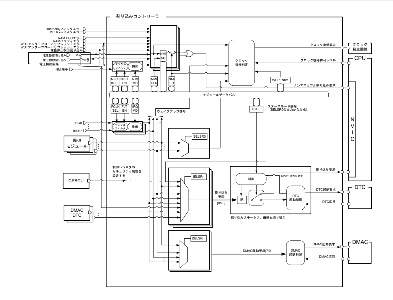
図 13.1 ICU のブロック図
