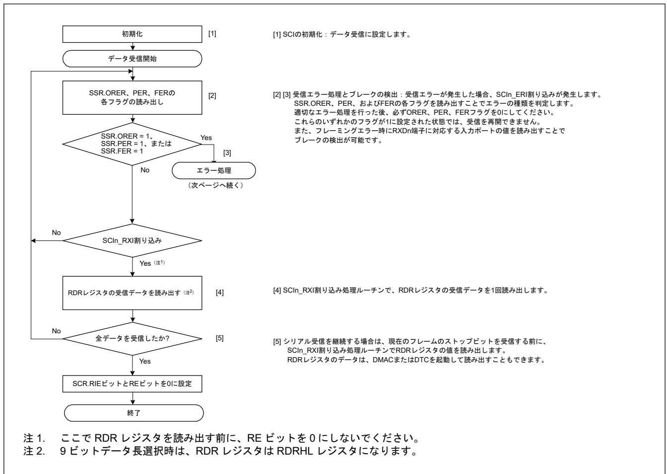
図 27.20 調歩同期式モードにおけるシリアル受信のフローチャート例（非 FIFO 選択、アドレス一致検出無効時） (1)
