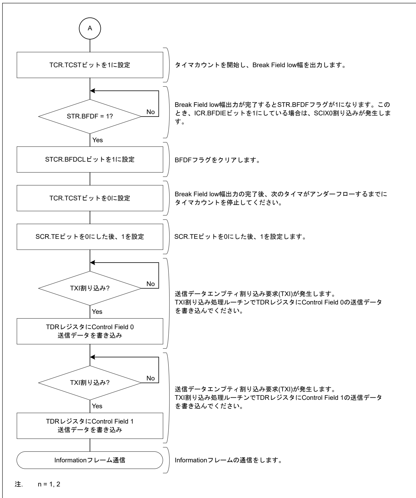
図 27.104 Start Frame 送信フローチャート例 (2/2)
