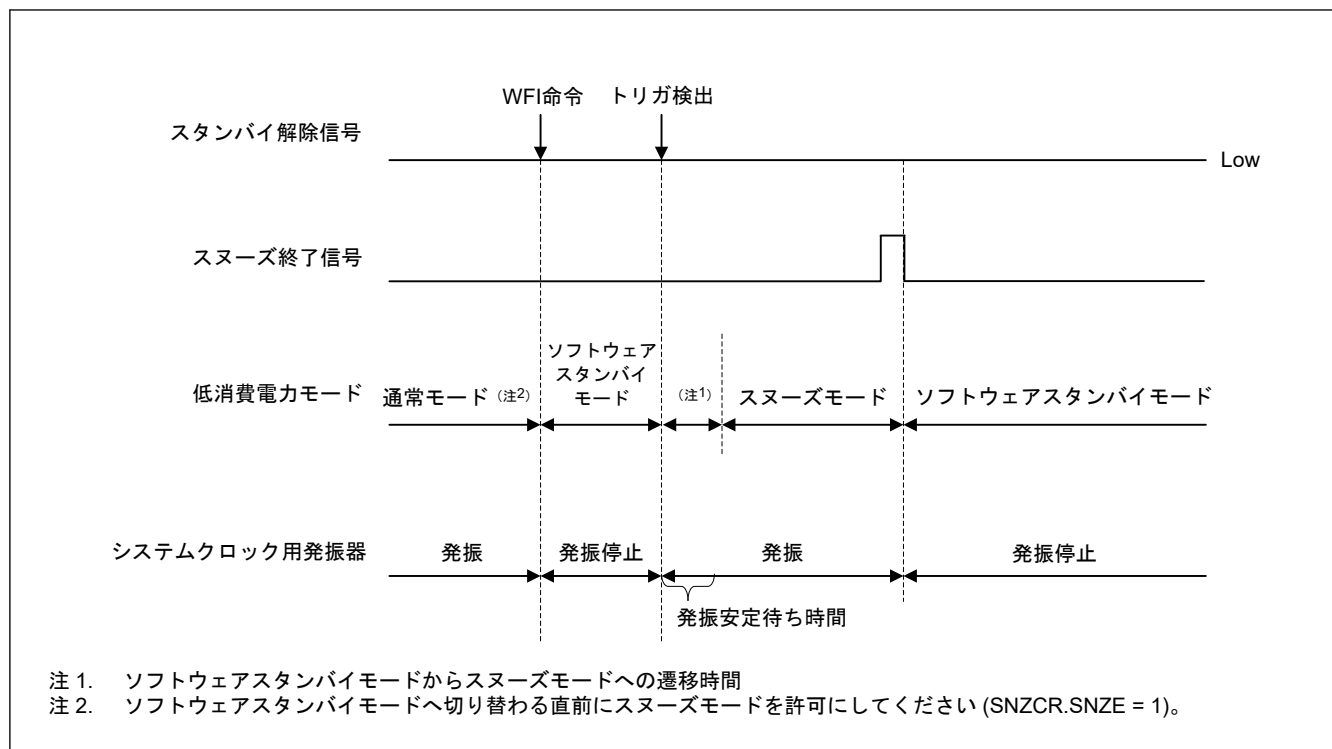
図 10.8 割り込み要求信号が発生しない場合のスヌーズモードの解除
