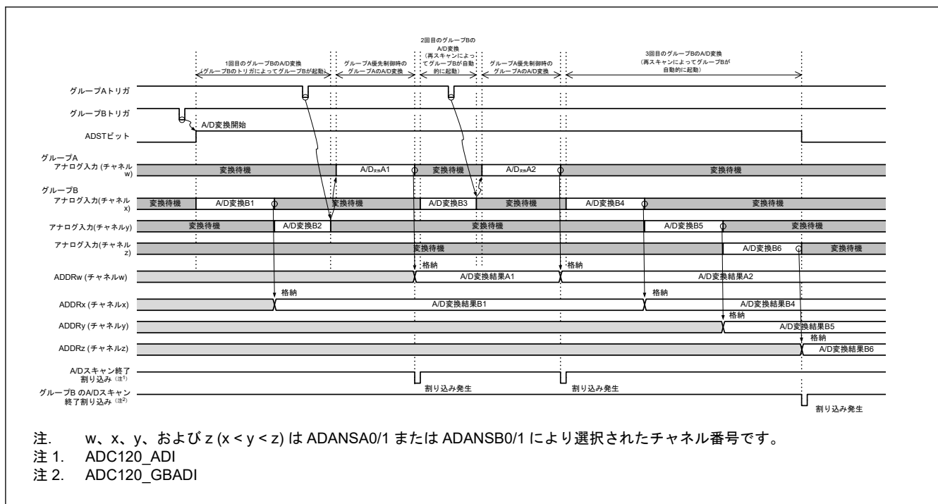
図 37.19 グループ優先動作の例 1-2: グループ B 再スキャン中のグループ A トリガ入力、再スキャンあり (ADGSPCR.GBRSCN = 1、ADGSPCR.GBRP = 0、および ADGSPCR.LGRRS = 0 の場合)
