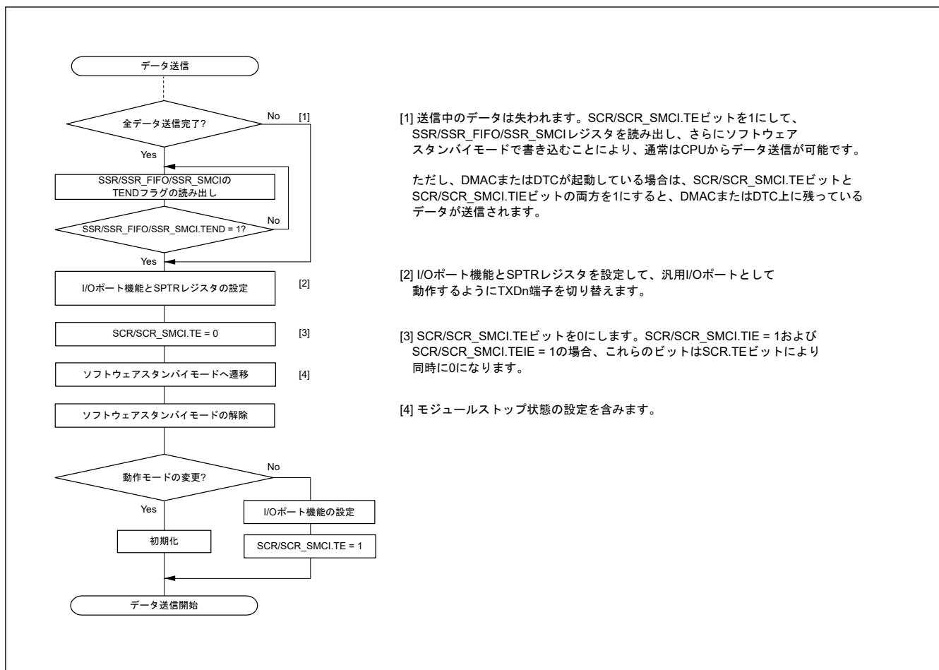
図 27.118 送信中にソフトウェアスタンバイモードへ遷移する場合のフローチャート例
