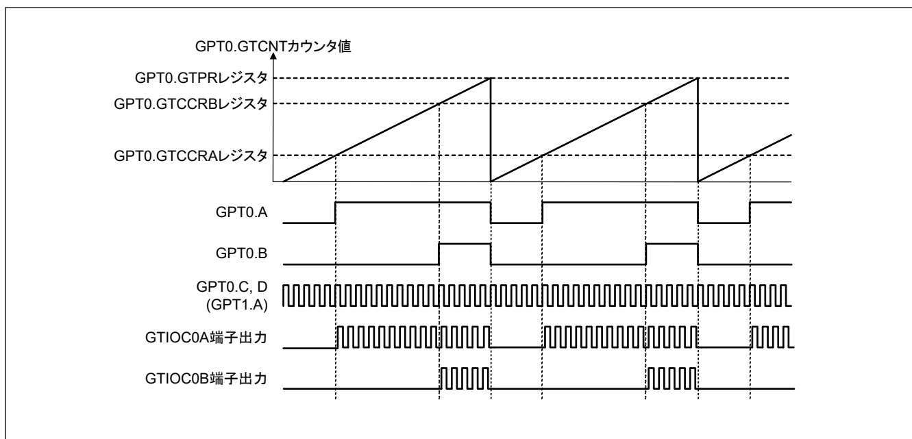
図 21.62 チャンネル間論理演算の例
