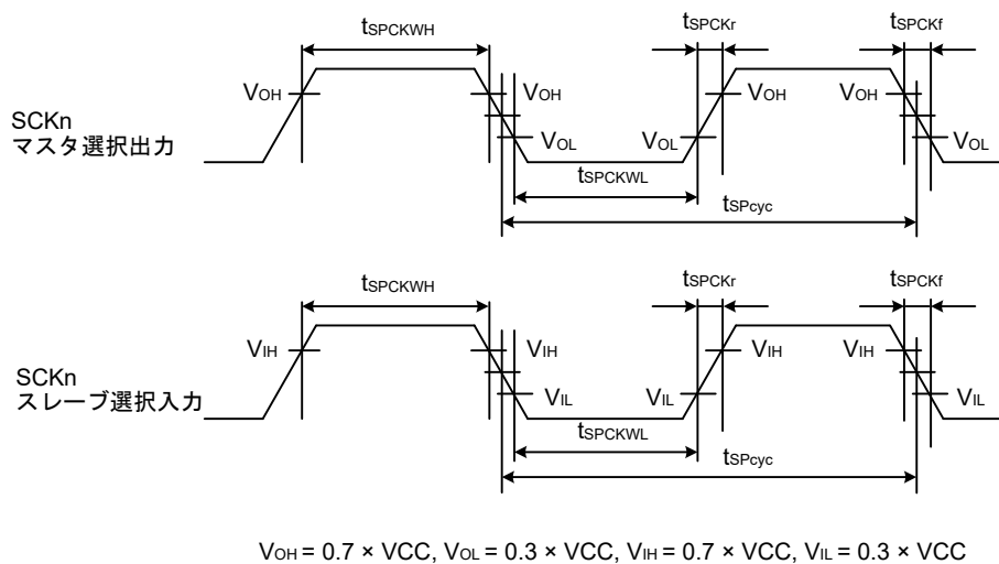
図 47.28 SCI 簡易 SPI モードクロックタイミング
