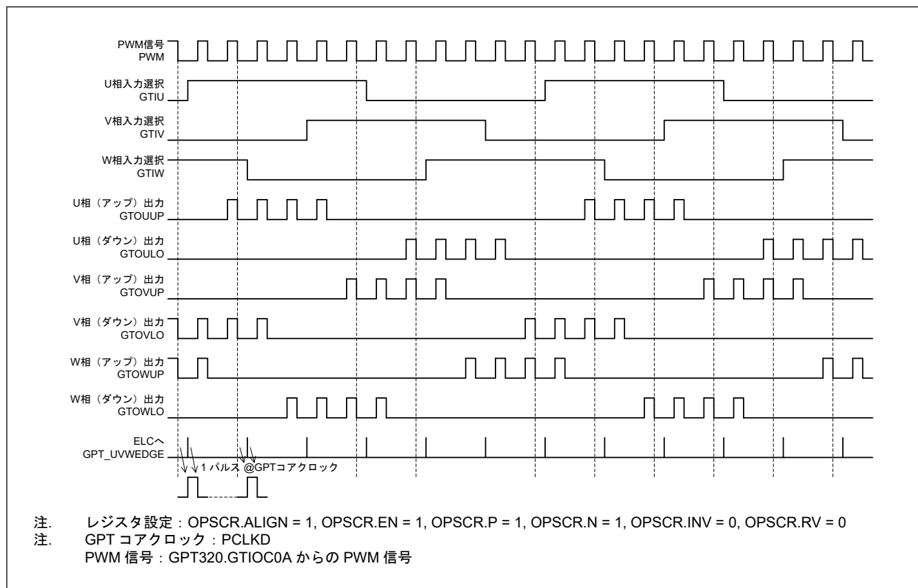
図 21.59 6 相 PWM 出力動作例 (チョッパ制御)
