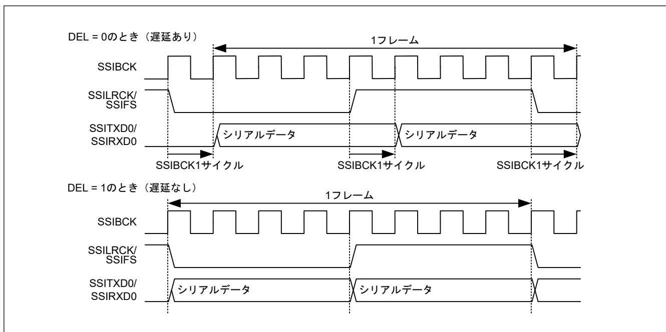
図 32.6 シリアルデータにおける遅延の設定
