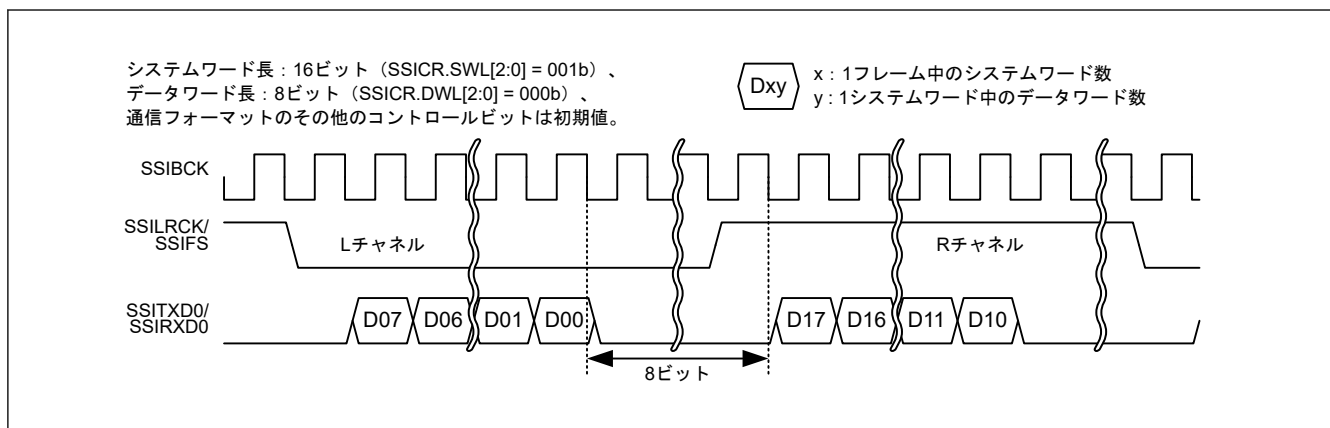
図 32.35 パディングビット転送の例 (I 2 S フォーマット、システムワード長 > データワード長)
