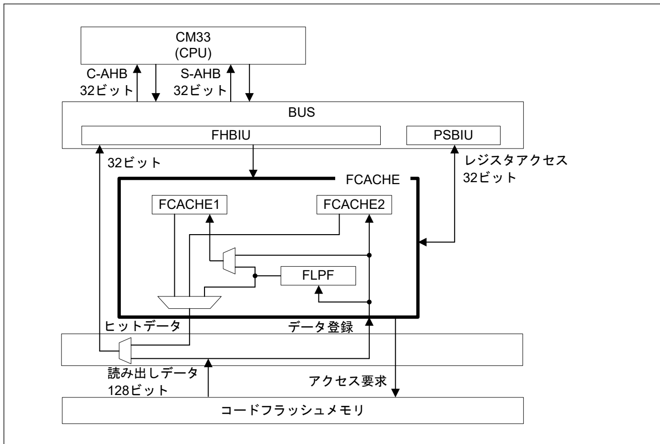
図 44.4 FCACHE のブロック図
