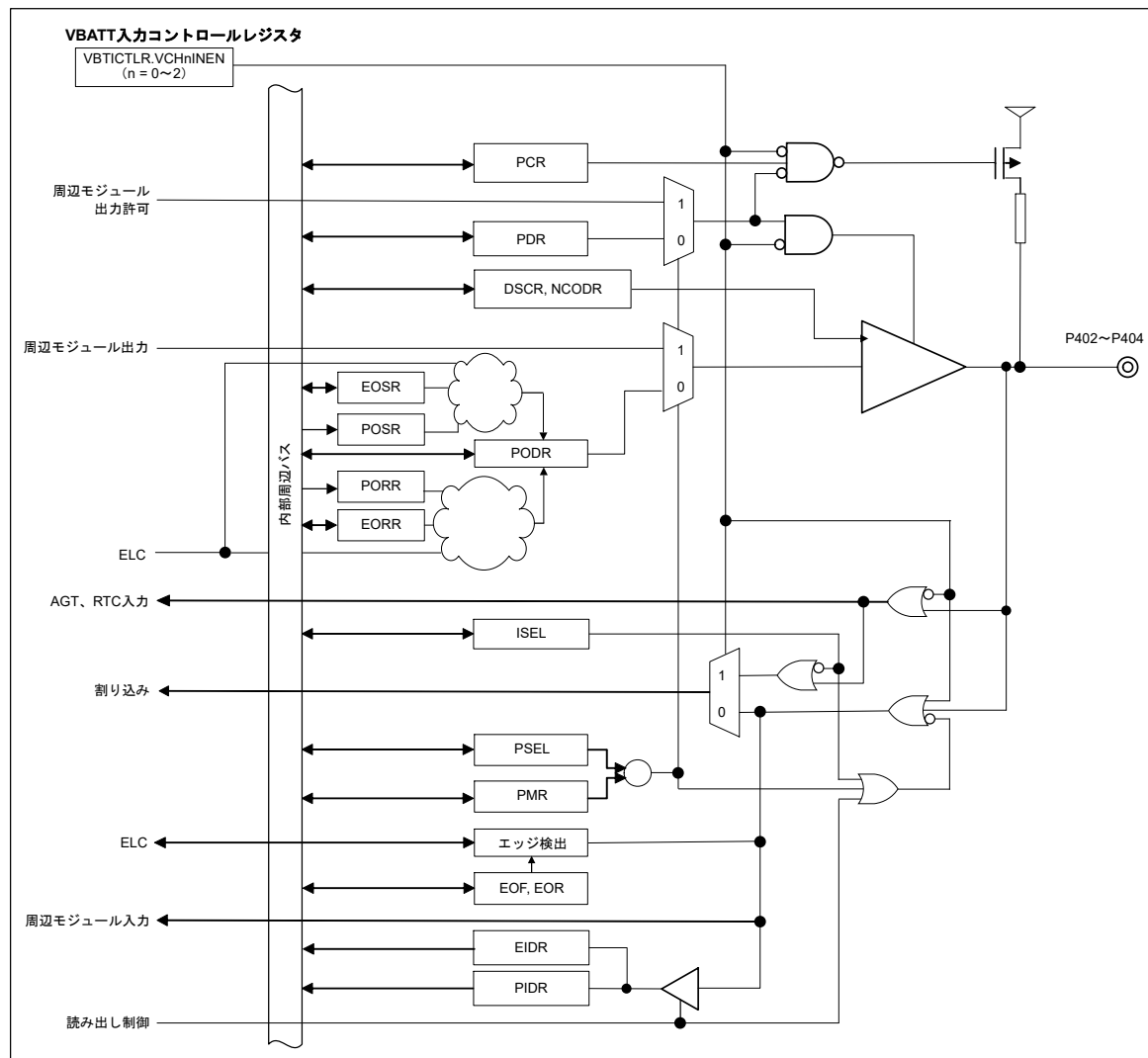
図 19.5 P402、P403、P404 の接続図
