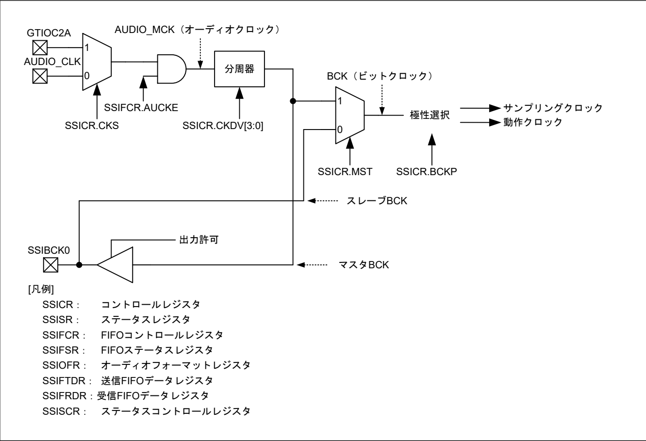
図 32.3 SSIE クロック構成
