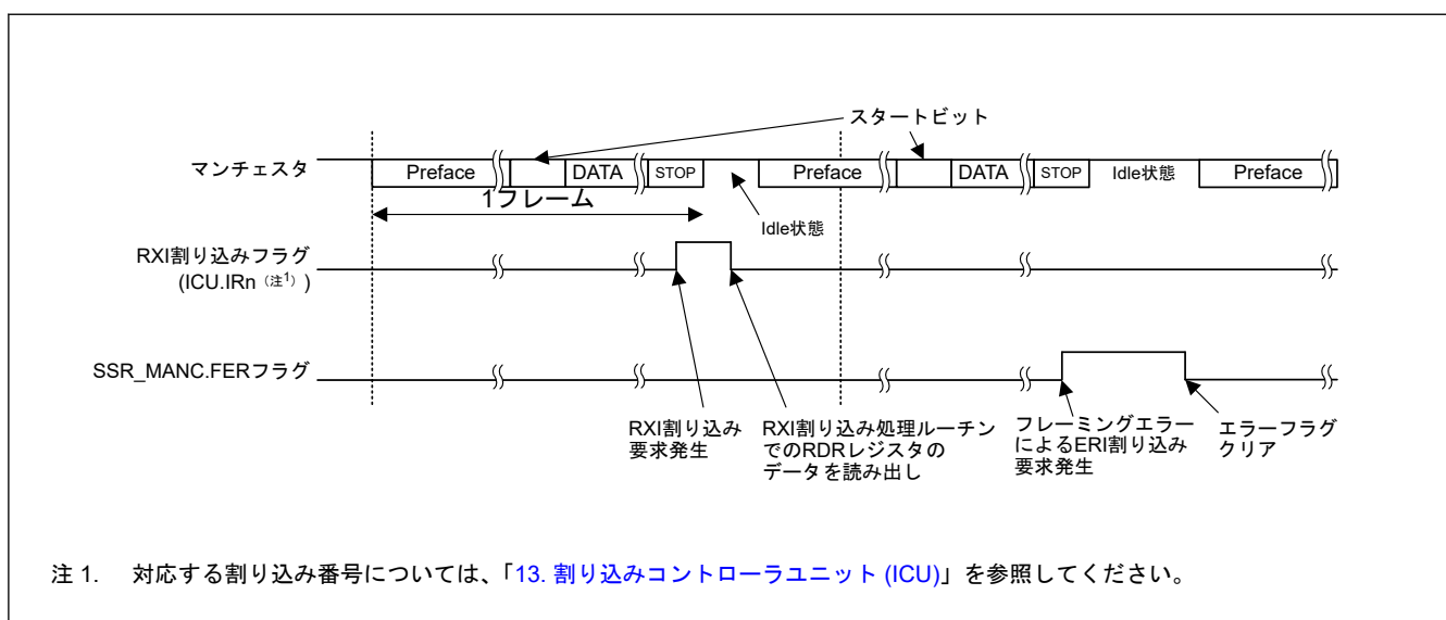
図 27.60 マンチェスタモードにおけるシリアルデータ受信の動作例 (プレフィスあり)
