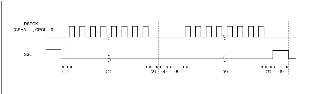
図 30.46 SSLKP ビットを利用したバースト転送の動作例 (BFDS = 0)
