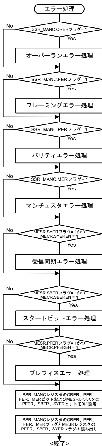
図 27.62 マンチェスタモードにおけるシリアル受信フローチャートの例（エラー処理）
