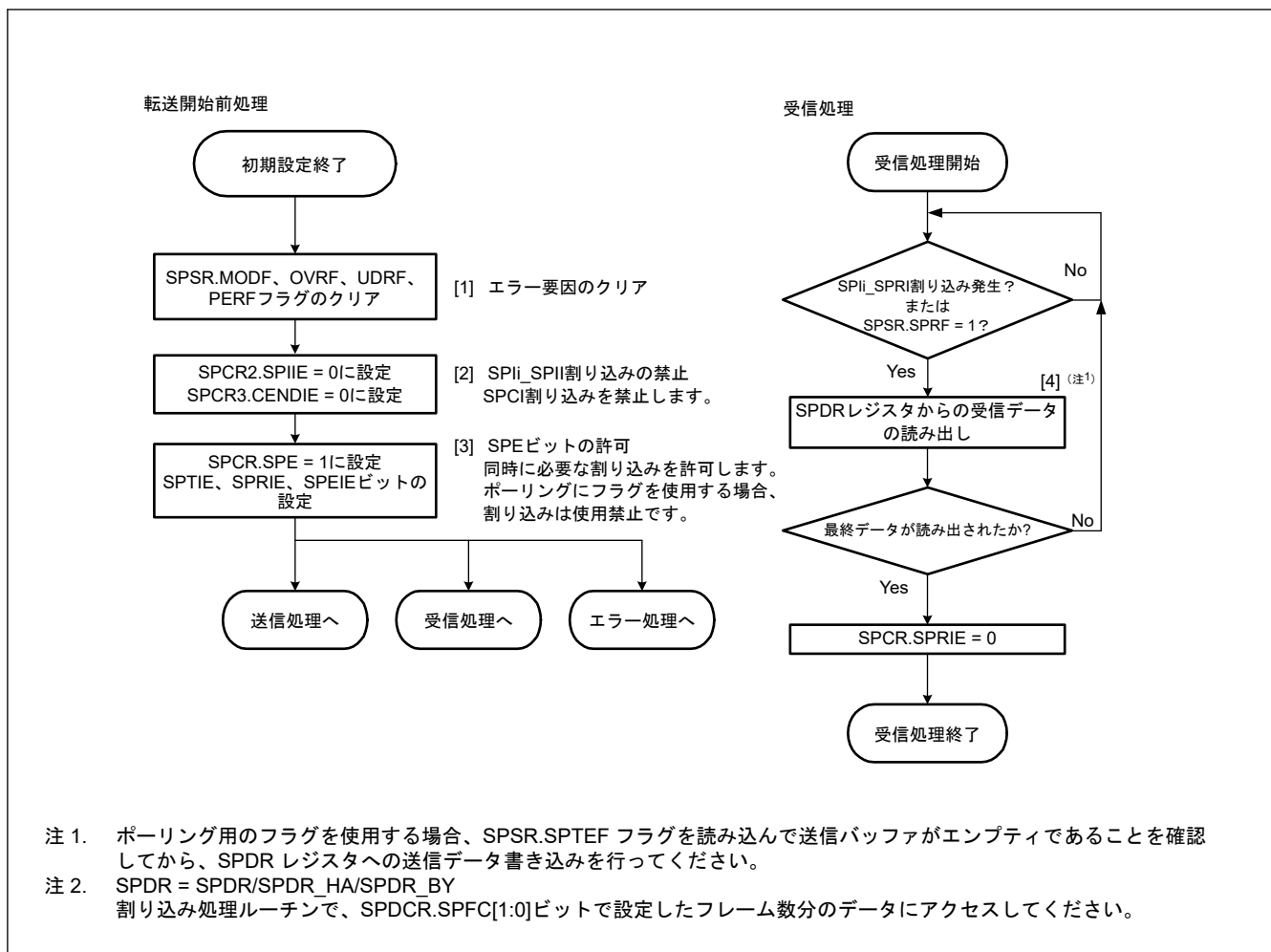
図 30.54 スレーブモードでの受信フロー
