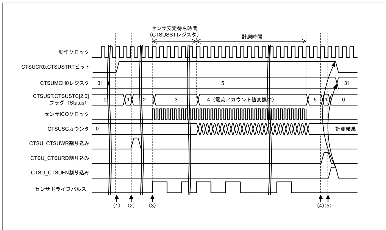
図 40.13 自己容量シングルスキャンモードのタイミング（計測開始条件がソフトウェアトリガの場合）
