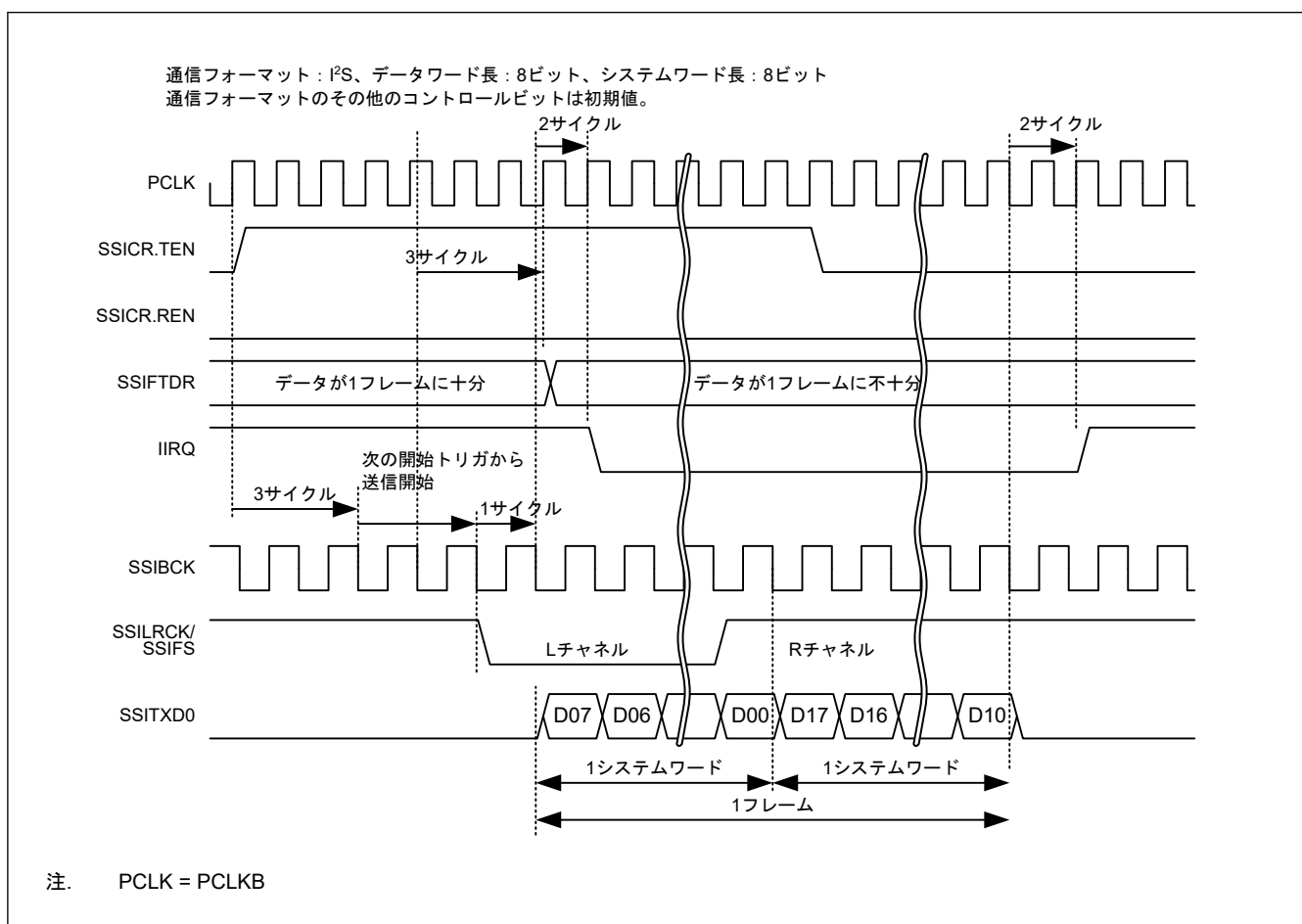
図 32.13 IIRQ 設定タイミング (送信)
