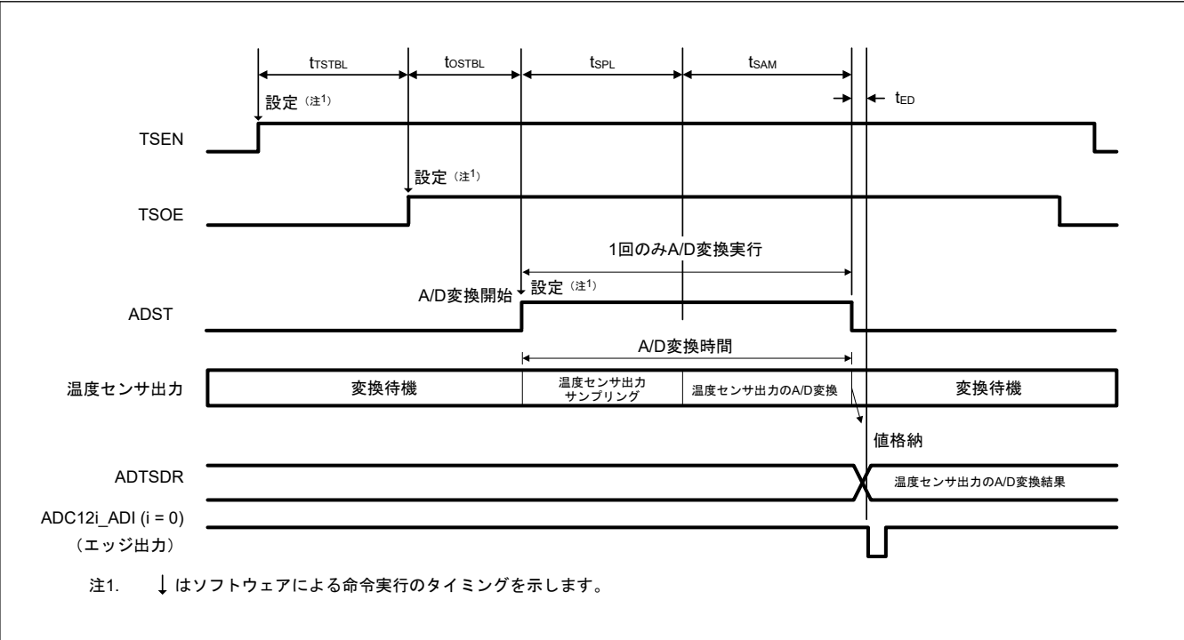
図 39.3 温度センサの動作開始から A/D 変換完了までのタイミング
