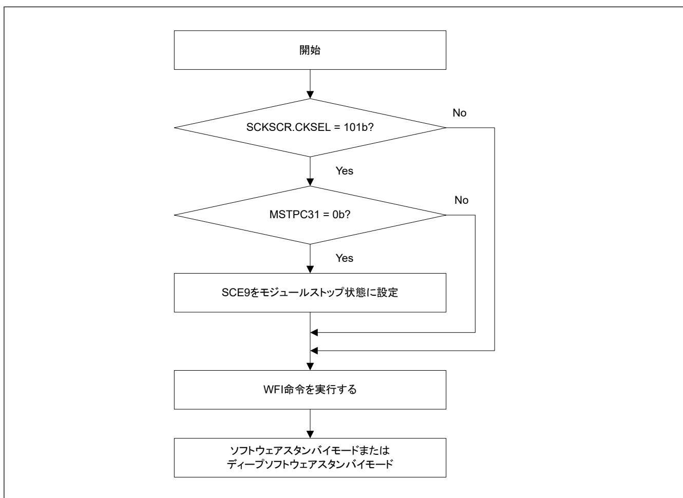
図 10.4 ソフトウェアスタンバイモードまたはディープソフトウェアスタンバイモード遷移時のフローチャート例
