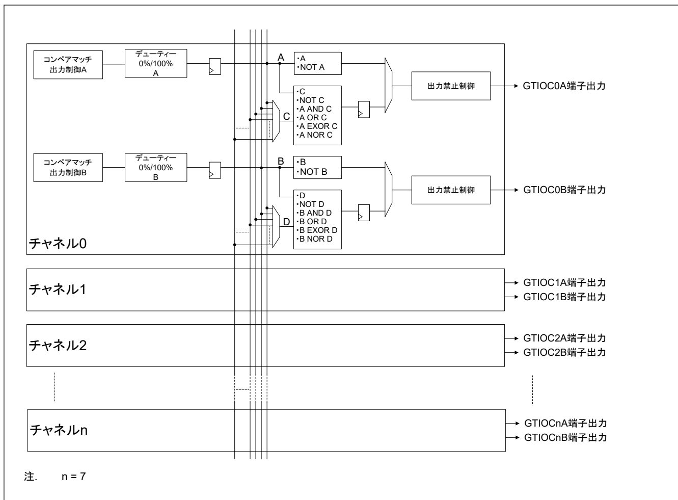
図 21.61 チャンネル間論理演算のブロック図
