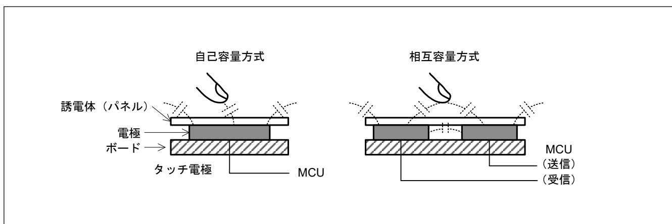
図 40.2 自己容量方式と相互容量方式
