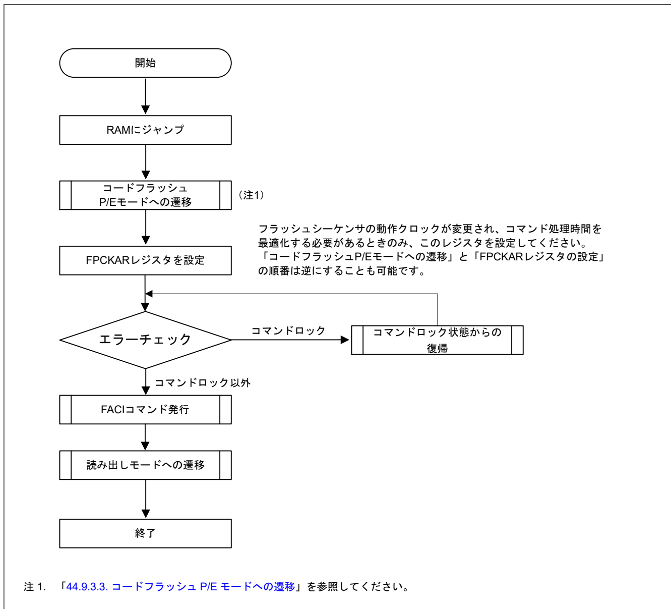
図 44.7 コードフラッシュ P/E モードでのコマンド使用概要
