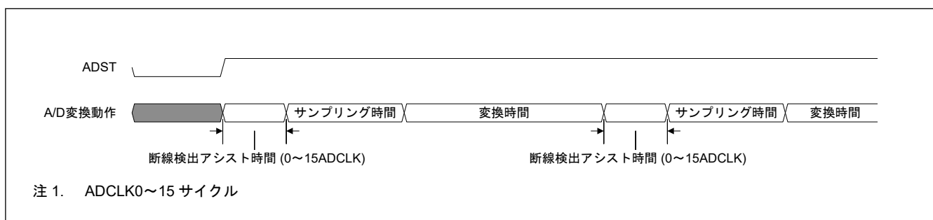
図 37.28 断線検出アシスト機能を使用した場合の A/D 変換動作図
