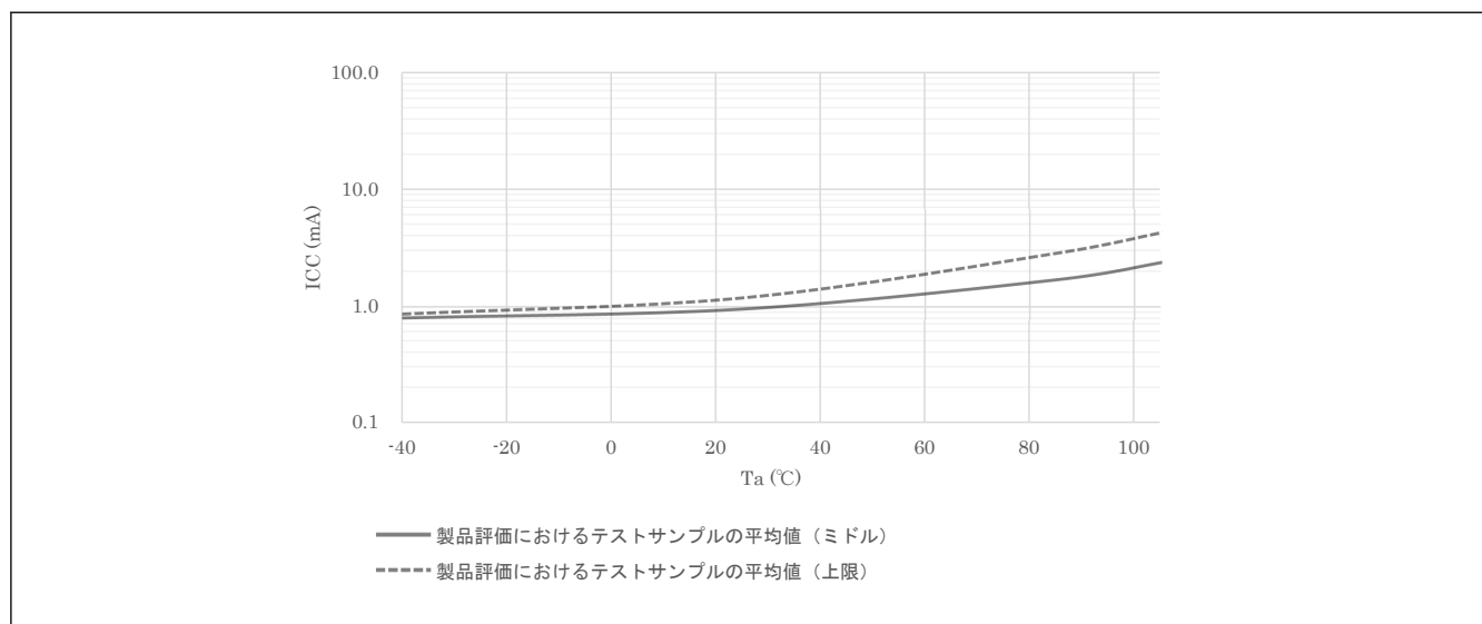
図 47.2 ソフトウェアスタンバイモード時の温度依存性 (参考データ)
