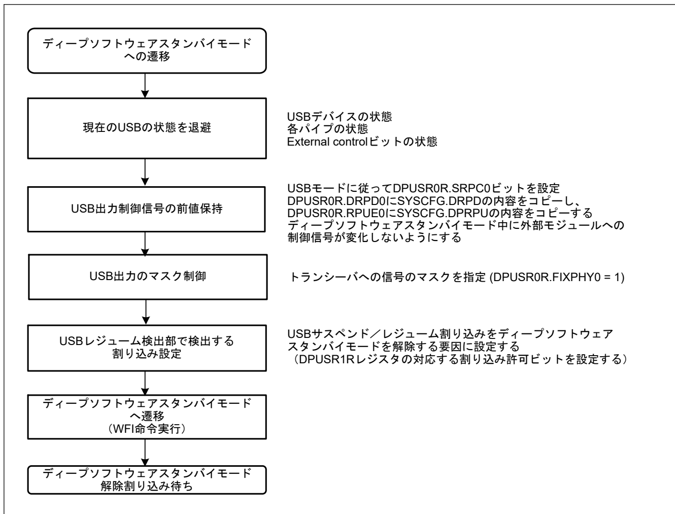
図 26.8 ホストコントローラ機能またはデバイスコントローラ機能選択時におけるディープソフトウェアスタンバイモード遷移時の USBFS 設定フロー
