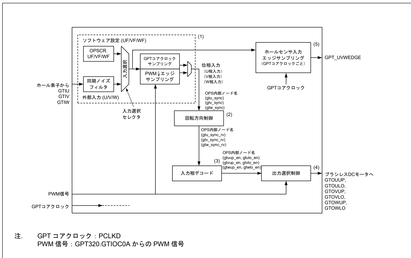
図 21.57 GPT_OPS 制御フロー概念図
