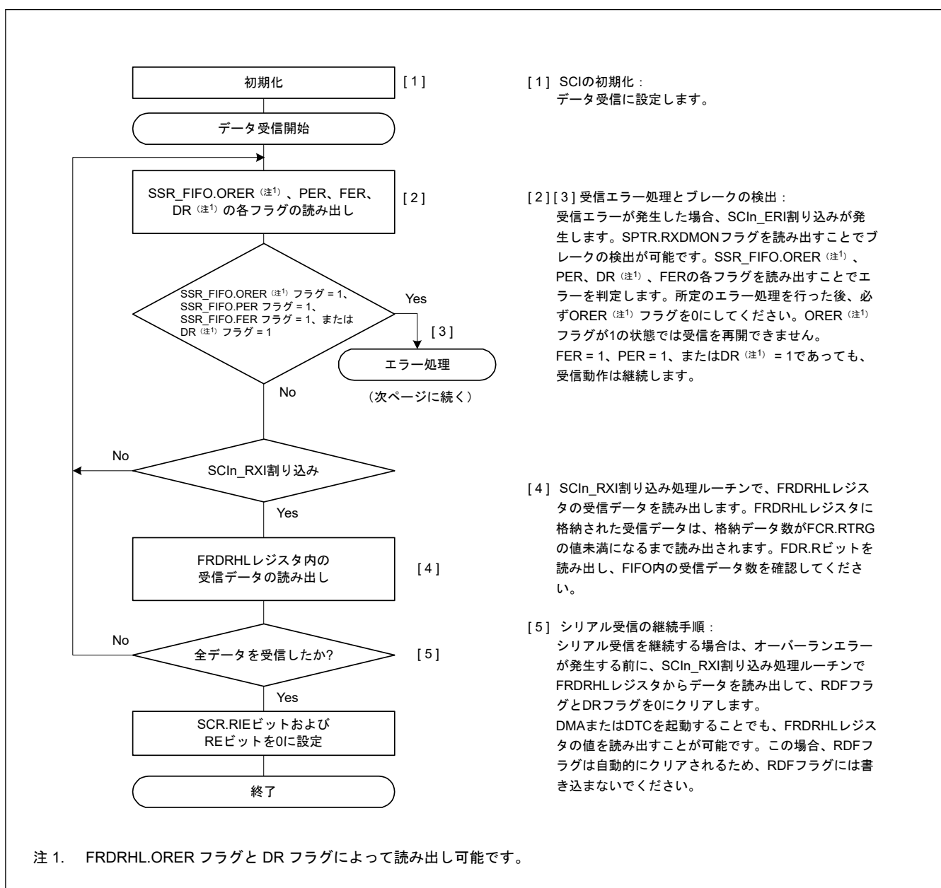
図 27.26 調歩同期式モードにおけるシリアル受信のフローチャート例 (FIFO 選択、アドレス一致検出有効時) (1)
