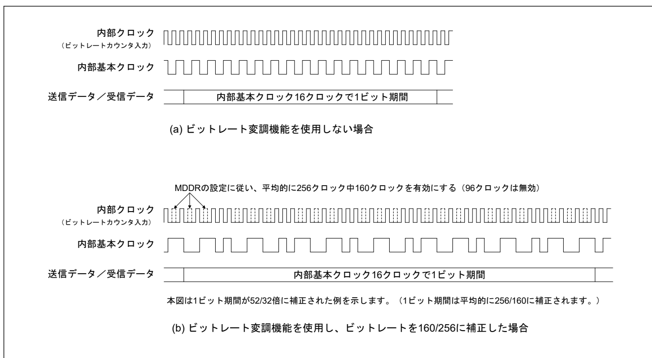
図 27.100 ビットレート変調機能使用時の内部基本クロックの例
