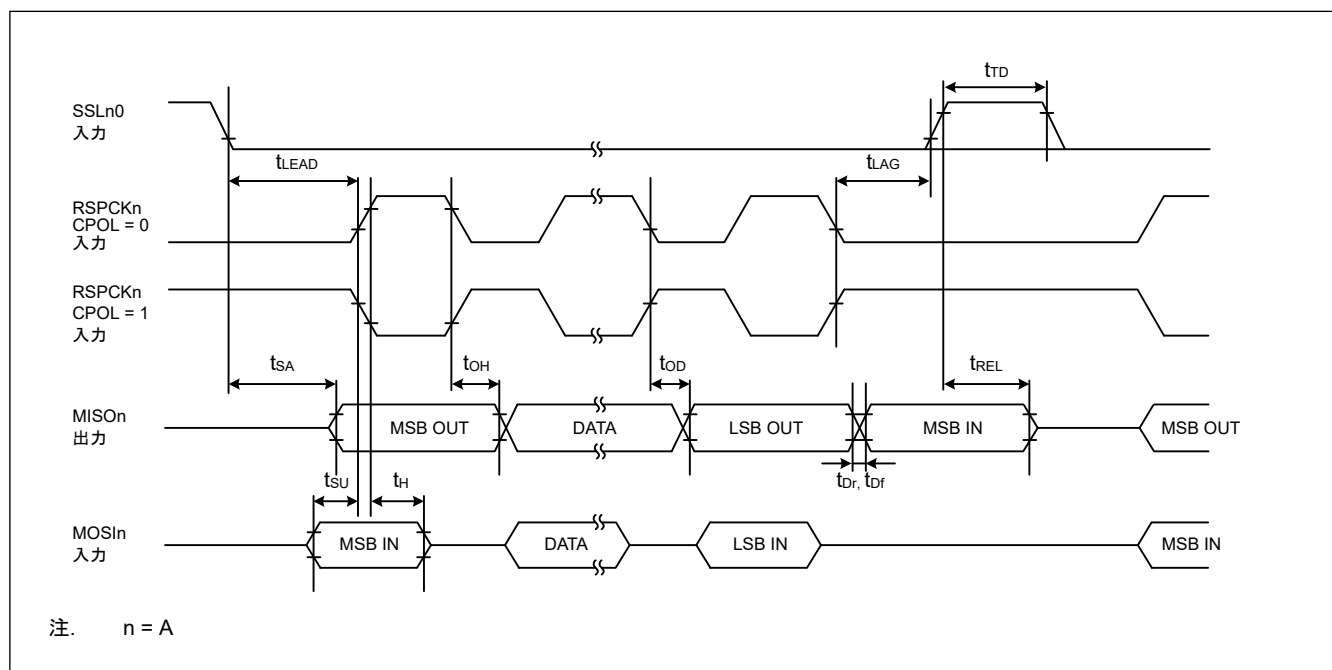
図 47.39 CPHA = 0 の場合におけるスレーブの SPI タイミング
