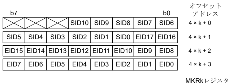
図 29.14 マスクレジスタの構造 ( j = 0 \sim 7 )
