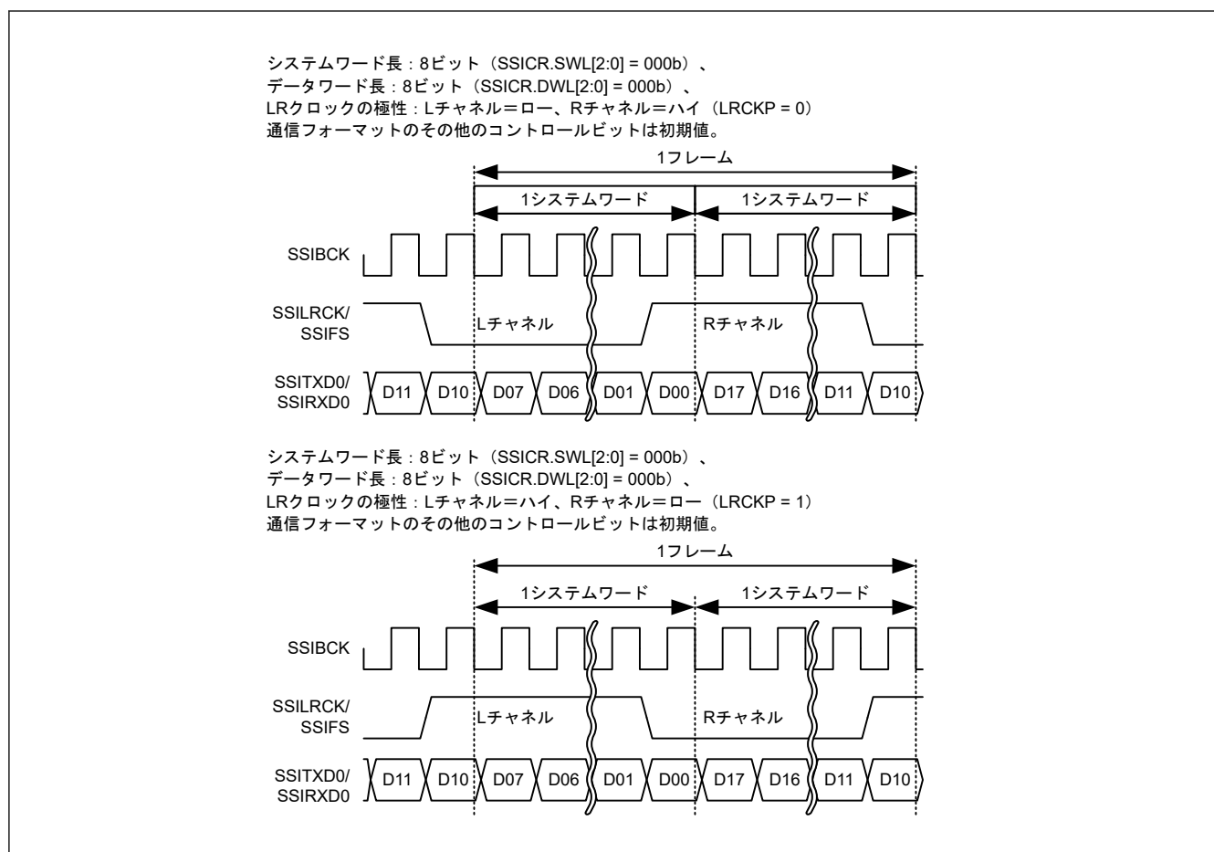
図 32.11 LR クロック/フレーム同期極性設定
