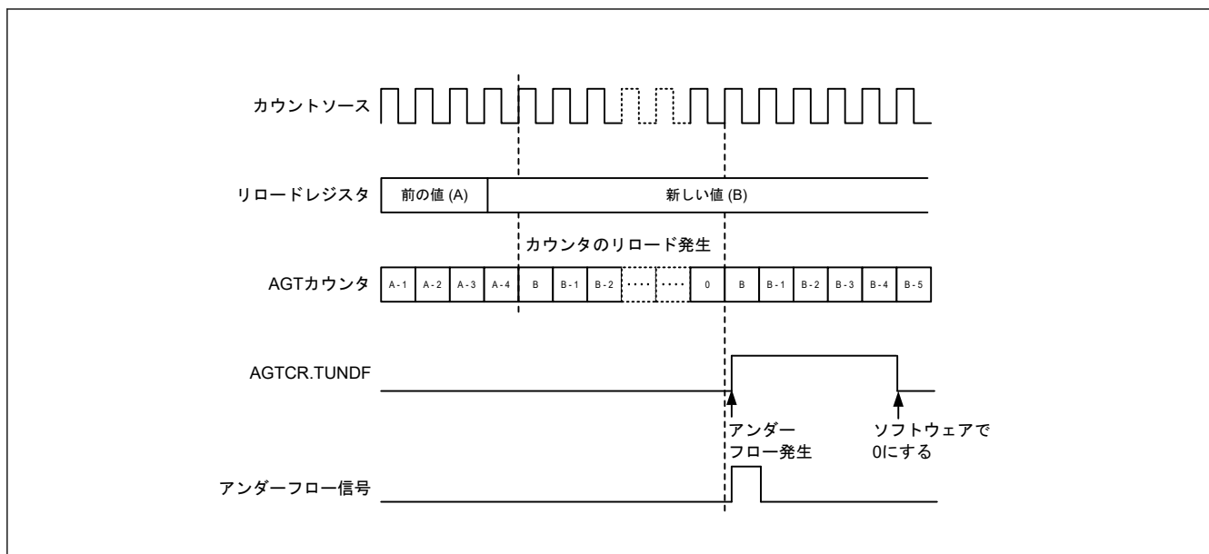
図 22.6 タイマモードでの動作例
