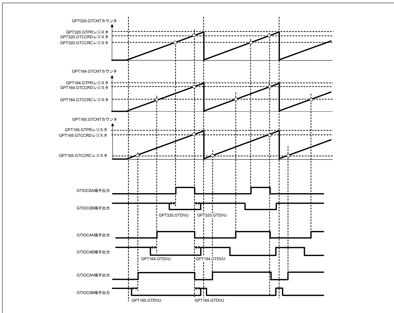
図 21.41 のこぎり波 3 相相補 PWM 出力例 (デッドタイム自動設定)
