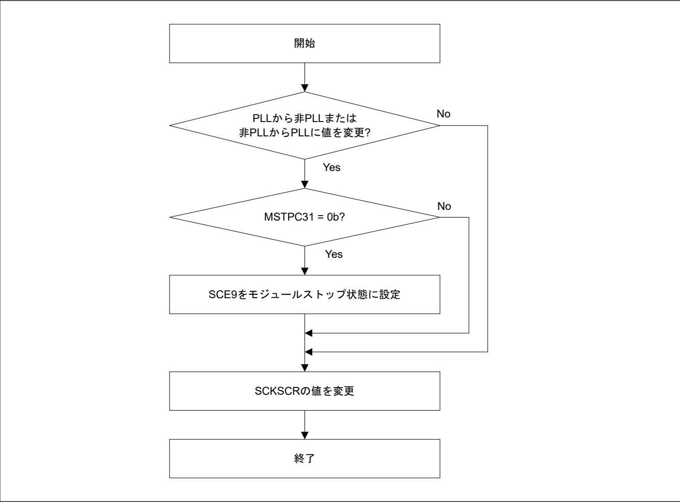
図 8.3 SCKSCR の値の変更フロー例
