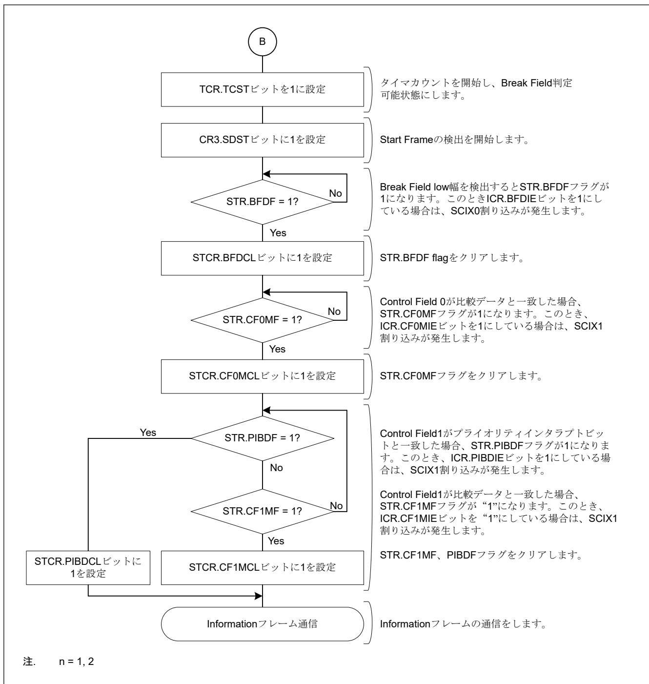
図 27.108 Start Frame 受信フローチャート例 (2)
