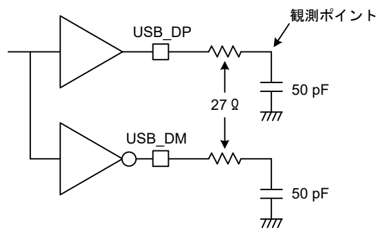
図 47.53 フルスピードモードにおける測定回路
