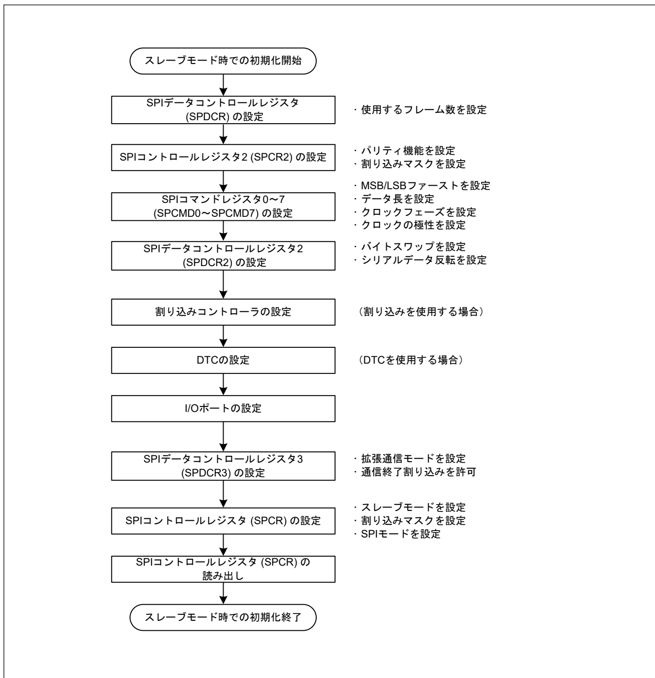
図 30.60 スレープモード時のクロック同期式動作の初期化フロー例
