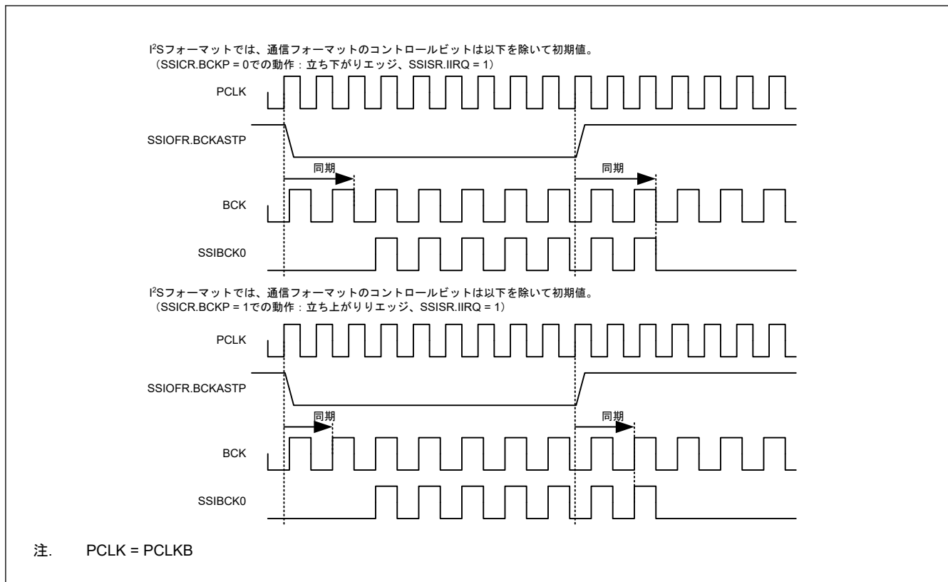
図 32.44 SSIOFR.BCKASTP による SSIBCK0 停止の例
