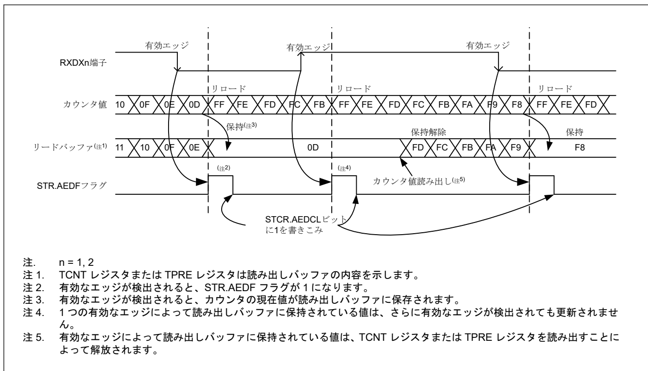
図 27.113 ビットレート測定機能動作例
