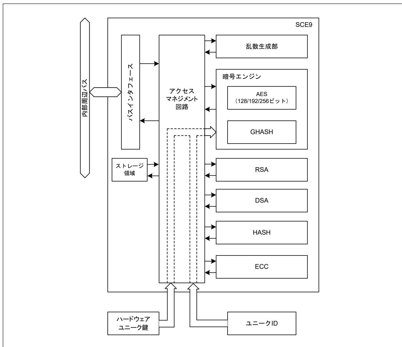
図 36.1 SCE9 のブロック図
