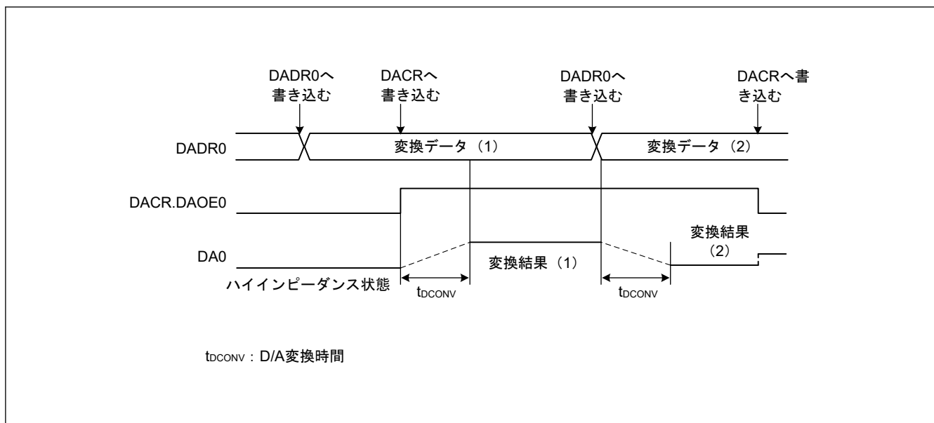
図 38.2 DAC12 の動作例
