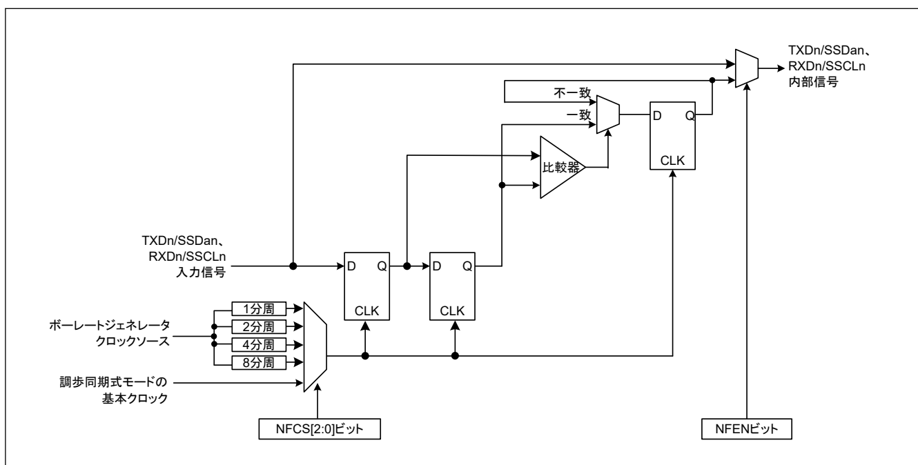
図 27.117 デジタルノイズフィルタ回路のブロック図
