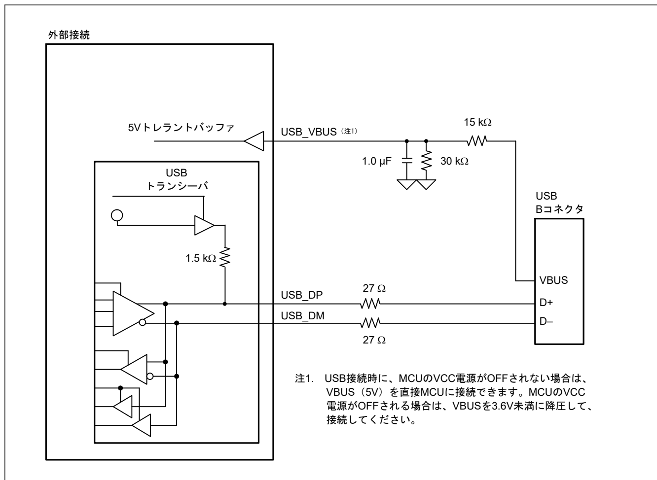
図 26.3 セルフパワードシステムでのデバイス接続例
