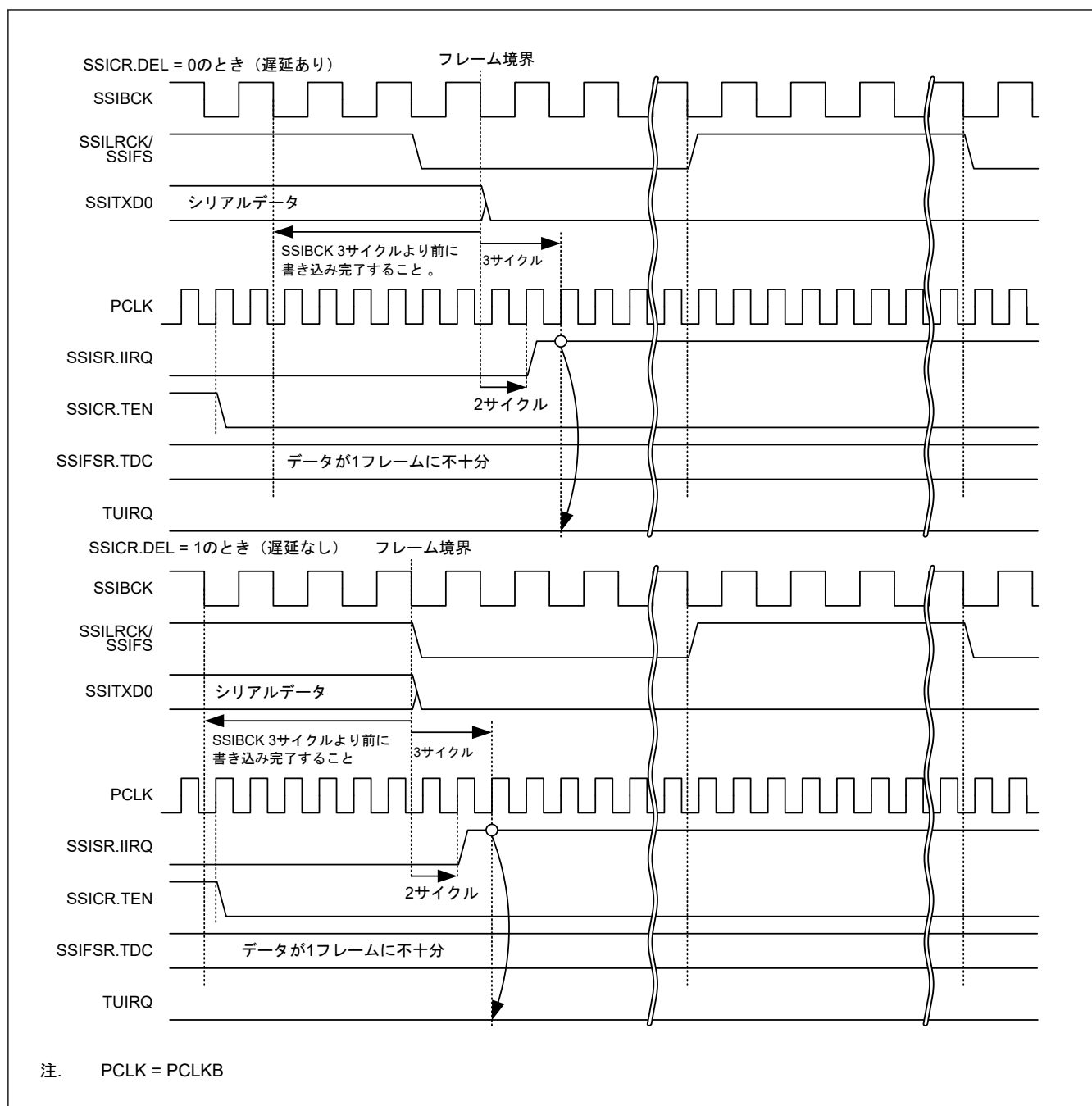
図 32.20 TUIRQ 設定タイミング (通信中断時)
