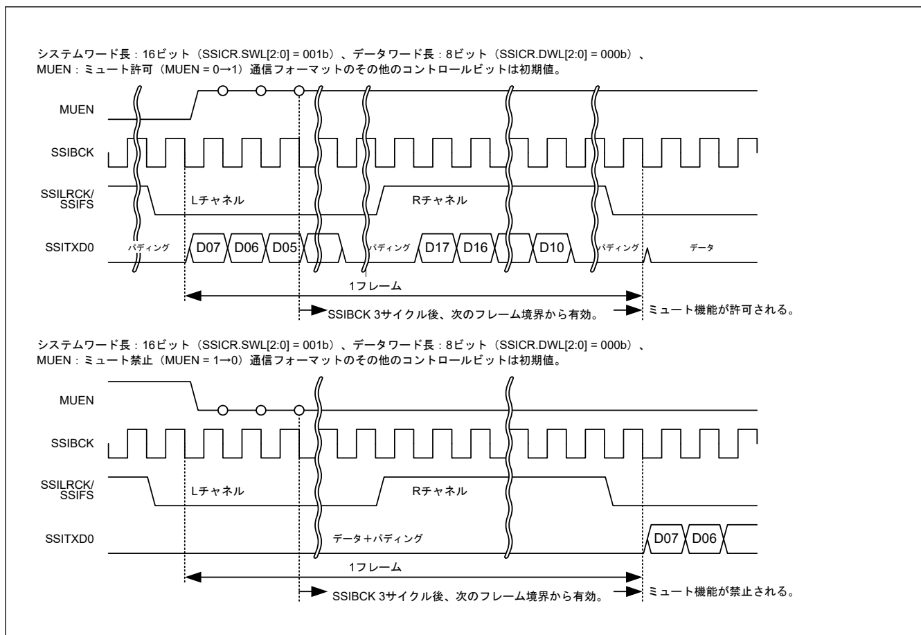
図 32.4 ミュート機能設定時のデータ送信
