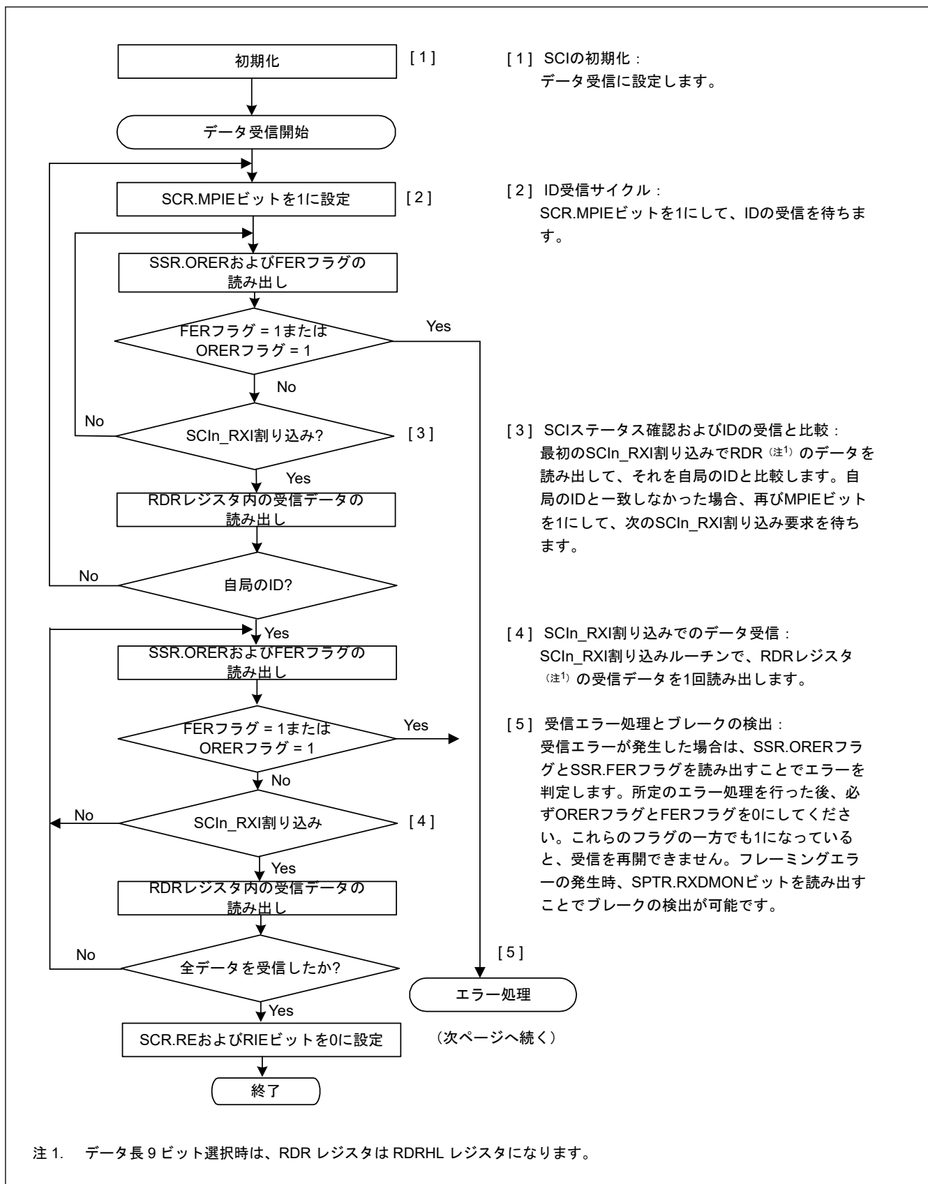
図 27.45 マルチプロセッサシリアル受信のフローチャート例（非 FIFO 選択時）(1)
