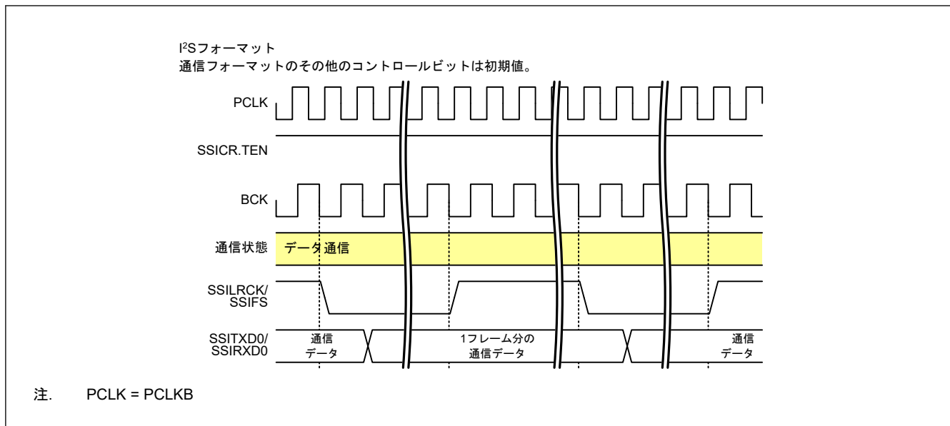
図 32.46 データ通信の継続
