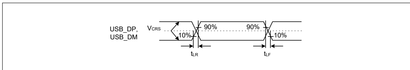
図 47.50 Low-speed モードにおける USB_DP、USB_DM の出力タイミング
