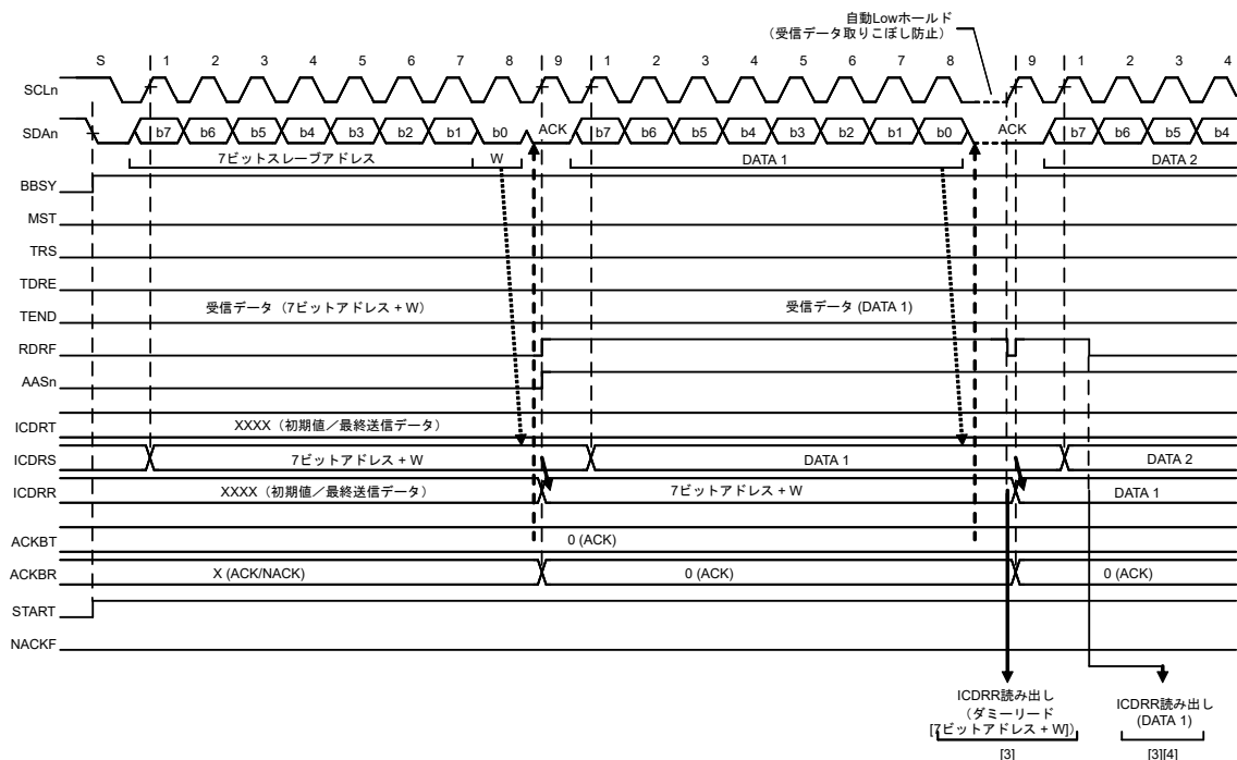
図 28.19 スレープ受信の動作タイミング (1) (7 ビットアドレスフォーマットで RDRFS = 0 の場合)
