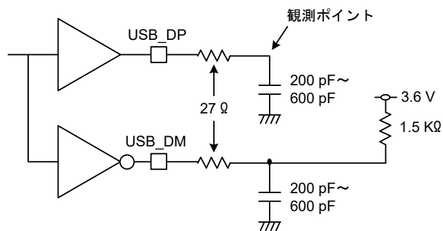
図 47.51 Low-speed モードにおける測定回路
