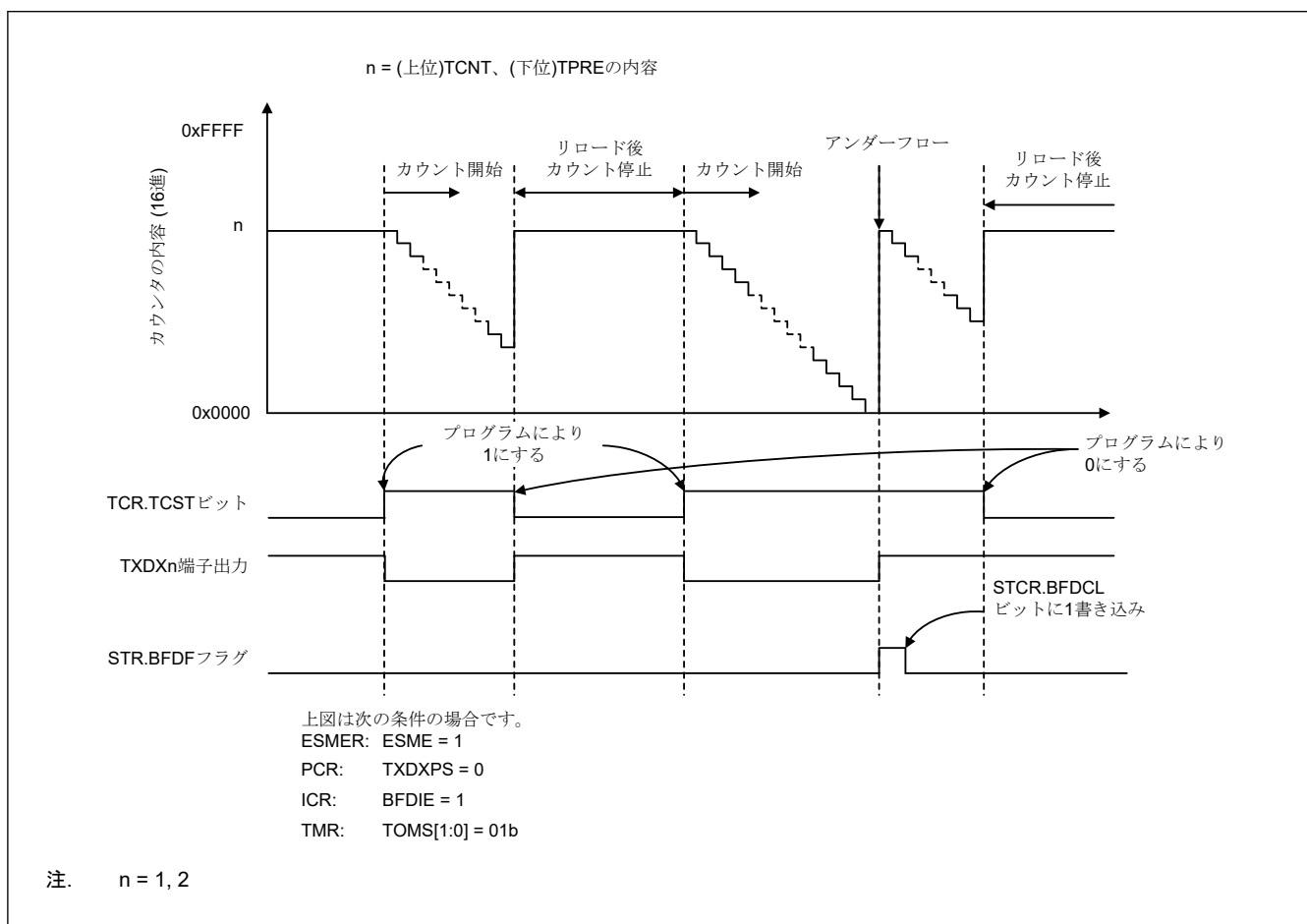
図 27.115 Break Field Low width 出力モードの動作例
