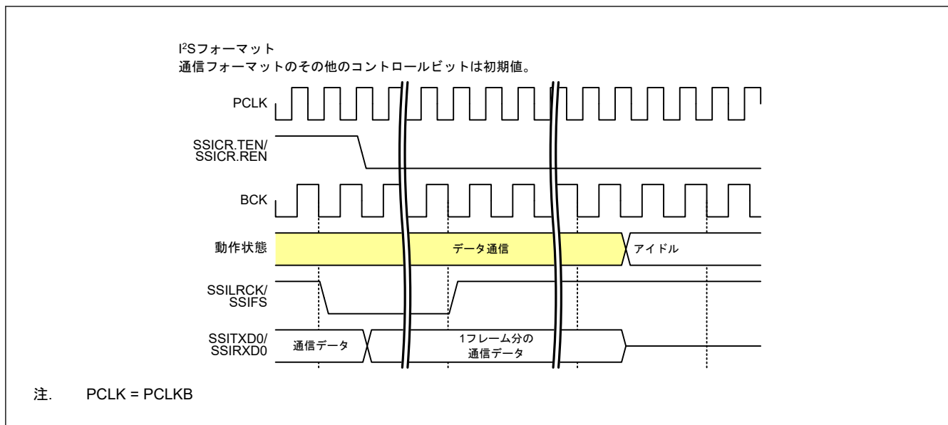
図 32.47 データ通信からの停止 (パディングビットなし)
