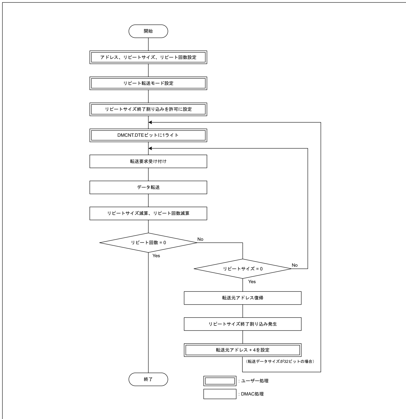
図 16.13 リピート転送モードにおけるオフセット加算による XY 変換フロー
