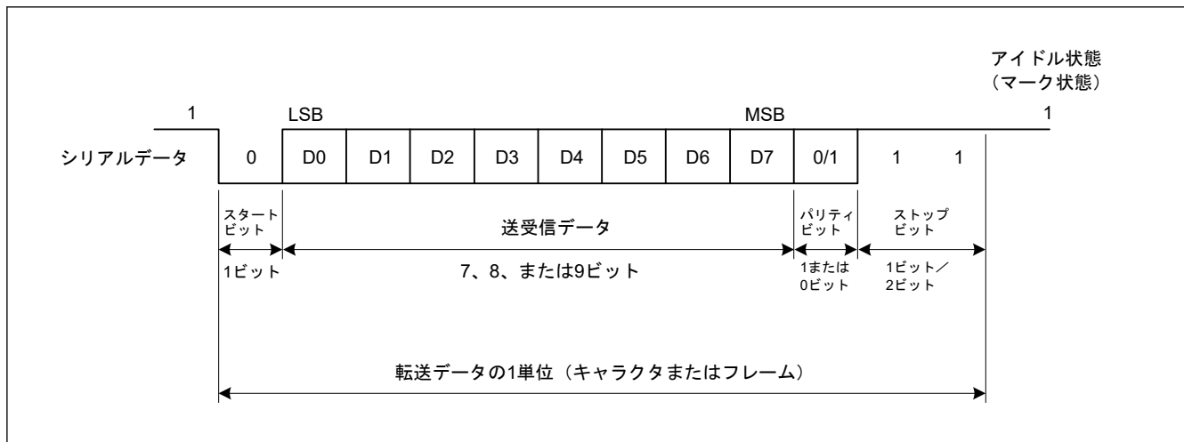
図 27.6 調歩同期式シリアル通信のデータフォーマット (8 ビットデータ／パリティあり／2 ストップビットの場合)
