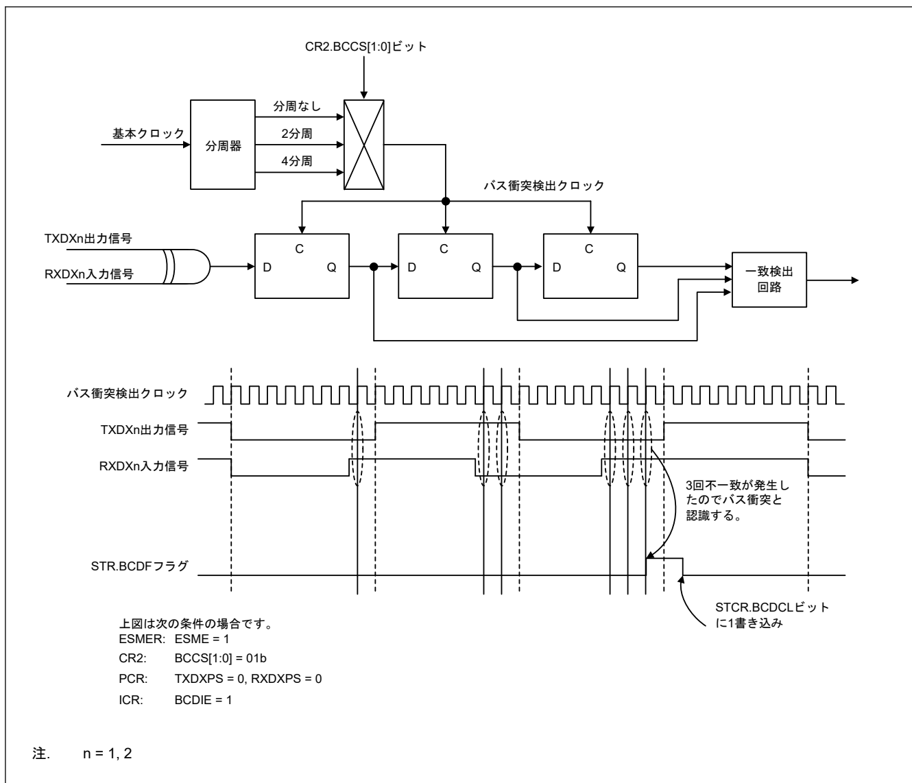
図 27.111 バス衝突検出機能の動作例
