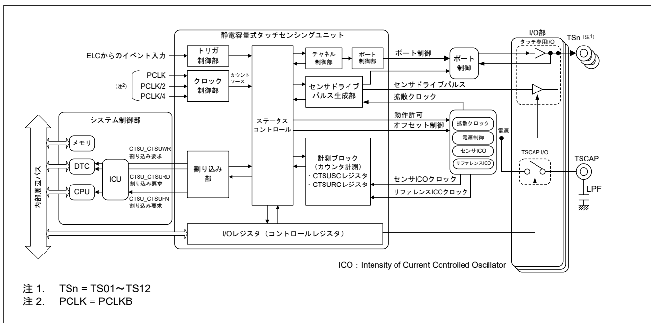
図 40.3 CTSU ブロック図
