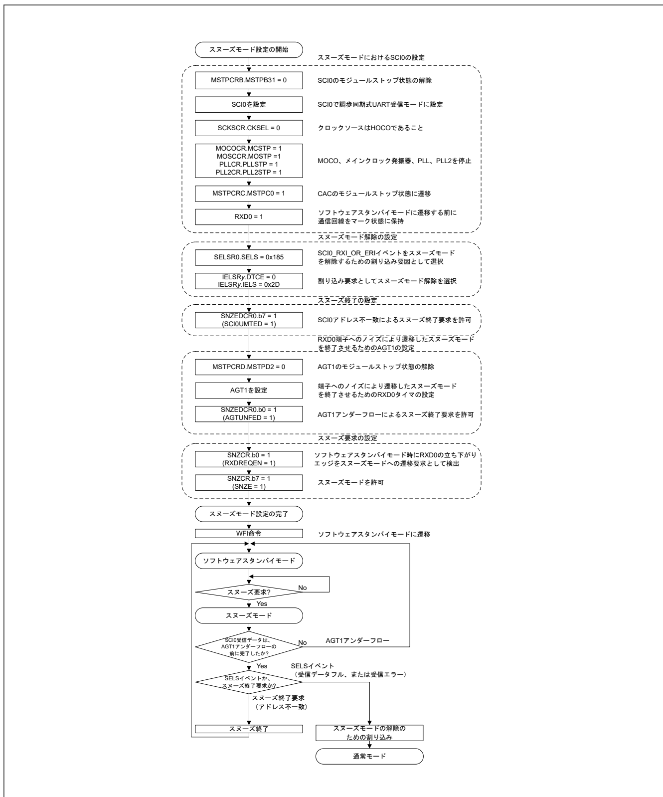
図 10.10 スヌーズモードエントリで SCI0 を使用するための設定例
