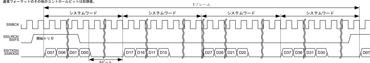
図 32.41 TDM フォーマット（パディングあり、システムワード長 > データワード長）
