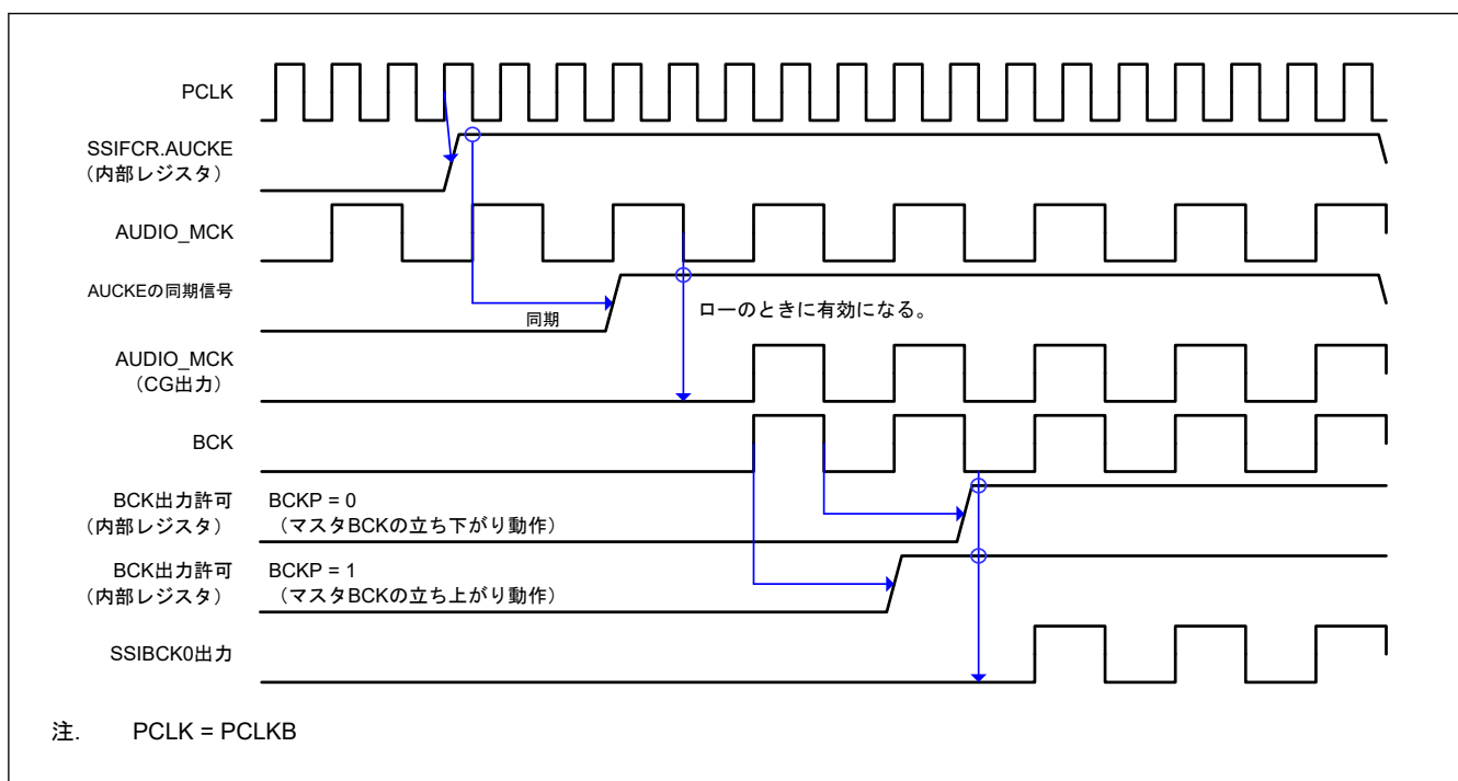
図 32.25 システムリセットからマスタモード通信開始までの動作のタイミング図
