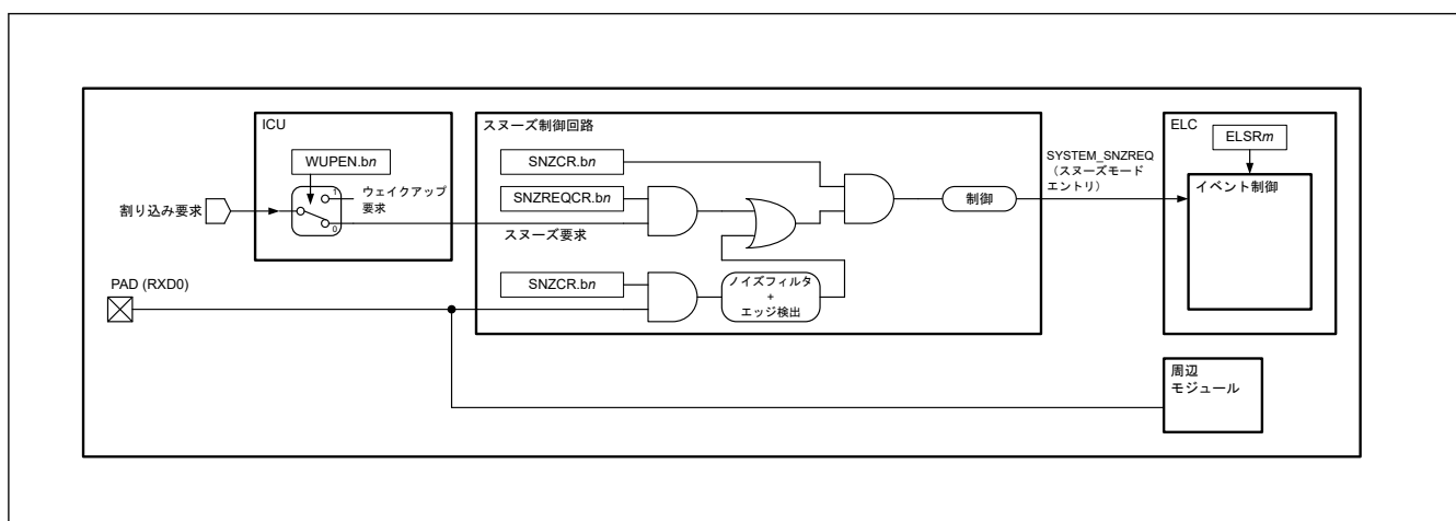
図 10.6 スヌーズモードへの遷移時構成
