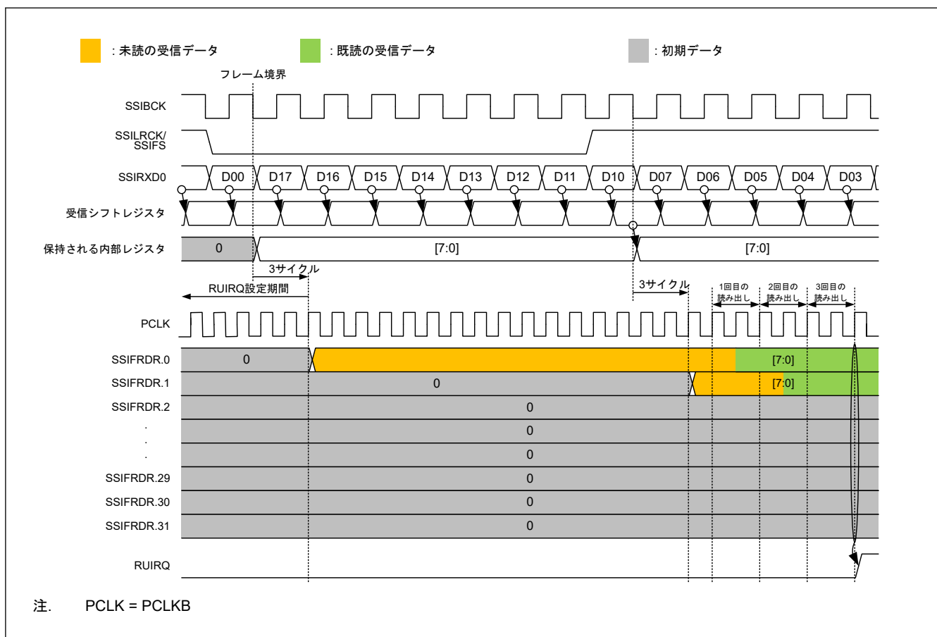
図 32.16 RUIRQ 設定タイミング
