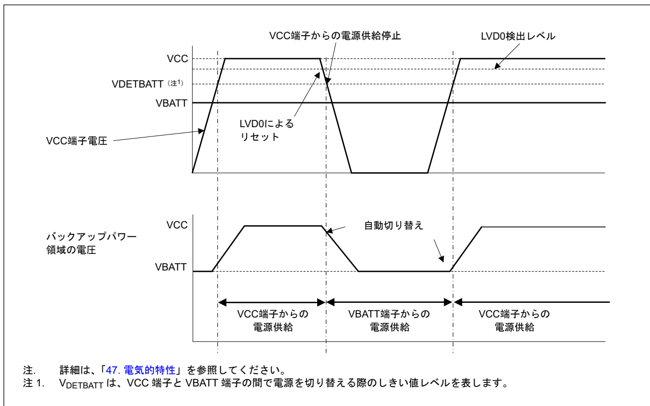
図 11.2 バッテリバックアップ機能の切り替え順序
