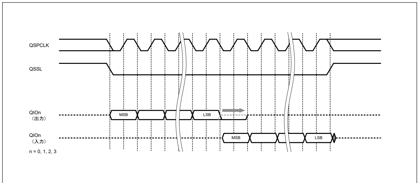
図 31.13 SFMOEX ビットを使用した出力許可ホールド時間調整（標準リード）
