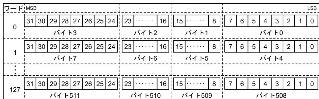
図 33.4 SD_BUF 格納データ
