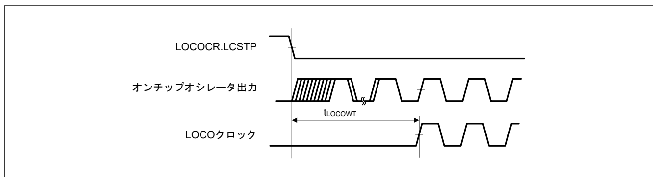
図 47.9 LOCO クロック発振開始タイミング
