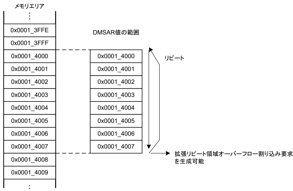
図 16.7 拡張リピート領域の動作例
