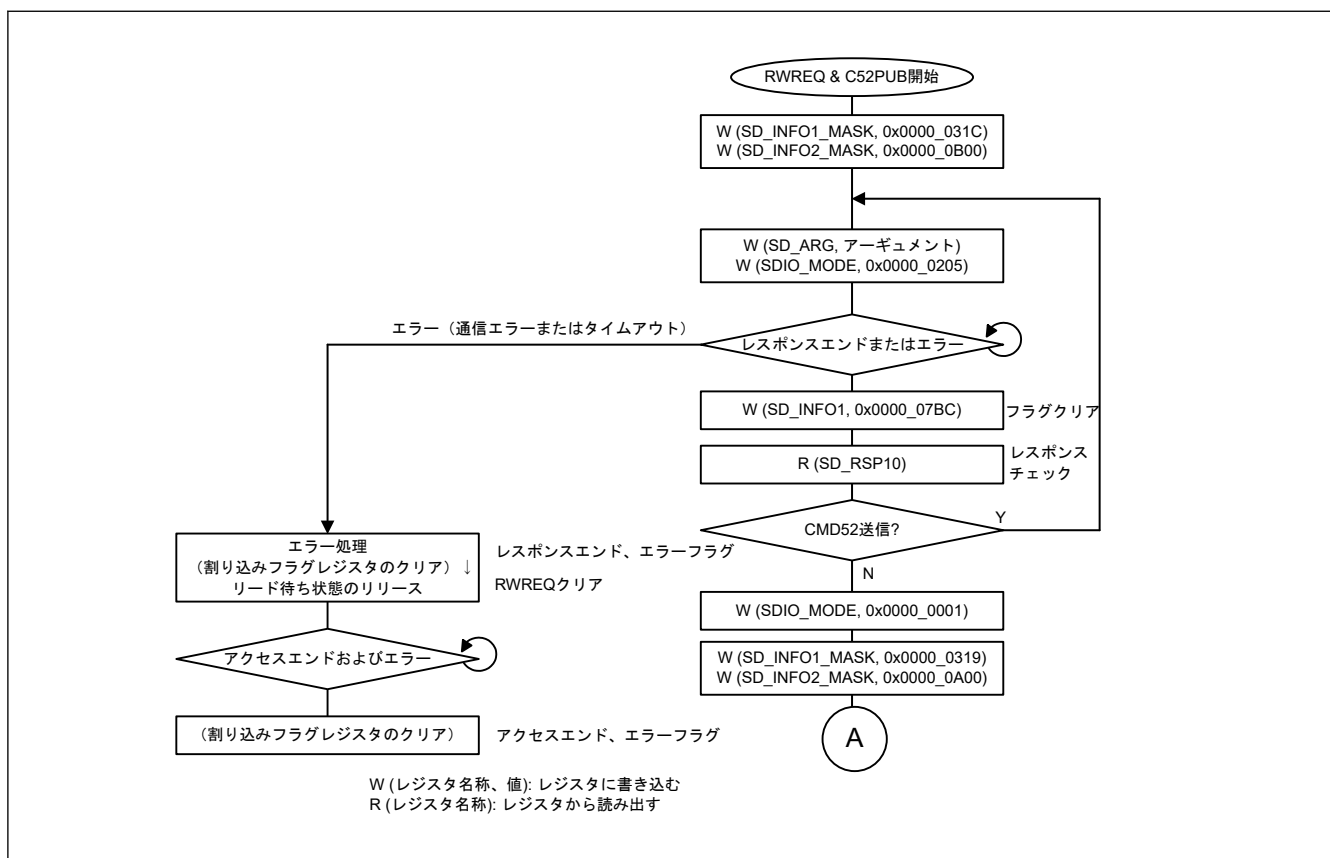
図 33.18 SD ホストインタフェースがリード待ち状態で、CMD53 マルチブロックリード時に CMD52 (SDIO none abort) が送信される場合のフロー
