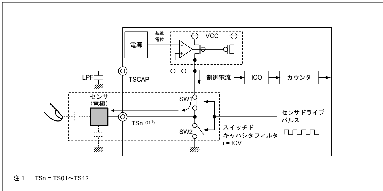
図 40.5 充電動作
