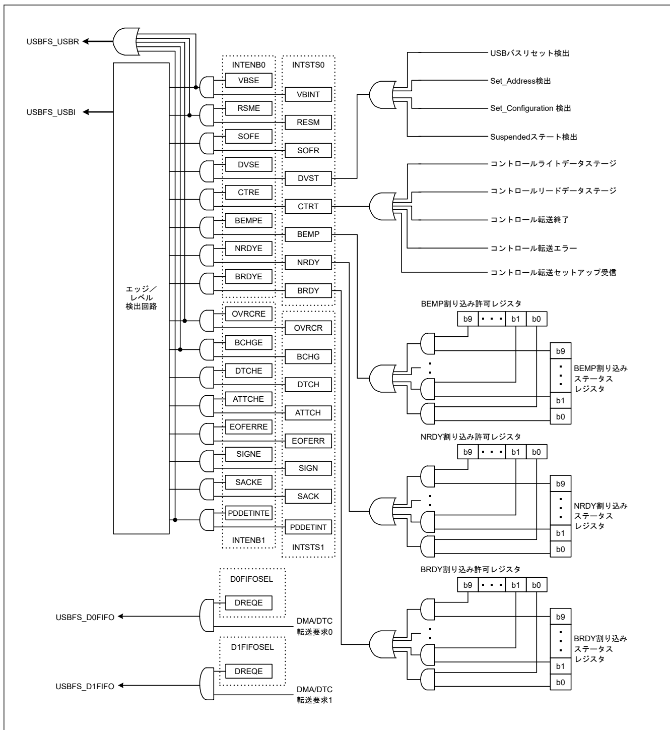
図 26.11 USBFS 割り込みに関連する回路
