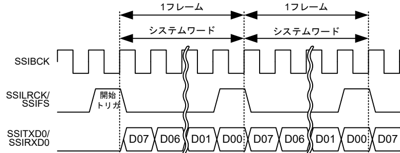
図 32.37 モノラルフォーマットにおけるショートフレーム（パディングなし、システムワード長 = データワード長）
