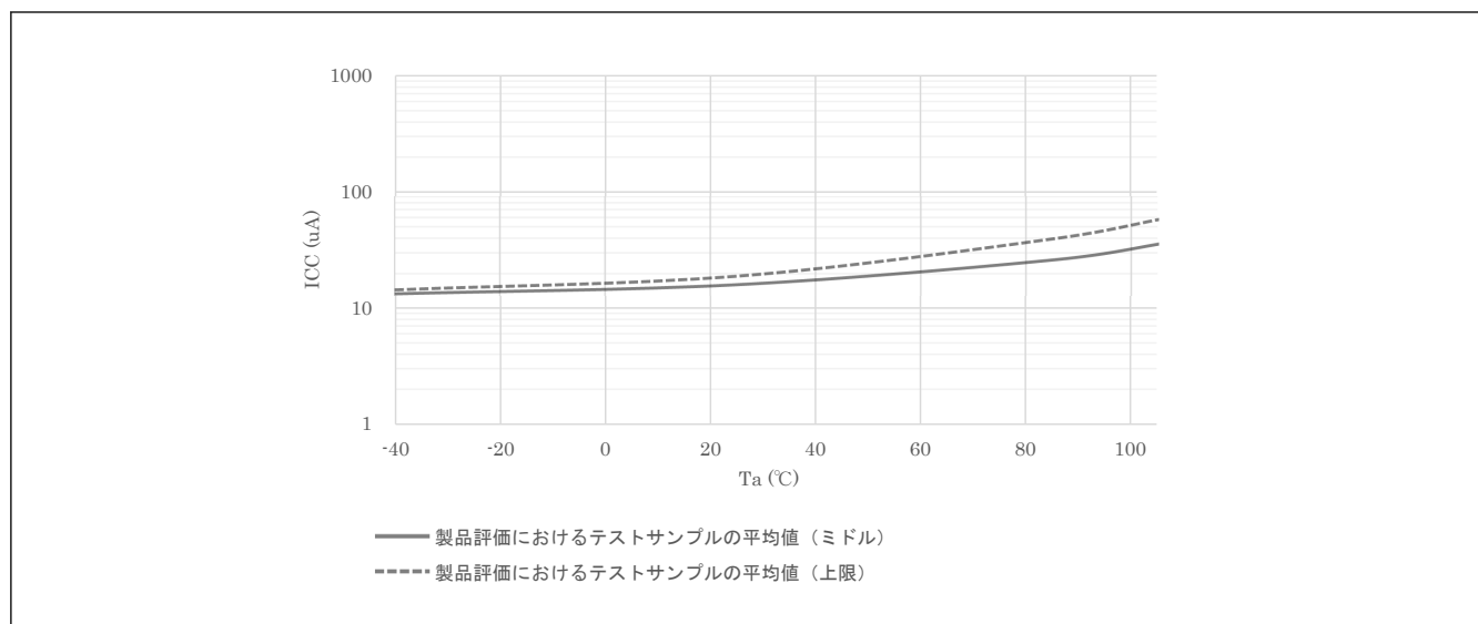
図 47.3 ディープソフトウェアスタンバイモード時の温度依存性、スタンバイ SRAM および USB レジューム検出部への電源供給あり (参考データ)
