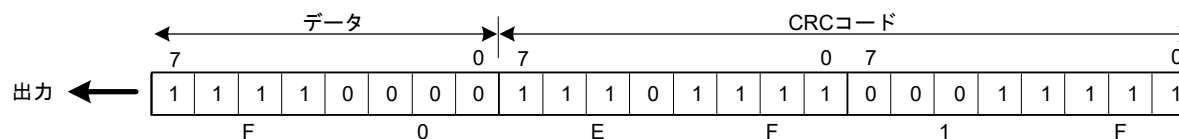
図 34.3 MSB ファーストのデータ送信
