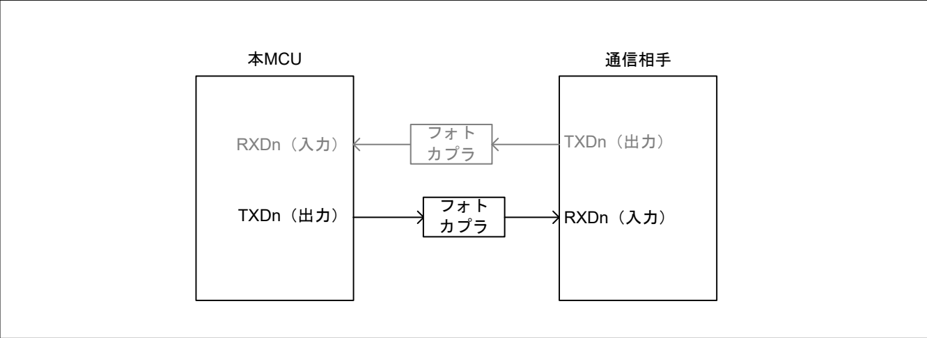
図 27.35 フォトカプラを通過する送信のブロック図イメージ
