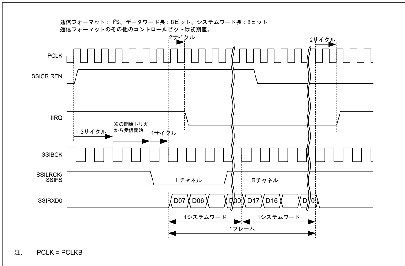
図 32.14 IIRQ 設定タイミング (受信)
