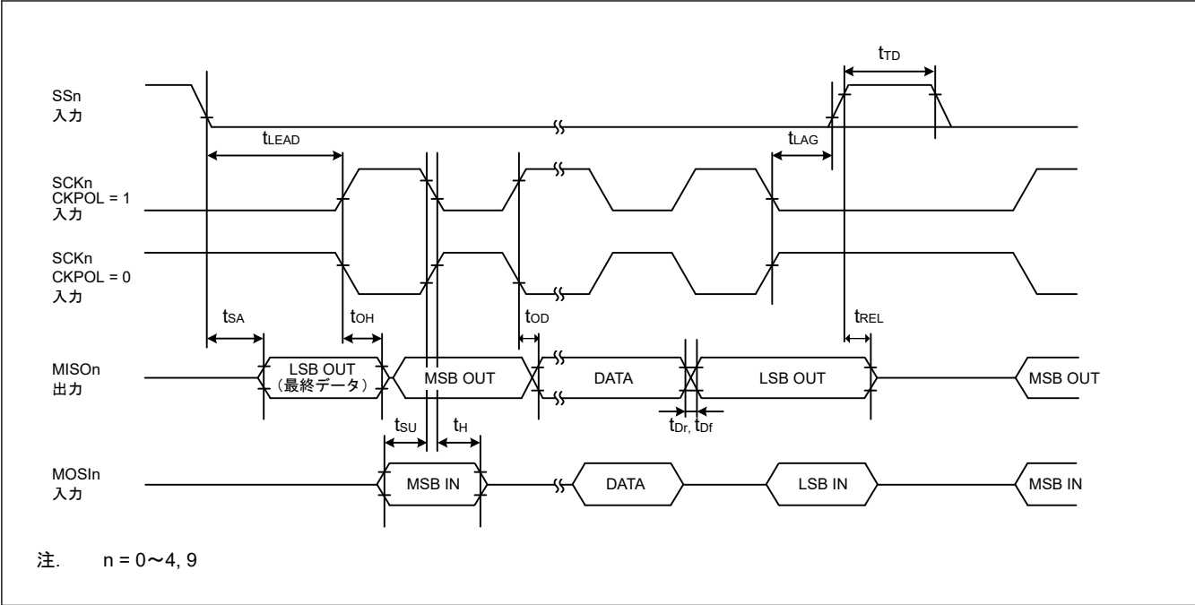
図 47.32 CKPH = 0 の場合におけるスレーブの SCI 簡易 SPI モードタイミング
