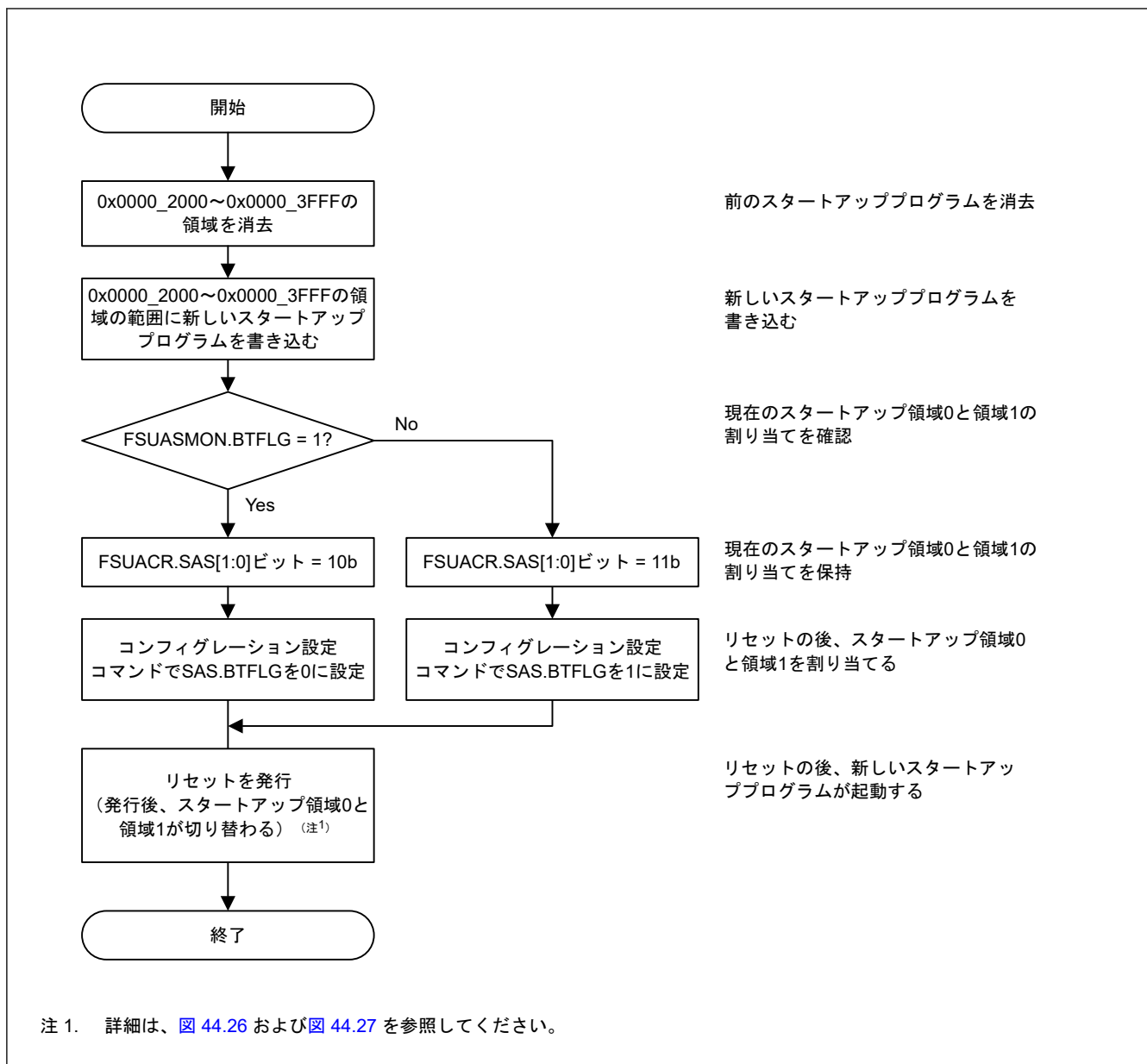
図 44.28 スタートアッププログラムプロテクションの概念
