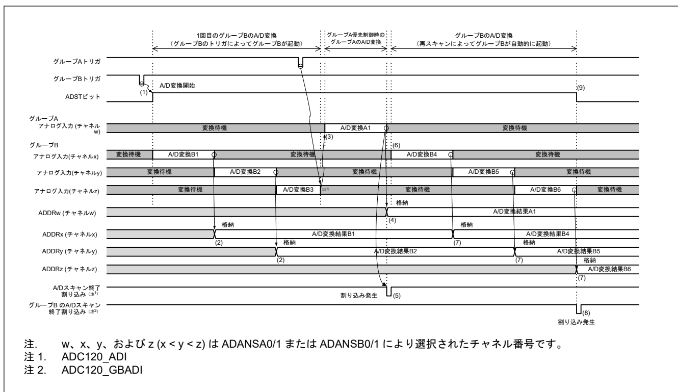
図 37.18 グループ優先動作の例 1-1: グループ B スキャン中のグループ A トリガ入力、再スキャンあり (ADGSPCR.GBRSCN = 1、ADGSPCR.GBRP = 0、および ADGSPCR.LGRRS = 0 の場合)
