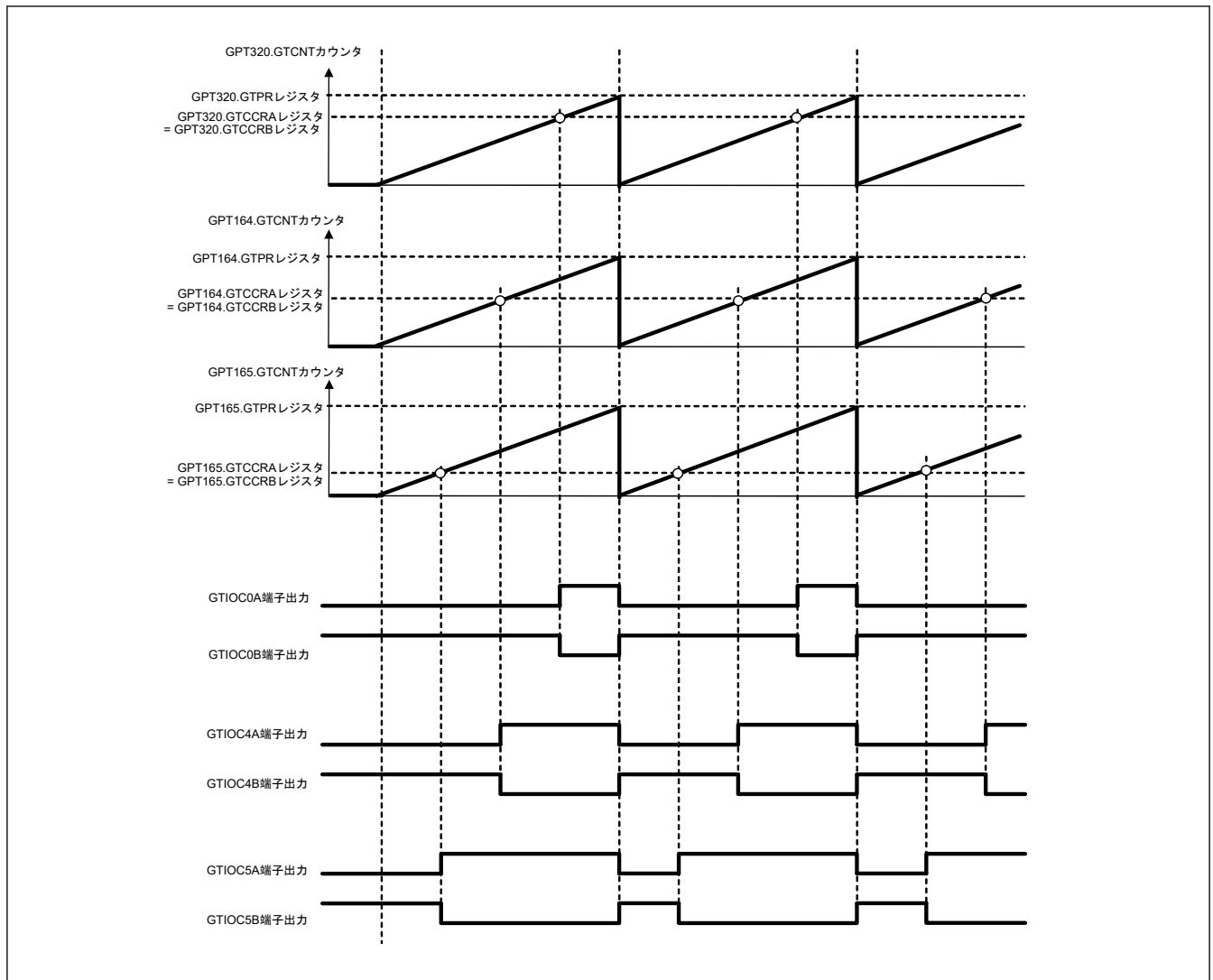
図 21.40 のこぎり波 3 相相補 PWM 出力例
