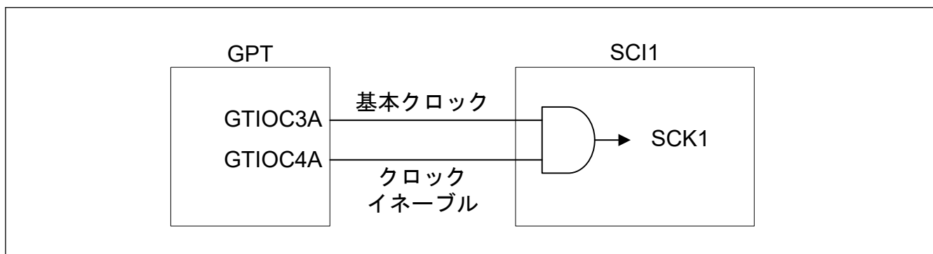
図 27.3 GPT と SCI の接続例
