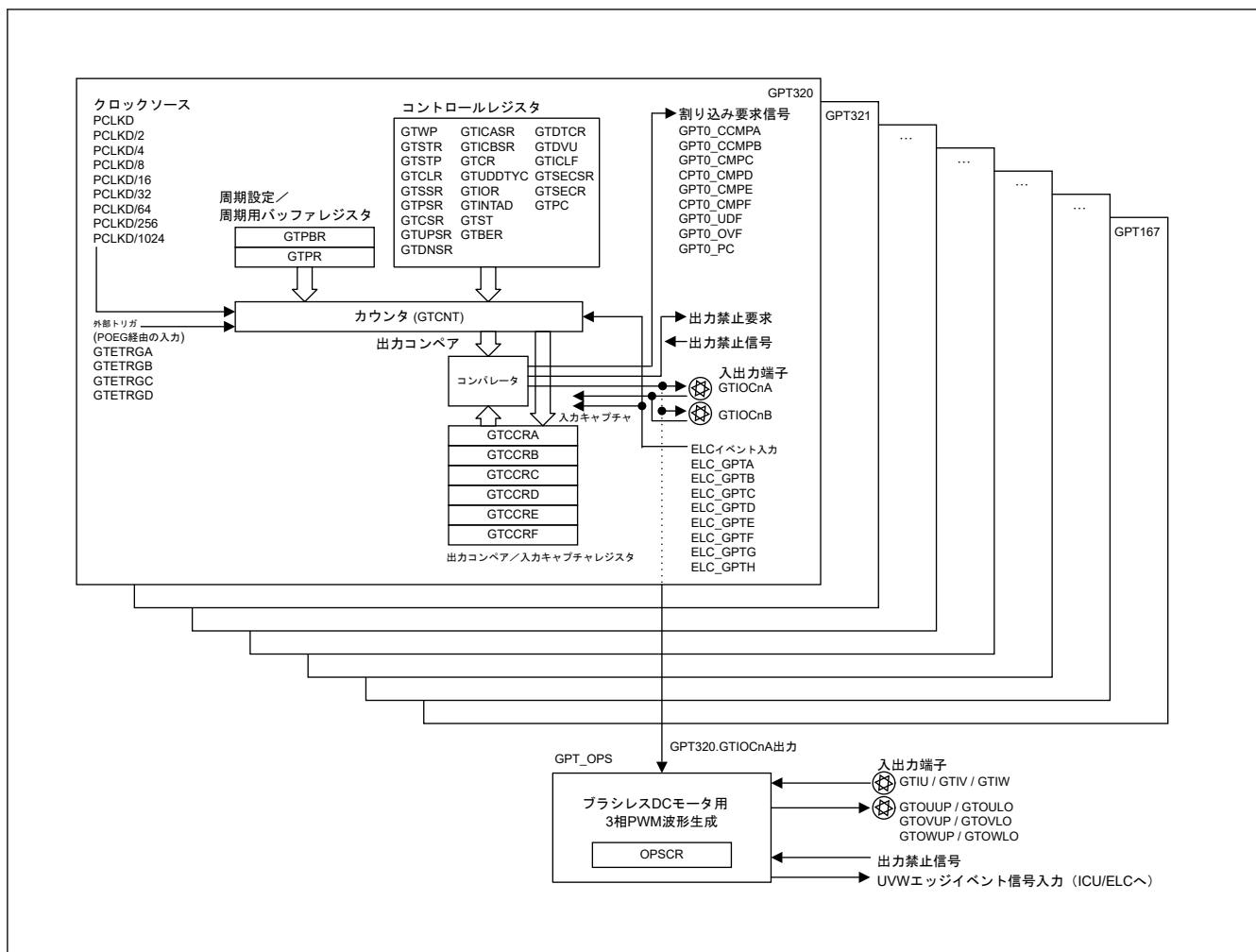
図 21.1 GPT のブロック図
