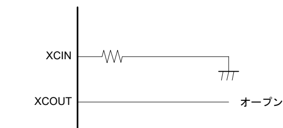
図 8.9 サブクロック発振器を使用しない場合の端子処理
