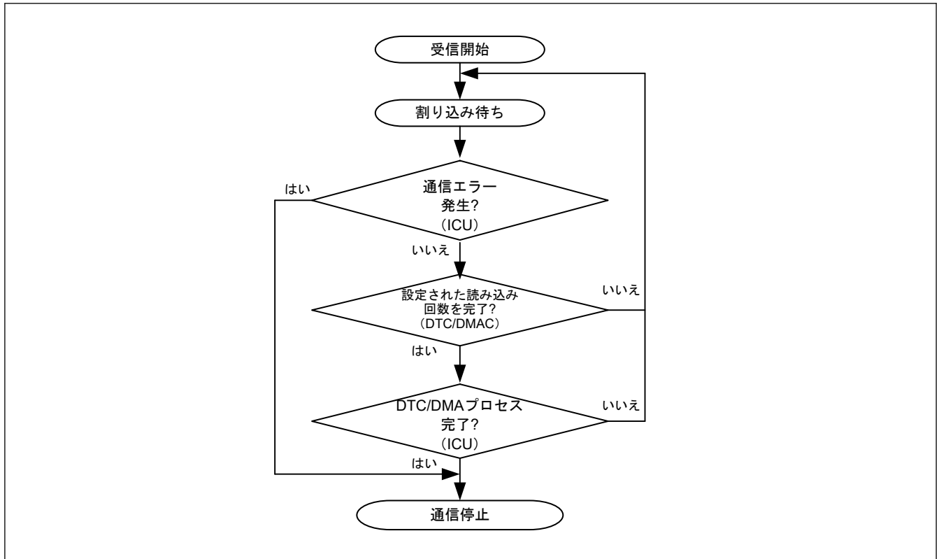
図 32.54 受信手順
