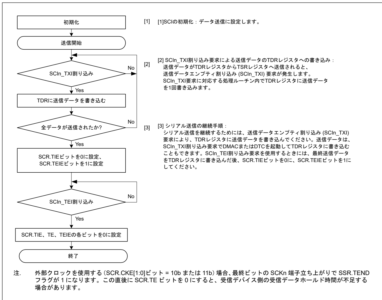
図 27.69 クロック同期式モードにおけるシリアル送信のフローチャート例 (非 FIFO 選択時)
