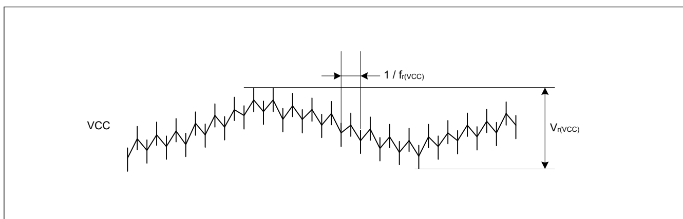
図 47.6 リップル波形
