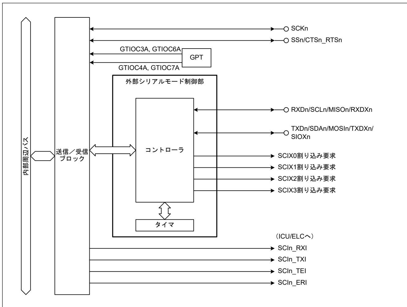
図 27.2 SCIn (n = 1, 2) 拡張シリアルモードコントローラのブロック図
