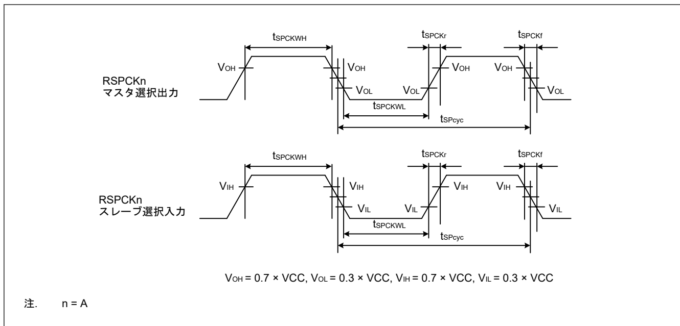
図 47.34 SPI クロックタイミング
