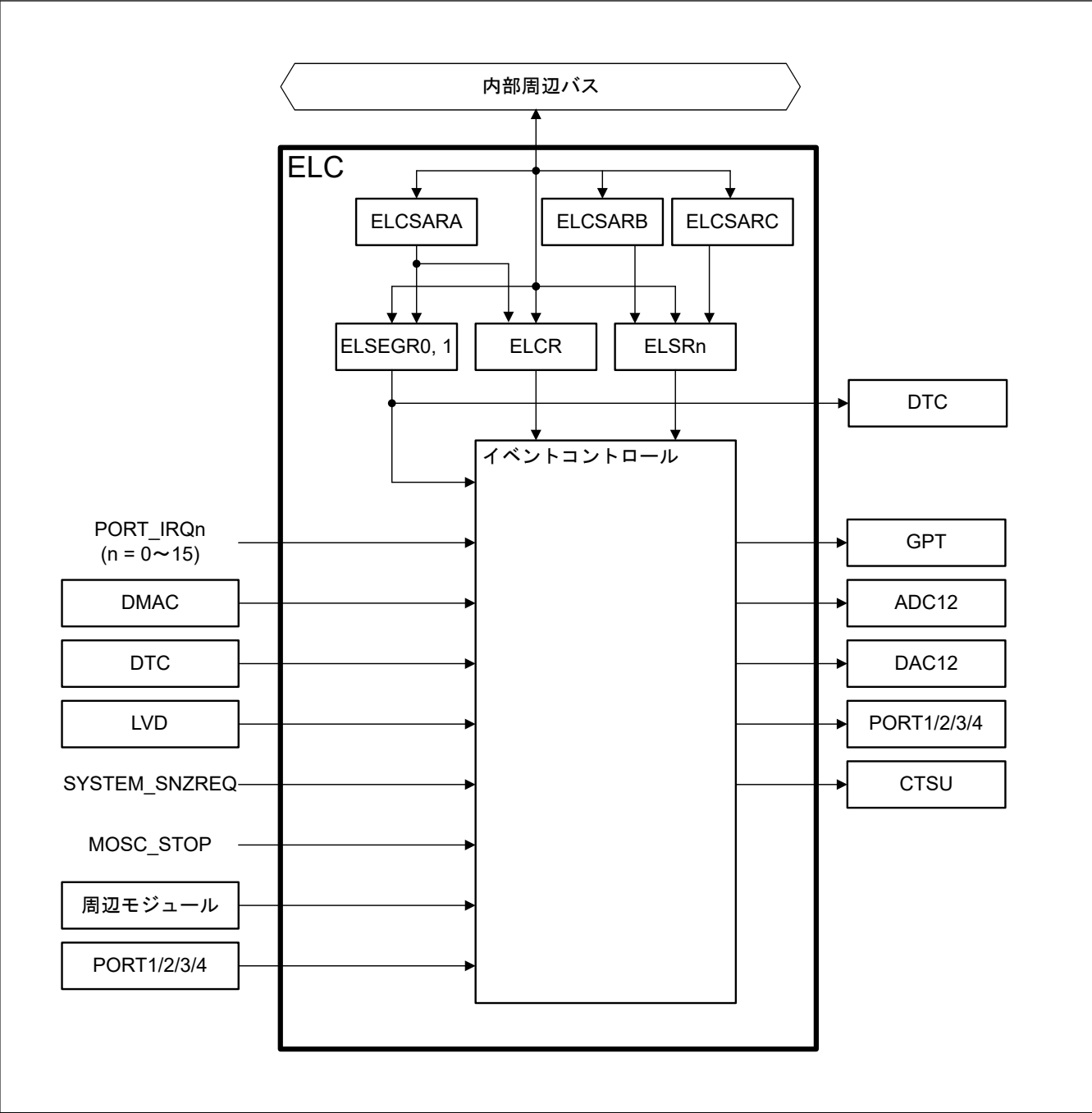
図 18.1 ELC のブロック図
