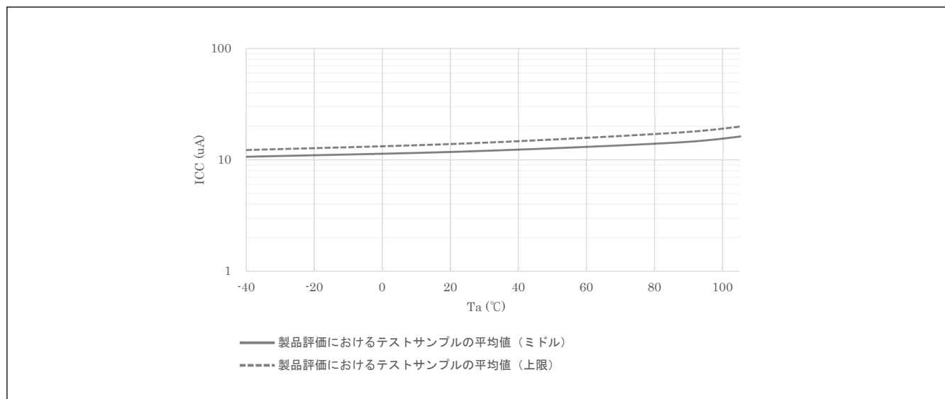
図 47.4 ディープソフトウェアスタンバイモード時の温度依存性、SRAM および USB レジューム検出部への電源供給なし、パワーオンリセット回路、低消費電力機能無効（参考データ）
