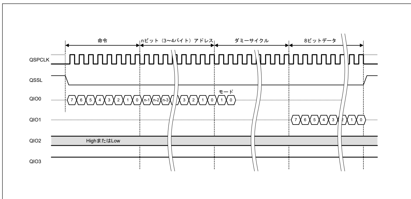
図 31.4 シングル SPI プロトコル例 (ファストリード)
