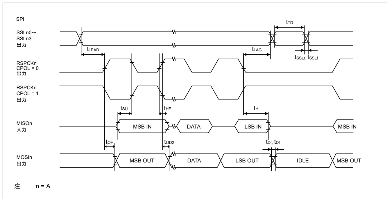
図 47.38 CPHA = 1 でビットレートが PCLKA/2 に設定されている場合におけるマスタの SPI タイミング
