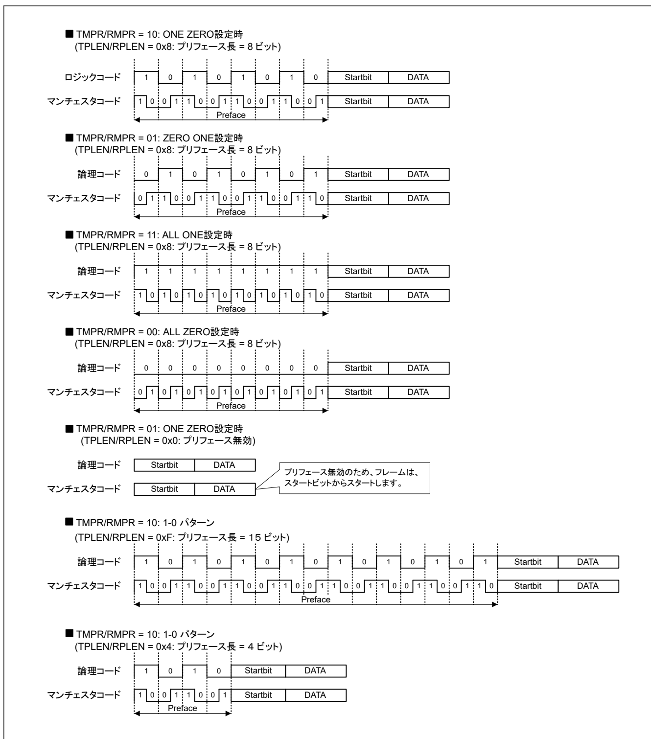
図 27.51 プレフィスパターンの設定例
