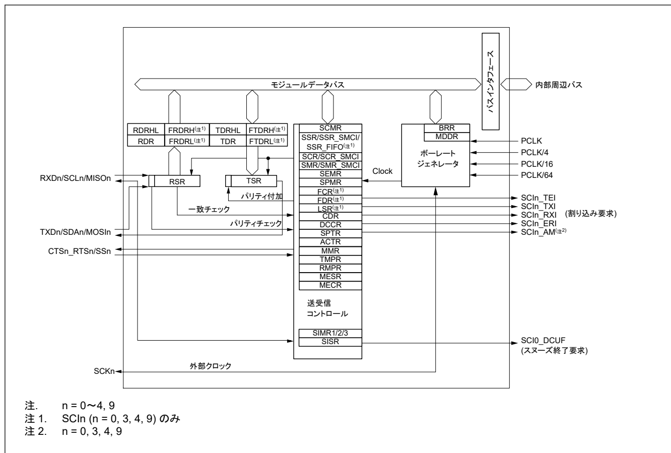
図 27.1 SCI のブロック図
