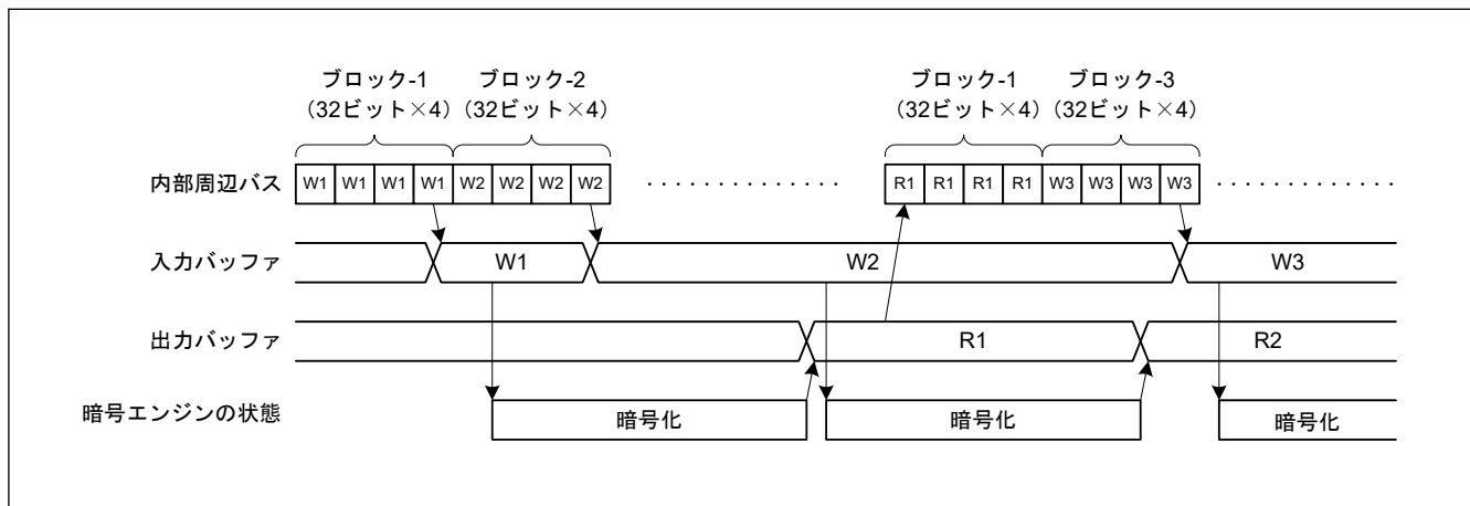
図 36.3 暗号／復号処理タイミング (AES)
