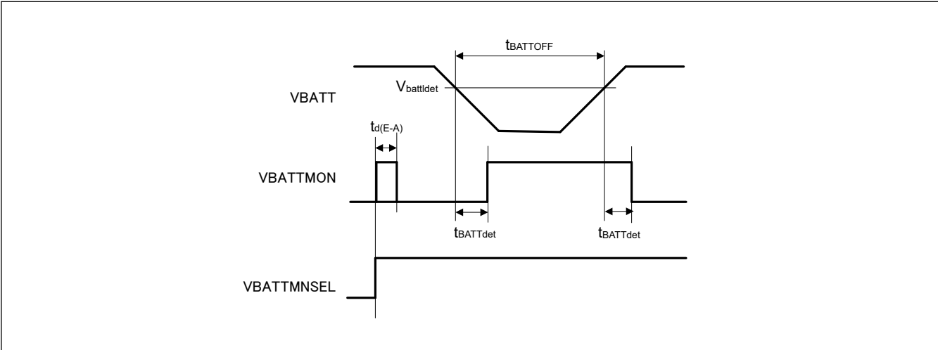
図 47.61 バッテリバックアップ機能特性
