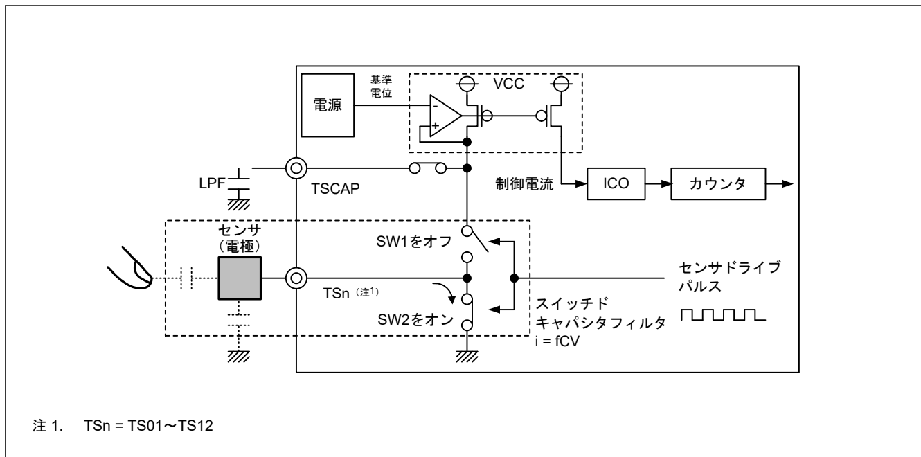
図 40.6 放電動作
