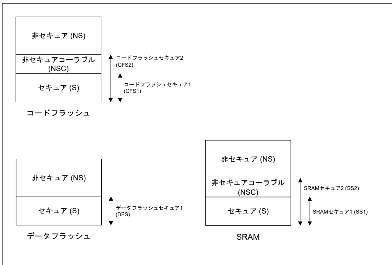
図 46.1 メモリマッピング
