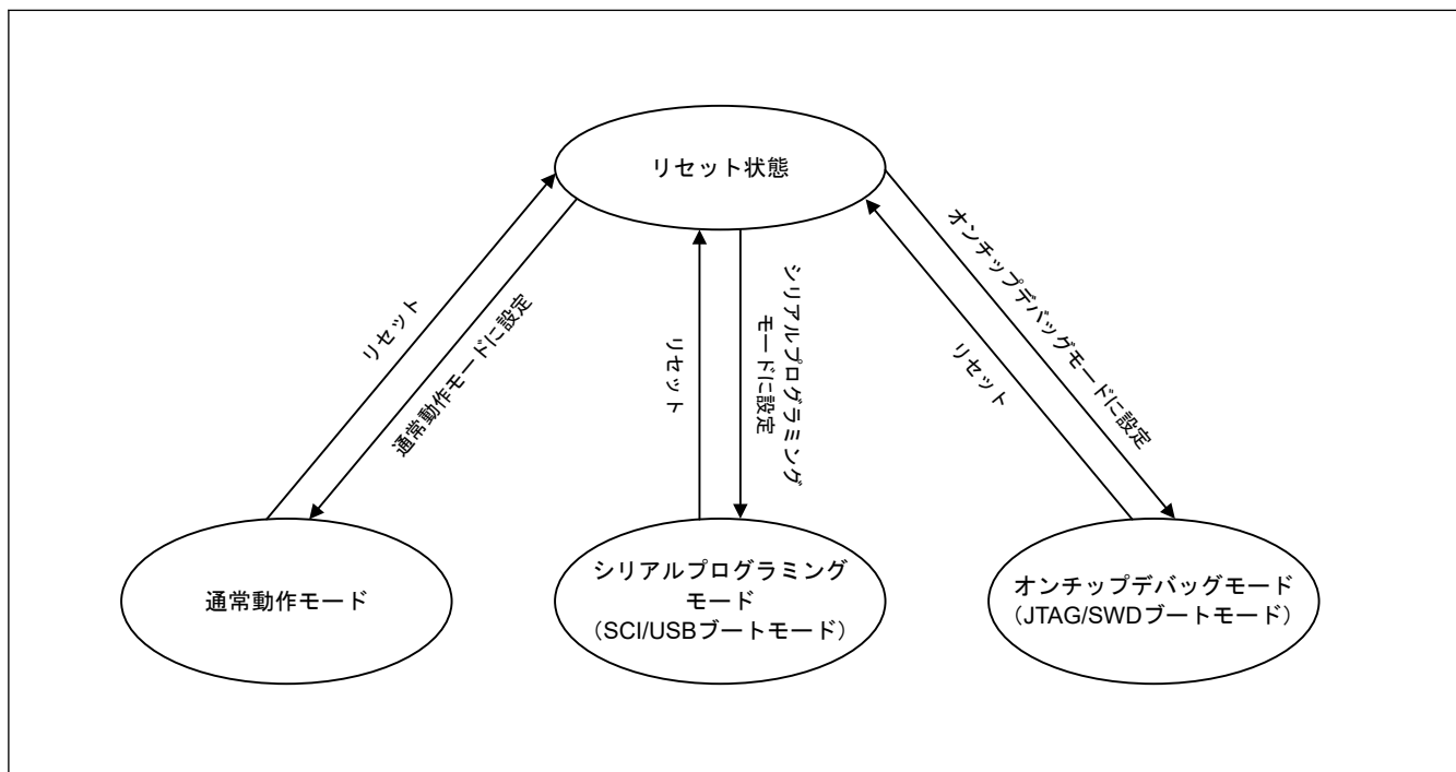
図 44.5 フラッシュメモリに関するモード遷移図
