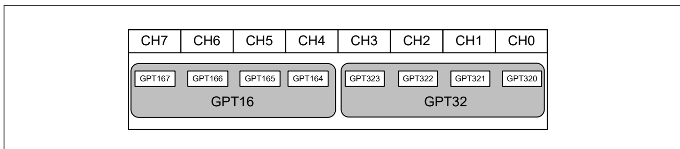
図 21.2 GPT チャネルとモジュール名の関係
