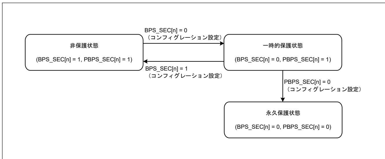
図 44.30 BPS_SEC[n]ビットおよび PBPS_SEC[n]ビットによるフラッシュシーケンサの状態遷移
