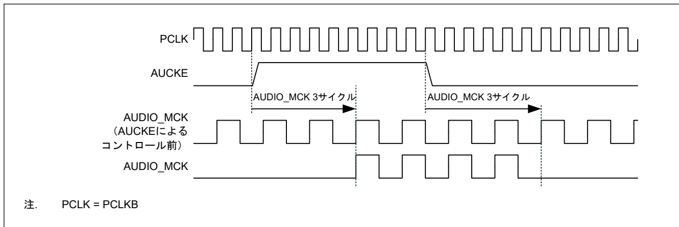
図 32.24 AUDIO_MCK の停止／再開
