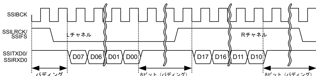
図 32.10 パディングビットの極性
