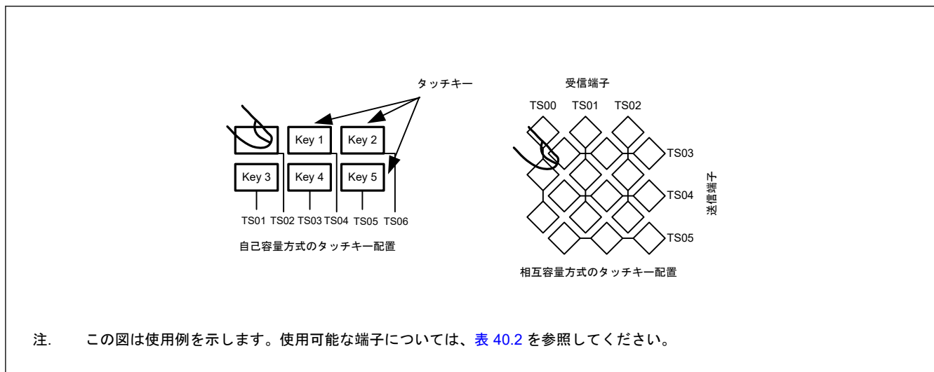
図 40.8 自己容量方式と相互容量方式の概要
