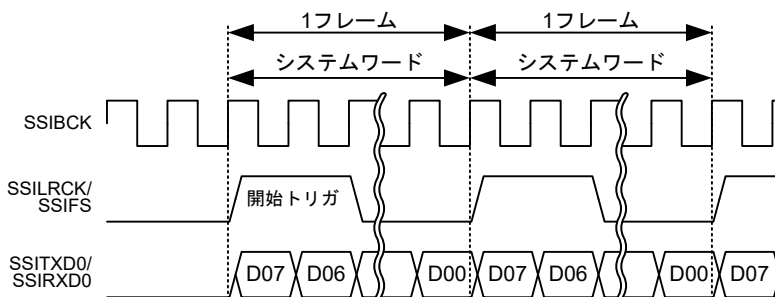
図 32.39 モノラルフォーマットにおけるロングフレーム（パディングなし）
