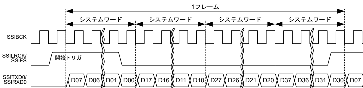
図 32.40 TDM フォーマット（パディングなし、システムワード長 = データワード長）
