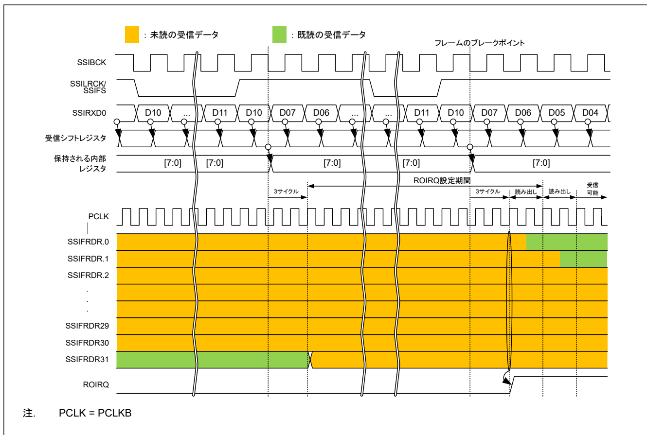
図 32.15 ROIRQ 設定タイミング
