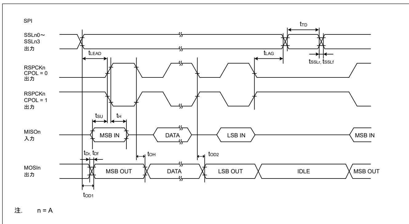
図 47.35 CPHA = 0 の場合におけるマスタの SPI タイミング
