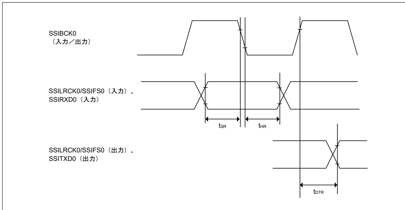
図 47.47 SSICR.BCKP = 1 の場合の SSIE データ送受信タイミング
