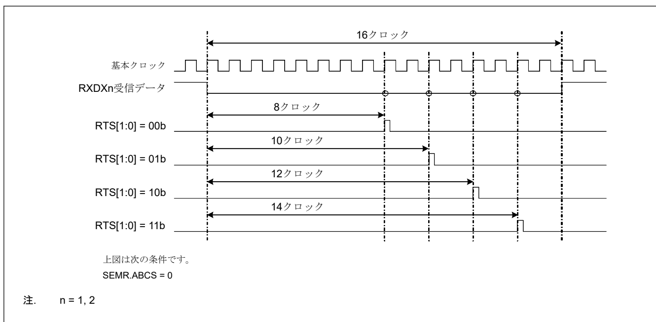
図 27.114 RXDXn 受信データサンプリングタイミング
