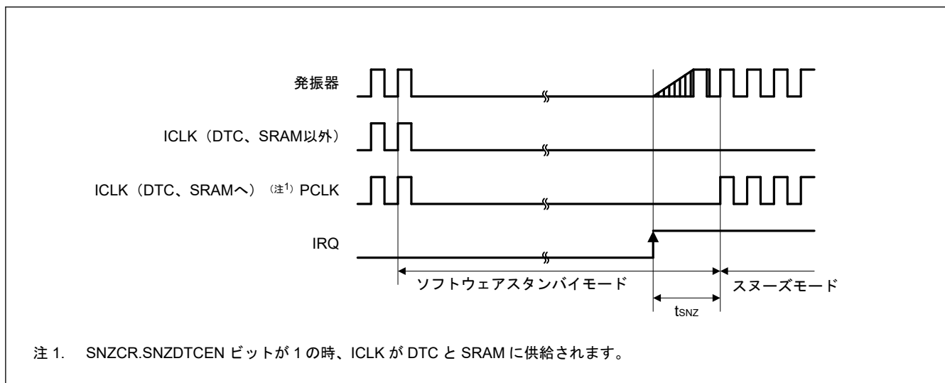
図 47.16 ソフトウェアスタンバイモードからスヌーズモードへの復帰タイミング
