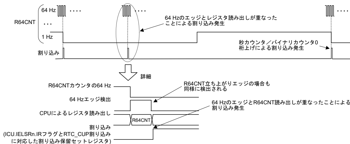
図 23.12 桁上げ割り込み (RTC_CUP) のタイミング図
