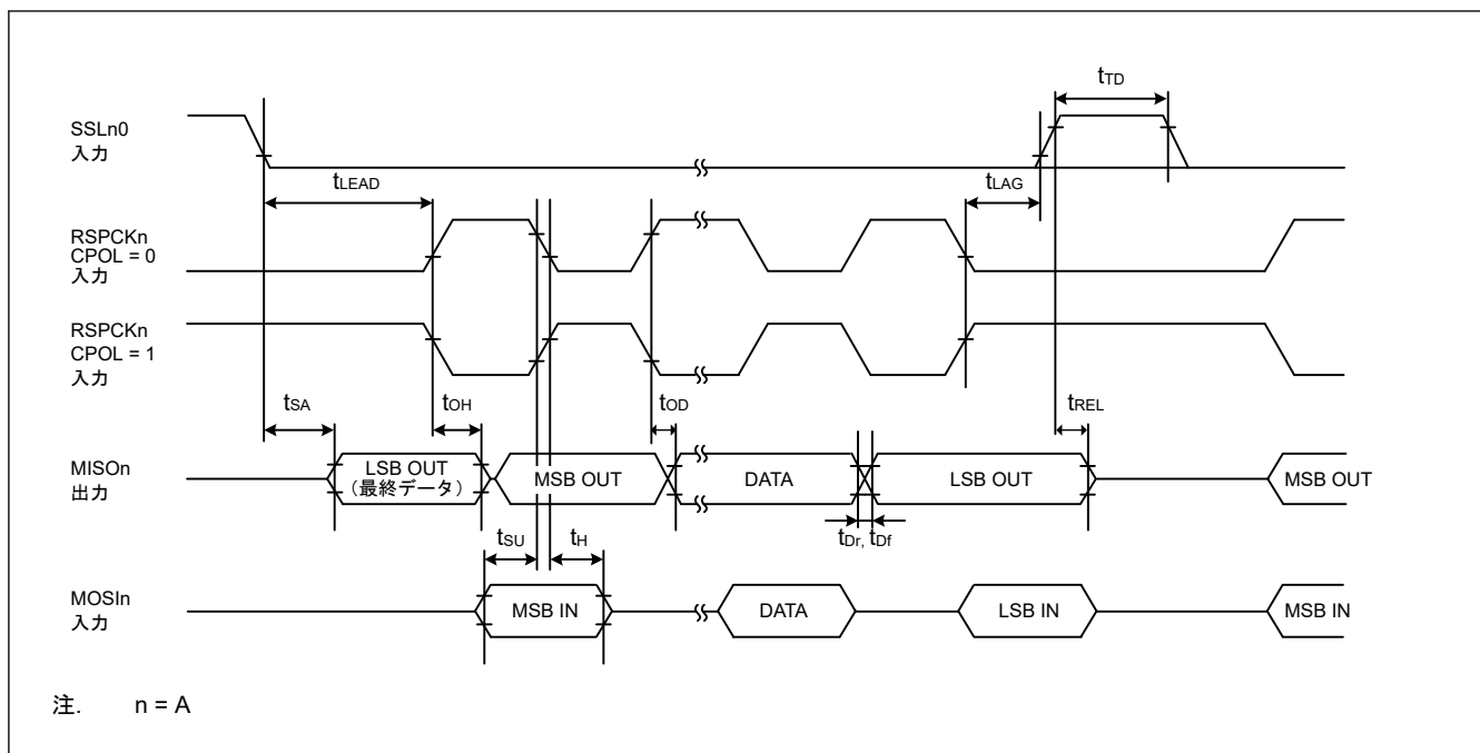
図 47.40 CPHA = 1 の場合におけるスレーブの SPI タイミング
