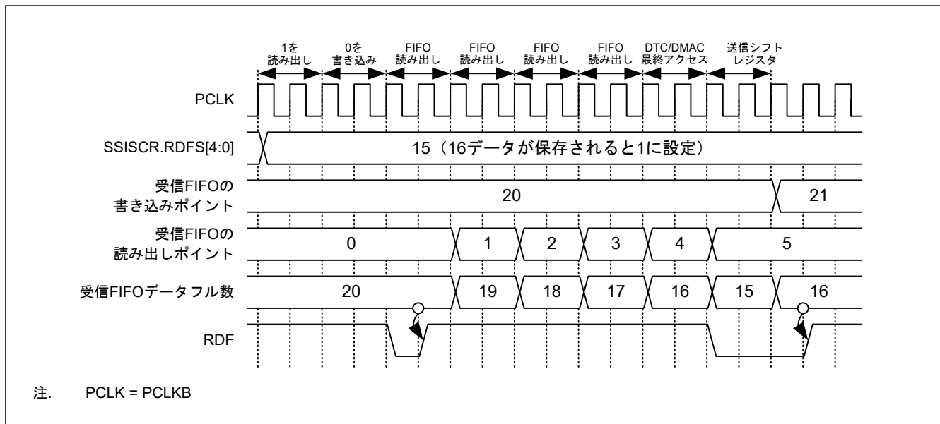
図 32.27 RDF の設定およびクリアに関するタイミング図
