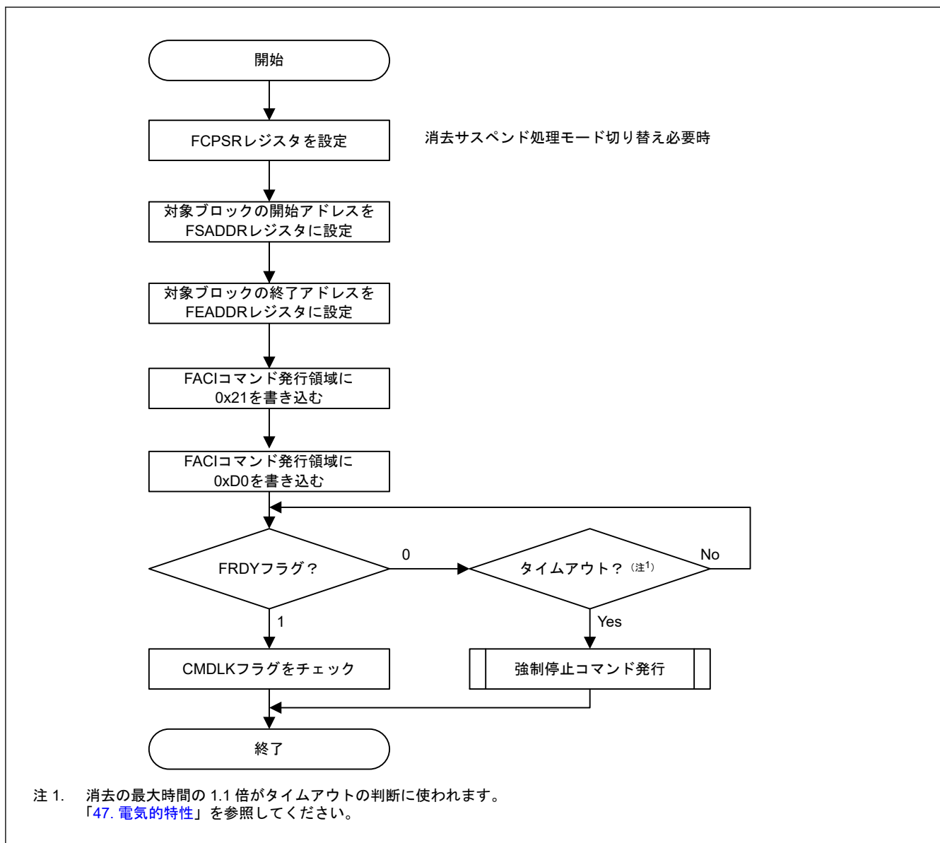
図 44.15 マルチブロックコマンドの使用フロー
