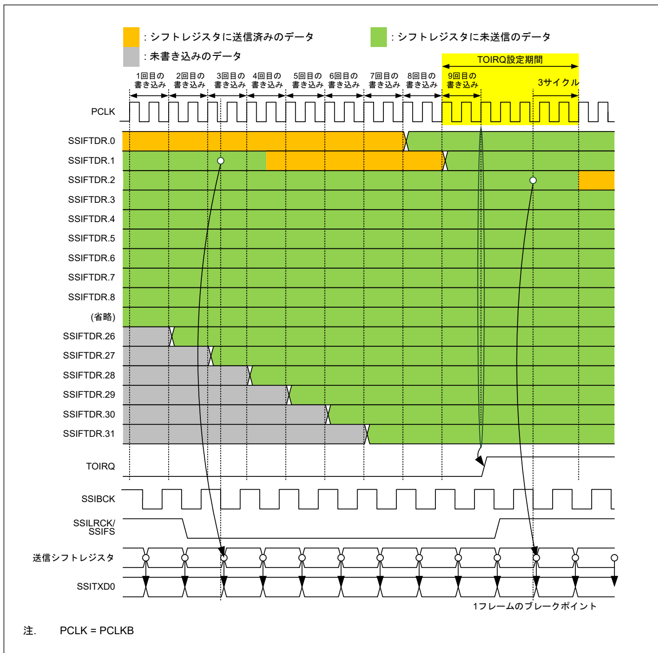
図 32.17 TOIRQ 設定タイミング
