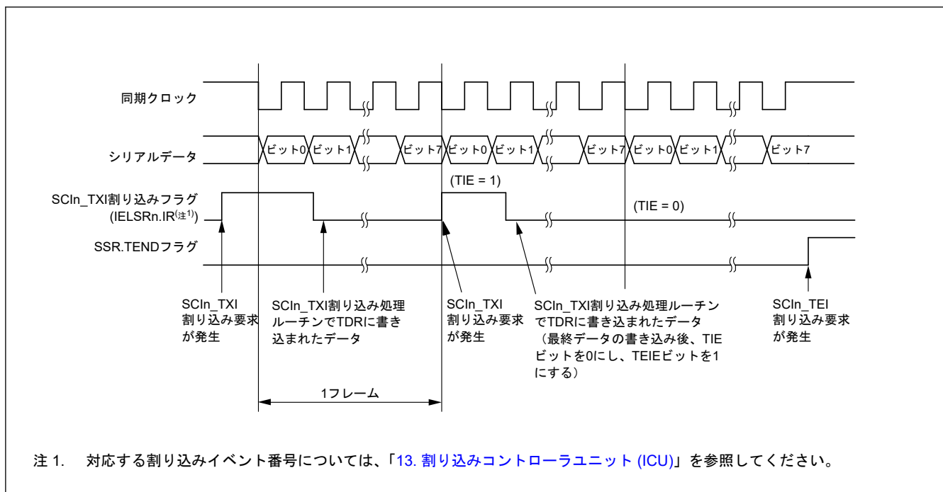
図 27.68 クロック同期式モードにおけるシリアル送信の動作例 (送信中～送信終了時)
