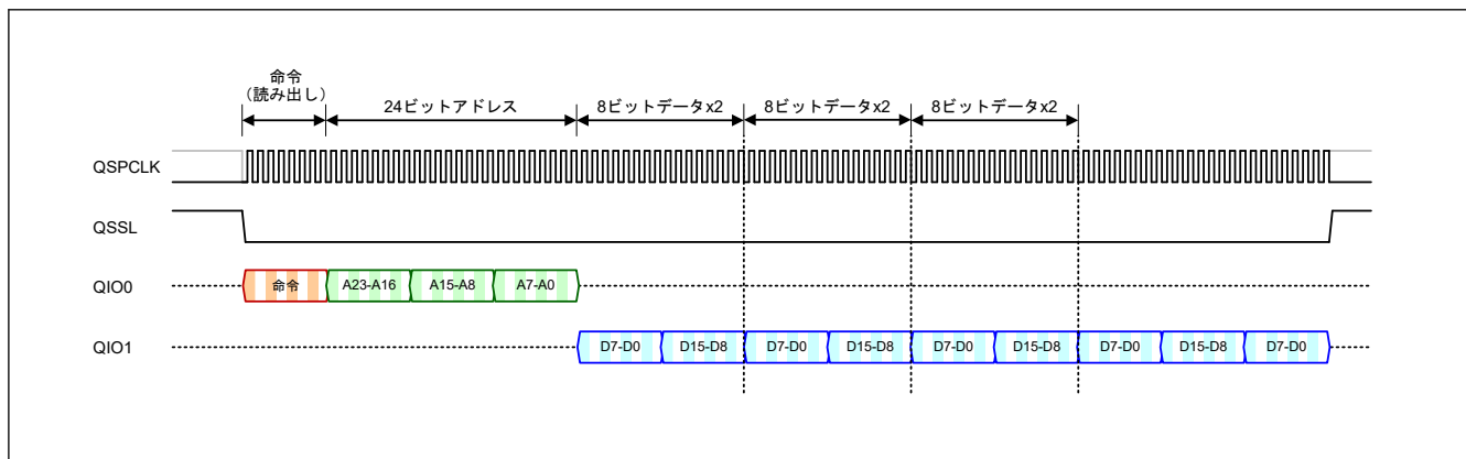
図 31.33 プリフェッチ機能を使用した連続データリード動作
