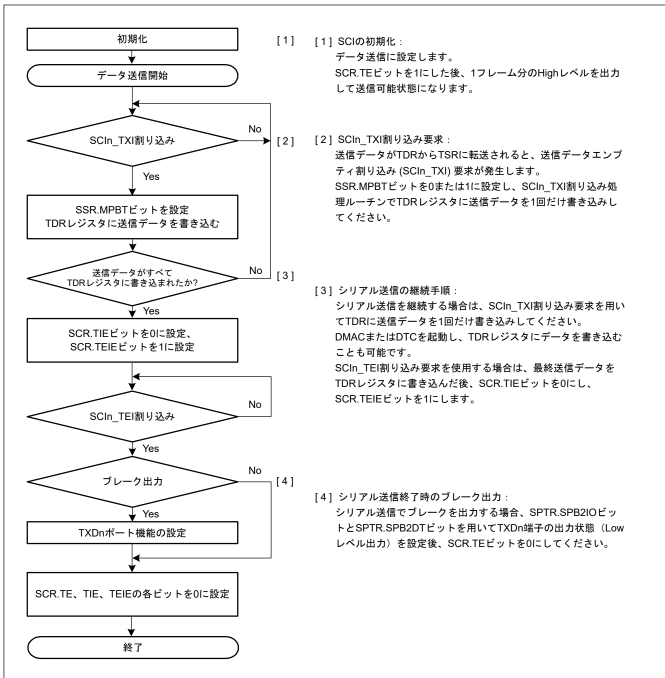
図 27.41 マルチプロセッサシリアル送信のフローチャート例 (非 FIFO 選択時)
