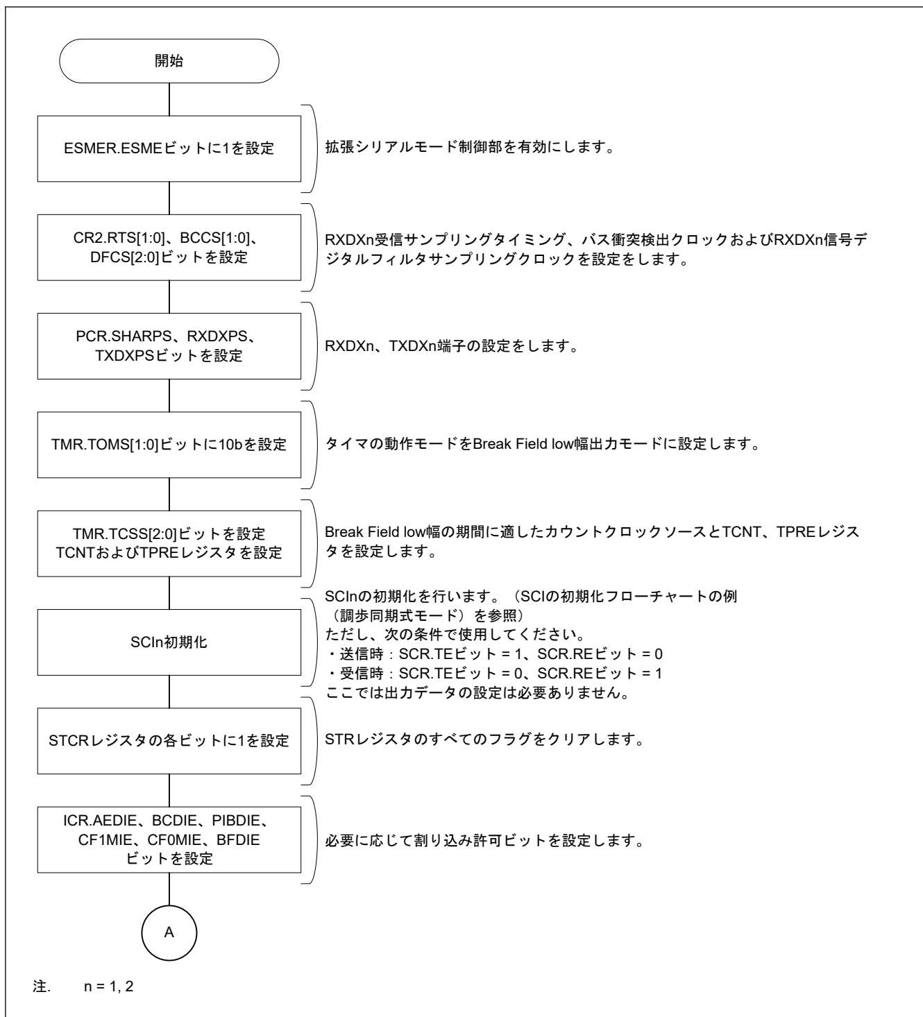
図 27.103 Start Frame 送信フローチャート例 (1/2)
