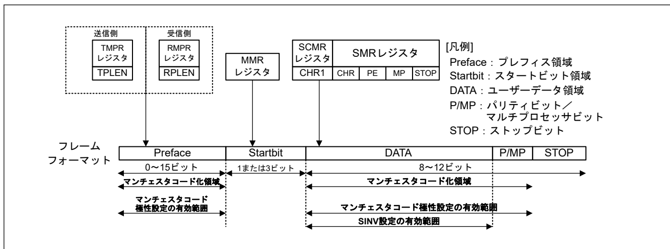
図 27.50 マンチェスタモードでのフレームフォーマット
