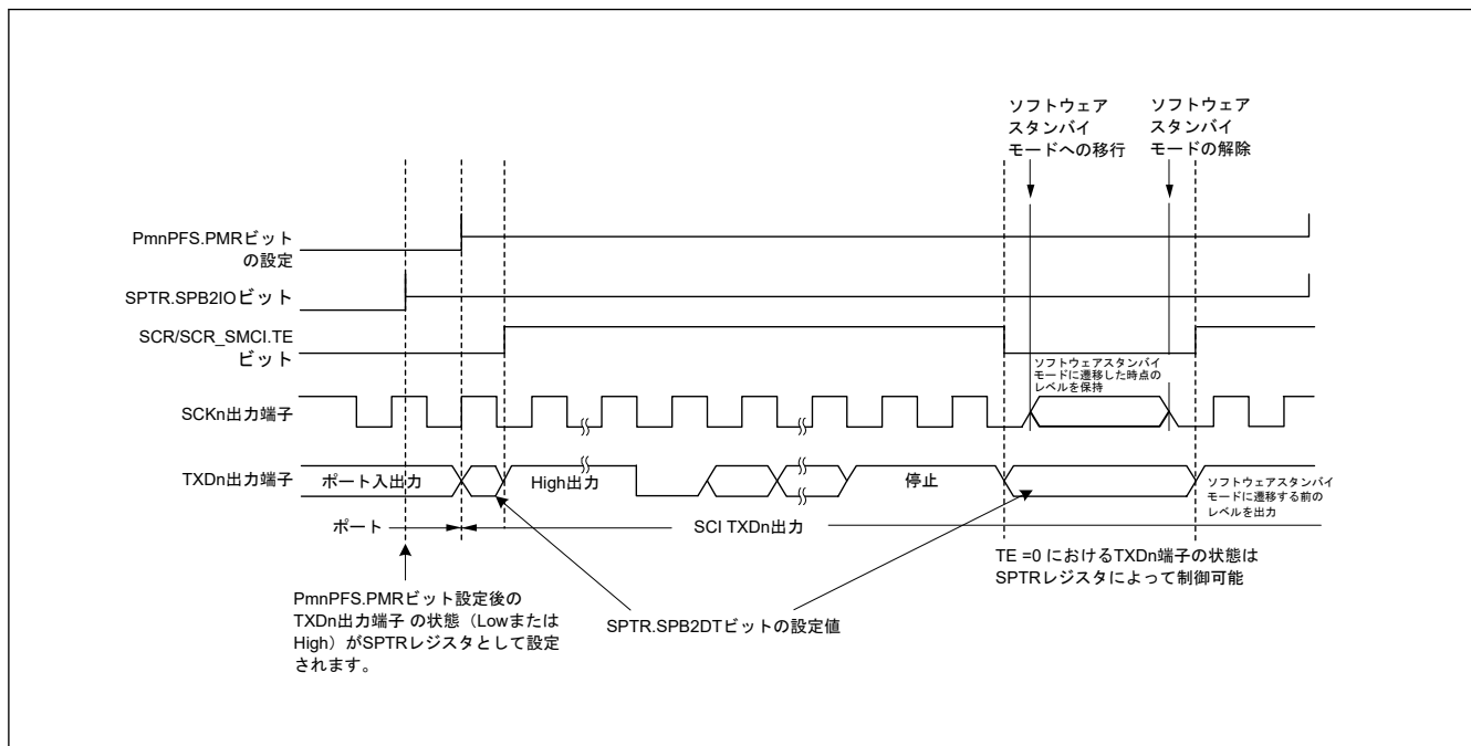
図 27.119 ソフトウェアスタンバイモード遷移中のポートの端子状態 (内部クロック、調歩同期式送信)
