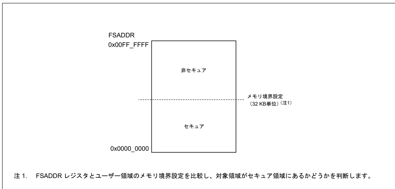
図 44.31 ユーザー領域のセキュア／非セキュア領域
