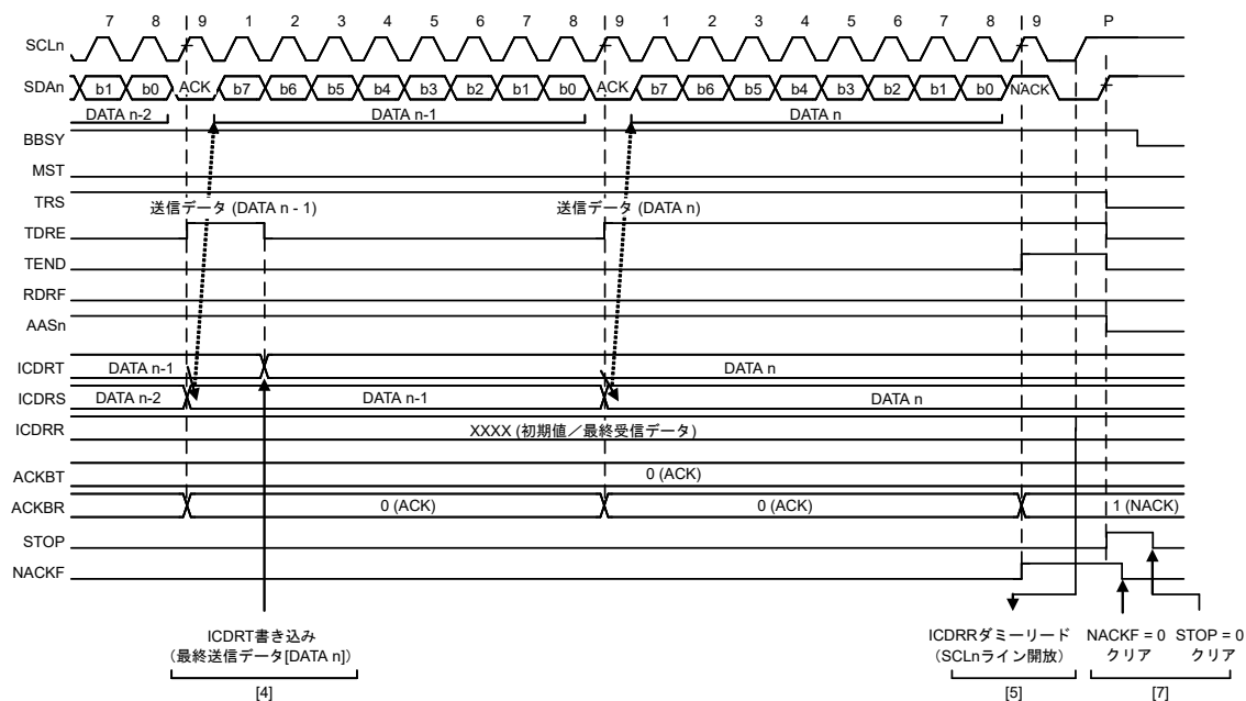
図 28.17 スレープ送信の動作タイミング (2)
