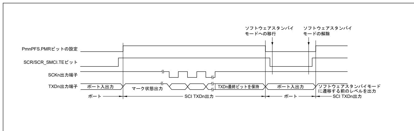
図 27.120 ソフトウェアスタンバイモード遷移中のポートの端子状態（内部クロック、クロック同期式送信）
