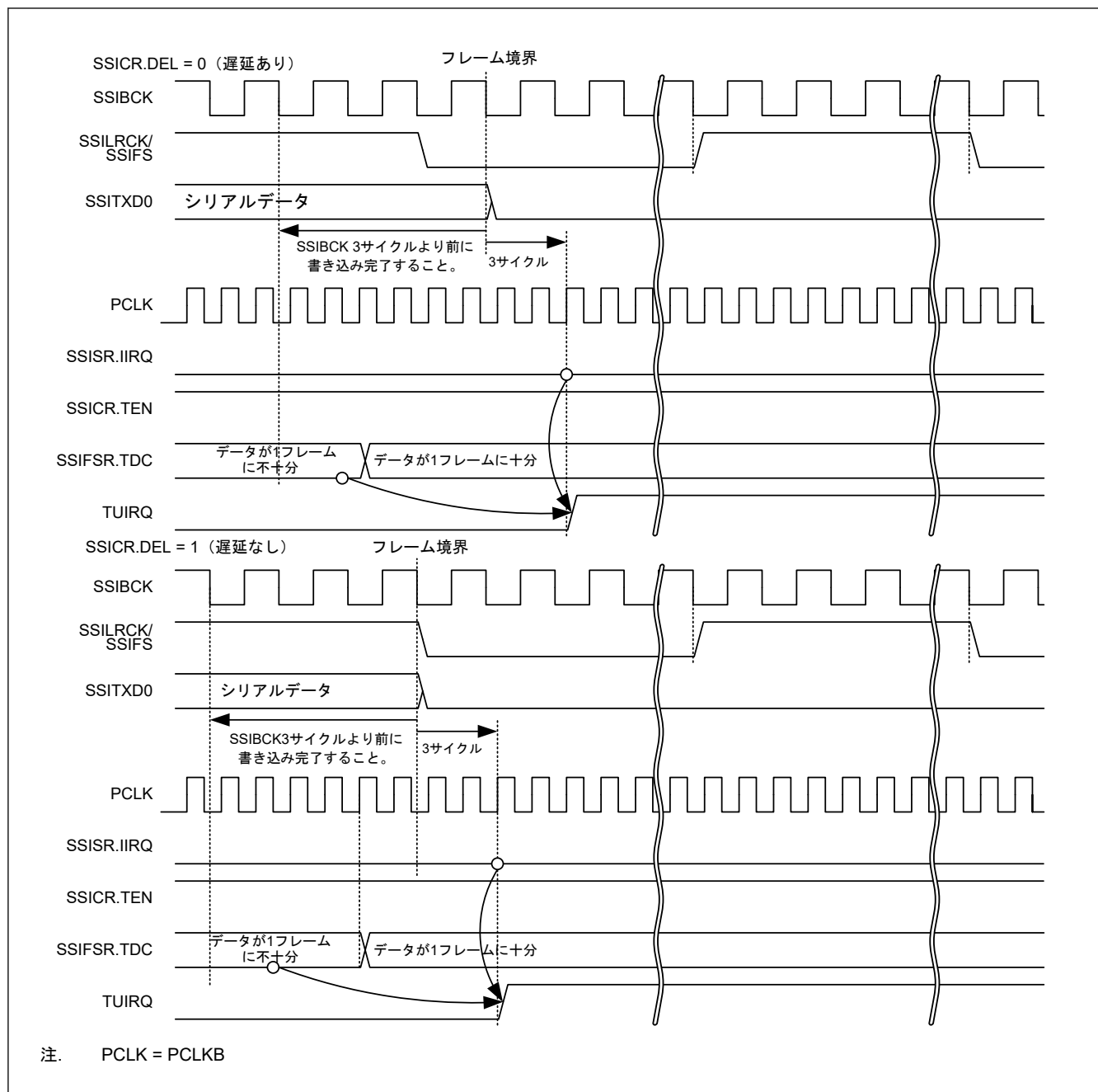
図 32.19 TUIRQ 設定タイミング (通信継続時)
