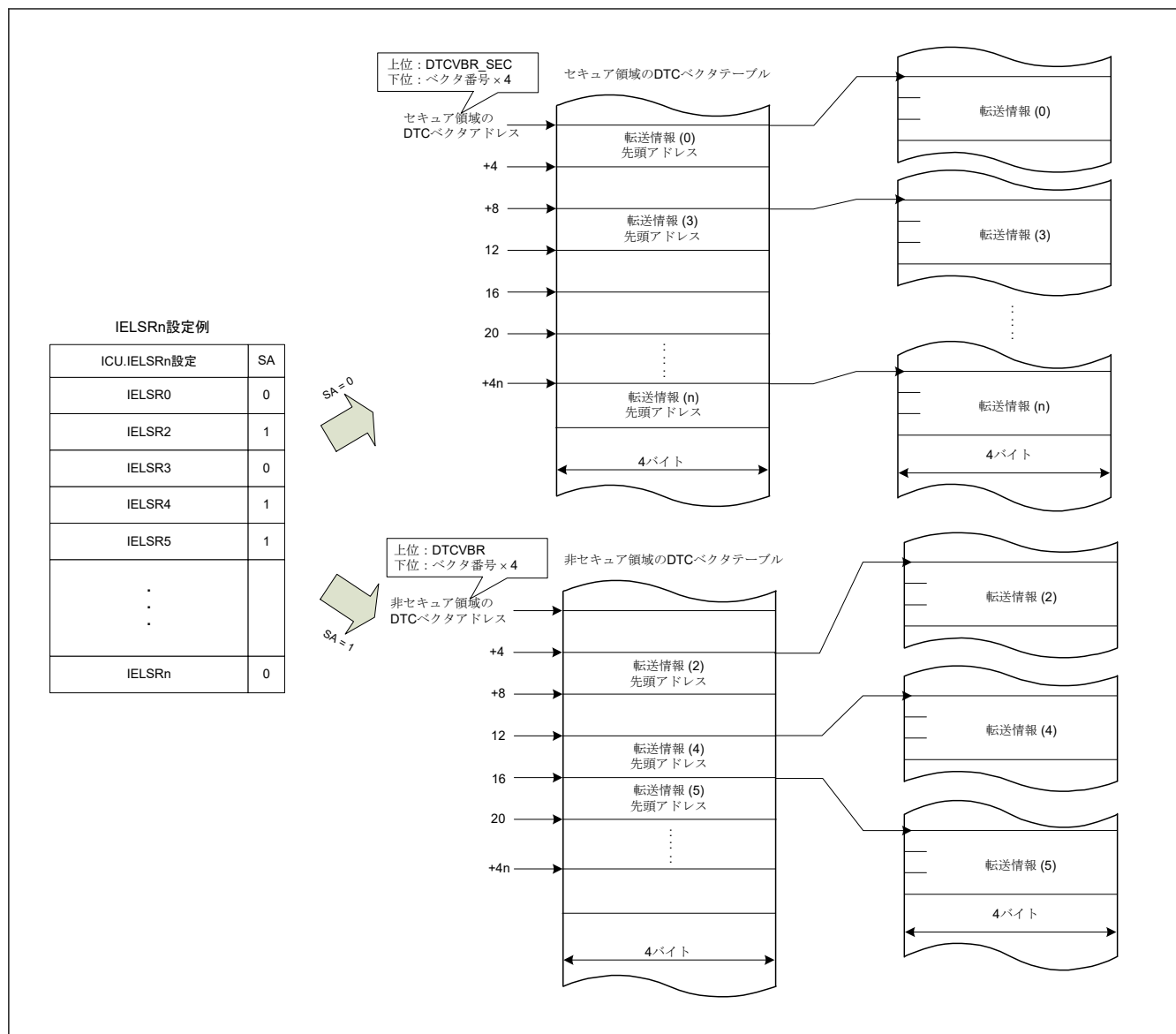
図 17.2 DTC ペクタテーブルと転送情報の対応関係
