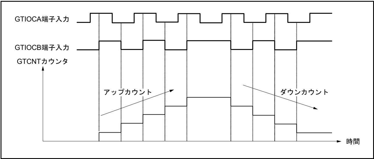
図 23.74 位相計数モード4 動作例
