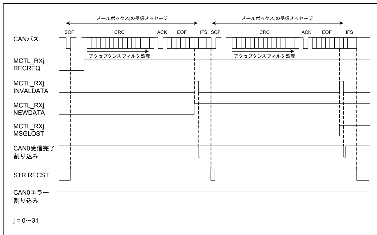
図 31.18 データフレーム受信時の動作例（オーバーライトモードの場合）
