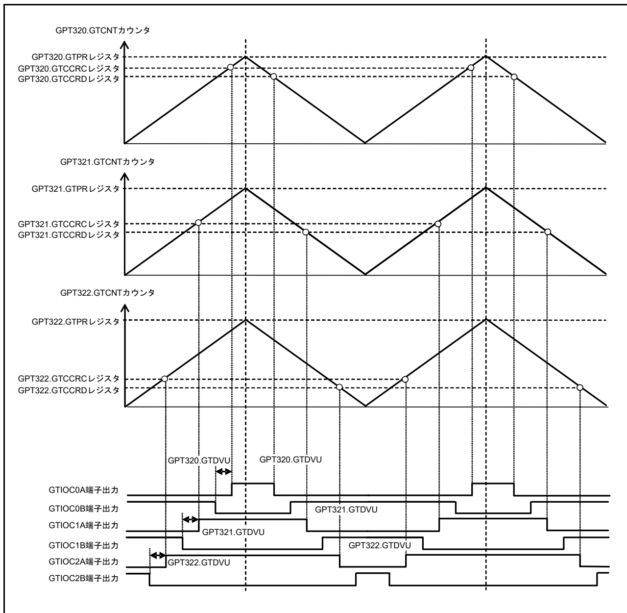
図 23.66 非対称三角波 3 相相補 PWM 出力例 (デッドタイム自動設定)
