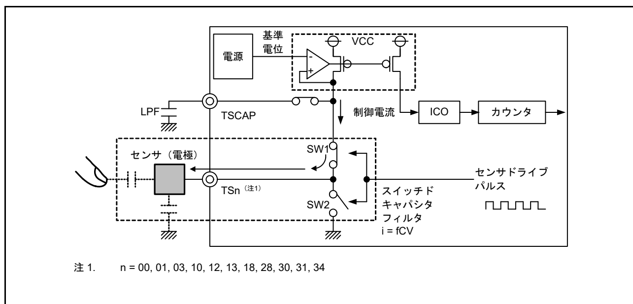
図 40.5 充電動作
