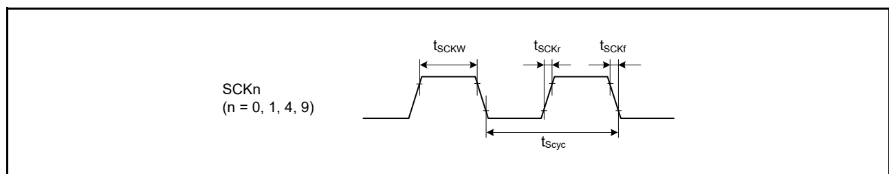
図 48.41 SCK クロック入力タイミング
