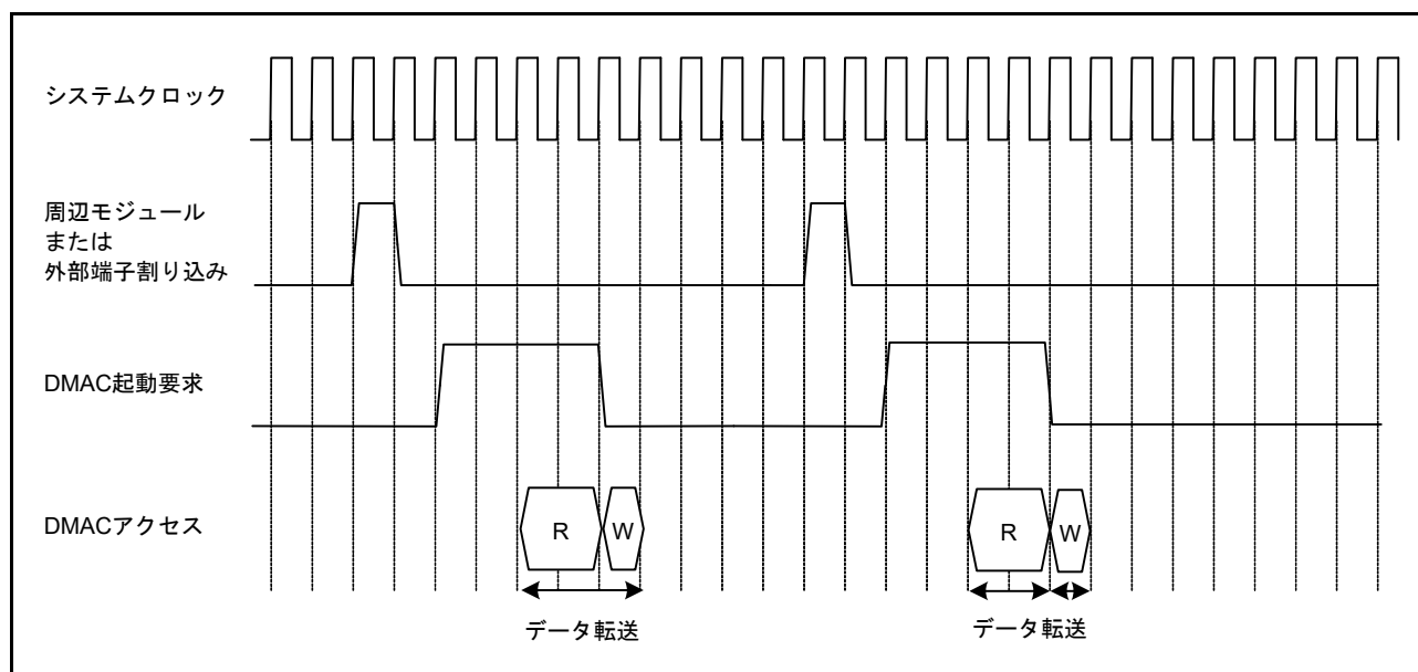
図 17.10 DMAC 動作タイミング例 1 (ノーマル転送モードまたはリポート転送モードでの周辺モジュール/外部割り込み入力端子からの割り込みによる DMA 起動)
