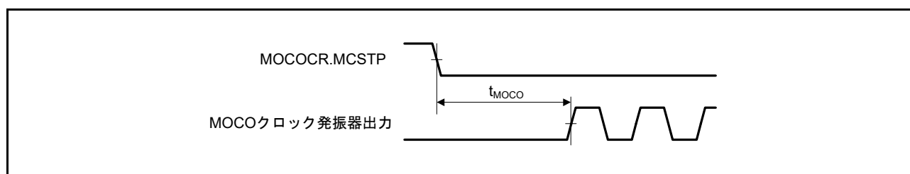
図 48.28 MOCO クロック発振開始タイミング
