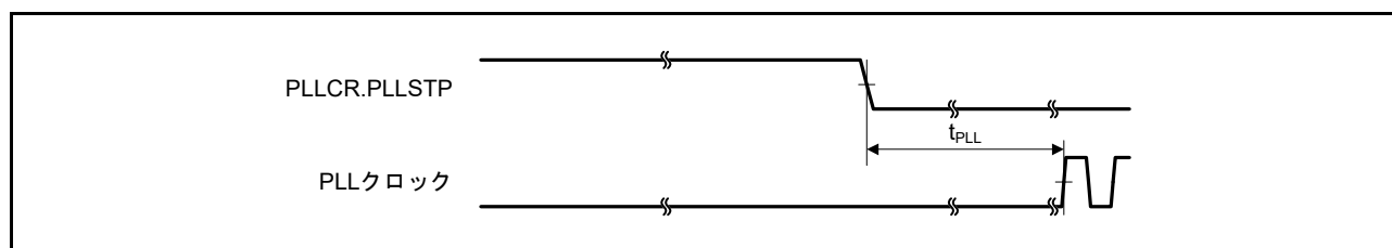
図 48.26 PLL クロック発振開始タイミング（メインクロックの発振安定後に PLL を動作させたとき）
