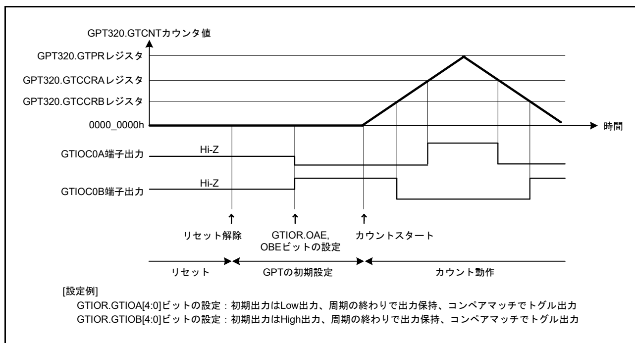
図 23.85 リセット後の端子設定例
