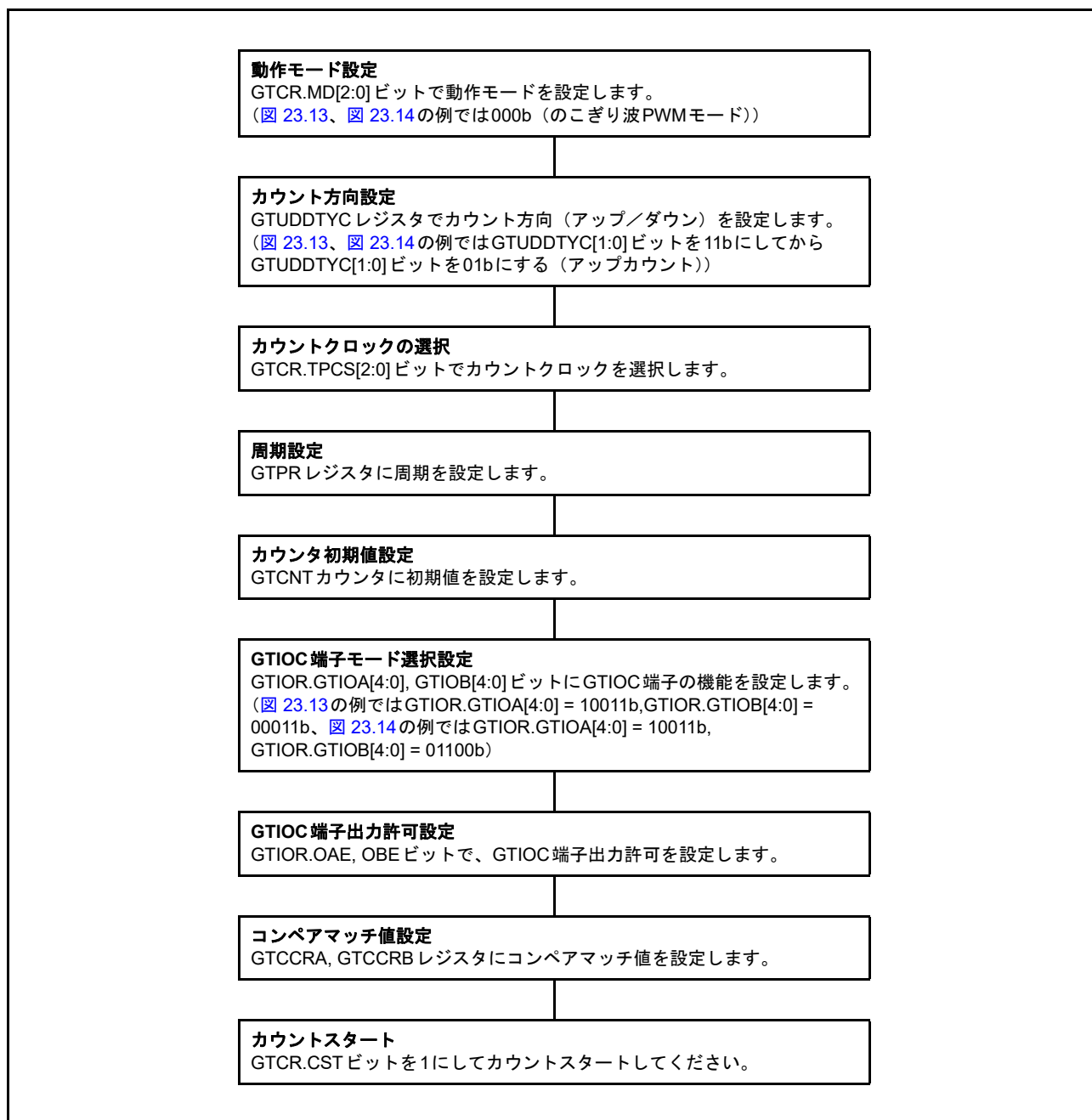
図 23.15 トグル出力動作の設定例
