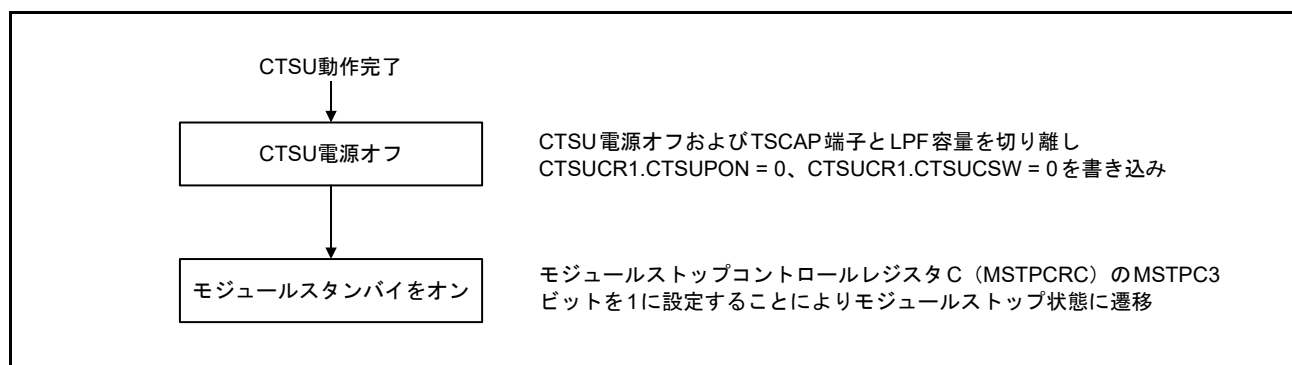
図 40.10 CTSU 停止フロー
