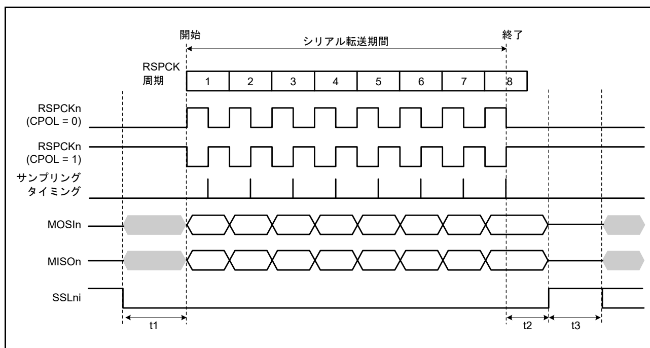
図 32.27 SPI 転送フォーマット (CPHA ビット = 1)
