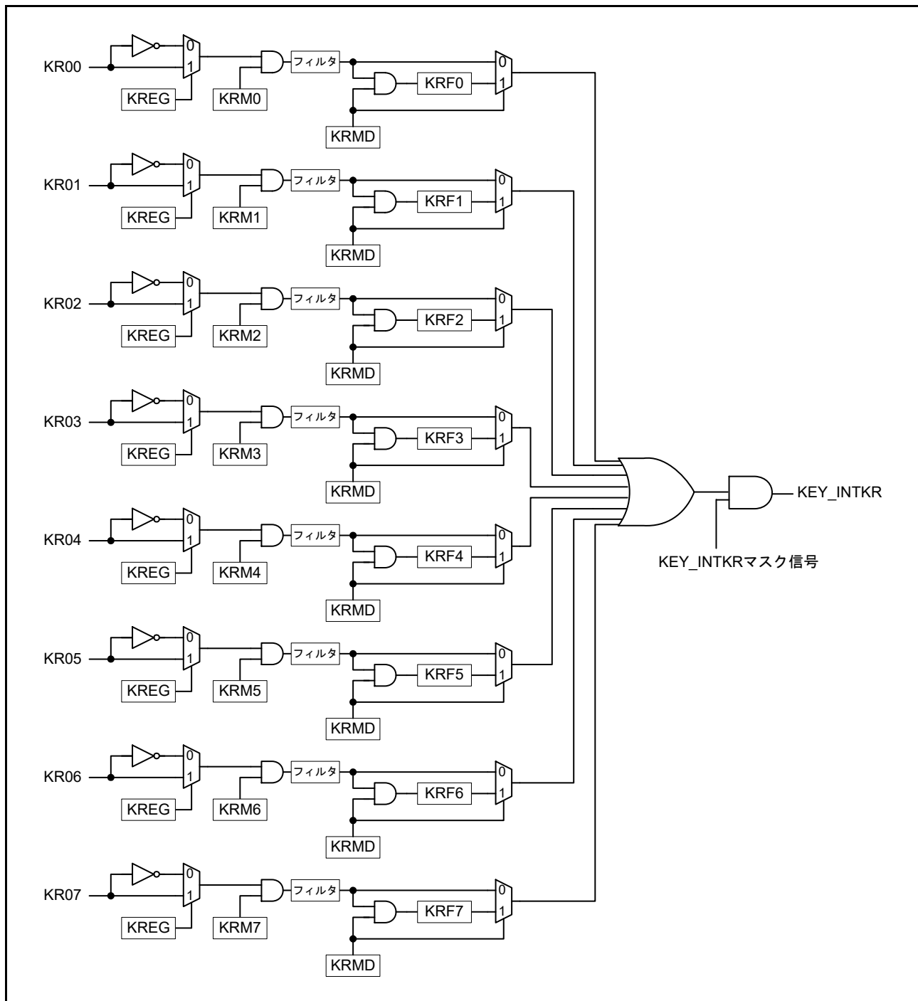
図 21.1 キー割り込み機能のブロック図
