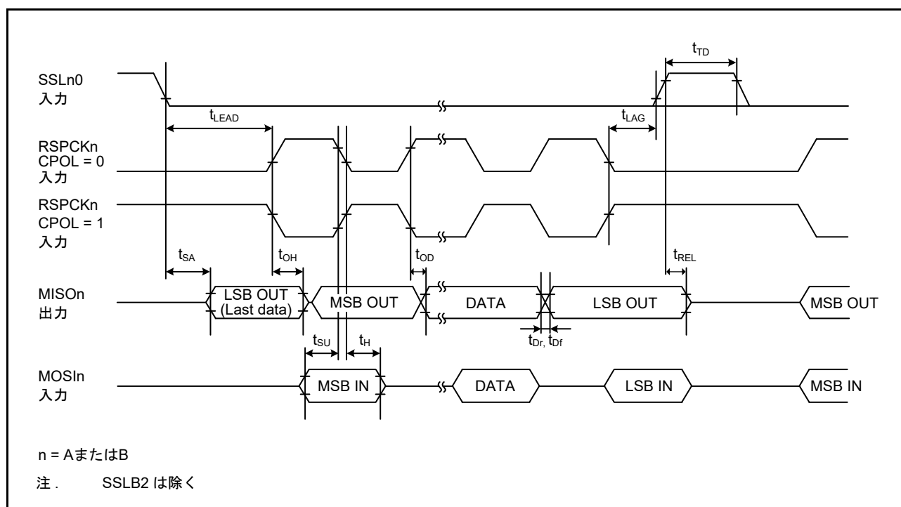
図 48.55 SPI タイミング (スレーブ、CPHA = 1)
