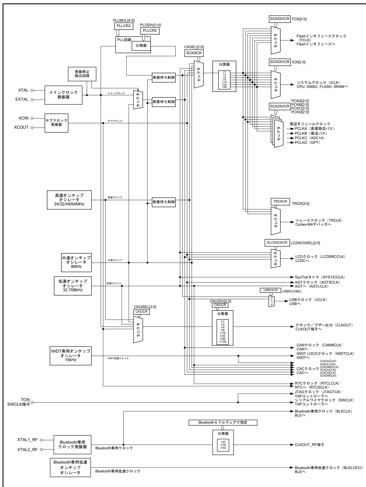
図 9.1 クロック発生回路のブロック図
