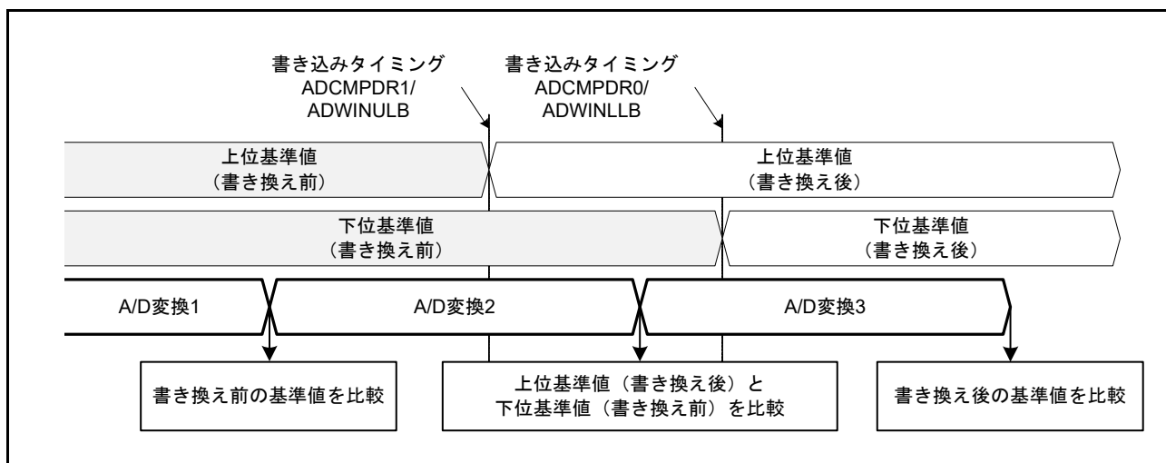
図 34.4 書き換え前後の上側基準値と下側基準値の比較
