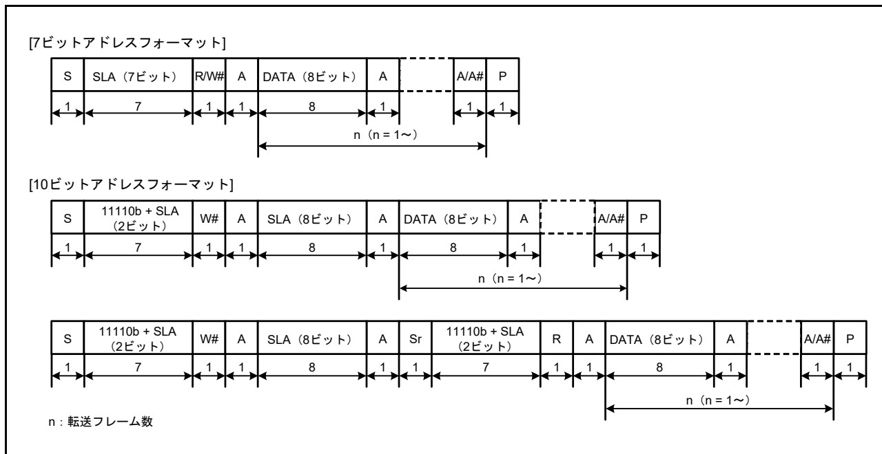
図 30.3 I 2 C バスフォーマット
