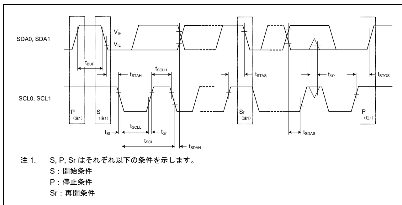
図 48.56 I 2 C バスインタフェース入出力タイミング
