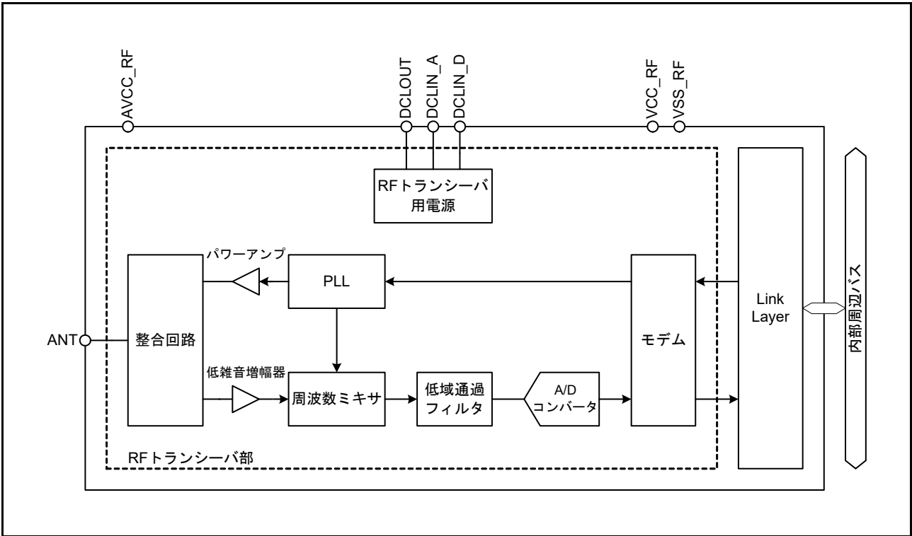
図 46.1 BLE のブロック図
