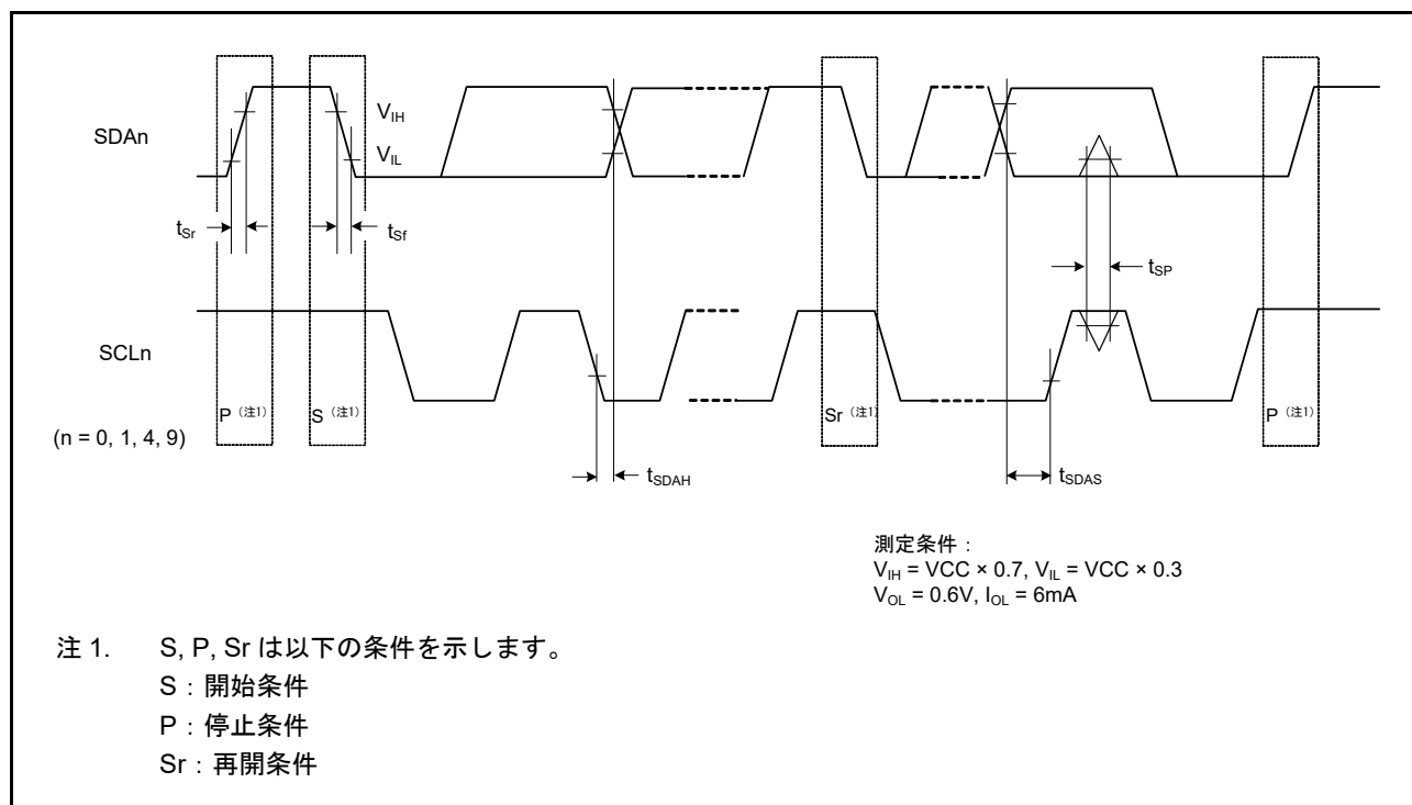
図 48.48 SCI 簡易 IIC モードタイミング
