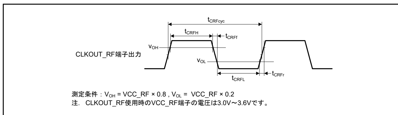
図 48.58 CLKOUT_RF 出力タイミング
