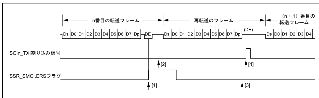
図 29.52 SCI 送信モードでの再転送動作
