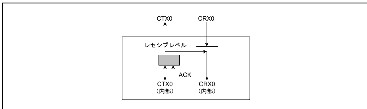
図 31.8 セルフテストモード 1 選択時の接続
