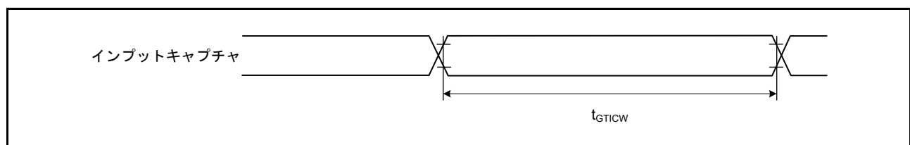
図 48.37 GPT インプットキャプチャタイミング
