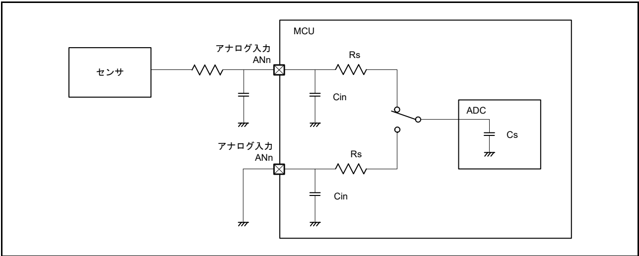
図 48.63 アナログ入力の等価回路
