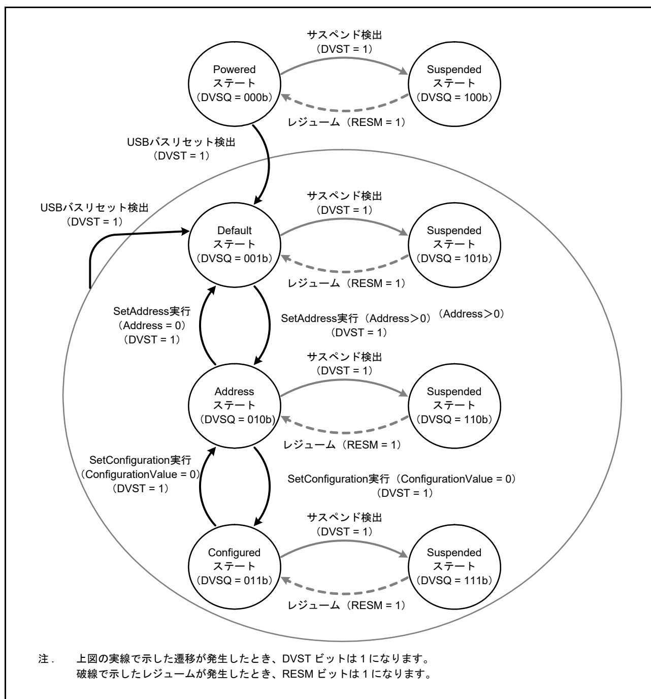
図 28.11 デバイスステートの遷移
