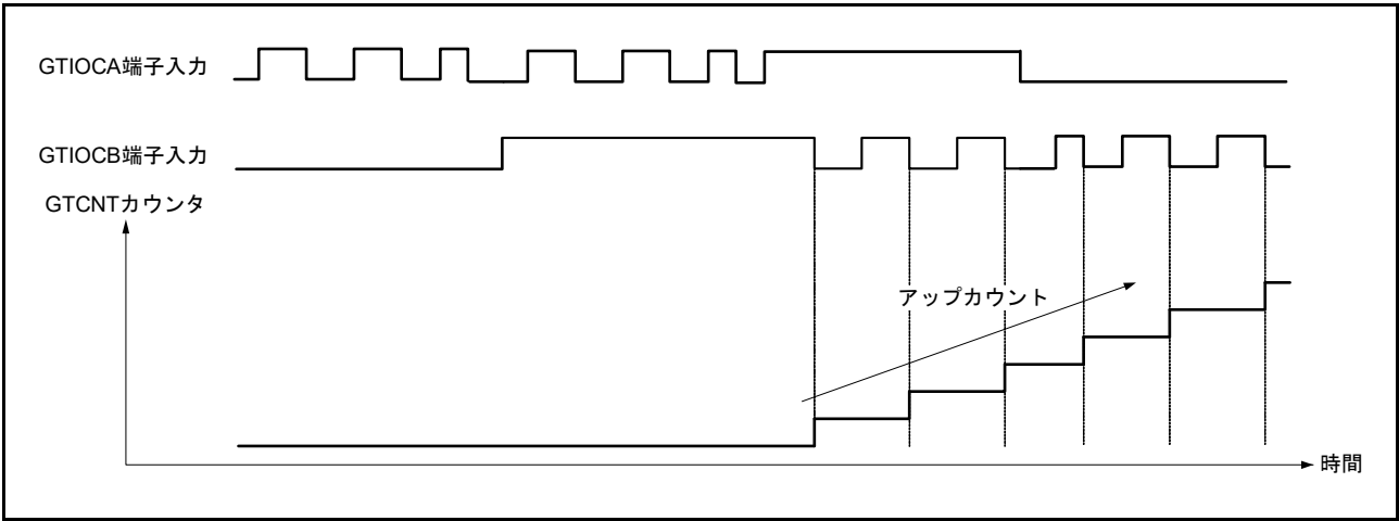
図 23.76 位相計数モード 5 動作例 (B)
