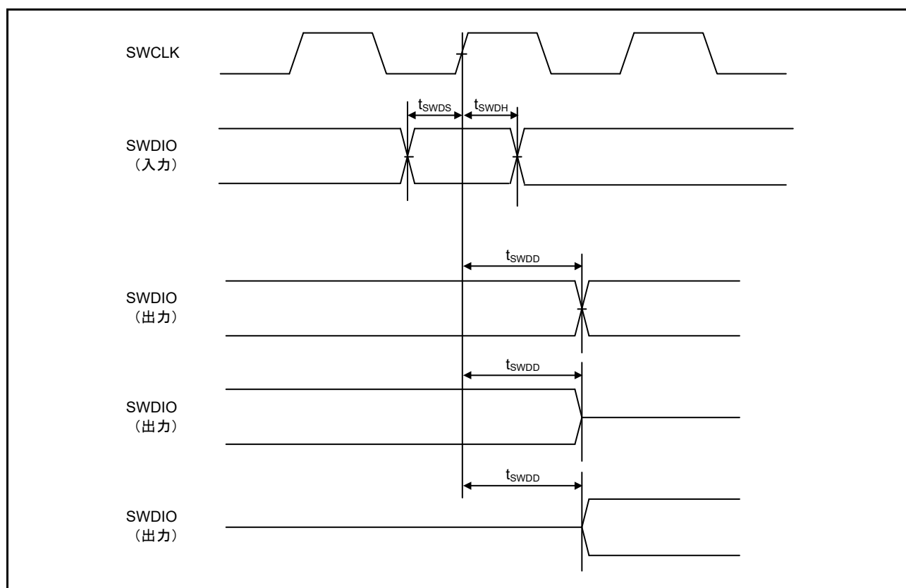
図 48.77 SWD 入出力タイミング
