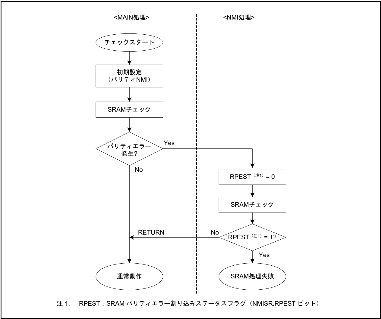
図 42.3 SRAM パリティ割り込み許可の場合の SRAM パリティチェックのフロー
