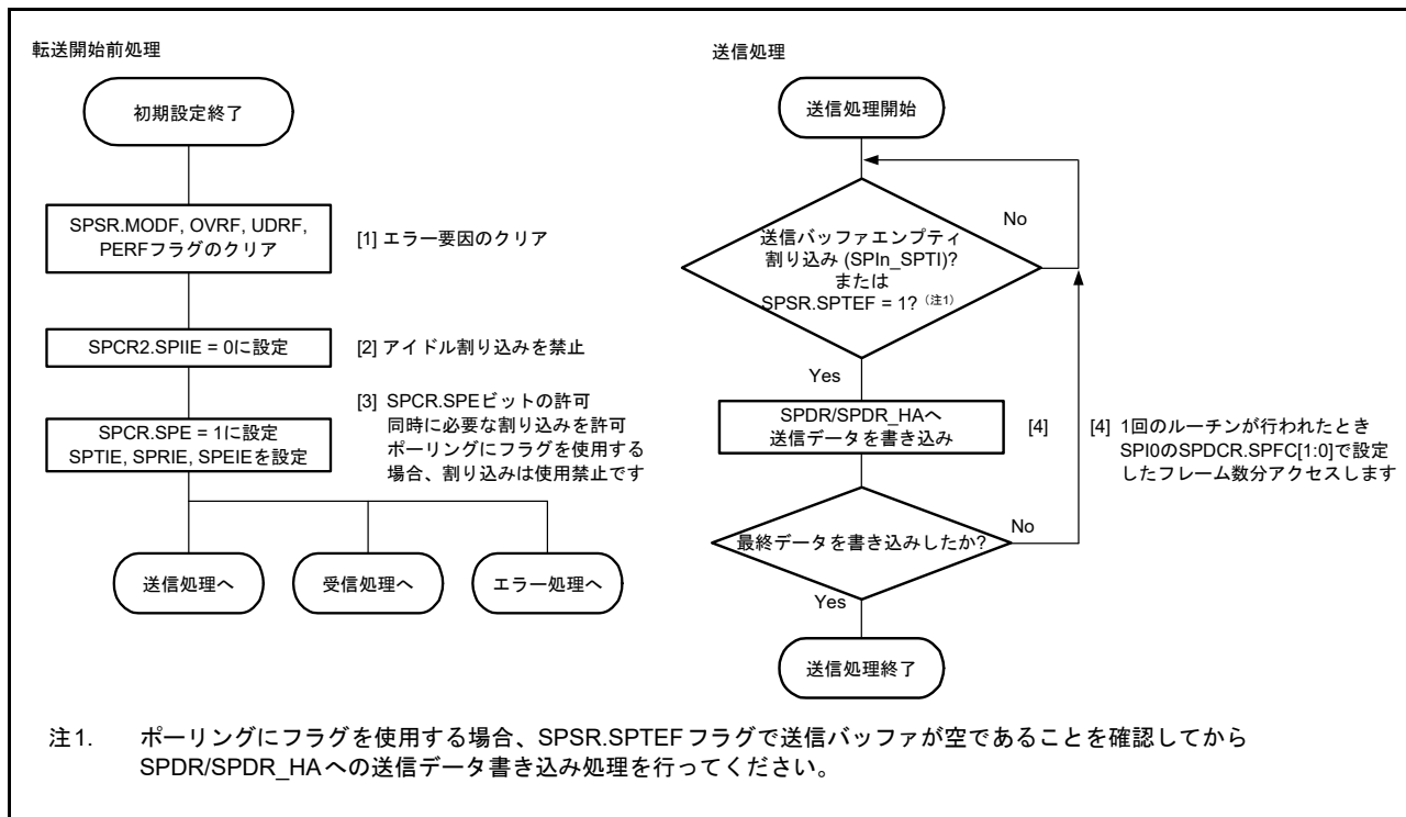
図 32.48 スleepモードでの送信フロー
