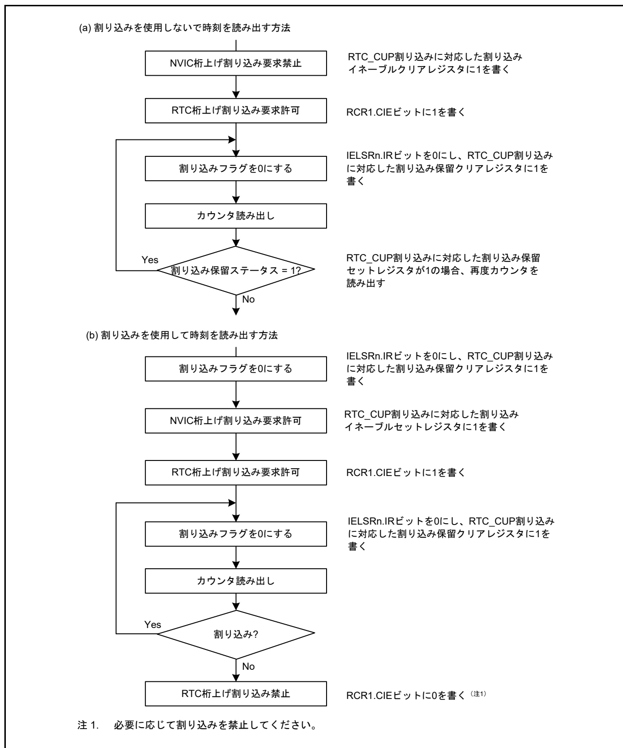
図 25.6 時刻読み出し
