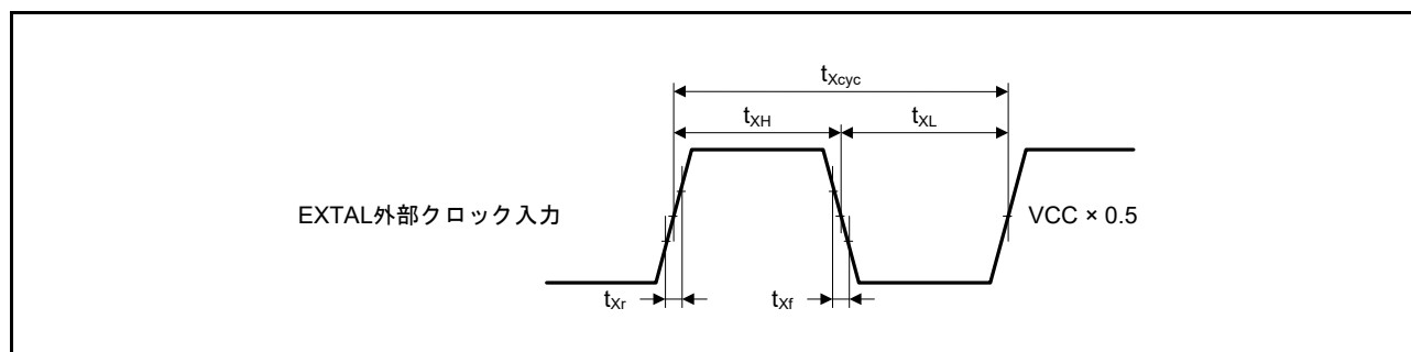
図 48.22 EXTERNAL 外部クロック入力タイミング
