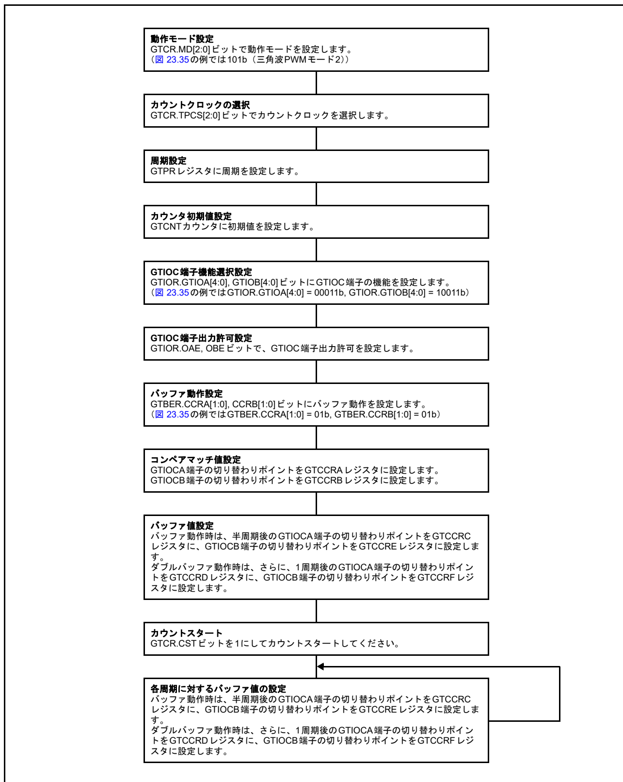
図 23.36 三角波 PWM モード 2 の設定例
