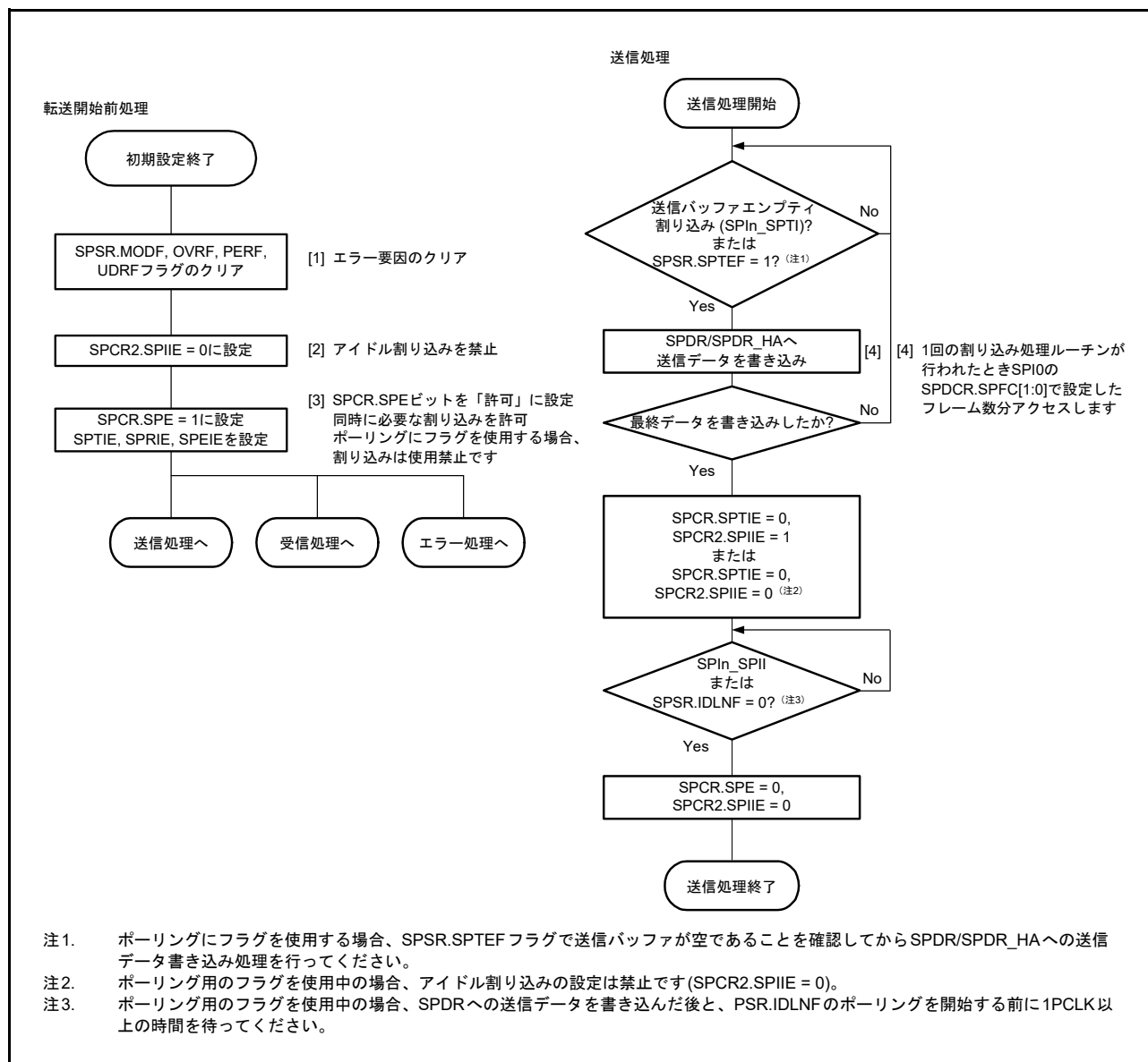
図 32.44 マスタモードでの送信フロー
