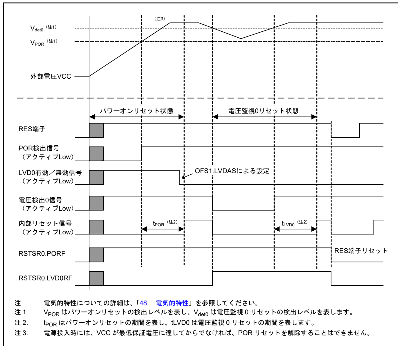
図 8.3 電圧監視 0 リセットの動作例
