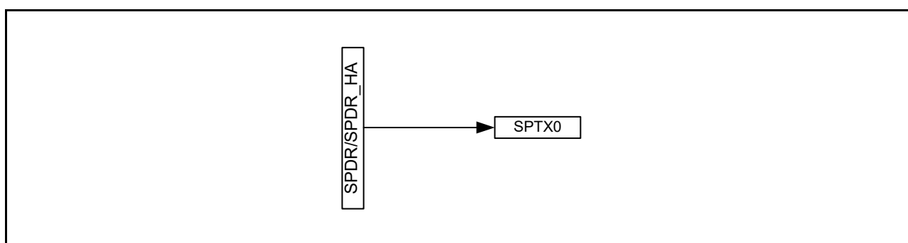
図 32.5 書き込み時の SPDR/SPDR_HA レジスタの構成図 (SPI1 の場合)
