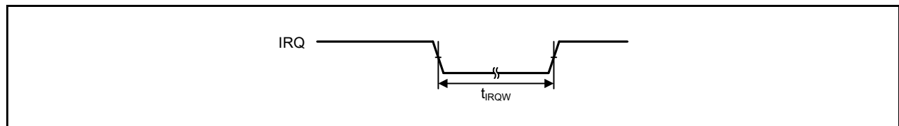
図 48.34 IRQ 割り込み入力タイミング
