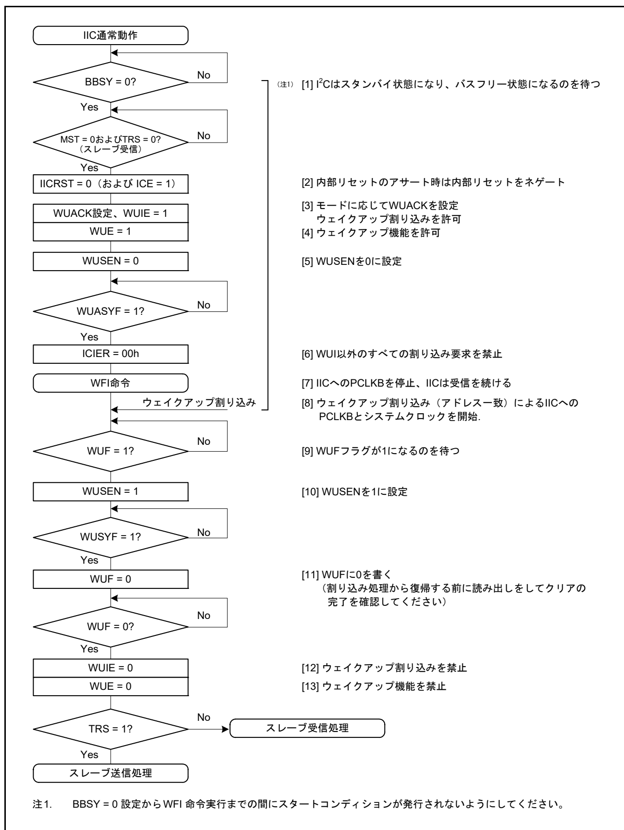
図 30.30 ノーマルウェイクアップモード1の動作例（スレープアドレス一致時のウェイクアップ割り込みによるウェイクアップの場合）
