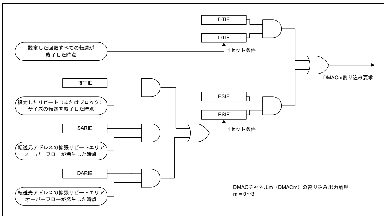
図 17.13 割り込み出力 (DMAC0 ~ DMAC3) の概略論理図
