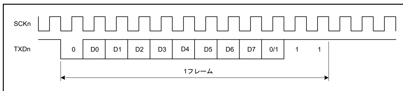
図 29.4 出力クロックと送信データの位相関係 (調歩同期式モード : SEMR.CHR = 0、PE = 1、MP = 0、STOP = 1)
