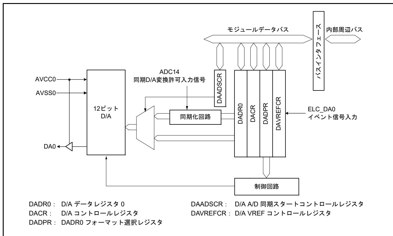
図 35.1 DAC12のブロック図
