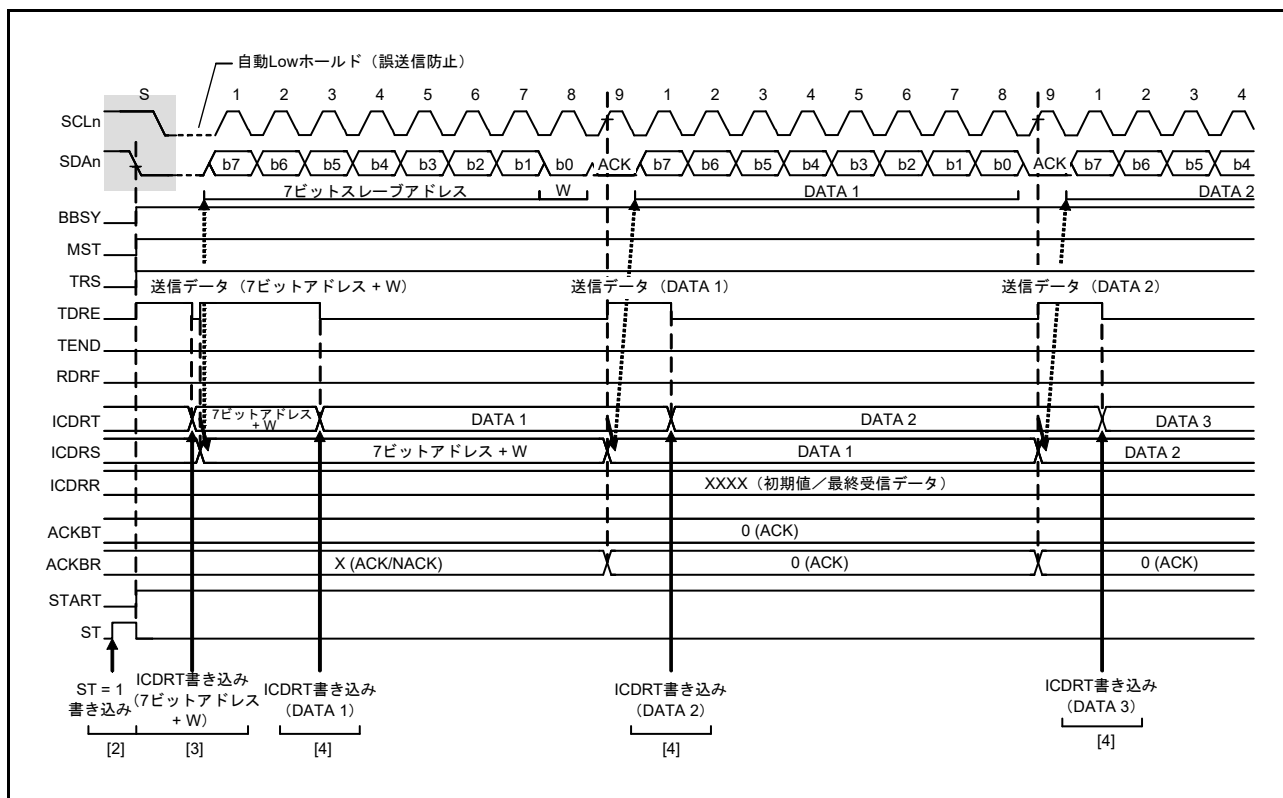
図 30.7 マスタ送信の動作タイミング (1) (7 ビットアドレスフォーマット)
