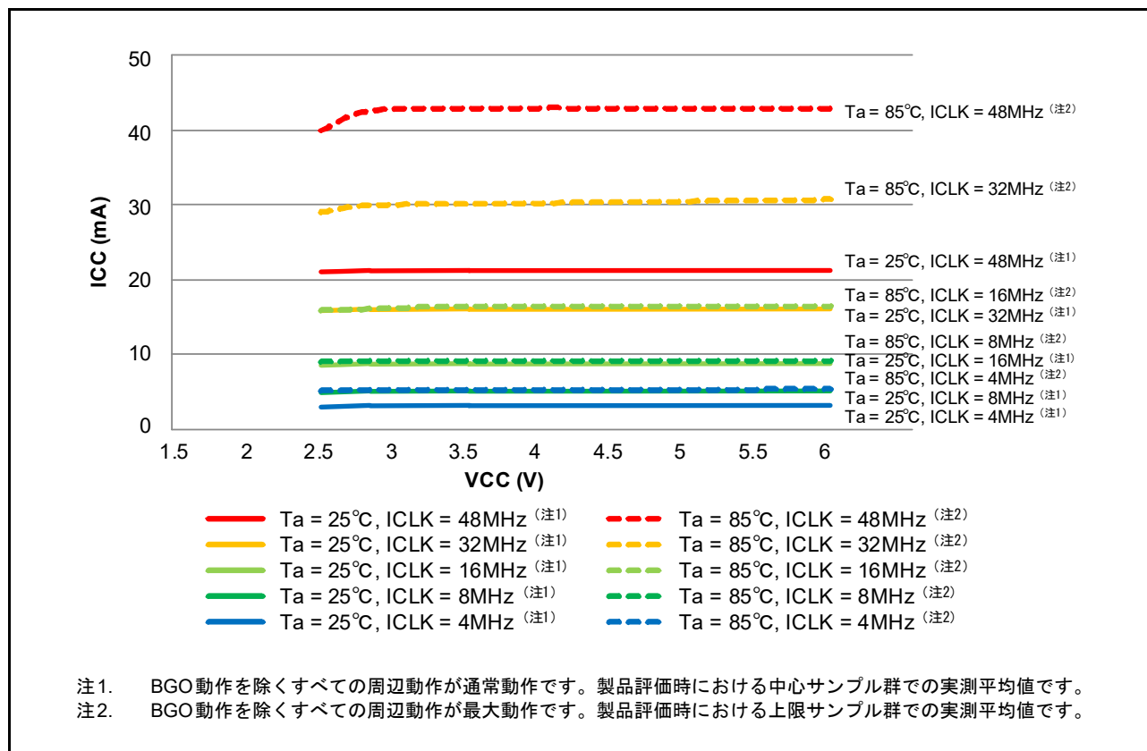
図 48.14 High-speed モードにおける電圧依存性 (参考データ)
