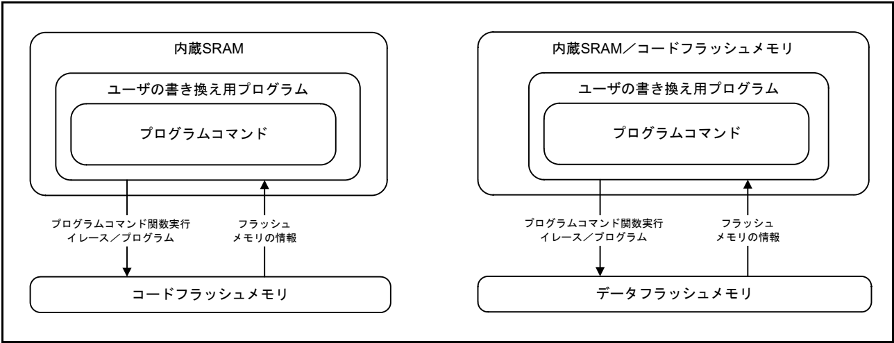
図 43.12 セルフプログラミングの概念
