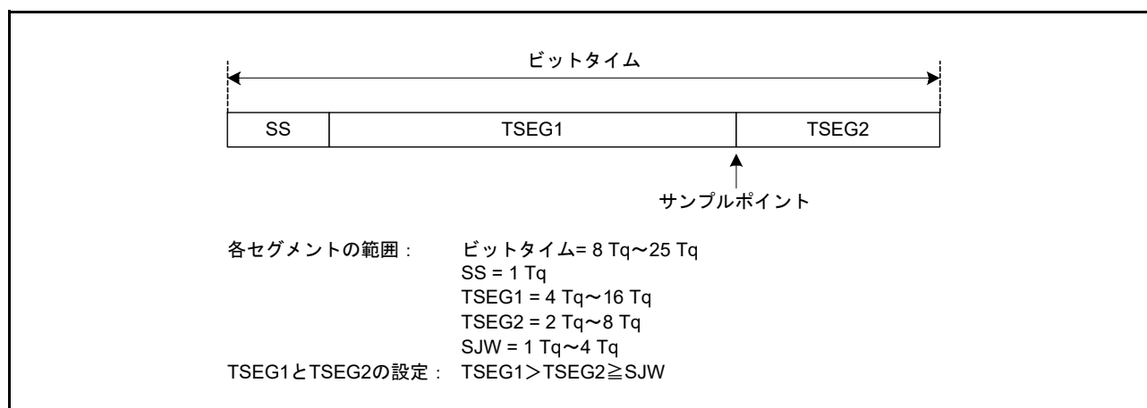
図 31.12 ビットタイミング
