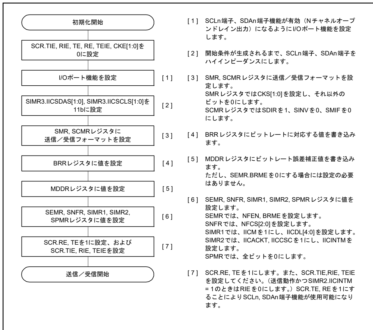
図 29.63 SCI の初期化フローチャート例 (簡易 IIC モード)
