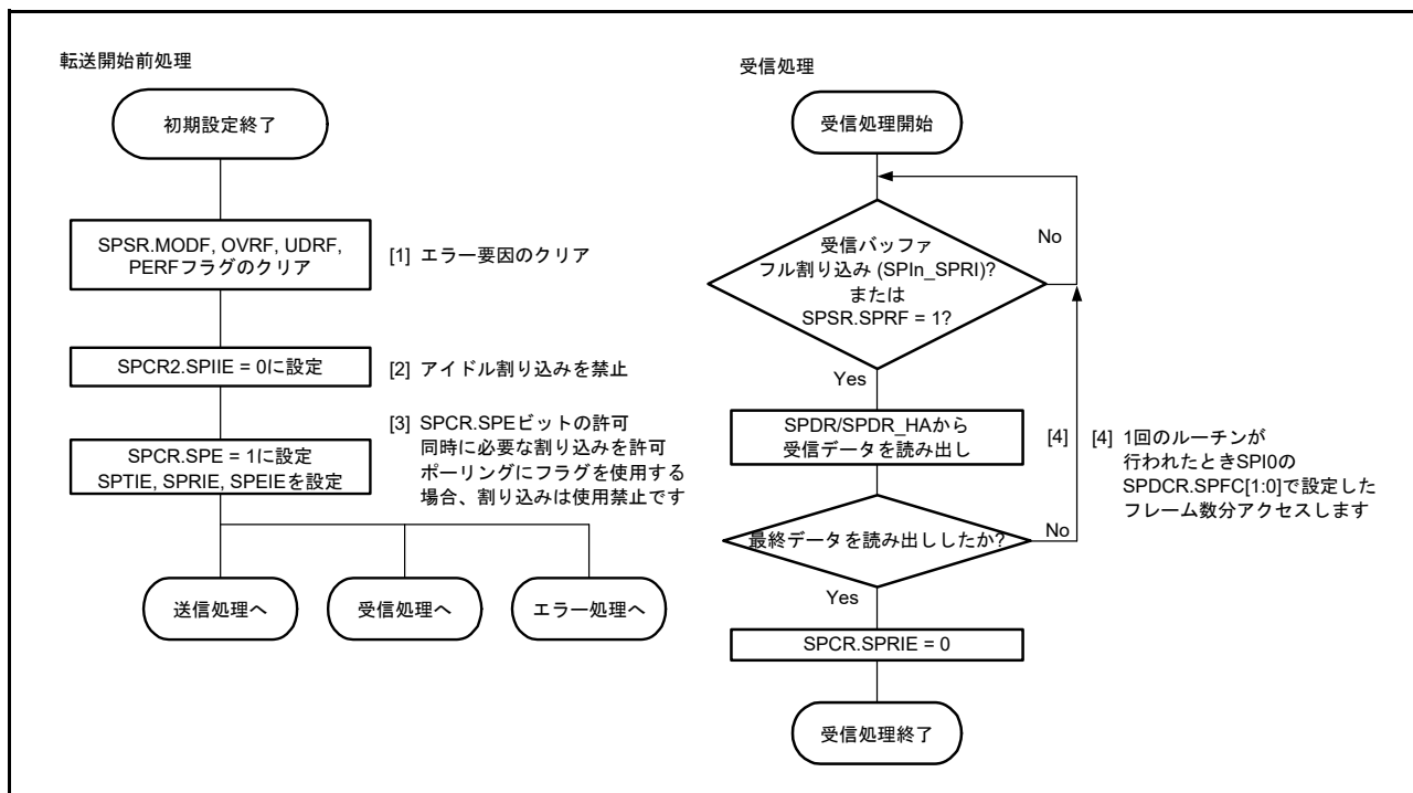
図 32.49 スleepモードでの受信フロー
