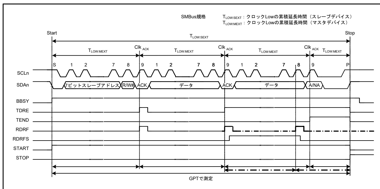
図 30.50 SMBus タイムアウト測定
