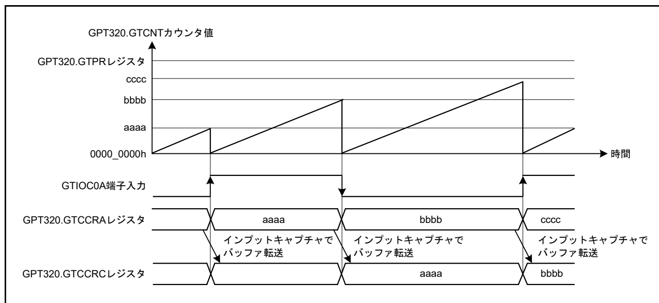
図 23.26 GTCCRA、GTCCRB レジスタのバッファ動作例 (GTIOC0A 端子入力の両エッジでインプットキャプチャ、のこぎり波でアップカウント、GTIOC0A 端子入力の両エッジで GTCNT カウンタクリアの場合)
