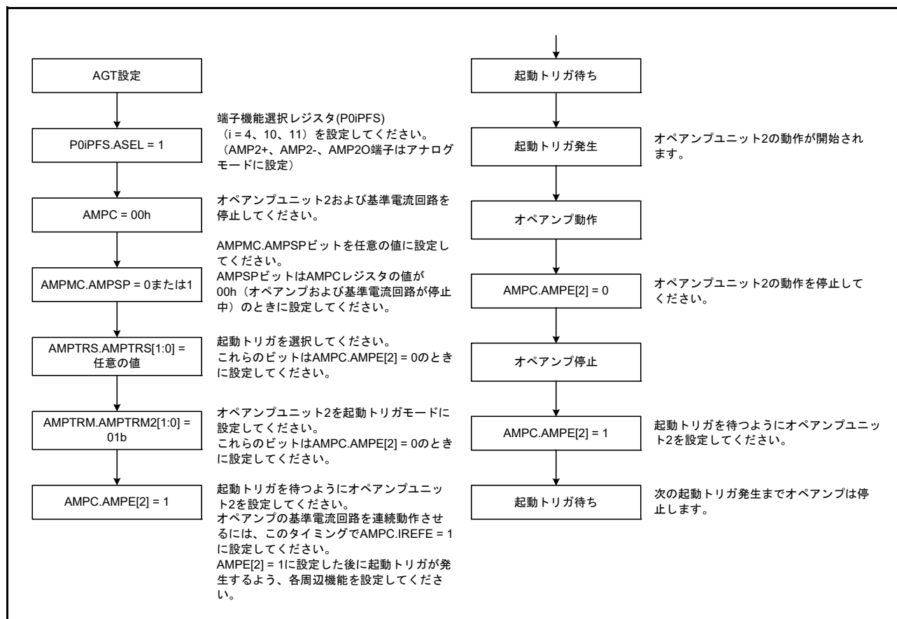
図 37.8 起動トリガモードでの OPAMP 起動および停止手順
