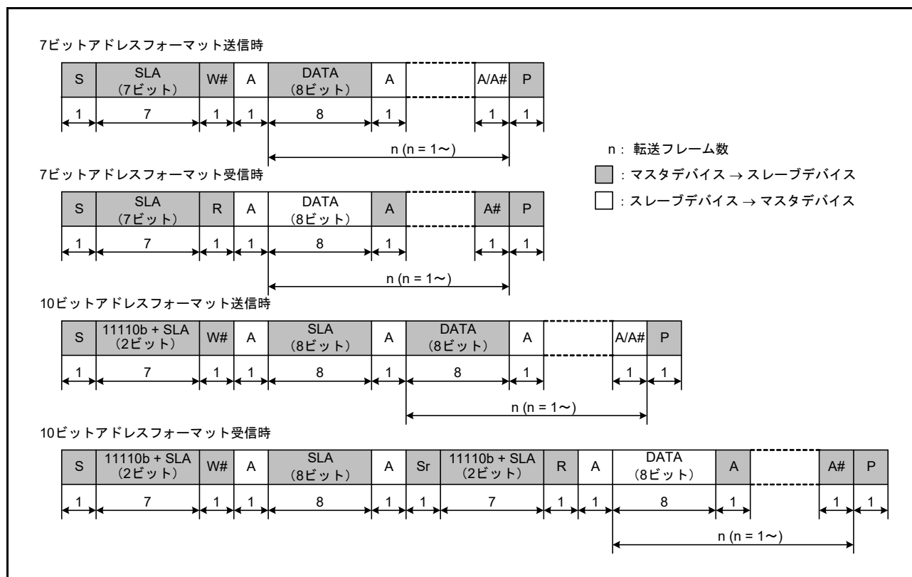
図 29.58 I 2 C バスフォーマット
