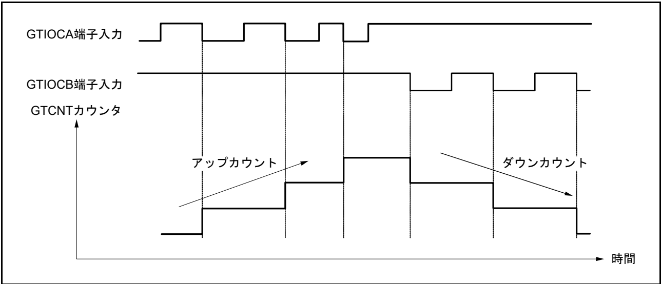
図 23.71 位相計数モード3 動作例 (A)
