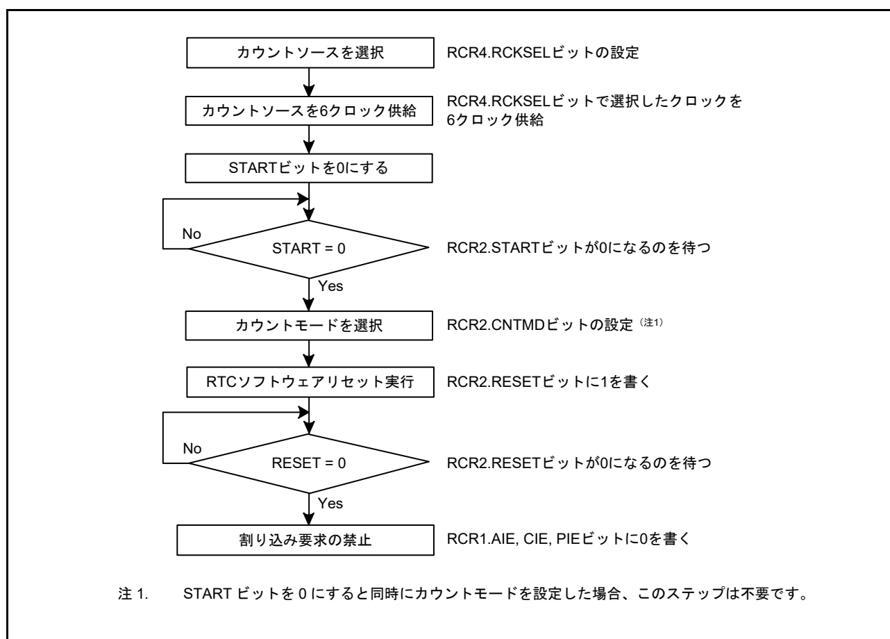
図 25.14 初期化手順
