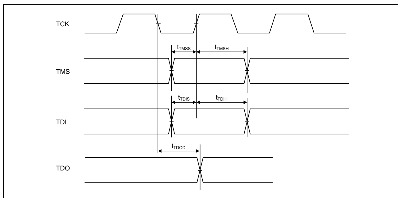
図 48.75 JTAG 入出力タイミング
