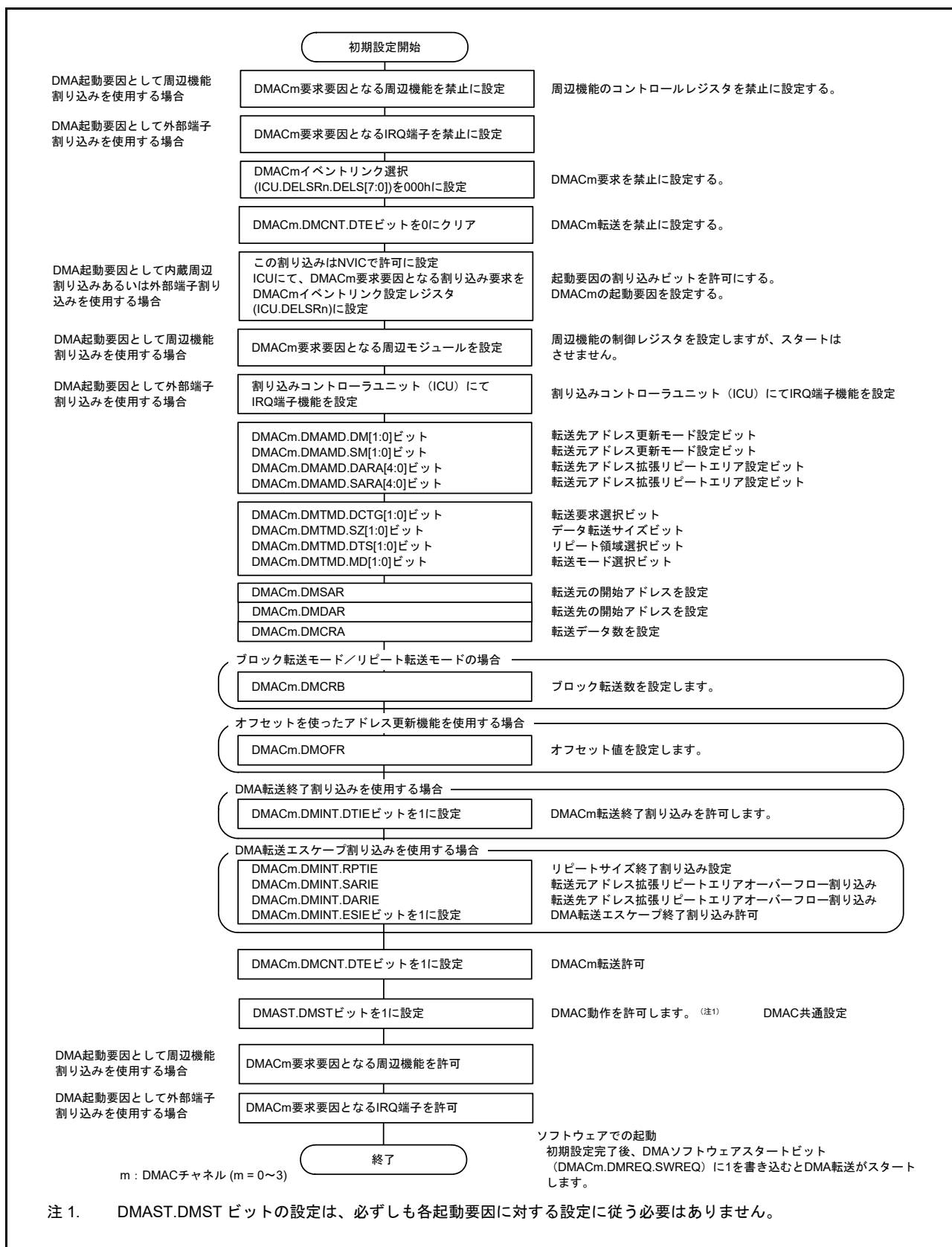
図 17.12 レジスタの設定手順
