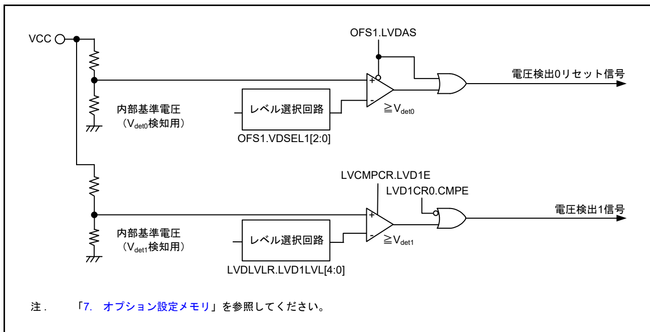
図 8.1 電圧検出 0、1 回路のブロック図
