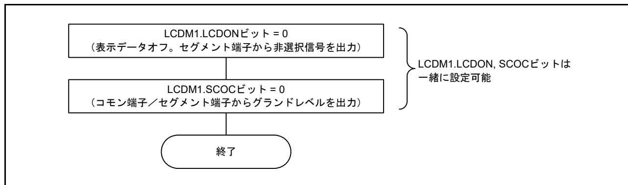
図 44.6 通常液晶波形 (A または B) 表示での動作停止手順
