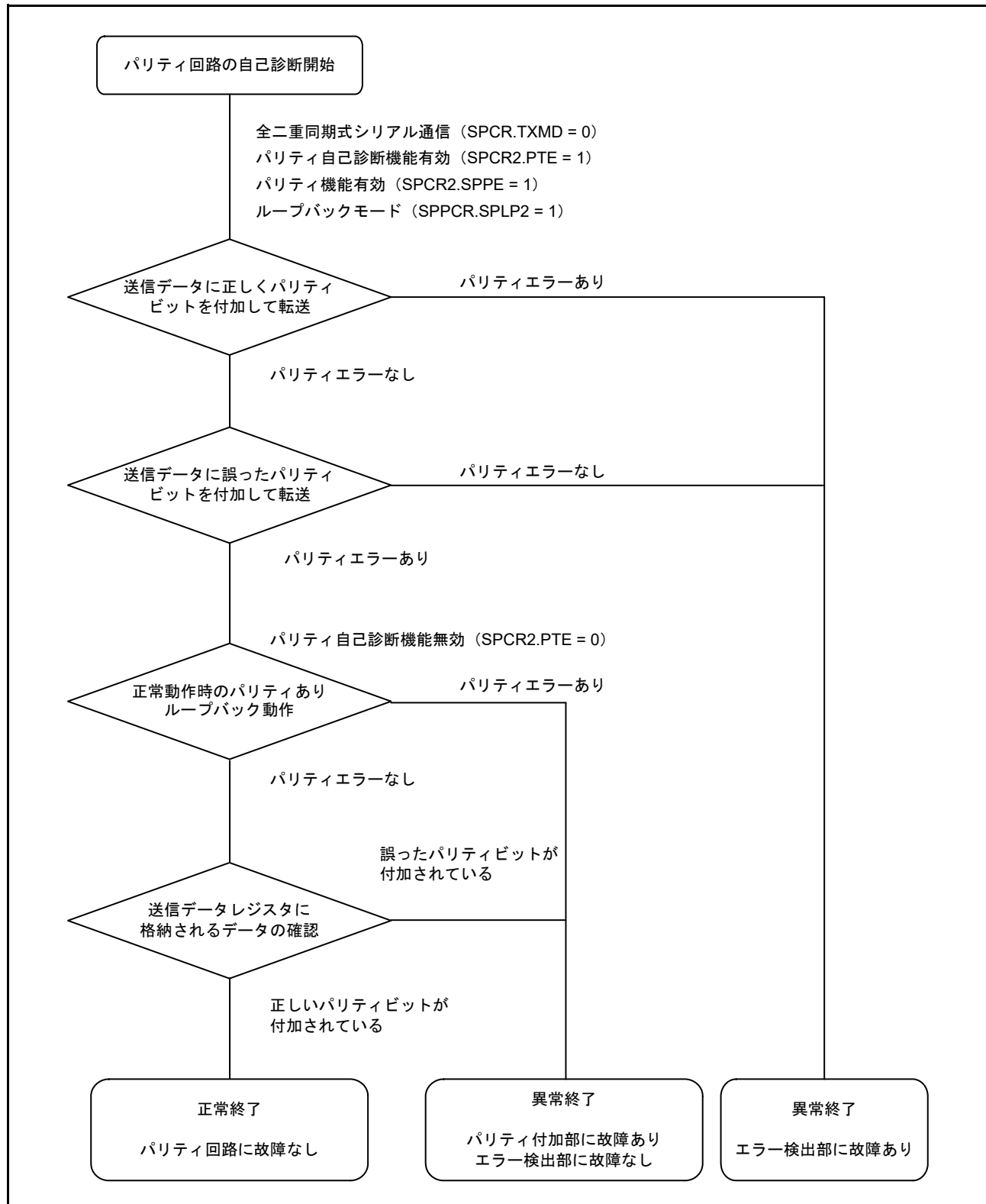
図 32.60 パリティ回路の自己診断フロー
