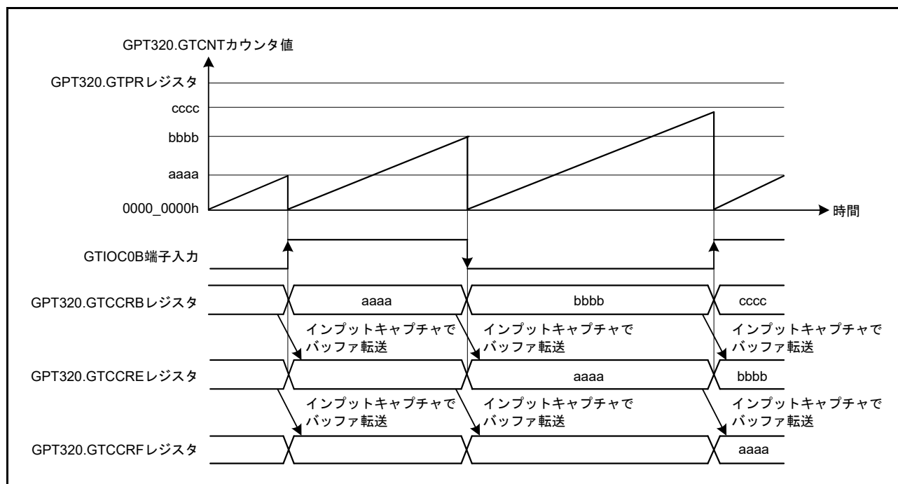
図 23.27 GTCCRA、GTCCRB レジスタのダブルバッファ動作例 (GTIOC0B 端子入力の両エッジでインプットキャプチャ、のこぎり波でアップカウント、GTIOC0B 端子入力の両エッジで GTCNT カウンタクリアの場合)
