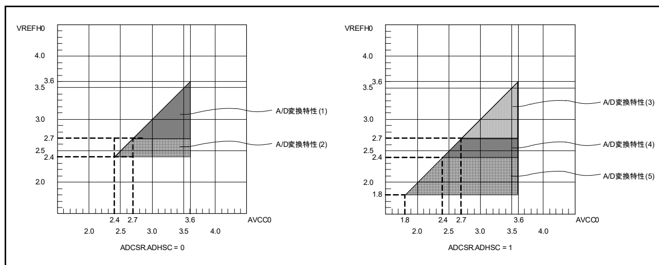
図 48.62 AVCC0 ~ VREFH0 電圧範囲
