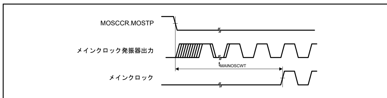
図 48.25 メインクロック発振開始タイミング
