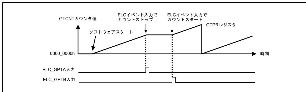
図 23.49 ハードウェア要因によるカウンストップ動作例 (ソフトウェアによるスタート、ELC_GPTA 入力でのストップ、ELC_GPTB 入力での再スタートの場合)
