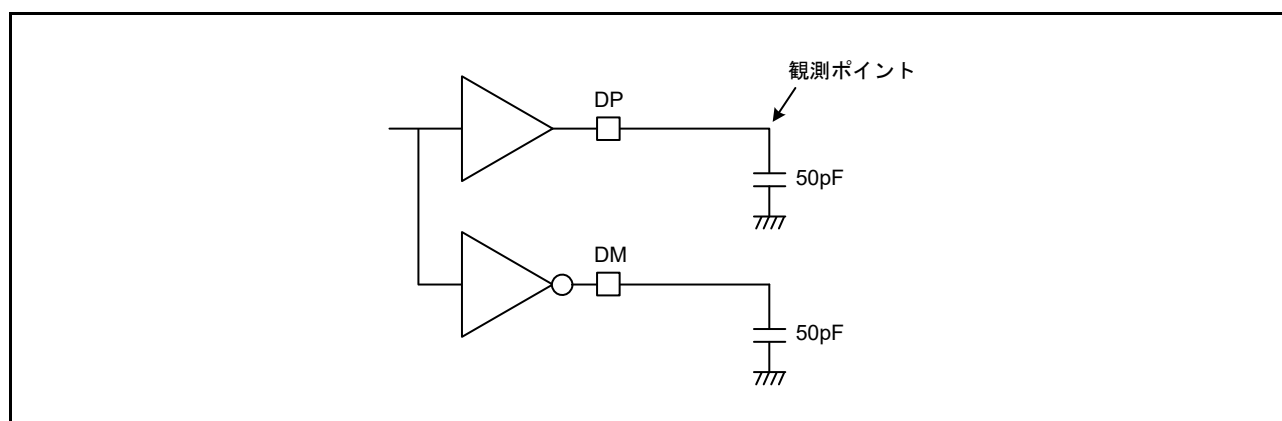
図 48.60 フルスピード (FS) 接続の測定回路
