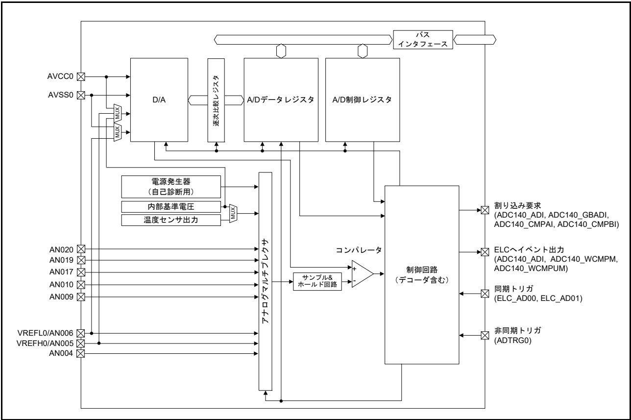
図 34.1 ADC14 のブロック図
