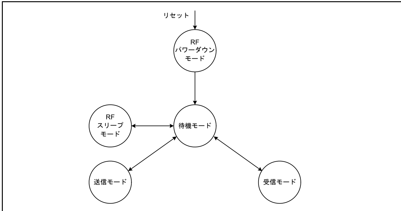
図 46.2 BLE の状態遷移図
