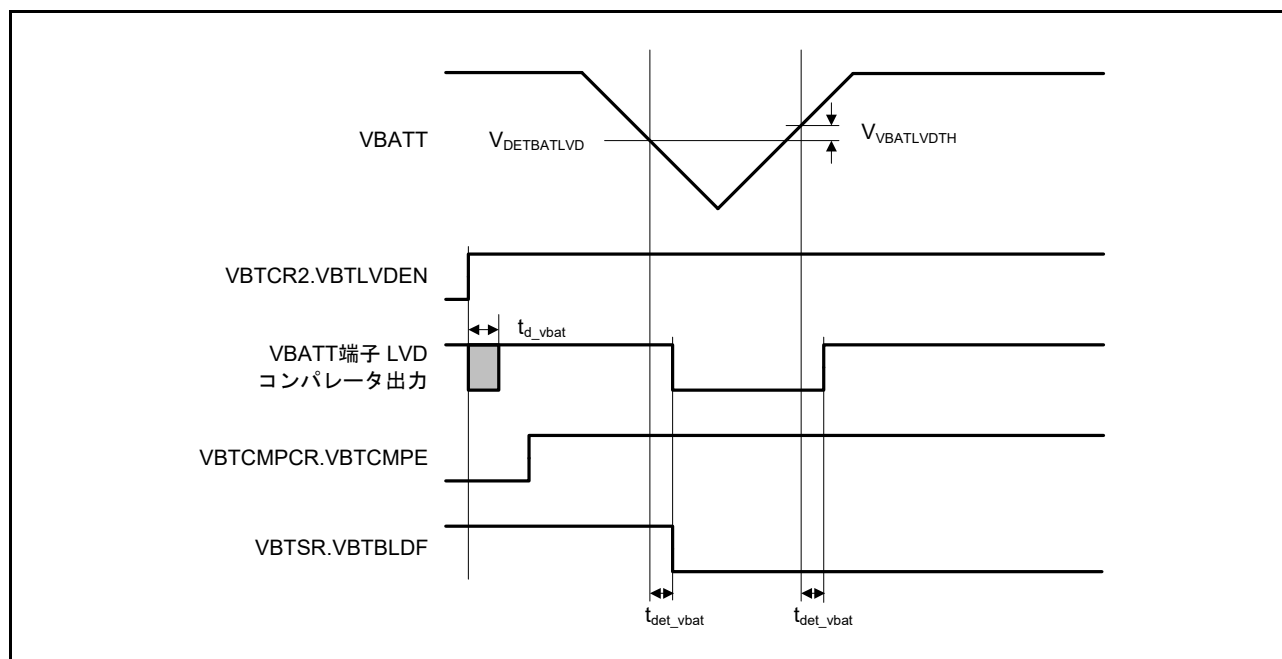
図 48.73 \text{VBATT} 端子電圧検出回路タイミング
