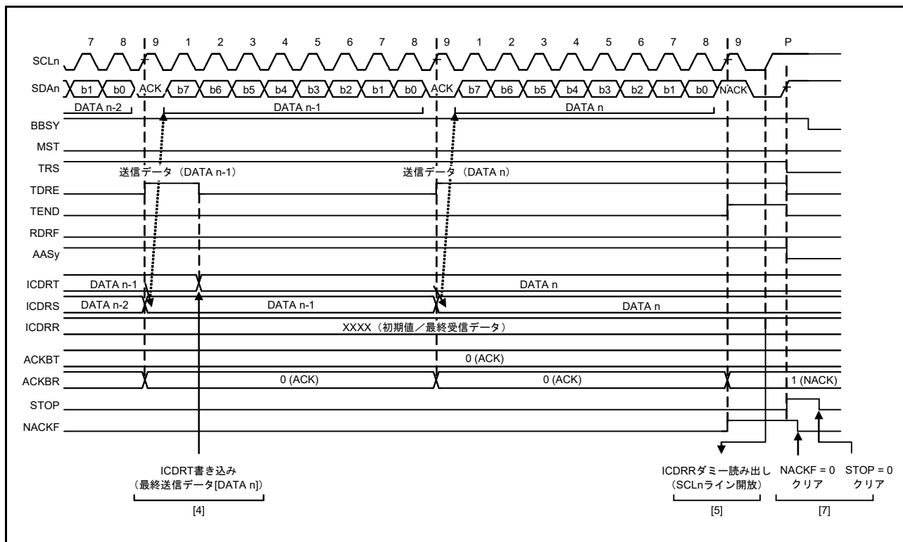
図 30.17 スレーブ送信の動作タイミング (2)
