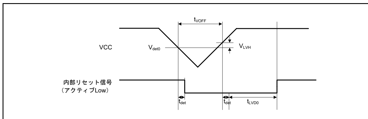
図 48.69 電圧検出回路タイミング ( V_{det0} )
