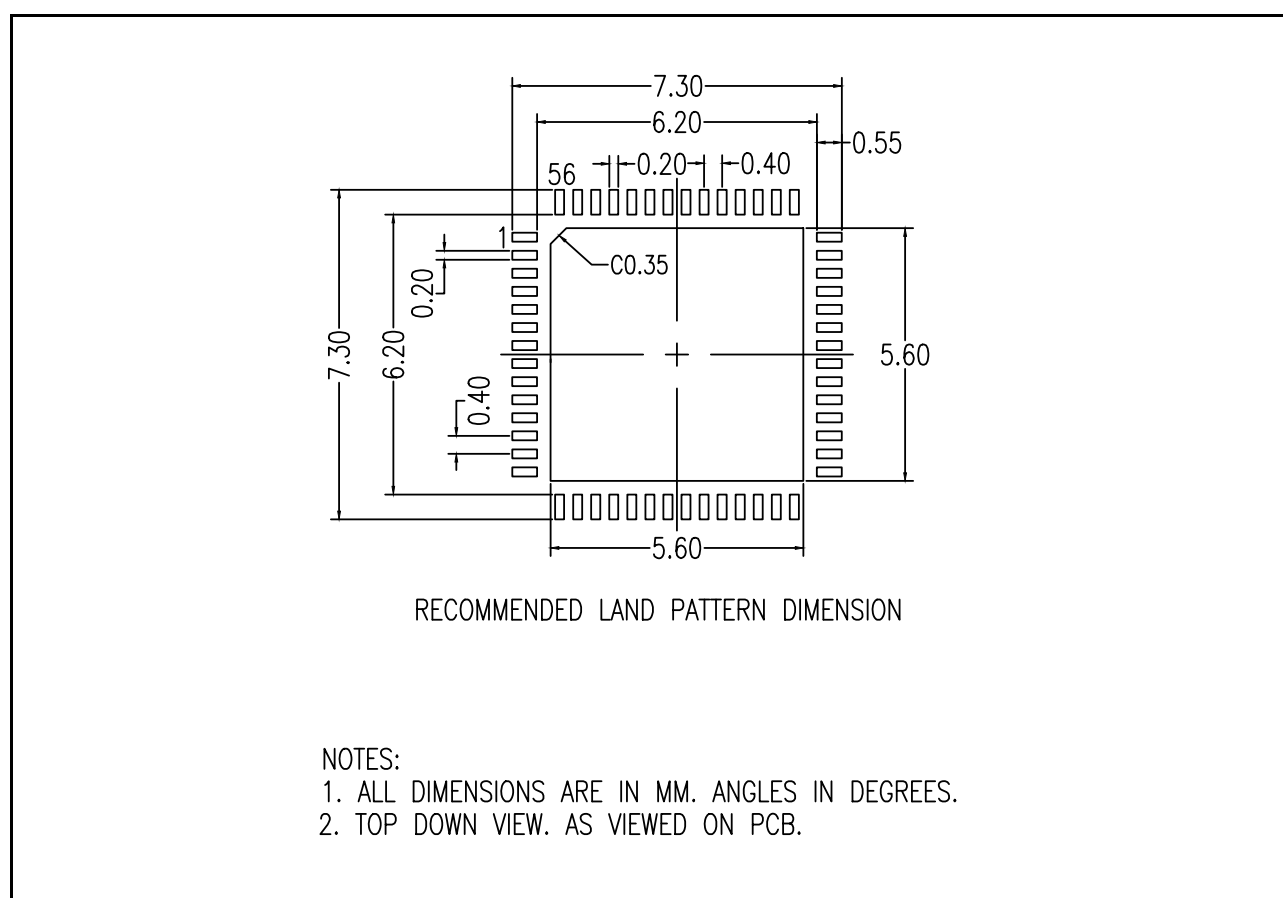
図 2.2 ランドボタン
