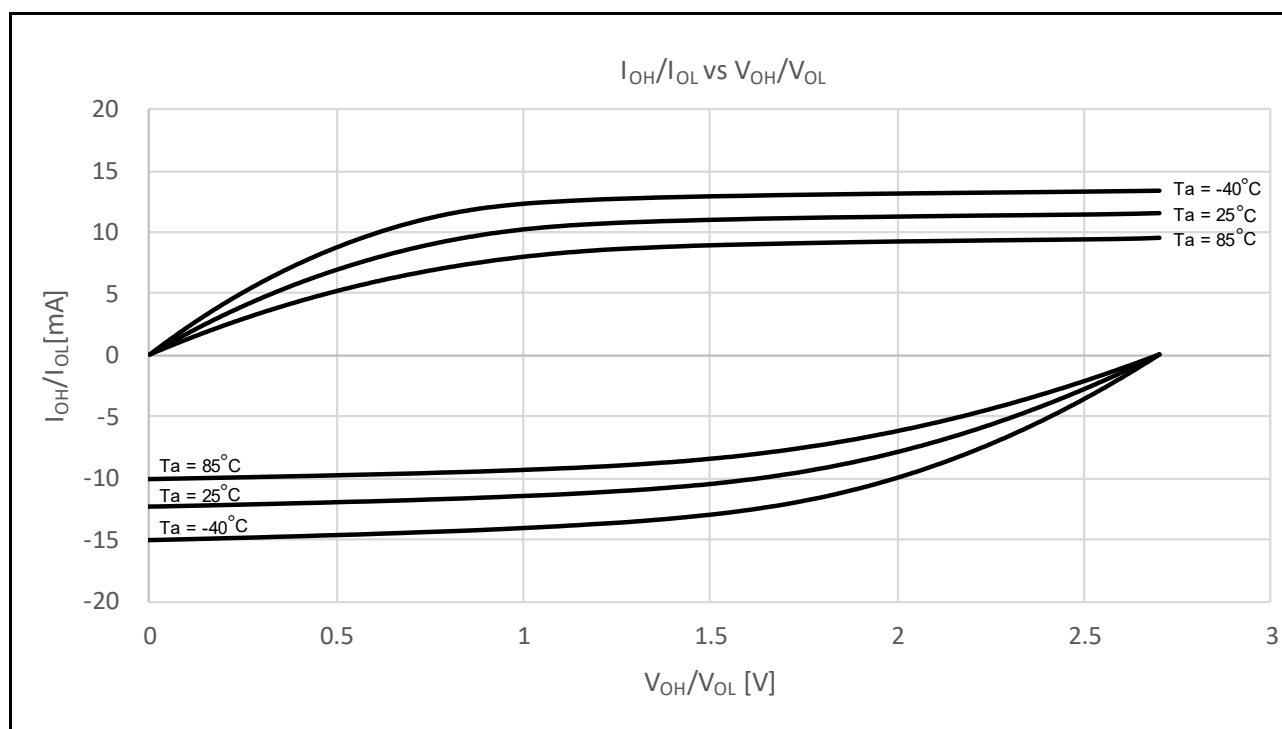
図 48.4 低駆動出力選択時の V_{CC} = 2.7\text{V} での V_{OH}/V_{OL} および I_{OH}/I_{OL} 温度特性 (参考データ)
