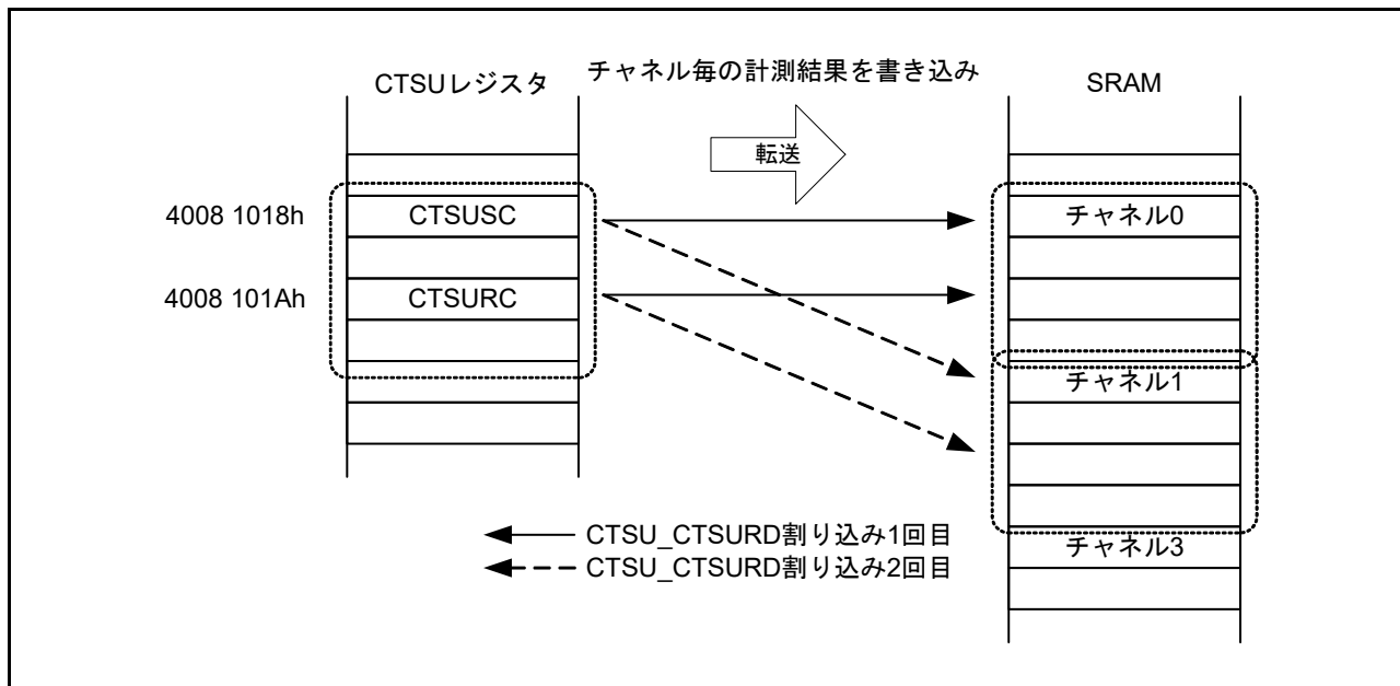
図 40.20 CTSU_CTSURD 割り込みを用いた DTC 転送動作例
