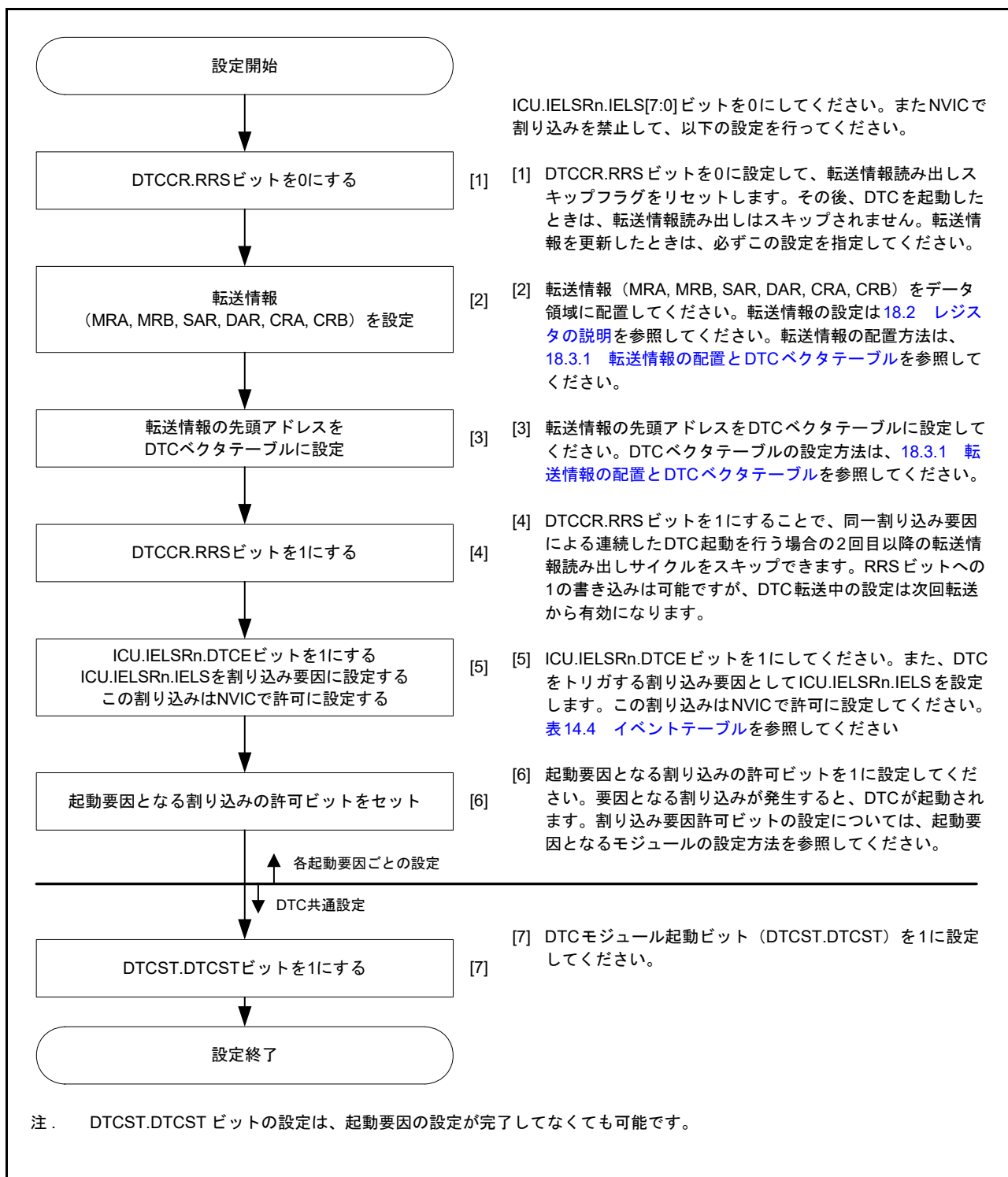
図 18.13 DTC の設定手順
