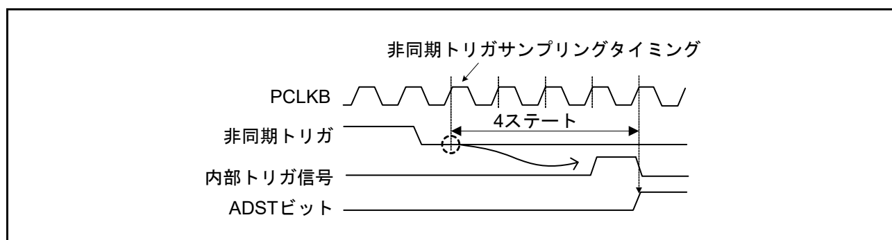
図 34.29 非同期トリガ入力タイミング
