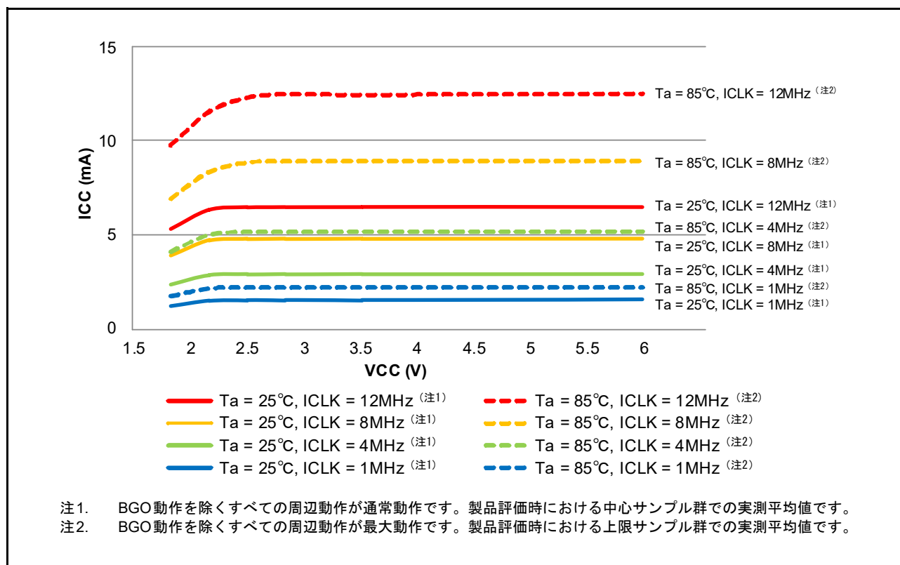
図 48.15 Middle-speed モードにおける電圧依存性 (参考データ)
