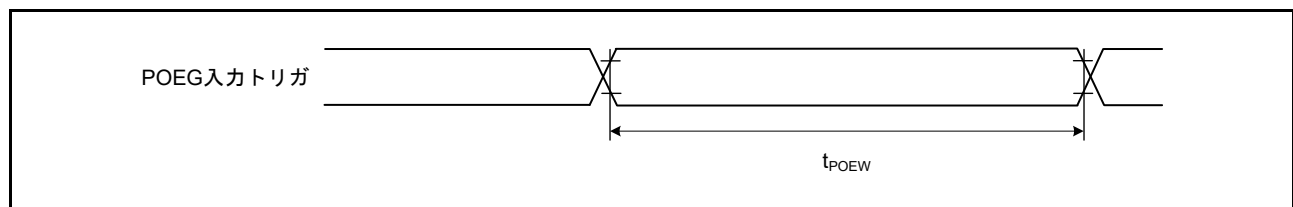
図 48.36 POEG 入力トリガタイミング
