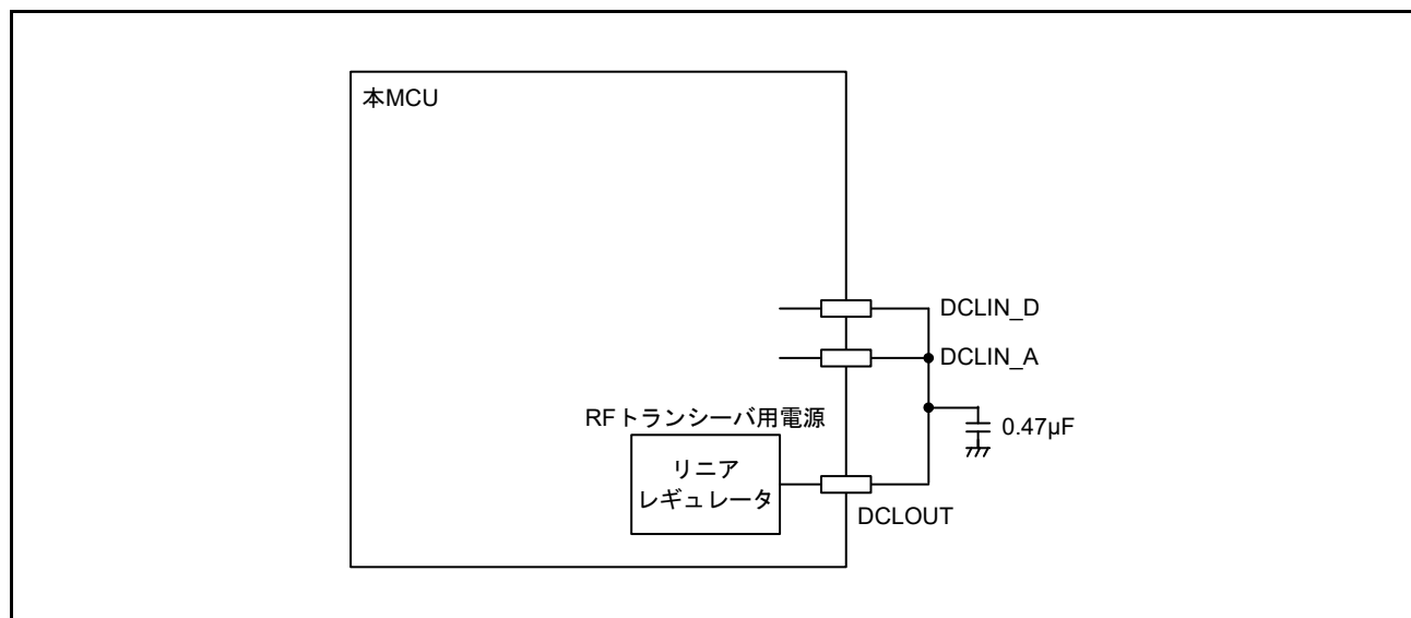
図 46.4 リニアレギュレータ選択時の BLE 外部接続回路例
