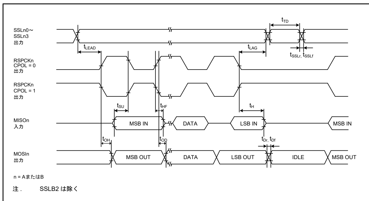
図 48.53 SPI タイミング (マスタ、CPHA = 1) (ビットレート : PCLKA を 2 分周に設定)
