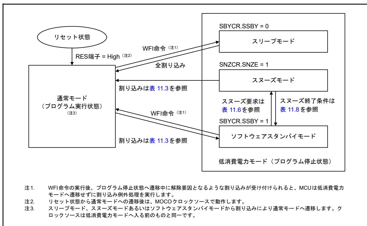
図 11.1 モード遷移
