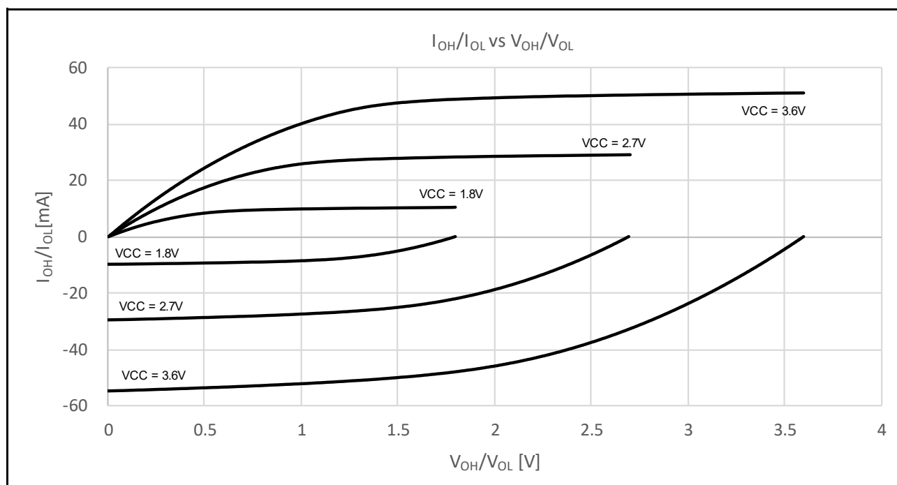
図 48.6 中駆動出力選択時の T_a = 25^\circ\text{C} での V_{OH}/V_{OL} および I_{OH}/I_{OL} 電圧特性 (参考データ)
