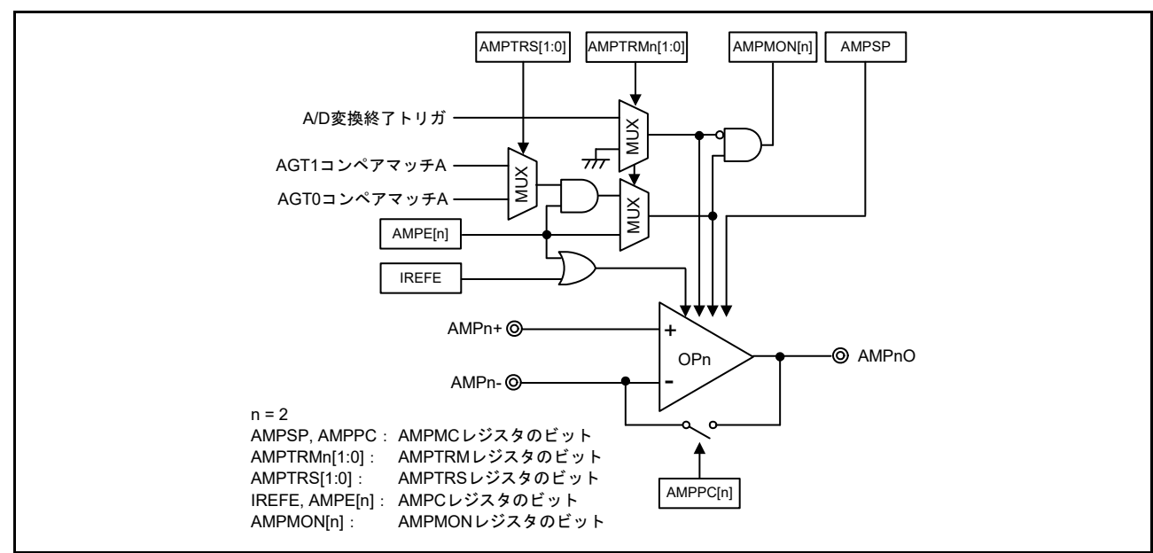
図 37.1 オペアンプのブロック図
