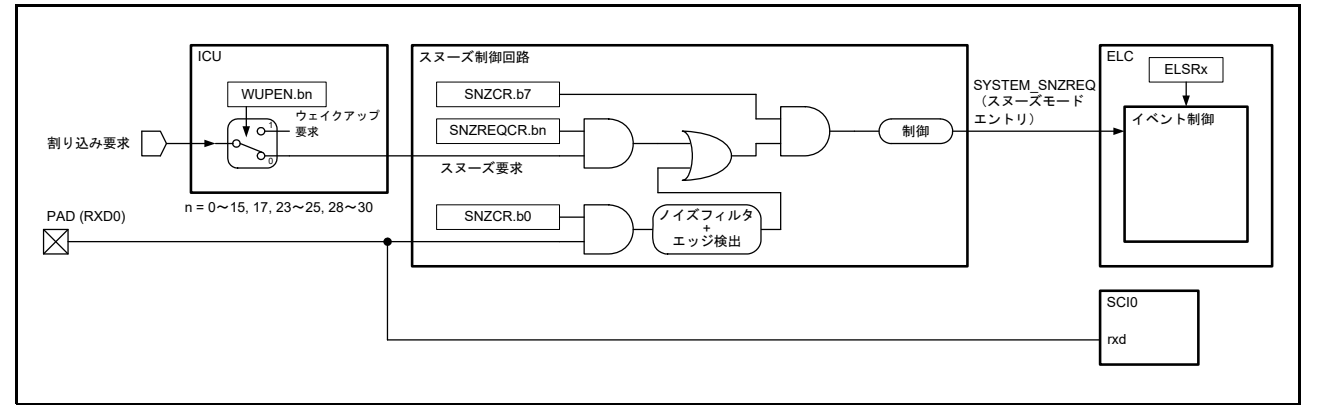
図 11.8 スヌーズモードエントリの構成
