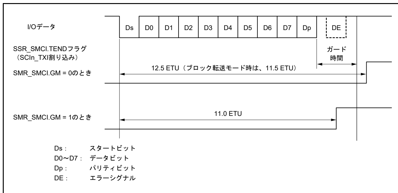
図 29.53 送信中の SSR.TEND フラグの発生タイミング
