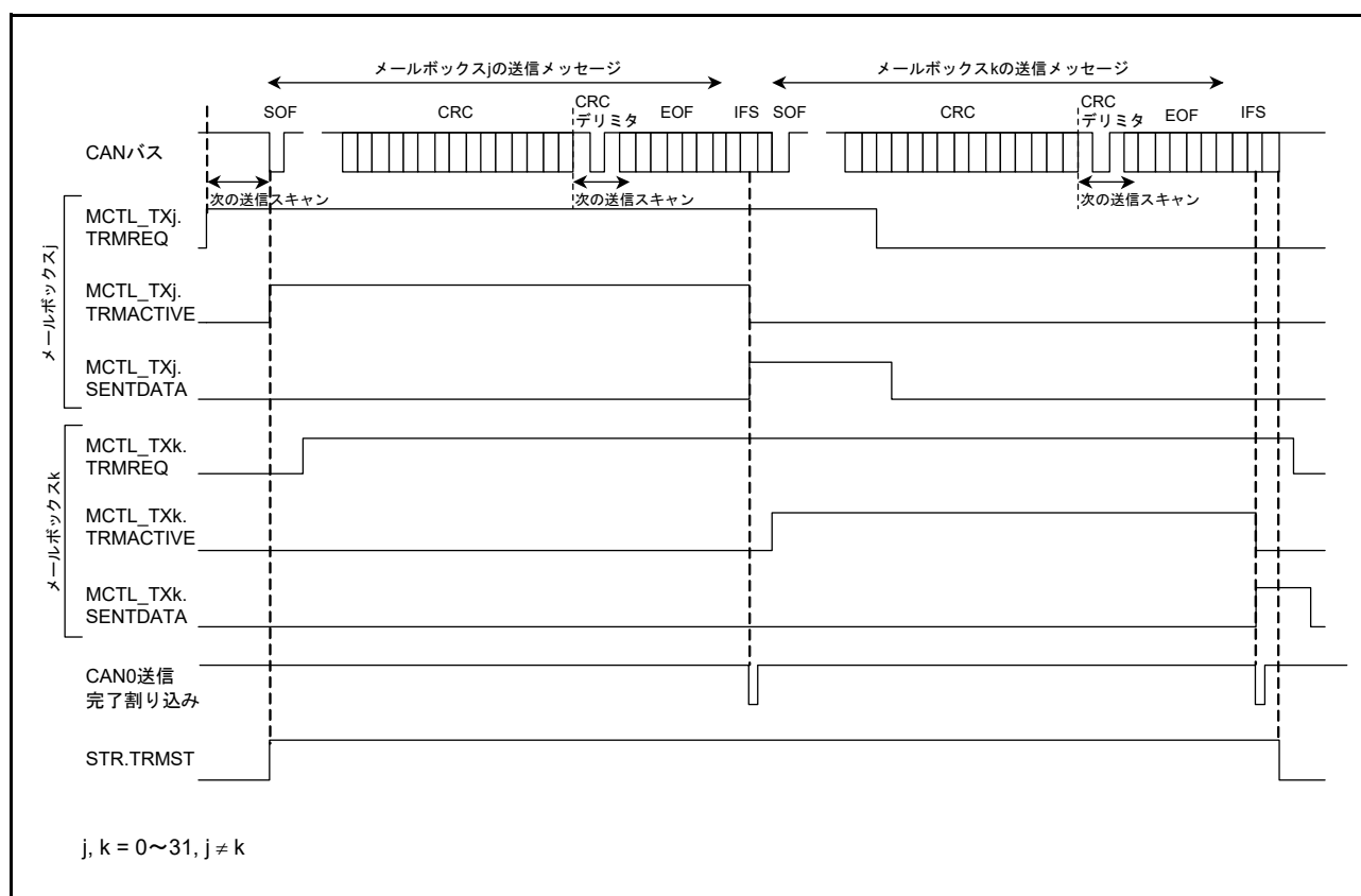
図 31.20 データフレーム送信時の動作例
