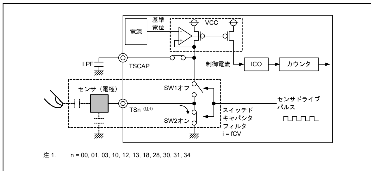
図 40.6 放電動作
