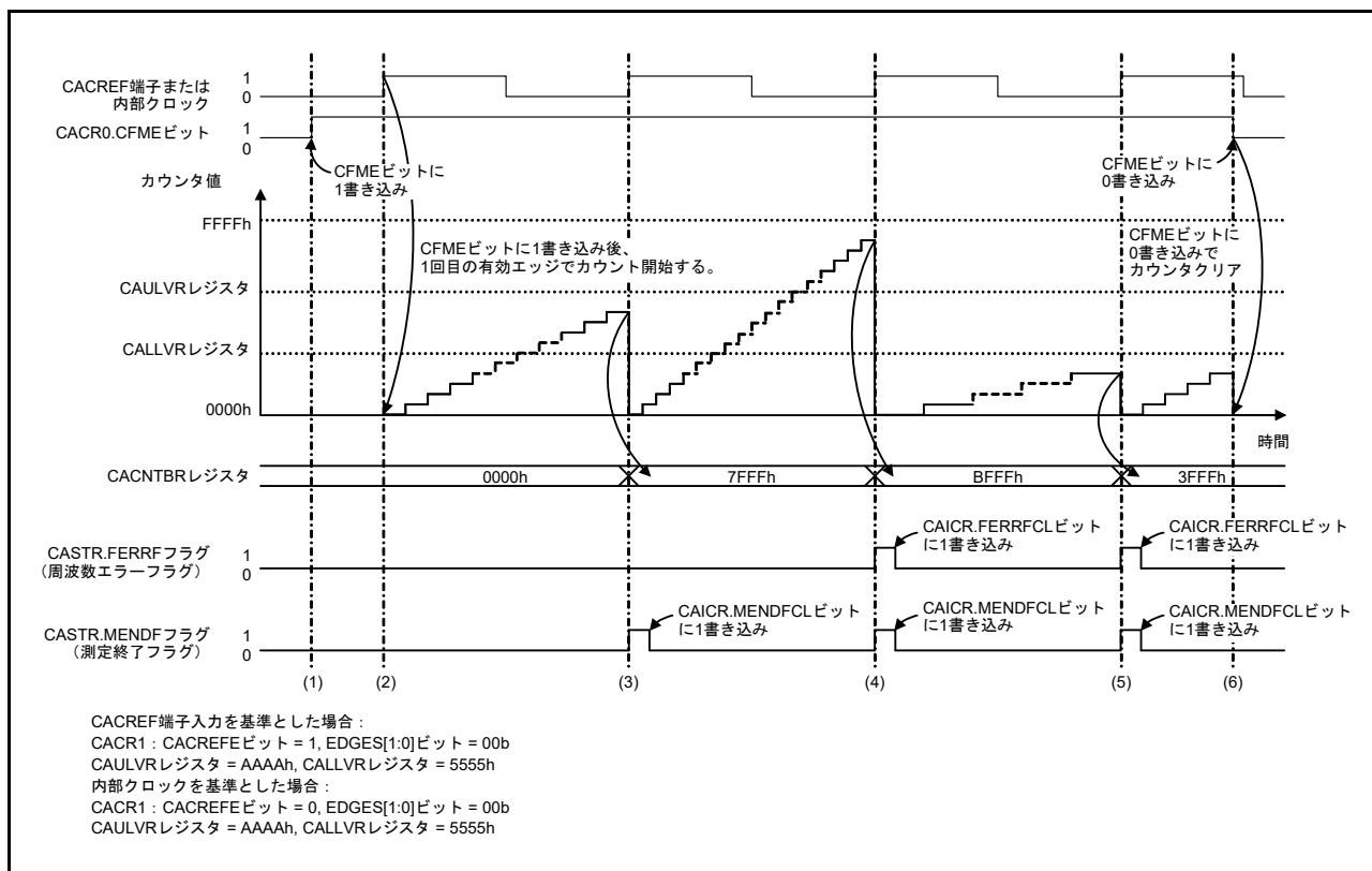
図 10.2 CAC の動作例
