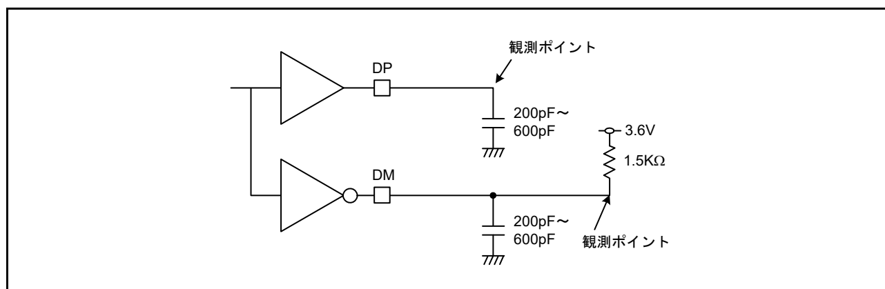
図 48.61 ロースピード (LS) 接続の測定回路
