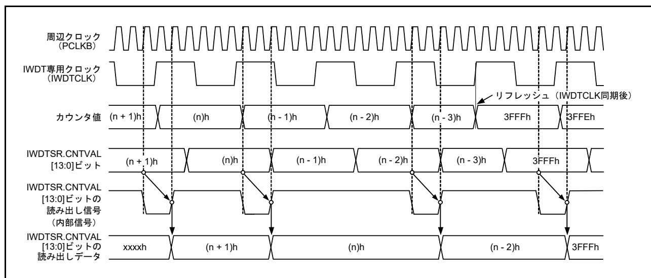
図 27.5 IWDT カウンタ値の読み出し処理 (OFS0.IWDTCKS[3:0] = 0000b、OFS0.IWDTTOS[1:0] = 11b の場合)
