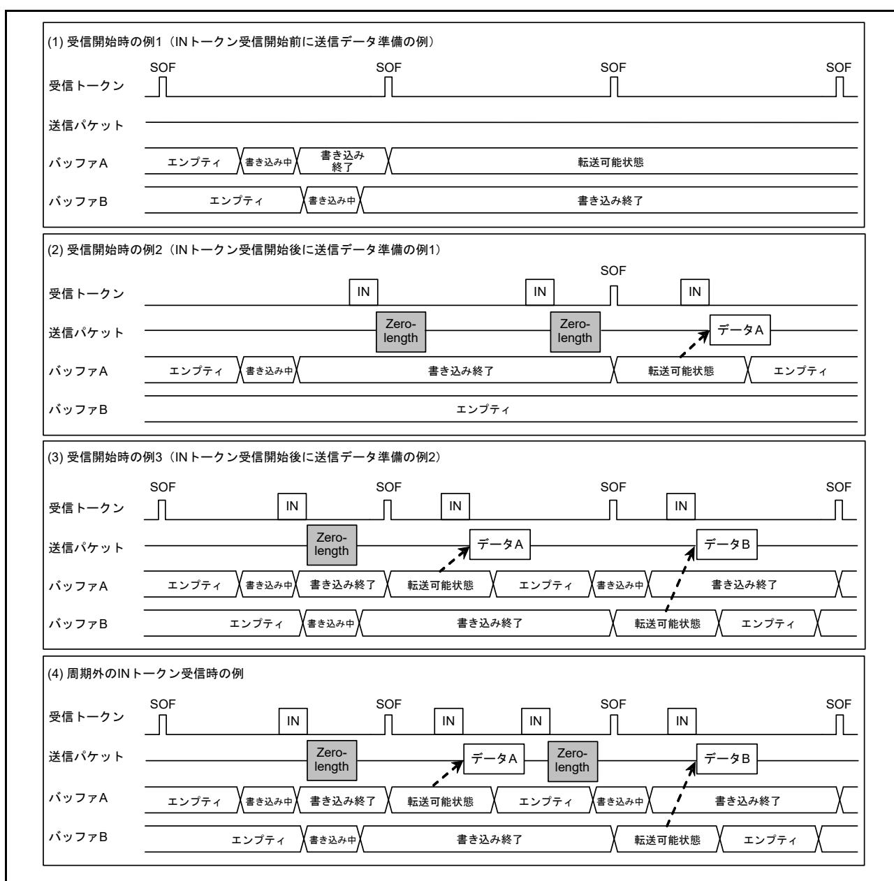
図 28.17 データセットアップ動作例
