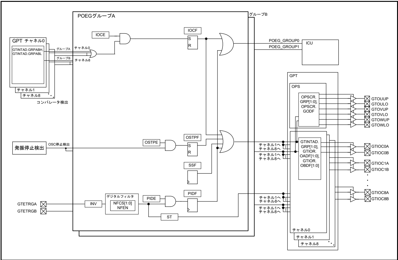
図 22.1 POEG のブロック図
