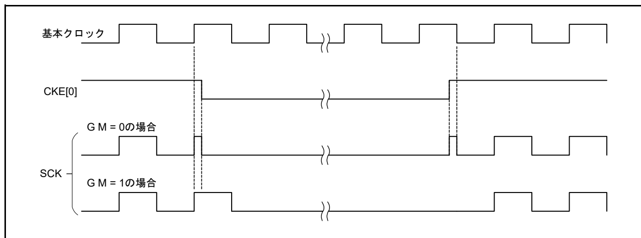
図 29.57 クロック出力制御
