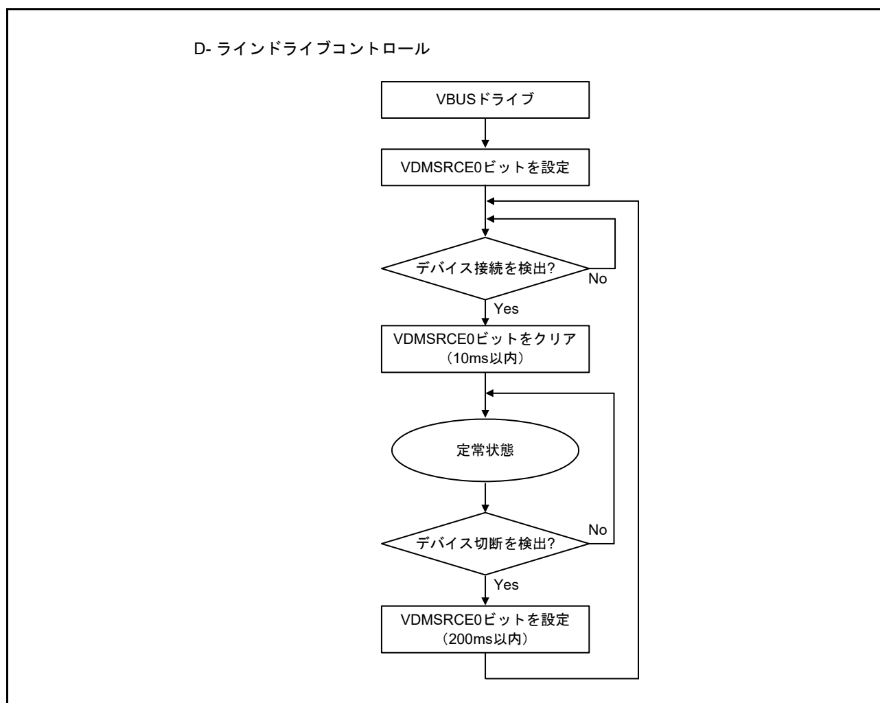
図 28.22 チャージングダウンストリームポートとして動作する場合の処理フロー（ステップ a ～ b）
