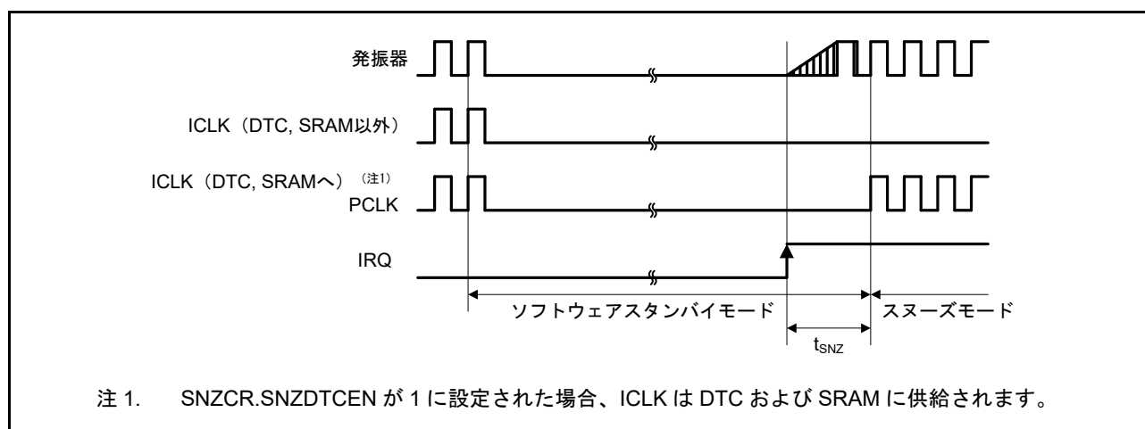
図 48.32 ソフトウェアスタンバイモードからスリープモードへの復帰タイミング
