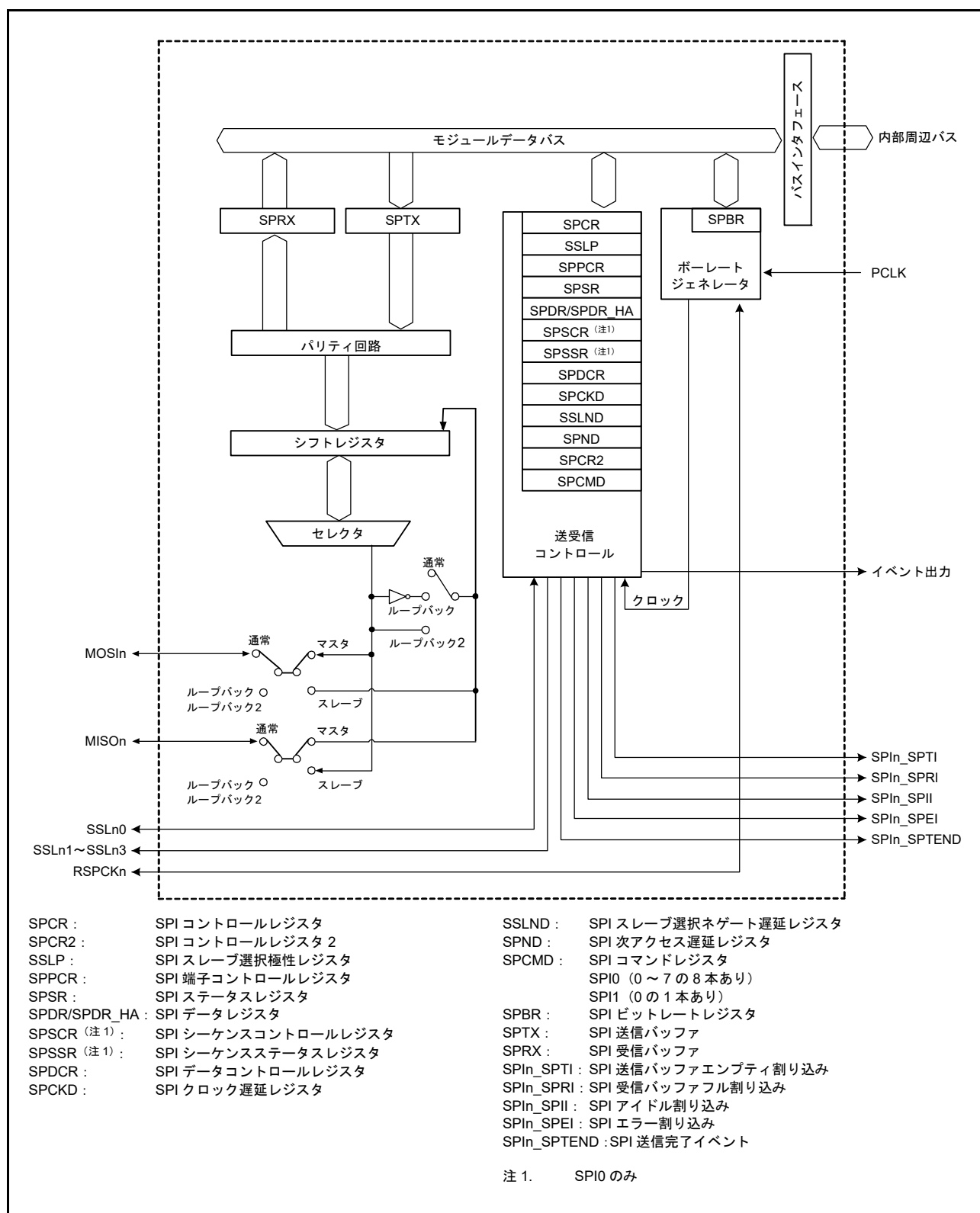
図 32.1 SPI のブロック図
