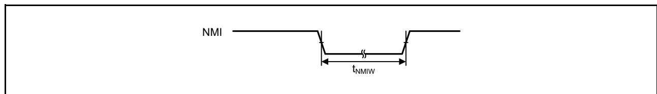
図 48.33 NMI 割り込み入力タイミング
