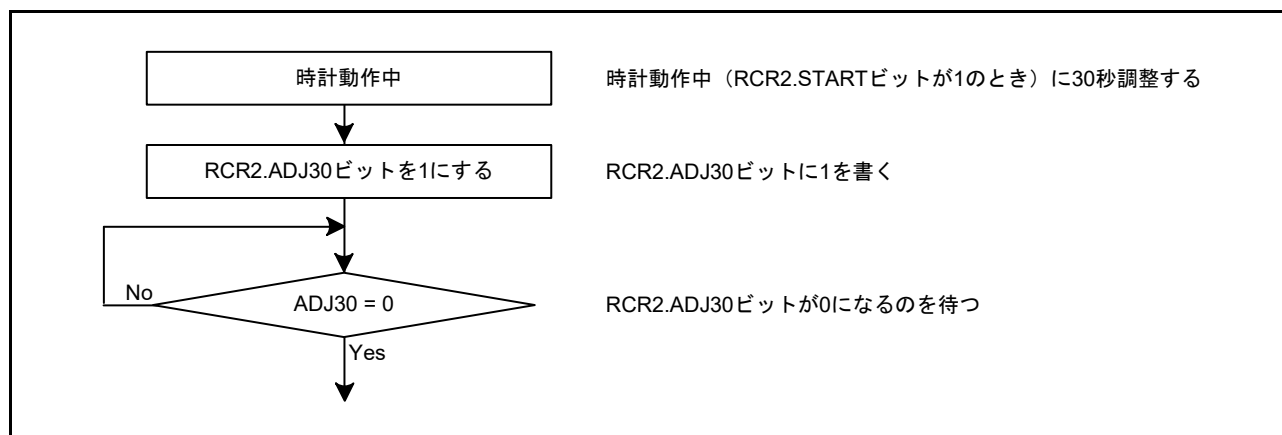
図 25.5 30 秒調整
