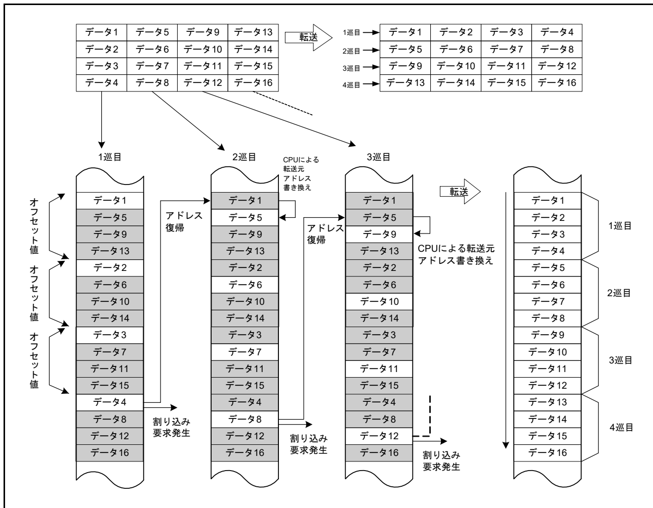
図 17.8 リピート転送モード+オフセット加算によるXY変換動作
