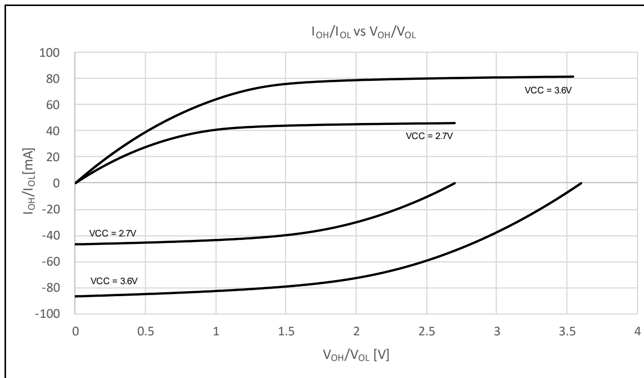
図 48.10 中駆動出力選択時の T_a = 25^\circ\text{C} での V_{OH}/V_{OL} および I_{OH}/I_{OL} 電圧特性 (参考データ)
