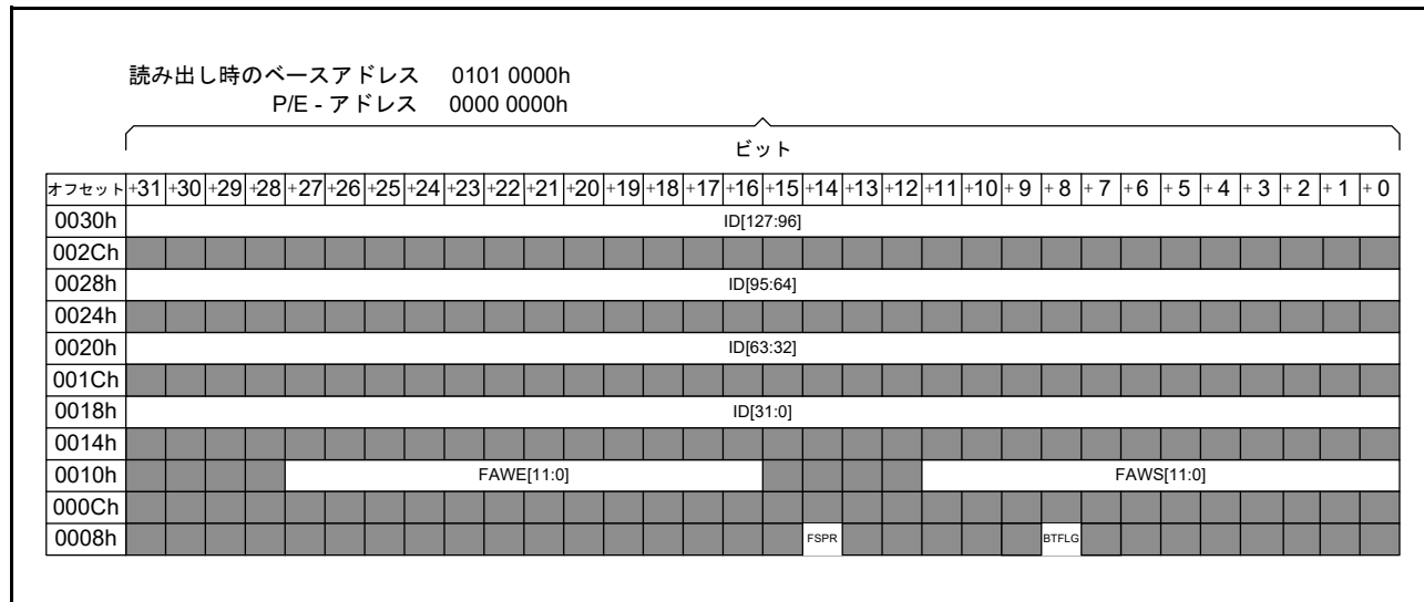
図 43.6 構成領域ビットマップ
