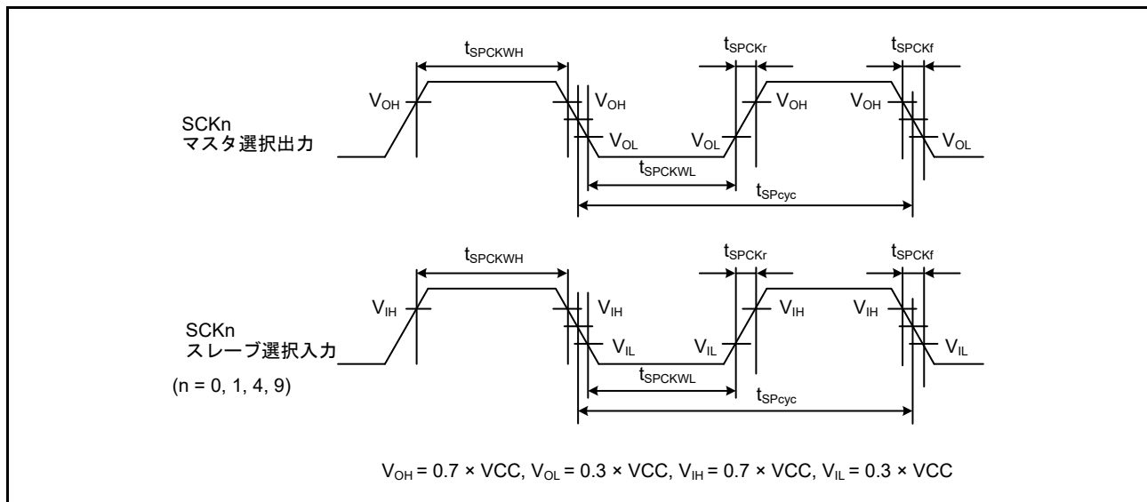
図 48.43 SCI 簡易 SPI モードクロックタイミング
