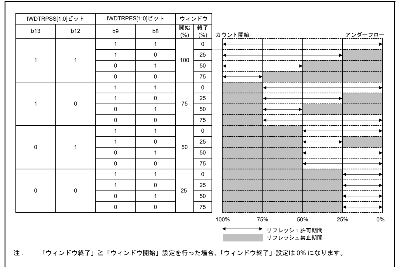
図 27.2 IWDTRPSS[1:0] および IWDTRPES[1:0] ビットとリフレッシュ許可期間
