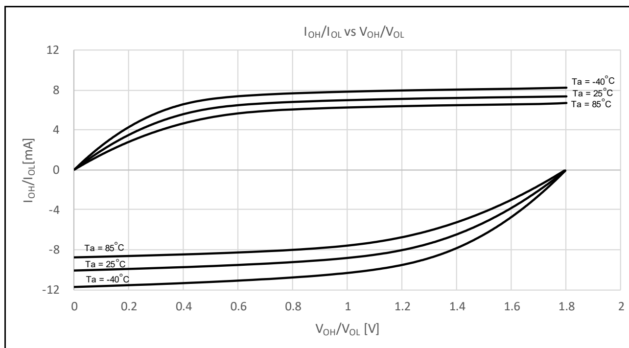
図 48.7 中駆動出力選択時の V_{CC} = 1.8\text{V} での V_{OH}/V_{OL} および I_{OH}/I_{OL} 温度特性 (参考データ)
