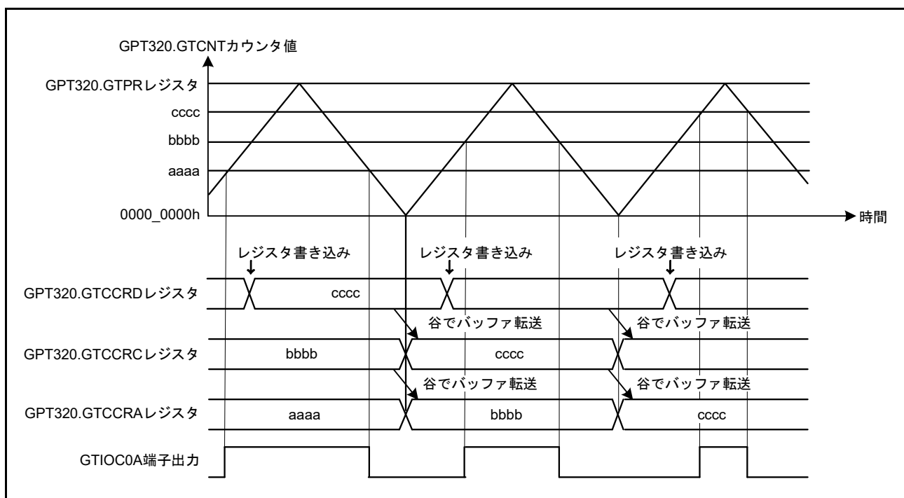
図 23.23 GTCRA、GTCCRB レジスタのダブルバッファ動作例（アウトプットコンペア、三角波、谷でバッファ動作、GTCCRA レジスタのコンペアマッチでトグル出力、周期の終わりで出力保持の場合）
