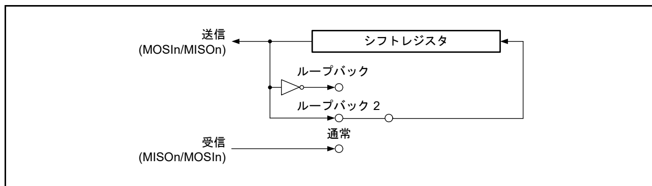
図 32.59 ループバックモード時のシフトレジスタ入出力経路の構成 (マスタモード)
