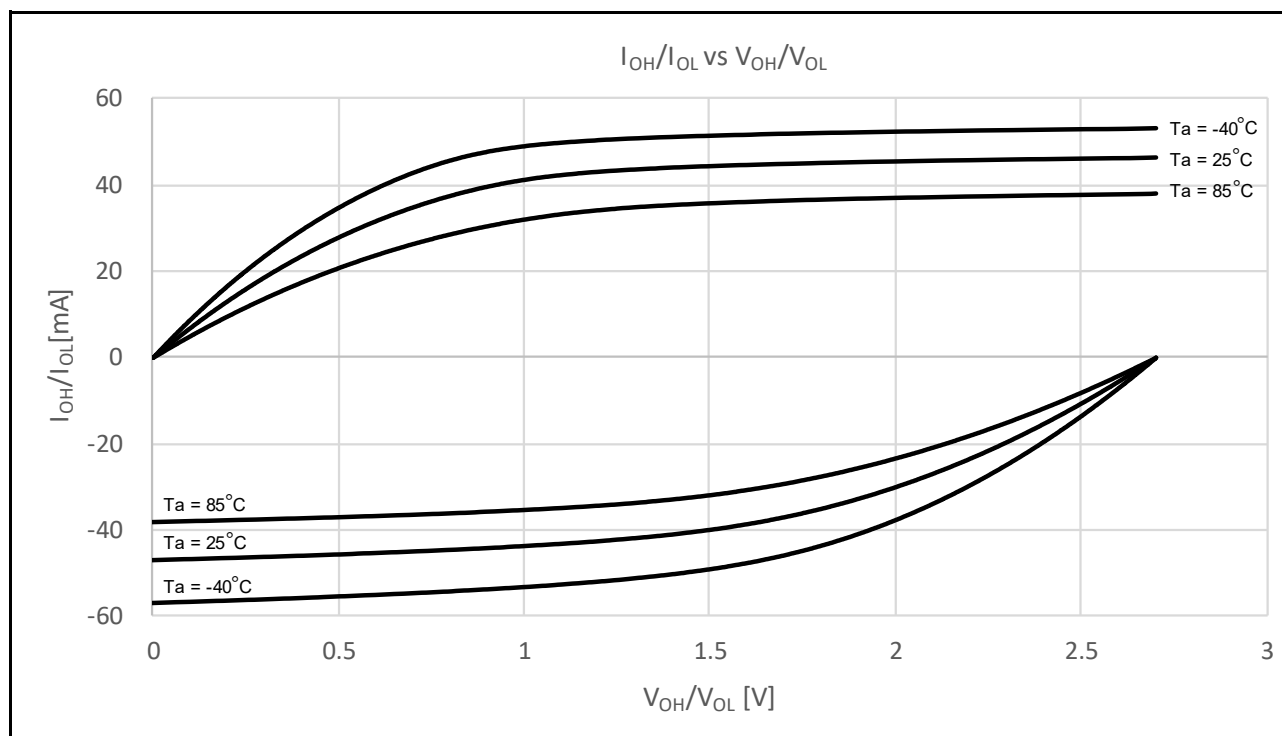
図 48.11 中駆動出力選択時の V_{CC} = 2.7\text{V} での V_{OH}/V_{OL} および I_{OH}/I_{OL} 温度特性 (参考データ)
