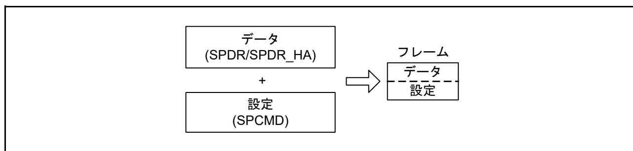
図 32.37 フレームの概念図 (SPI0)
