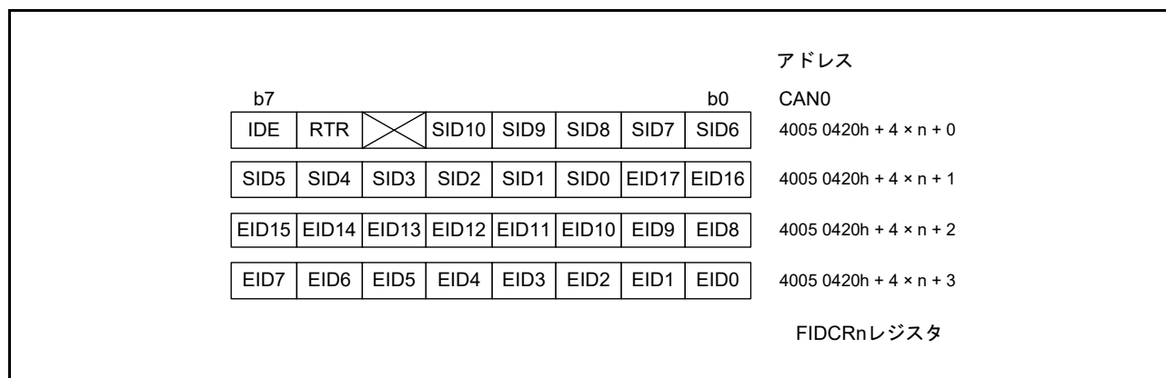
図 31.15 FIDCRn レジスタの構成 (n = 0, 1)
