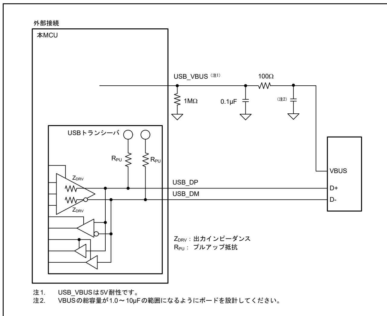
図 28.2 セルフパワード状態でのデバイス接続例
