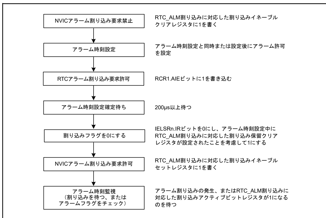
図 25.7 アラーム機能の使用法
