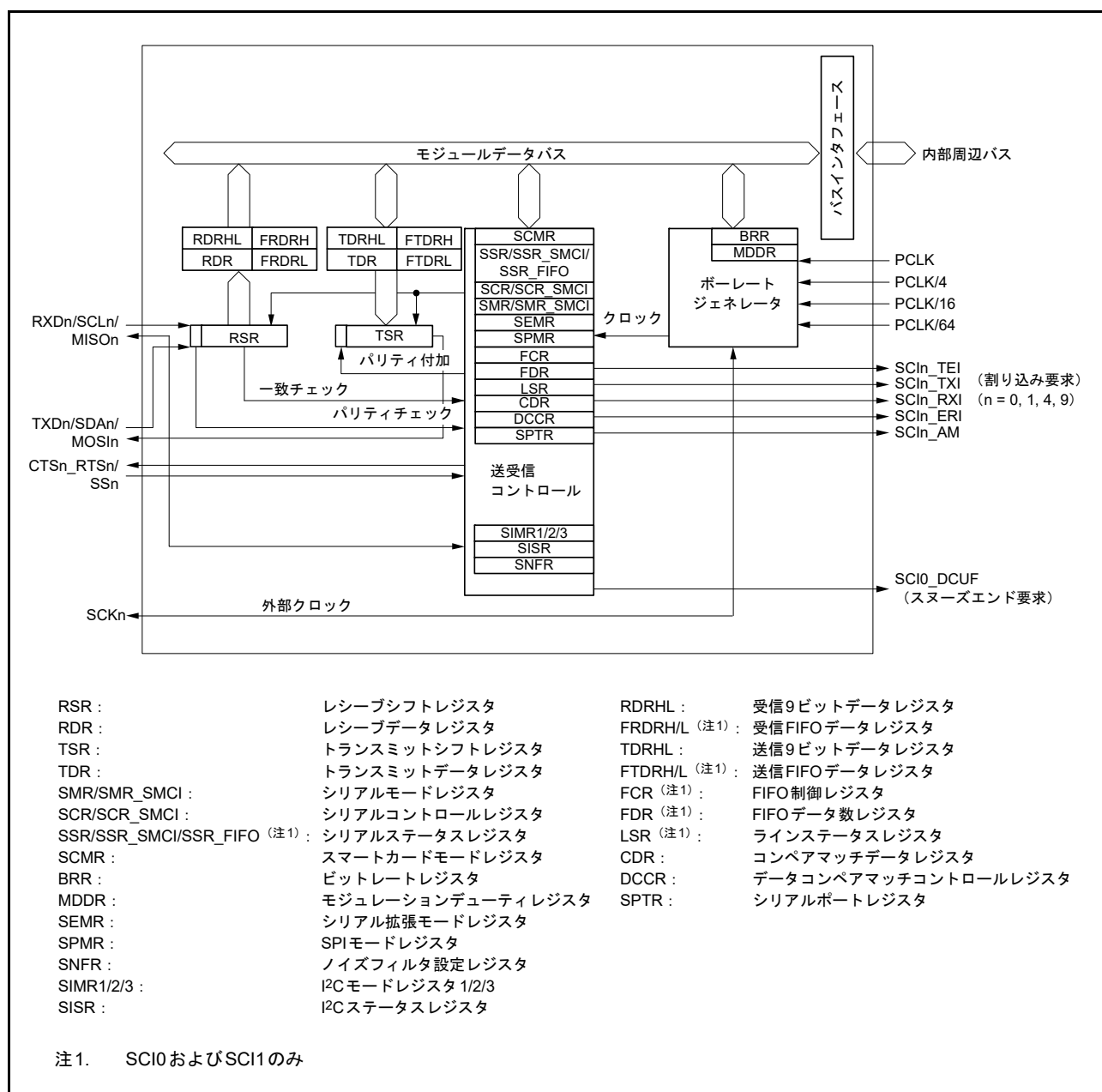
図 29.1 SCI のブロック図
