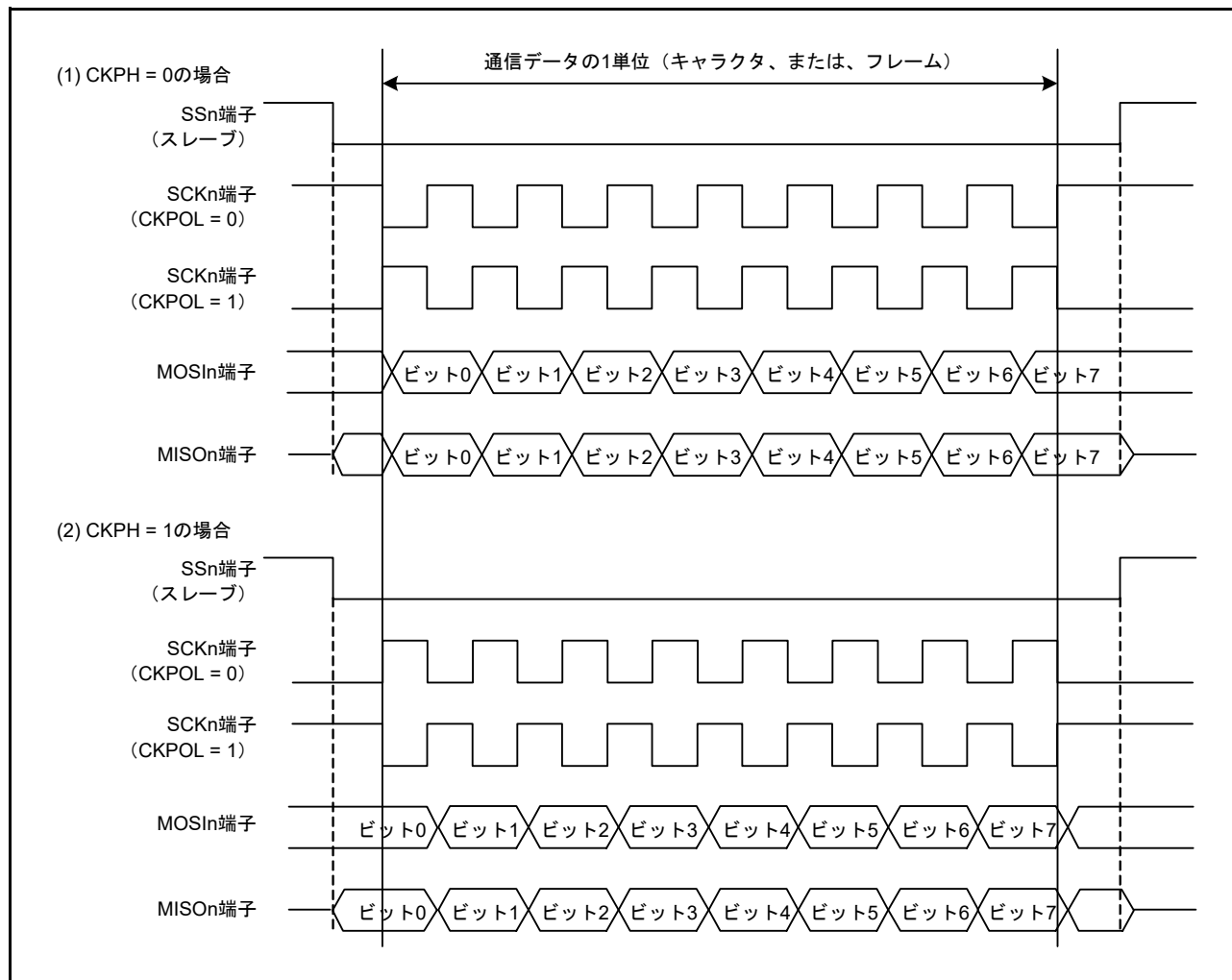
図 29.70 簡易 SPI モードにおけるクロックと送受信データの間係
