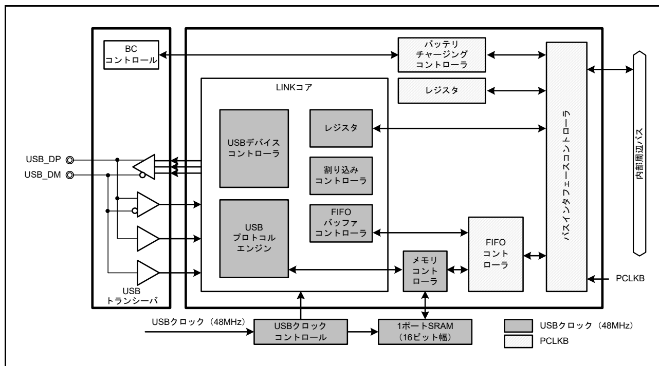
図 28.1 USBFS のブロック図
