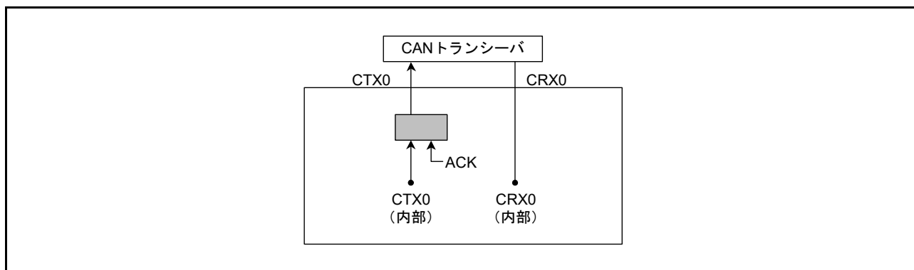
図 31.7 セルフテストモード 0 選択時の接続
