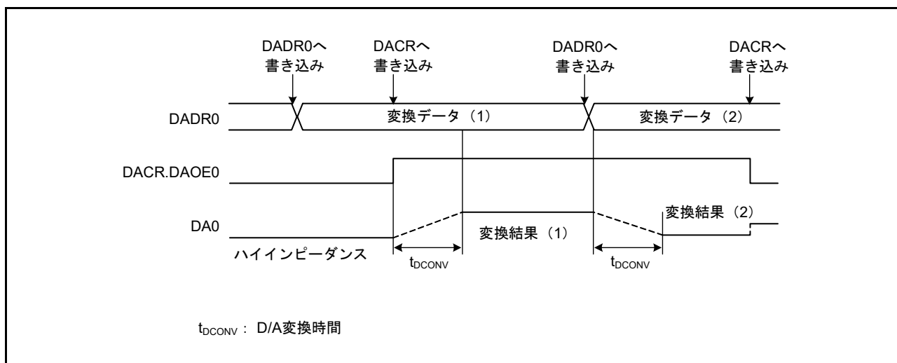
図 35.2 DAC12 の動作例
