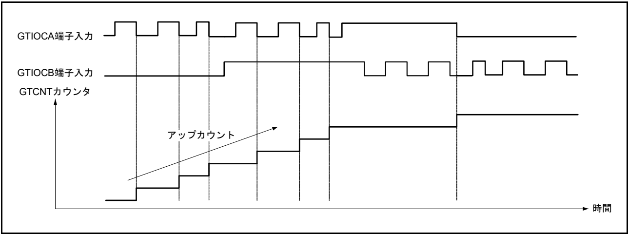
図 23.75 位相計数モード5 動作例（A）
