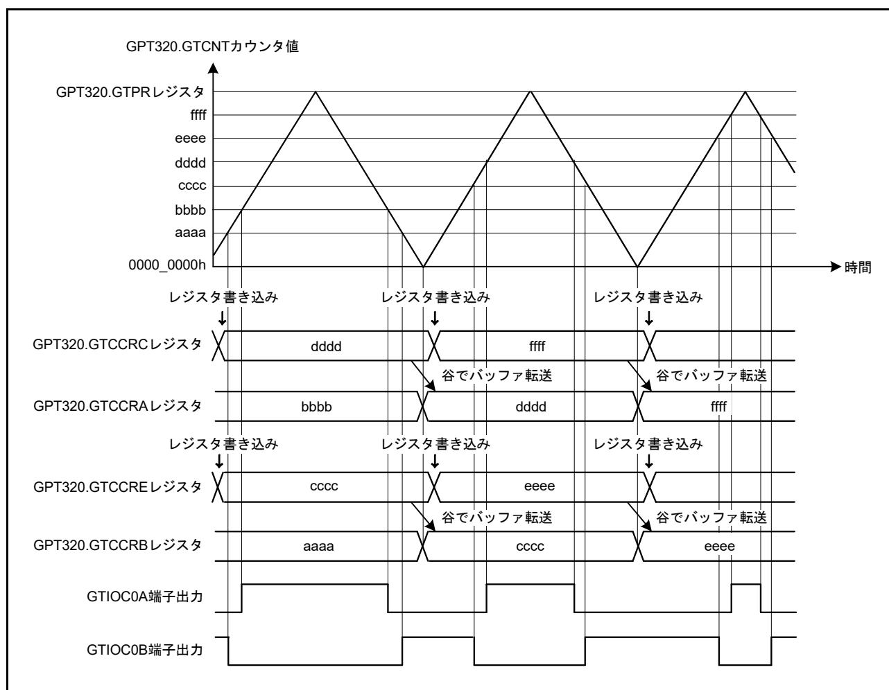
図 23.33 三角波 PWM モード 1 動作例 (バッファ動作、カウントスタート時 GTIOCA 端子 = Low 出力 / GTIOCB 端子 = High 出力、GTCCRA/GTCCRB レジスタのコンペアマッチでトグル出力、周期の終わりで出力保持の場合)
