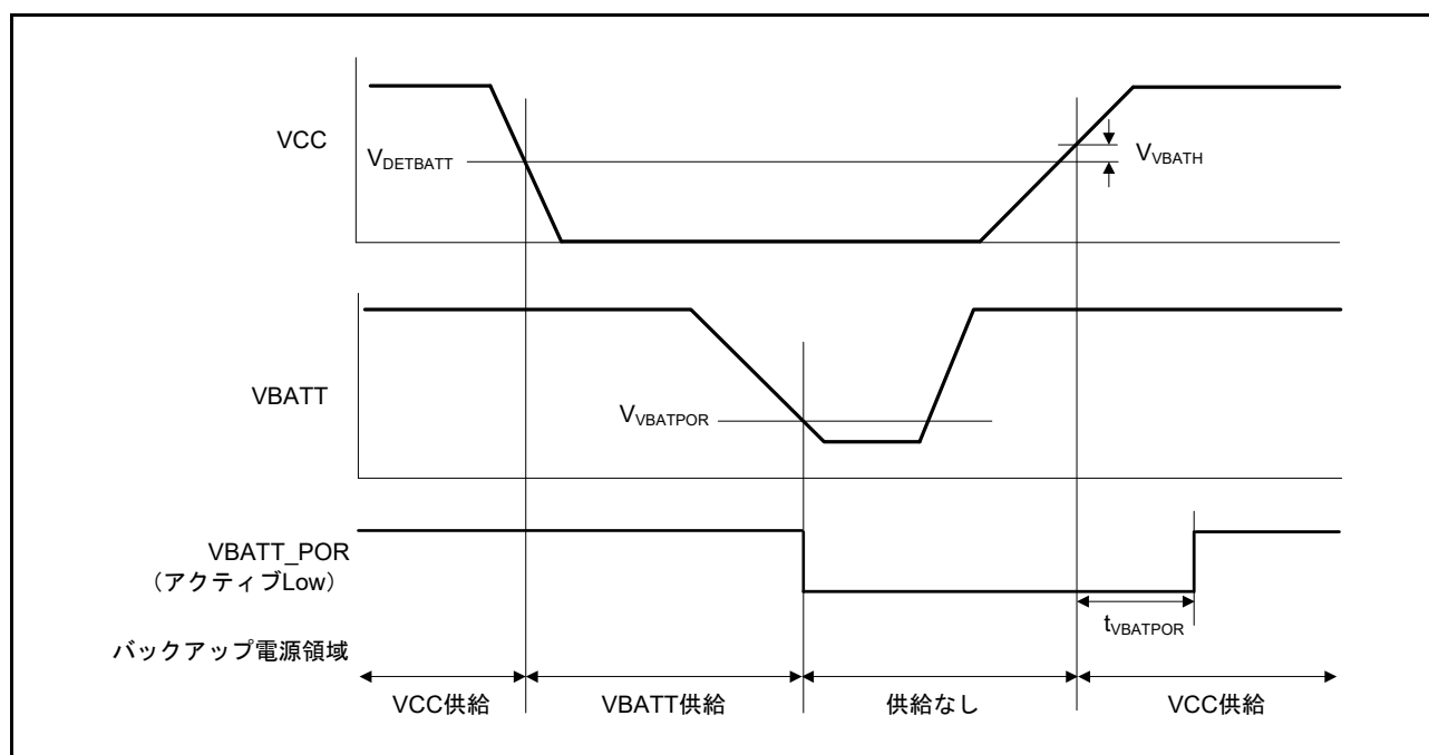
図 48.72 \text{VBATT\_POR} リセットタイミング
