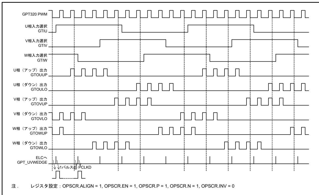
図 23.79 6 相 PWM 出力動作例（チョップパ制御）
