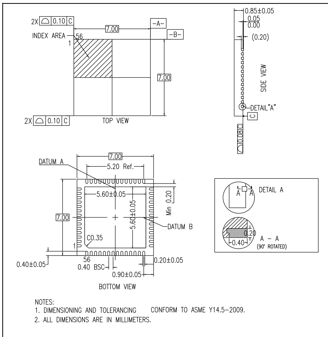
図 2.1 56-pin QFN
