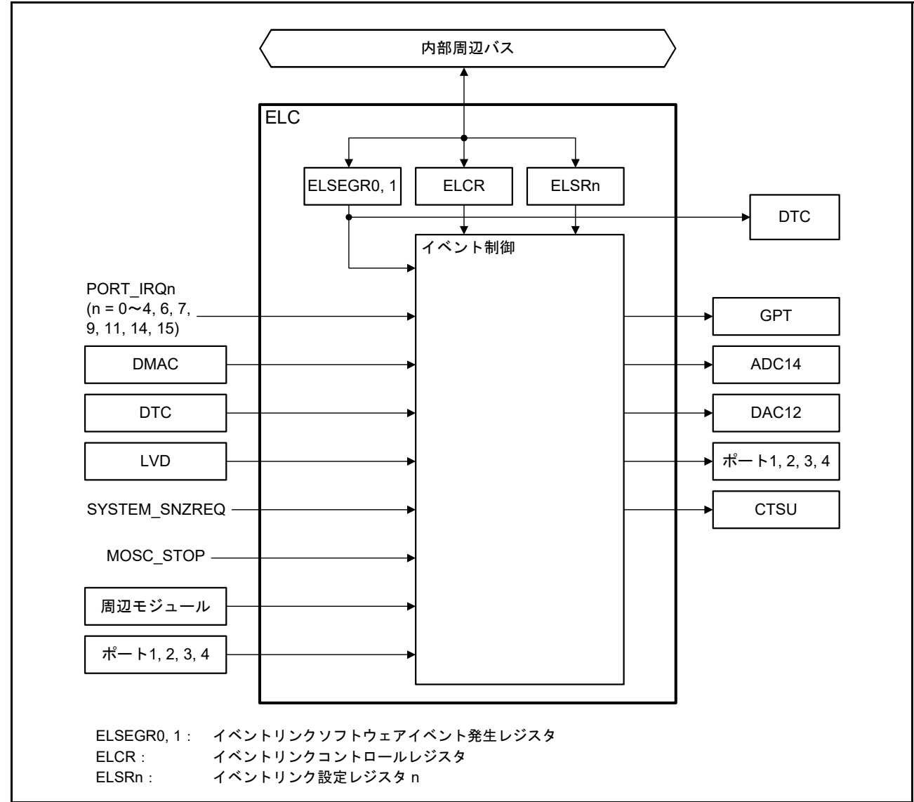
図 19.1 ELC のブロック図 (n = 0 ~ 9、12、14 ~ 18)
