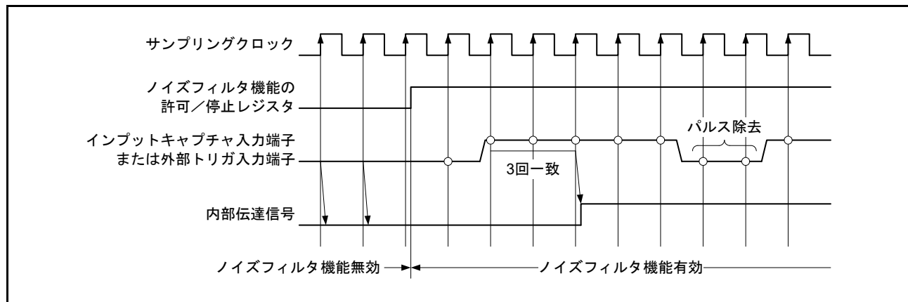
図 23.82 ノイズフィルタのタイミング
