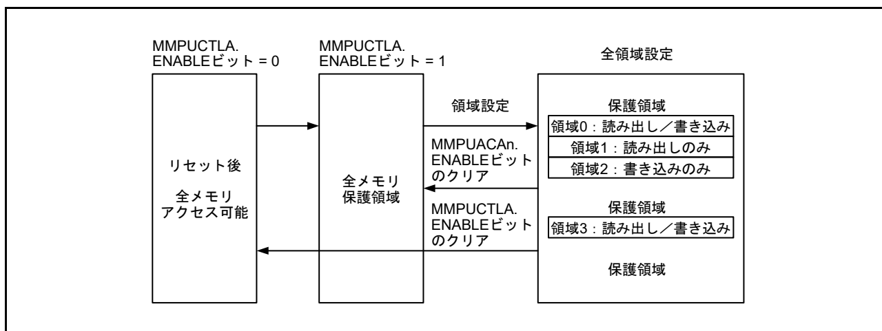
図 16.5 バスマスタ MPU の使用例
