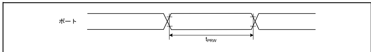
図 48.35 I/O ポート入力タイミング
