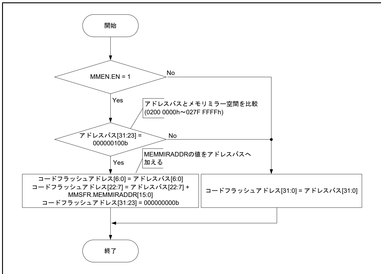
図 5.4 メモリミラー機能の動作フローチャート
