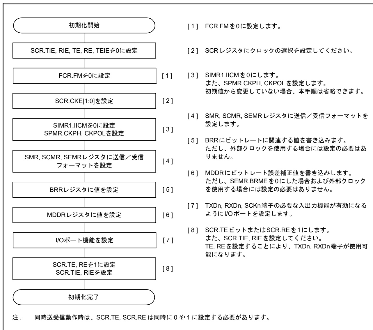
図 29.32 クロック同期式モードにおける SCI の初期化フローチャート例 (非 FIFO 選択時)
