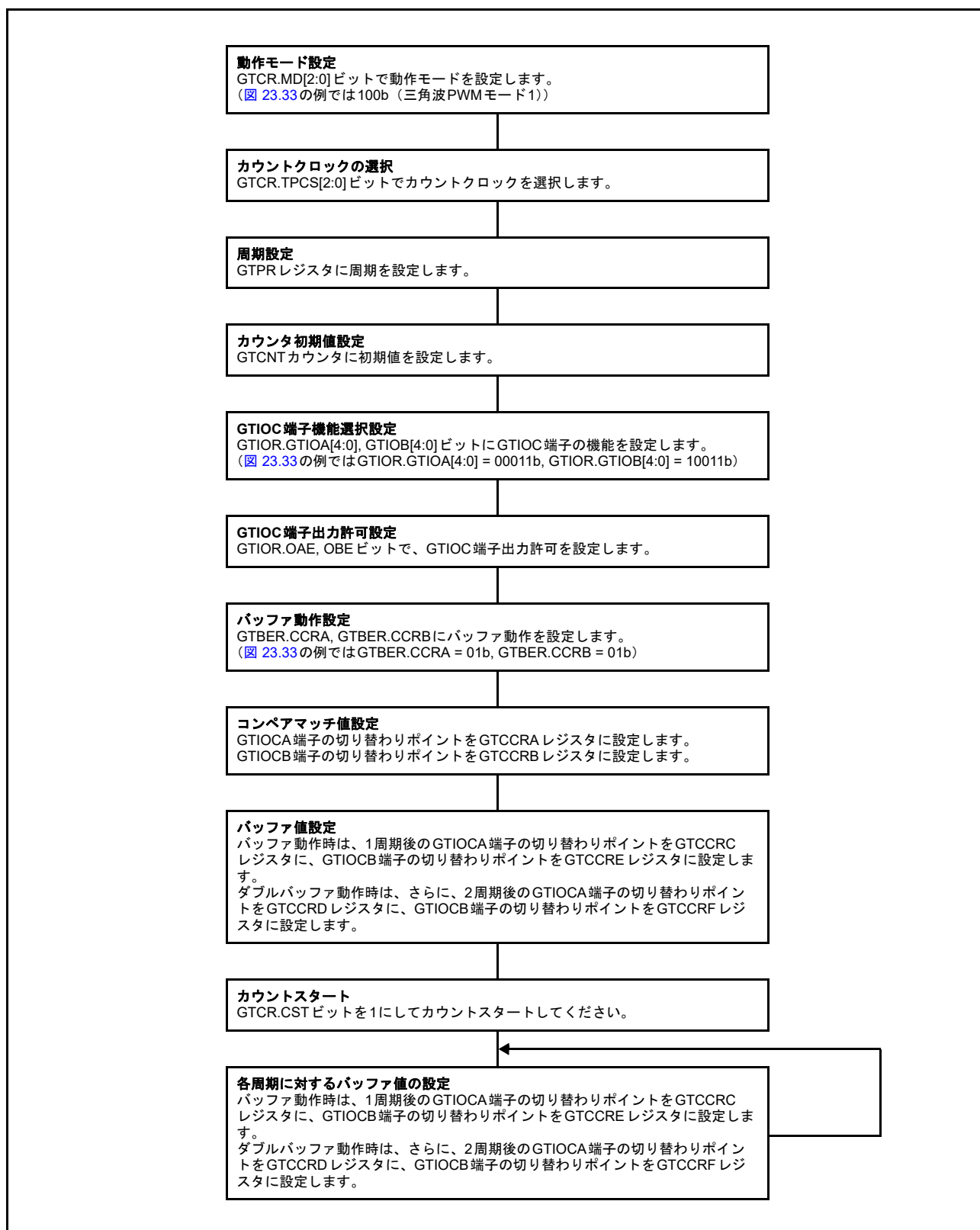
図 23.34 三角波 PWM モード 1 の設定例
