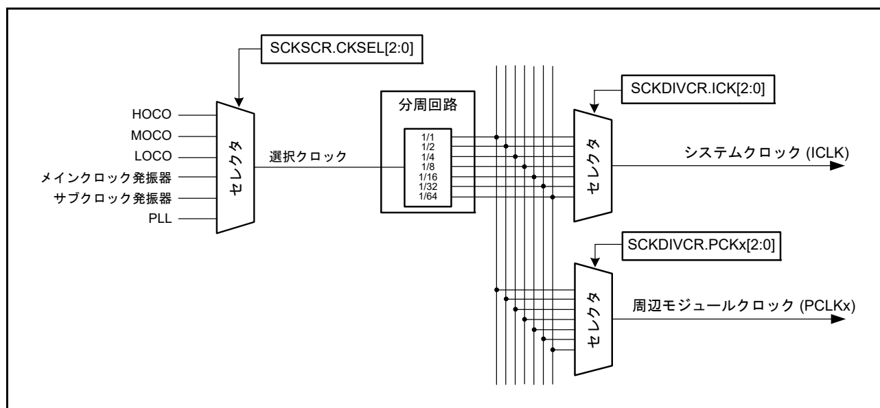
図 9.10 クロックソース選択ブロック図
