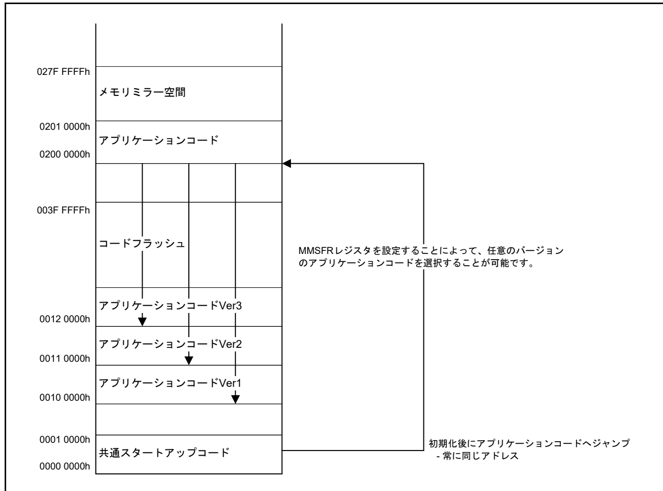
図 5.6 メモリミラー機能
