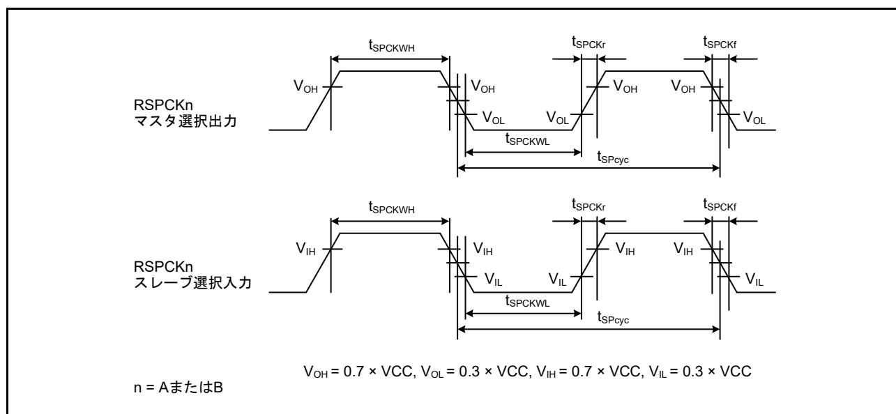
図 48.49 SPI クロックタイミング
