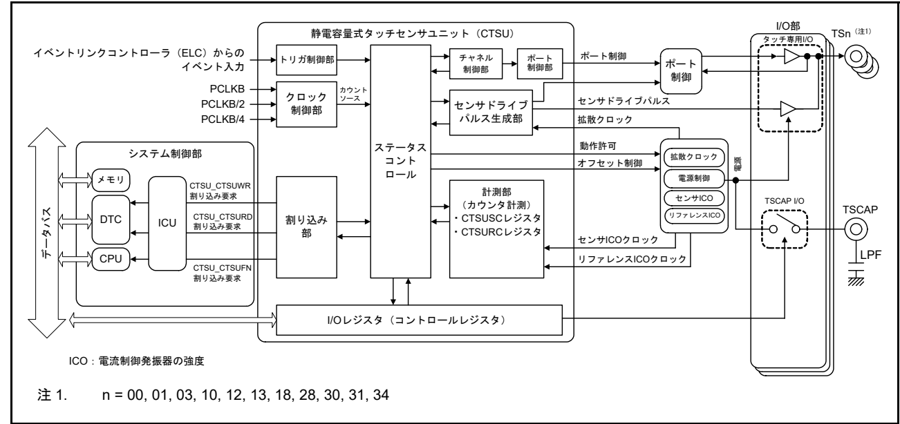
図 40.3 CTSU のブロック図
