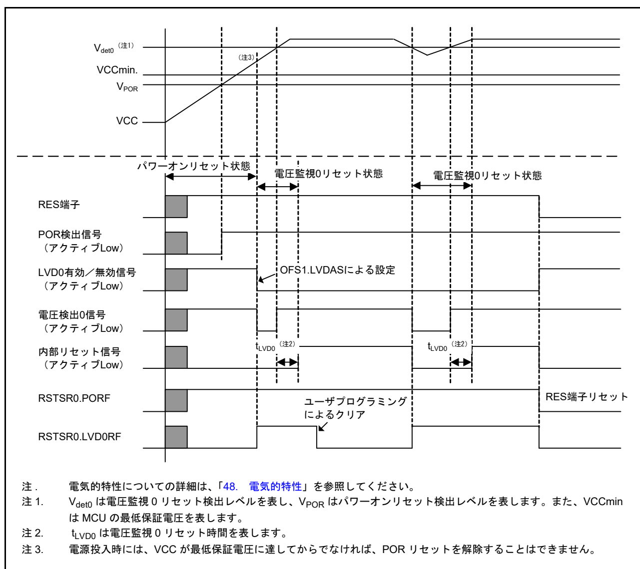
図 6.1 パワーオンリセットおよび電圧監視 0 リセット時の動作例
