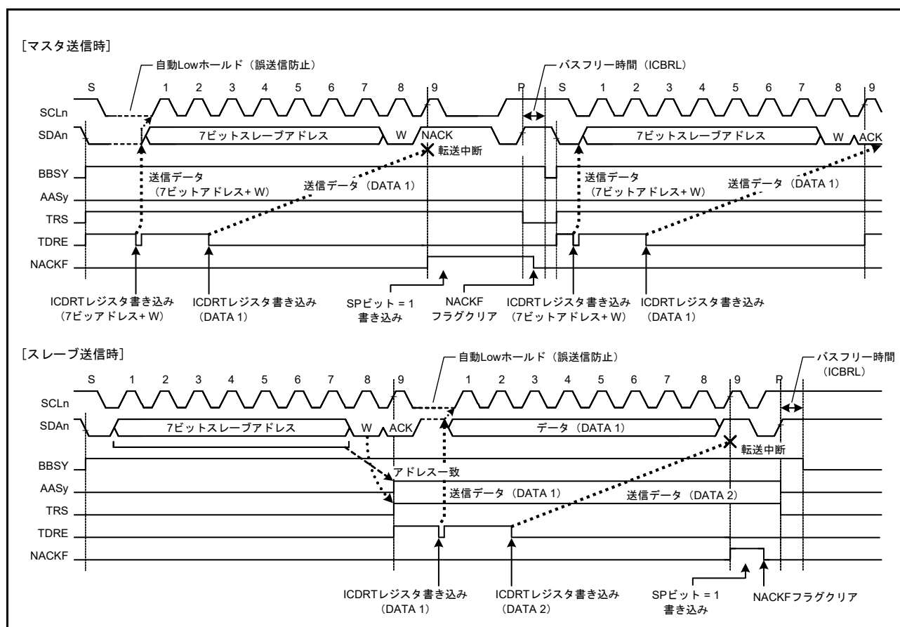
図 30.39 NACK 受信時のデータ転送中断動作 (NACKF = 1 の場合)
