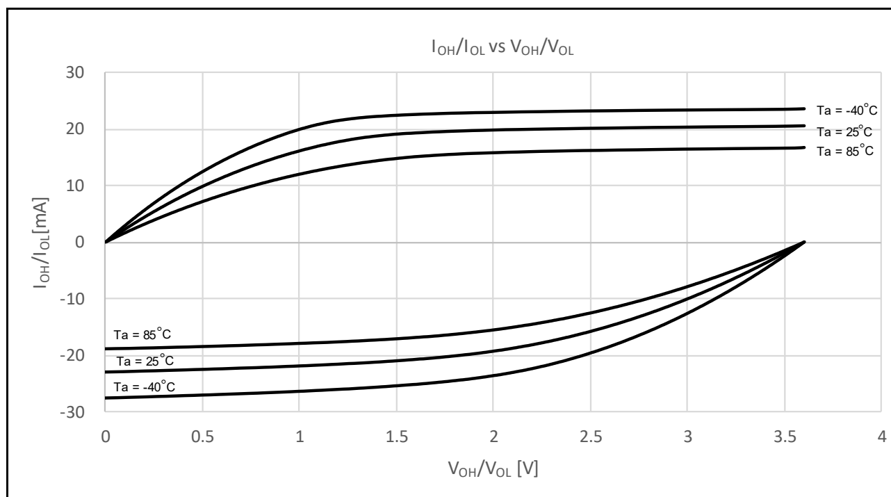
図 48.5 低駆動出力選択時の V_{CC} = 3.6\text{V} での V_{OH}/V_{OL} および I_{OH}/I_{OL} 温度特性 (参考データ)
