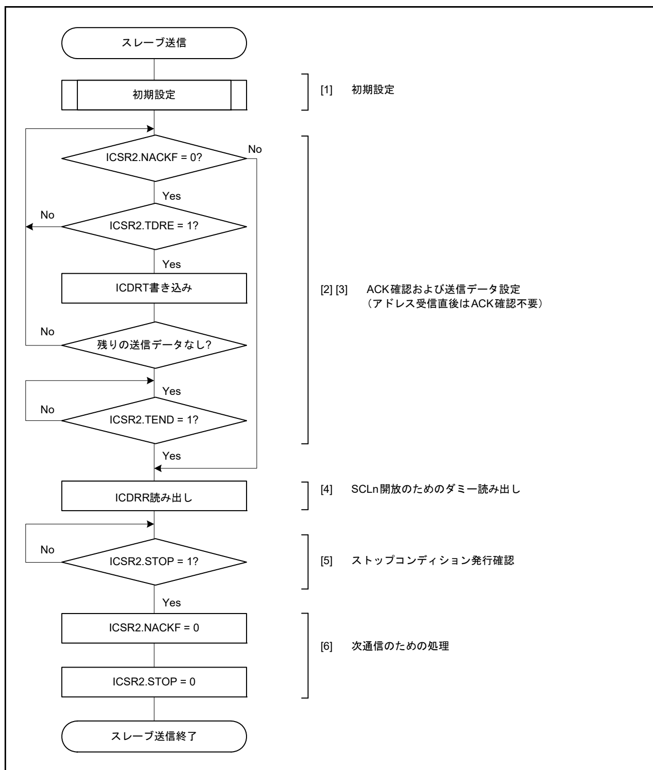
図 30.15 スレーブ送信のフロー例
