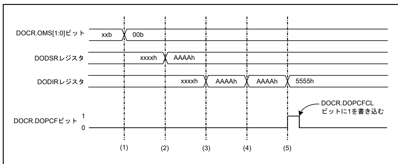
図 41.2 データ比較モードの動作例
