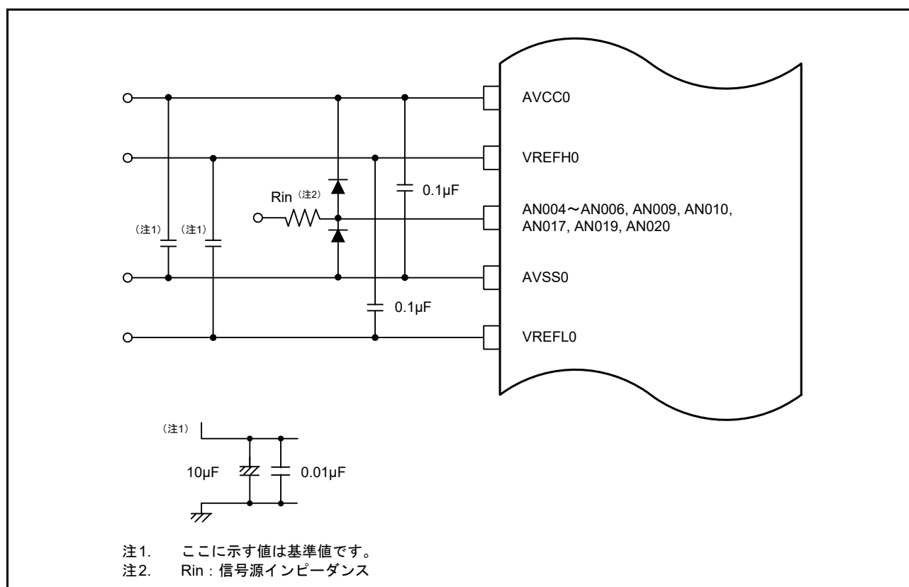
図 34.32 アナログ入力用保護回路例
