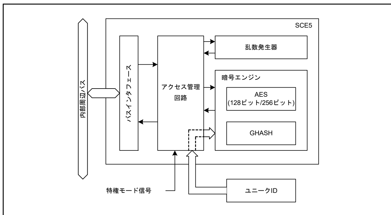
図 45.1 SCE5 ブロック図
