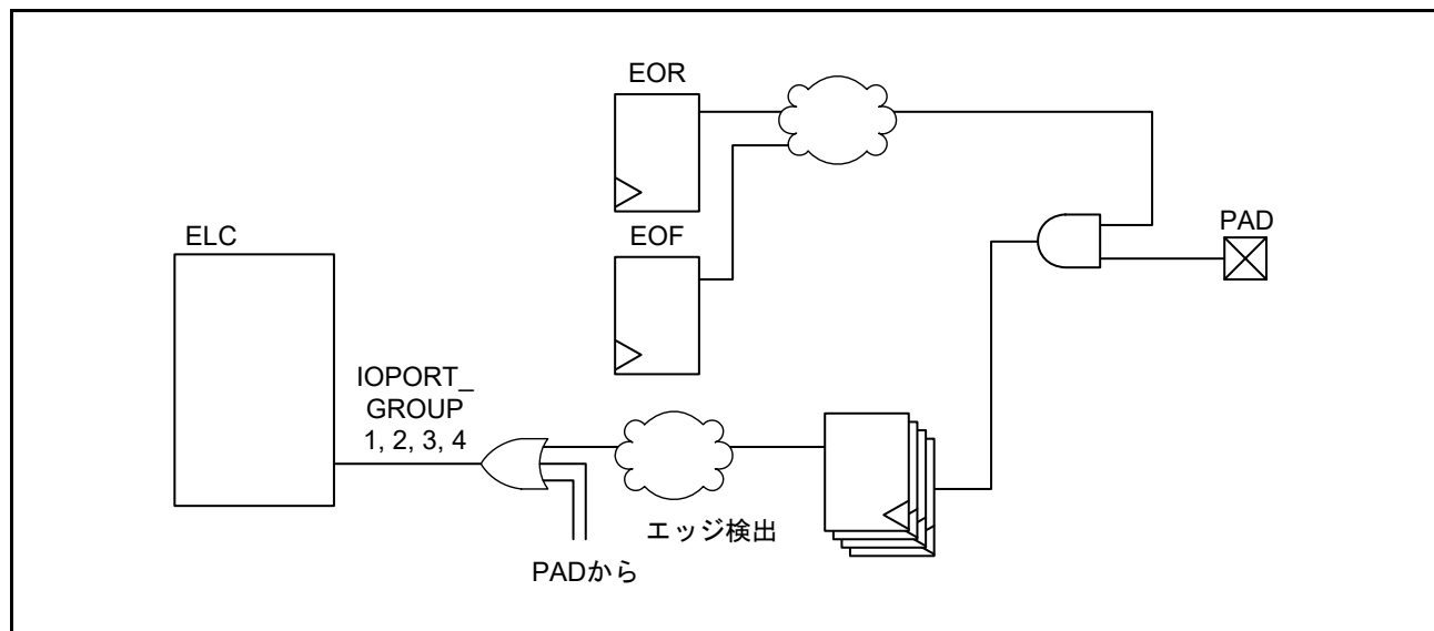
図 20.4 イベントパルスの発生
