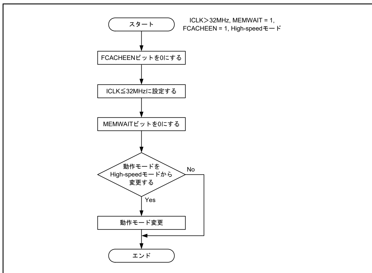
図 9.3 ICLK > 32MHz の状態から ICLK ≤ 32MHz に設定する場合
