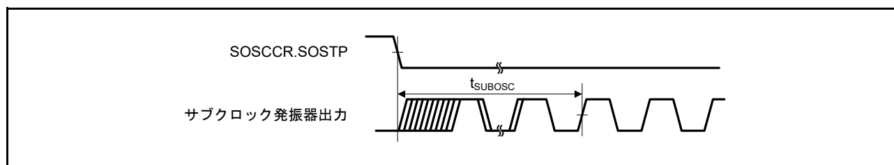
図 48.27 サブクロック発振開始タイミング
