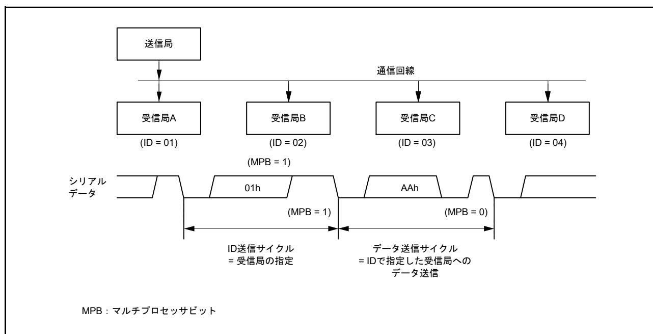
図 29.22 マルチプロセッサフォーマットを使用した通信例（データ AAh を受信局 A に送信する場合）
