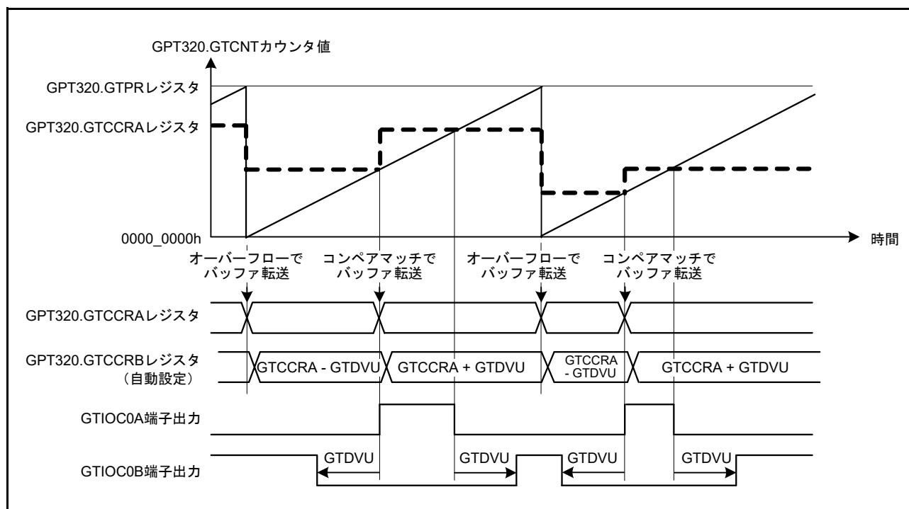
図 23.39 デッドタイム自動設定機能の動作例 (のこぎり波ワンショットパルスモード、アップカウント、アクティブ High の場合)
