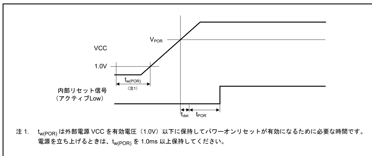
図 48.68 パワーオンリセットタイミング
