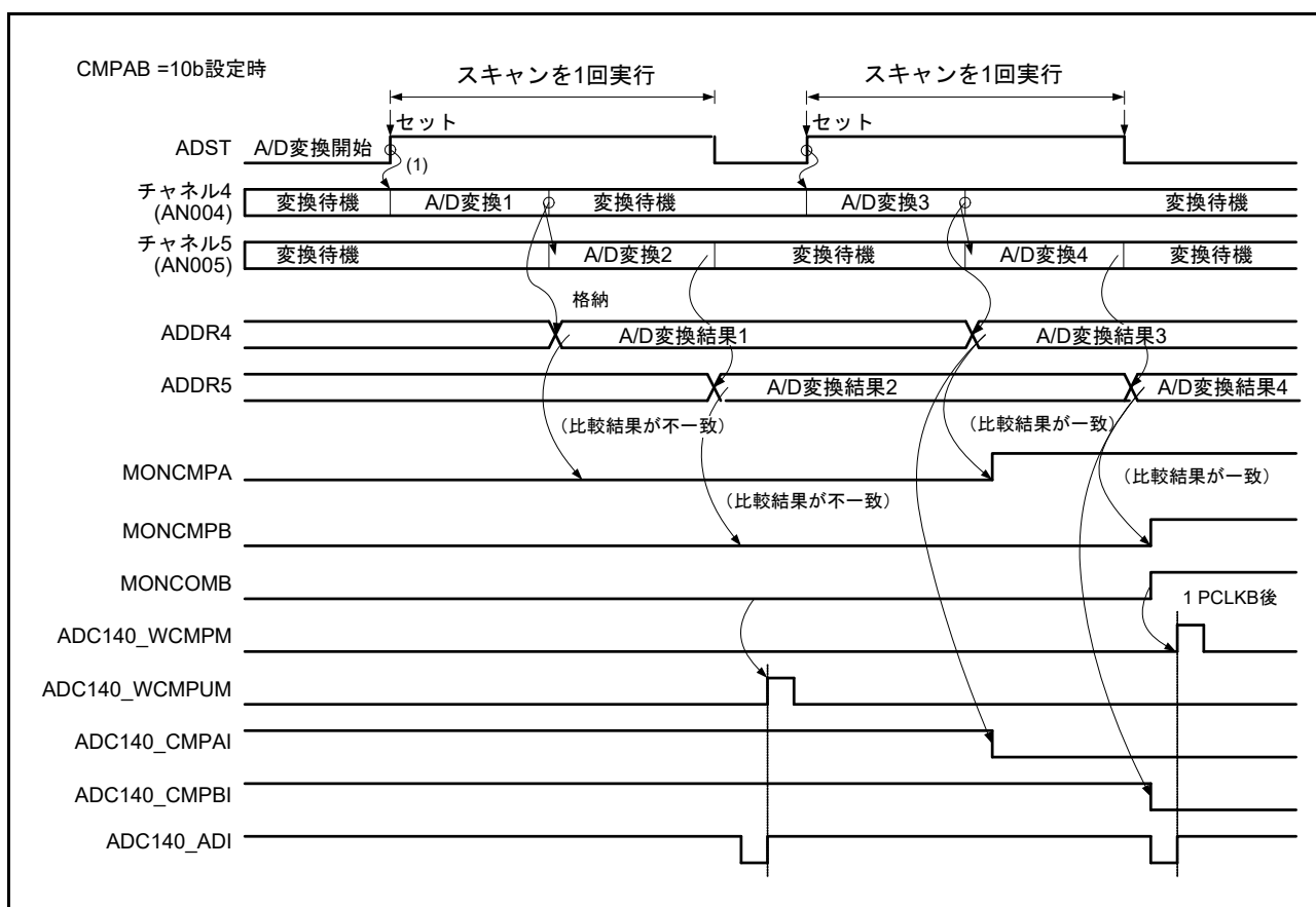
図 34.23 コンペア機能のイベント出力動作例 (AN004 ~ AN005 を比較)
