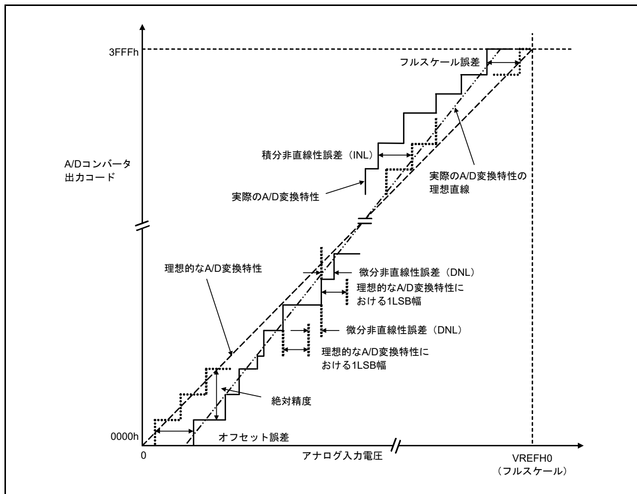
図 48.64 14 ビット A/D コンバータ 特性用語の解説図
