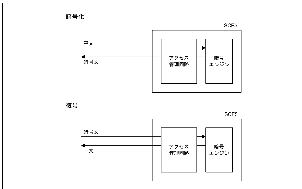
図 45.2 暗号エンジンによる暗号化と復号
