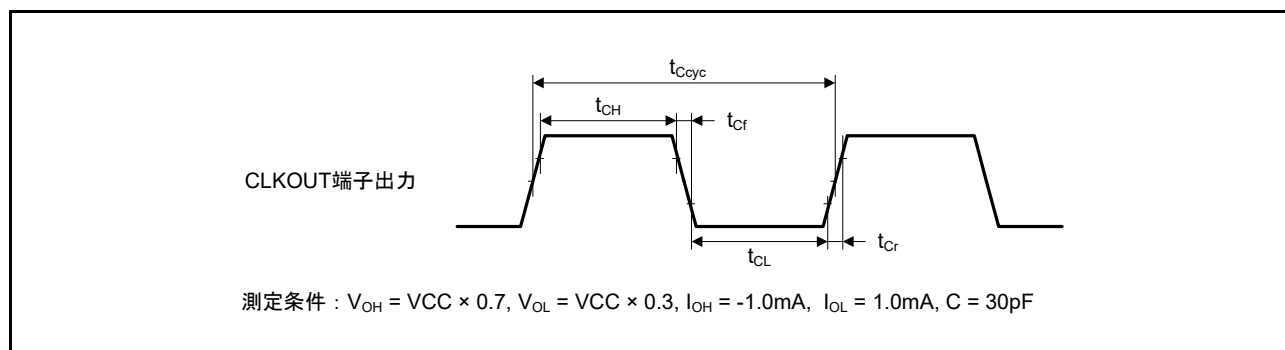
図 48.57 CLKOUT 出力タイミング
