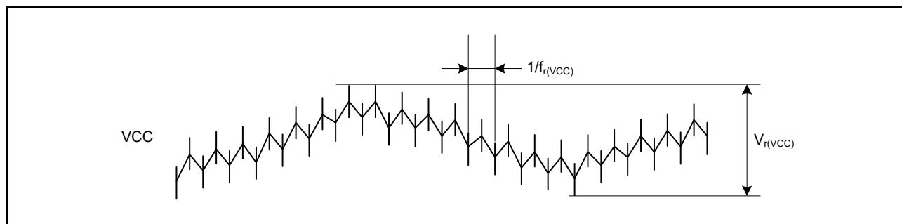
図 48.21 リップル波形
