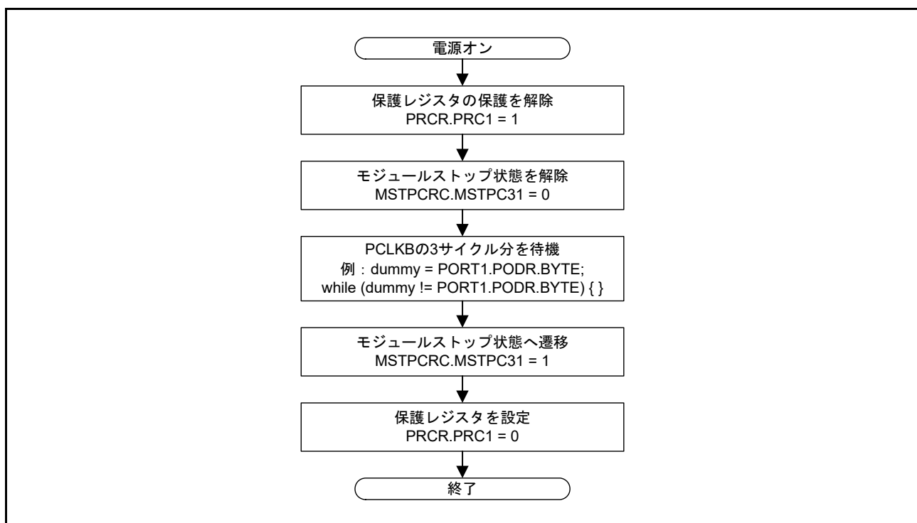
図 11.13 未使用回路の初期設定フロー例
