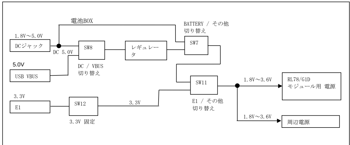
図 6-1 電源系統
