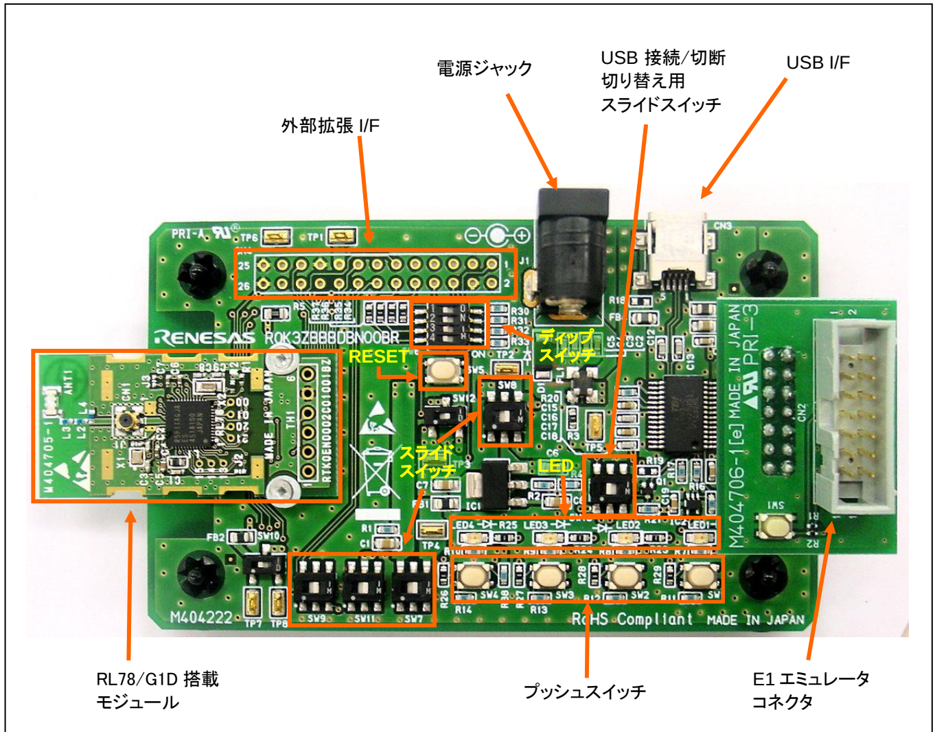
図 2-1 基板外観
