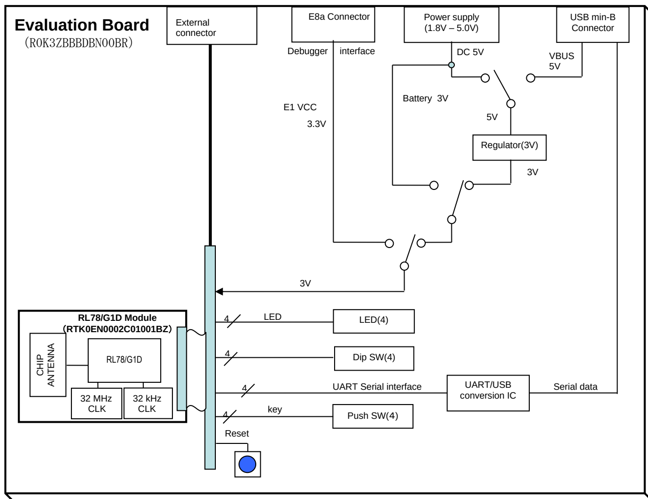
図 1-1 RL78/G1D 評価ボード（RTK0EN0001D01001BZ） ブロック図
