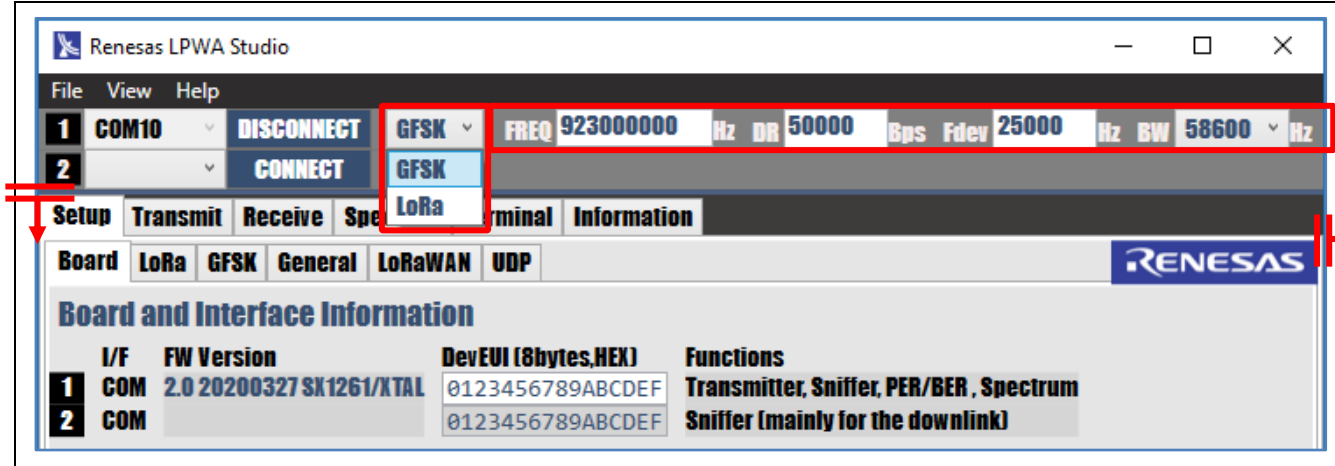
Figure 6. GFSK Parameters
