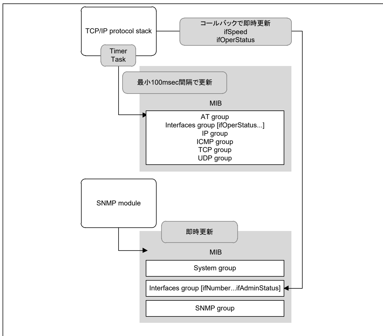
図2.1 MIB-IIのデータ更新
