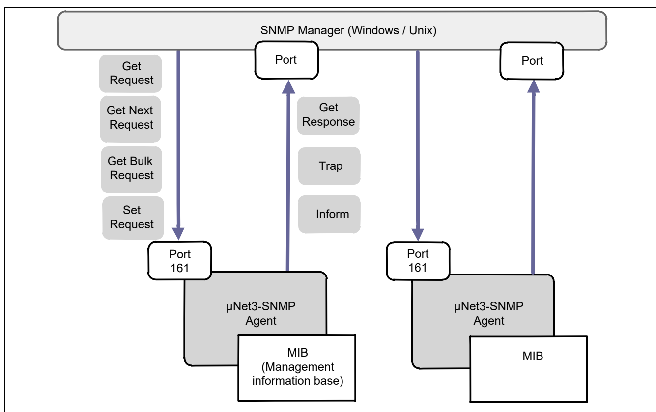
図 1.1 SNMPのマネージャーとエージェント
