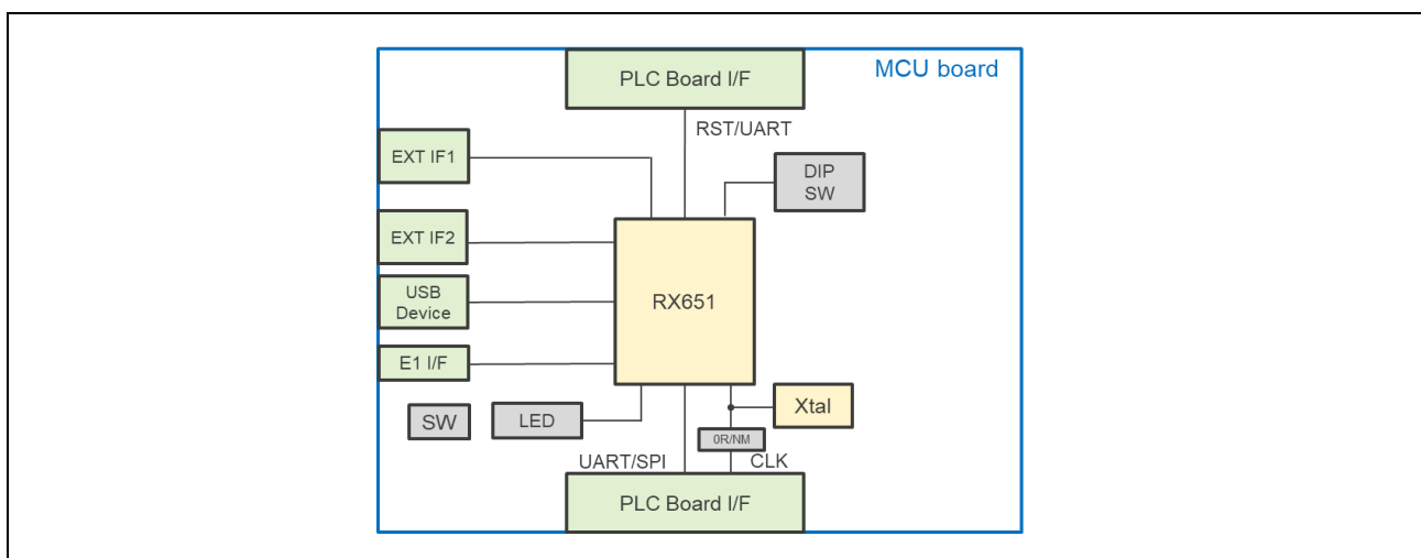
Figure 1-3 MCU回路機能ブロック図
