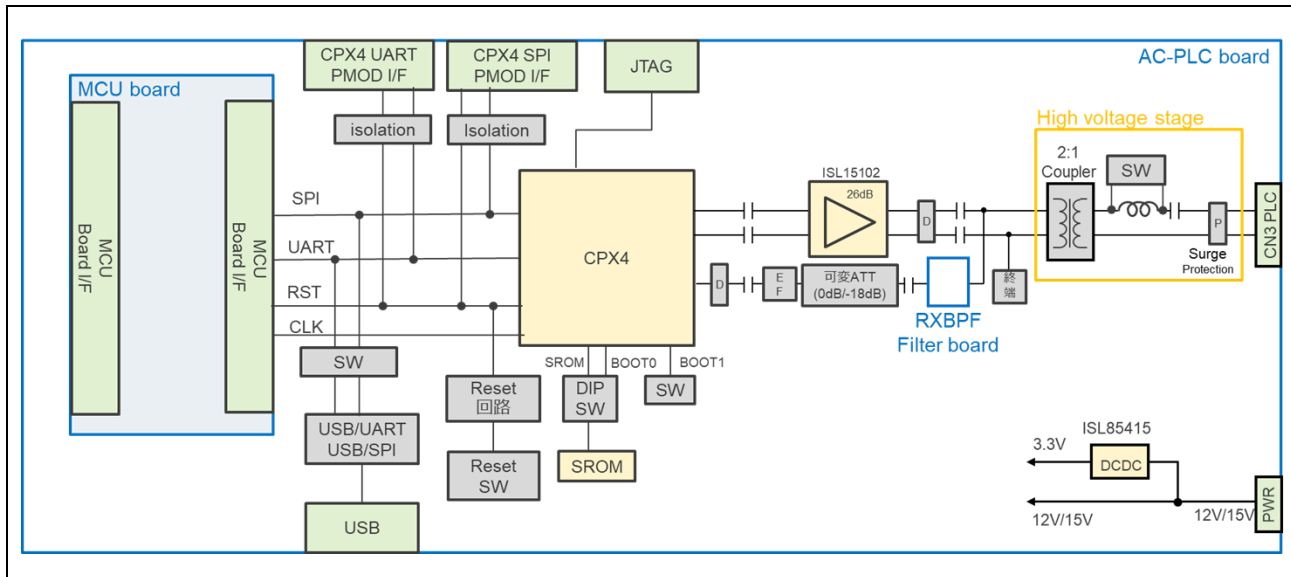
Figure 1-2 AC-PLC回路機能ブロック図
