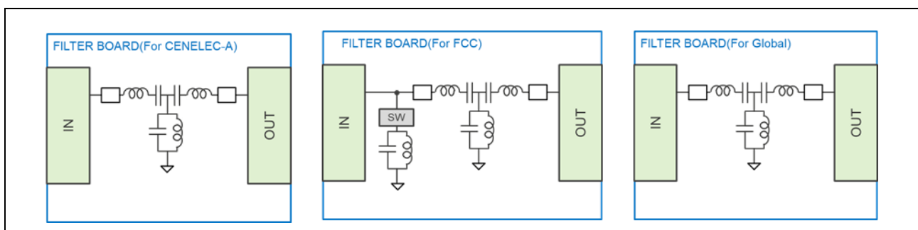
Figure 1-4 フィルタボード回路機能ブロック図
