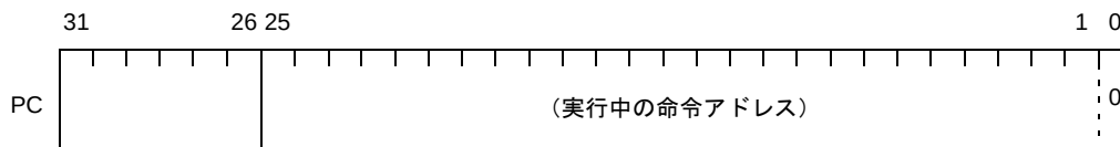
図 4—11 プログラム・カウンタ【V850ES, V850E1】
