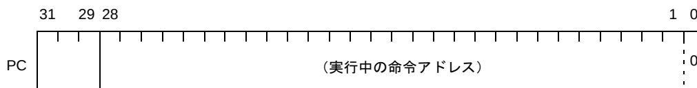
図 4—12 プログラム・カウンタ【V850E2】
