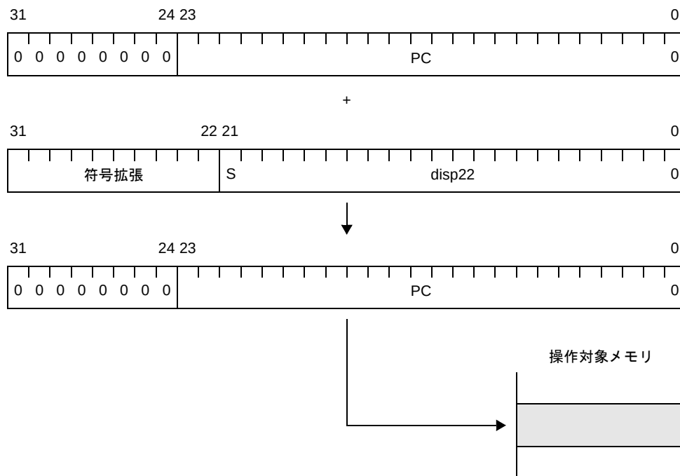
図 4—47 レラティブ・アドレッシング（JR disp22 / JARL disp22, reg2）【V850 マイクロコントローラ】
