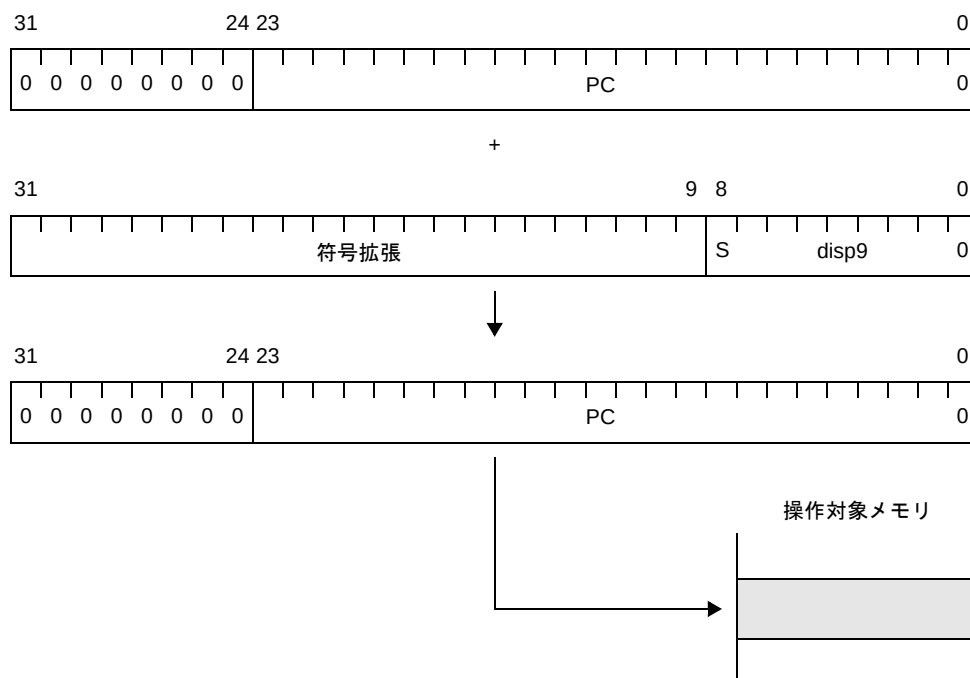
図 4—51 レラティブ・アドレッシング (Bcnd disp9) 【V850 マイクロコントローラ】
