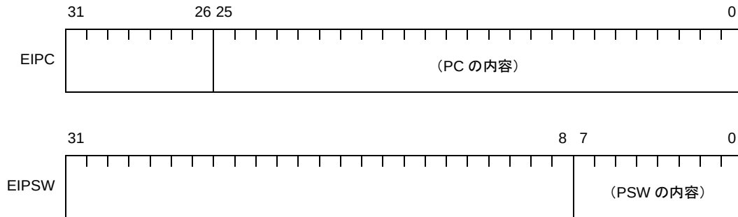
図 4—14 割り込み時状態退避レジスタ【V850ES】
