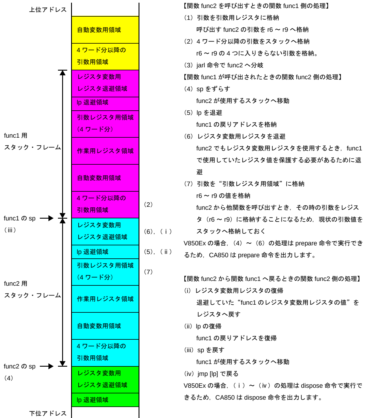
図 3—18 スタック・フレームの生成／消滅（引数レジスタ領域がスタックの中央にくる場合）
