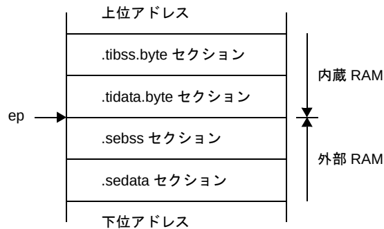
図 4—4 外部 RAM (.sedata, / .sebss セクション) のメモリ配置イメージ
