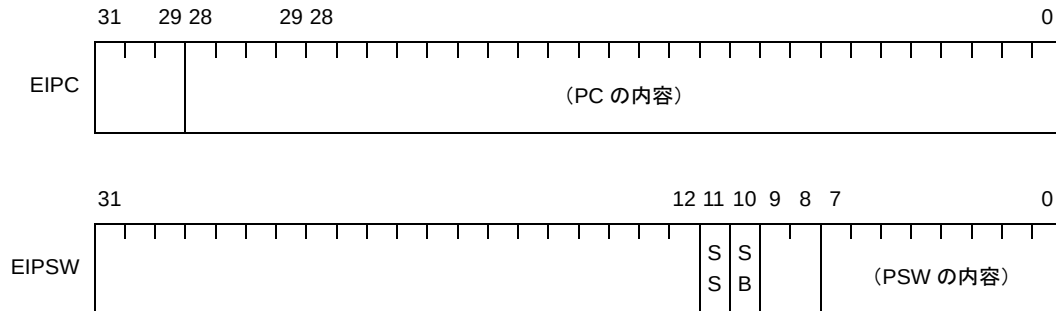
図 4—16 割り込み時状態退避レジスタ【V850E2】
