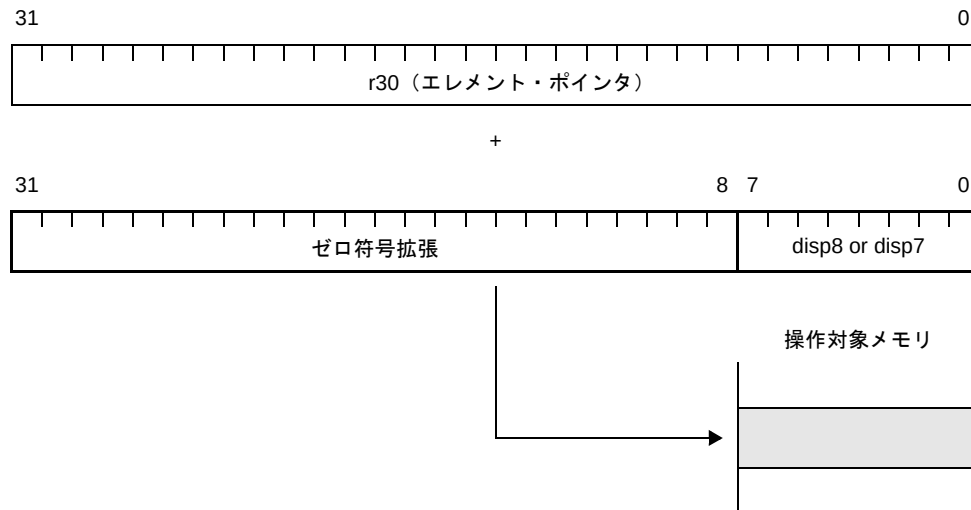
図 4—59 ペースト・アドレッシング (タイプ2) 【V850 マイクロコントローラ, V850ES, V850E1, V850E2】
