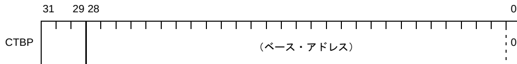
図 4—32 CALLT ベース・ポインタ 【V850E2】
