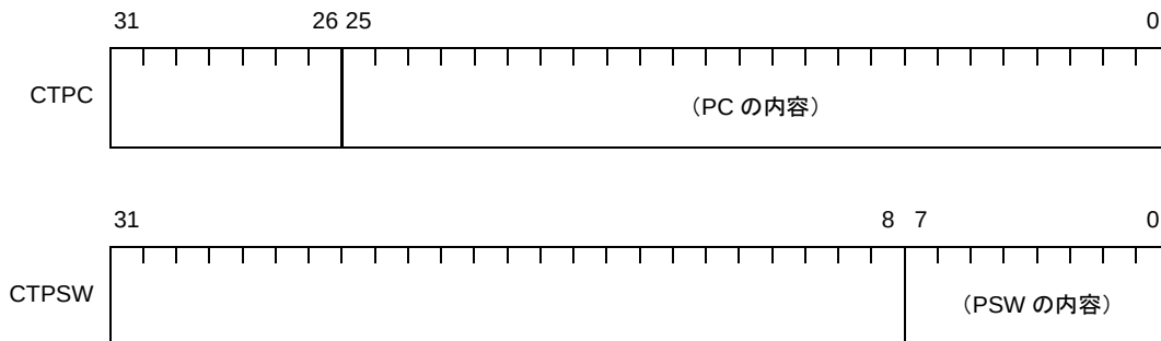
図 4—25 CALLT 実行時状態退避レジスタ 【V850ES】
