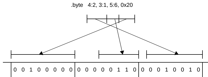
図 4—6 ビット幅を指定した割り付けの例
