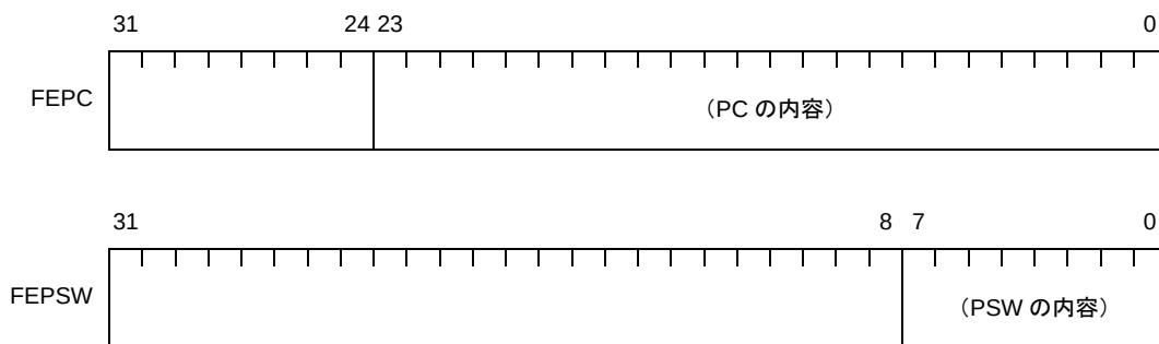
図 4—17 NMI 時状態退避レジスタ 【V850】
