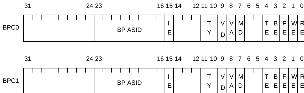
図 4—36 ブレークポイント制御レジスタ 【V850E1】
