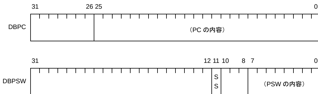
図 4—29 例外／デバッグ・トラップ時状態退避レジスタ【V850E1】
