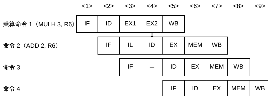
図 4—80 乗算命令実行結果の参照例
