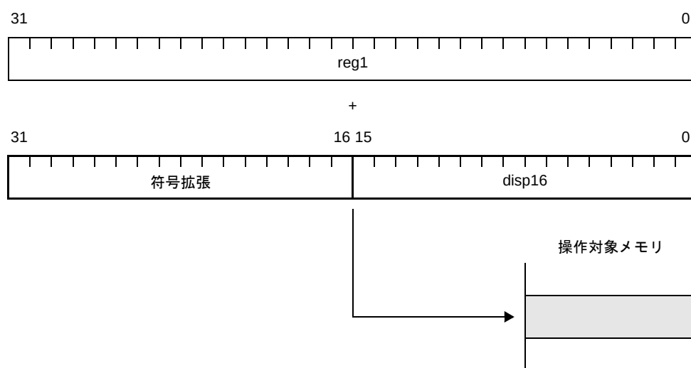
図4—58 ペースト・アドレッシング（タイプ1）【V850 マイクロコントローラ, V850ES, V850E1, V850E2】
