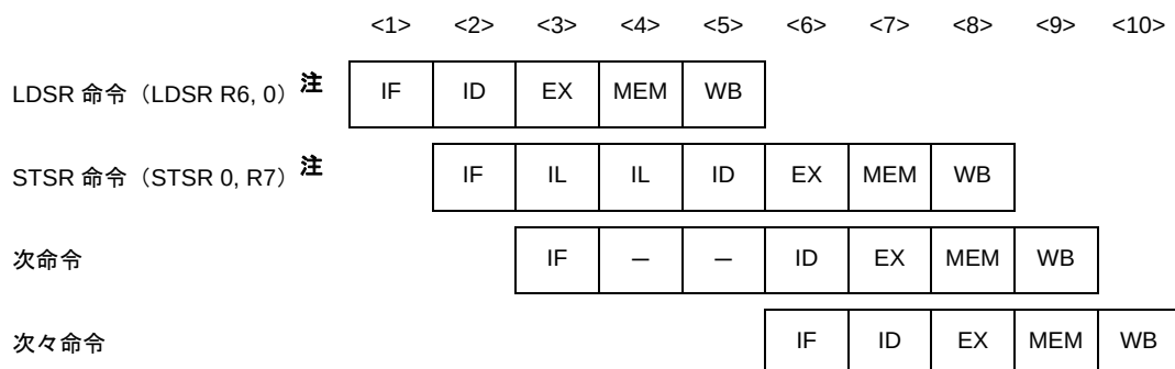
図 4—68 EIPC, FEPC を対象とする LDSR 命令実行結果の参照例
