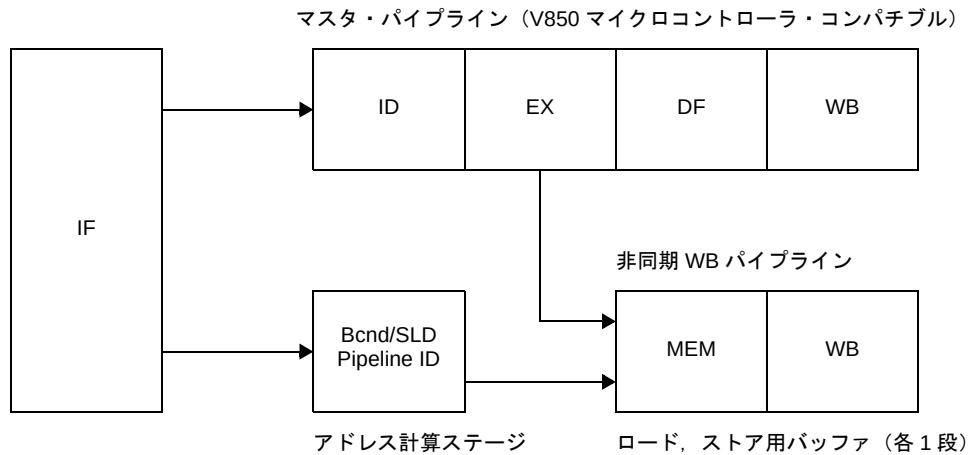
図4—77 パイプライン構成（V850E1）
