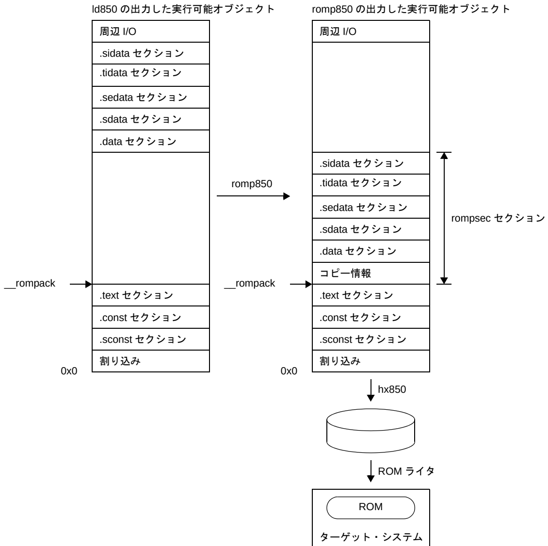
図 8—10 ROM 化のイメージ 1
