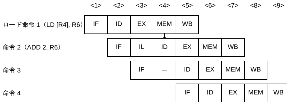
図 4—79 ロード命令実行結果の参照例
