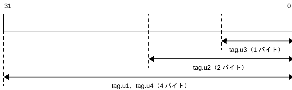
図 3—7 共用体型の内部表現
