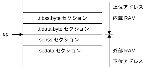
図4—62 外部 RAM (.sedata / .sebss セクション) のメモリ配置イメージ
