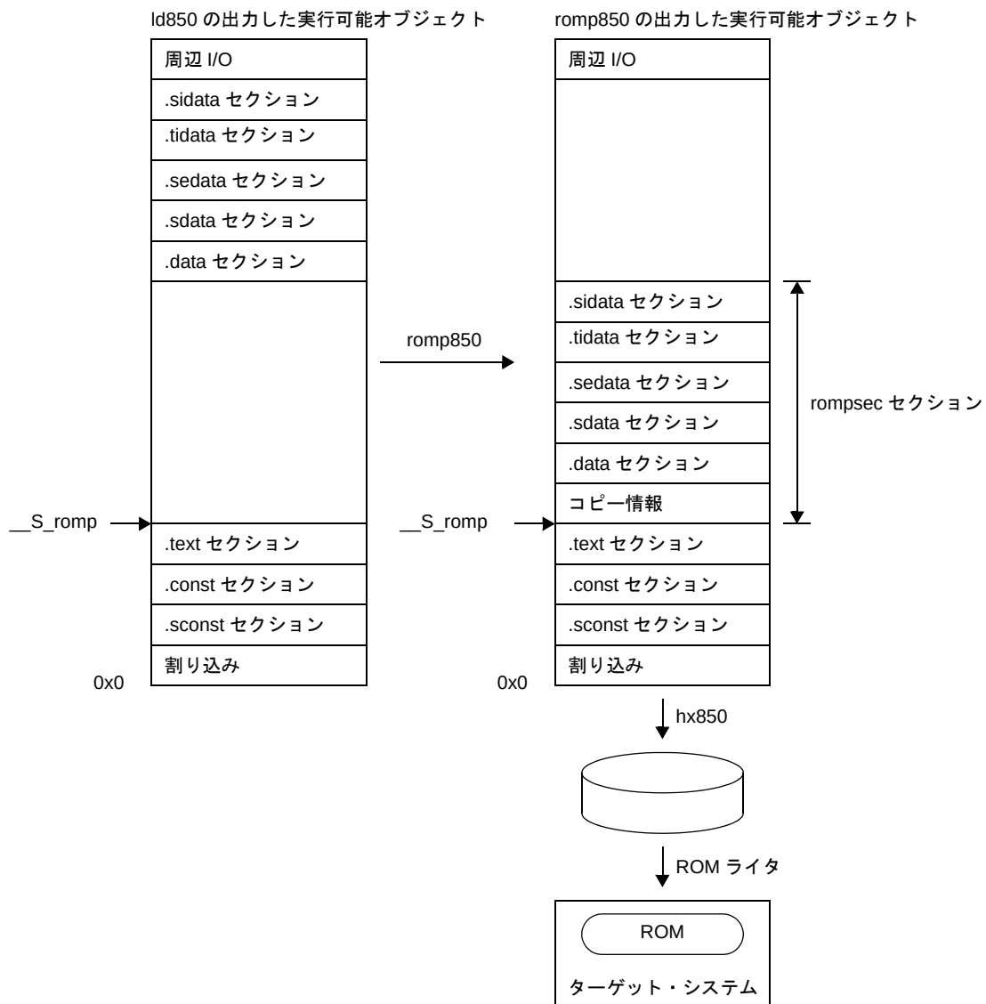
図 8—6 ROM 化のイメージ 1
