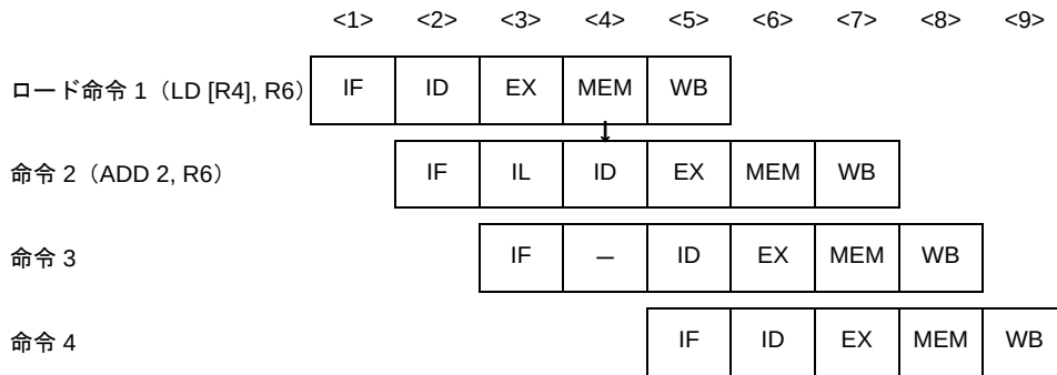
図 4—72 ロード命令実行結果の参照例
