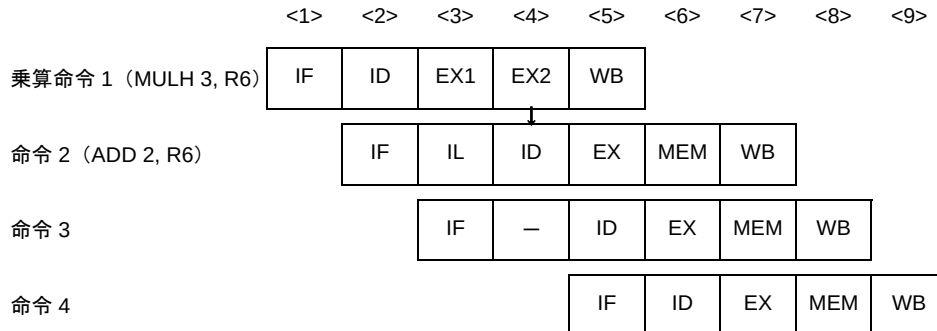
図 4—67 乗算命令実行結果の参照例
