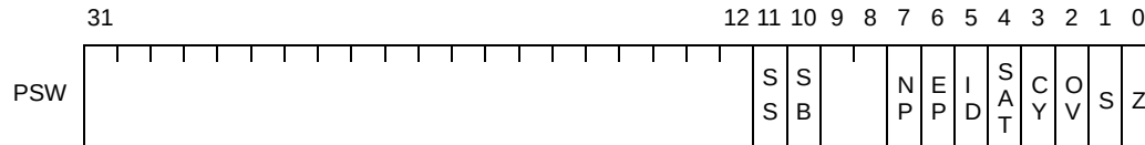
図 4—24 プログラム・ステータス・ワード【V850E2】
