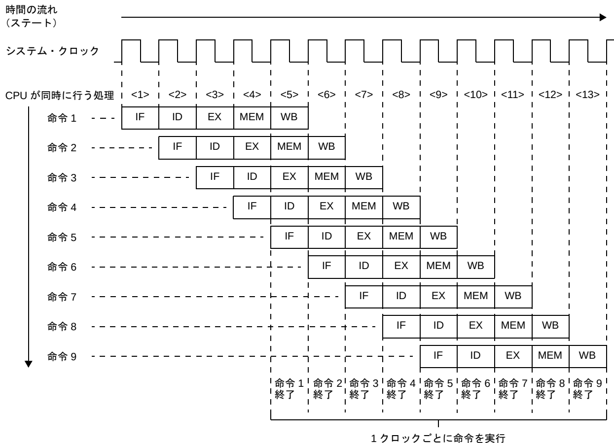
図 4—76 標準的な命令を 9 個続けて実行する例
