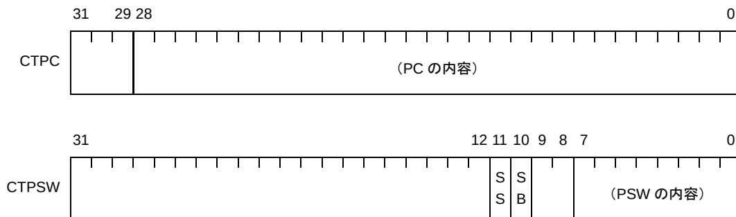
図 4—27 CALLT 実行時状態退避レジスタ【V850E2】
