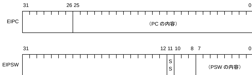
図 4—15 割り込み時状態退避レジスタ【V850E1】
