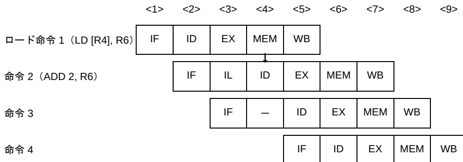
図 4—66 ロード命令実行結果の参照例
