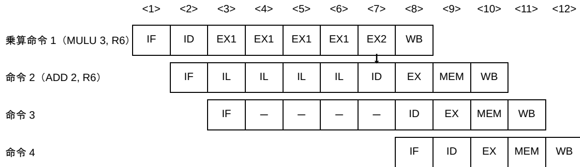
図 4—74 乗算命令実行結果の参照例（ワード乗算命令の場合）
