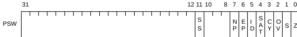
図 4—23 プログラム・ステータス・ワード【V850E1】
