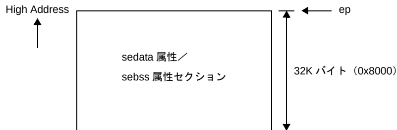
図 3—12 sdata 属性／sibss 属性セクション
