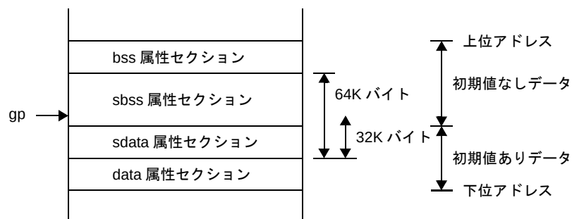
図 4—63 gp オフセット参照セクションのメモリ配置イメージ
