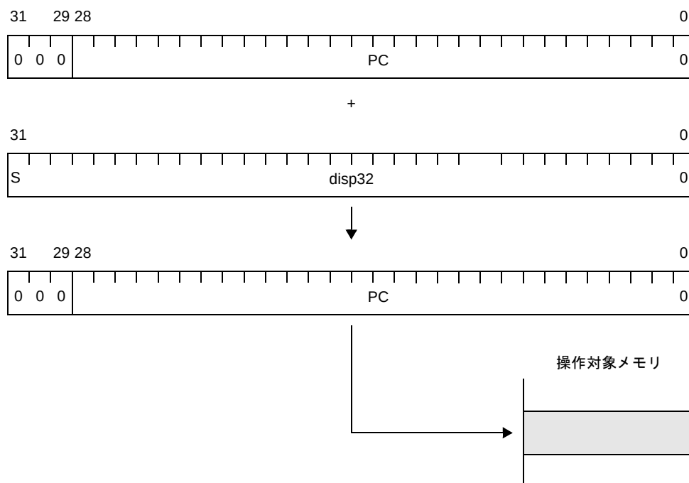
図 4—50 レラティブ・アドレッシング (JR disp32 / JARL disp32, reg2) 【V850E2】
