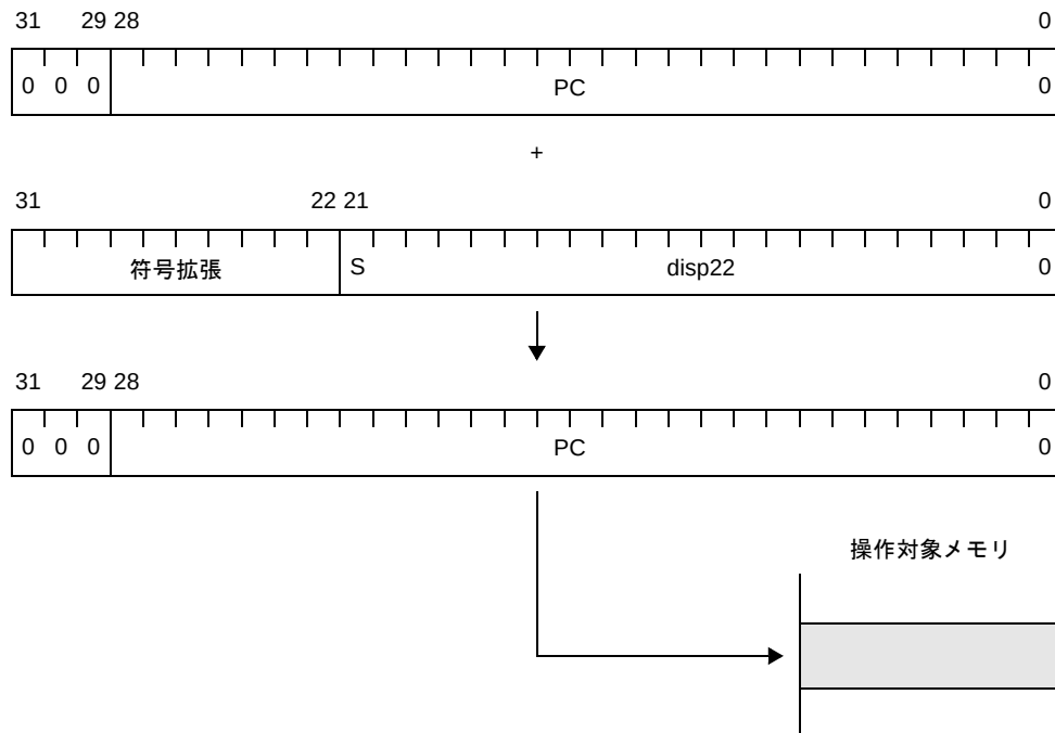
図 4—49 レラティブ・アドレッシング (JR disp22 / JARL disp22, reg2) 【V850E2】
