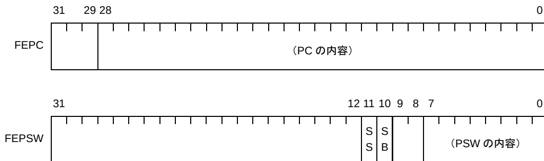
図 4—20 NMI 時状態退避レジスタ【V850E2】
