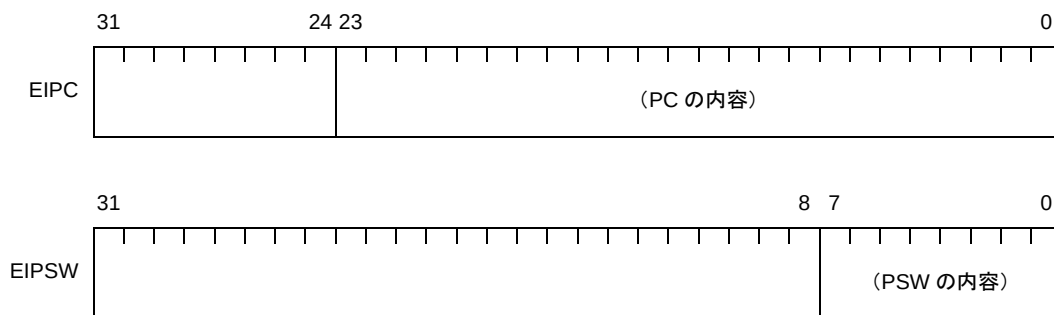
図 4—13 割り込み時状態退避レジスタ【V850】
