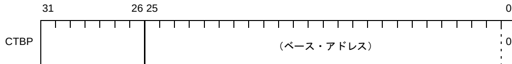
図 4—31 CALLT ベース・ポインタ 【V850ES, V850E1】
