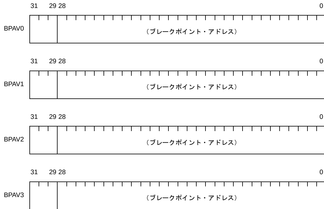
図 4—40 ブレークポイント・アドレス設定レジスタ【V850E2】
