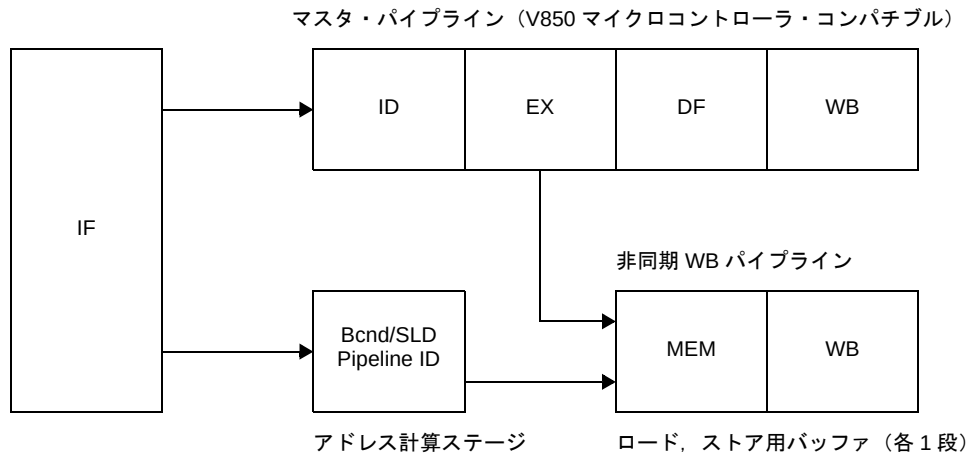
図4—70 パイプライン構成（V850ES）
