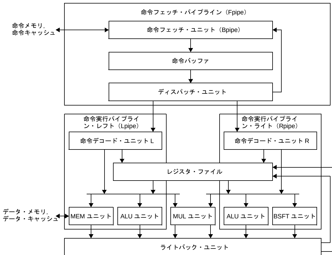
図 4—83 パイプライン構成（V850E2）
