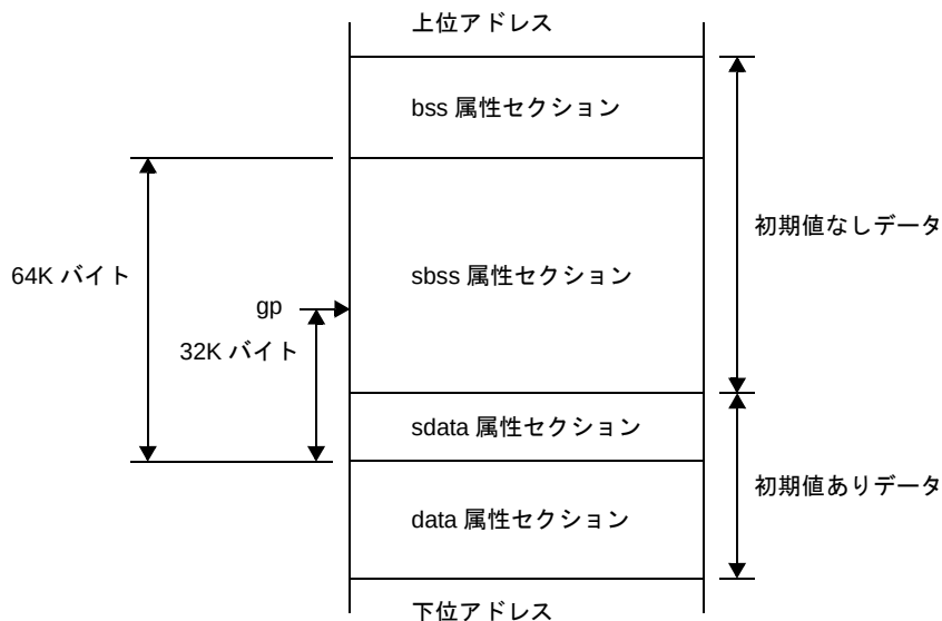
図 4—5 gp オフセット参照セクションのメモリ配置イメージ
