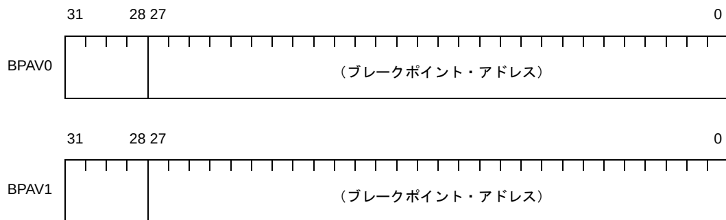
図 4—39 ブレークポイント・アドレス設定レジスタ 【V850E1】
