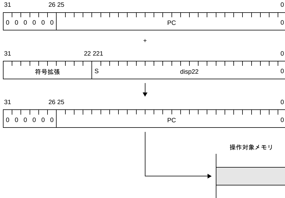
図 4—48 レラティブ・アドレッシング (JR disp22 / JARL disp22, reg2) 【V850ES, V850E1】
