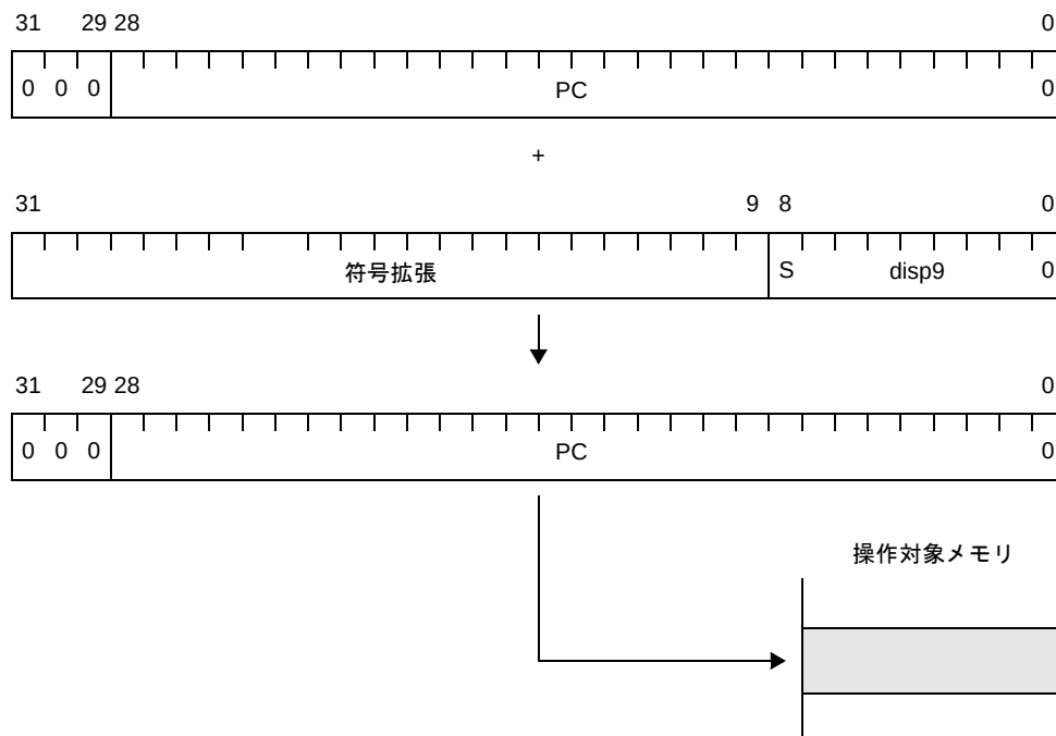
図 4—53 レラティブ・アドレッシング (Bcnd disp9) 【V850E2】
