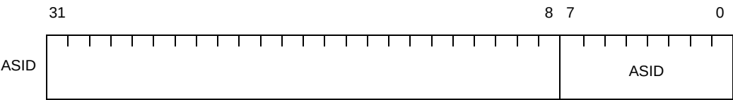
図 4—38 プログラム ID レジスタ 【V850E1, V850E2】
