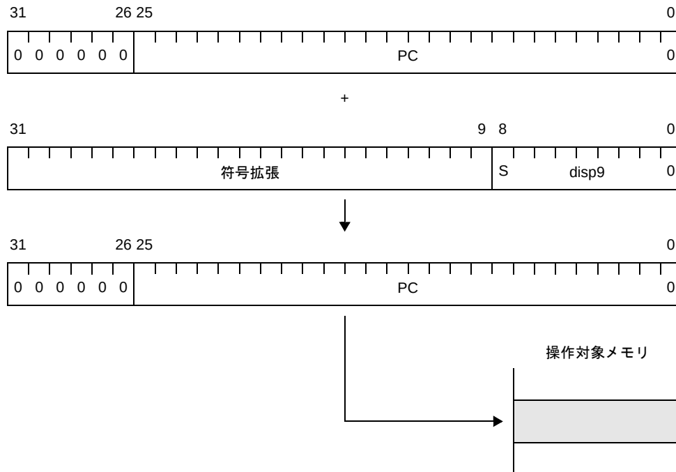
図 4—52 レラティブ・アドレッシング (Bcnd disp9) 【V850ES, V850E1】
