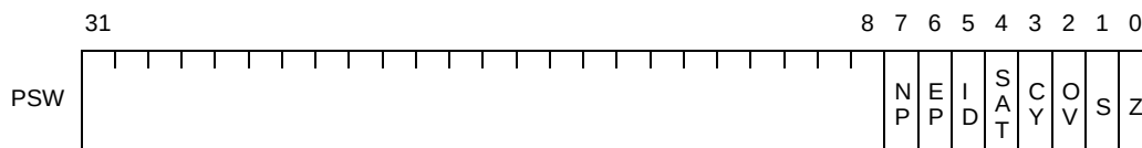
図 4—22 プログラム・ステータス・ワード【V850, V850ES】
