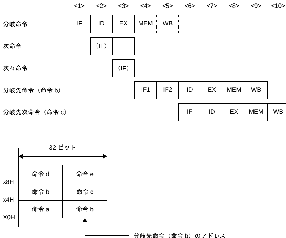
図4—65 アライン・ハザードの例
