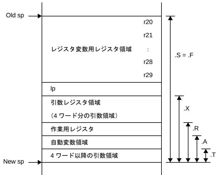
図 3—16 スタック・フレーム（引数レジスタ領域がスタック中央になる場合）
