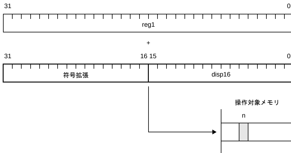
図 4—60 ビット・アドレッシング【V850 マイクロコントローラ, V850ES, V850E1, V850E2】
