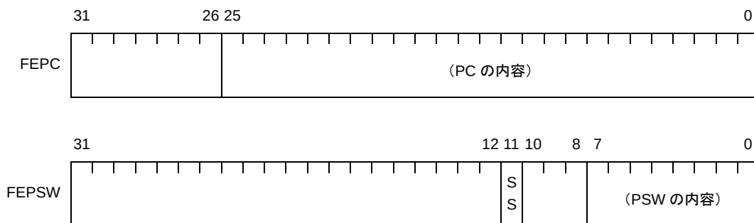
図 4—19 NMI 時状態退避レジスタ【V850E1】
