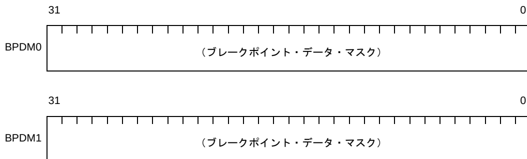
図 4—45 ブレークポイント・データ・マスク・レジスタ【V850E1】
