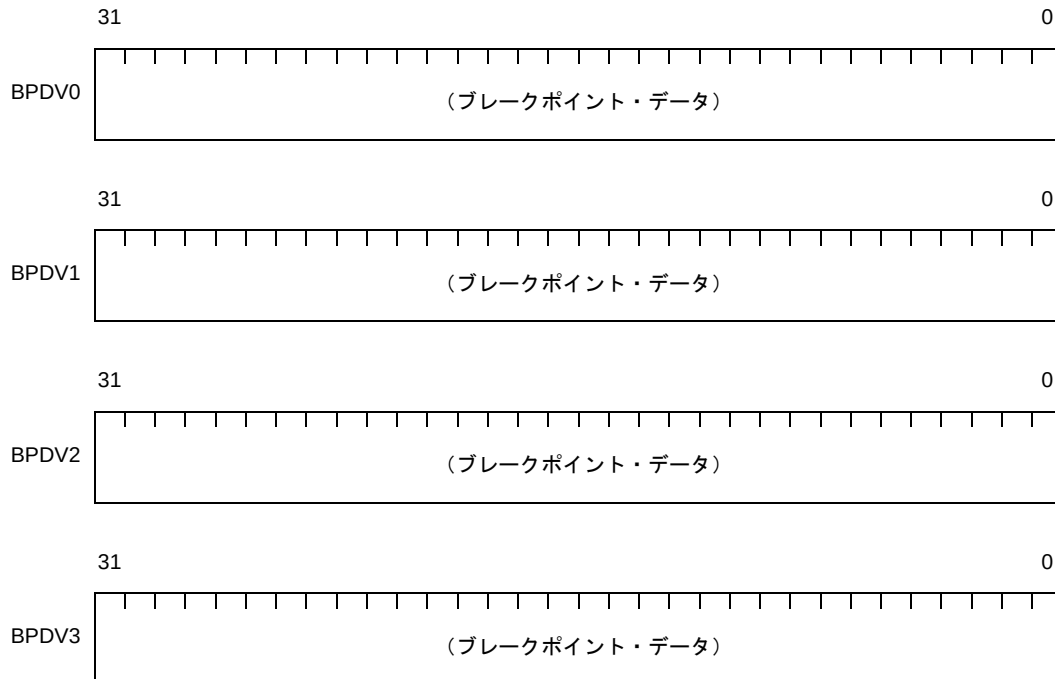
図 4—44 ブレイクポイント・データ設定レジスタ【V850E2】
