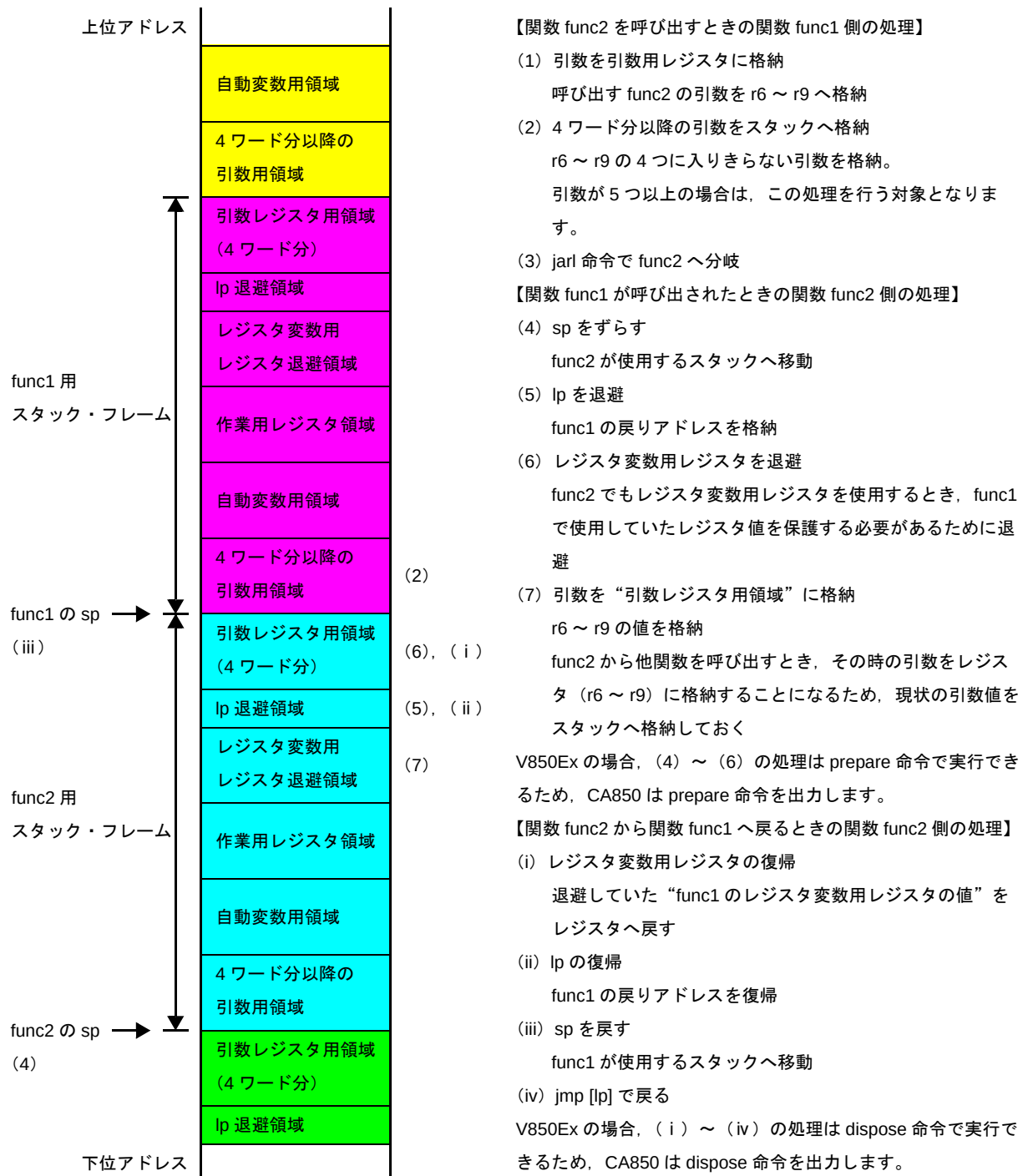
図 3—20 スタック・フレームの生成／消滅（引数レジスタ領域がスタックの先頭にくる場合）
