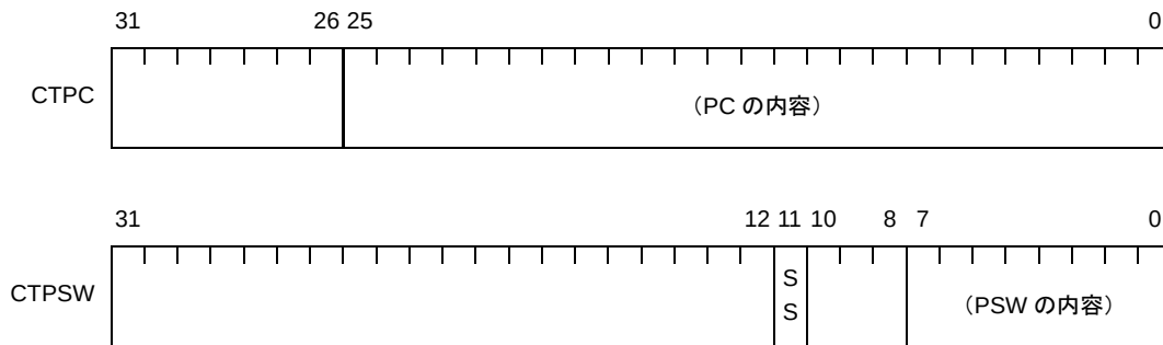
図 4—26 CALLT 実行時状態退避レジスタ【V850E1】
