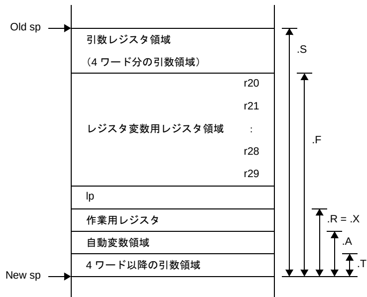
図 3—17 スタック・フレーム（引数レジスタ領域がスタック先頭になる場合）
