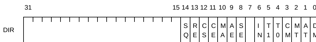
図 4—34 デバッグ・インタフェース・レジスタ【V850E1】
