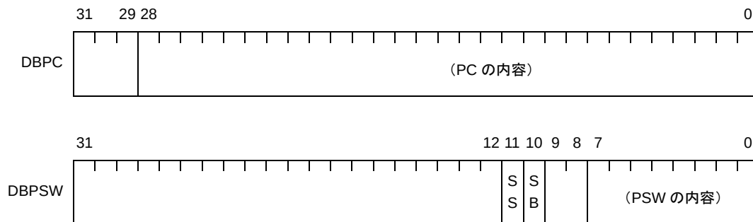
図 4—30 例外／デバッグ・トラップ時状態退避レジスタ【V850E2】
