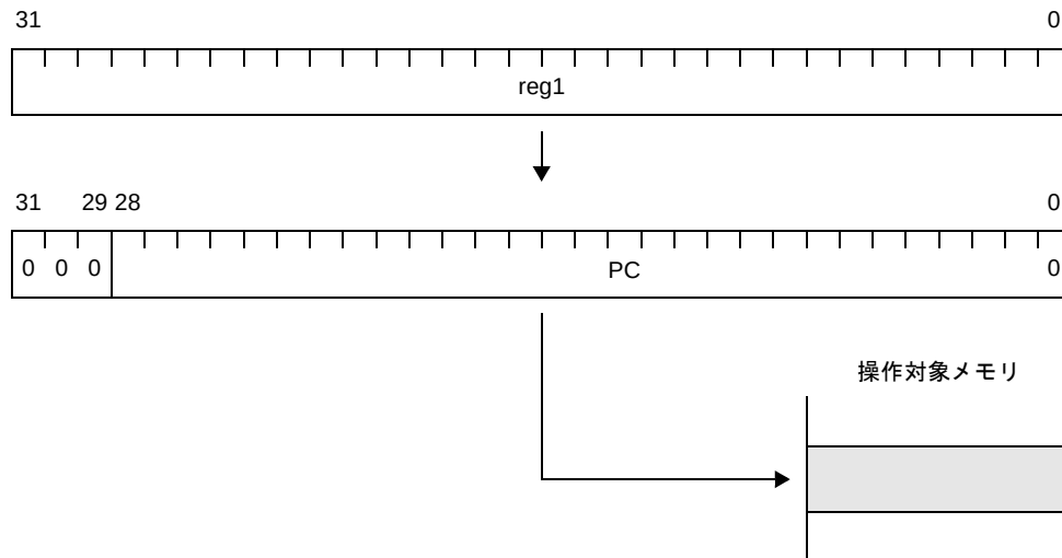
図 4—56 レジスタ・アドレッシング (JMP [reg1]) 【V850E2】
