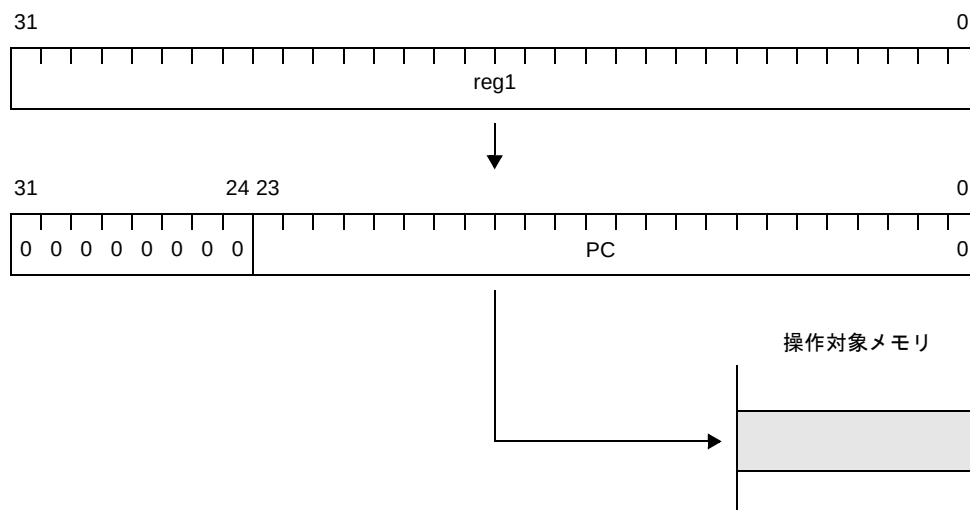
図 4—54 レジスタ・アドレッシング（JMP [reg1]）【V850 マイクロコントローラ】
