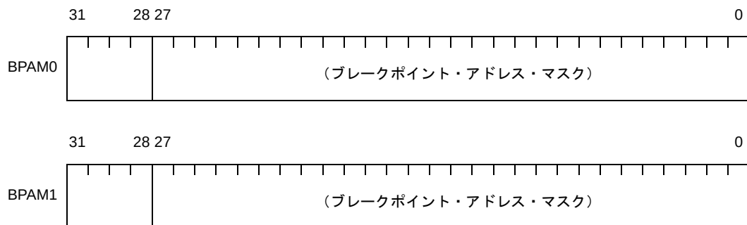
図 4—41 ブレークポイント・アドレス・マスク・レジスタ【V850E1】
