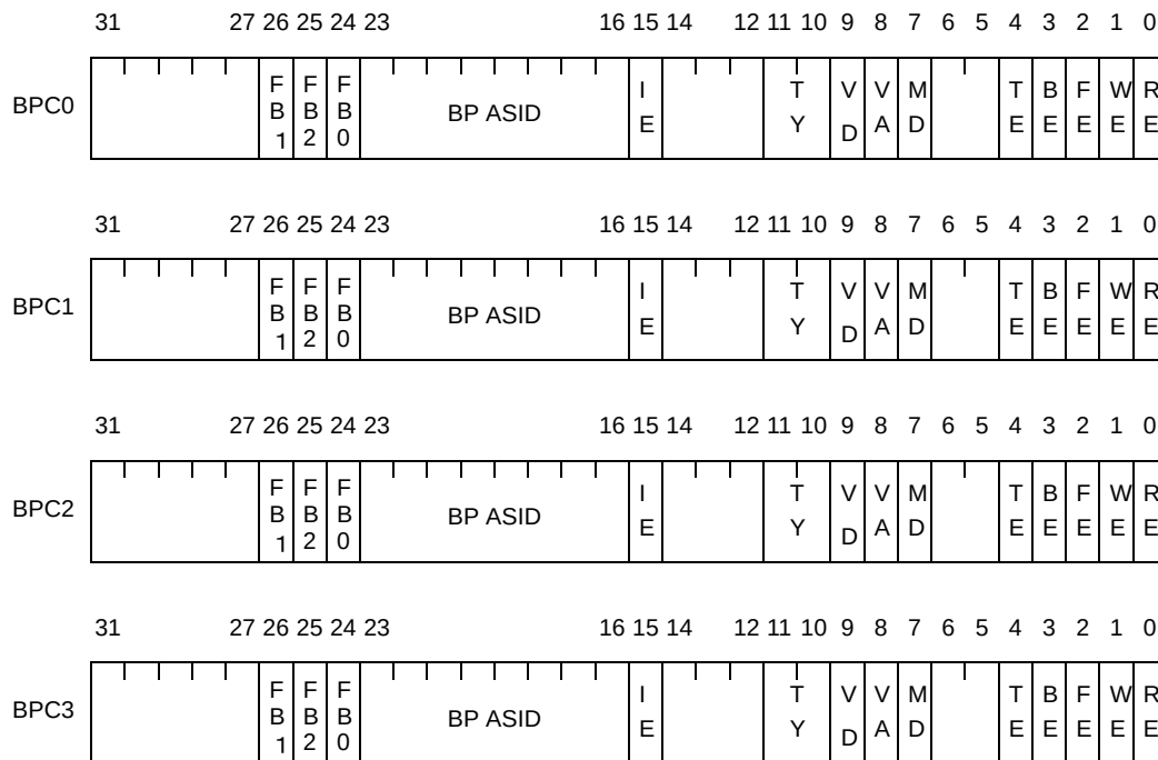
図 4—37 ブレークポイント制御レジスタ【V850E2】
