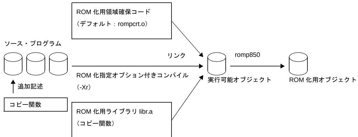
図 8—1 ROM 化用オブジェクトの作成
