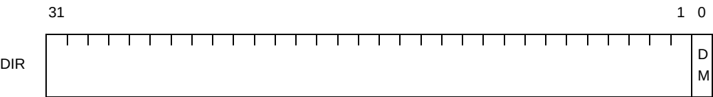
図 4—33 デバッグ・インタフェース・レジスタ 【V850ES】
