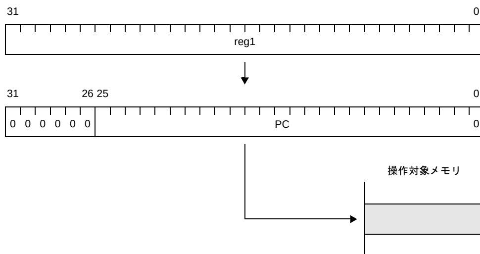
図 4—55 レジスタ・アドレッシング（JMP [reg1]）【V850ES, V850E1】
