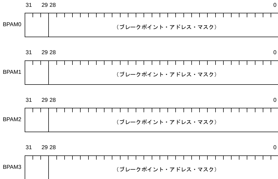
図 4—42 ブレークポイント・アドレス・マスク・レジスタ【V850E2】
