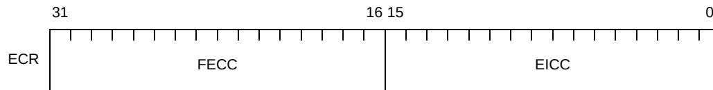
図 4—21 割り込み要因レジスタ 【V850, V850ES, V850E1, V850E2】
