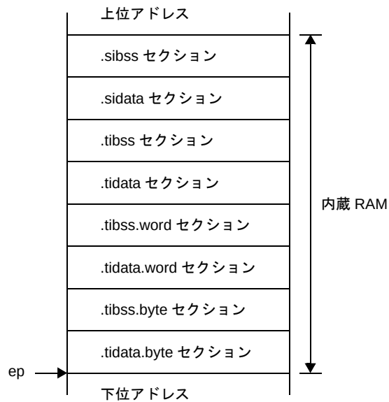
図 4—3 内蔵 RAM のメモリ配置イメージ
