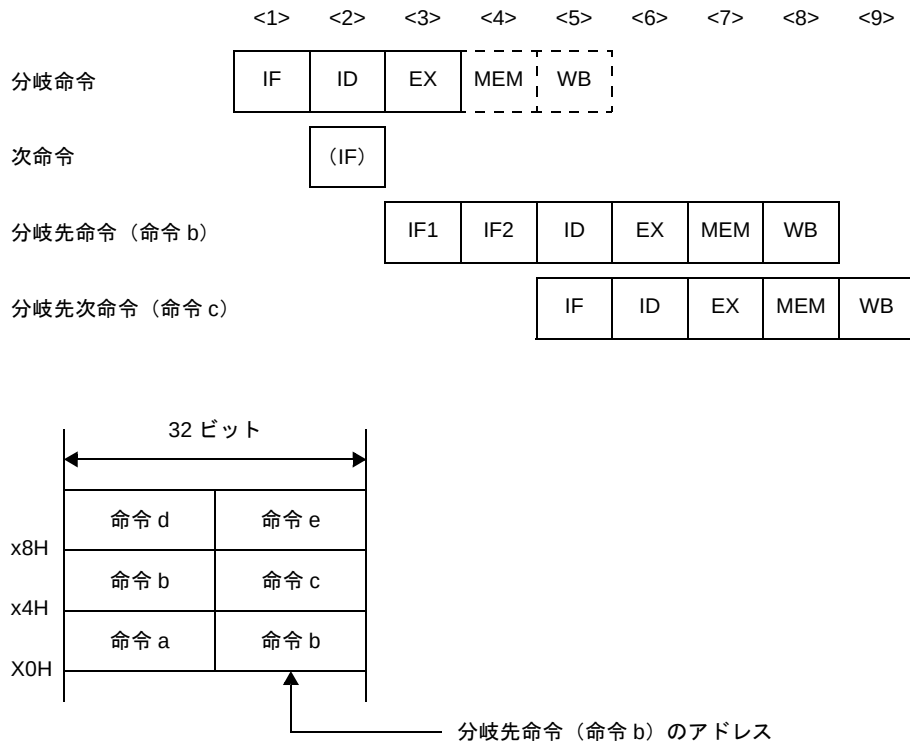
図 4—78 アライン・ハザードの例
