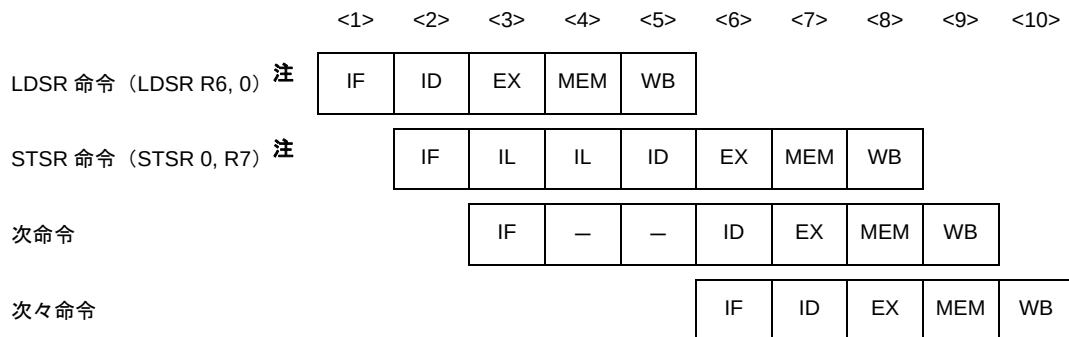
図 4—81 EIPC, FEPC を対象とする LDSR 命令実行結果の参照例
