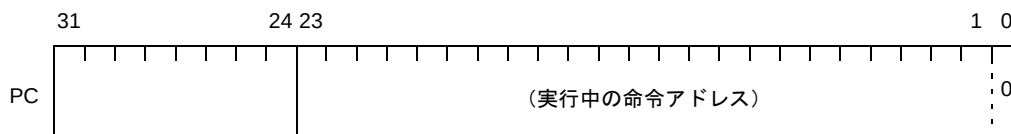
図 4—10 プログラム・カウンタ【V850】
