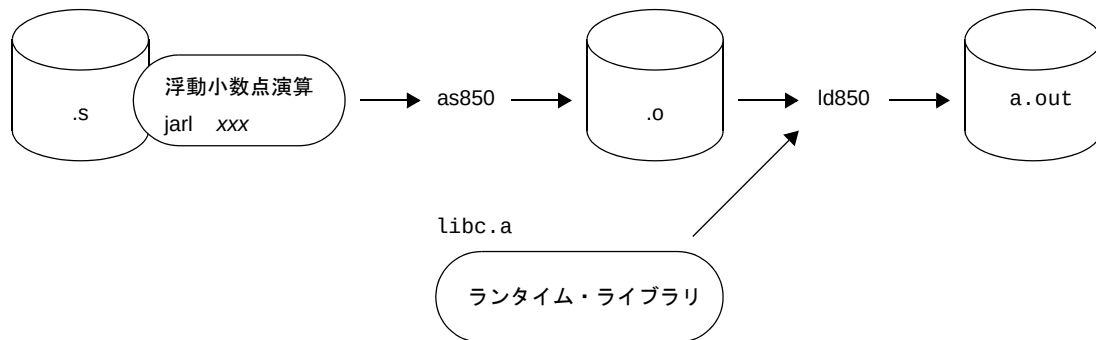
図 6—1 ランタイム・ライブラリ使用イメージ
