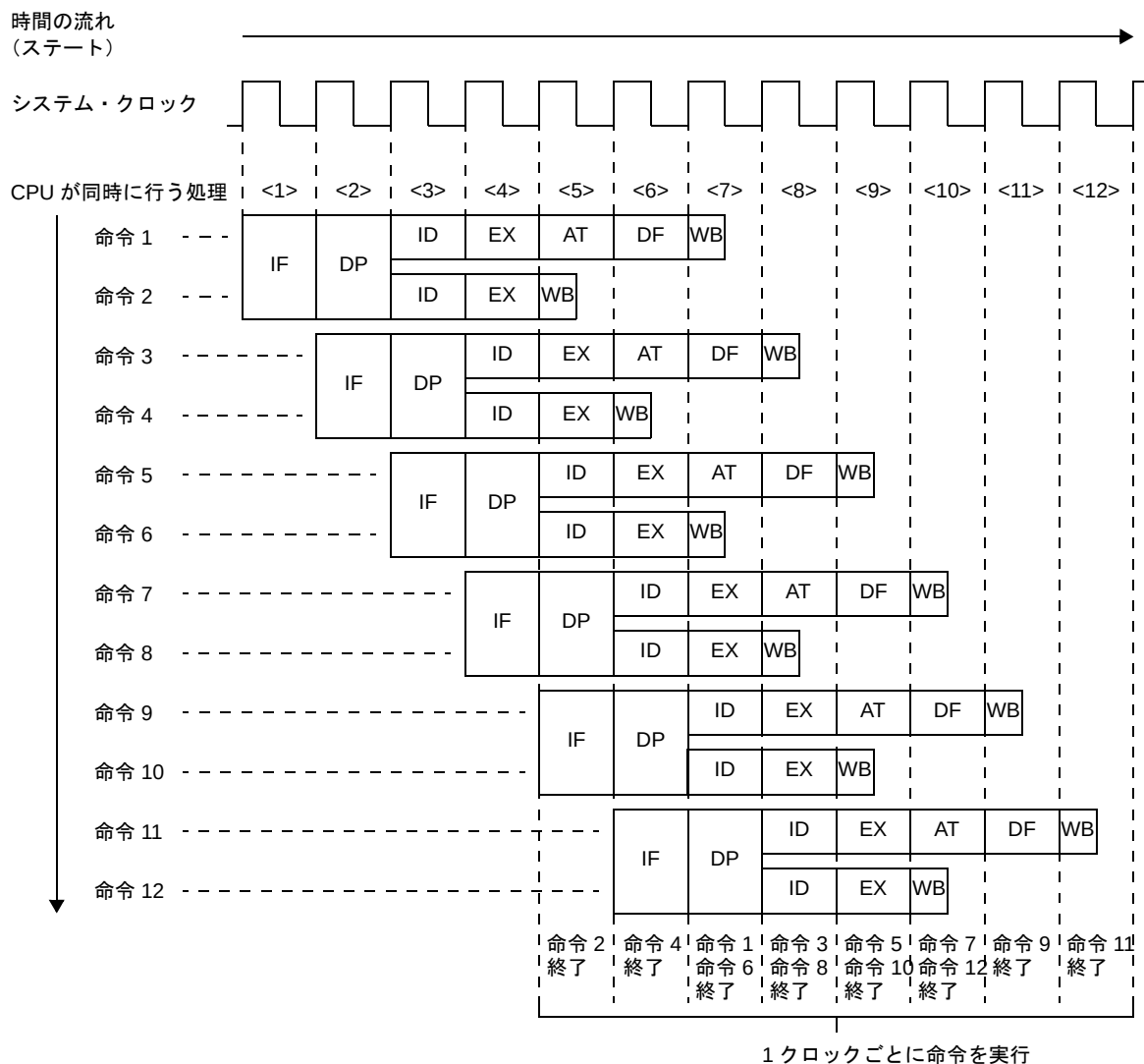
図 4—82 標準的な命令を 12 個続けて実行する例
