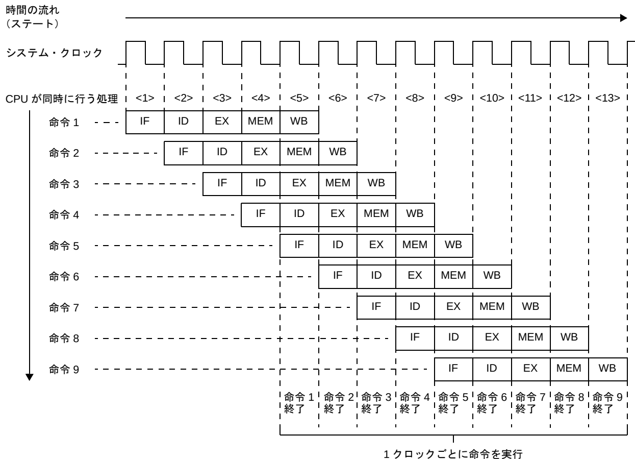
図 4—64 標準的な命令を 9 個続けて実行する例
