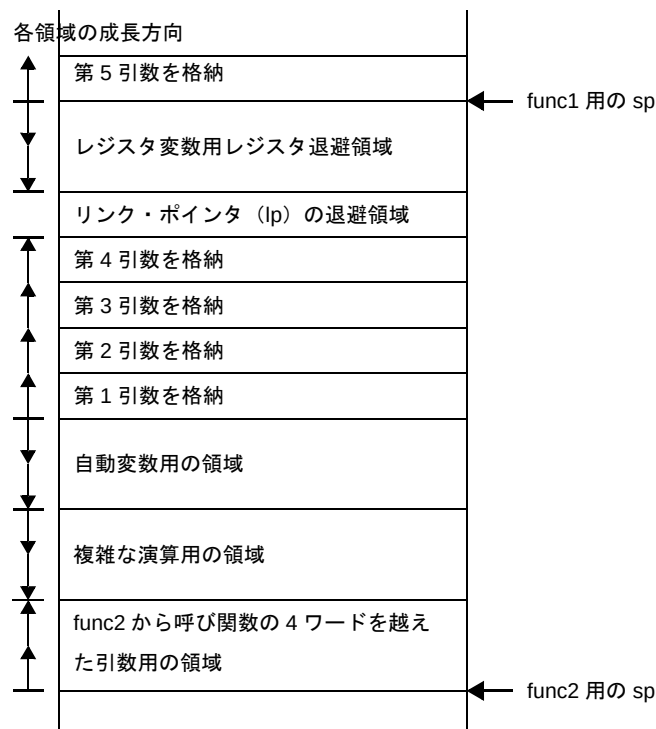
図 3—19 スタック・フレームの各領域のスタック成長方向
