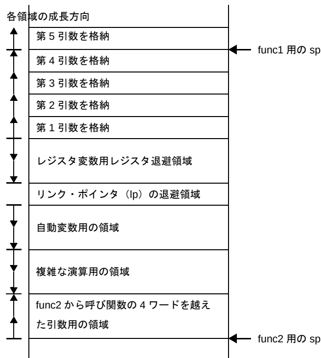
図 3—21 スタック・フレームの各領域のスタック成長方向
