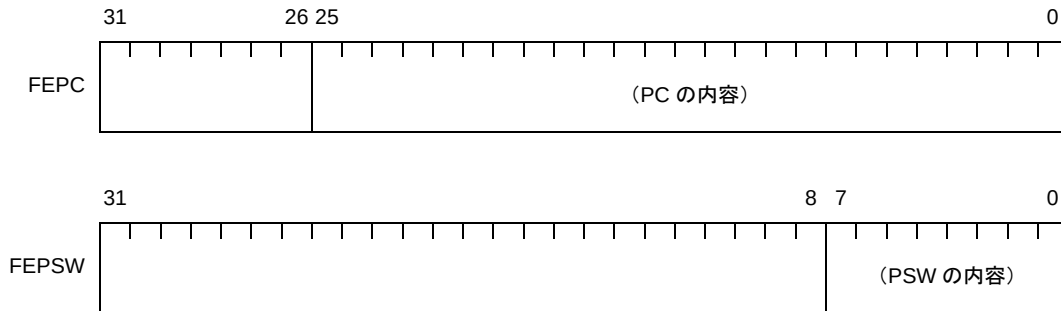
図 4—18 NMI 時状態状態退避レジスタ【V850ES】
