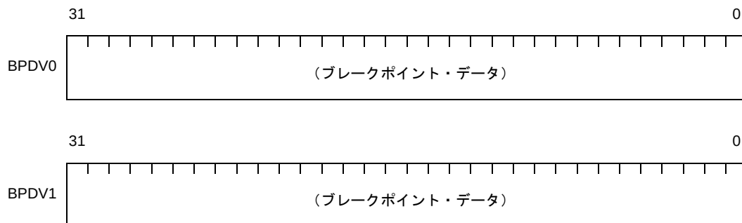
図 4—43 ブレークポイント・データ設定レジスタ 【V850E1】
