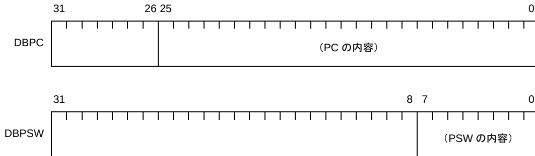
図 4—28 例外／デバッグ・トラップ時状態退避レジスタ【V850ES】
