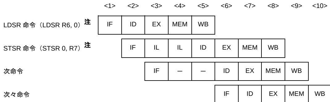
図 4—75 EIPC, FEPC を対象とする LDSR 命令実行結果の参照例
