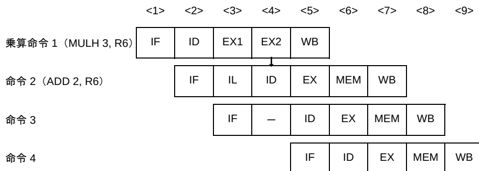
図 4—73 乗算命令実行結果の参照例（ハーフワード乗算命令の場合）
