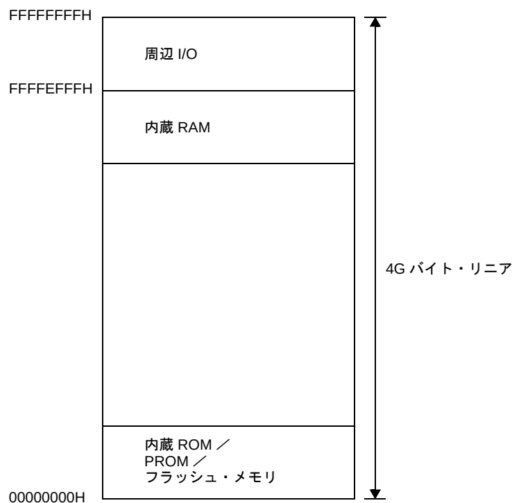
図 4—7 V850 マイクロコントローラのメモリ・マップ
