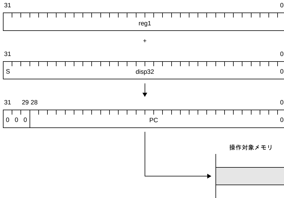
図 4—57 レジスタ・アドレッシング（JMP disp32[reg1]）【V850E2】
