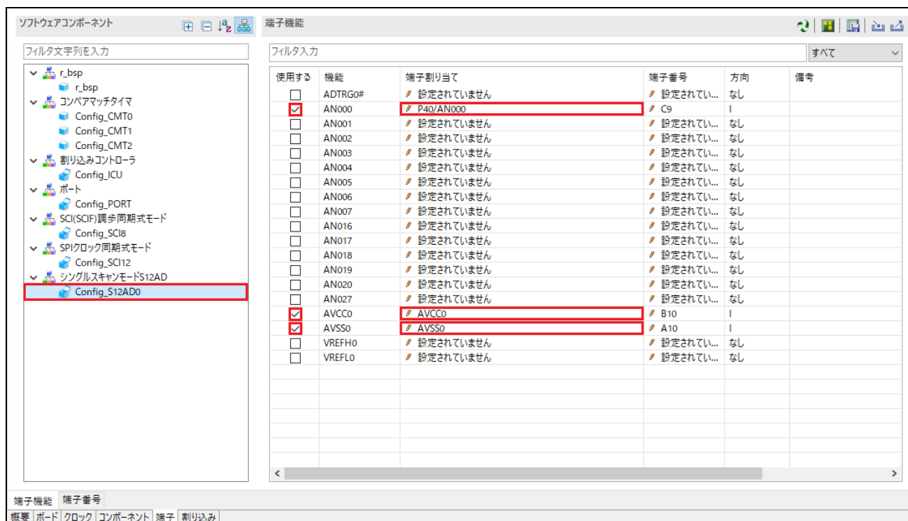
図 4-45 端子設定 - Config_S12AD0
