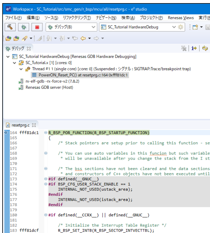
図 6-4 デバッガ・スタートアップ画面
