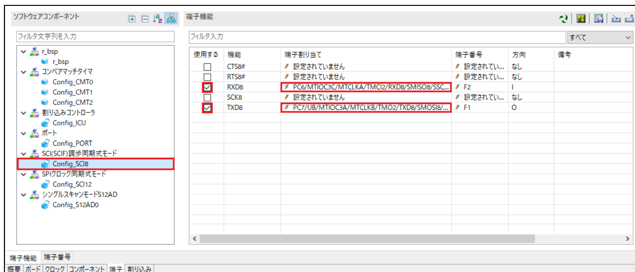
図 4-43 端子設定 - Config_SCI8
