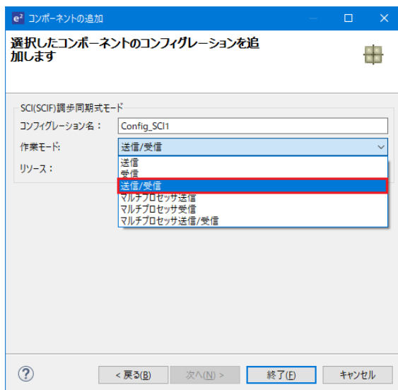
図 4-27 作業モード選択 - 送信/受信
