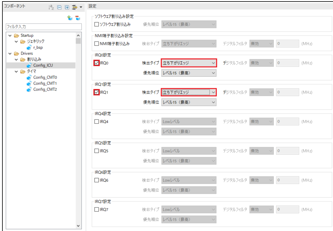
図 4-17 Config_ICU 設定
