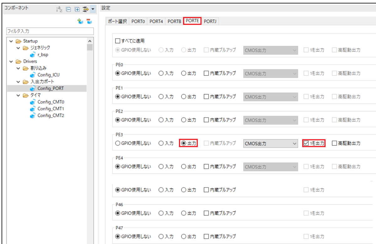
図 4-24 PORTE タブ選択
