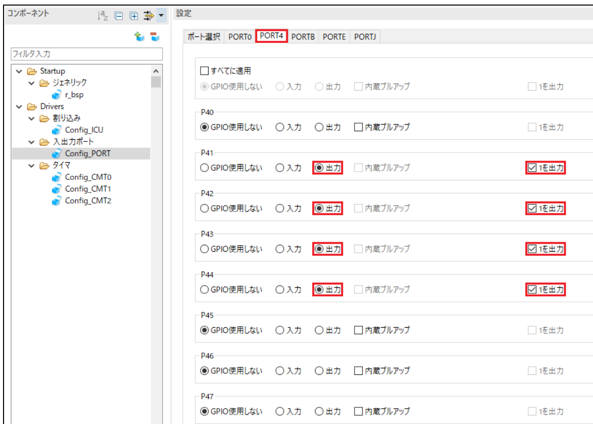
図 4-22 PORT4 タブ選択
