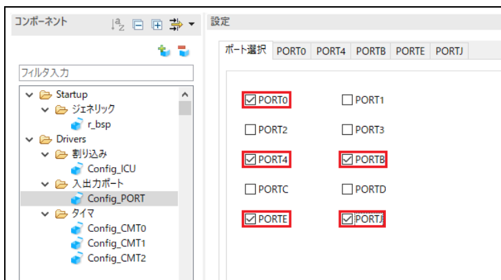
図 4-20 ポート選択
