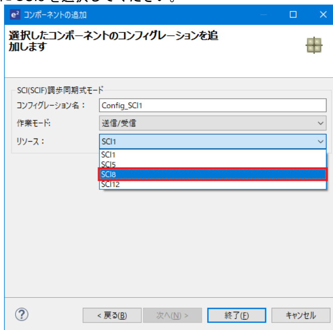
図 4-28 リソース選択 - SCI8
