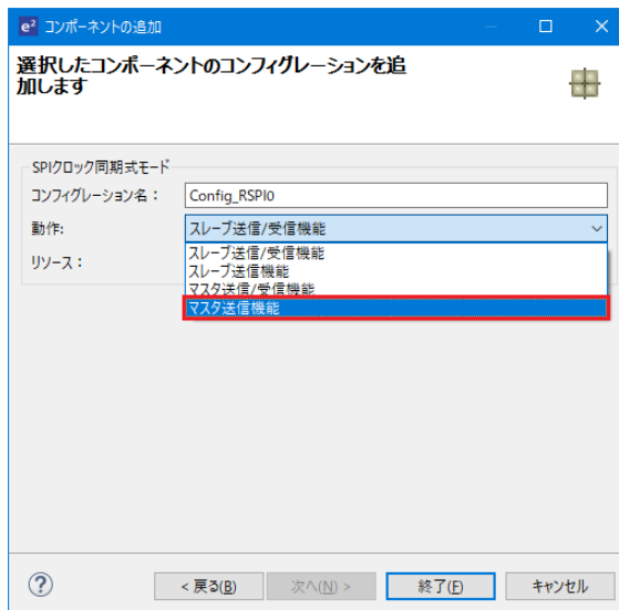
図 4-32 動作選択 – マスタ送信機能
