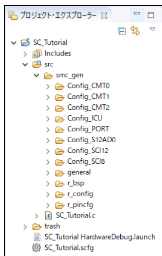
図 4-48 スマート・コンフィグレータフォルダ構成
