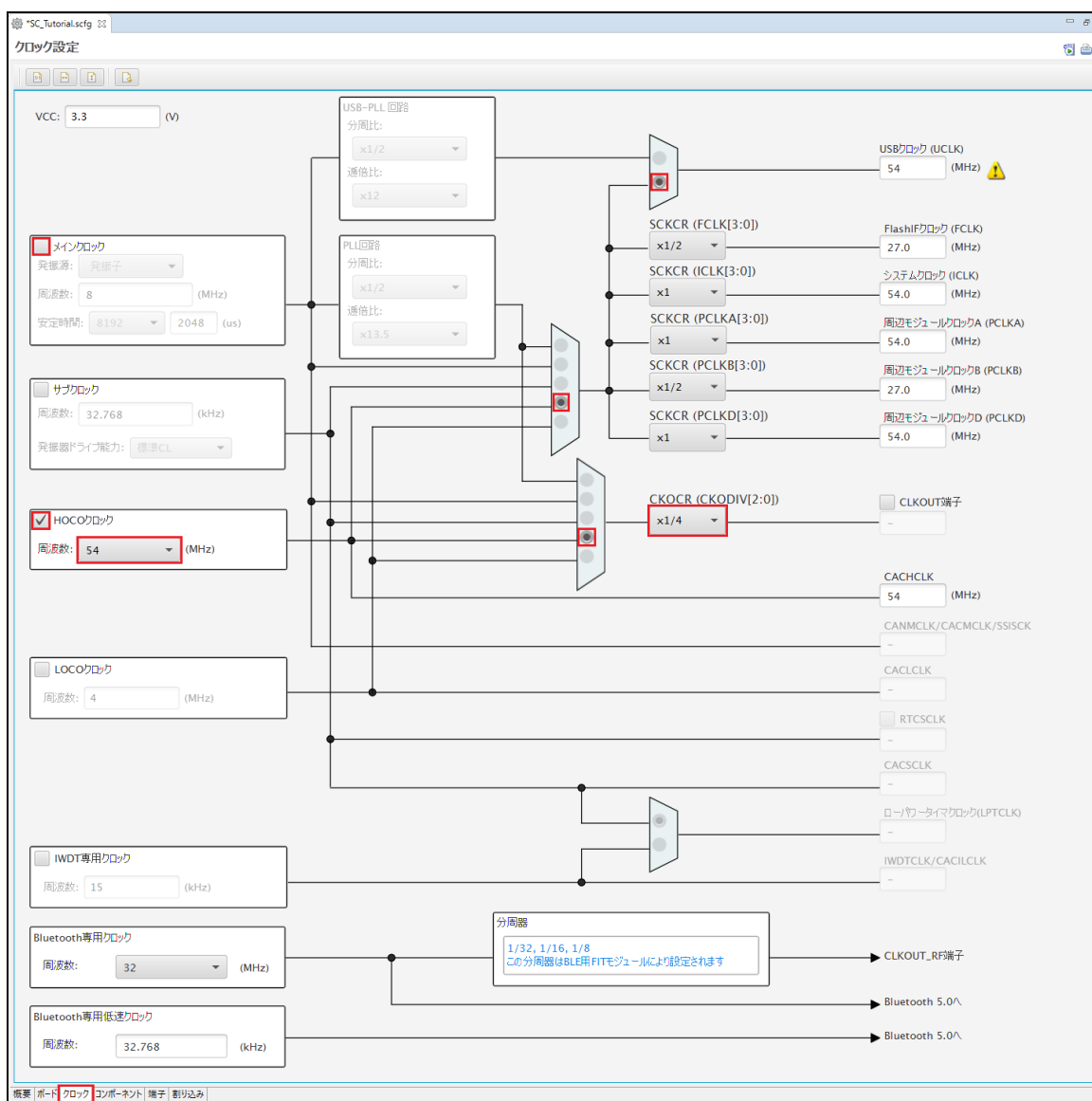
図 4-4 クロックページ
