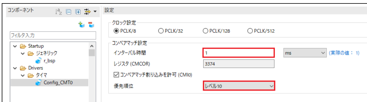
図 4-10 Config_CMT0 設定
