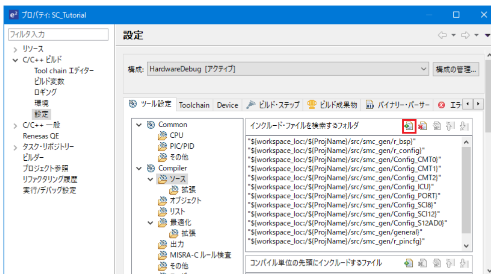
図 5-2 インクルードパス追加
