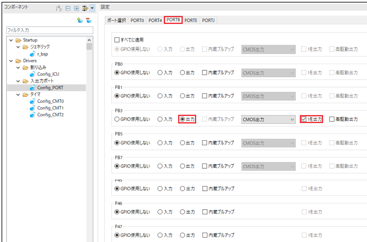
図 4-23 PORTB タブ選択
