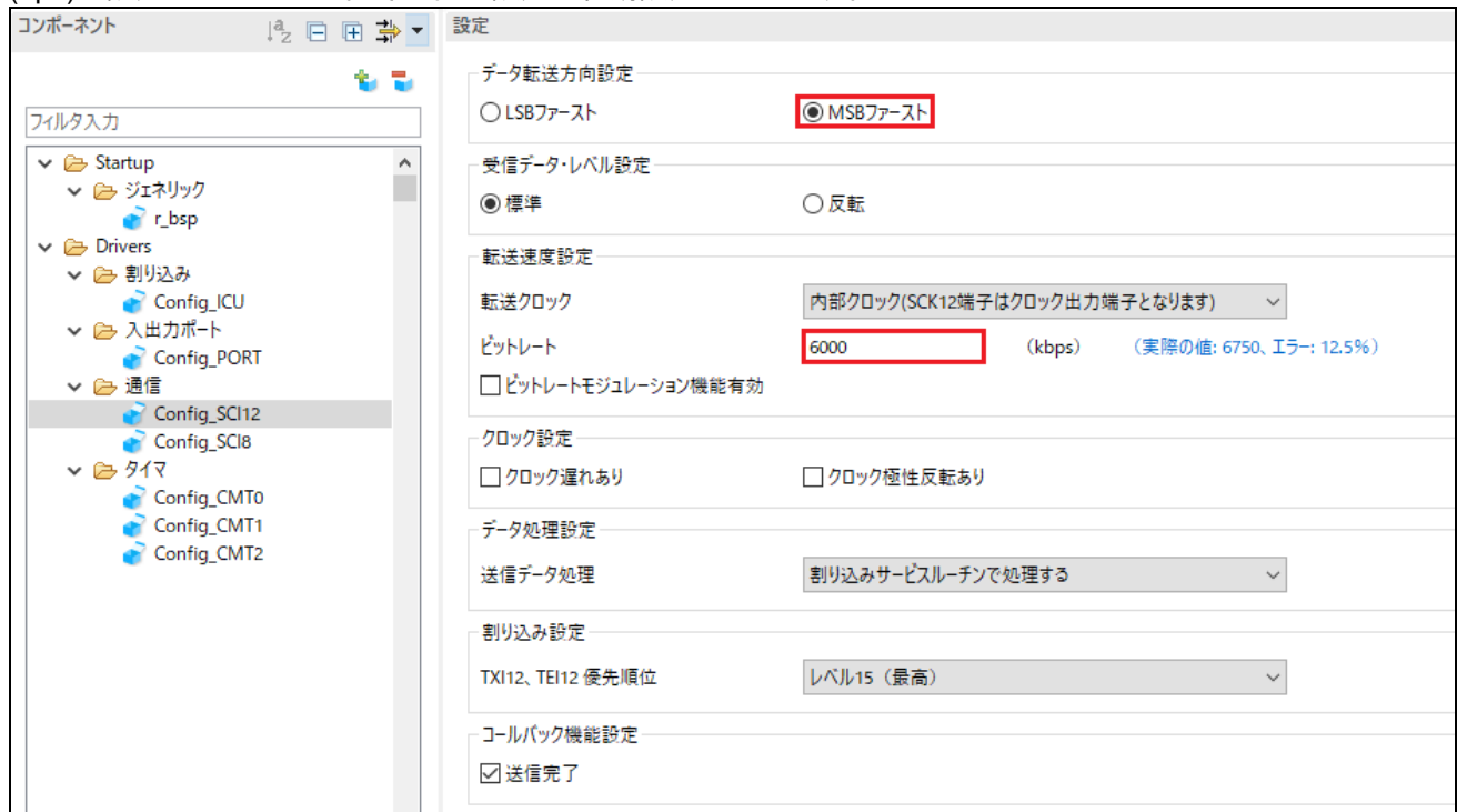
図 4-35 Config_SCI12 設定
