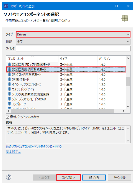
図 4-26 SCI(SCIF)調歩同期式モード選択
