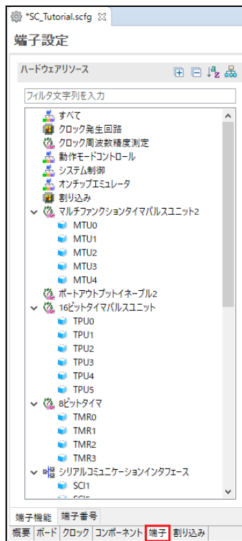
図 4-40 端子ページ
