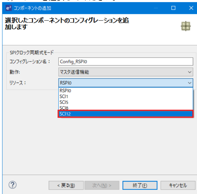
図 4-33 リソース選択 - SCI8
