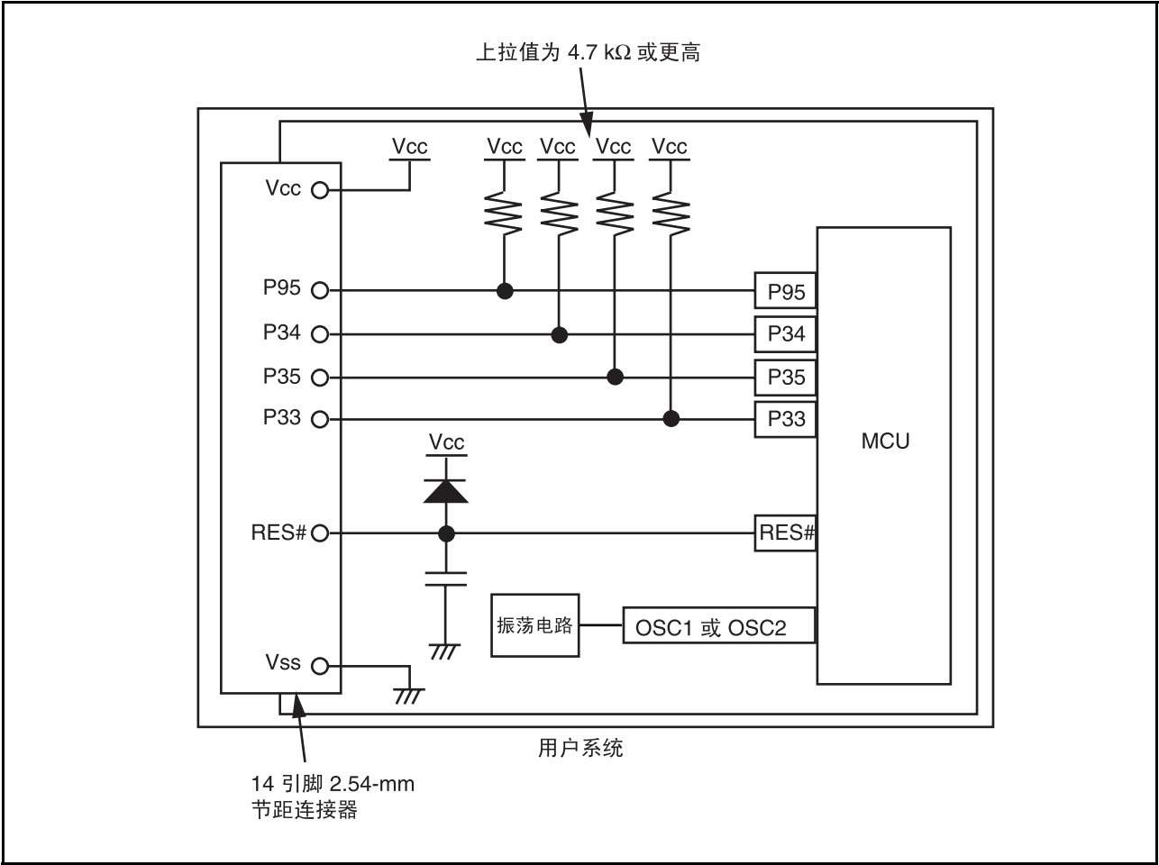
图 4.1 仿真器连接示例（使用 POR 时）
