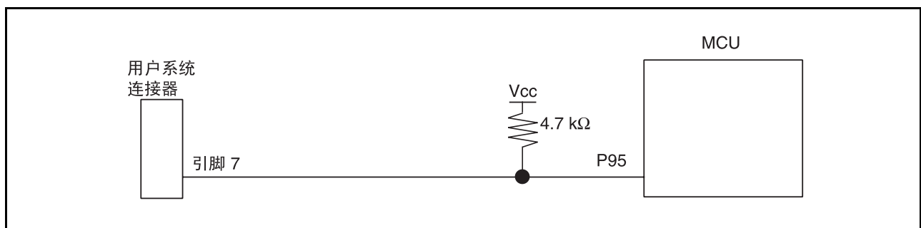
图 4.4 仿真器和 P95 引脚的连接
