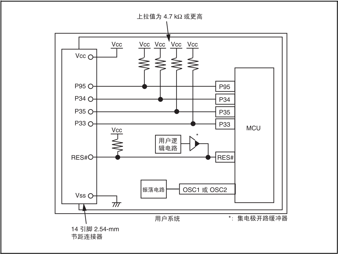
图 4.2 仿真器连接示例（未使用 POR 时）
