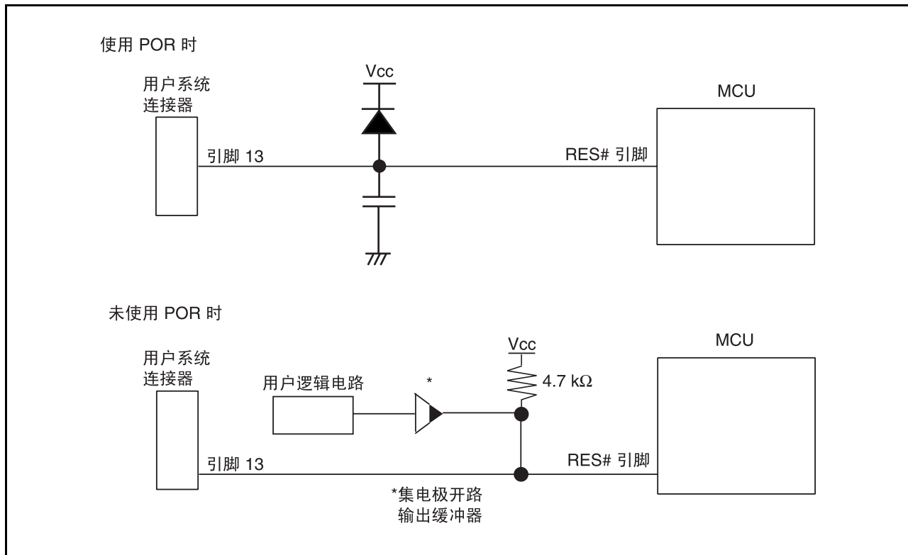
图 4.5 复位电路示例
