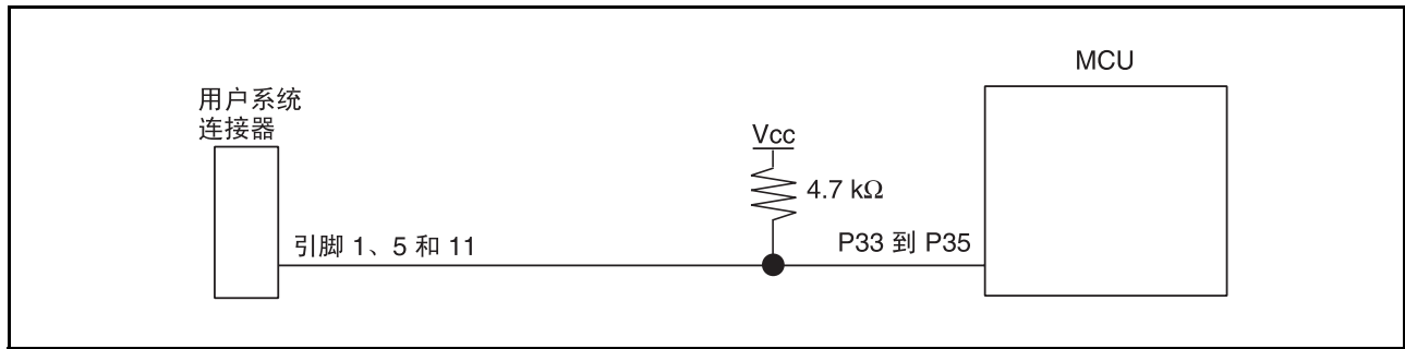
图 4.3 仿真器和 P33 到 P35 引脚的连接
