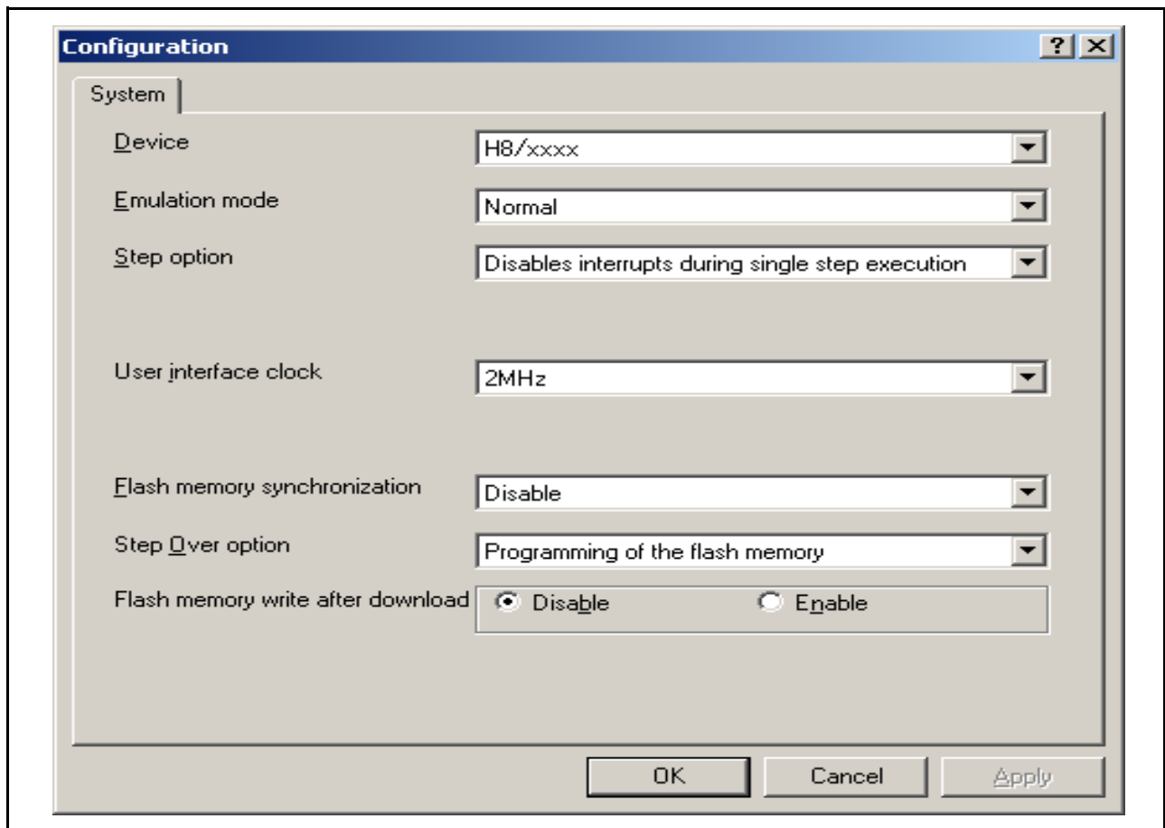
图 5.4 [Configuration]（配置）对话框（[System]（系统）页）
