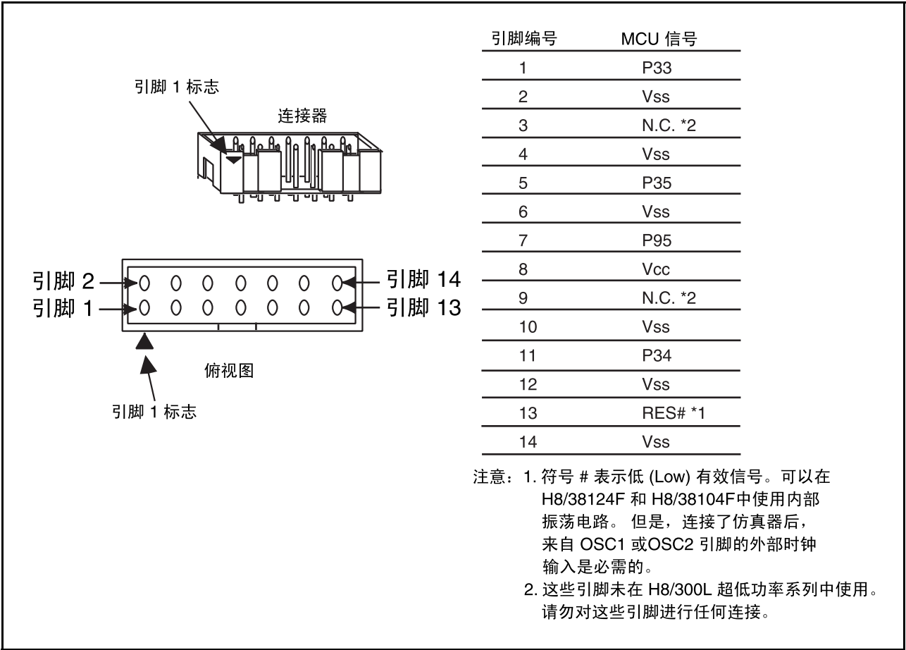
图 3.1 连接器的引脚分配
