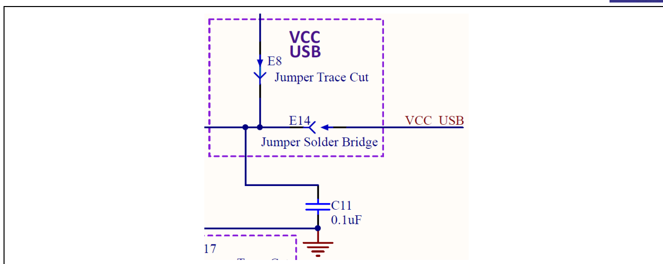
図 32 VCC_USB 回路
