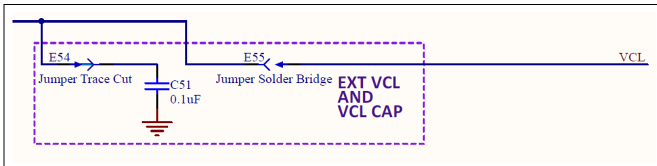
図 31 外部コンデンサと VCL 回路の接続
