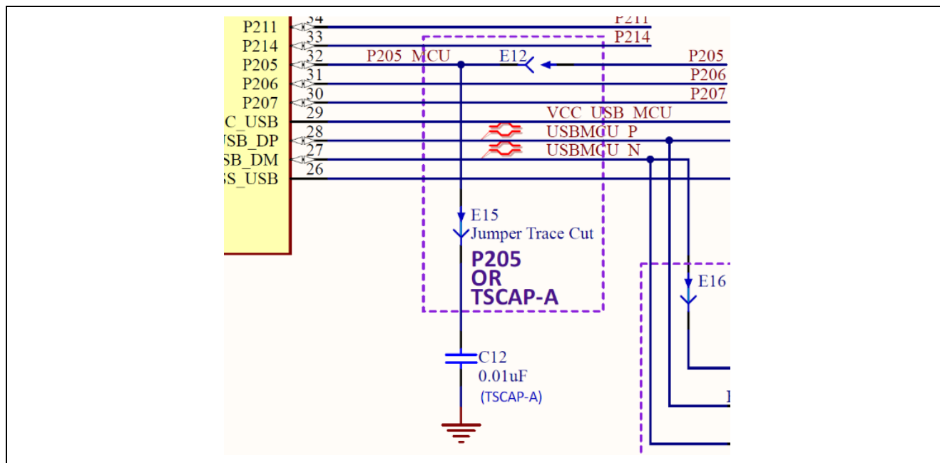
図 33 P205 Circuit
