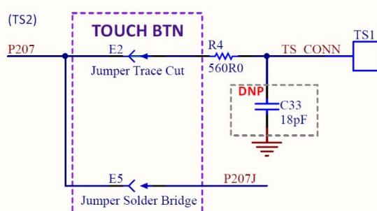
図 21 静電容量式タッチボタン回路
