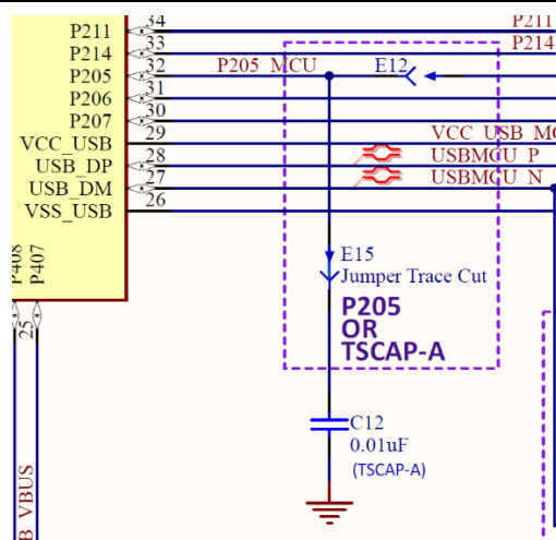
図 22 静電容量式タッチ TSCAP 回路
