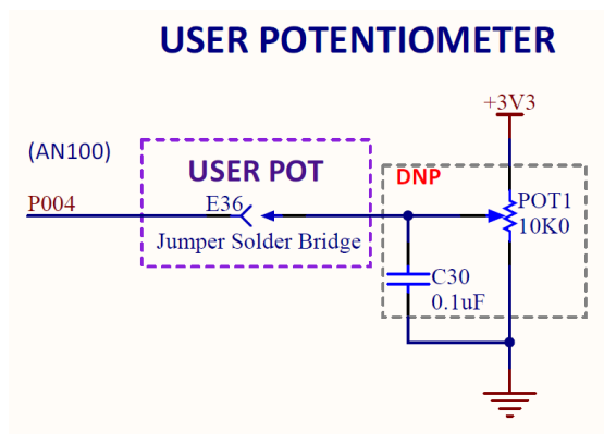
図 27 ユーザポテンショメータ回路
