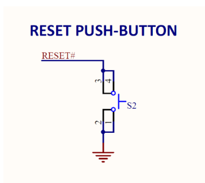
図 19 リセットスイッチ回路
