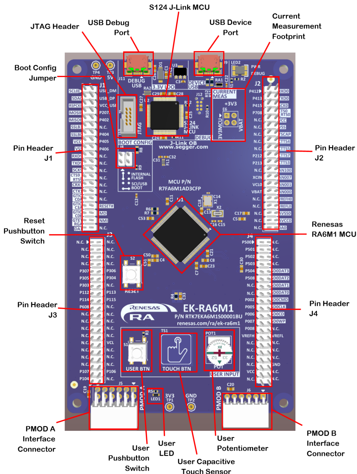
図1 メインボード（上面）
