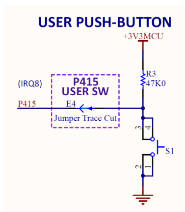
図 17 ユーザスイッチ回路
