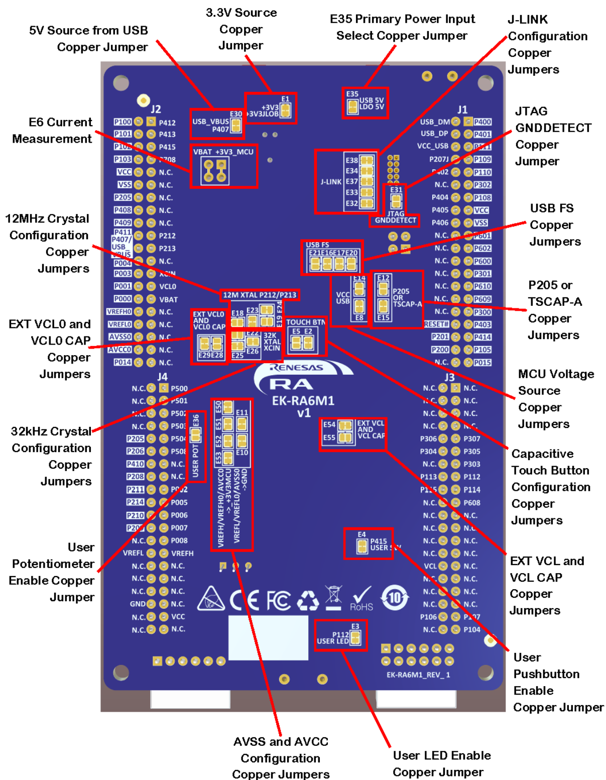
図2 メインボード（裏面）
