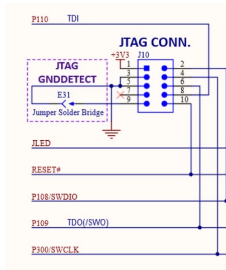
図 15 JTAG 回路
