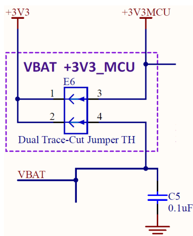
図 12 MCU 電流計測回路
