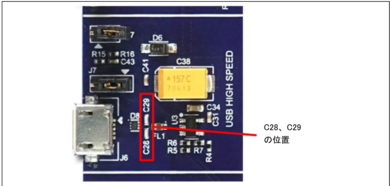
図 1 C28、C29 の位置
