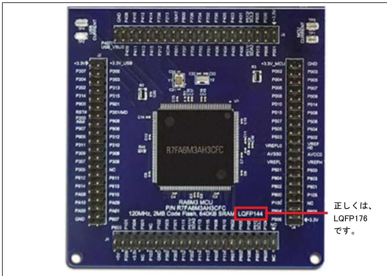
図2 シルクスクリーン印刷によるパッケージタイプ表示
