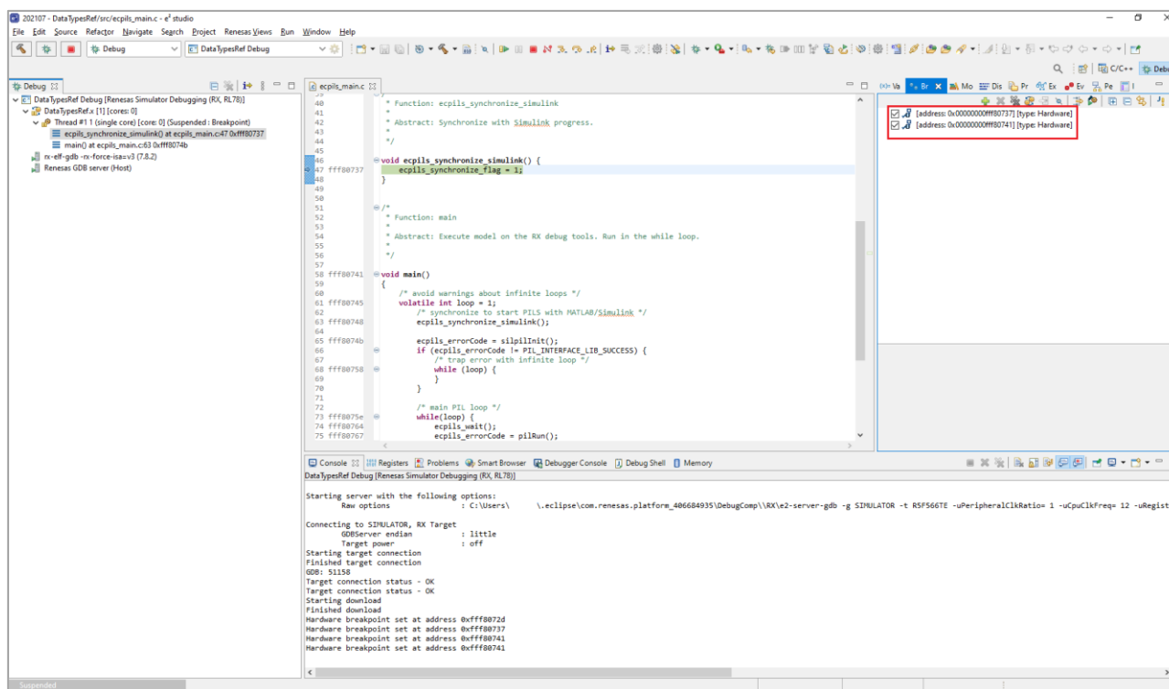
図 3-29 ecpils_main.cに自動的に設定される2つのブレーク・ポイント(e² studio)
