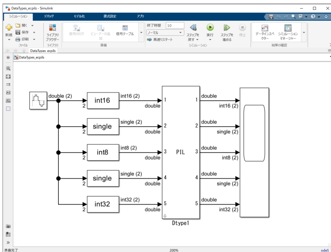
図 3-14 PILシミュレーションの実行
