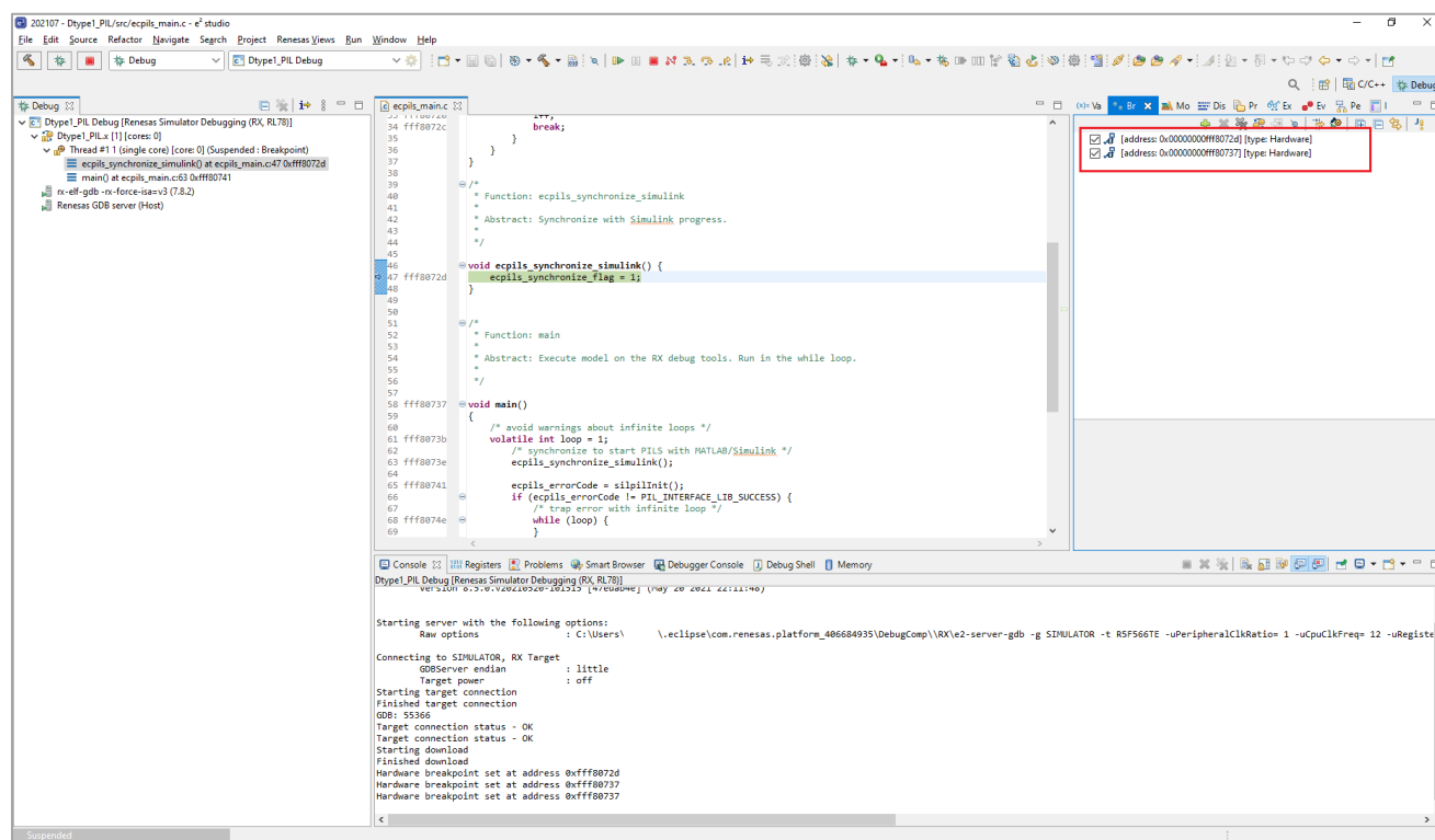
図 3-18 ecplis_main.cに自動的に設定される2つのブレーク・ポイント(e2 studio)
