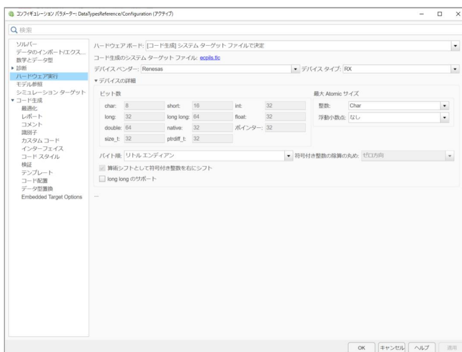
図 3-19 [ハードウェア実行]オプション
