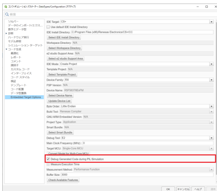
図 3-16 PILシミュレーション中の生成コードデバッグの有効化
