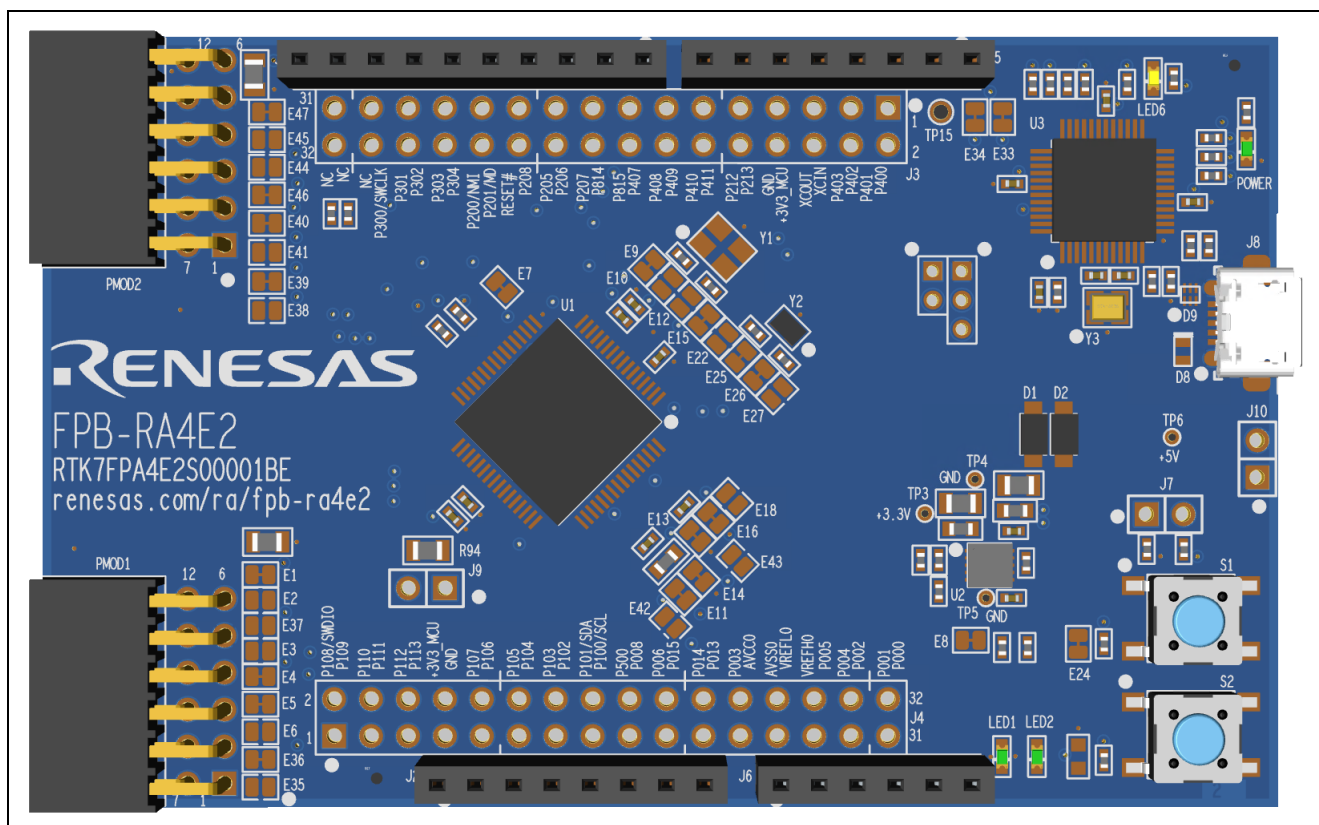
図3 FPB-RA4E2 ボード
