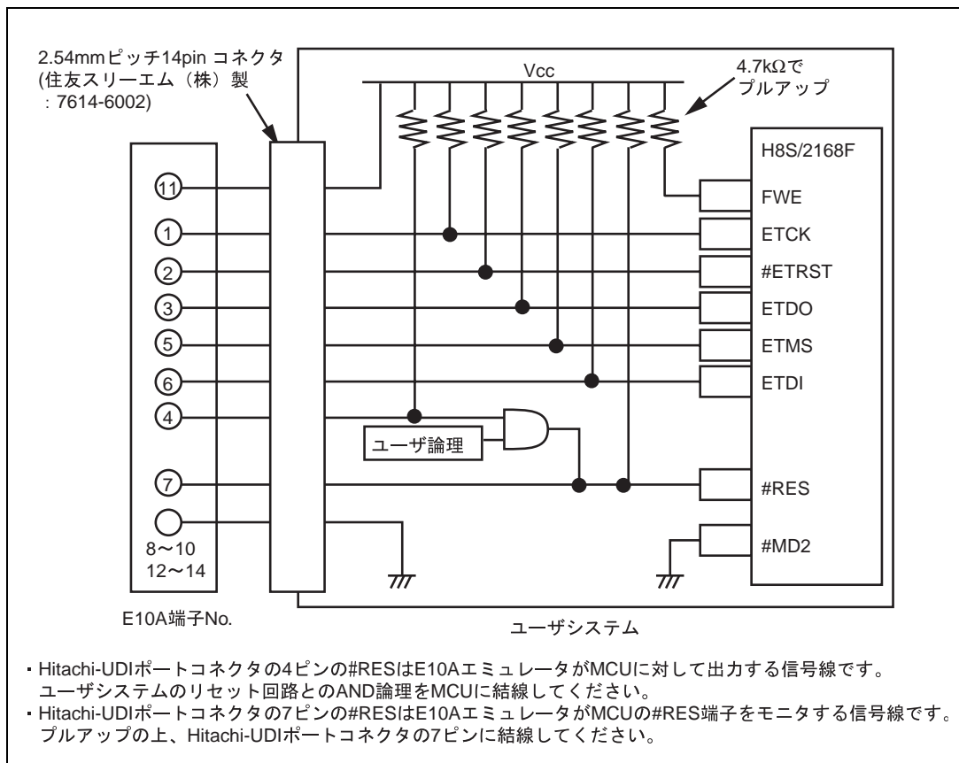
図 6.2 E10A との接続例
