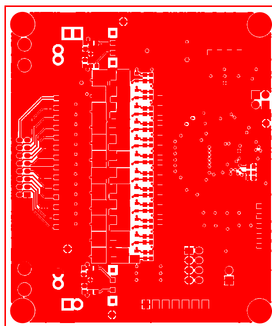
Figure 21. Bottom Layer
