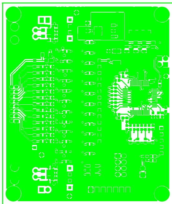
Figure 18. Top Layer
