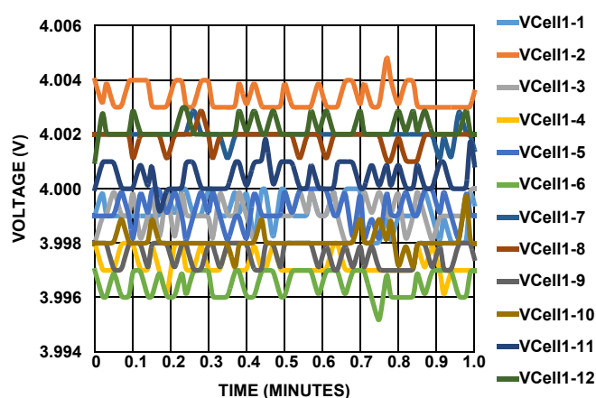
Figure 31. SN1 V_{CELLS} V_{BAT} 24V
