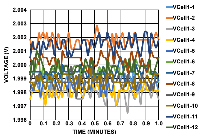
Figure 30. SN1 V_{CELLS} V_{BAT} 24V
