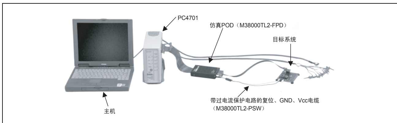
图 2.1 系统全体图
