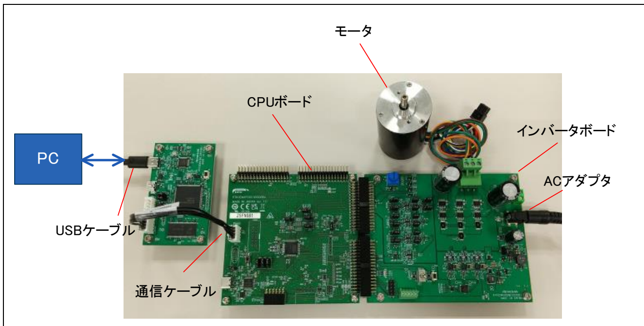
図 4-5 ボード接続例
