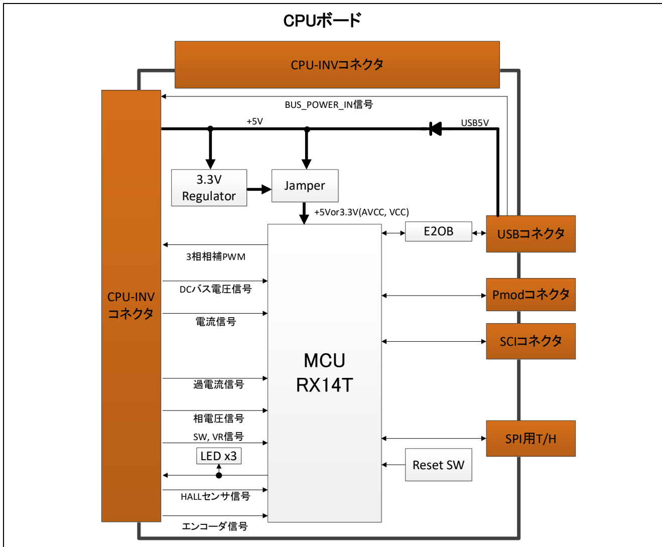
図 4-1 CPU ボードのブロック図
