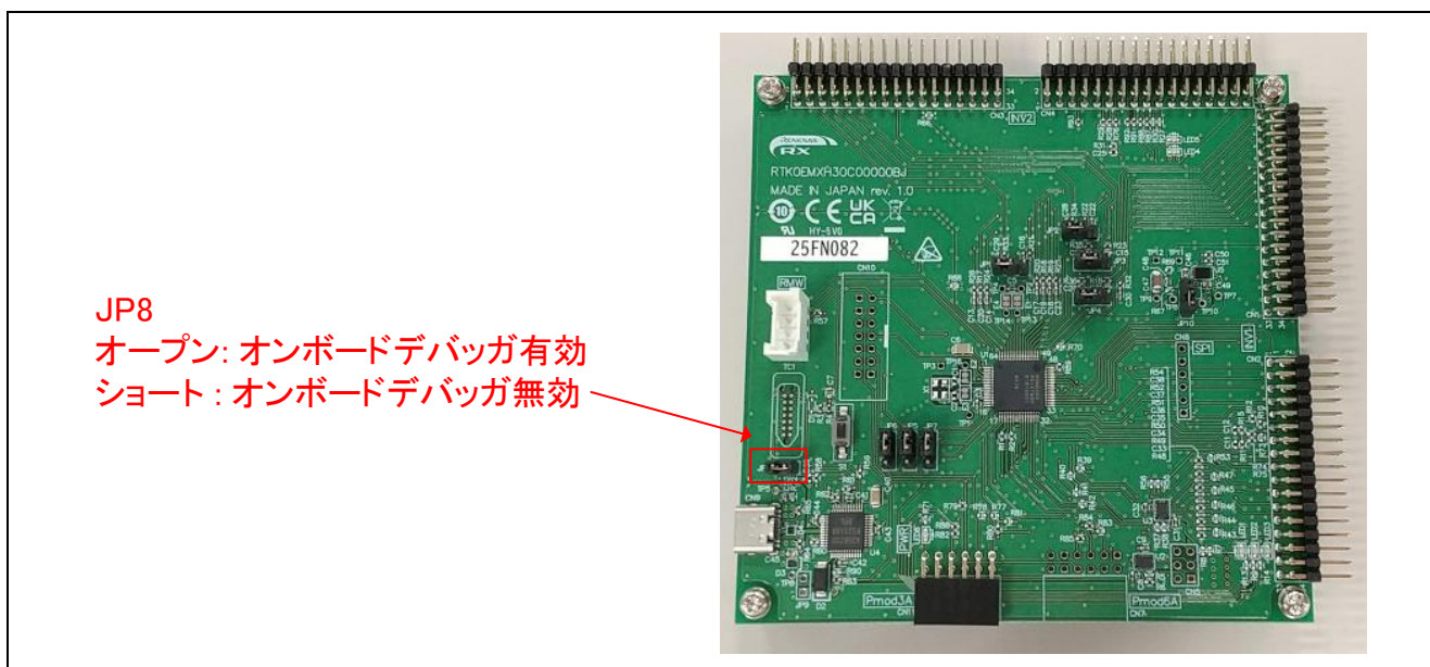
図 5-1 ジャンパーピン JP8 の設定
