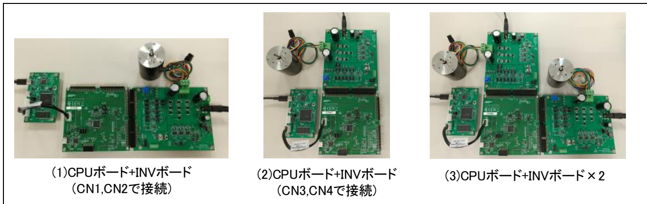
図 5-2 CPU ボードとインバータボードおよび通信ボードの接続図
